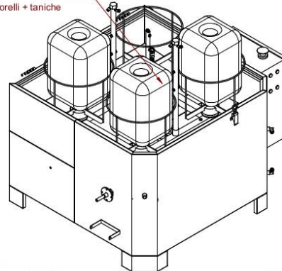
Cod. A9005302 Assieme telaio + platorelli + taniche
