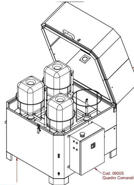
Cod. A4001008 Ass. base + Kit disoleatore
