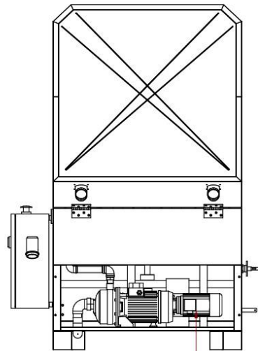
Cod. A2000039 Assieme motoriz. cesto Washer con puleggia
