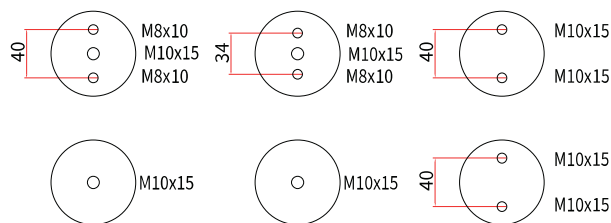
HC-60L-F1 EM-3
