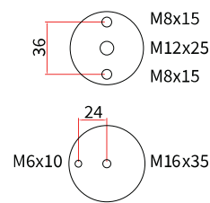
HC-210A-D3
