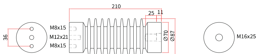
HC-210D-A1
