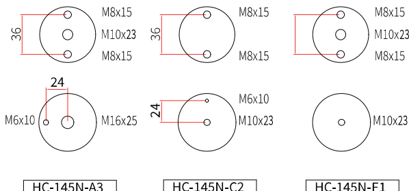
HC-145N-A3
