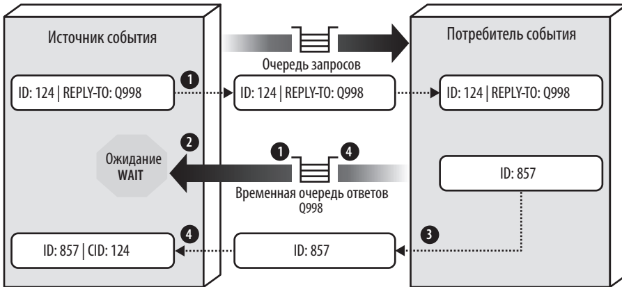
Рис. 14.21. Обработка сообщений по принципу запрос — ответ с использованием временной очереди
