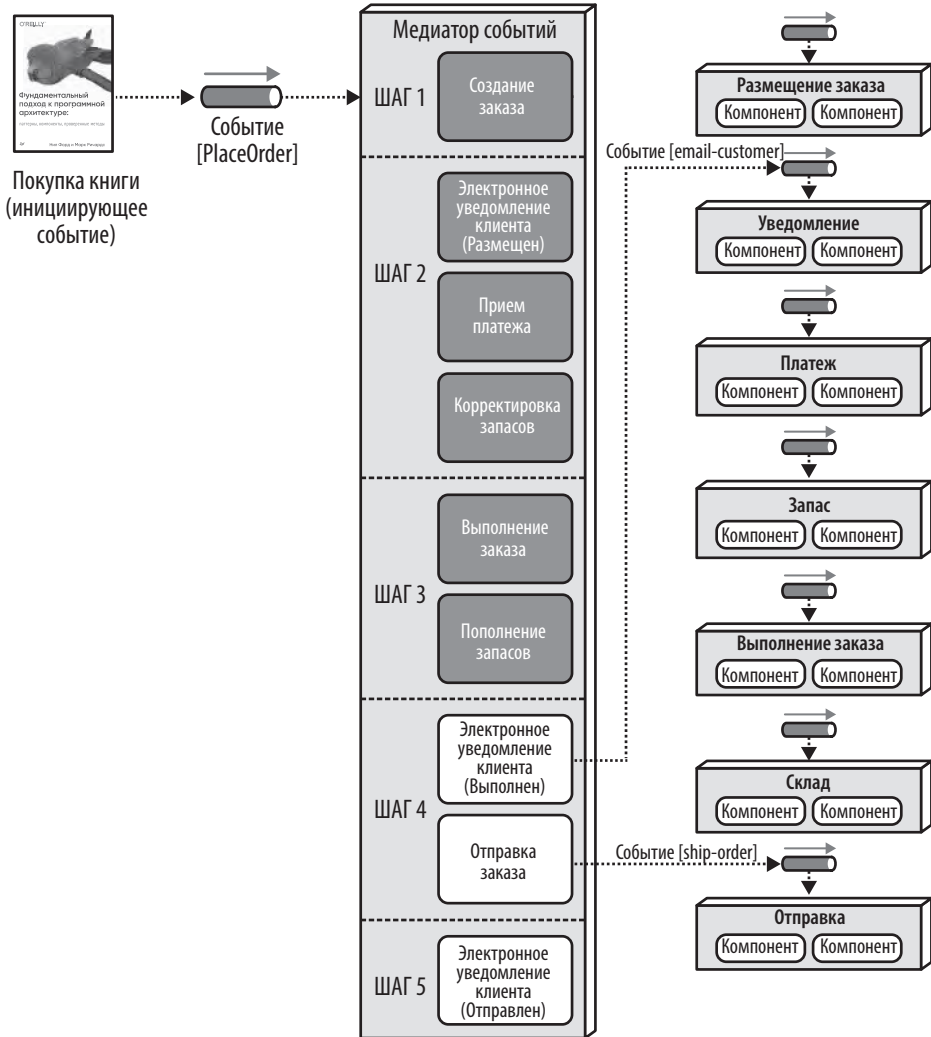
Рис. 14.11. Модератор, шаг 4
