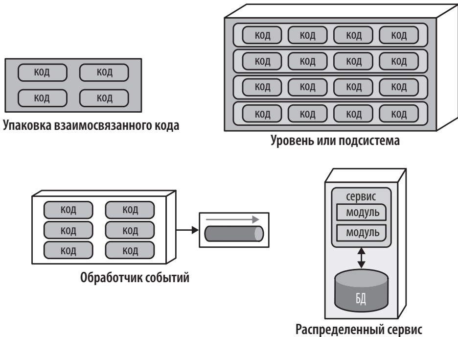
Рис. 8.1. Многообразие компонентов
