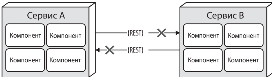
Рис. 9.2. Сеть ненадежна
