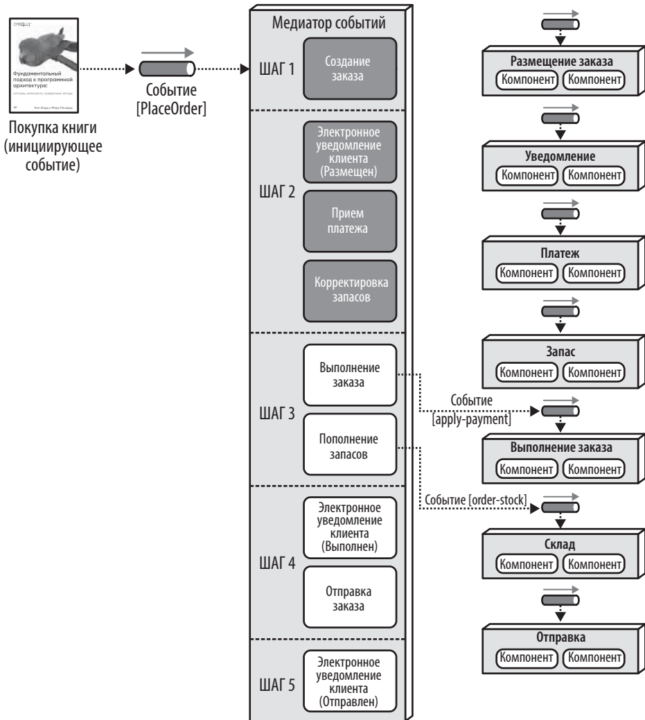
Рис. 14.10. Медиатор, шаг 3
