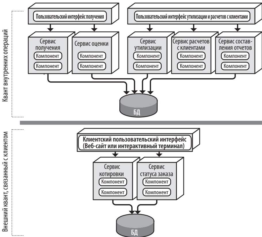
Рис. 13.10. Отдельные кванты в архитектуре на основе сервисов
