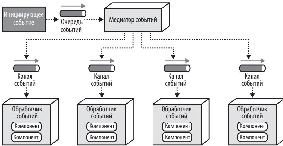
Рис. 14.5. Топология медиатора
