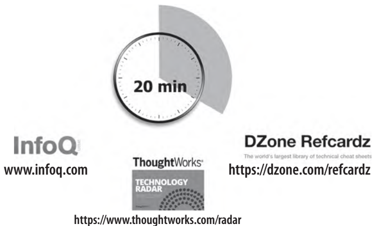
Рис. 24.1. Правило 20 минут
