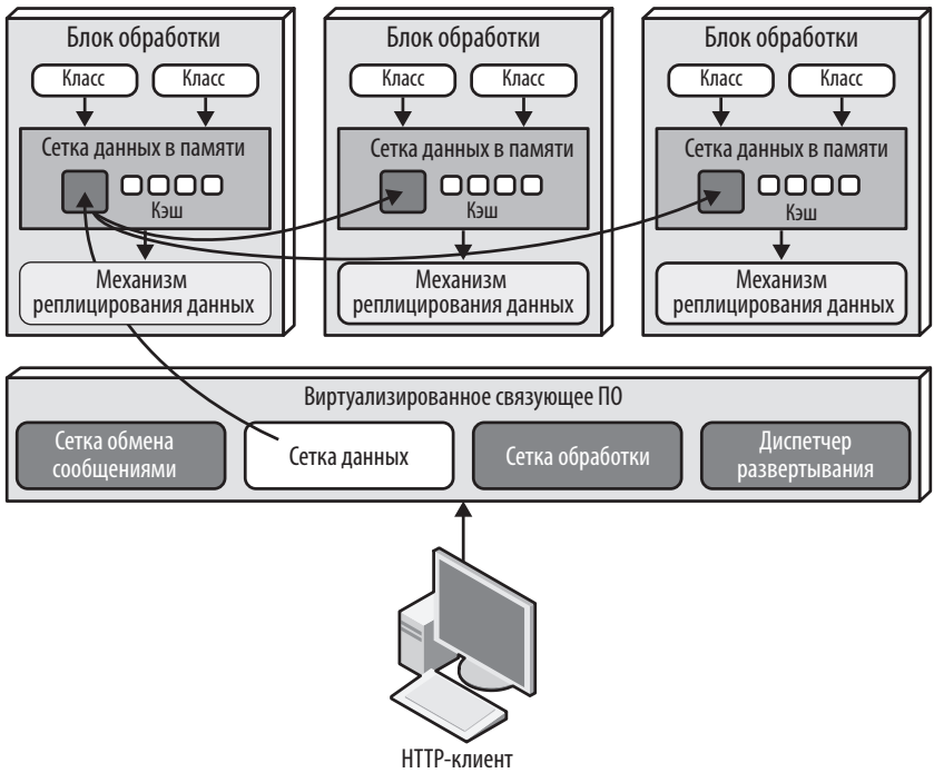
Рис. 15.5. Сетка данных
