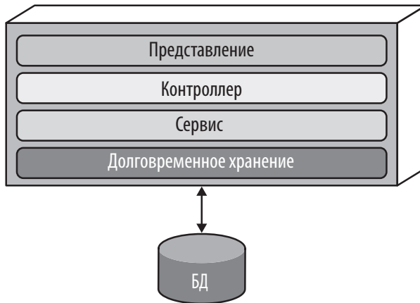
Рис. 6.4. Многоуровневая архитектура
