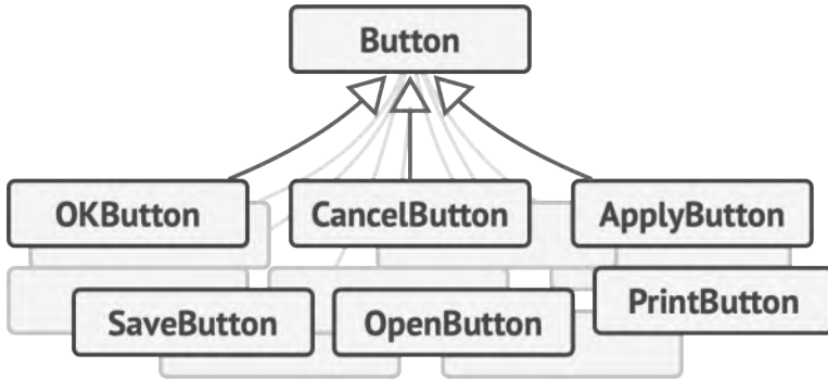
Множество подклассов кнопок.
