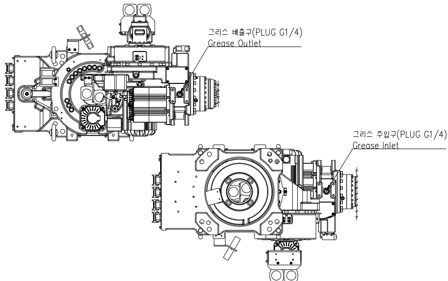
그림 5.7 Arm Frame 그리스 주입/배출구
