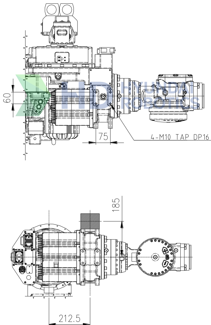
그림 2.6 ARM FRAME 상부 부착부 상세도: [YS140D]
