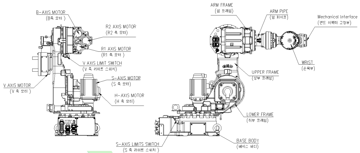
그림 3.1 본체 각 부위 명칭 [YS140D]
