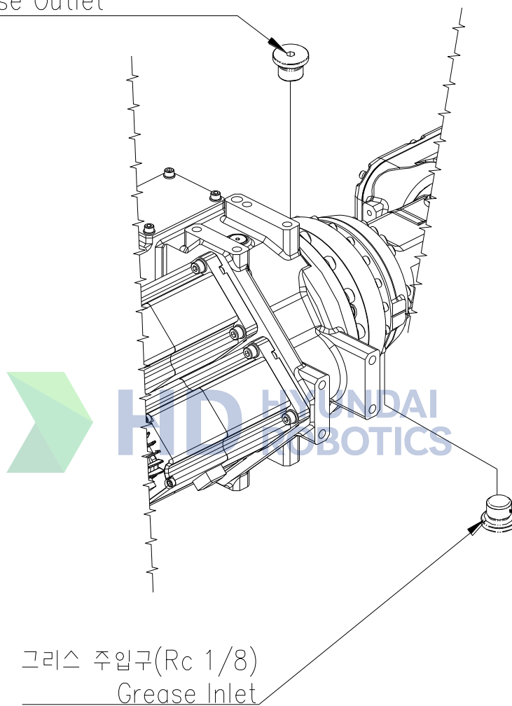
그림 5.4 R2 축 감속기 그리스 주입/배출구
