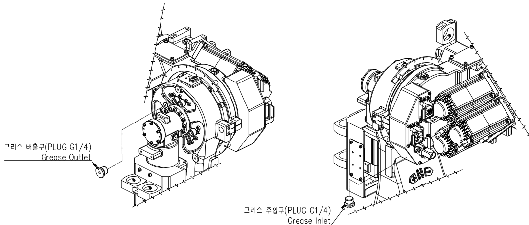
그림 5.3 V 축 감속기 그리스 주입/배출구
