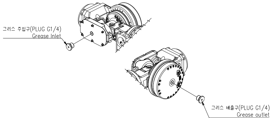
그림 5.5 B 축 감속기 그리스 주입/배출구(YS1400)
