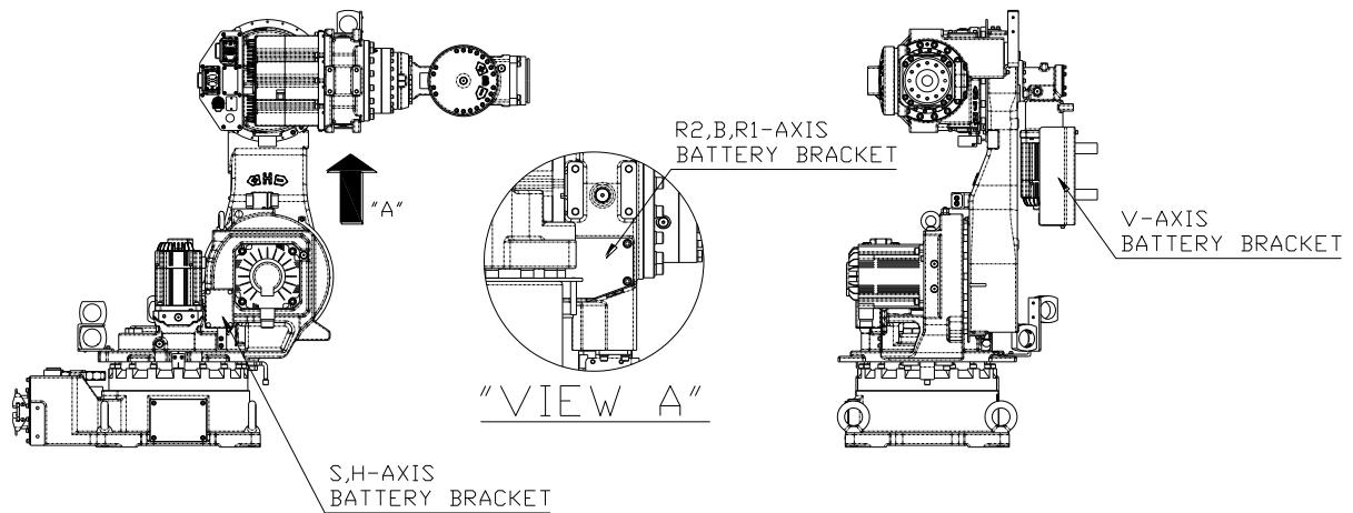
그림 5.8 배터리 교환 위치
