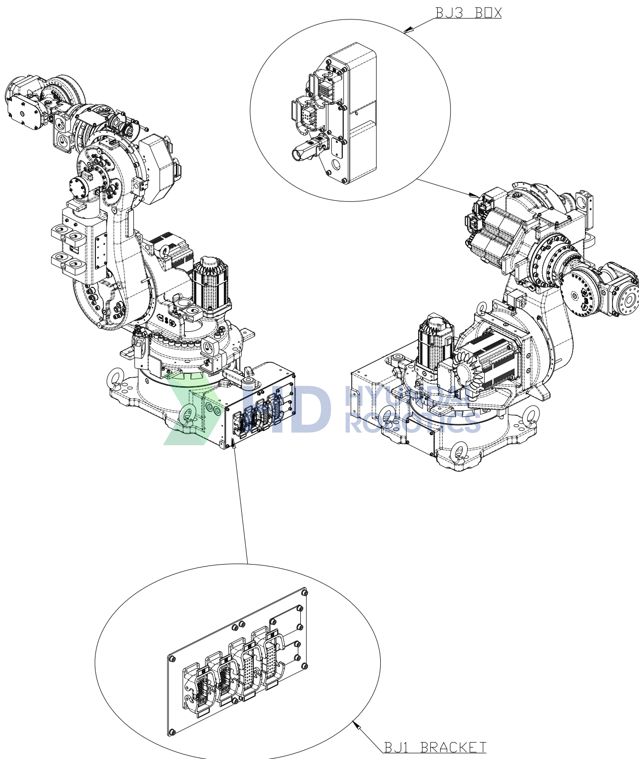
그림 9.1 본체 부품 배치 [YS1400]
