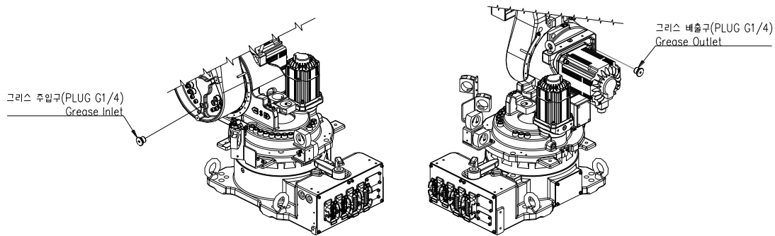
그림 5.2 H 축 감속기 그리스 주입/배출구
