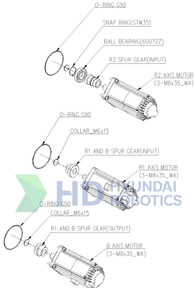
그림 6.4 R2/B/R1 축 모터 ASSEMBLY
