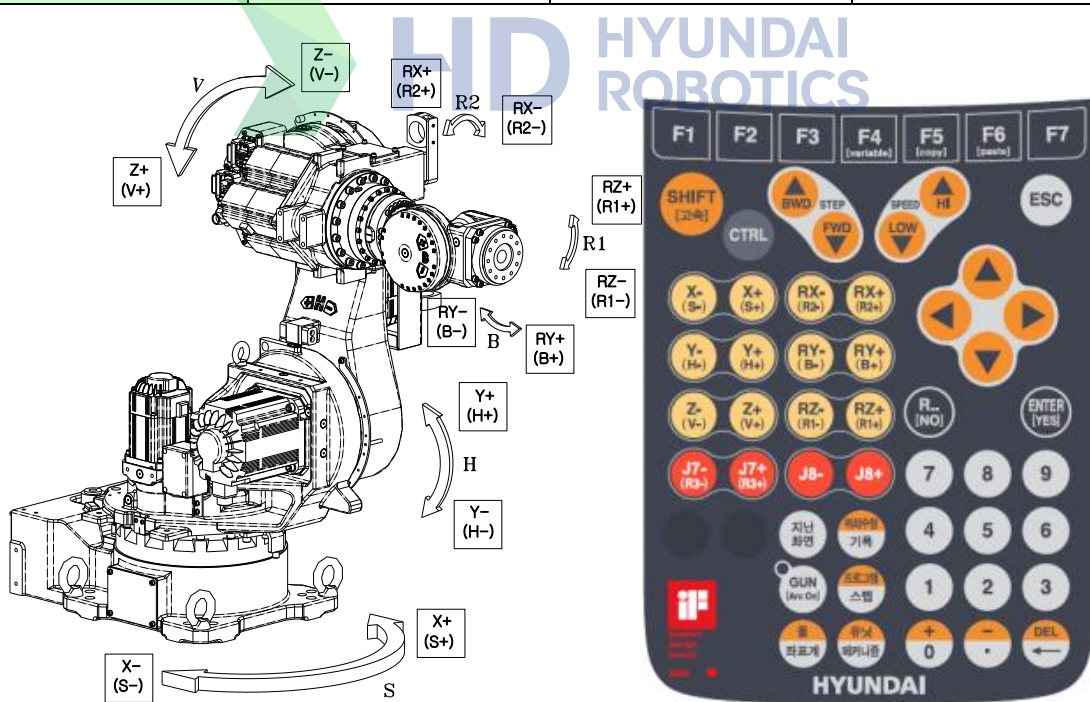
그림 2.4 본체 외관 및 동작 축 [YS140D]
