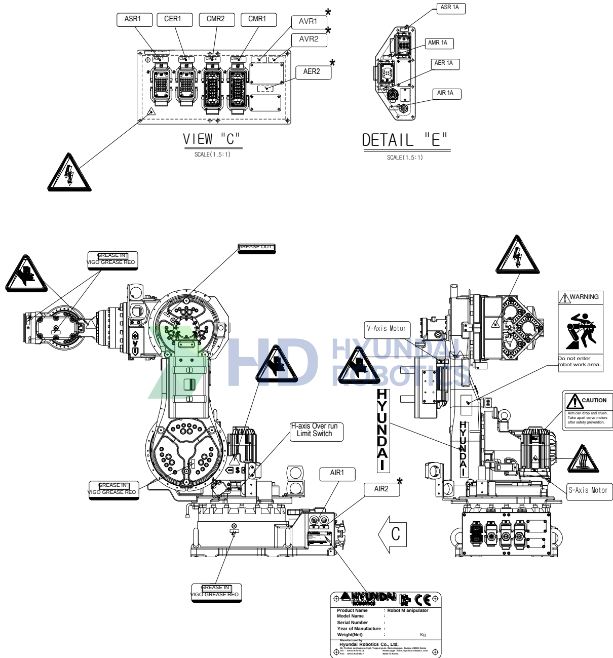
그림 3.3 안전 명판 위치[YS140D]
