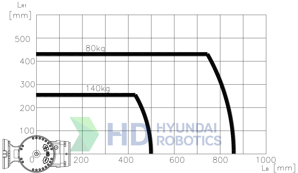
그림 3.9 손목축 토크 선도: [YS140D]
