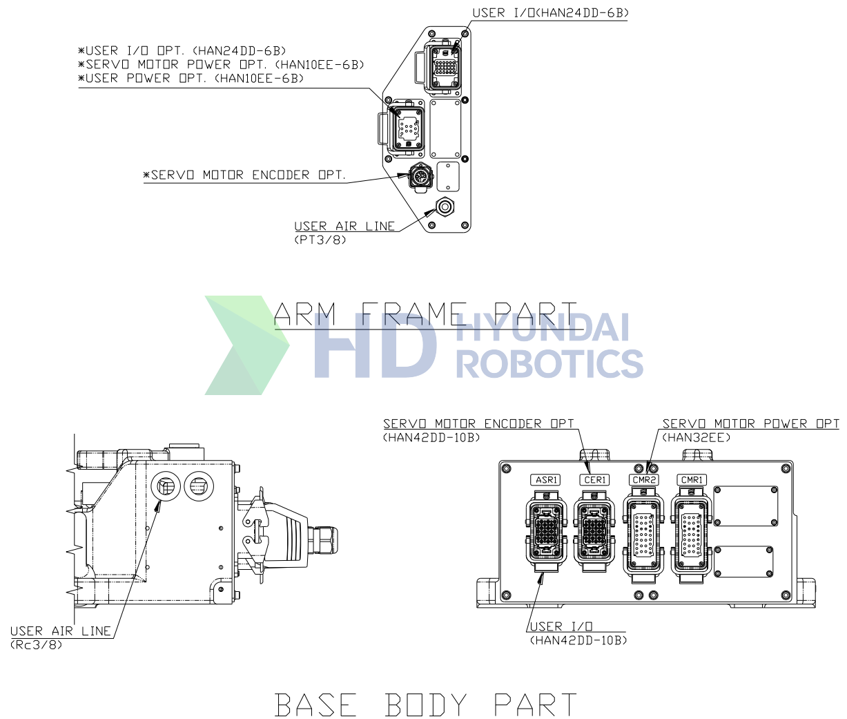
그림 2.7 어플리케이션용 배선 및 배관도: [YS140D]
