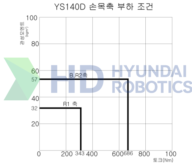
그림 3.10 손목축 부하조건: [YS140D]
