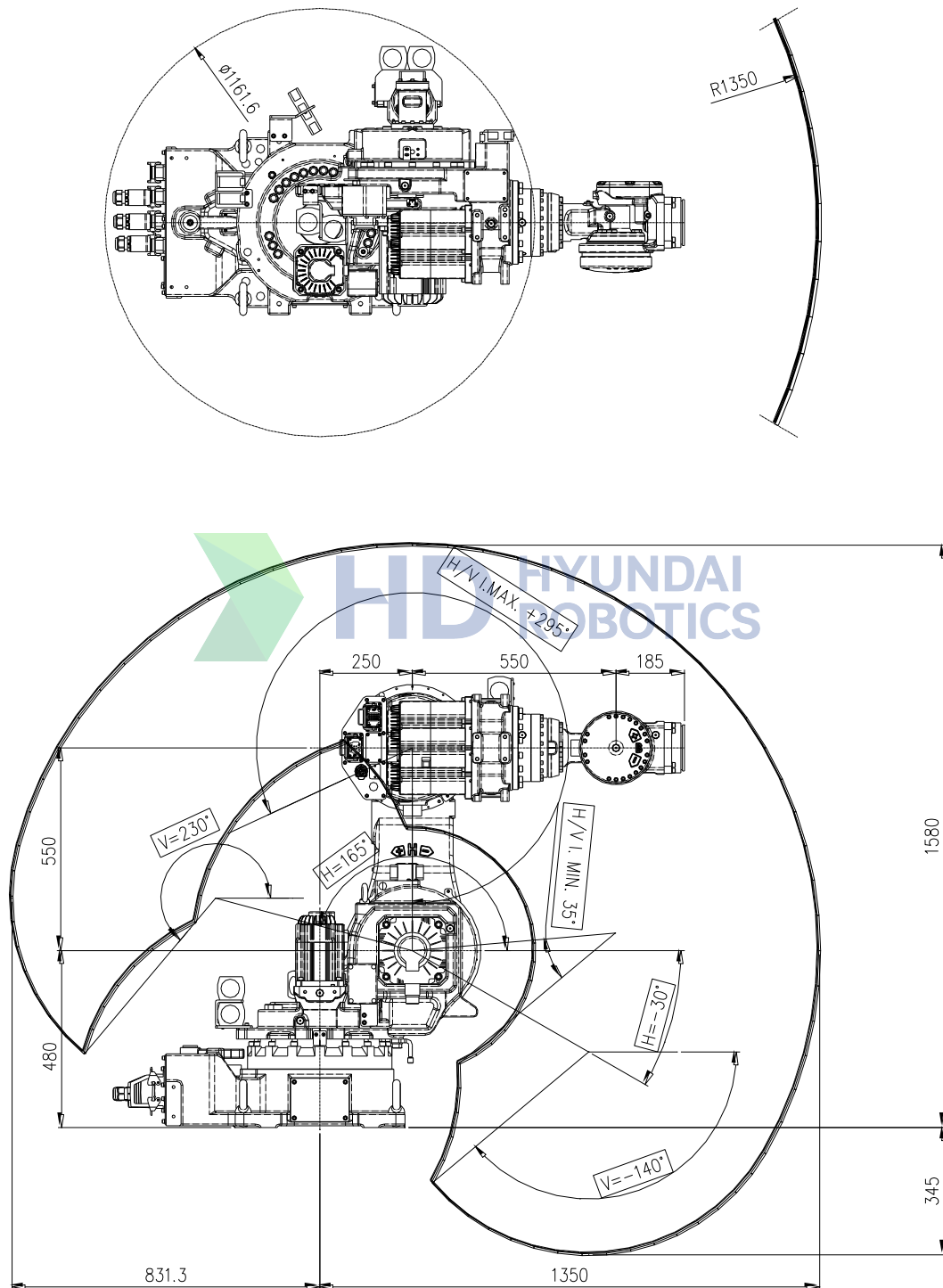
그림 2.3 로봇 본체 외형 치수 및 동작 영역 [YS140D]
