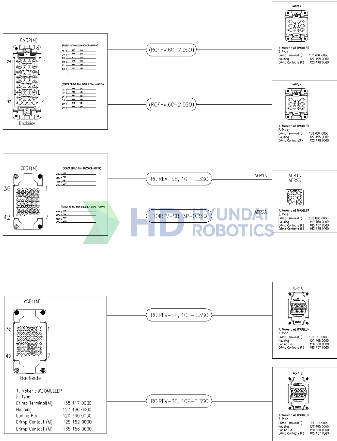
그림 2.8 어플리케이션 커넥터 상세 : [YS140D]
