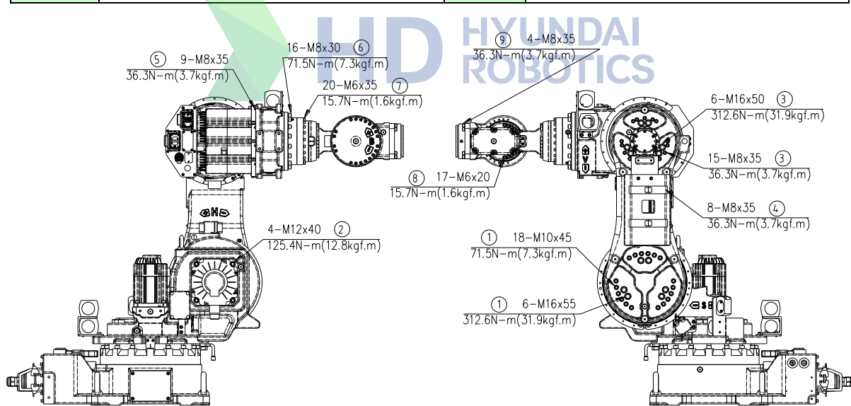
그림 4.1 주요 볼트 점검 부위 [YS1400]
