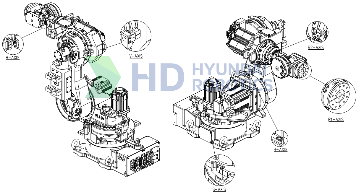
그림 6.5 원점 설정 방법 [YS140D]
