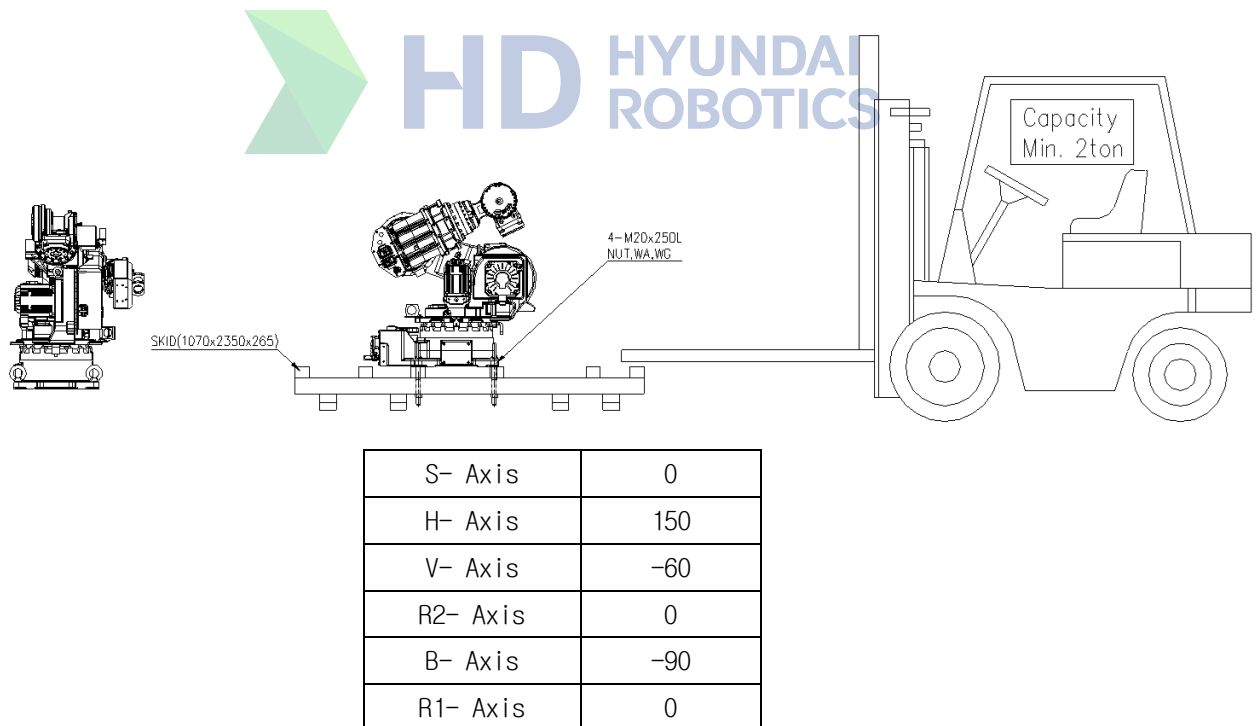
그림 3.5 운송 방법 : 지게차 이용
