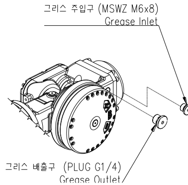
그림 5.6 R1 축 감속기 그리스 주입/배출구
