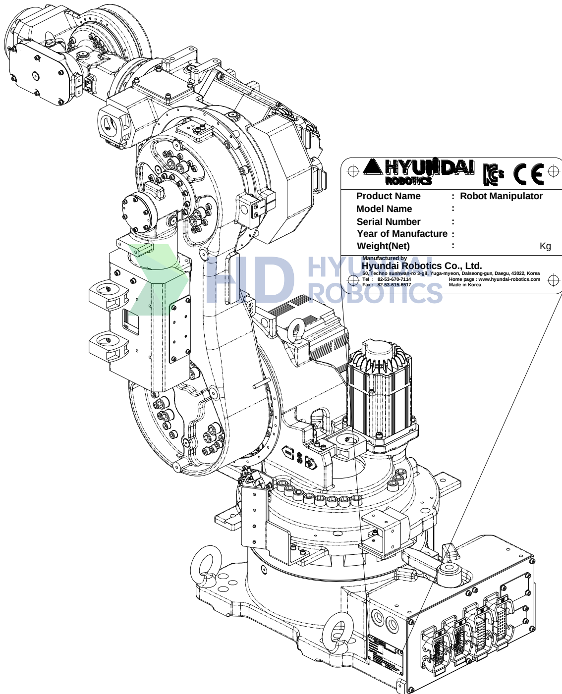
그림 2.2 로봇 명판 부착 위치
