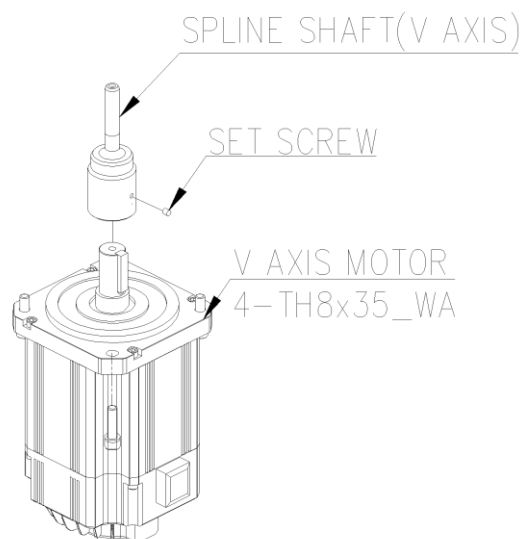
그림 6.3 V 축 모터 ASSEMBLY
