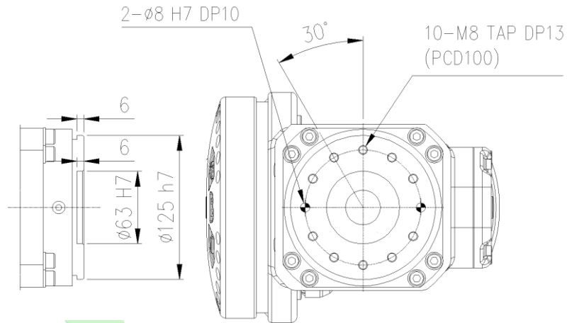
그림 2.5 손목축 취부면 상세도 : [YS140D]
