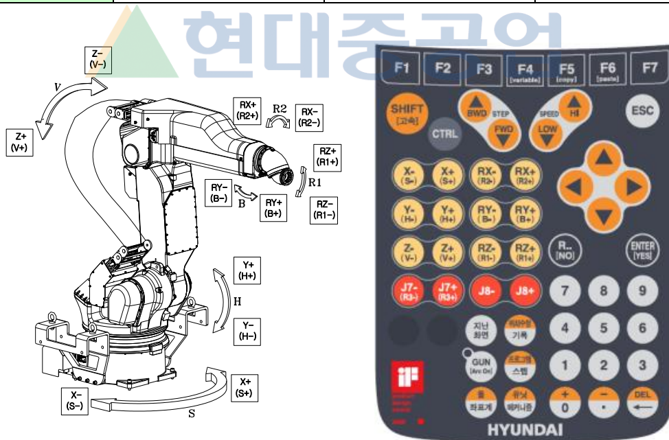
그림 2.4 본체 외관 및 동작 축 [YP020-29]
