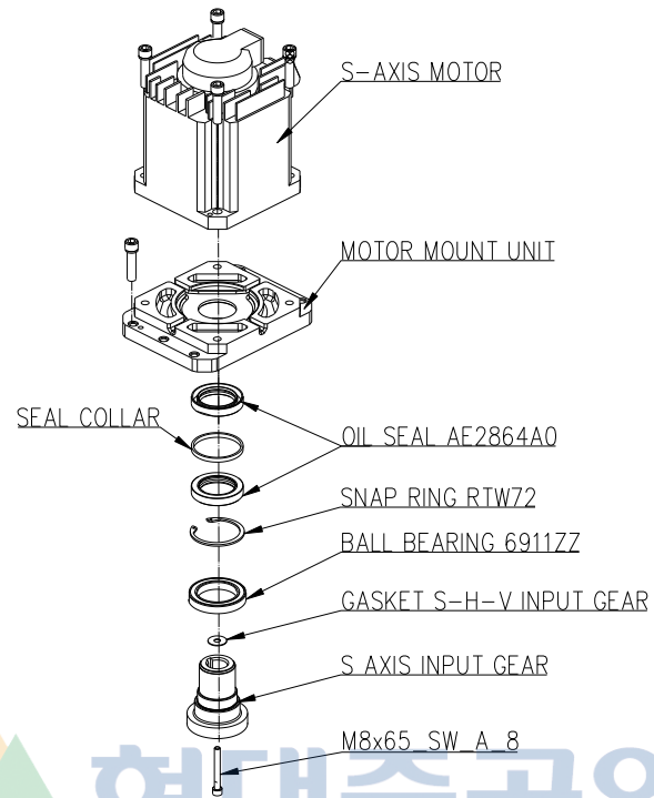
그림 6.1 S 축 모터 ASSEMBLY
