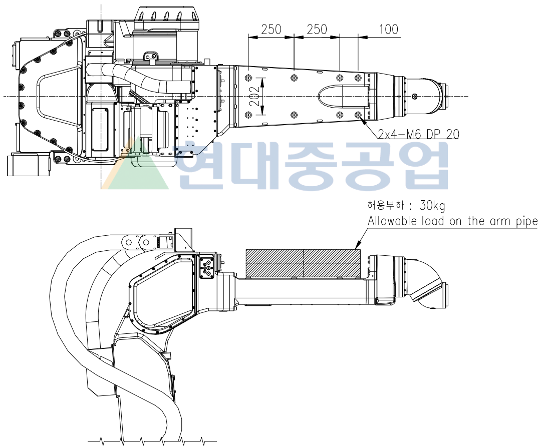
그림 2.6 ARM FRAME 상부 부착부 상세도: [YP020-29]
