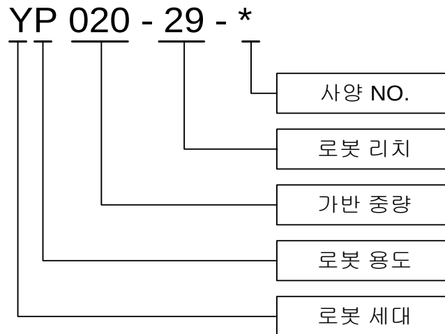
그림 2.1 로봇 기구부 형식
