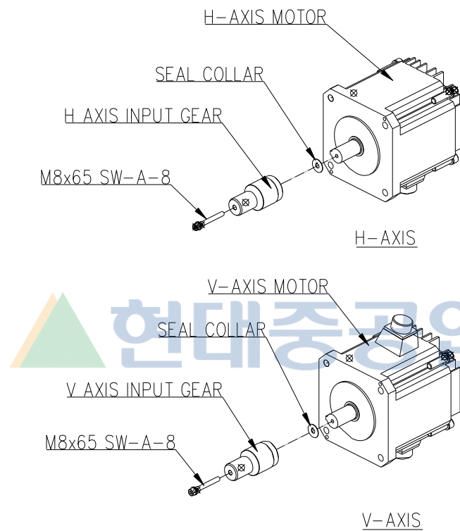
그림 6.2 H&V 축 모터 ASSEMBLY
