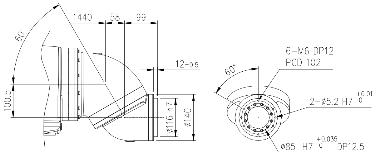
그림 2.5 손목축 취부면 상세도: [YP020-29]
