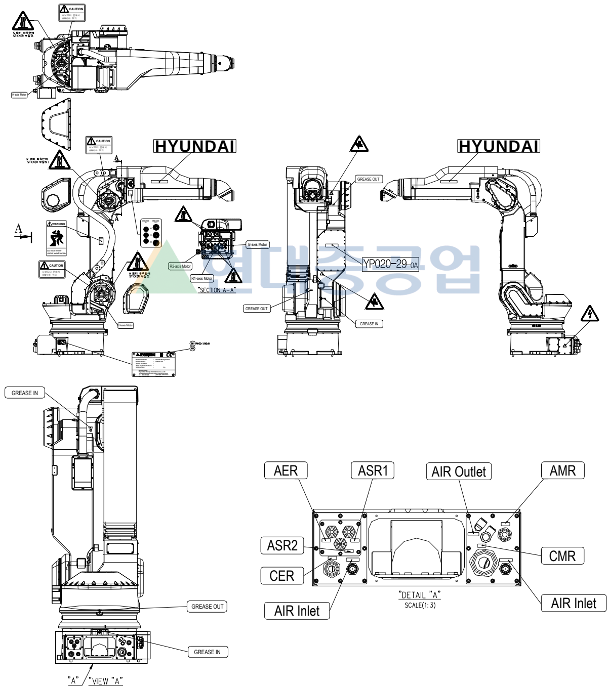
그림 3.2 안전 명판 위치
