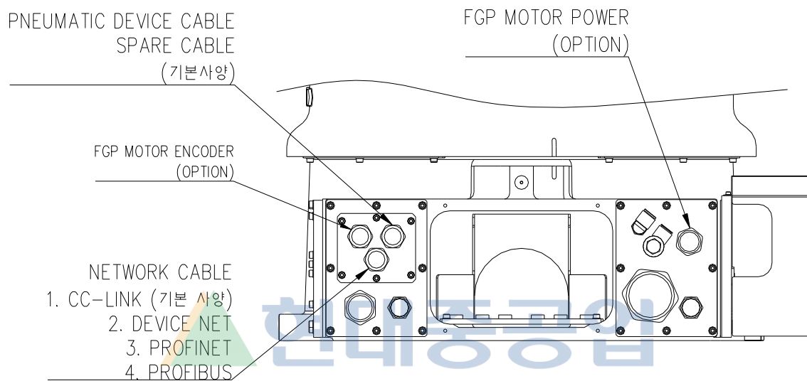
그림 2.7 어플리케이션용 배선 및 배관도: [YP020-29]
