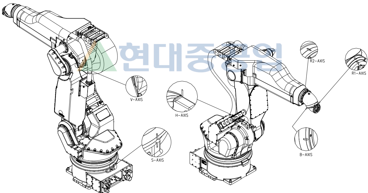
그림 6.4 원점 설정 방법 [YP020-29]
