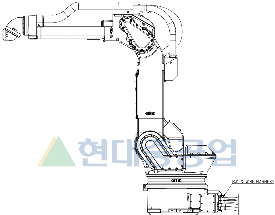
그림 8.1 본체 부품 배치
