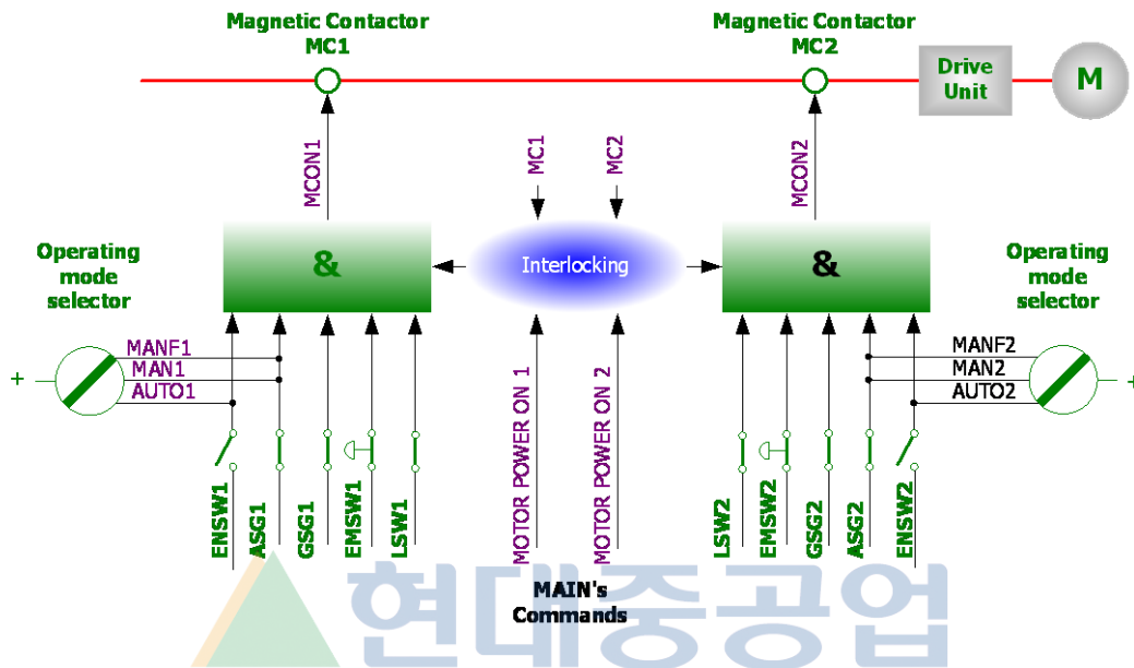
그림 1.5 안전체인 구성도
