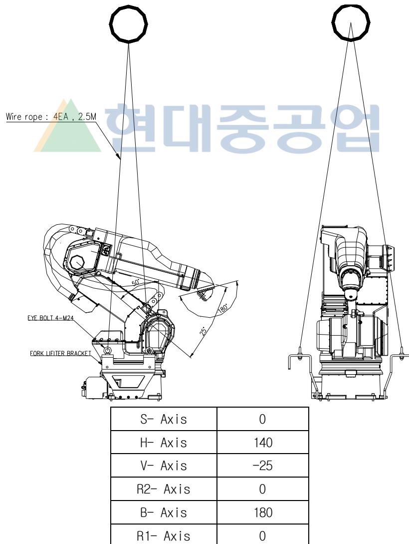
그림 3.3 운송 방법: 크레인 이용 [YP020-29]
