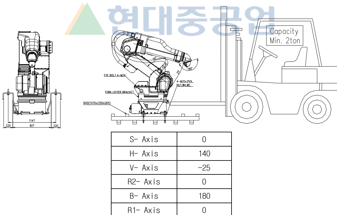
그림 3.4 운송 방법: 지게차 이용 [YP020-29]
