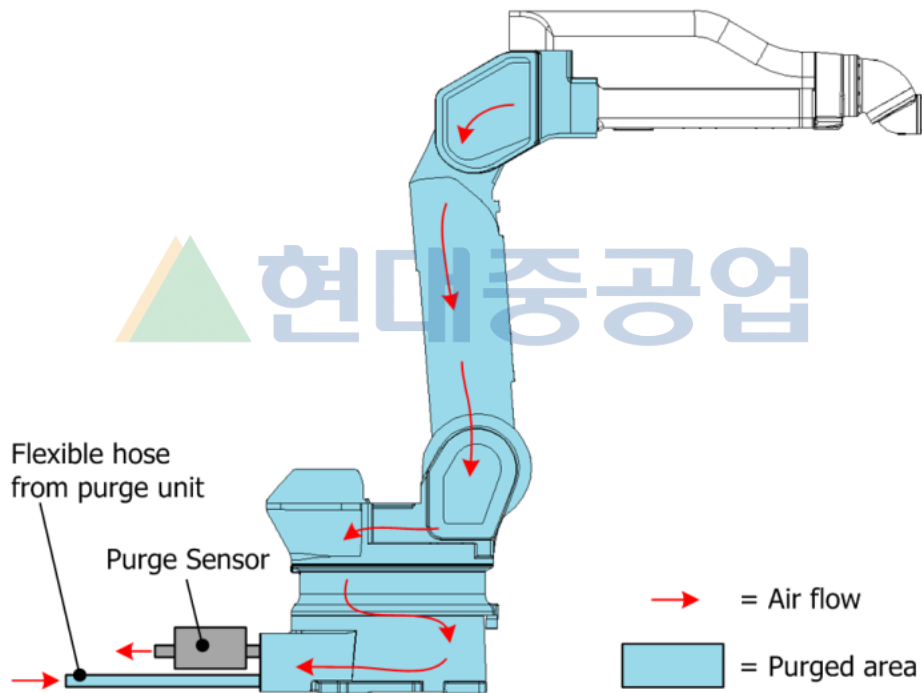
그림 2.8 압력방폭시 공기 흐름도: [YP020-29]
