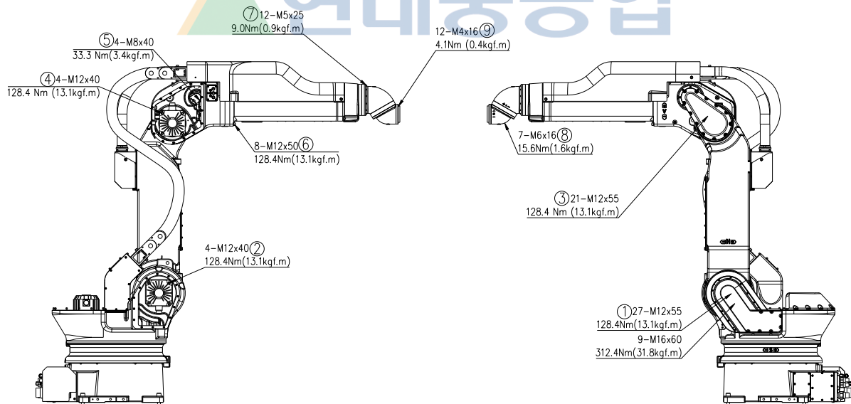
그림 4.1 주요 볼트 점검 부위
