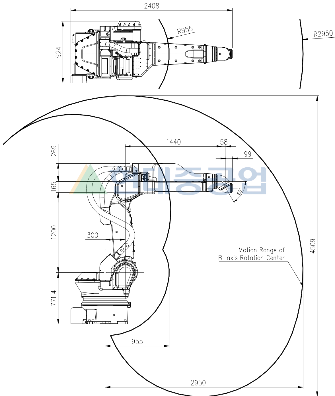
그림 2.3 로봇 본체 외형 치수 및 동작 영역: [YP020-29]
