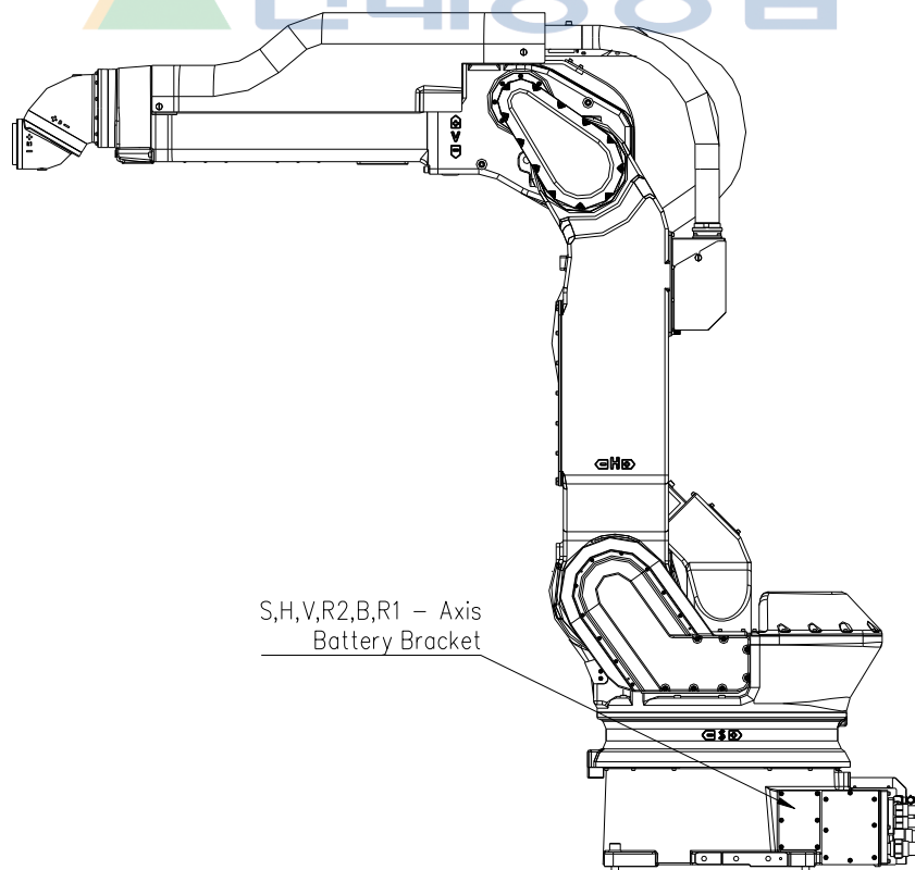
그림 5.1 배터리 교환 위치
