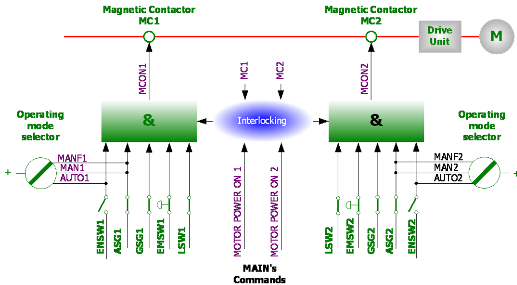
HYUNDAI ROBOTICS 그림 1.5 안전체인 구성도
