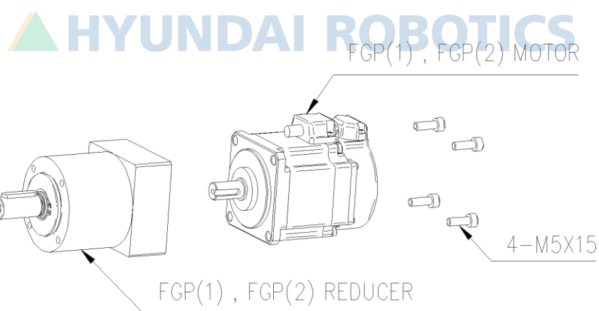
그림 6.4 손목축 모터 ASSEMBLY
