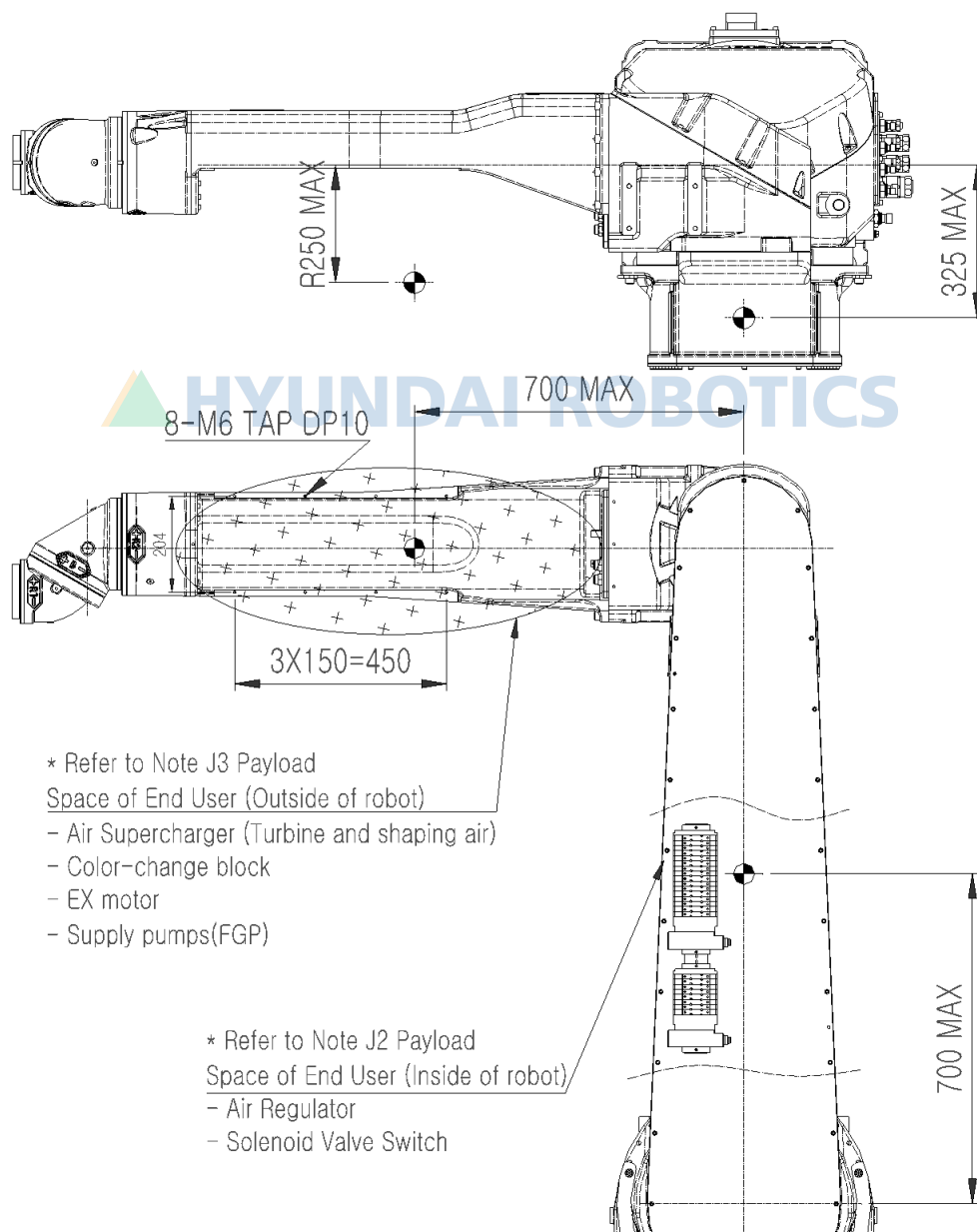
그림 2.6 ARM 부착부 상세도
