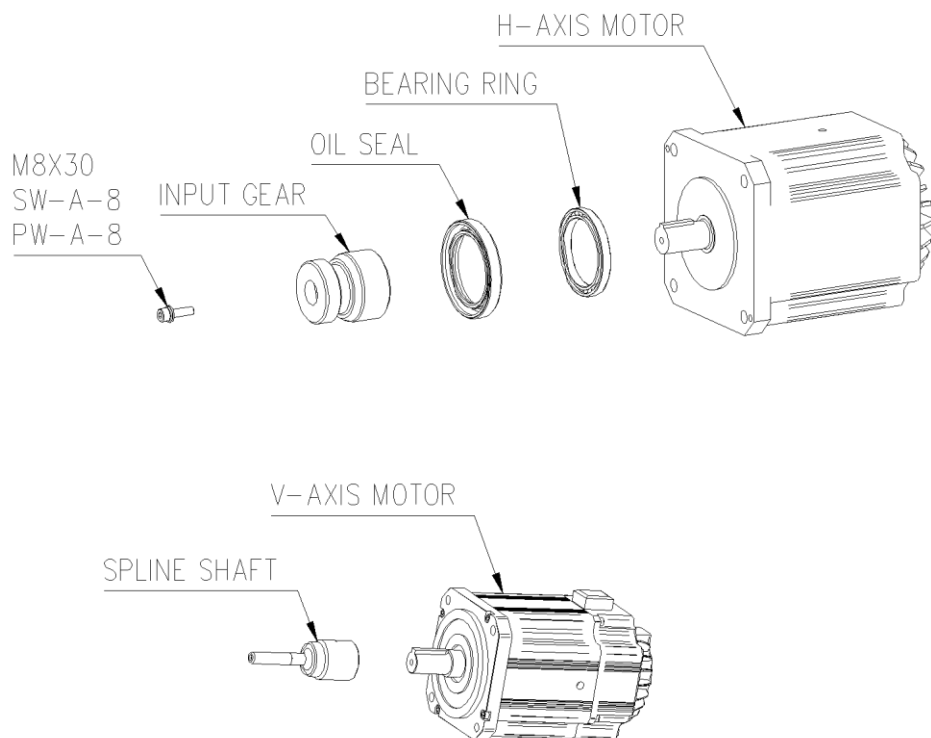
그림 6.3 H&V 축 모터 ASSEMBLY
