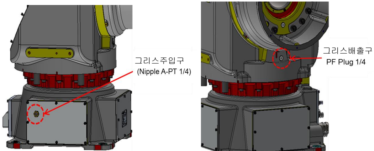
그림 5.1 S 축 구리스 주입/배출구 위치
