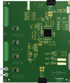
그림 2.15 퍼지 제어 보드
