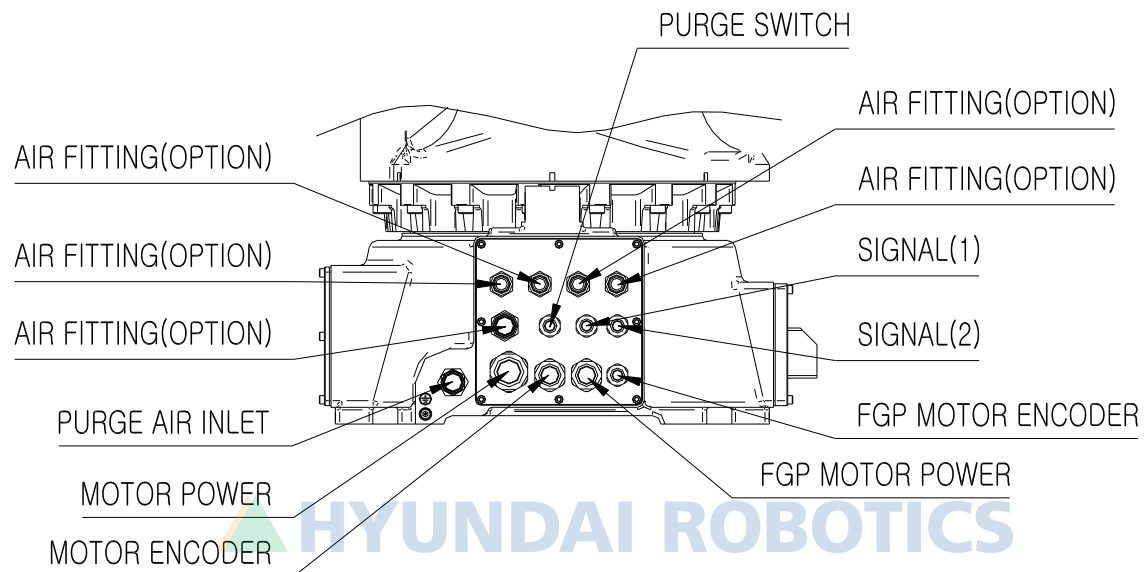
그림 2.12 공압 및 전원 결선 : [Standard]
