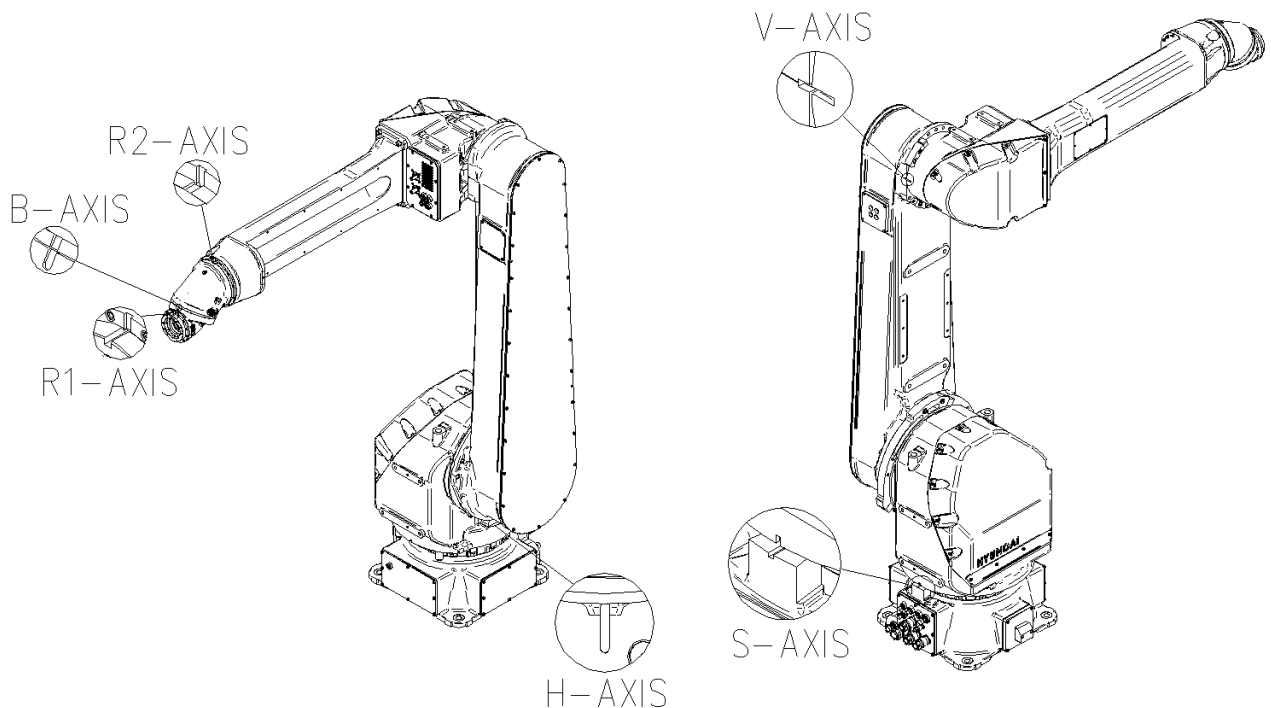
그림 6.6 원점 설정 위치
