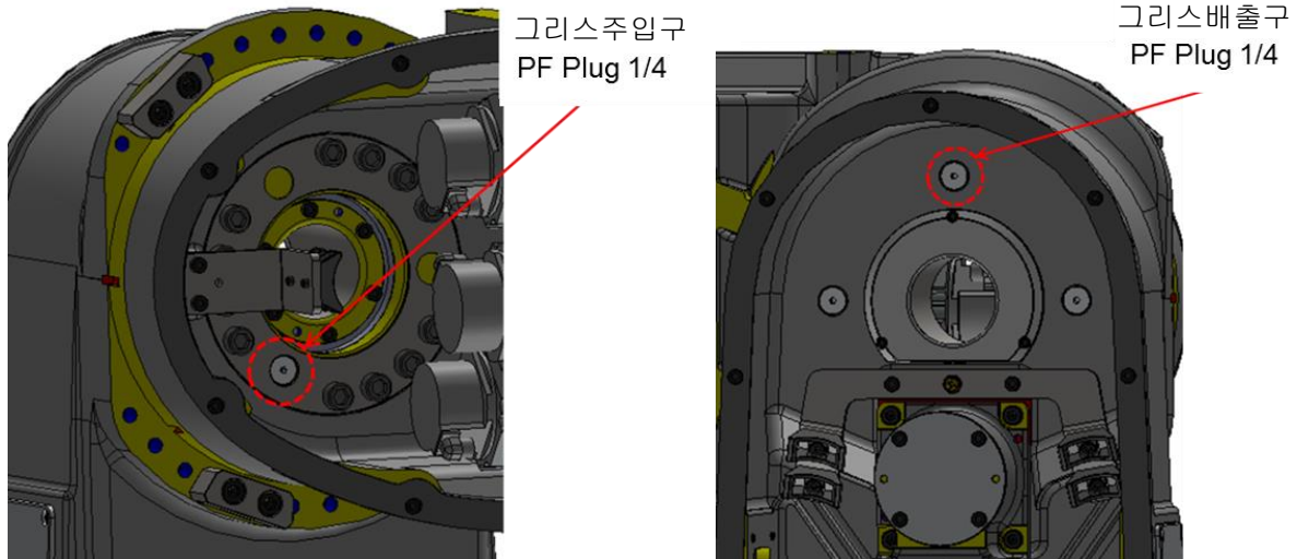
그림 5.3 V 축 그리스 주입/배출구 위치
