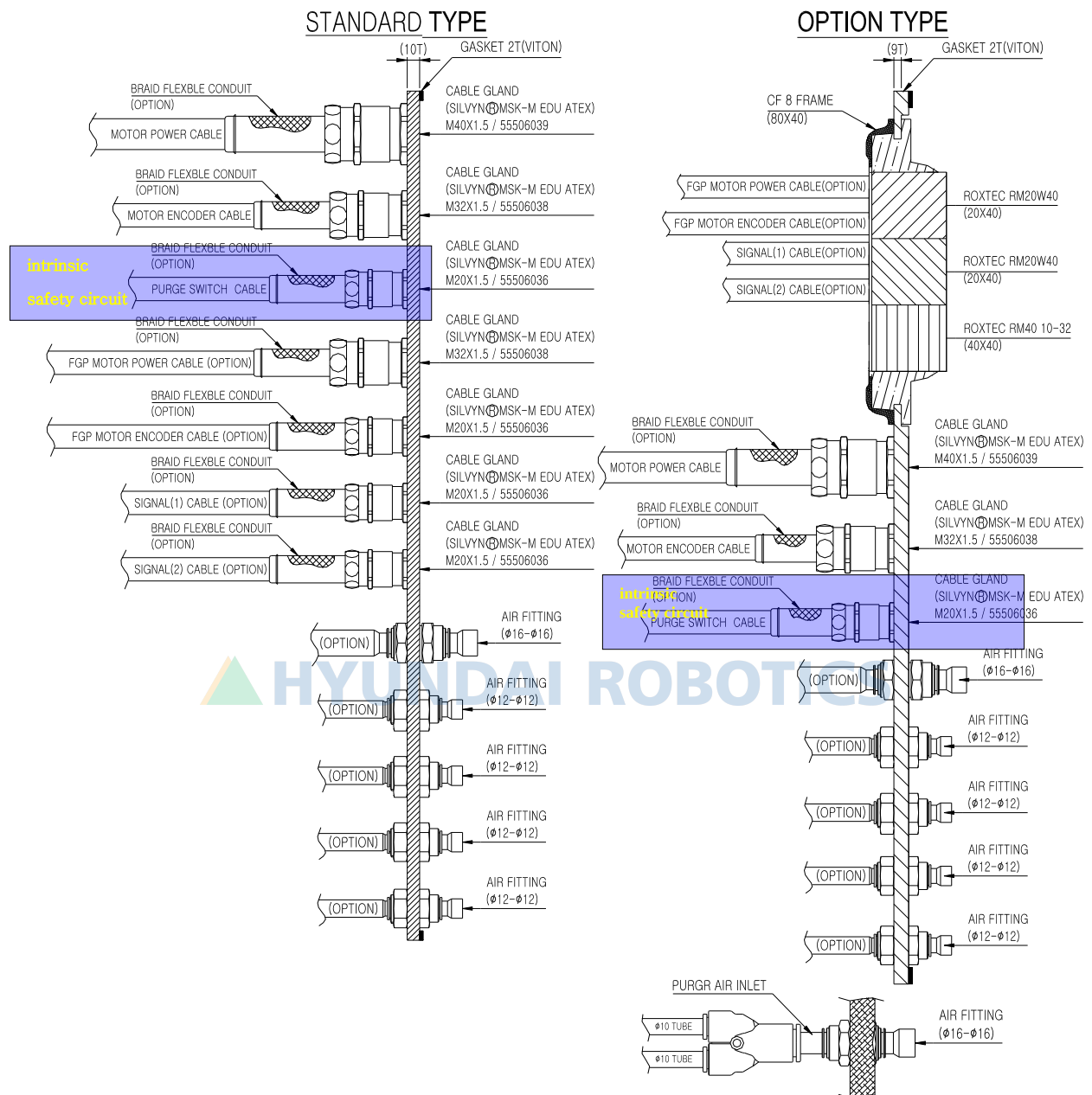
그림 2.14 공압 및 전원
