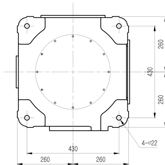
그림 3.6 로봇 설치면 치수
