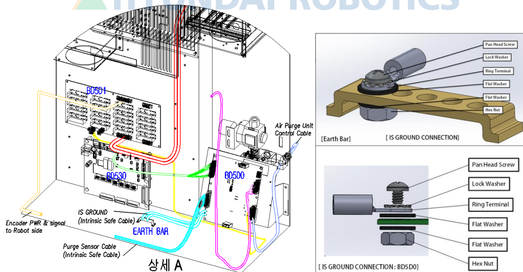
그림 2.16 제어기 내부 배선
