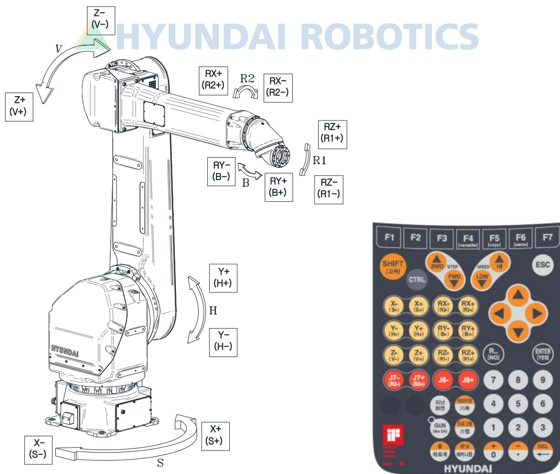
그림 2.4 본체 외관 및 동작 축
