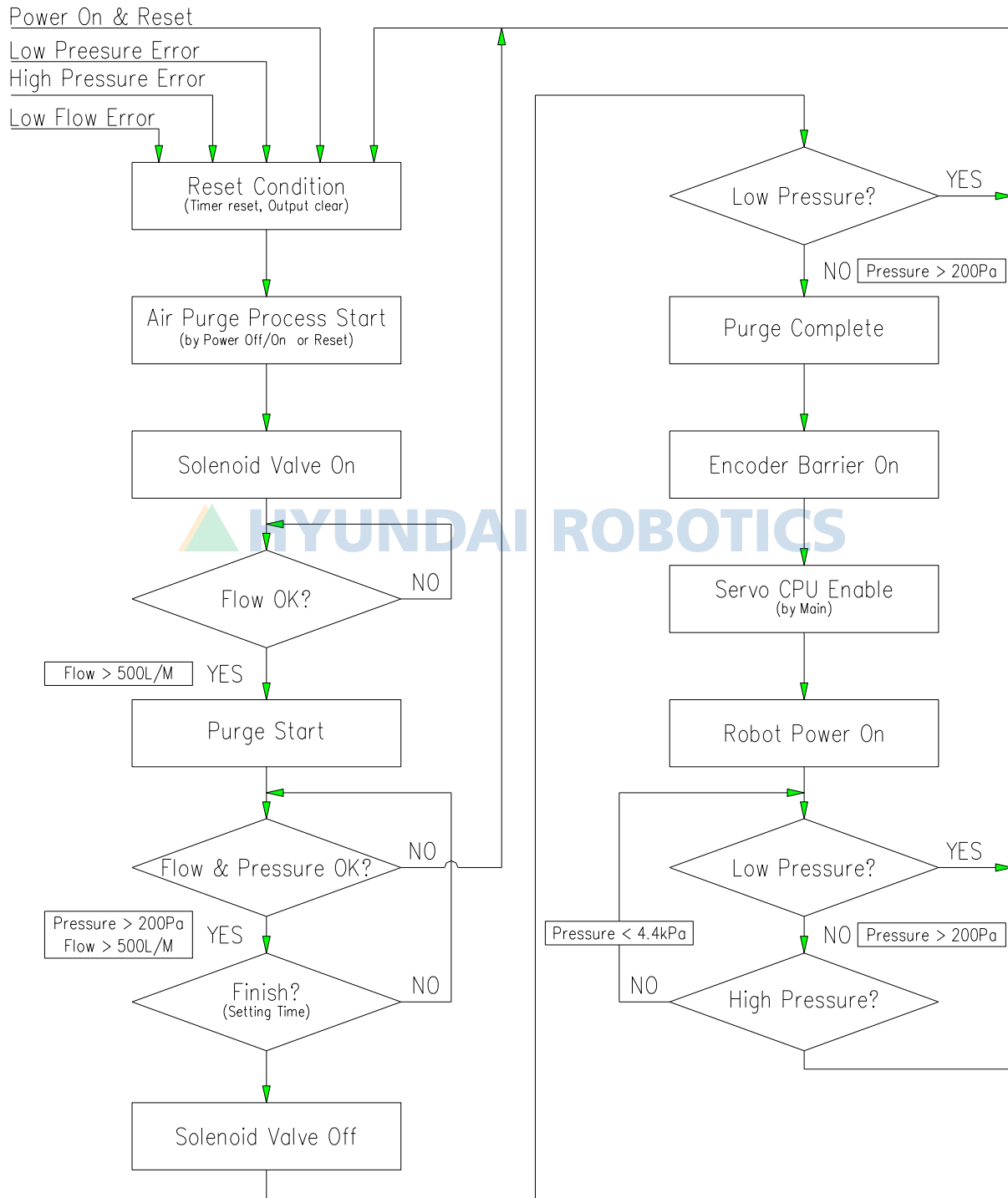
그림 2.10 퍼지 흐름 순서도
