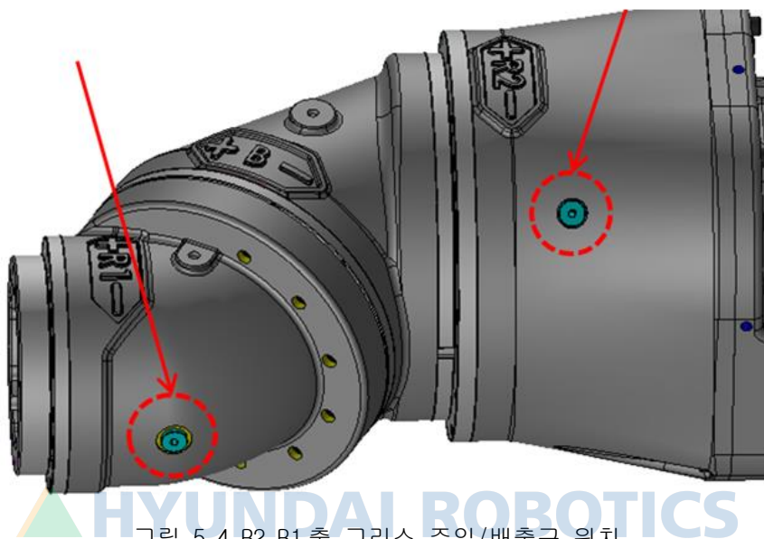
그림 5.4 R2,R1 축 그리스 주입/배출구 위치
