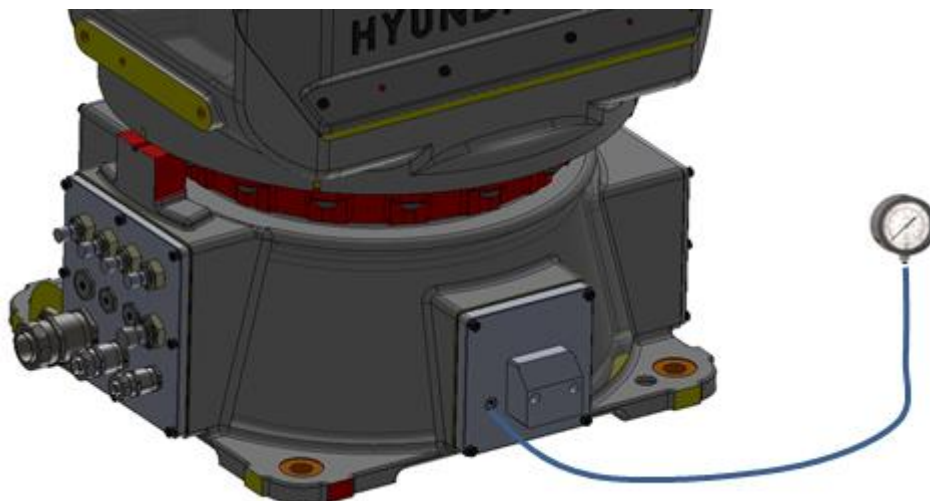
그림 6.1 시험용 포트
