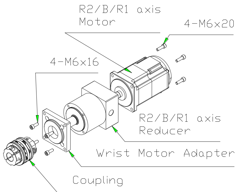
그림 6.4 손목축 모터 ASSEMBLY
