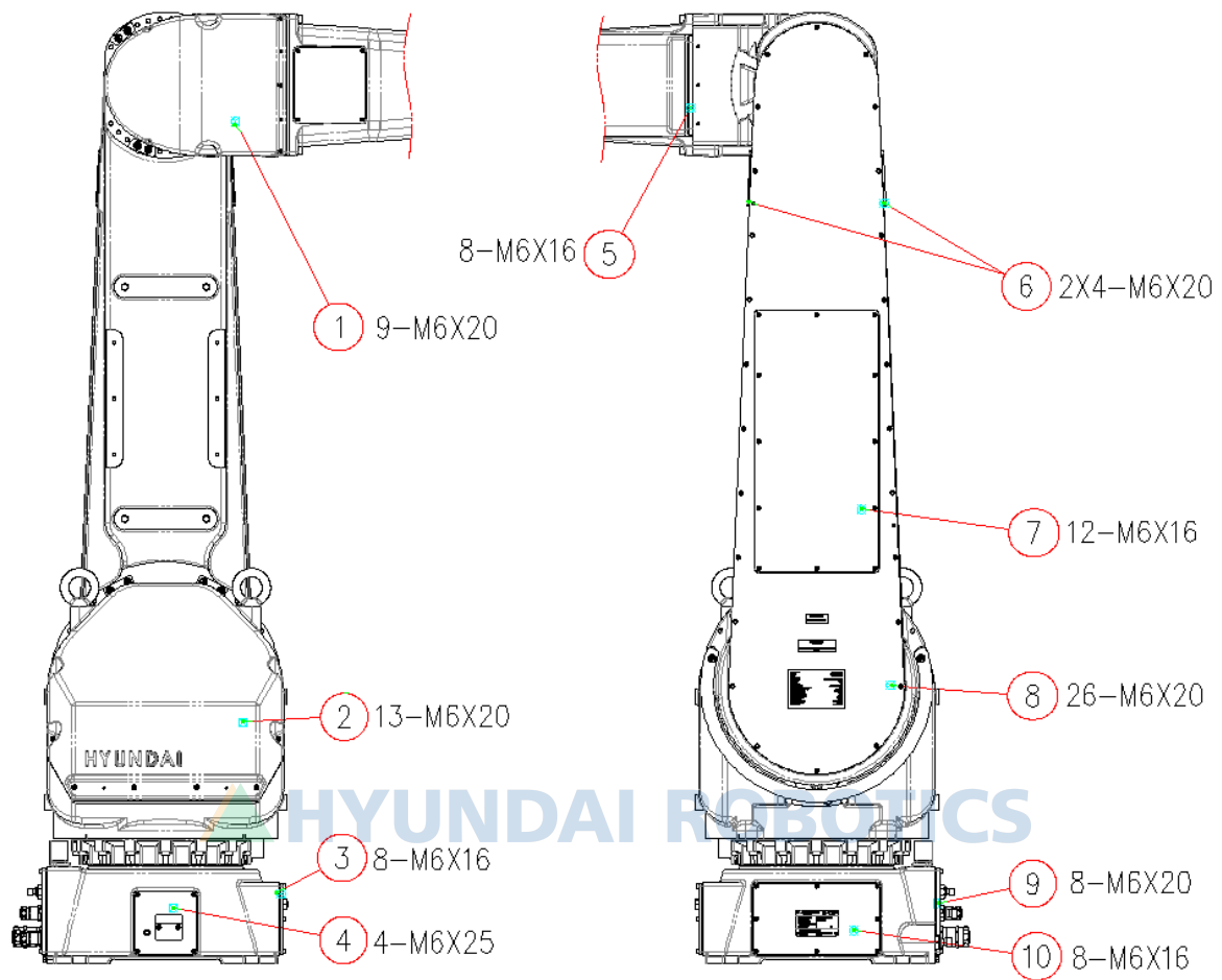
그림 4.2 각 커버 부의 볼트 위치
