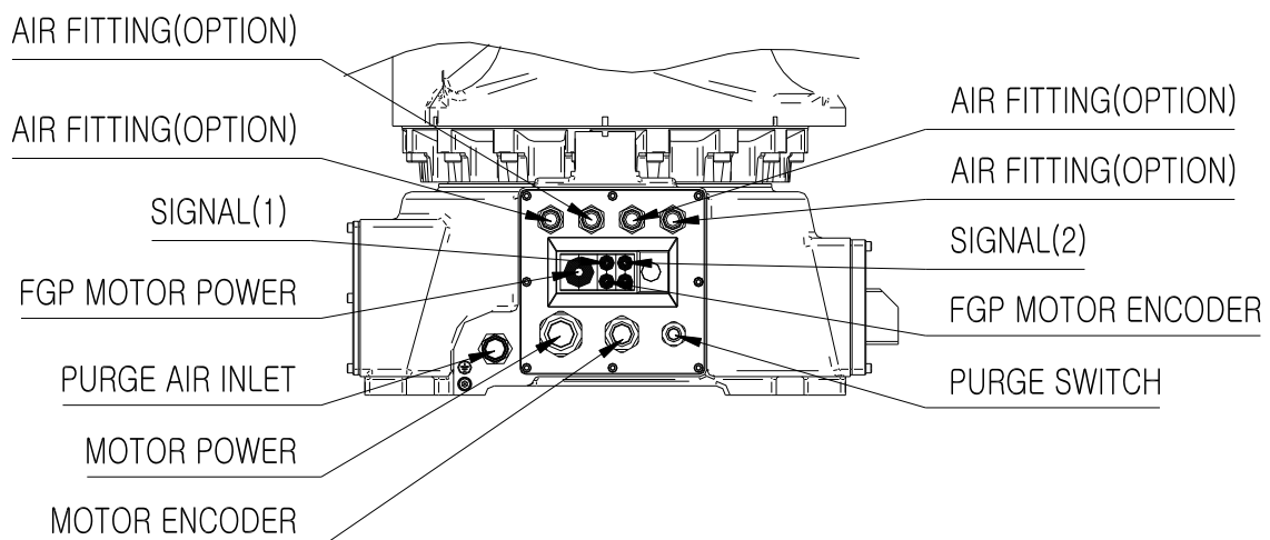
그림 2.13 공압 및 전원 결선 : [Option]
