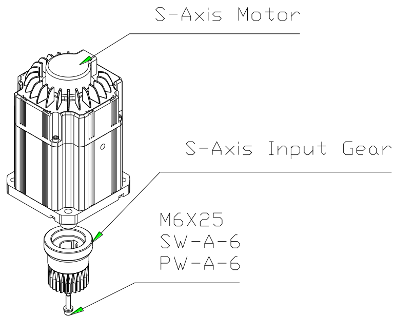
그림 6.2 S 축 모터 ASSEMBLY
