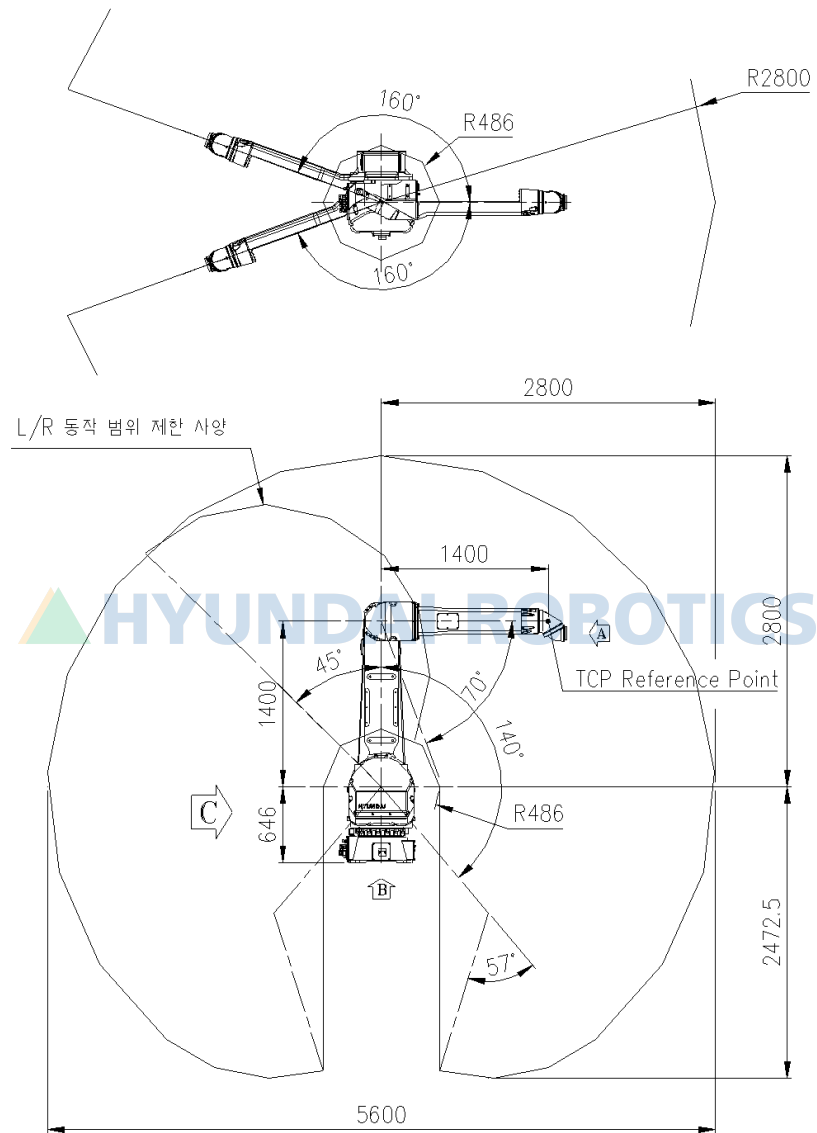
그림 2.3 로봇 본체 외형 치수 및 동작 영역
