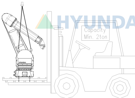
그림 3.4 운송 방법 : 지게차 이용
