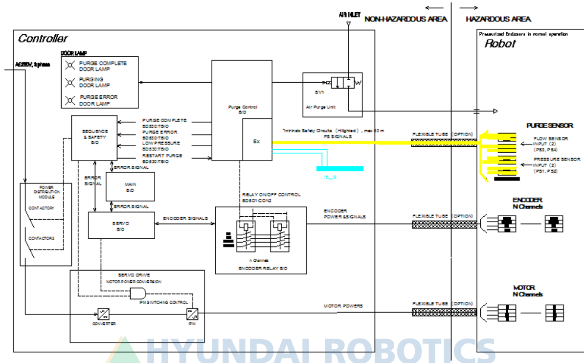
그림 2.8 에어 제어 회로도
