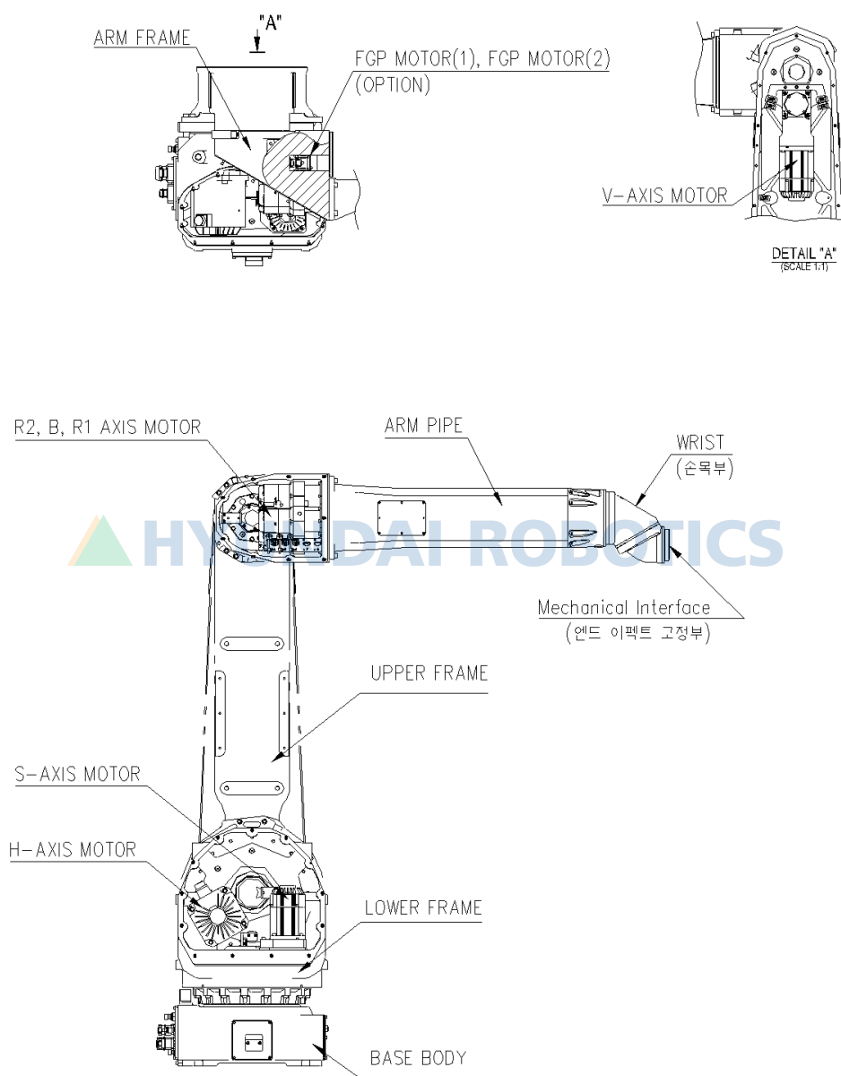
그림 3.1 본체 각 부위 명칭
