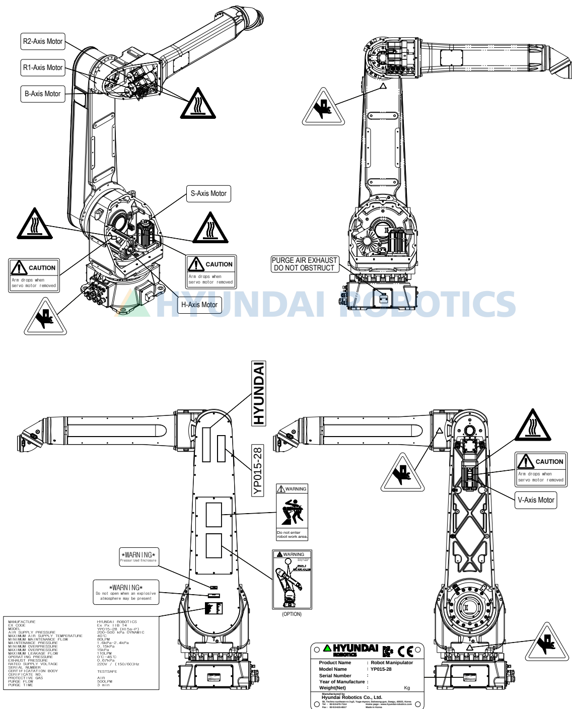
그림 3.2 안전 명판 위치
