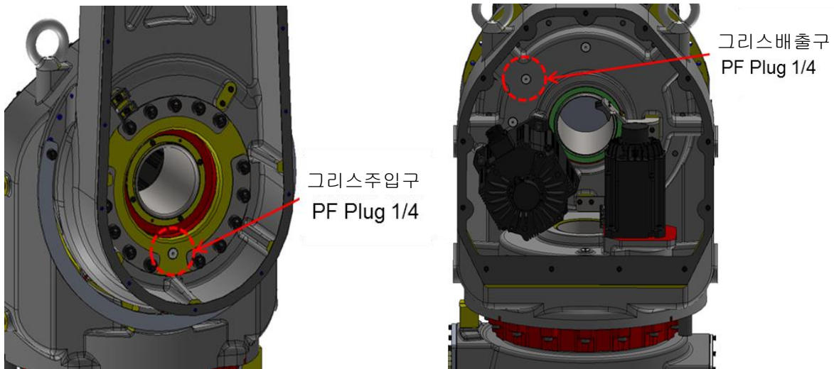
그림 5.2 H 축 그리스 주입/배출구 위치
