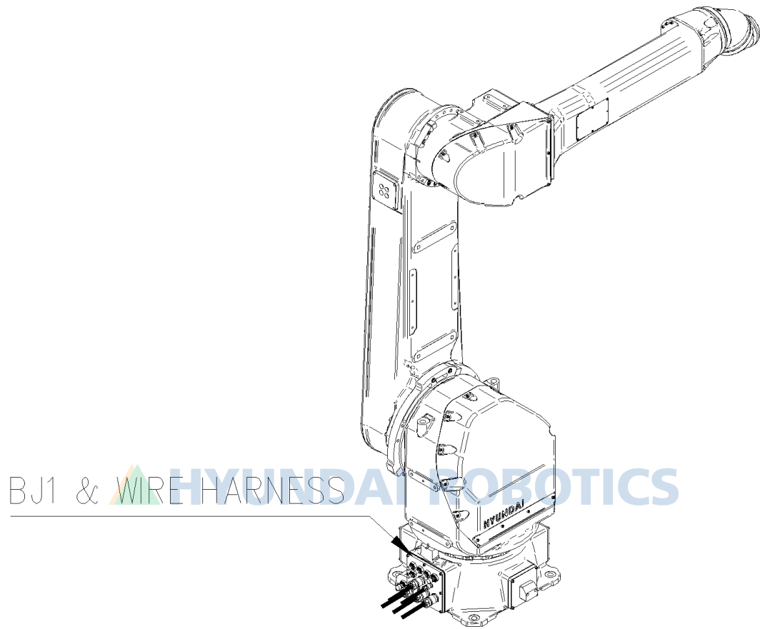
그림 9.1 본체 부품 배치
