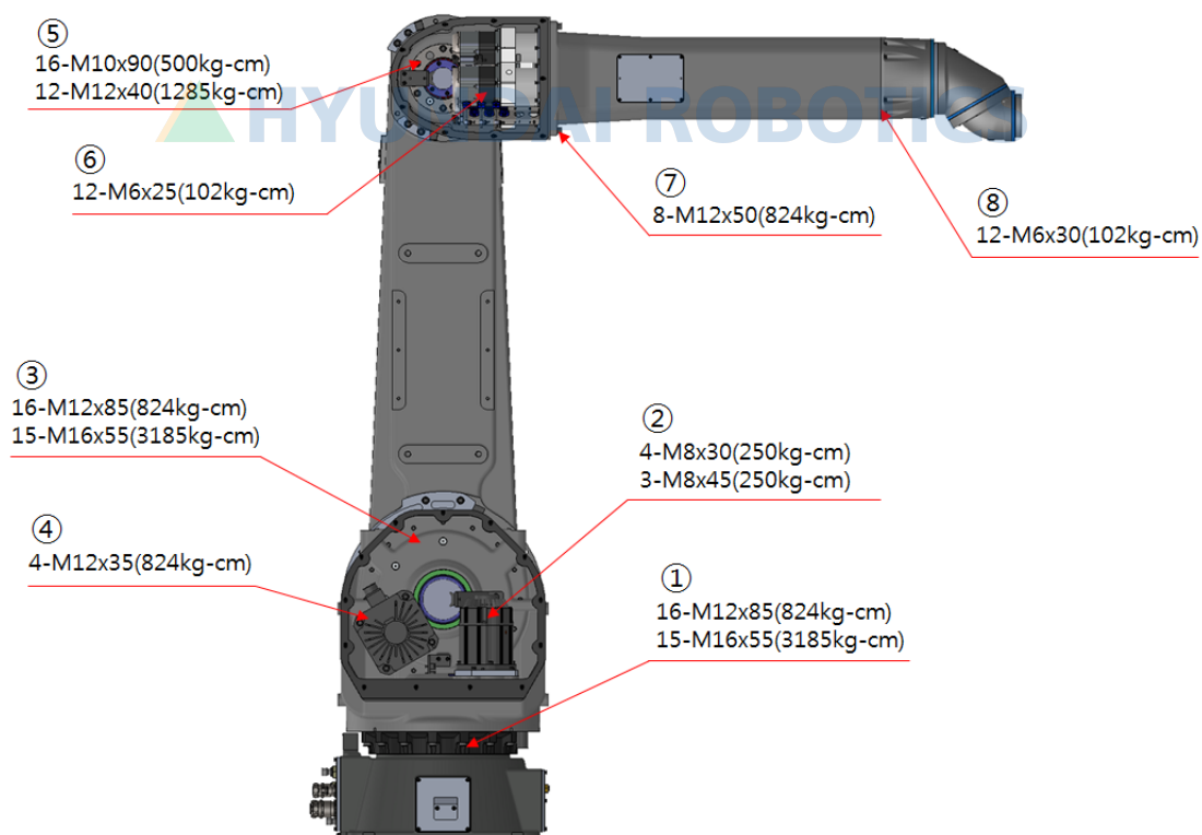
그림 4.1 주요 볼트 점검 부위
