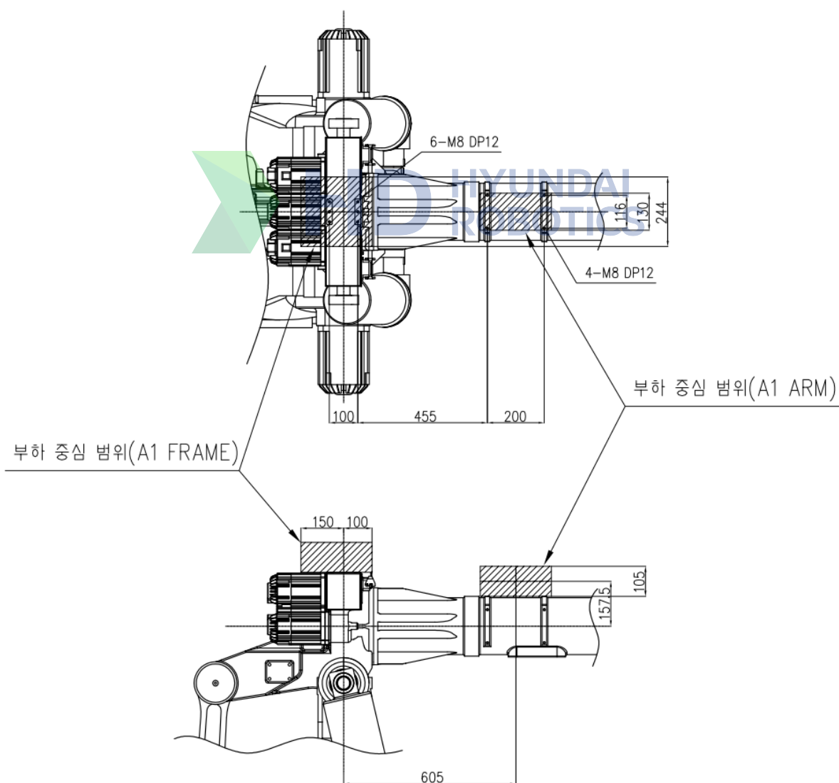
그림 2.6 제 1 암(Arm) 상부 부착부 상세도 : [HX500S]
