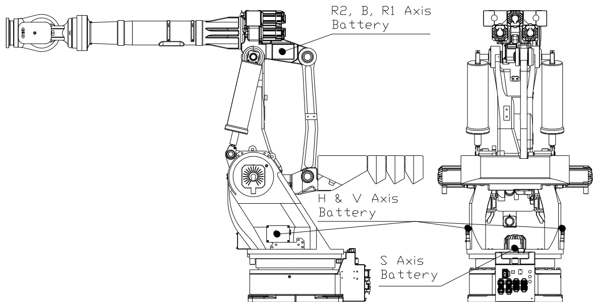
그림 5.1 배터리 교환 위치
