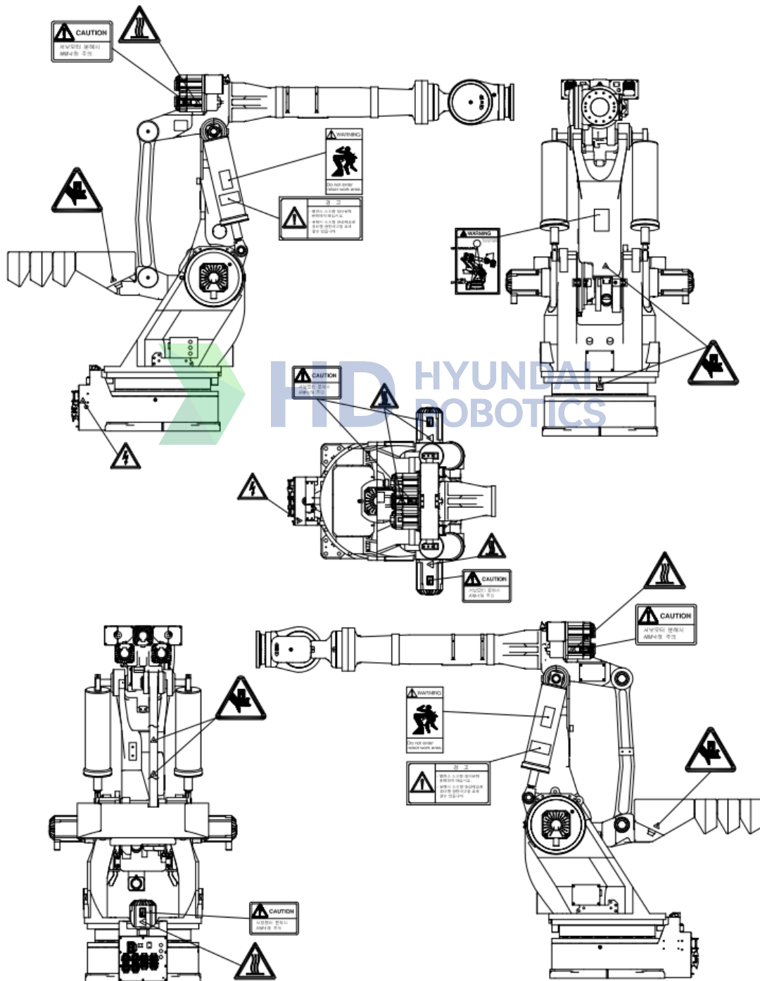
그림 3.2 안전 명판 위치
