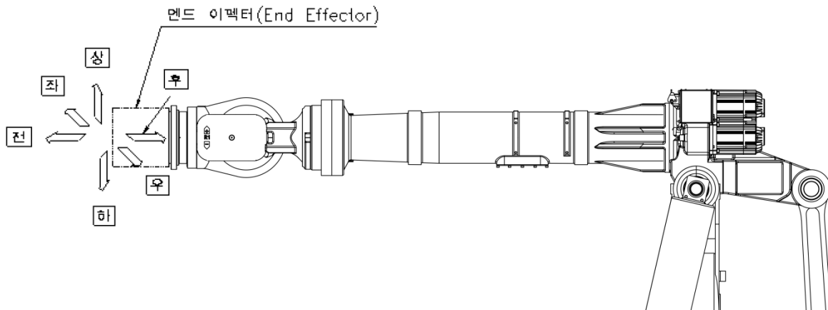
그림 4.2 유격 점검 방향 HD HYUNDAI ROBOTICS
