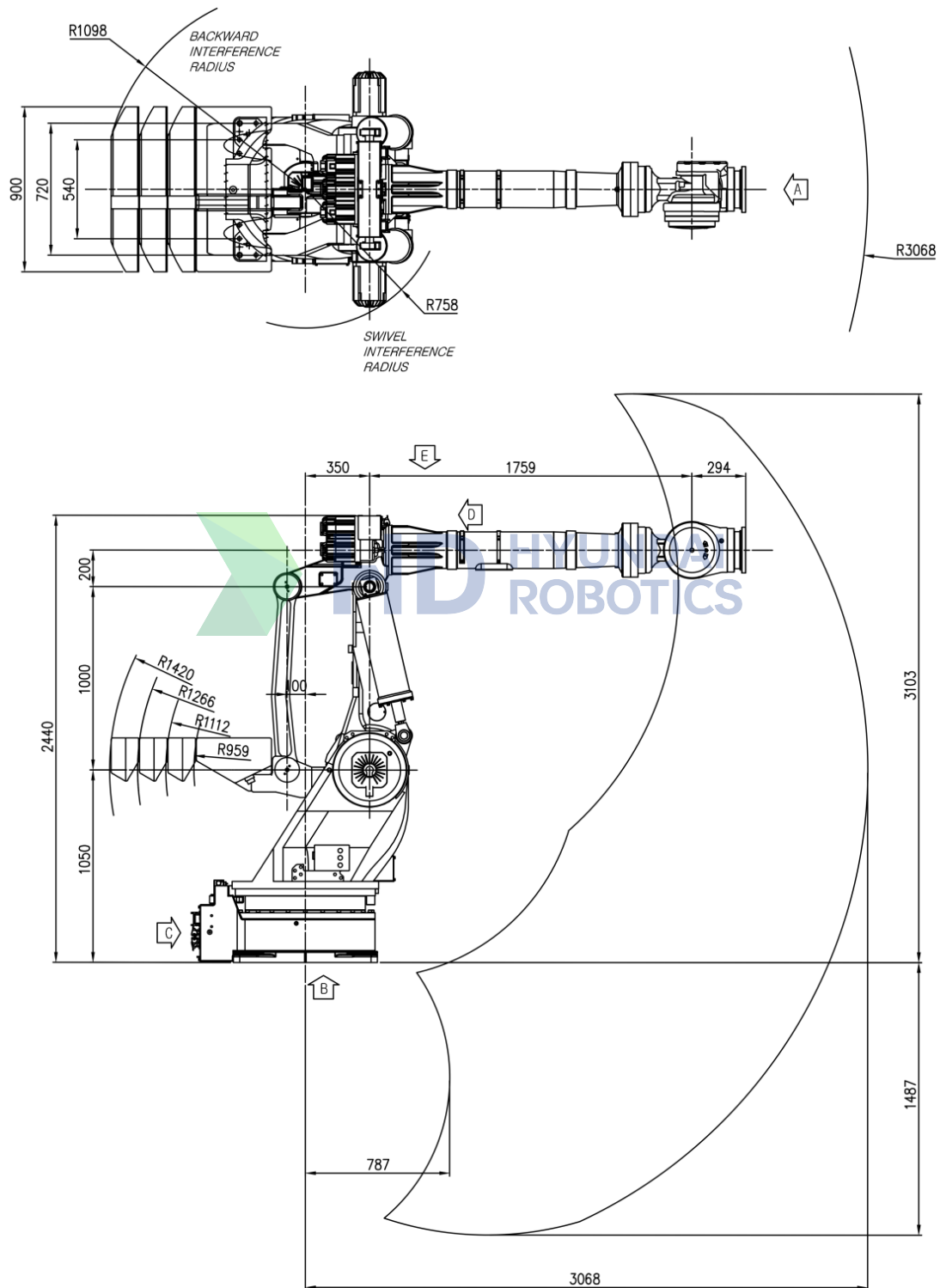
그림 2.3 로봇 본체 외형 치수 및 동작 영역 : [HX500S]
