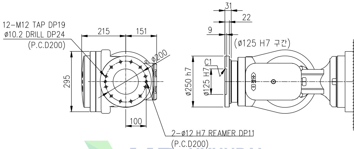
그림 2.5 손목축 취부면 상세도 : [HX500S]
