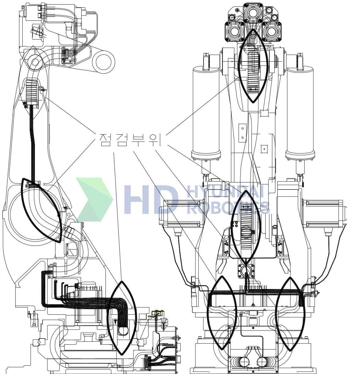
그림 4.3 케이블 점검 부위
