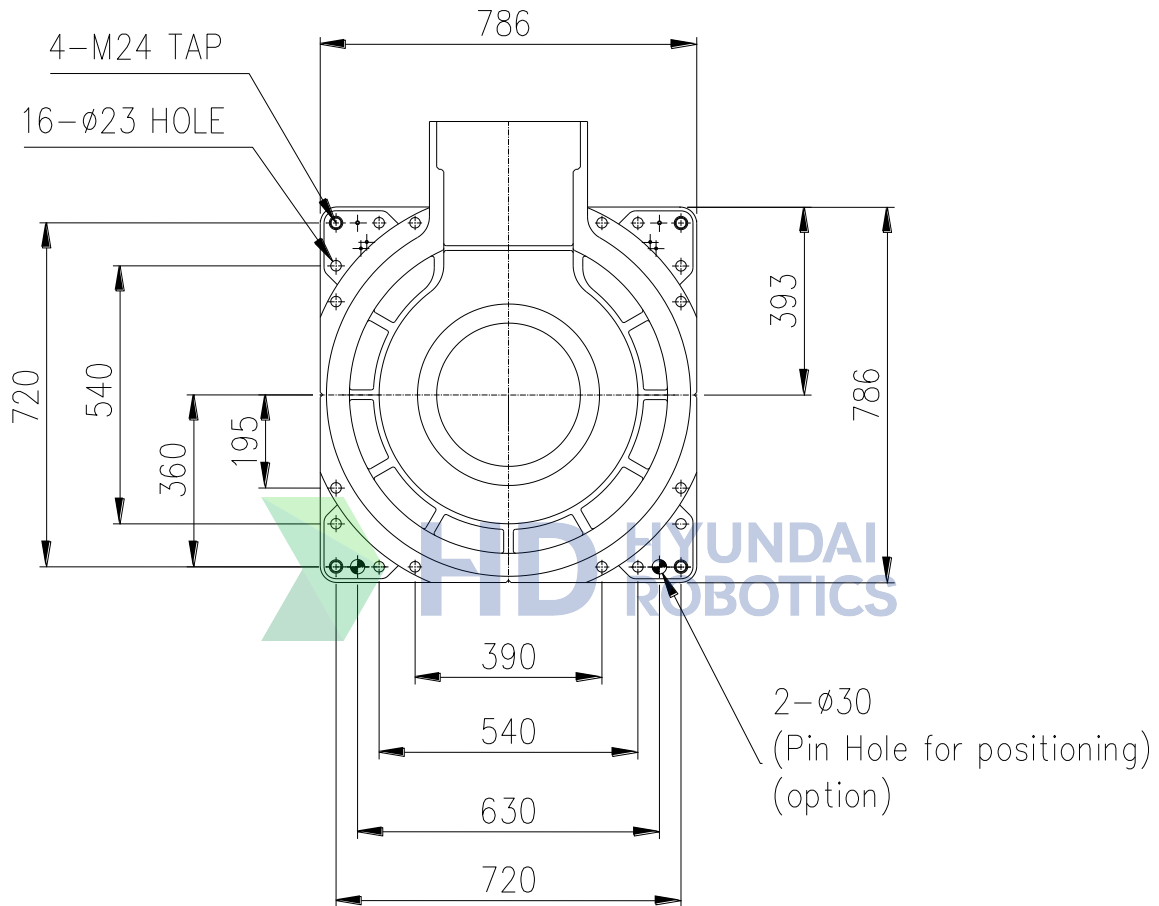
그림 3.6 로봇 본체 설치 치수
