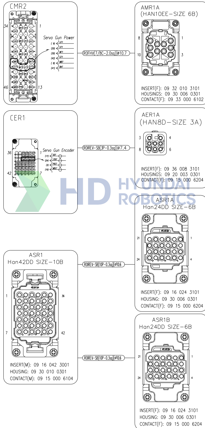
그림 2.8 어플리케이션 콘넥터 상세도
