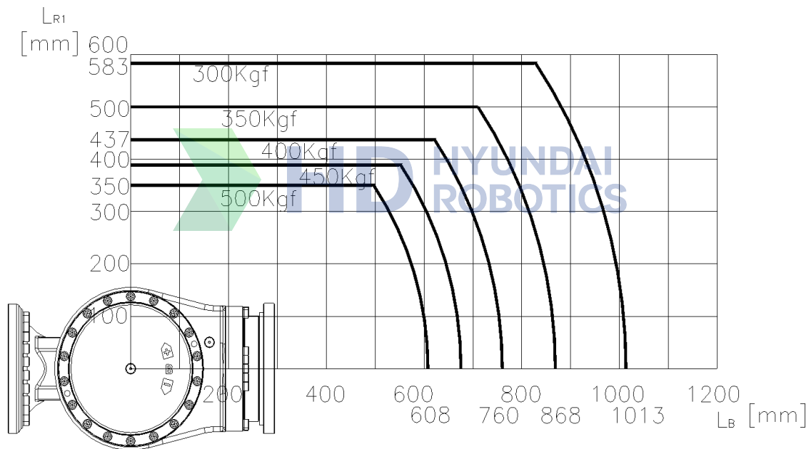
그림 3.7 손목축 토크 선도 [HX500S]
