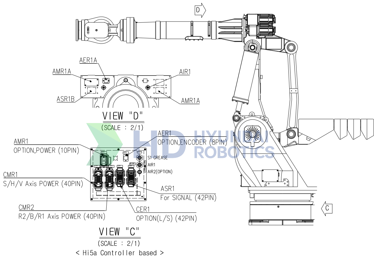
그림 2.7 어플리케이션용 배선 및 배관도: [HX500S]
