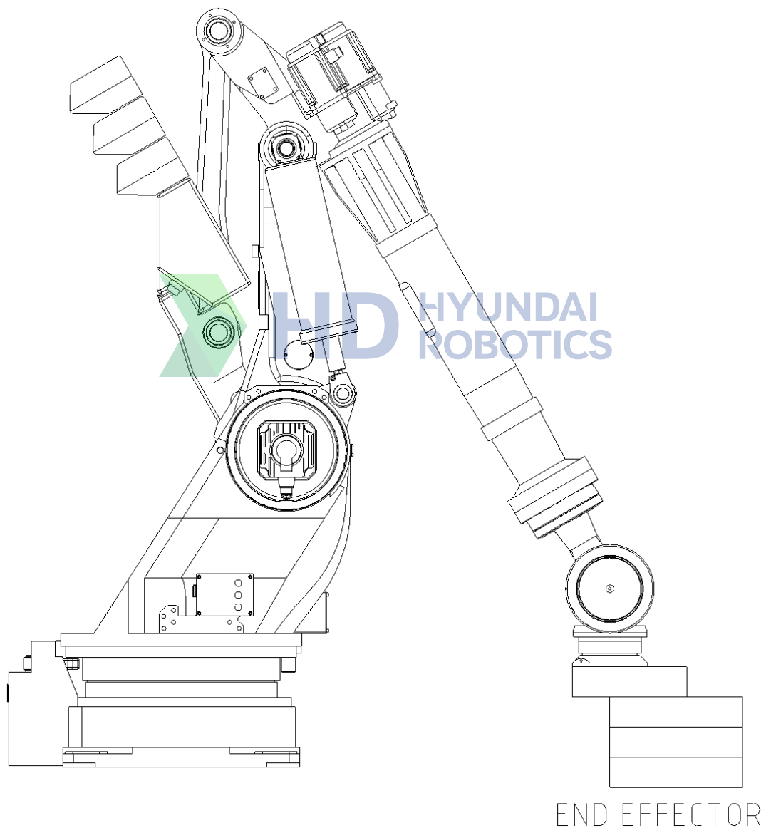
그림 3.8 권장 대기 자세
