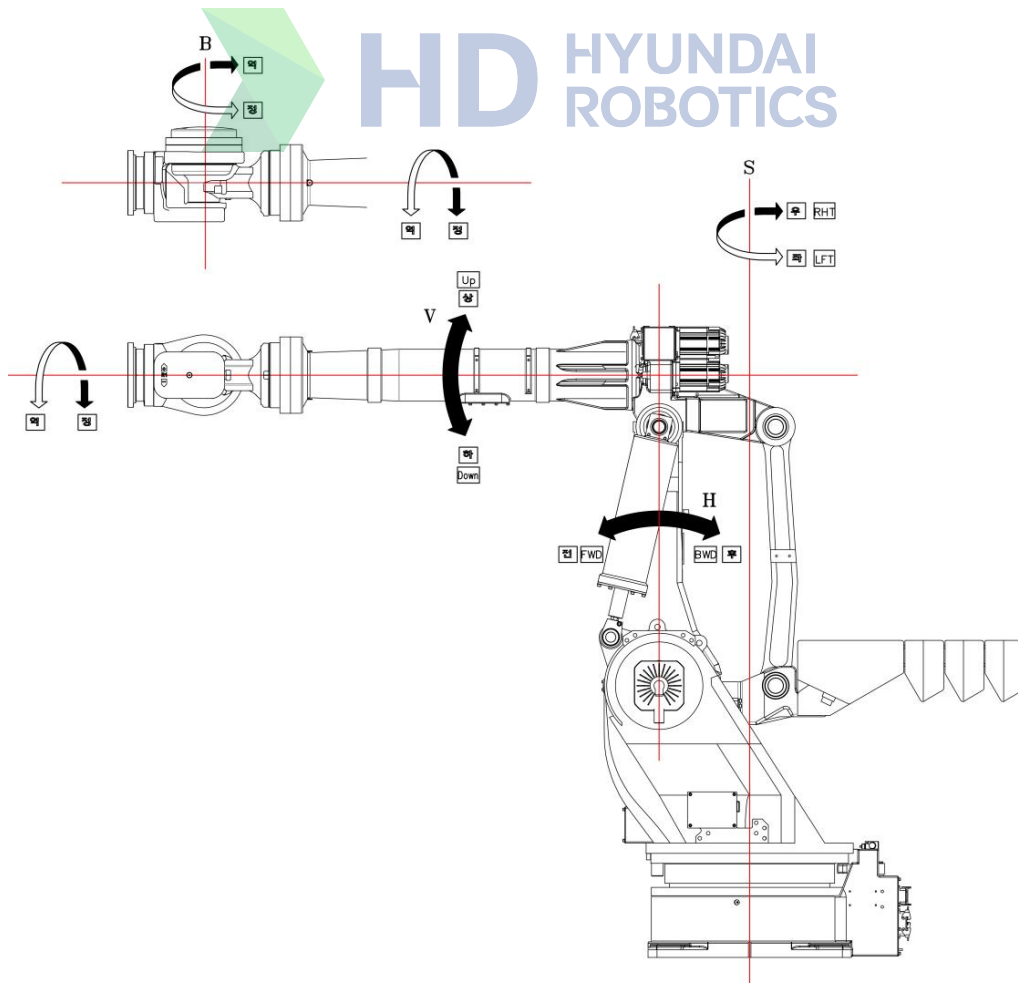
그림 2.4 본체 외관 및 동작 축 [HX500S]
