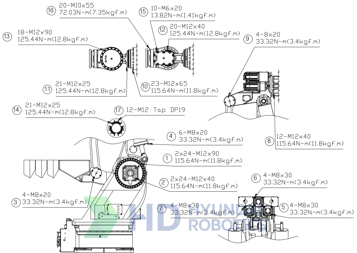
그림 4.1 주요 볼트 점검 부위 [HX500S]
