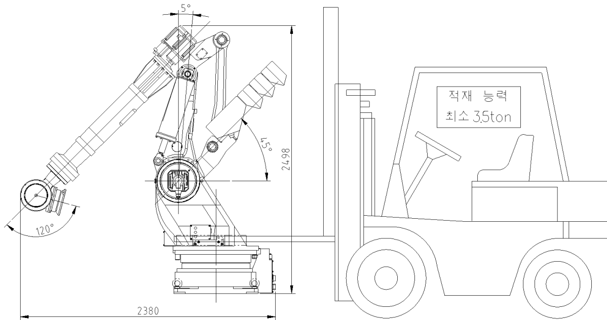
그림 3.4 운송 방법 : 지게차 이용[HX500S]
