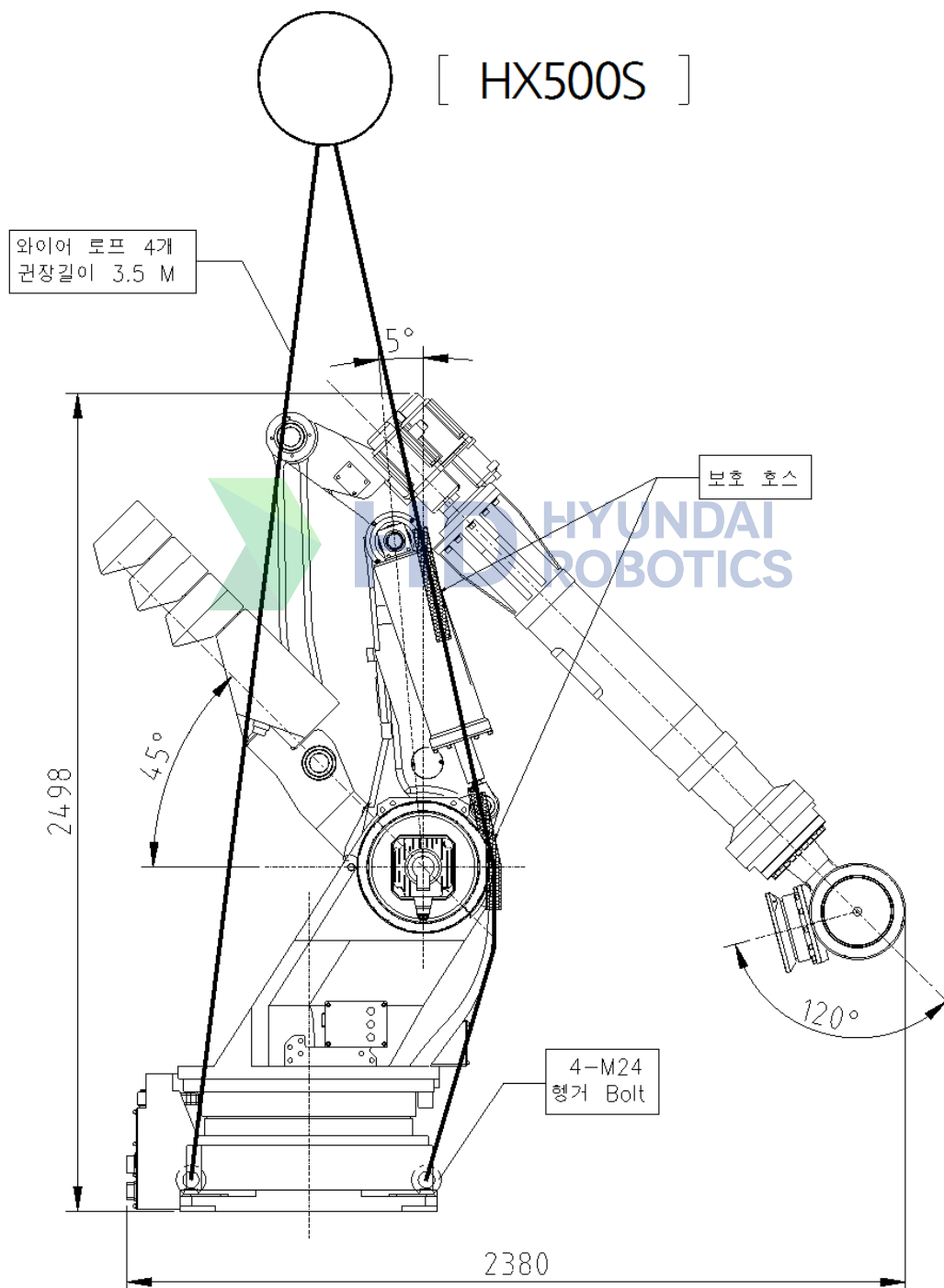
그림 3.3 운송 방법 : 크레인 이용 [HX500S]
