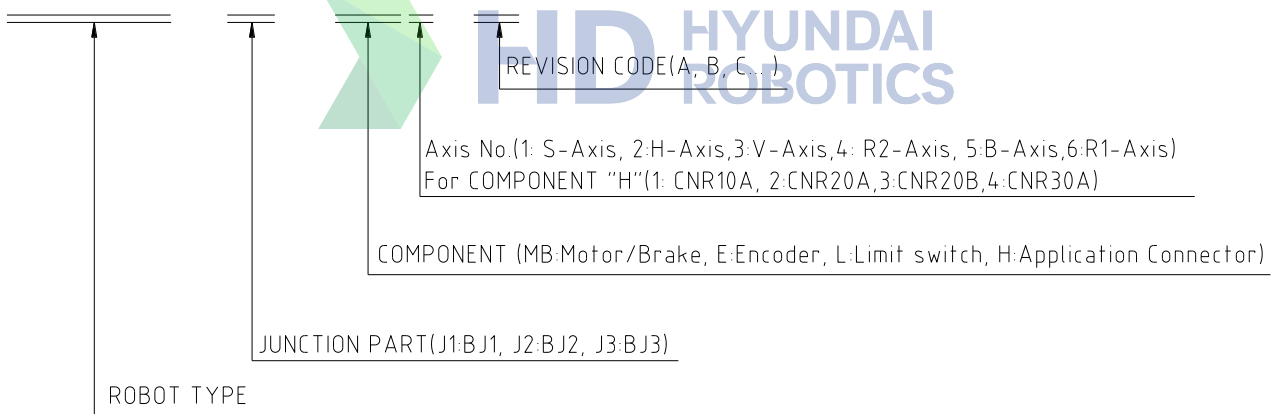
그림 5.2 본체 내 배선 기호 설명
