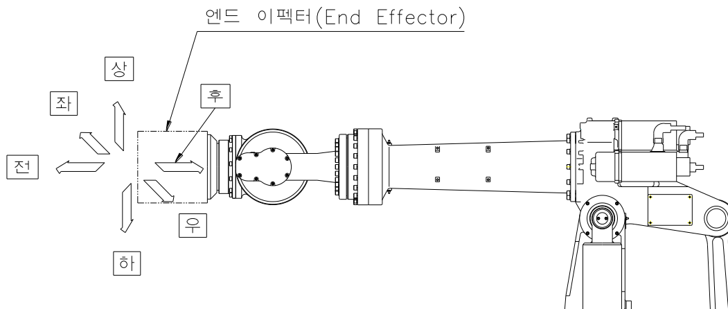
그림 4.2 유격 점검 방향
