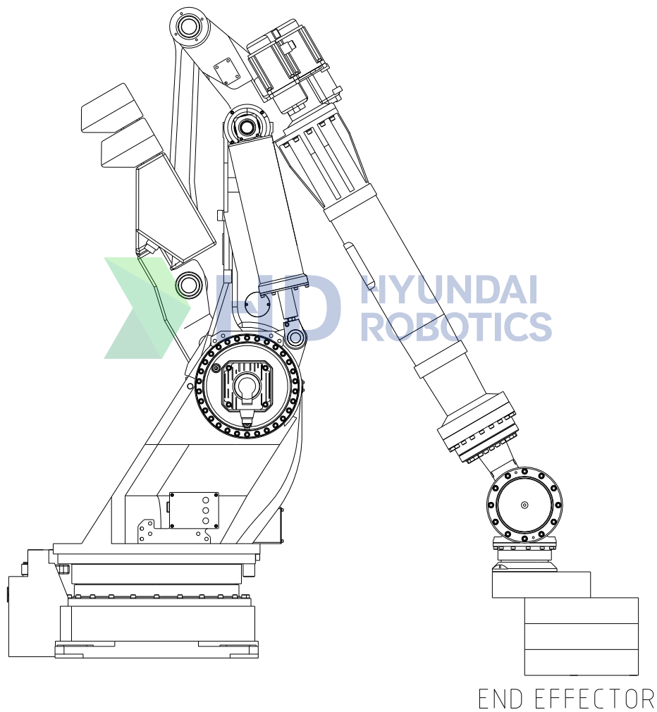
그림 3.10 권장 대기 자세
