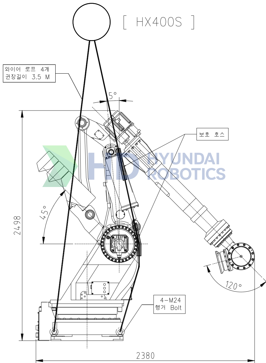
그림 3.3 운송 방법 : 크레인 이용 [HX400S]
