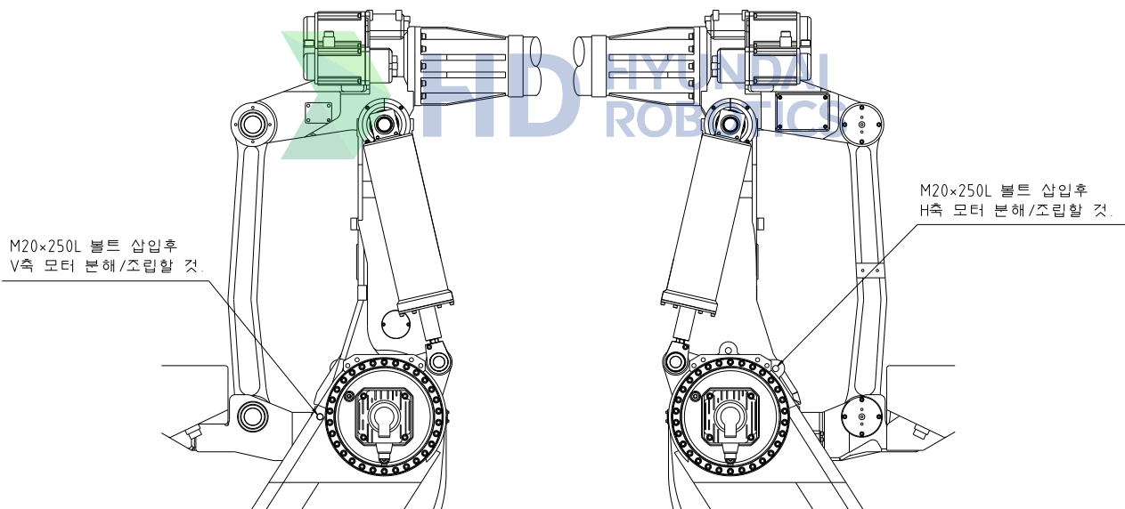
그림 6.1 H, V 축 암(Arm) 낙하 방지 방법
