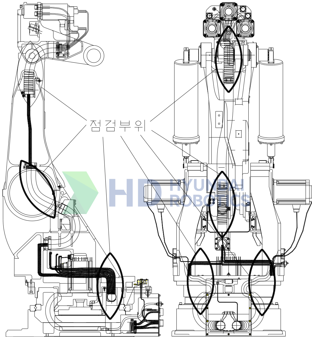
그림 4.3 케이블 점검 부위
