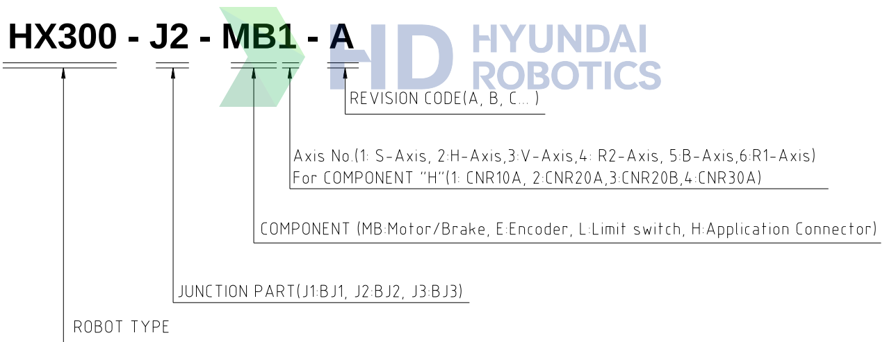
그림 5.2 본체 내 배선 기호 설명
