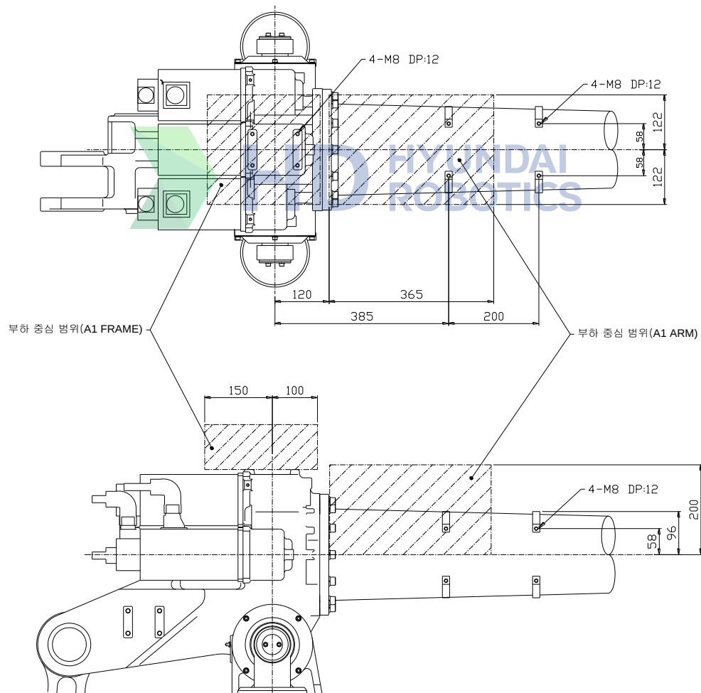
그림 2.6 제 1 암(Arm) 상부 부착부 상세도 : [HX400S]
