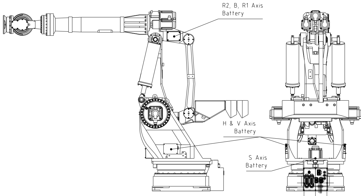
그림 5.1 배터리 교환 위치
