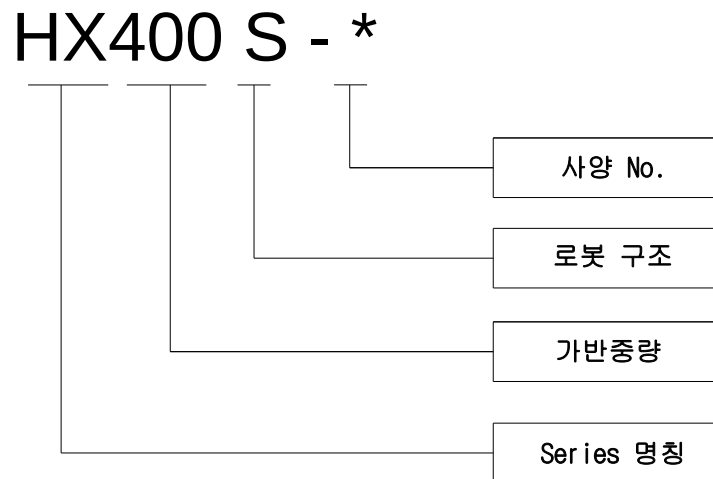
그림 2.1 로봇 기구부 형식
