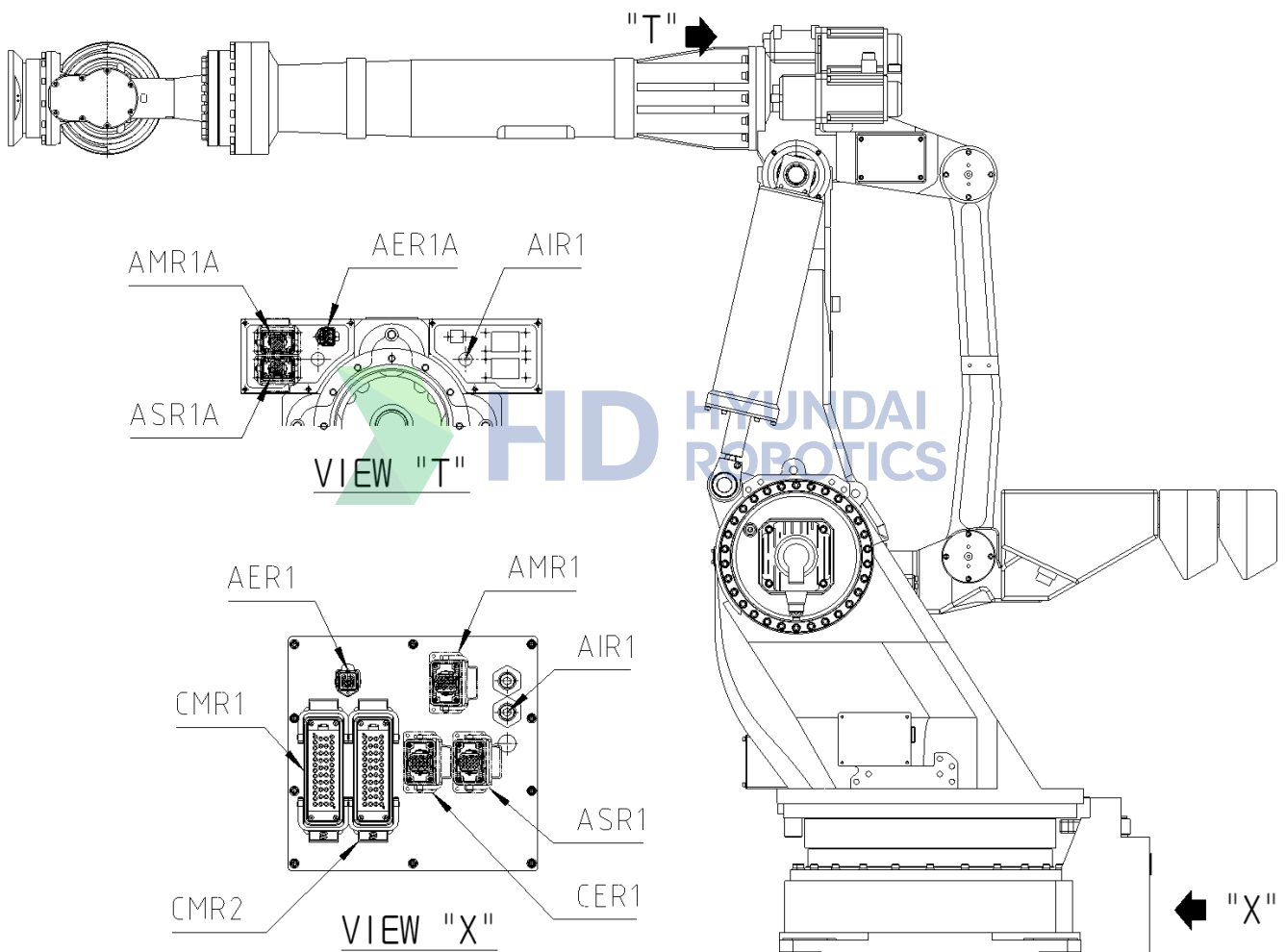
그림 2.7 어플리케이션용 배선 및 배관도: [HX400S]
