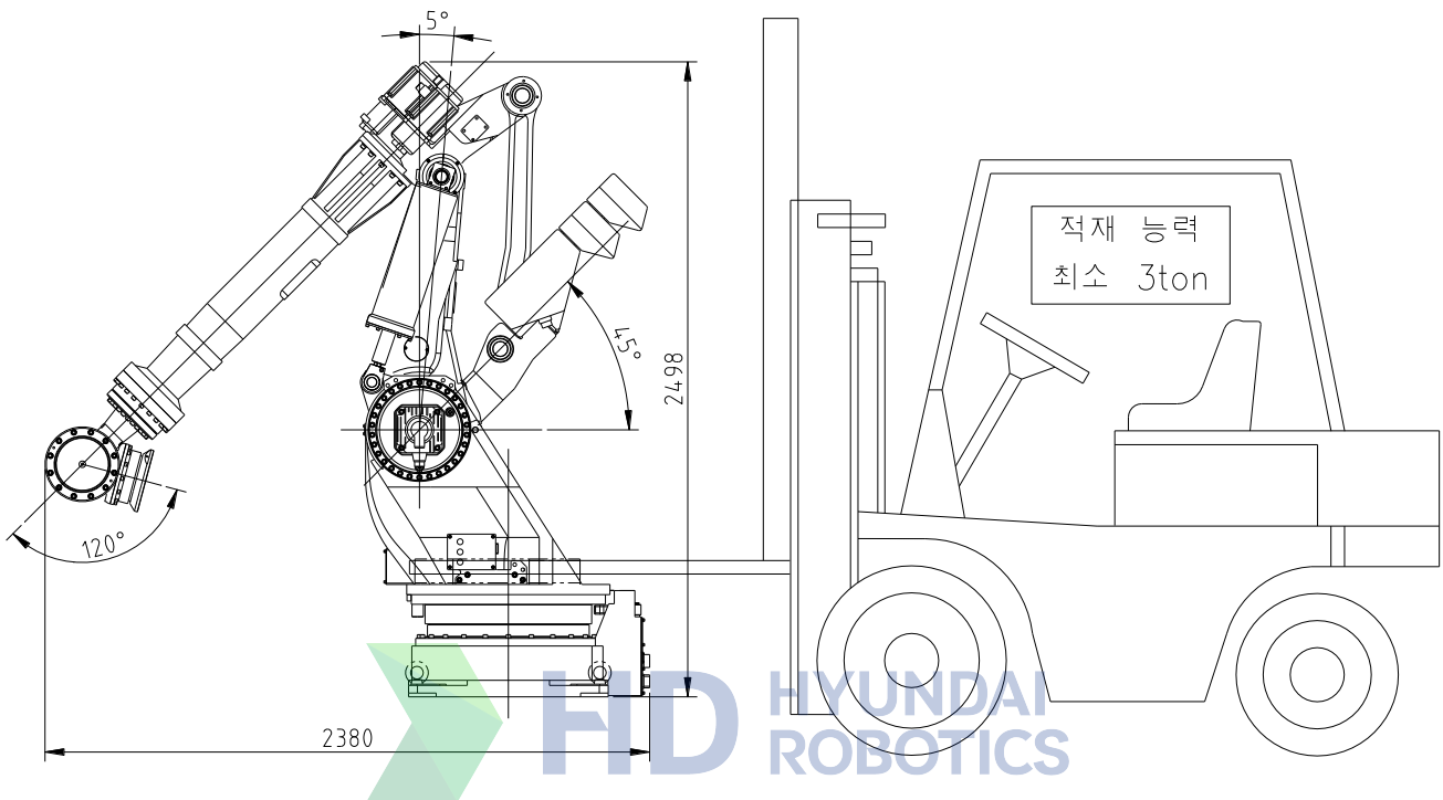
그림 3.4 운송 방법 : 지게차 이용
