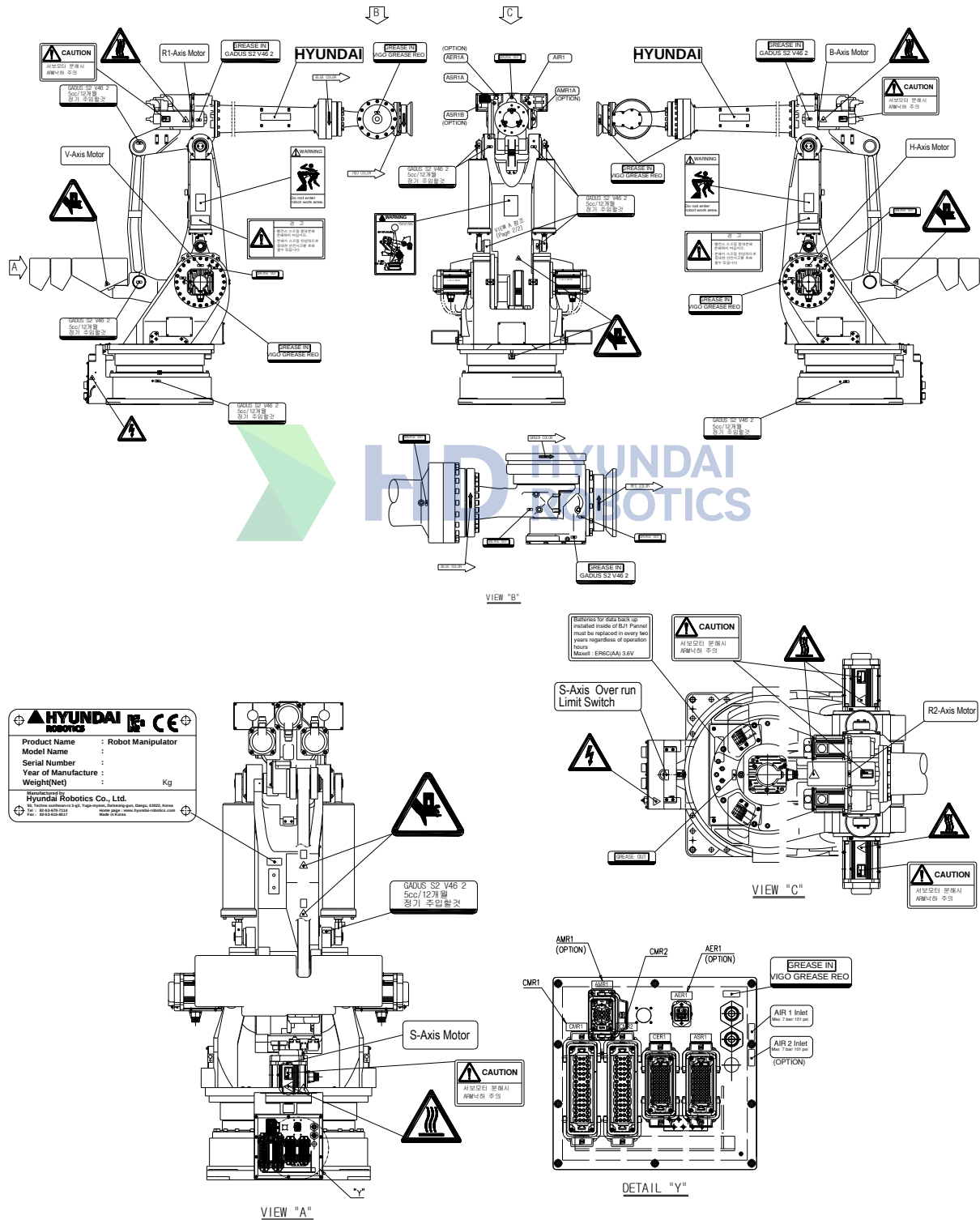
그림 3.2 안전 명판 위치
