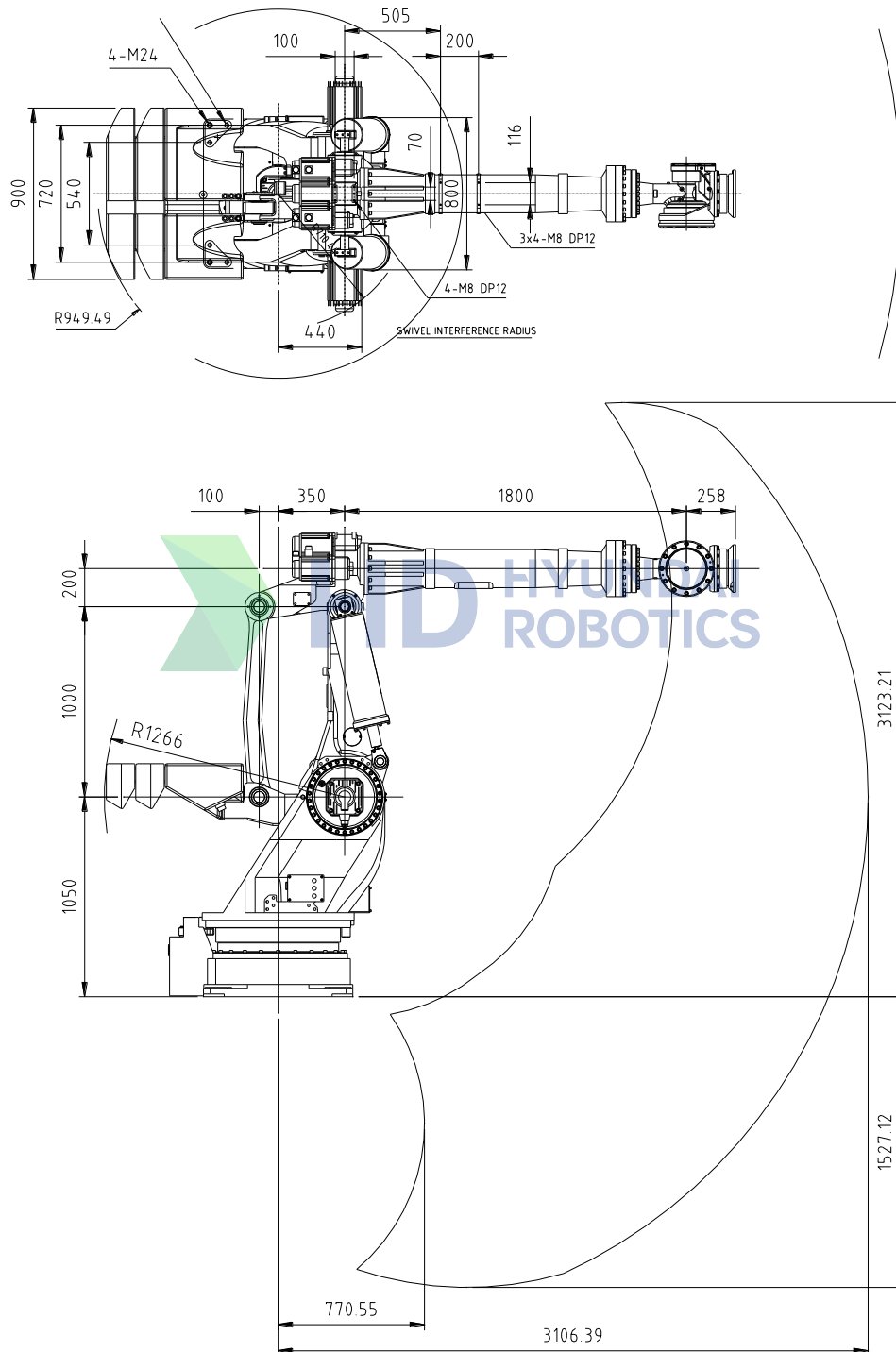
그림 2.3 로봇 본체 외형 치수 및 동작 영역 : [HX400S]
