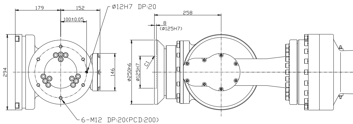
그림 2.5 손목축 취부면 상세도 : [HX400S]
