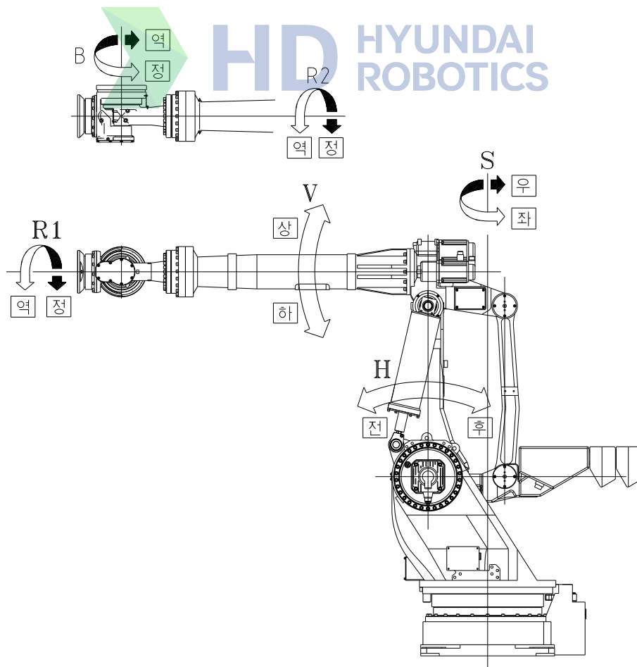
그림 2.4 본체 외관 및 동작 축 [HX400S]
