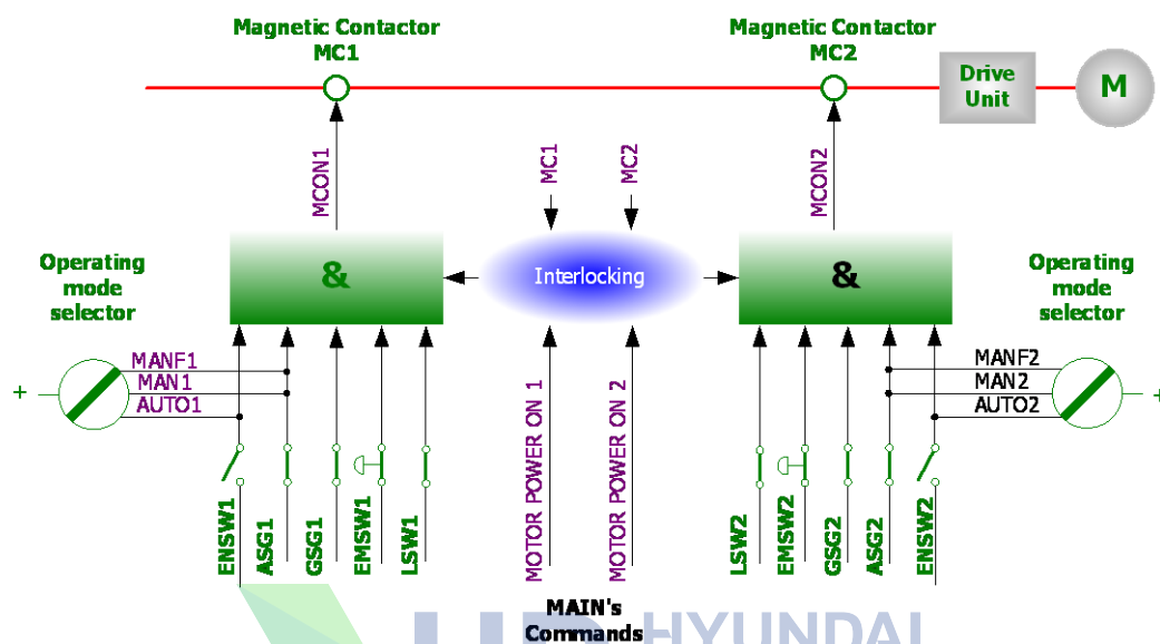
그림 1.5 안전체인 구성도
