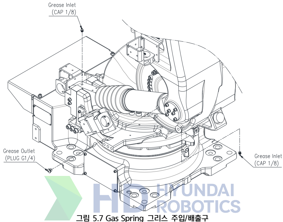
그림 5.7 Gas Spring 그리스 주입/배출구
