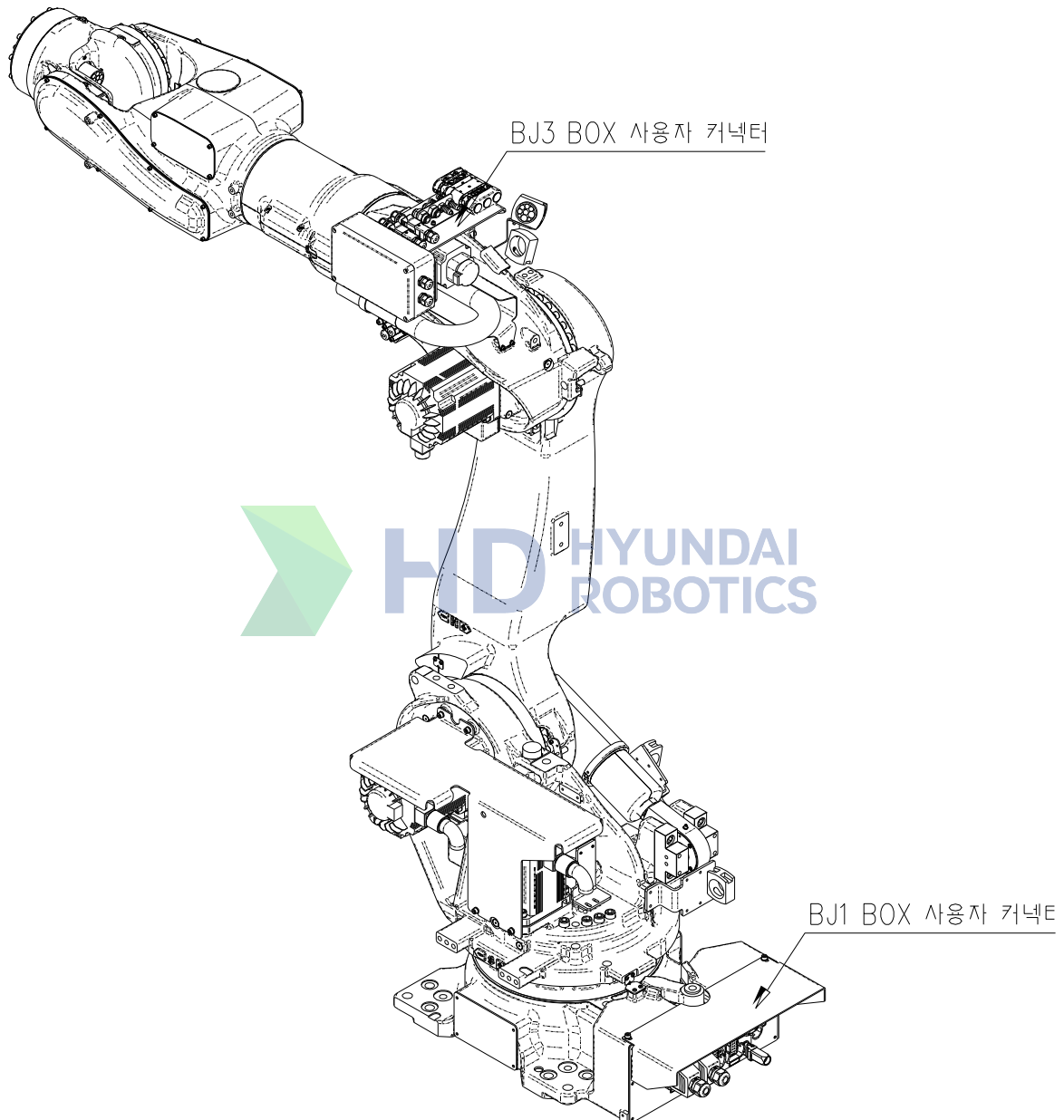
그림 10.1 본체 부품 배치
