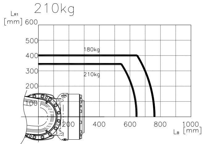
그림 3.8 손목축 토크 선도
