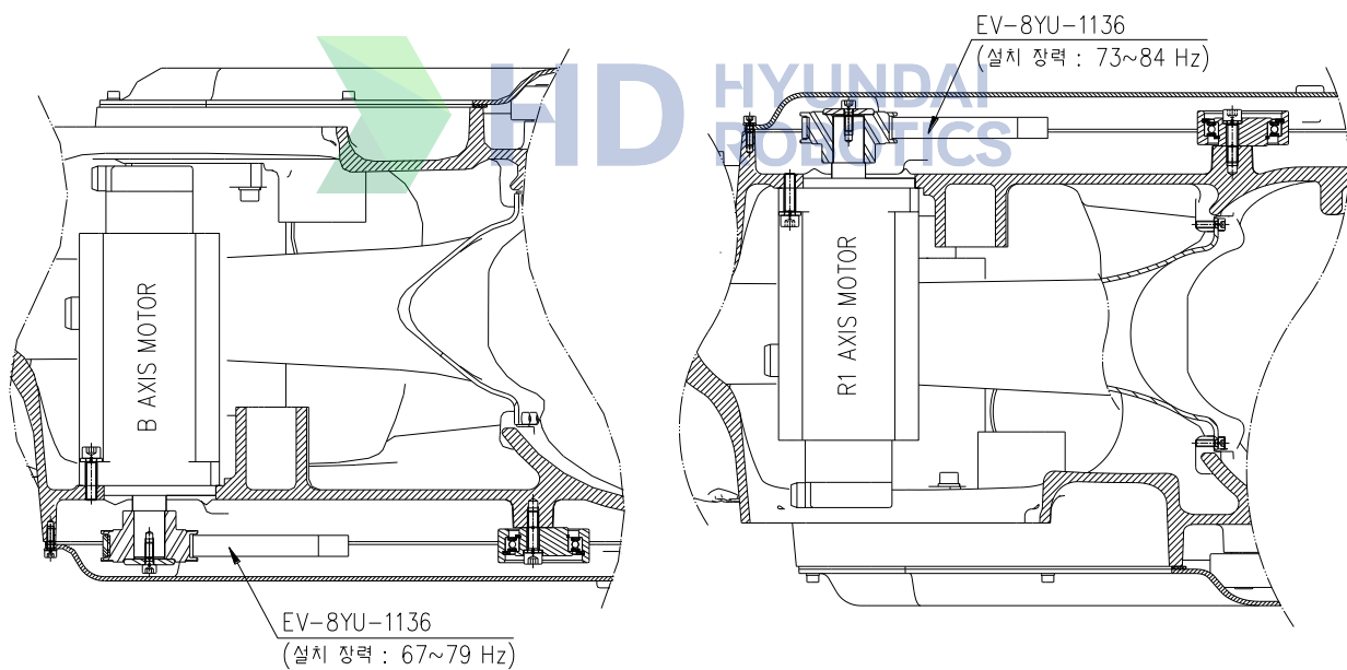
그림 4.2 타이밍 벨트 장력 체크 부위
