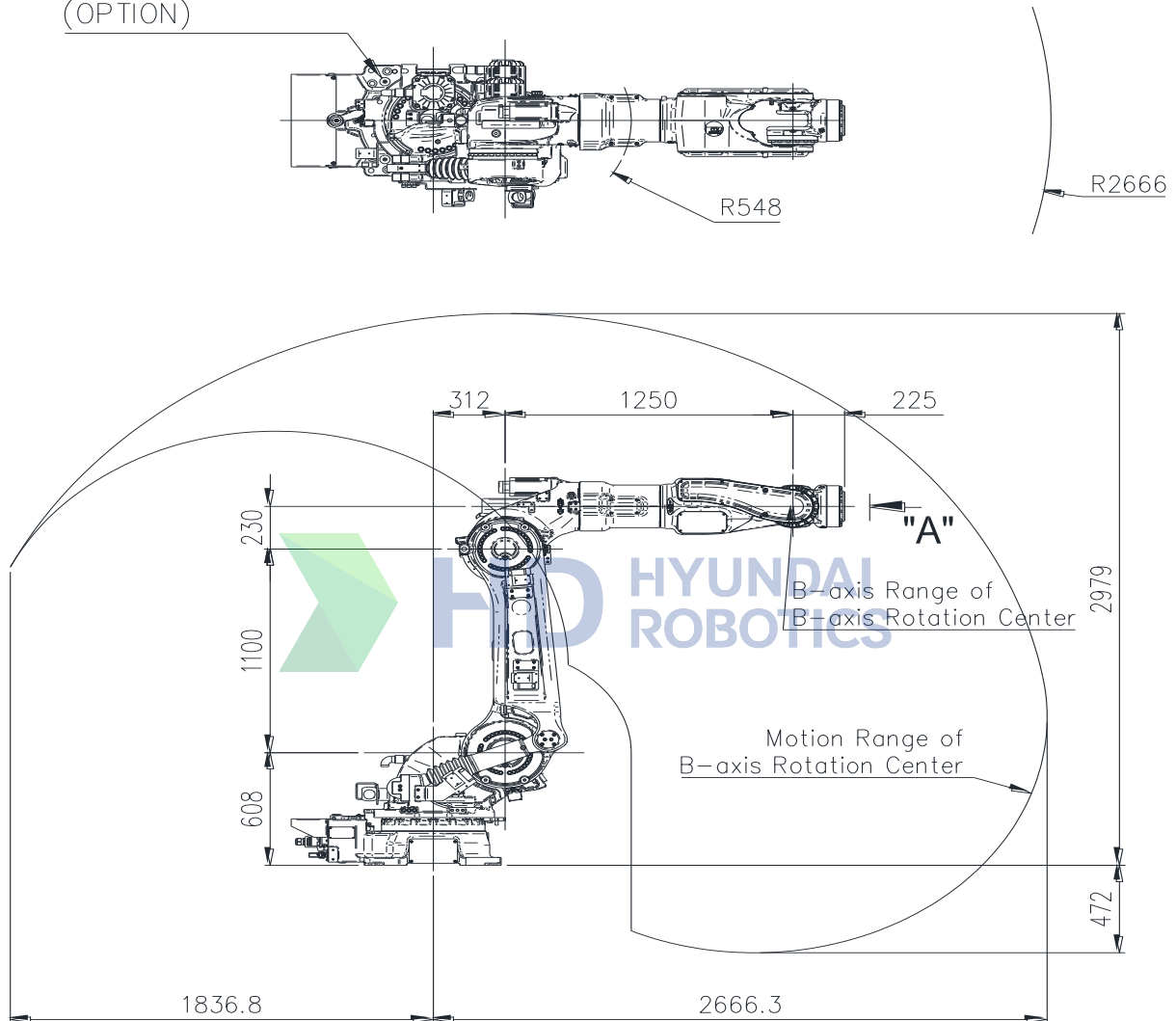
그림 2.3 로봇 본체 외형 치수 및 동작 영역
