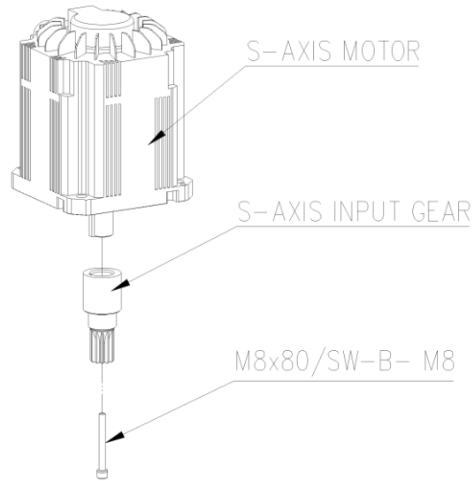
그림 6.3 H&V 축 모터 ASSEMBLY
