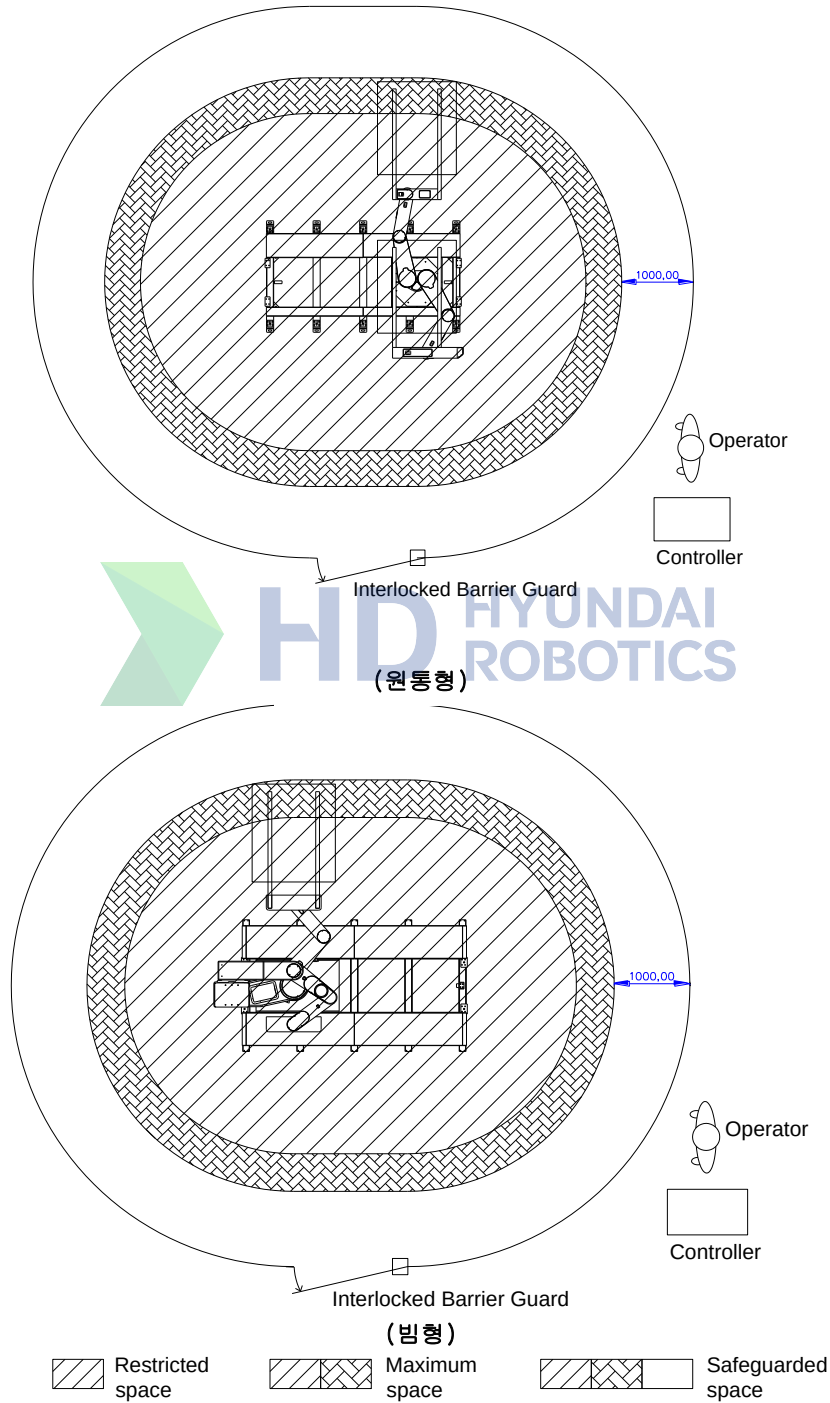
그림 1.3 LCD 용 로봇 주변장치와 작업자의 배치
