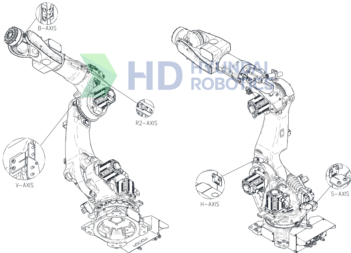
그림 6.6 원점 설정 방법 (HS210E)
