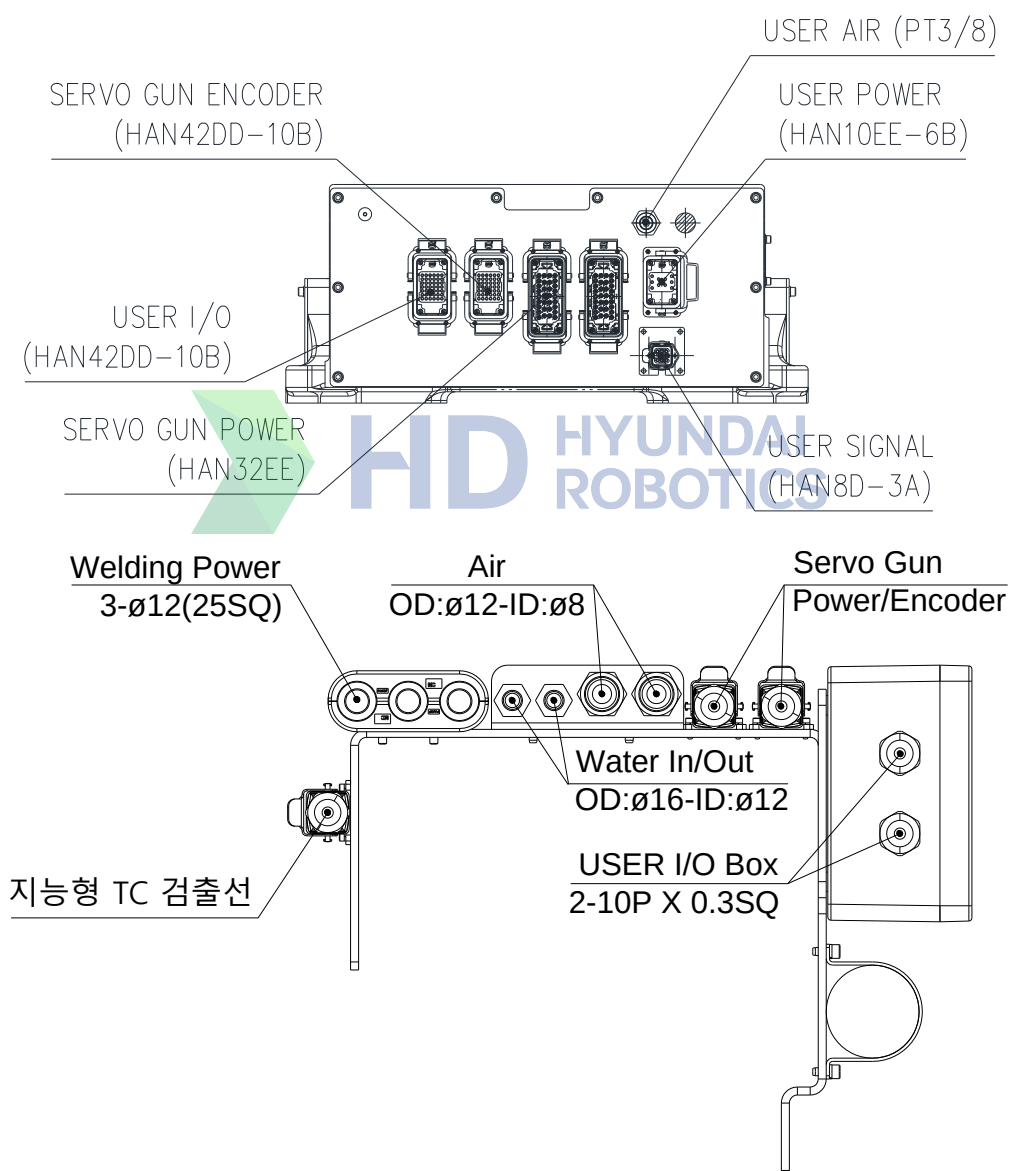
그림 2.6 어플리케이션용 배선 및 배관도
