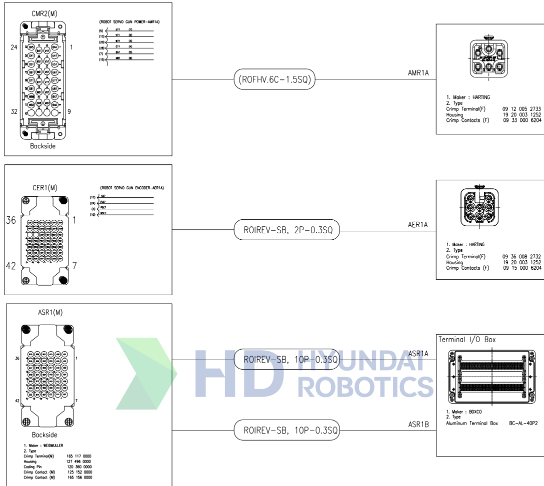
그림 2.7 어플리케이션 커넥터 상세
