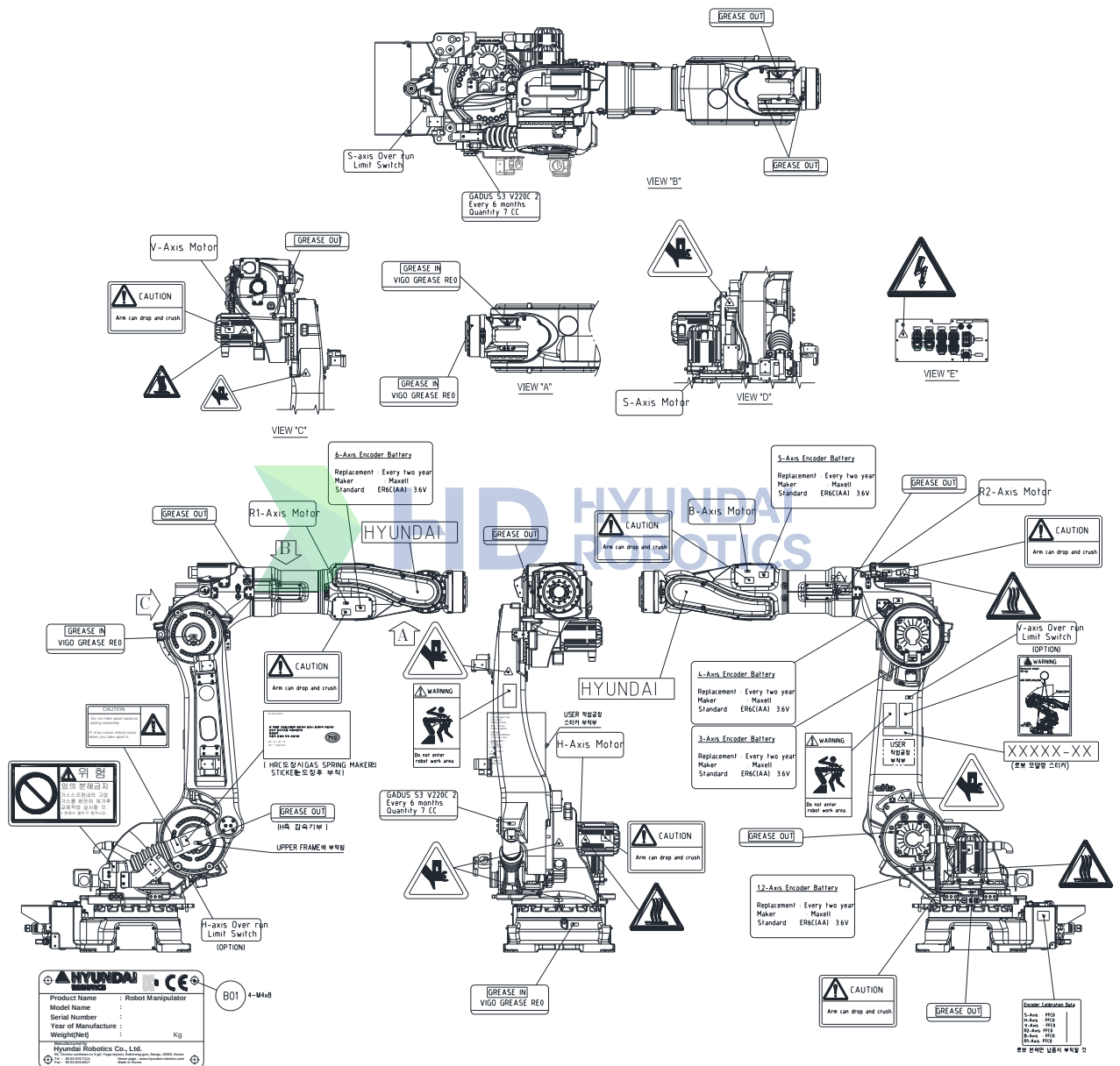
그림 3.2 안전 명판 위치 (HS210E)
