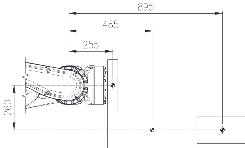
그림 3.10 3 차원 부하 모델 2D 형상 (HS210E)
