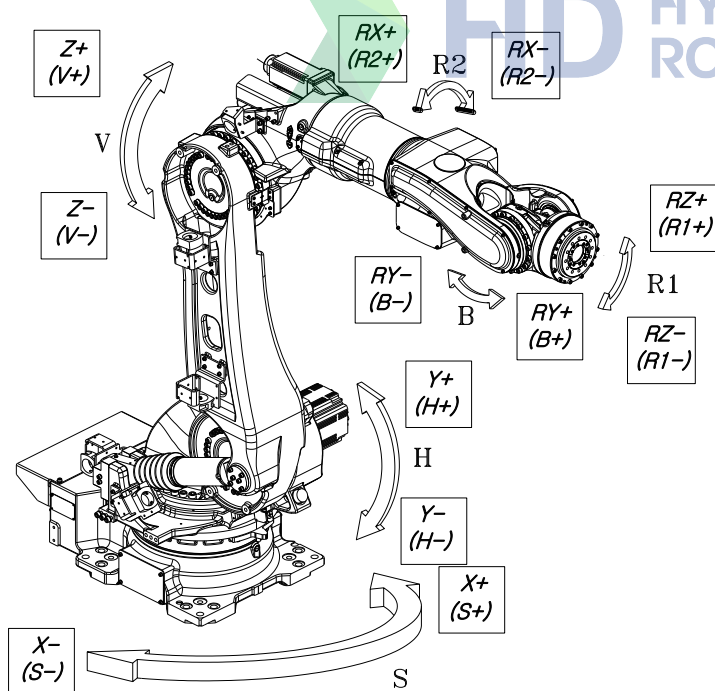
그림 2.4 본체 외관 및 동작 축
