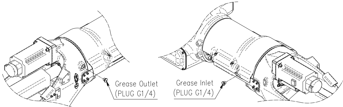
그림 5.4 R2 축 감속기 그리스 주입/배출구
