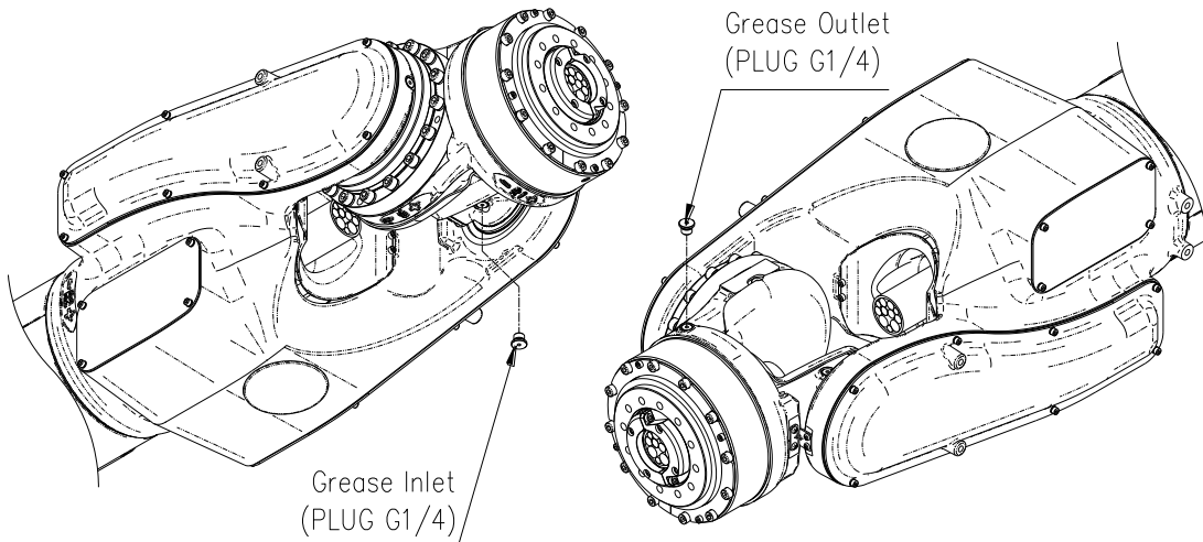
그림 5.6 R1 축 감속기 그리스 주입/배출구
