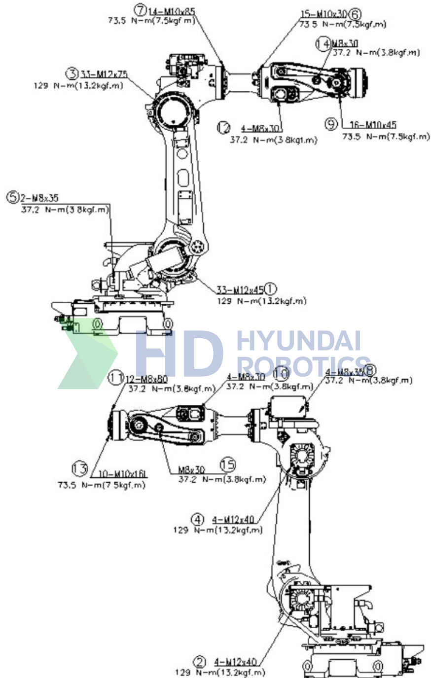
그림 4.1 주요 볼트 점검 부위
