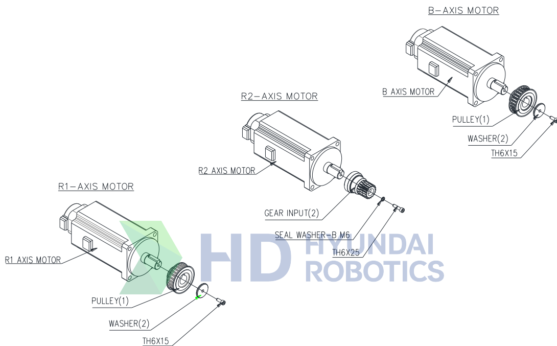
그림 6.5 손목축 모터 ASSEMBLY
