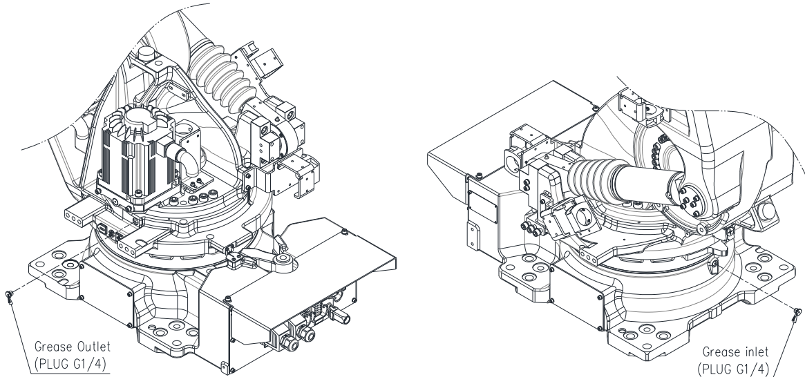
그림 5.1 S 축 감속기 그리스 주입/배출구
