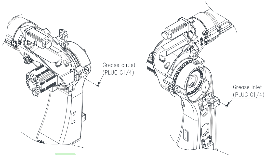
그림 5.3 V 축 감속기 그리스 주입/배출구
