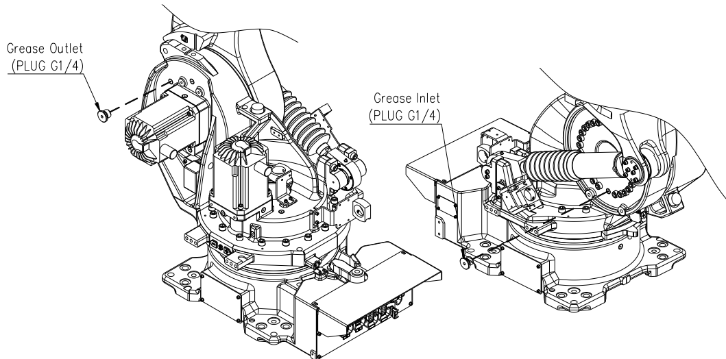
그림 5.2 H 축 감속기 그리스 주입/배출구
