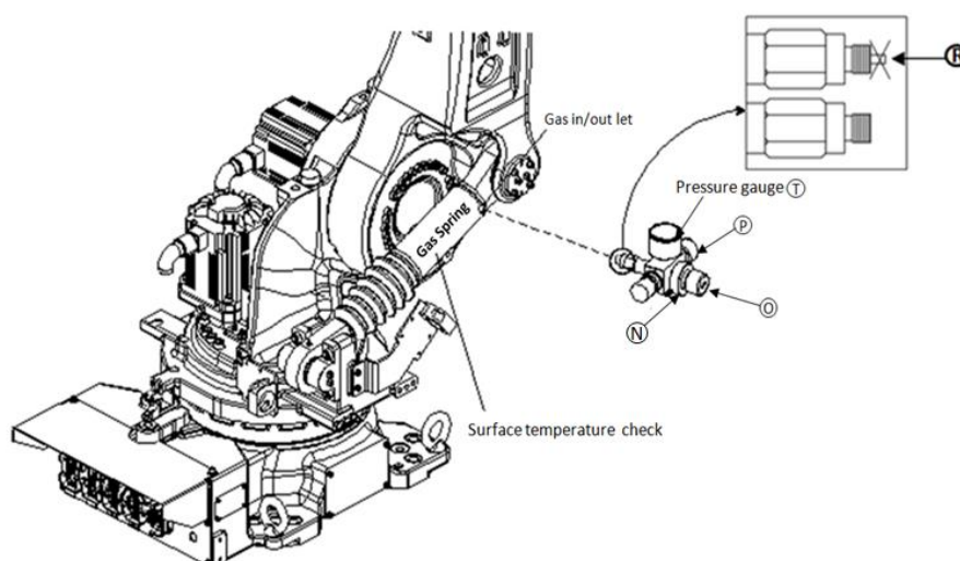
그림 9.4 가스 스프링의 Gas 배출
