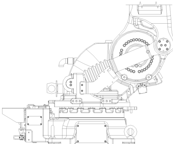
그림 9.6 가스 스프링 조립 자세
