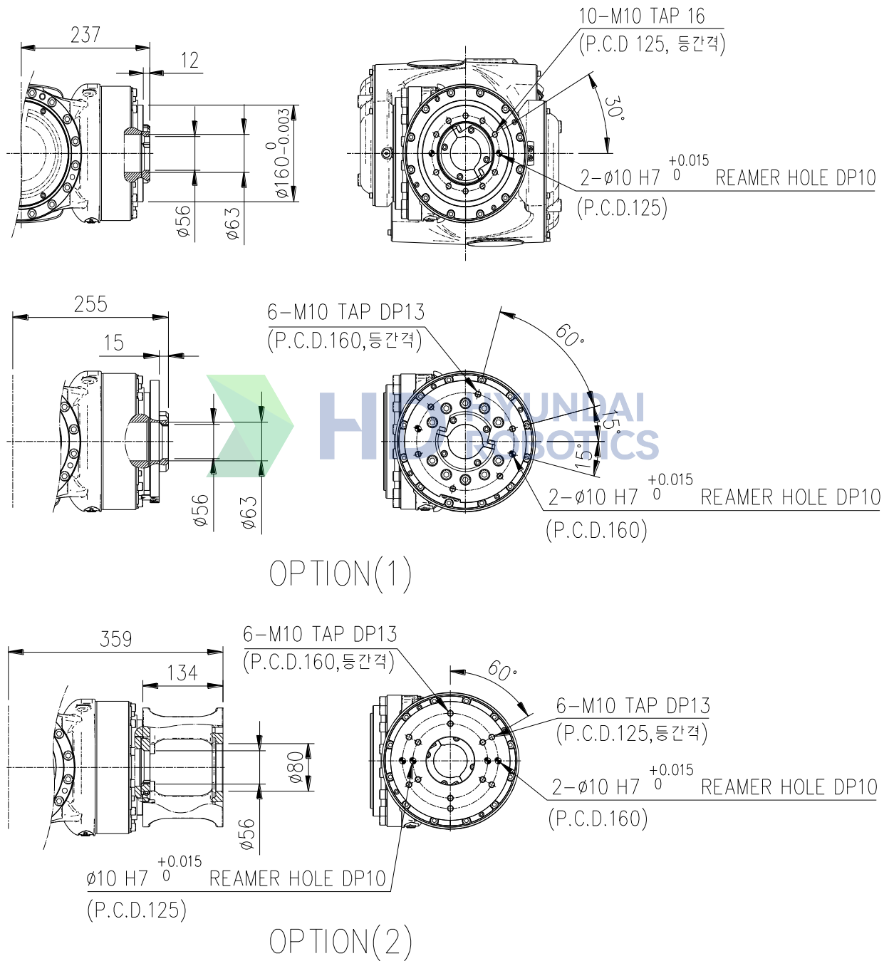
그림 2.5 손목축 취부면 상세도
