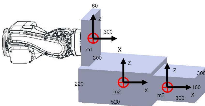
그림 3.11 3 차원 부하 모델 3D 형상
