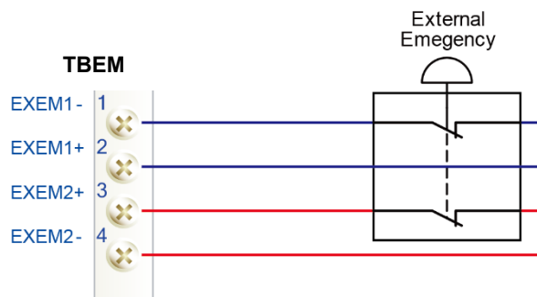
그림 1.6 시스템보드 터미널블록 TBEM 를 통한 외부비상정지스위치의 연결
