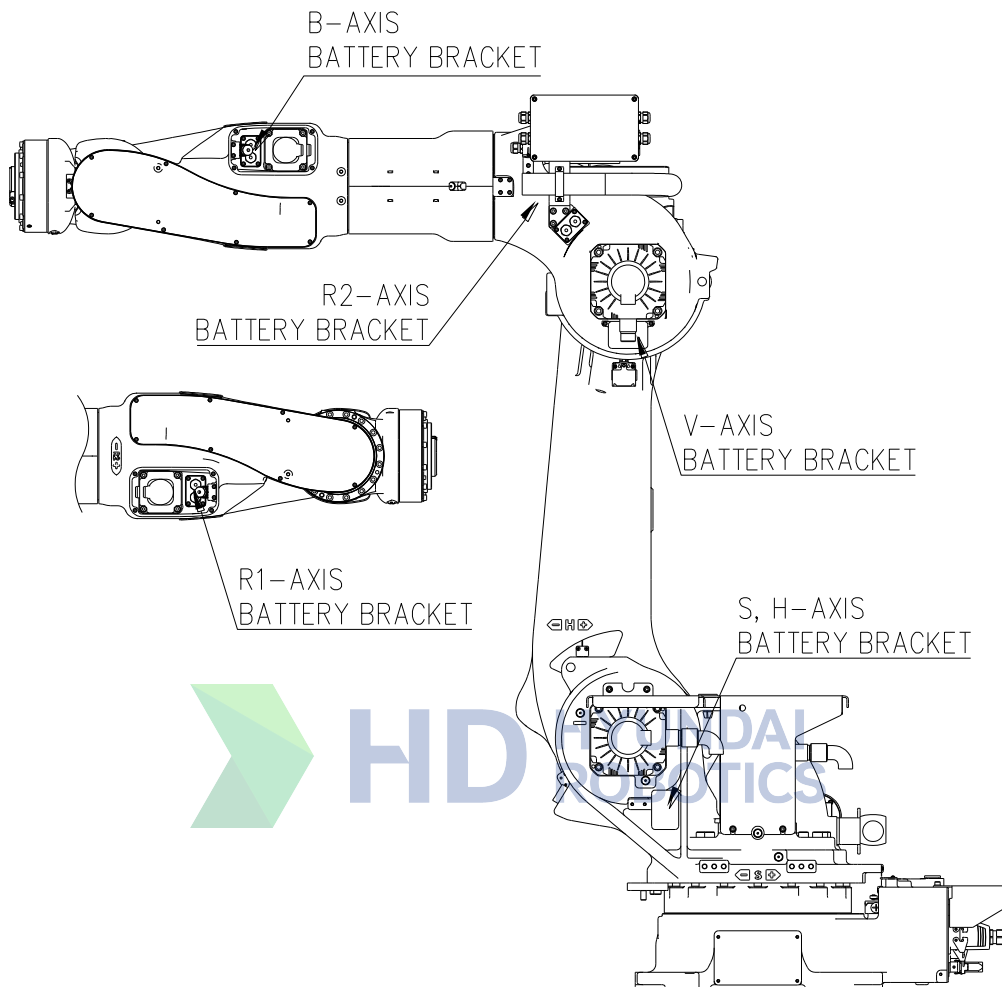
그림 5.8 배터리 교환 위치
