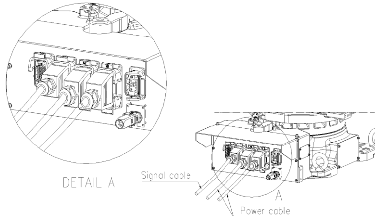
그림 3.7 로봇 Cable 연결 (HS210E)
