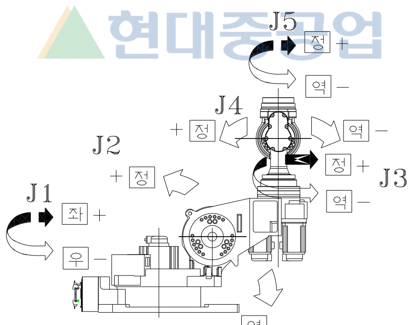
그림 2.4 본체 외관 및 동작 축
