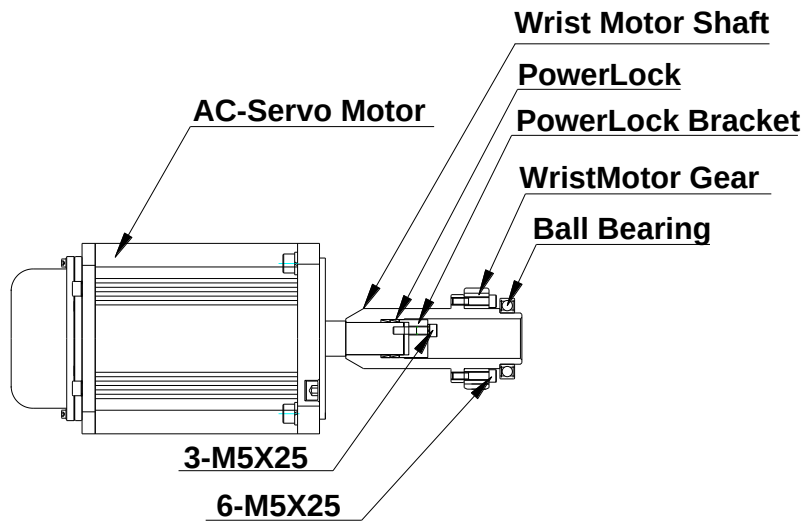
그림 6.4 손목 축 모터 ASSEMBLY
