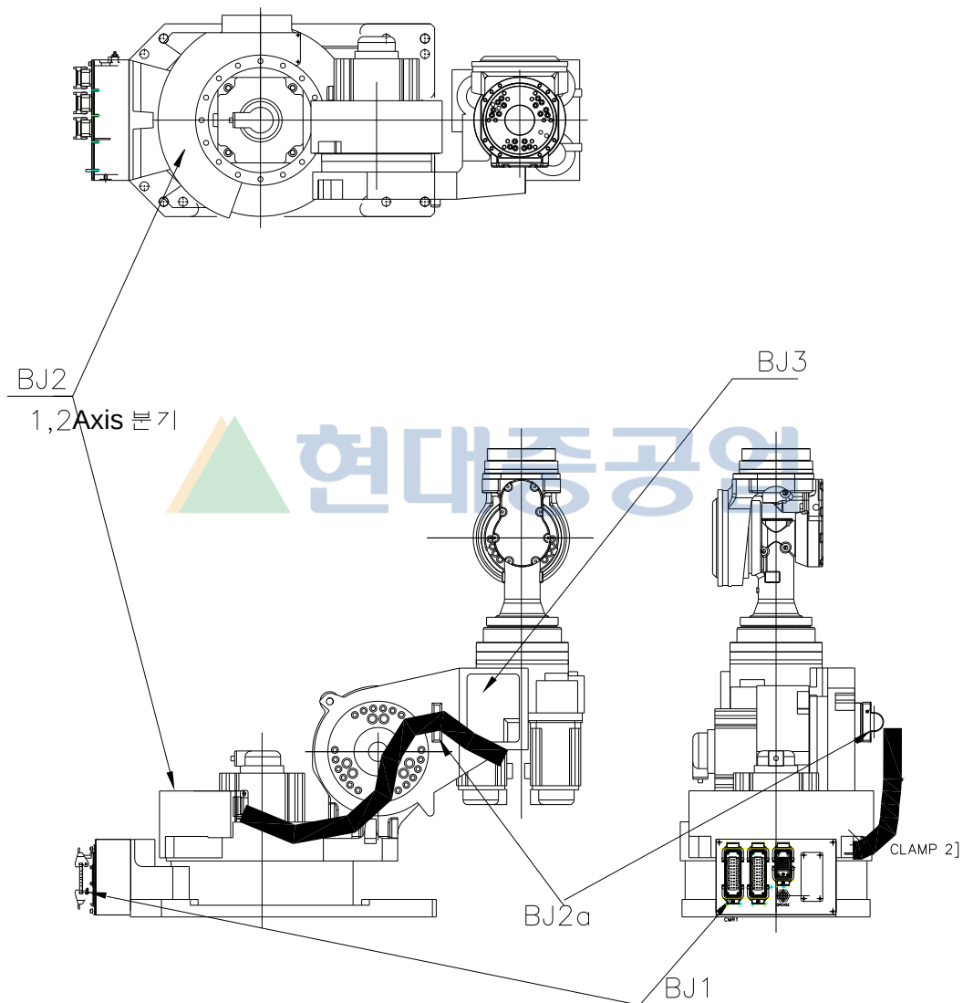
그림 8.1 본체 부품 배치
