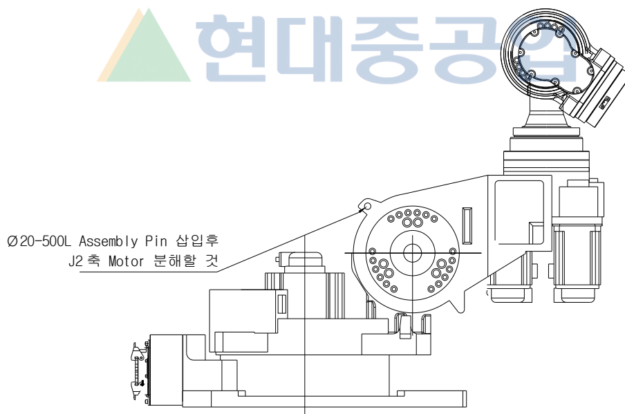
그림 6.1 J2 축 ARM 낙하 방지 방법
