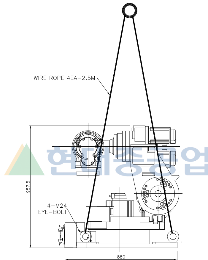
그림 3.3 운송 방법 : 크레인 이용
