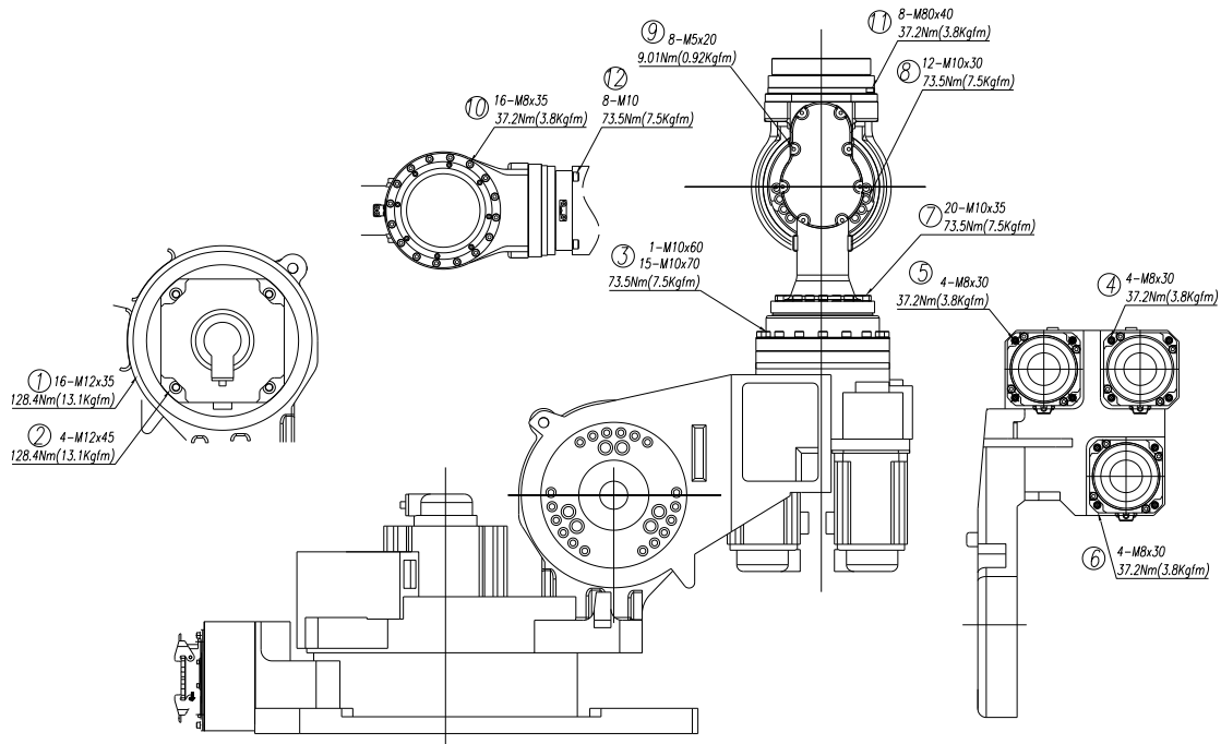
그림 4.1 주요 볼트 점검 부위
