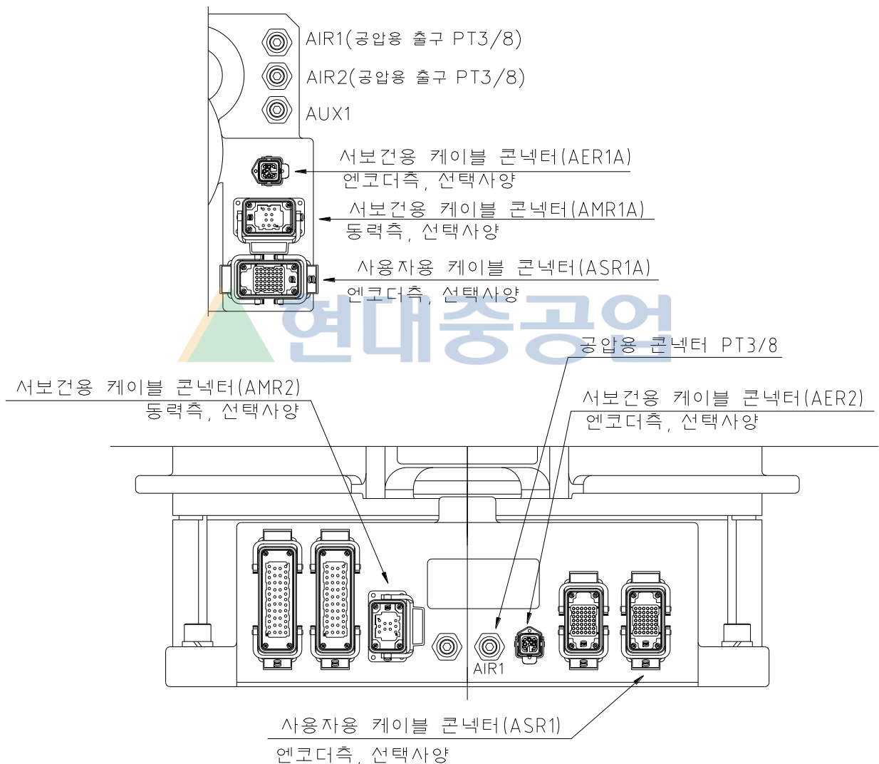
그림 2.7 어플리케이션용 배선 및 배관도
