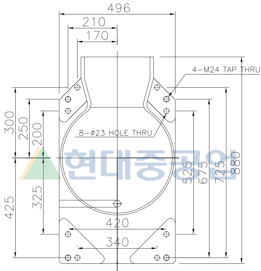
그림 3.5 로봇 설치면 치수
