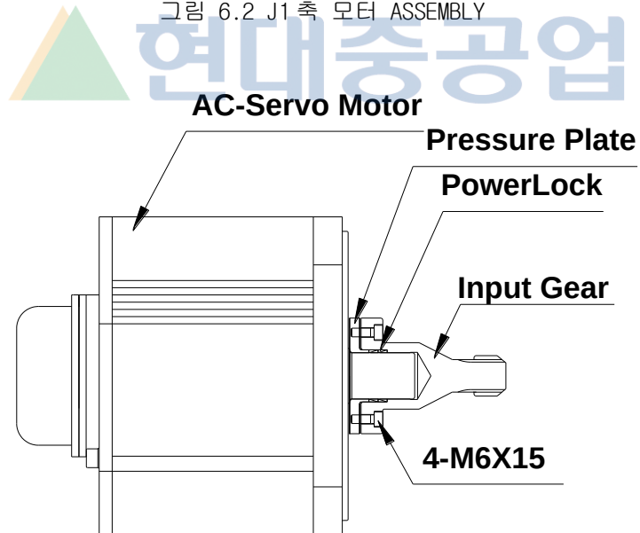
그림 6.2 J1 축 모터 ASSEMBLY
