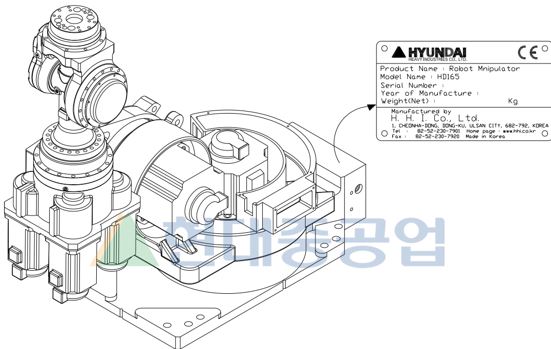
그림 2.2 로봇 명판 부착 위치
