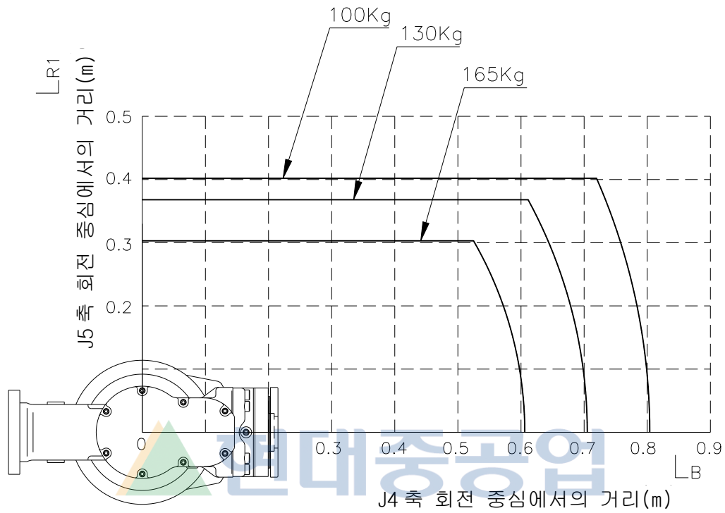
그림 3.6 손목 축 토크 선도
