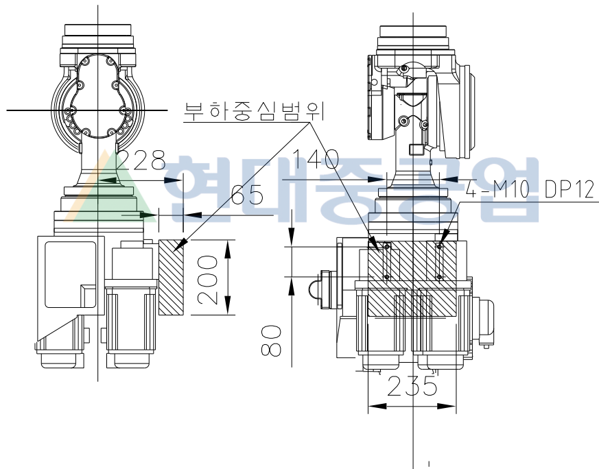
그림 2.6 제 1 암 상부 부착부 상세도
