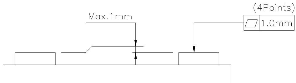
그림 3.4 로봇 설치면 정도
