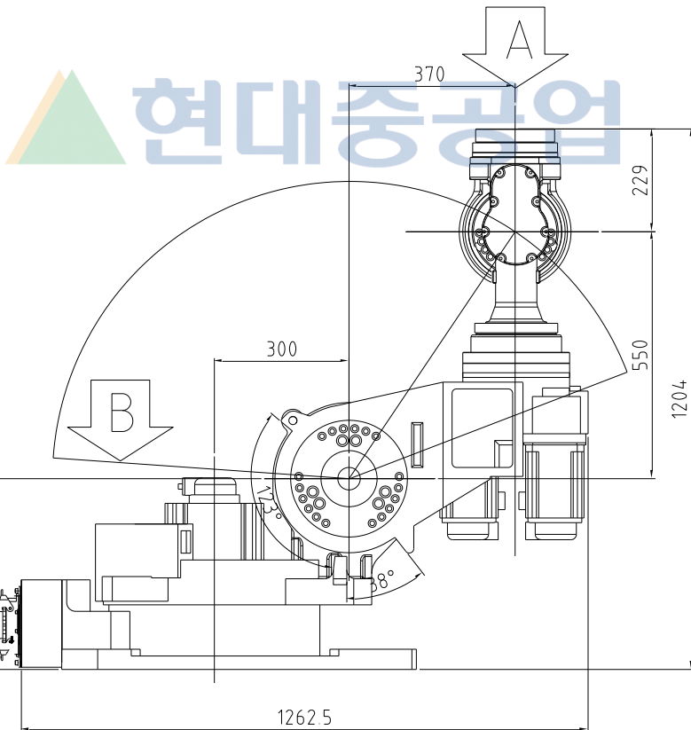
그림 2.3 로봇 본체 외형 치수 및 동작 영역
