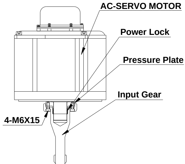
그림 6.2 J1 축 모터 ASSEMBLY
