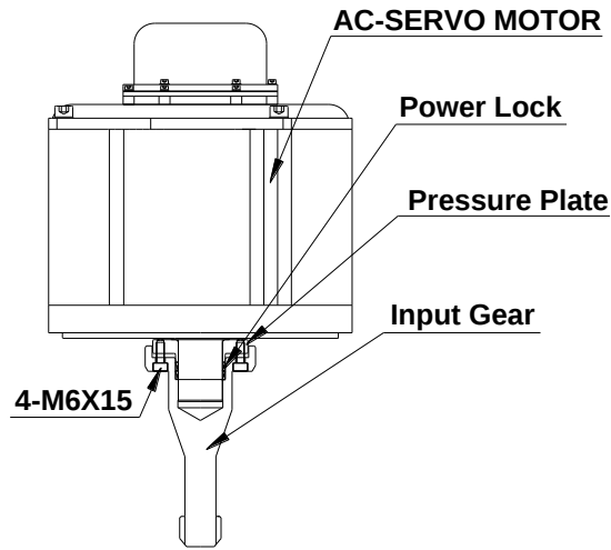
그림 6.2 S 축 모터 ASSEMBLY
