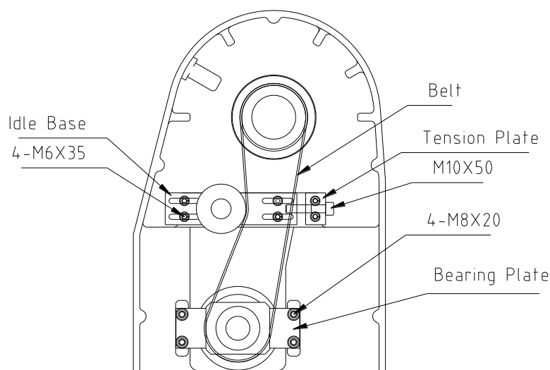
그림 4.4 V 축 타이밍 벨트 장력 체크 부위
