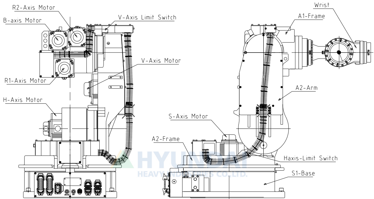
그림 3.1 본체 각 부위 명칭
