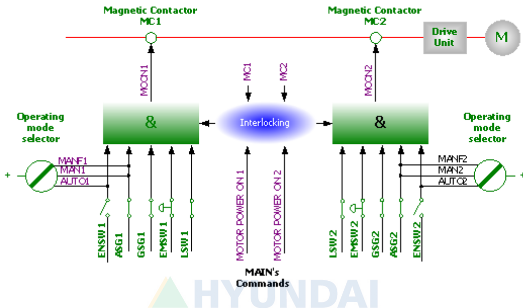
그림 1.5 안전체인 구성도, LTD.
