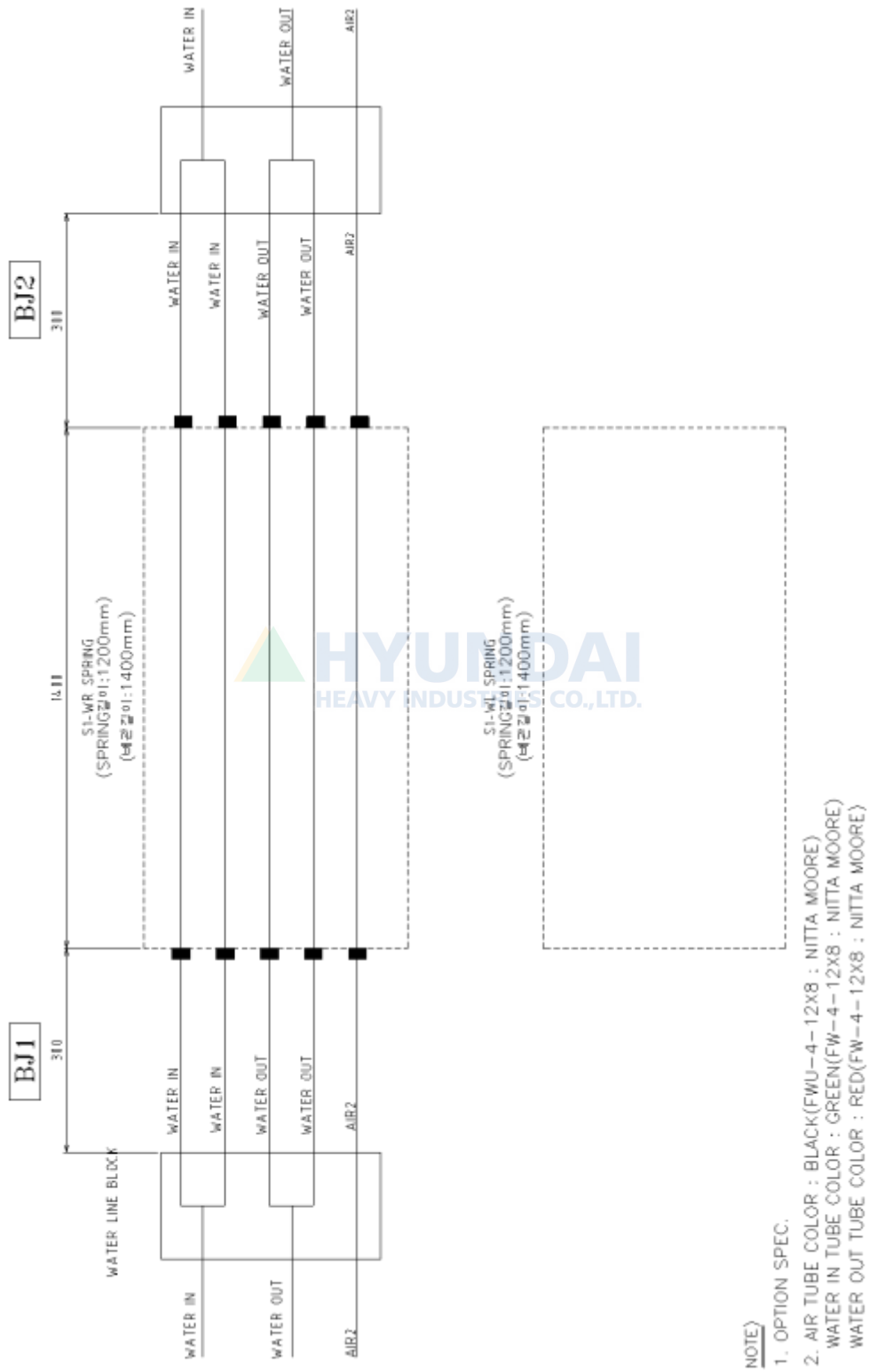
그림 8.12 AIR, WATER LINE
