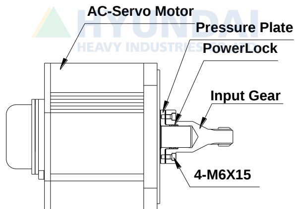
그림 6.3 H 축 모터 ASSEMBLY
