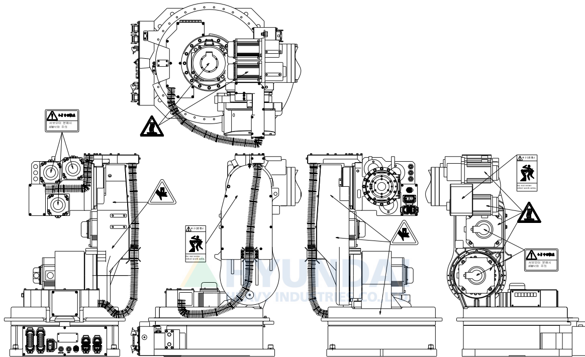
그림 3.2 안전 명판 위치
