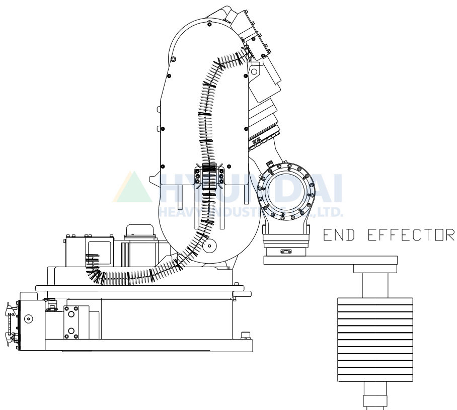
그림 3.10 권장 대기 자세
