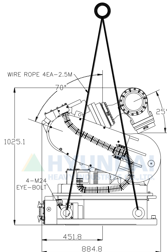
그림 3.3 운송 방법 : 크레인 이용
