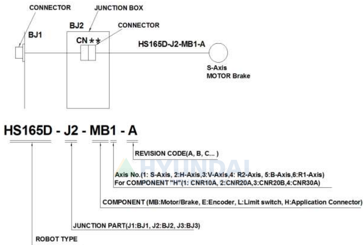
그림 5.2 본체 내 배선 기호 설명
