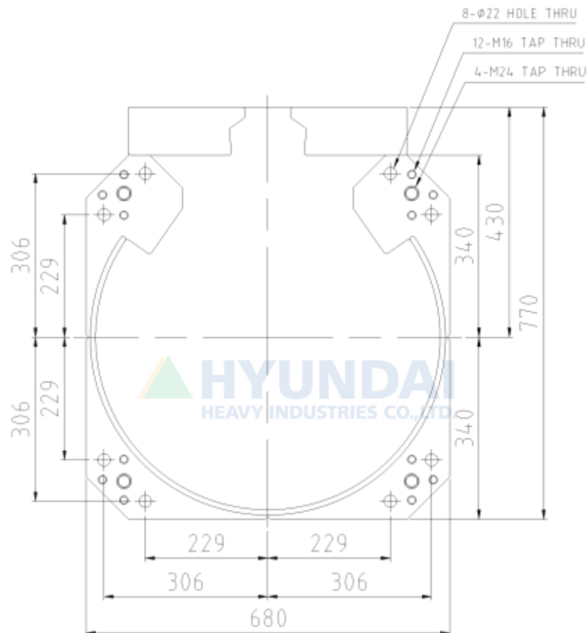
그림 3.5 로봇 설치면 치수
