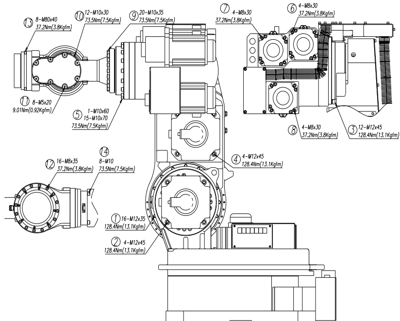
그림 4.1 주요 볼트 점검 부위
