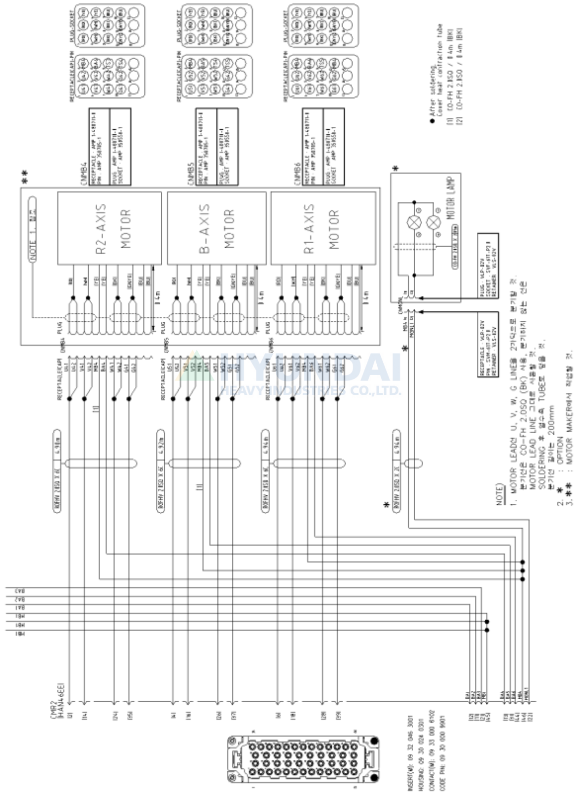
그림 8.4 POWER CABLE (R2,B,R1 AXIS)
