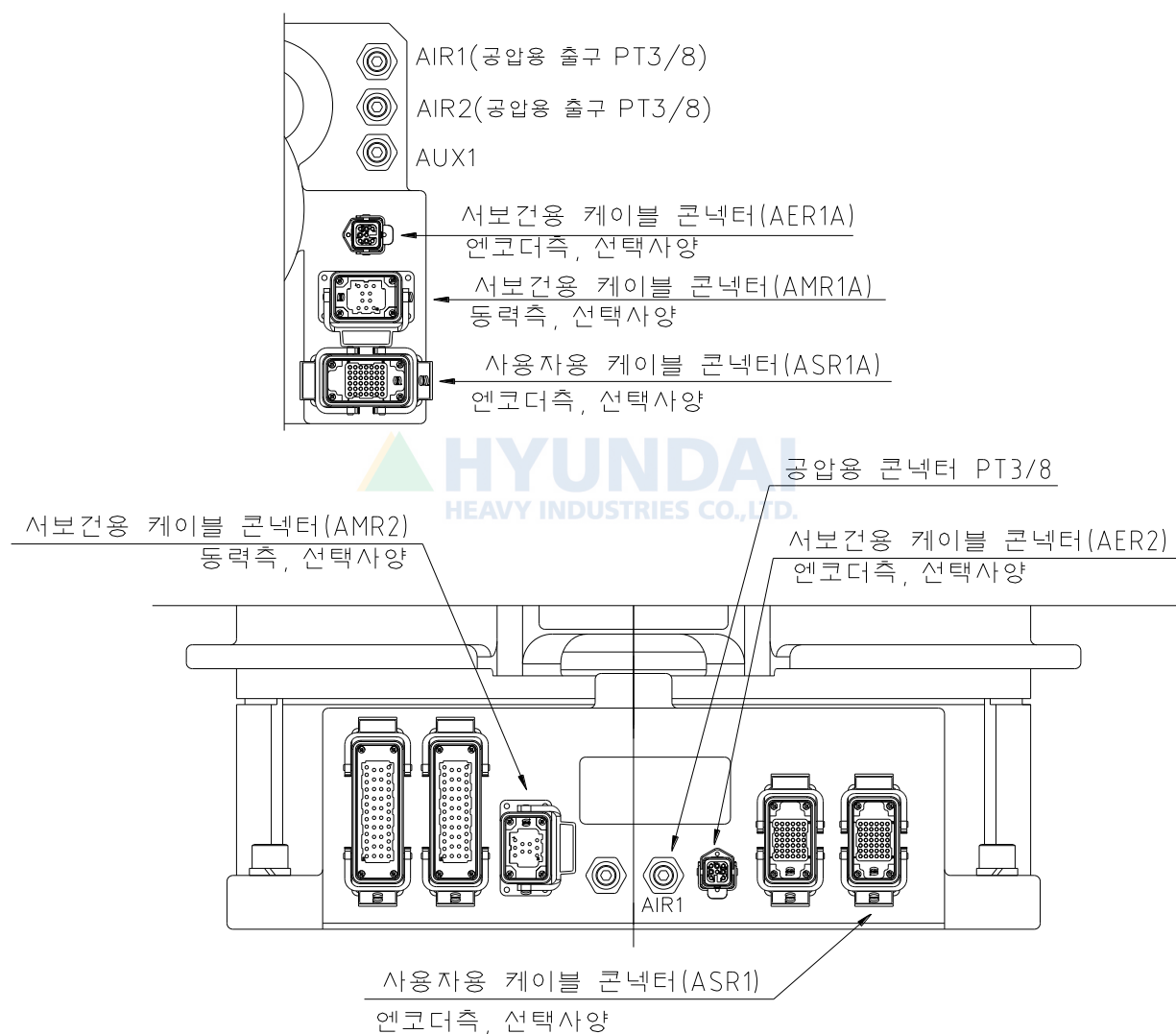
그림 2.7 어플리케이션용 배선 및 배관도
