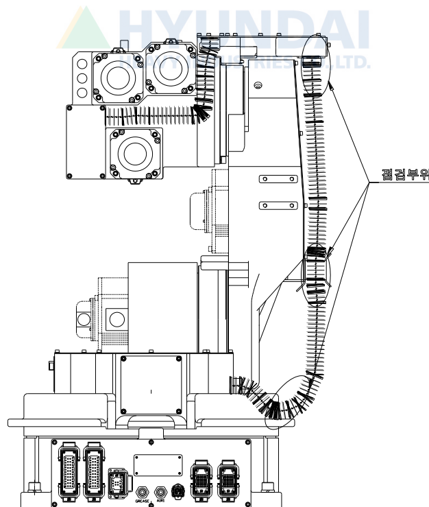
그림 4.3 케이블 점검 부위
