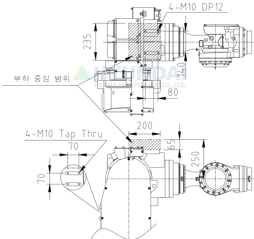
그림 2.6 제 1 암 상부 부착부 상세도
