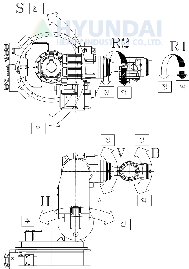
그림 2.4 본체 외관 및 동작 축
