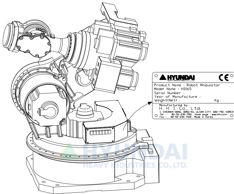
그림 2.2 로봇 명판 부착 위치
