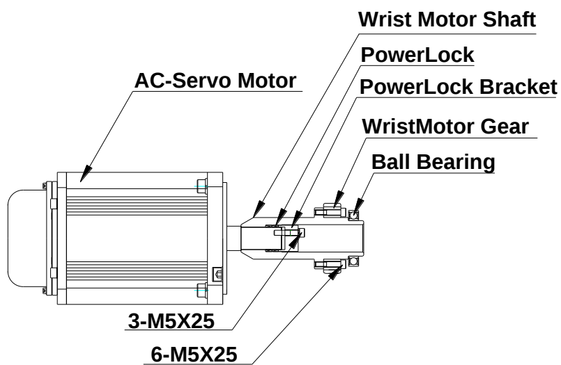
그림 6.5 손목 축 모터 ASSEMBLY
