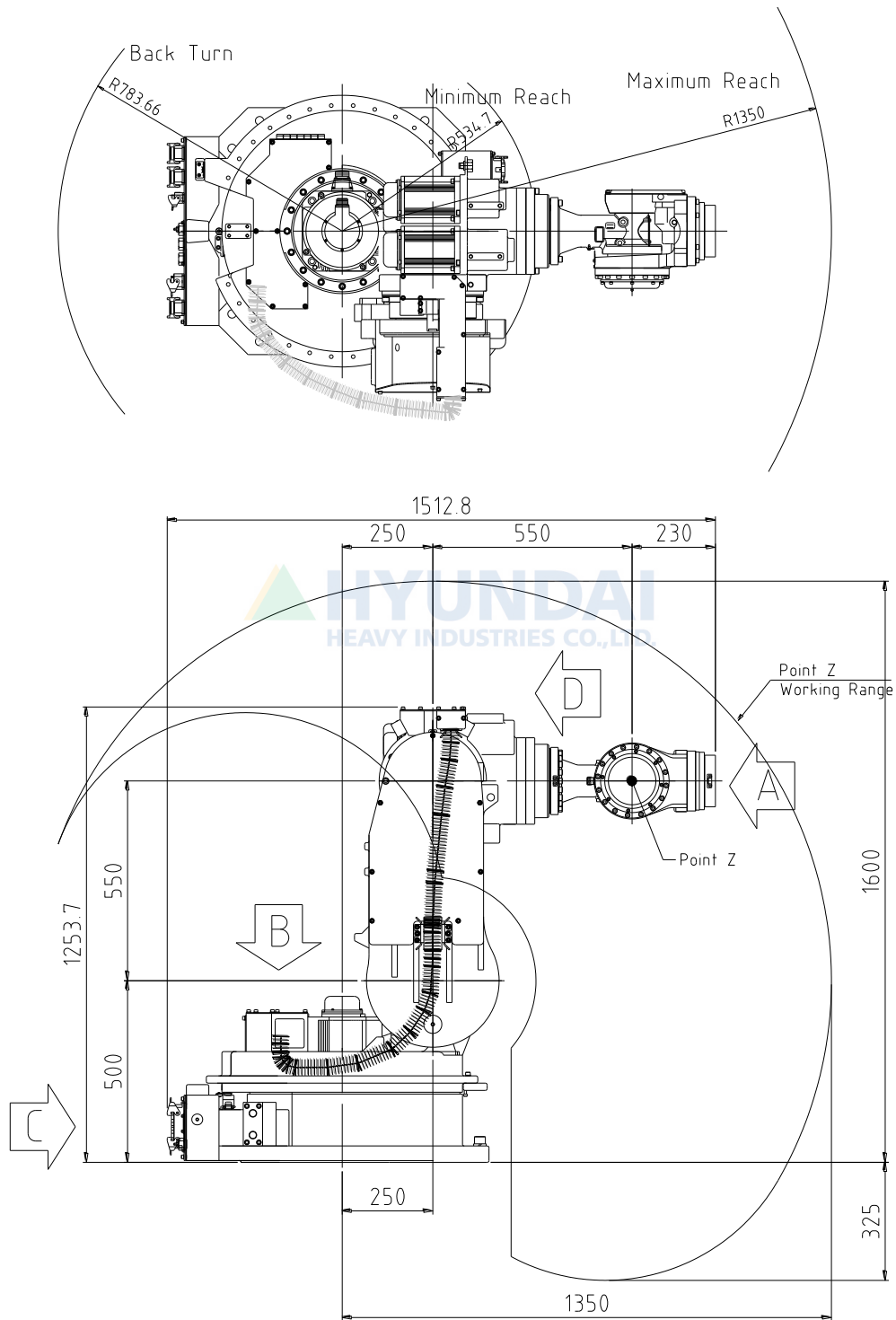
그림 2.3 로봇 본체 외형 치수 및 동작 영역
