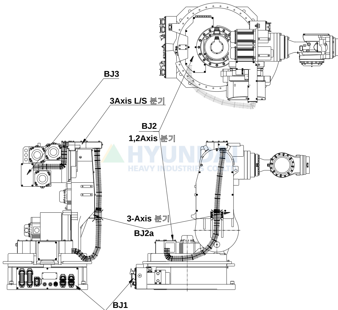
그림 8.1 본체 부품 배치
