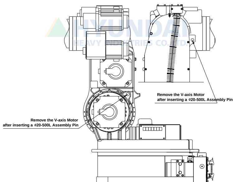
그림 6.1 H, V 축 ARM 낙하 방지 방법
