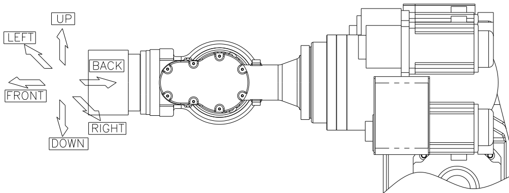
그림 4.2 유격 점검 방향
