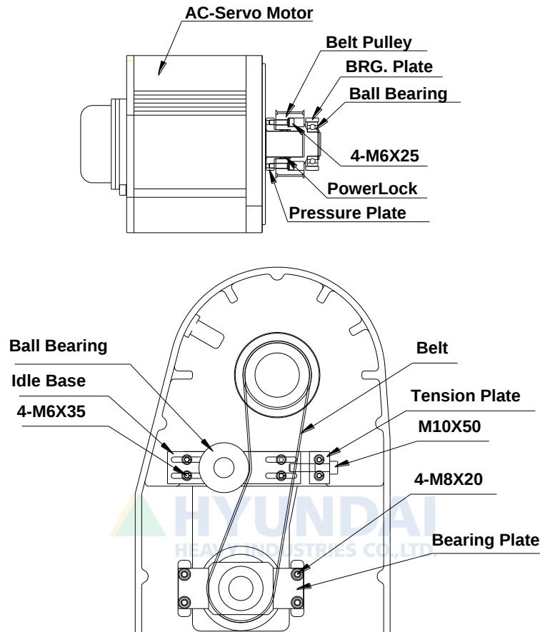
그림 6.4 V 축 모터 ASSEMBLY
