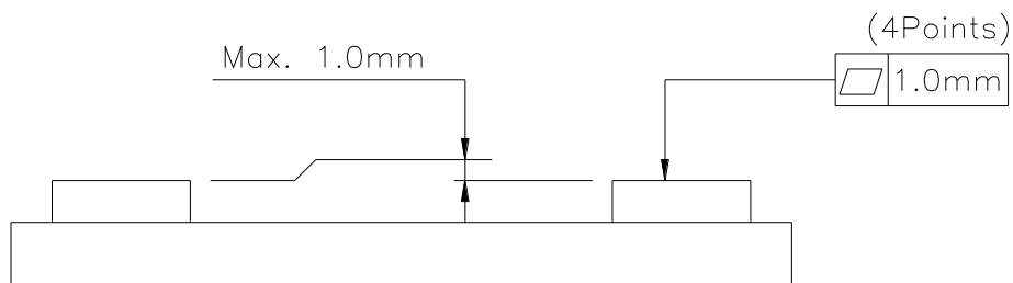
그림 3.4 로봇 설치면 정도
