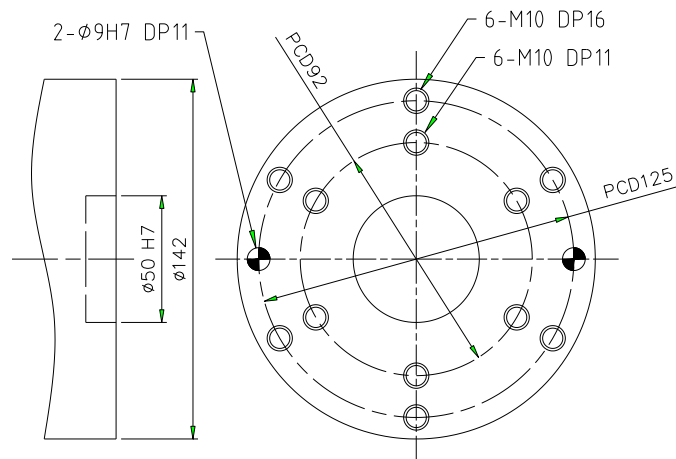
그림 2.5 손목 축 취부면 상세도
