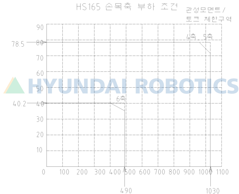
그림 3.10 손목축 부하조건: [HS165]
