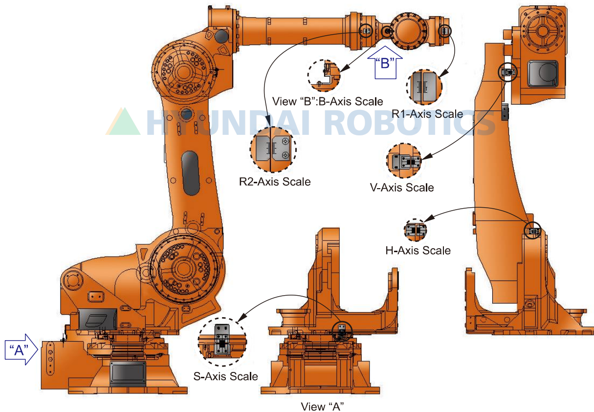
그림 6.6 원점 설정 방법 [HS165/HS200/HS150L]
