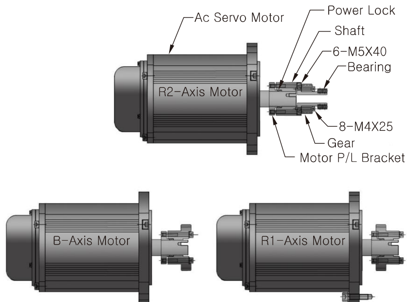
그림 6.5 손목축 모터 ASSEMBLY
