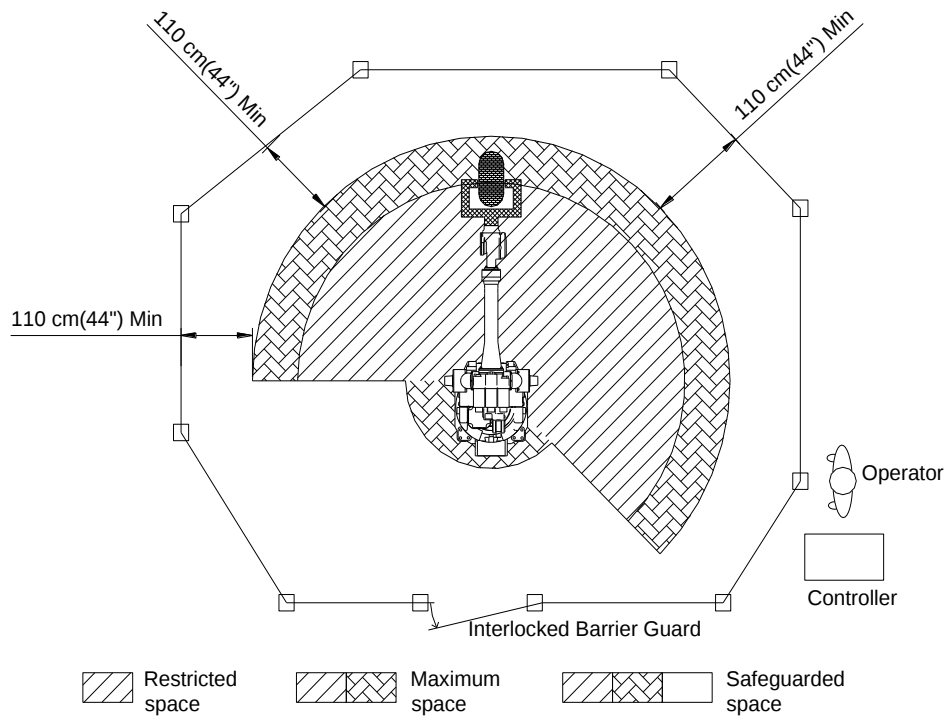
HYUNDAI ROBOTICS 그림 1.4 산업용 로봇 주변장치와 작업자의 배치
