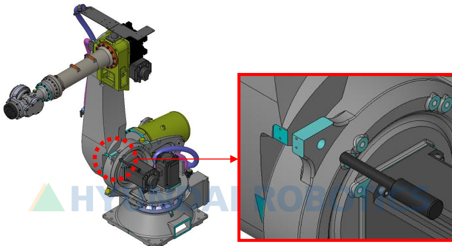
그림 6.1 제 1암(H 축) 고정용 Pin 삽입위치
