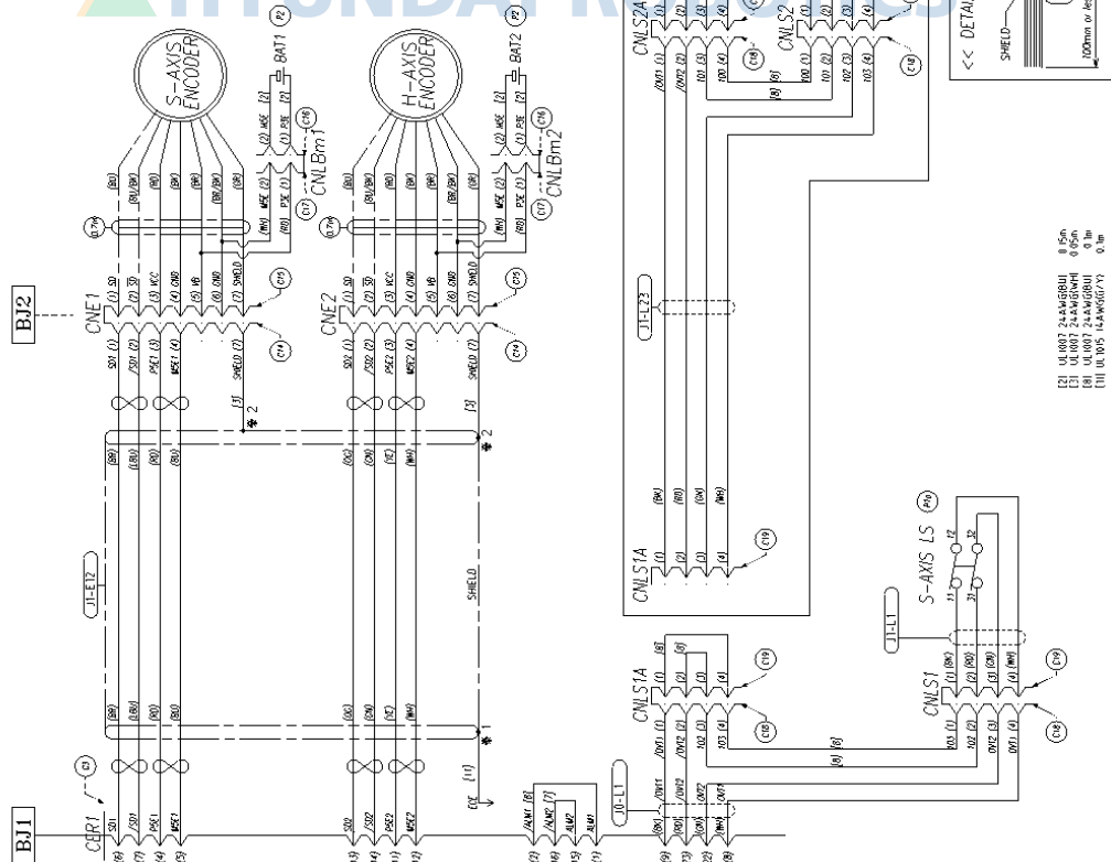
그림 8.5 ENCODER CABLE (1/2) [HS165/HS200/HS150L]
