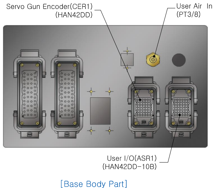
그림 2.9 어플리케이션용 배선 및 배관도 : [HS165/HS200/HS150L]
