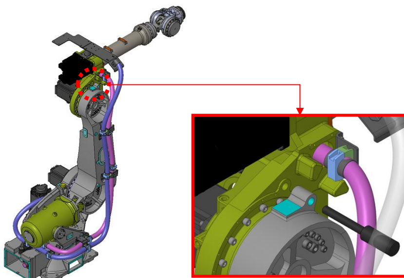
그림 6.2 제 2암(V 축) 고정용 Pin 삽입위치
