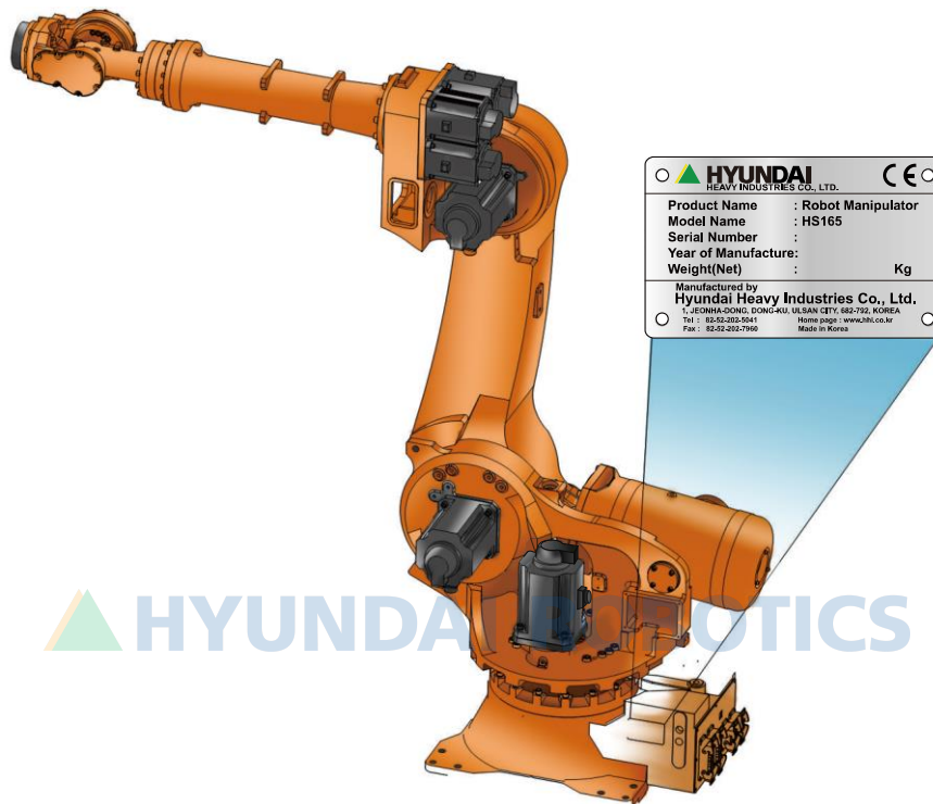
그림 2.2 로봇 명판 부착 위치
