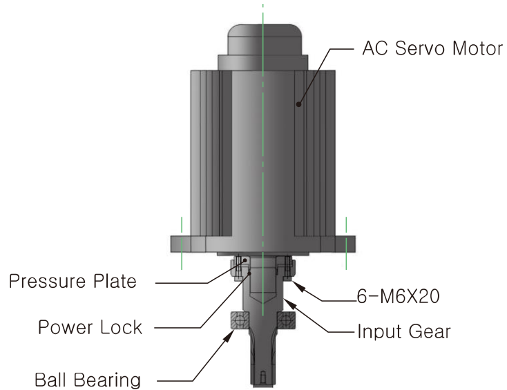
그림 6.3 S 축 모터 ASSEMBLY
