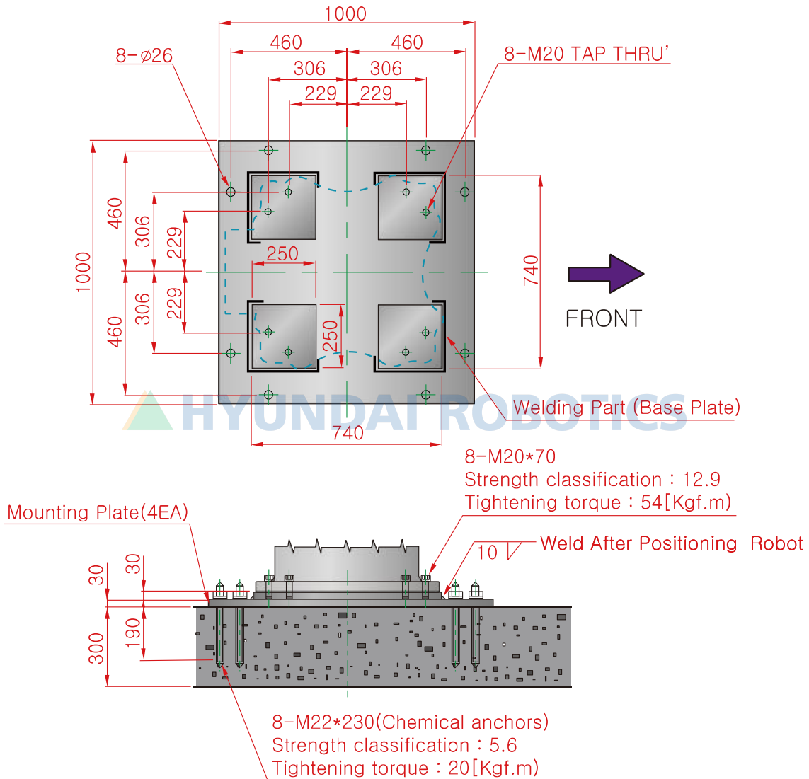
그림 3.6 로봇 설치면 치수 [HS165/HS200/HS150L]
