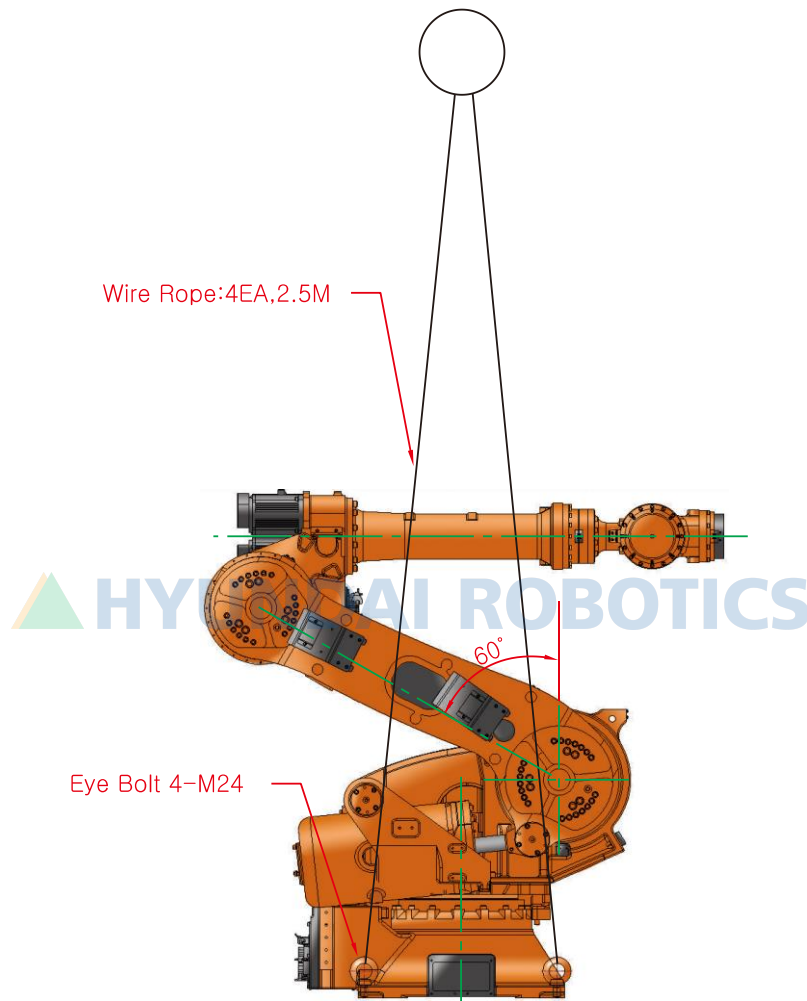
그림 3.3 운송 방법 : 크레인 이용 [HS165/HS200/HS150L]
