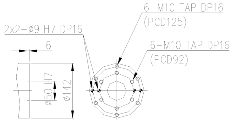
그림 2.6 손목축 취부면 상세도 : [HS165/HS150L]
