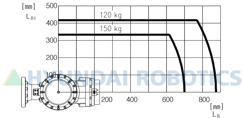
그림 3.9 손목축 토크 선도 : [HS150L]
