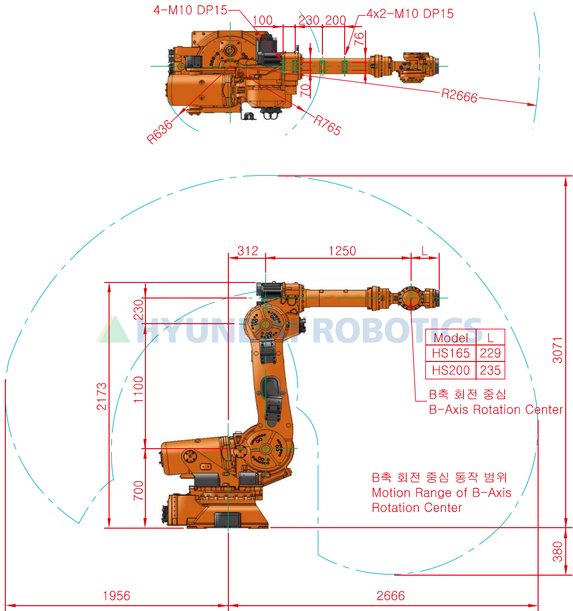
그림 2.3 로봇 본체 외형 치수 및 동작 영역 : [HS165/HS200]
