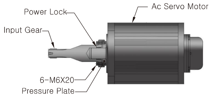
그림 6.4 H&V 축 모터 ASSEMBLY
