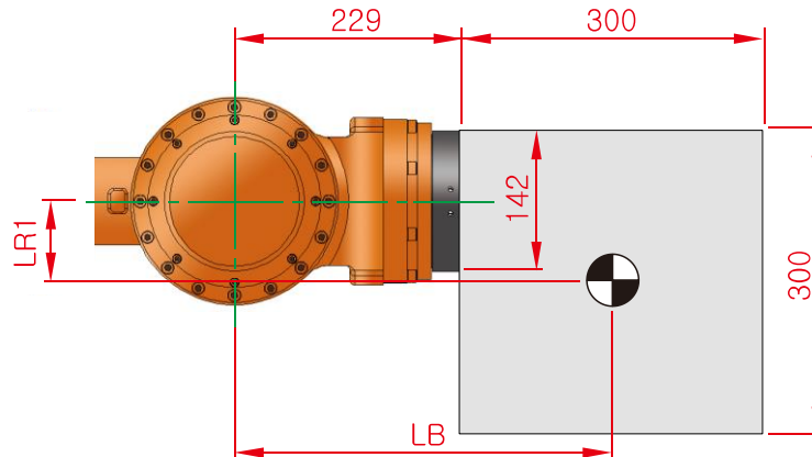
그림 3.11 HS165 2차원 부하 모델
