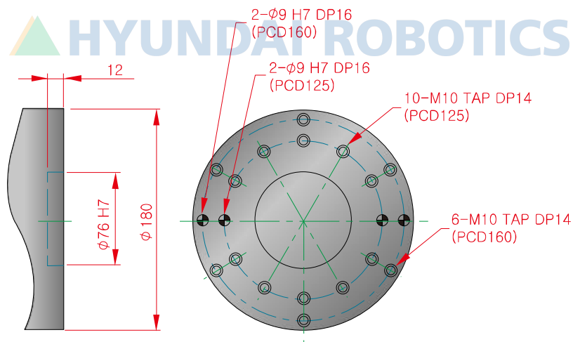
그림 2.7 손목축 취부면 상세도 : [HS200]
