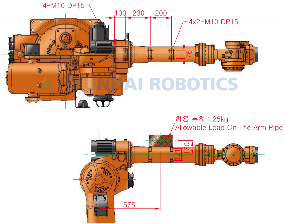
그림 2.8 ARM FRAME 상부 부착부 상세도 : [HS165/HS200/HS150L]
