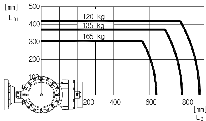
그림 3.7 손목축 토크 선도: [HS165]
