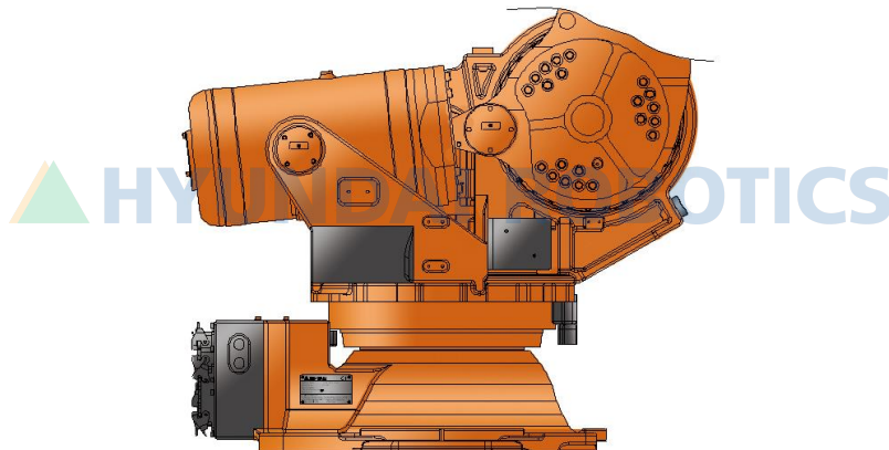
그림 9.1 밸런스 스프링 분리 자세
