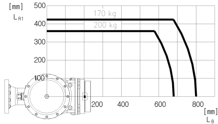
그림 3.8 손목축 토크 선도 : [HS200]
