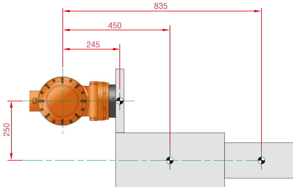
그림 3.12 HS165 3 차원 부하 모델 2D 형상
