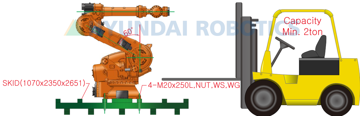
그림 3.4 운송 방법 : 지게차 이용 [HS165/HS200/HS150L]
