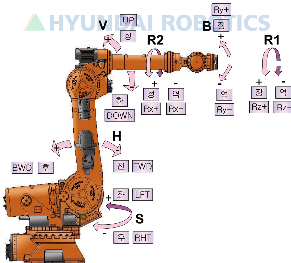
그림 2.5 본체 외관 및 동작 축 [HS165/HS200/HS150L]
