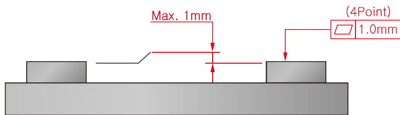
그림 3.5 로봇 설치면 정도
