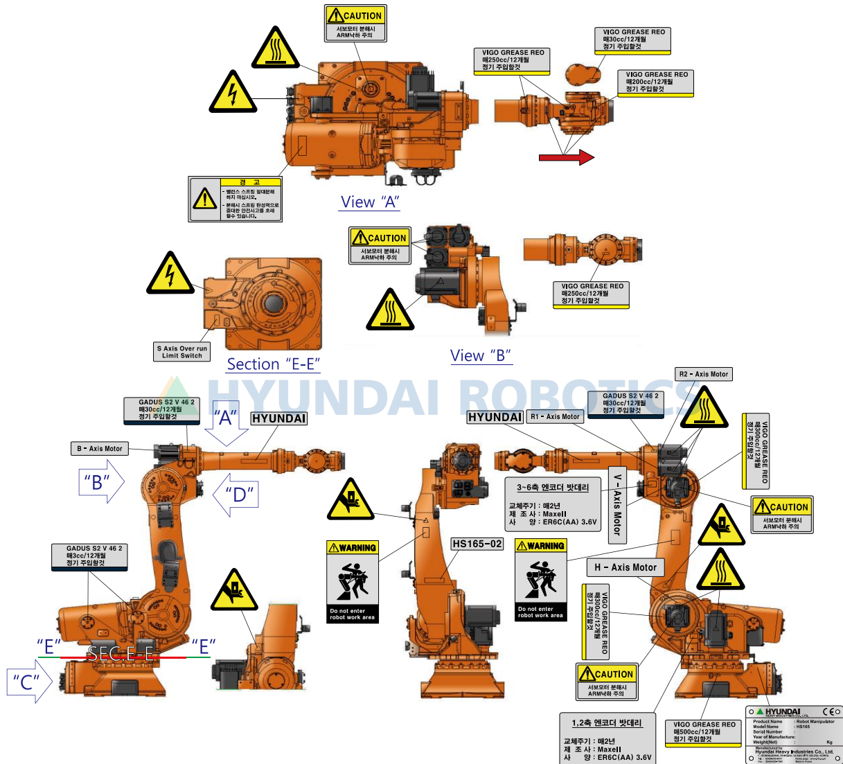
그림 3.2 안전 명판 위치
