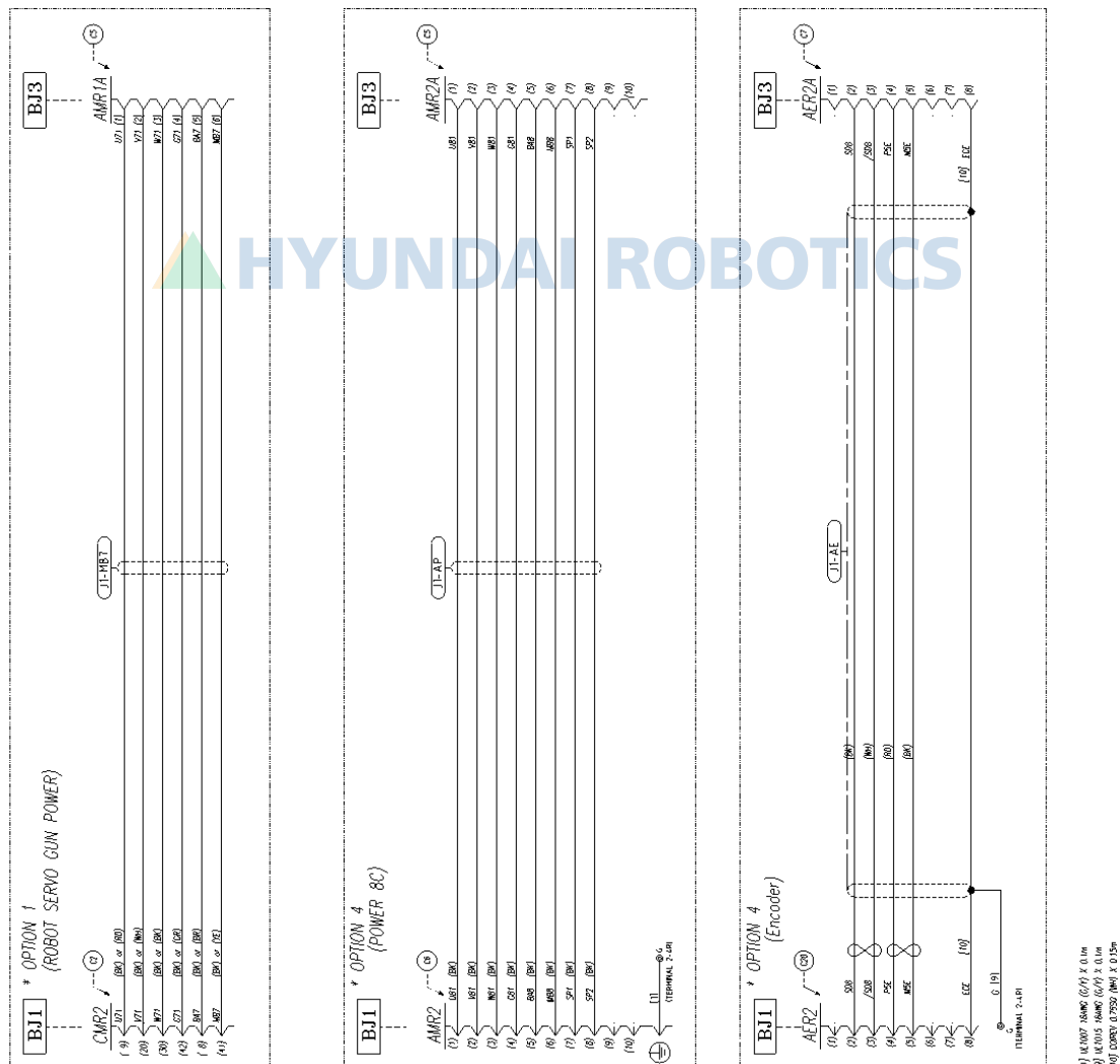
그림 8.7 ADD-AXIS/USER POWER CABLE [HS165/HS200/HS150L]
