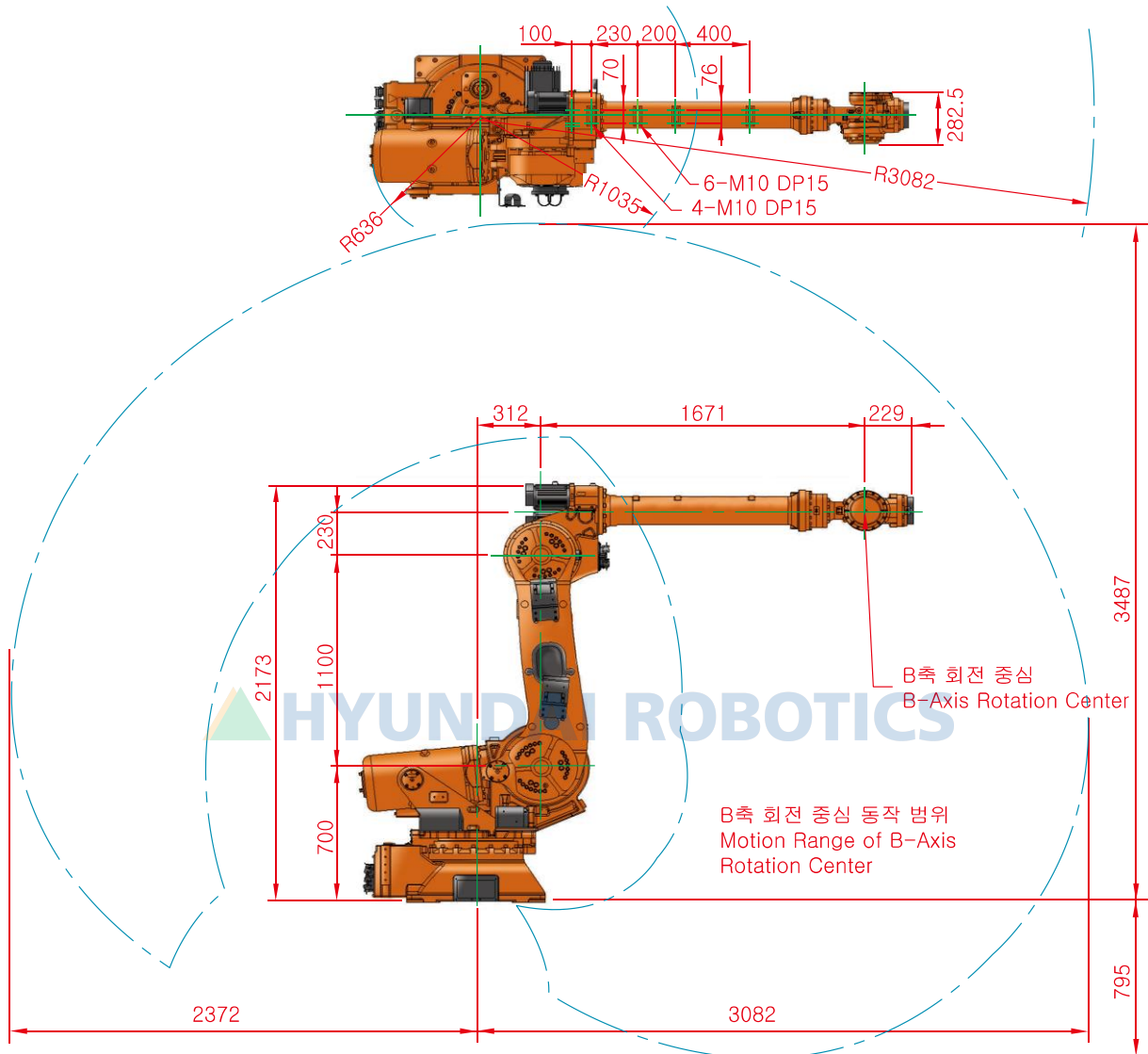
그림 2.4 로봇 본체 외형 치수 및 동작 영역 : [HS150L]
