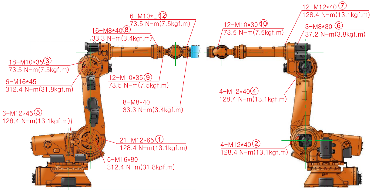
그림 4.1 주요 볼트 점검 부위 [HS165]
