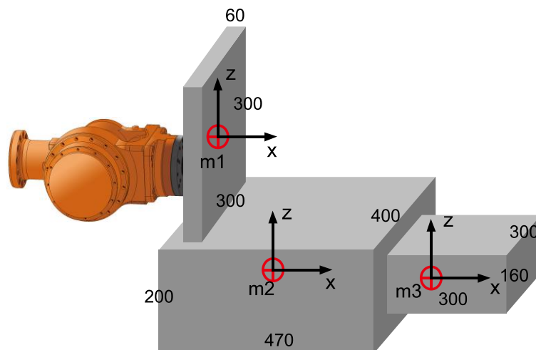
그림 3.13 HS165 3 차원 부하 모델 3D 형상
