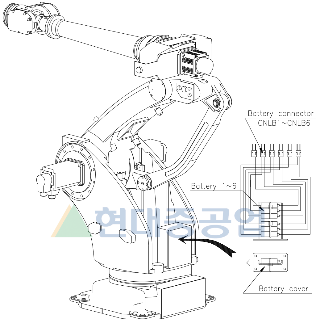
그림 5.1 배터리 교환 위치[HR0500P]
