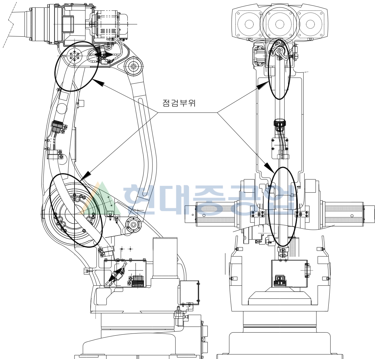
그림 4.3 케이블 점검 부위 : [HR050P]
