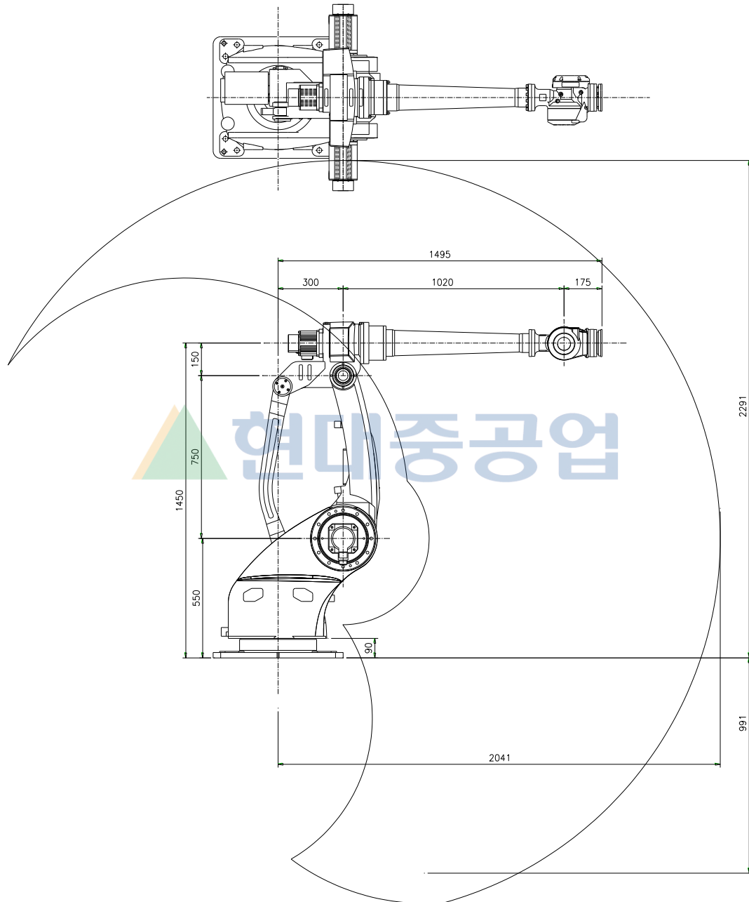
그림 2.3 로봇 본체 외형 치수 및 동작 영역 : [HR050P]
