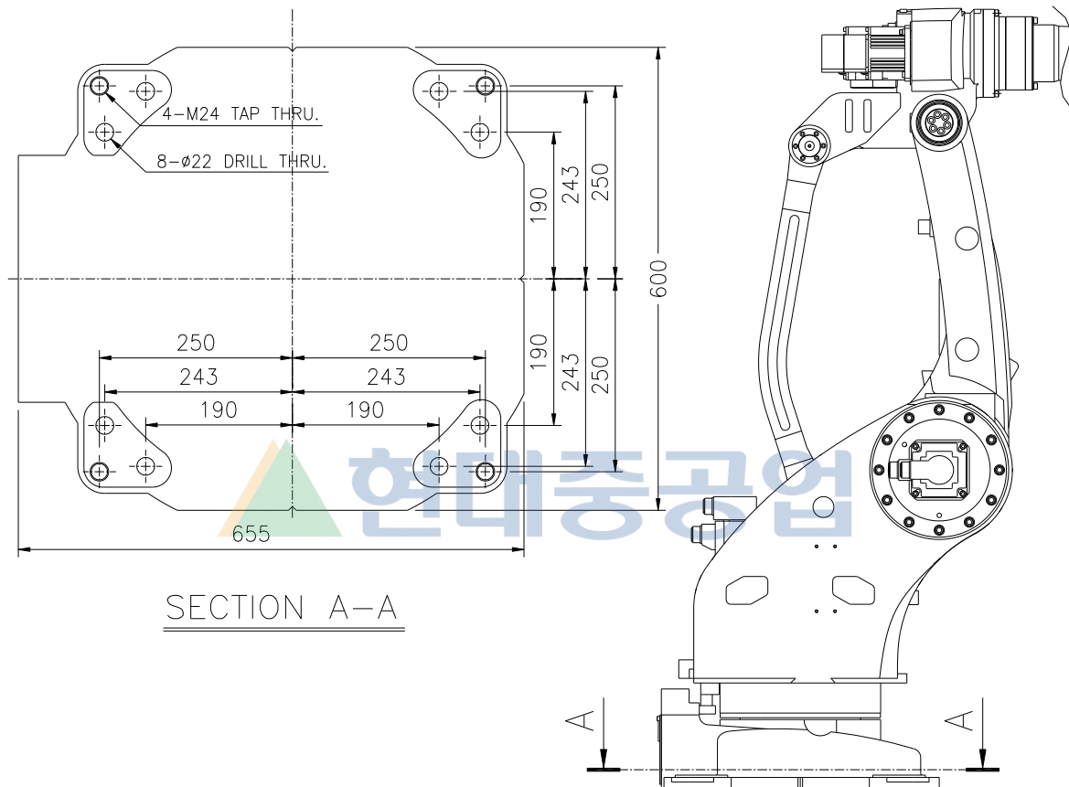
그림 3.6 로봇 설치면 치수 : [HR050P]
