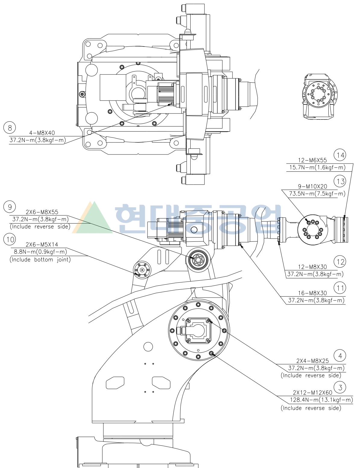
그림 4.1 주요 볼트 점검 부위 [HR050P]
