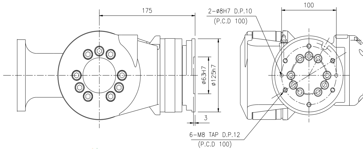
그림 2.5 손목 축 취부면 상세도 : [HR050P]
