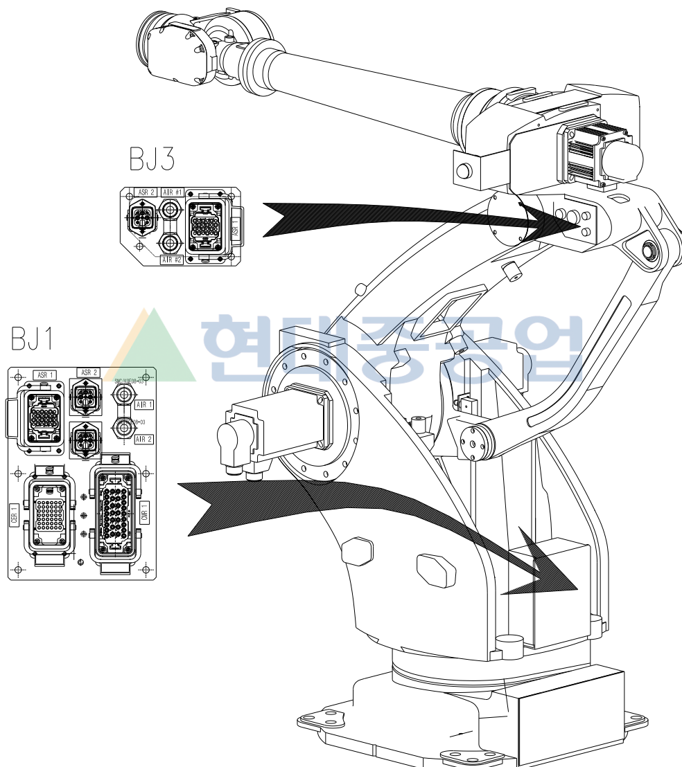
그림 2.7 어플리케이션용 배선 및 배관도 : [HR050P]
