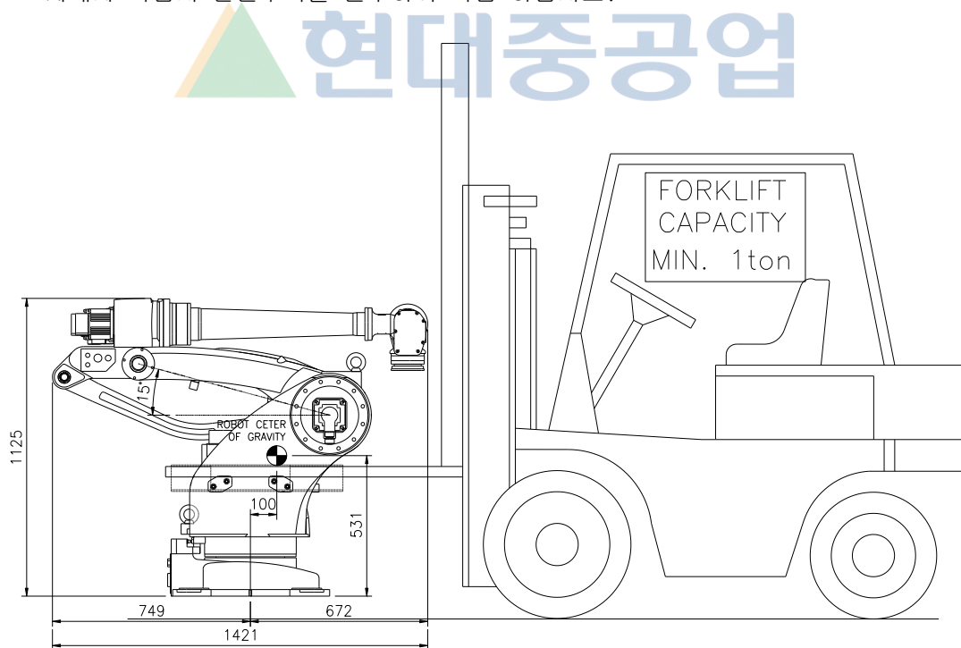
그림 3.4 운반 방법 : 지게차 이용 [HR050P]
