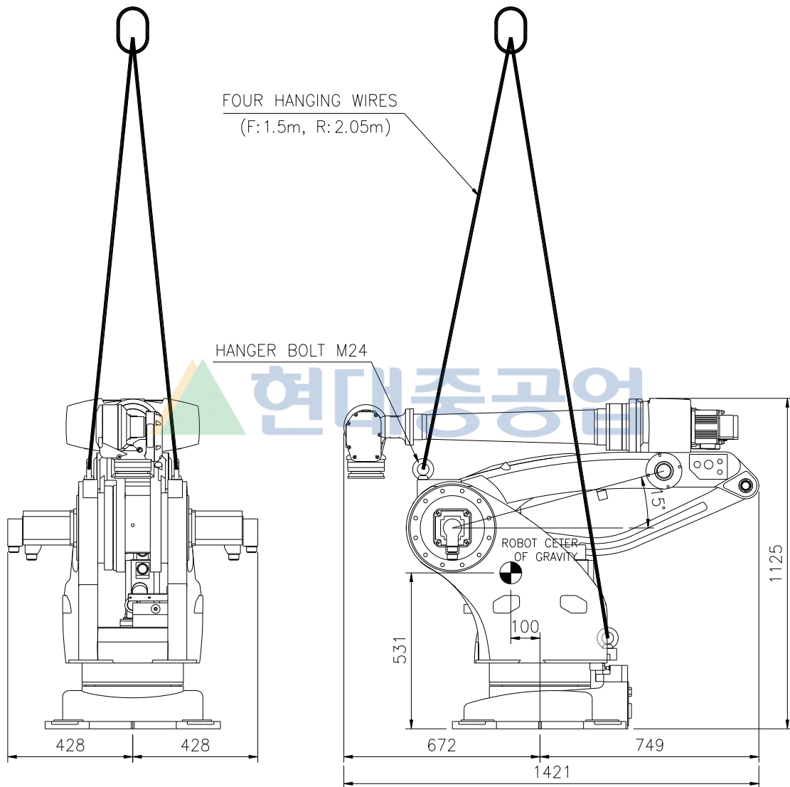
그림 3.3 운반 방법 : 크레인 이용 [HR050P]
