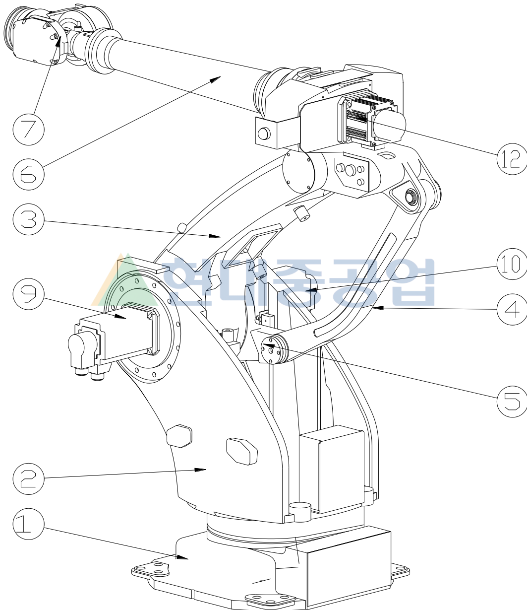
그림 3.1 본체 각 부위 명칭 : [HR050P]
