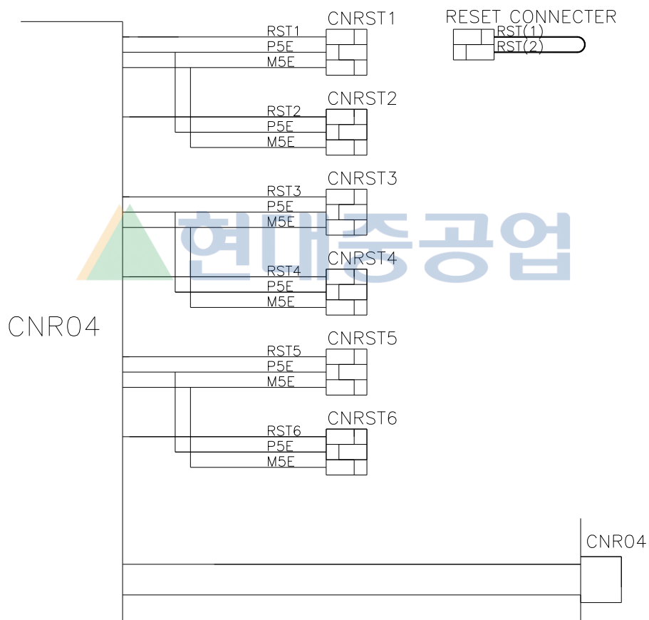
그림 6.2 엔코더 리셋 콘넥터 [HR050P]
