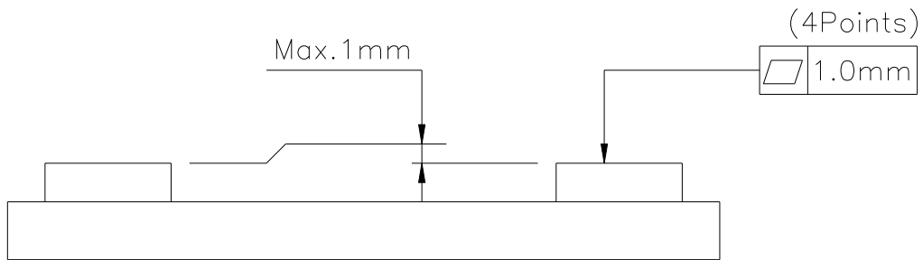
그림 3.5 로봇 설치면 정도
