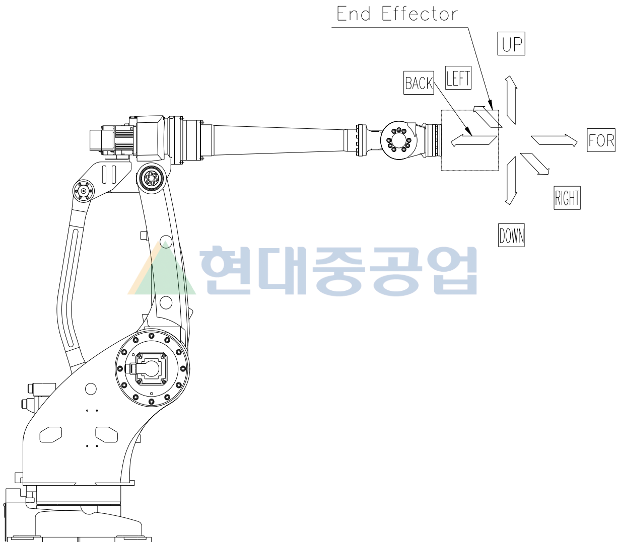
그림 4.2 유격 점검 방향 [HR050P]
