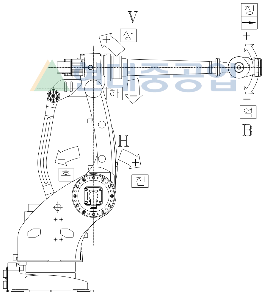
그림 2.4 본체 외관 및 동작 축 [HR050P]
