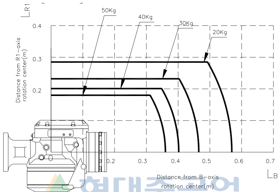
그림 3.7 손목 축 토크 선도 [HR050P]
