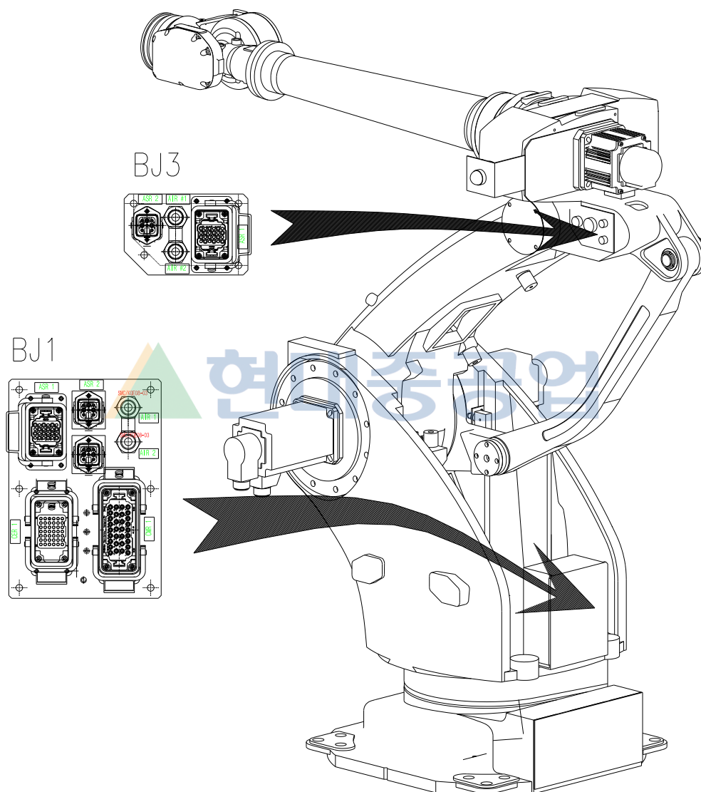
그림 8.1 본체 부품 배치 [HR050P]
