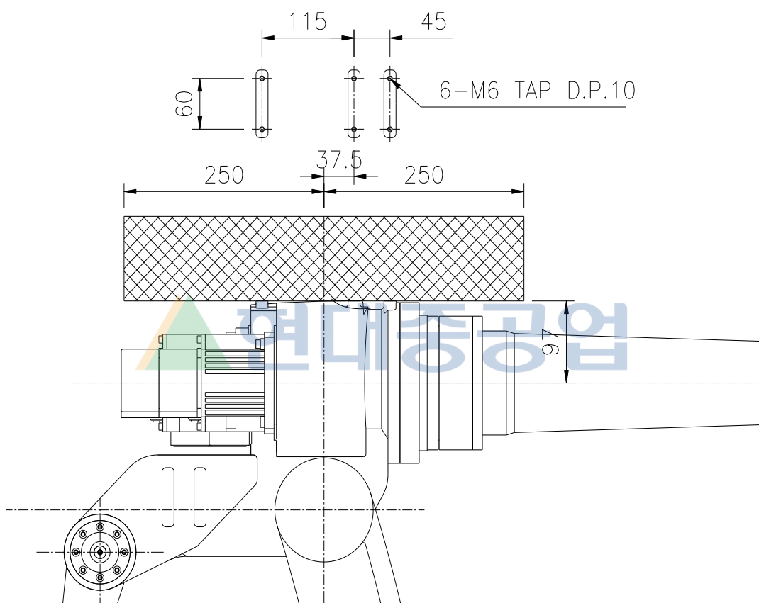
그림 2.6 제 1ARM 상부 부착부 상세도 : [HR050P]
