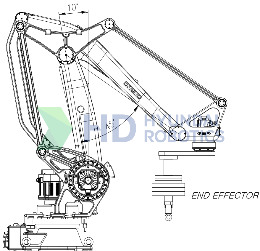
그림 3.10 권장 대기 자세
