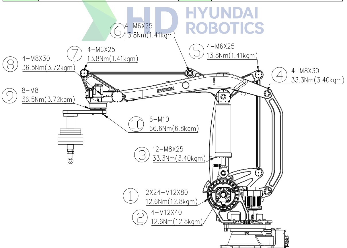
그림 4.1 주요 볼트 점검 부위
