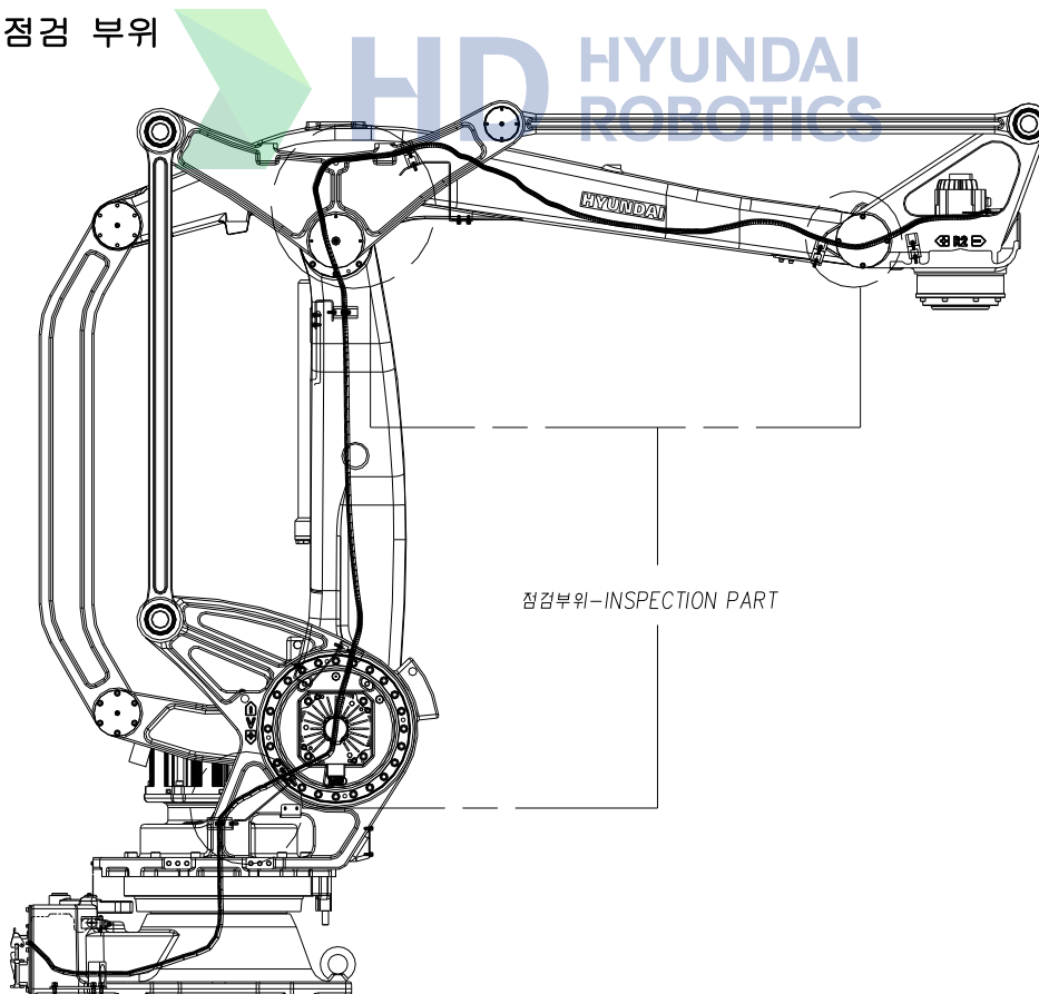
그림 4.3 케이블 점검 부위
