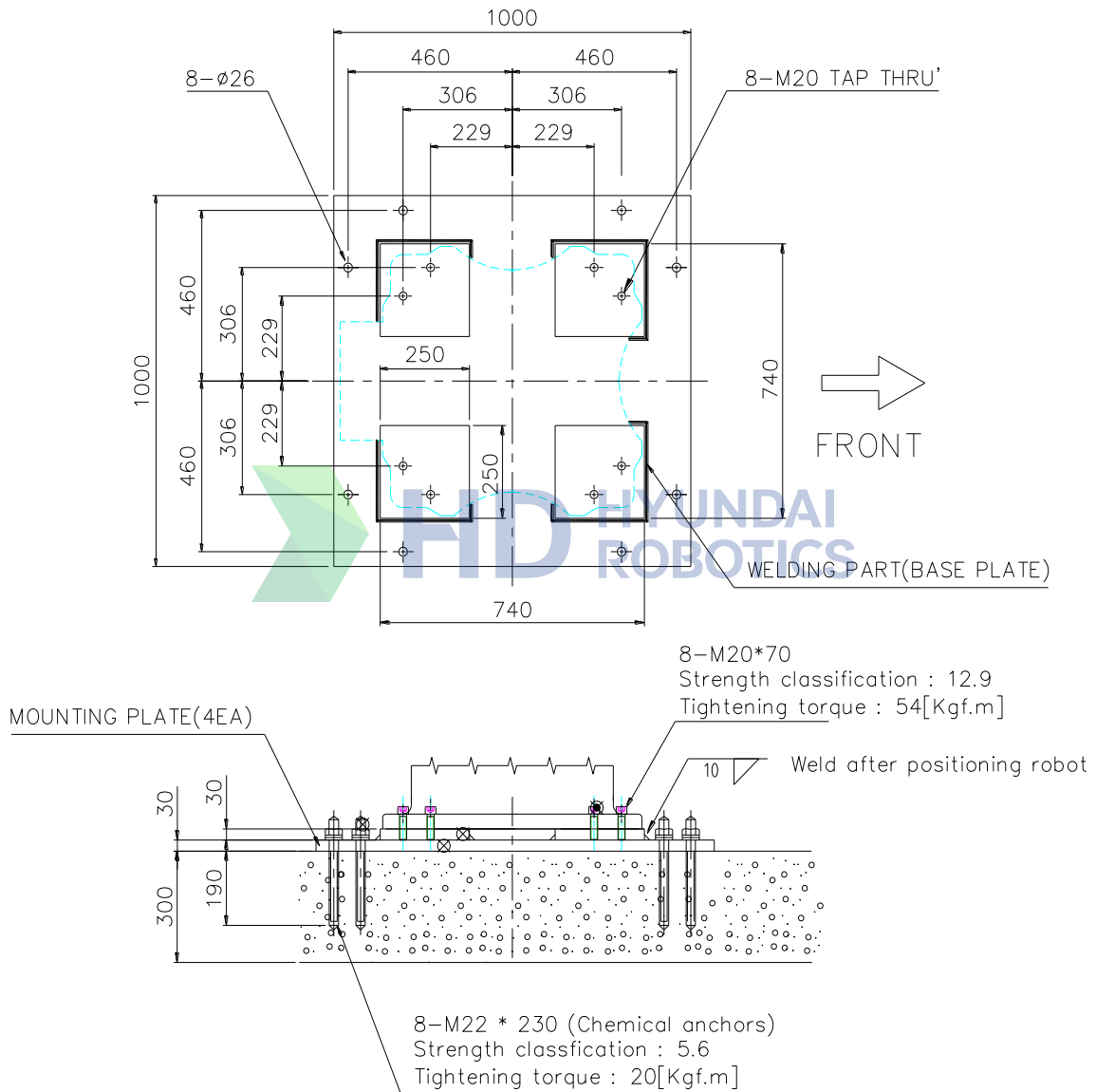
그림 3.6 로봇 본체 설치 치수
