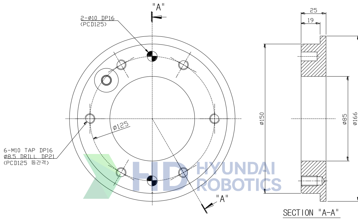
그림 2.7 손목축 취부면 상세도
