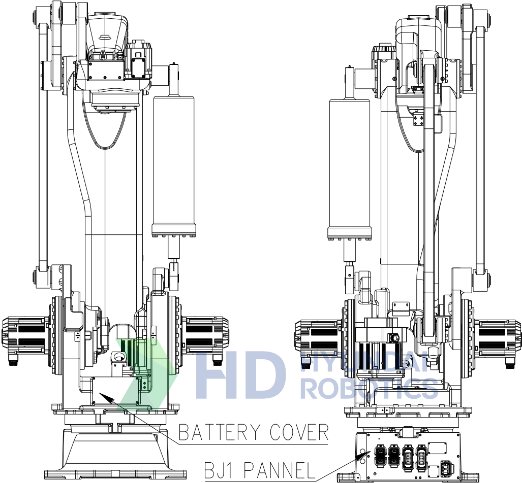
그림 9.1 본체 부품 배치
