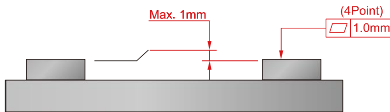
그림 3.5 로봇 설치면 정도
