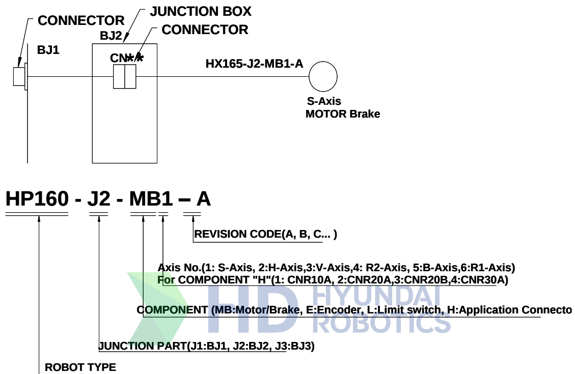
그림 5.1 본체 내 배선 기호 설명
