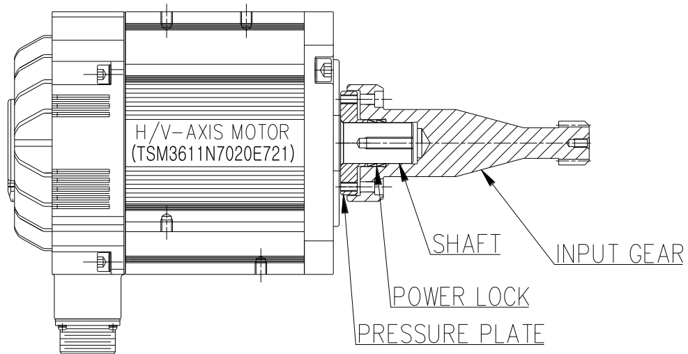
그림 6.3 H & V 축 모터 ASSEMBLY
