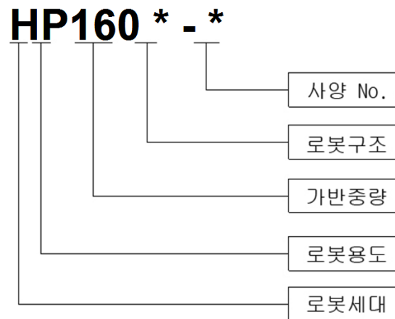
그림 2.1 로봇 기구부 형식
