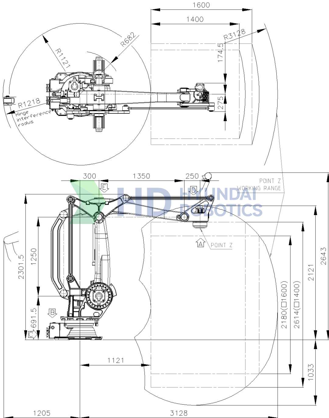
그림 2.3 로봇 본체 외형 치수 및 동작 영역
