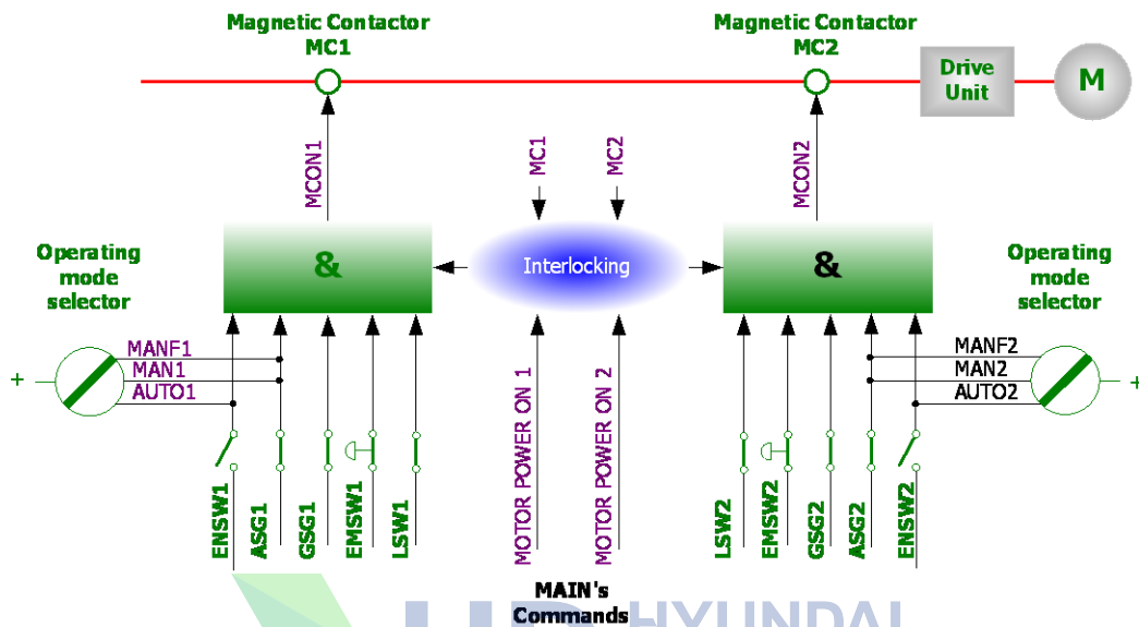
그림 1.5 안전체인 구성도
