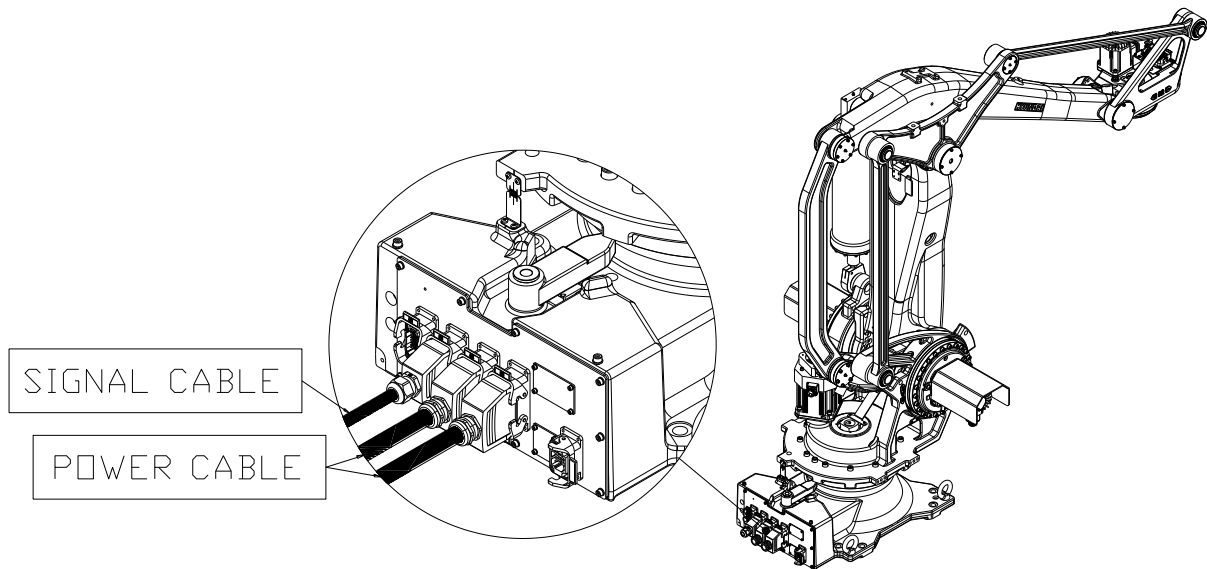
그림 3.7 로봇 Cable 연결
