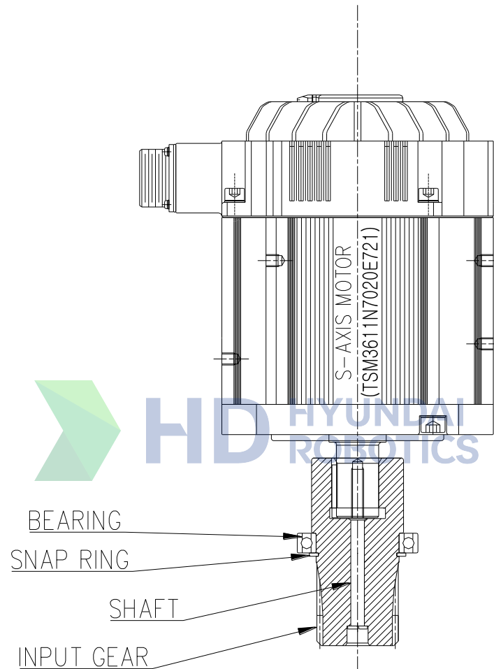
그림 6.2 S 축 모터 ASSEMBLY
