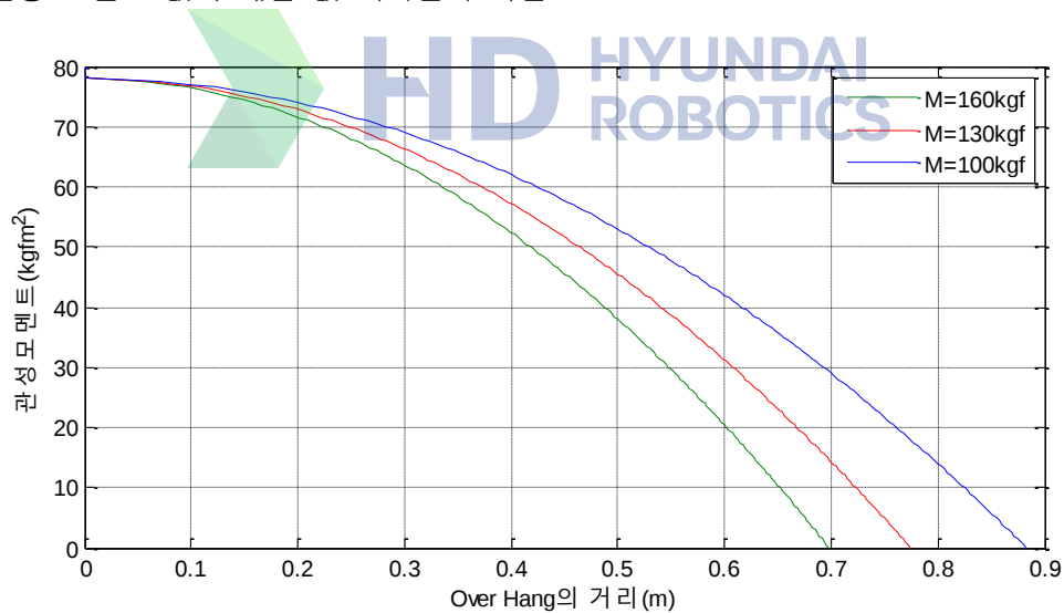
그림 3.8 손목축 부하조건
