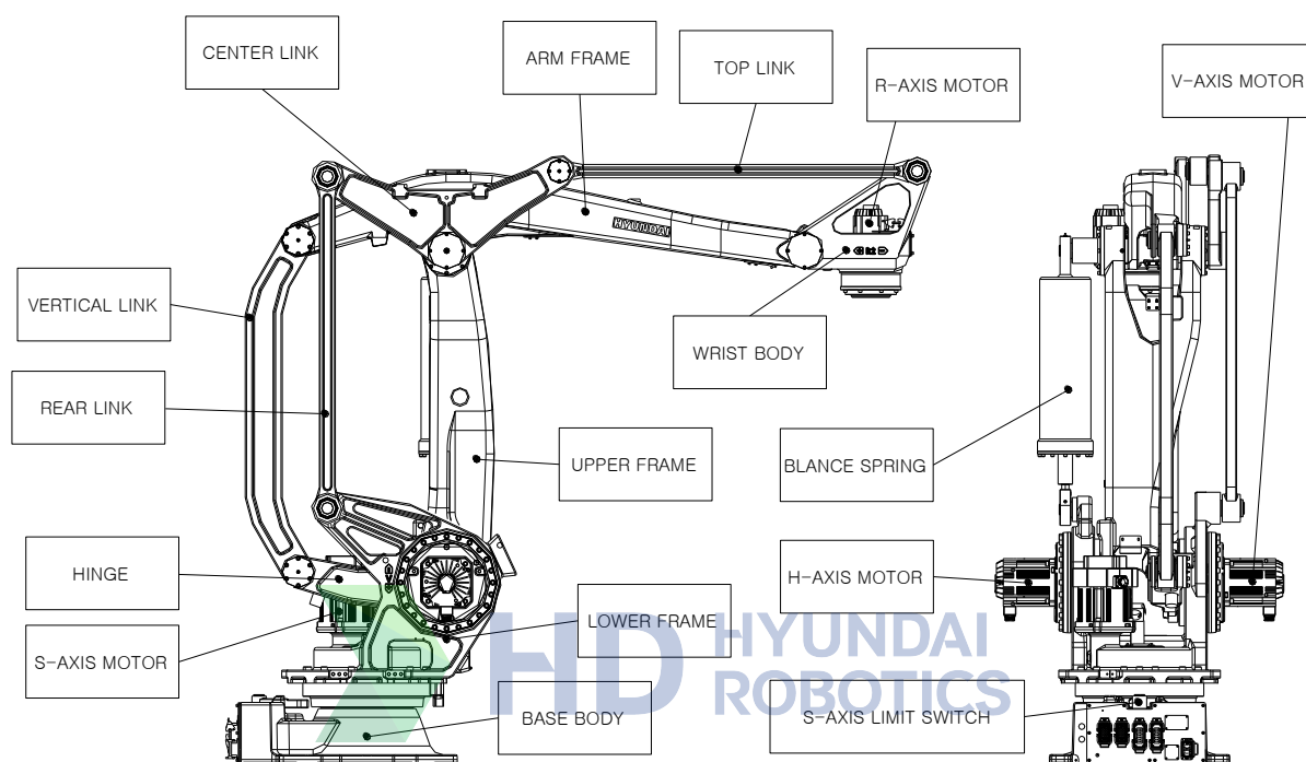
그림 3.1 본체 각 부위 명칭
