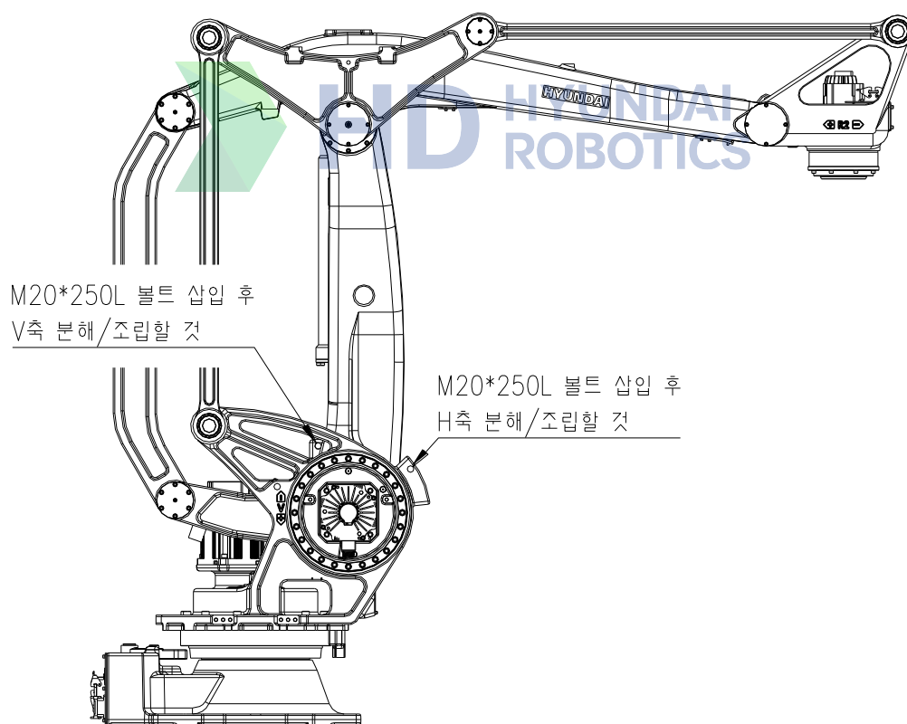
그림 6.1 H, V 축 ARM 낙하 방지 방법(HP160)
