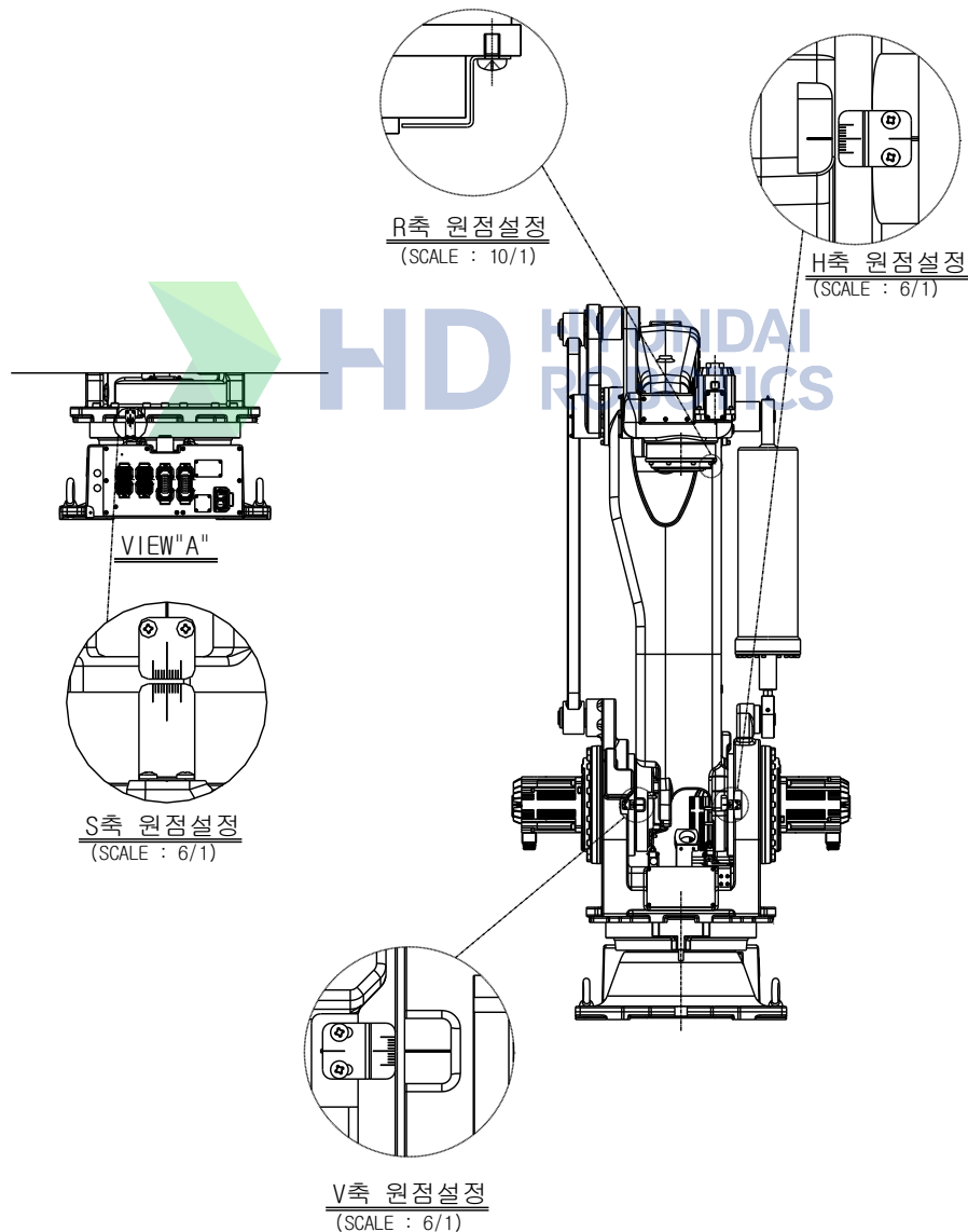
그림 6.5 원점 설정 방법
