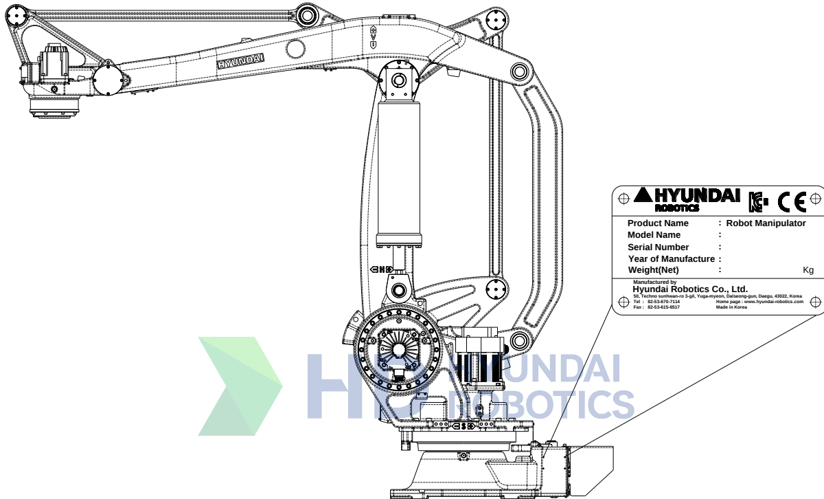
그림 2.2 로봇 명판 부착 위치
