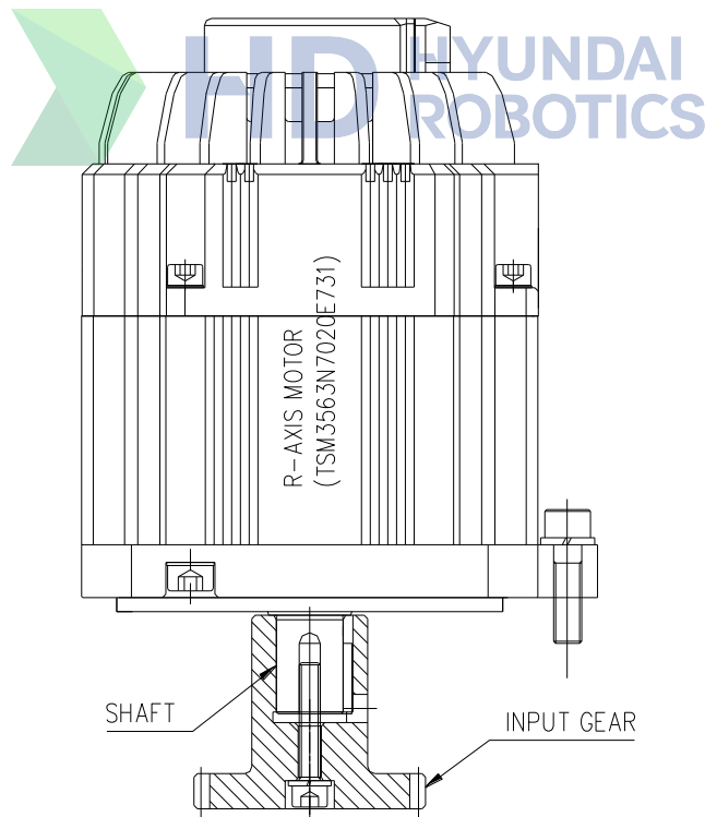
그림 6.4 손목축 모터 ASSEMBLY
