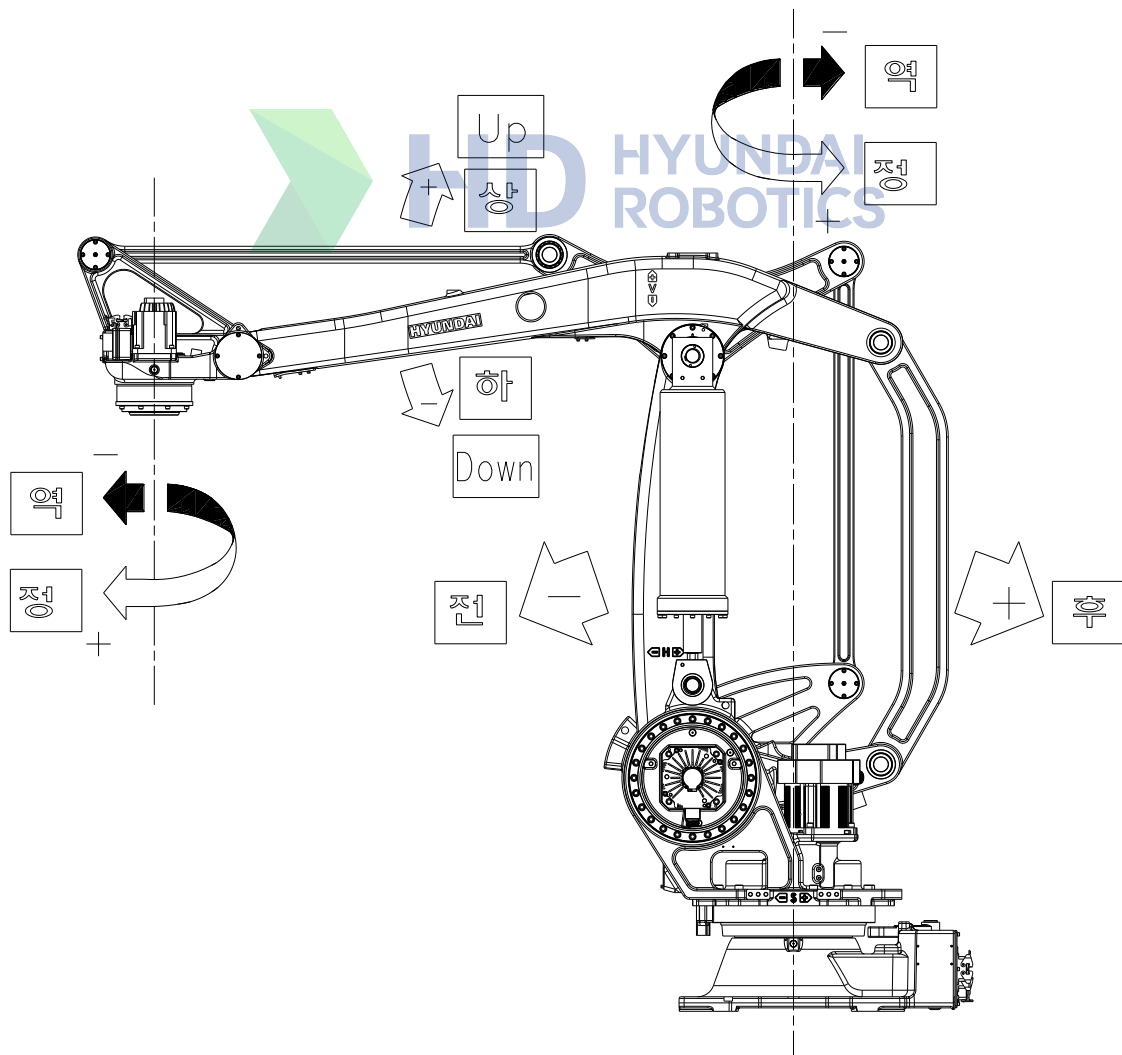
그림 2.4 본체 외관 및 동작 축
