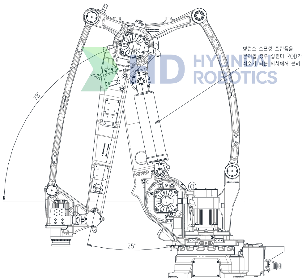
그림 8.1 밸런스 스프링 분리 자세
