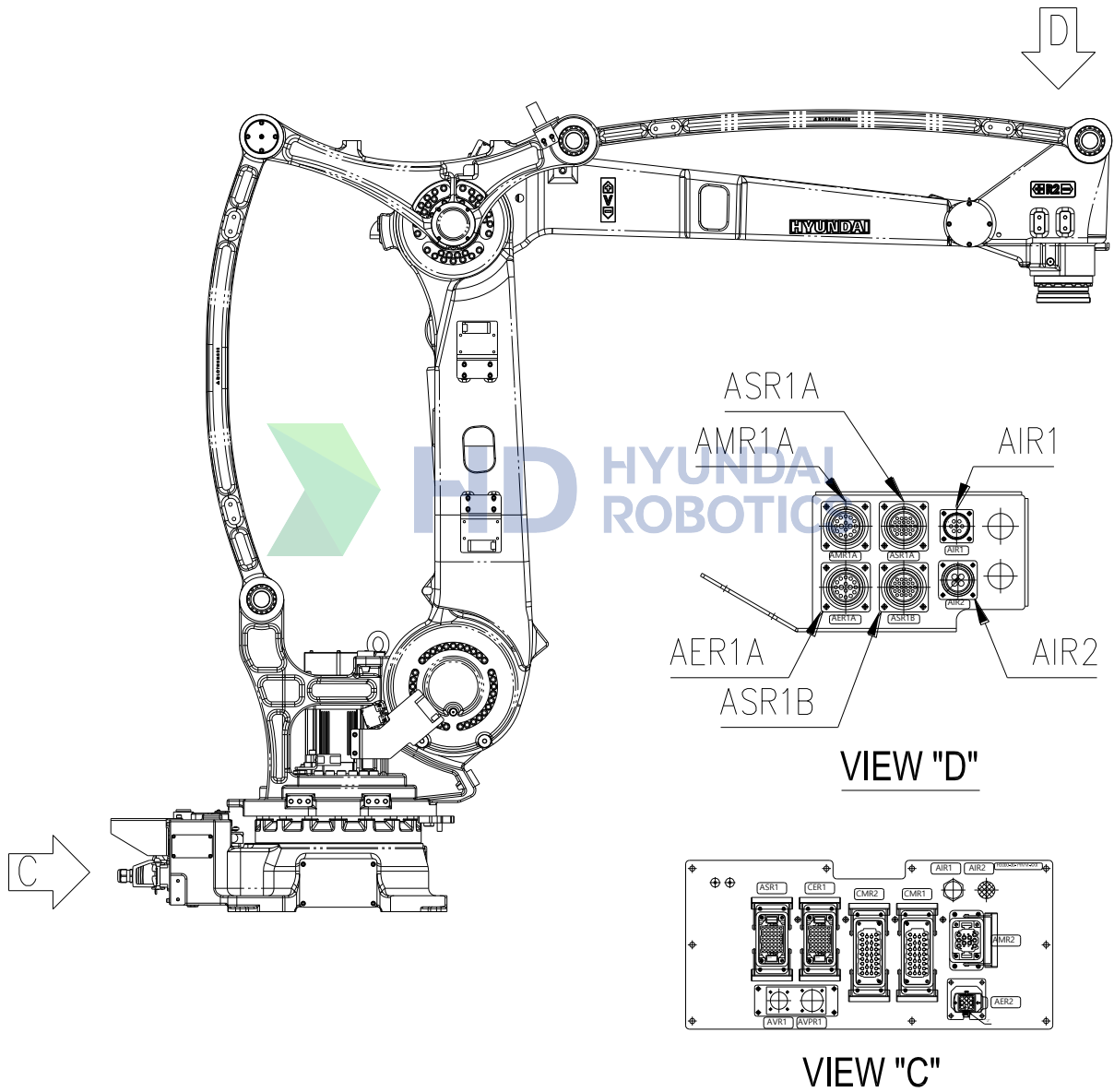
그림 2.5 어플리케이션용 배선 및 배관도
