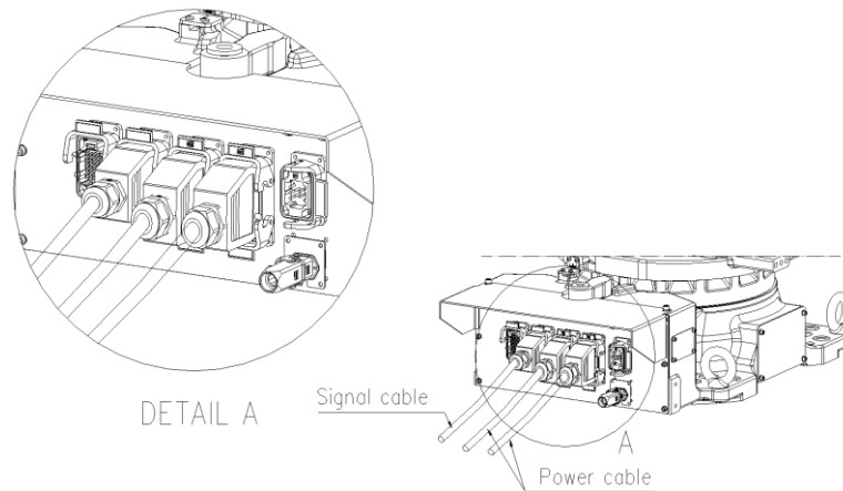
그림 3.7 로봇 Cable 연결
