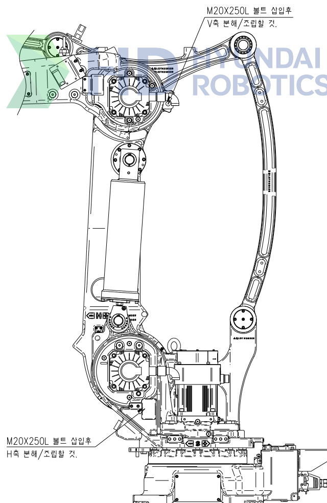
그림 6.1 H, V 축 ARM 낙하 방지 방법(HP130)
