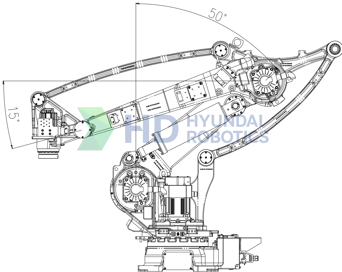
그림 3.9 권장 대기 자세
