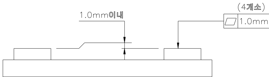
그림 3.4 로봇 설치면 정도
