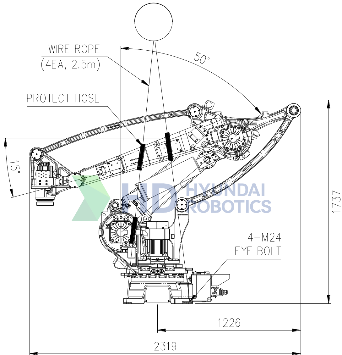
그림 3.3 운송 방법: 크레인 이용
