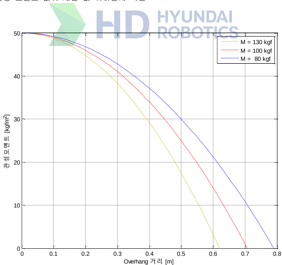
그림 3.6 손목축 부하조건
