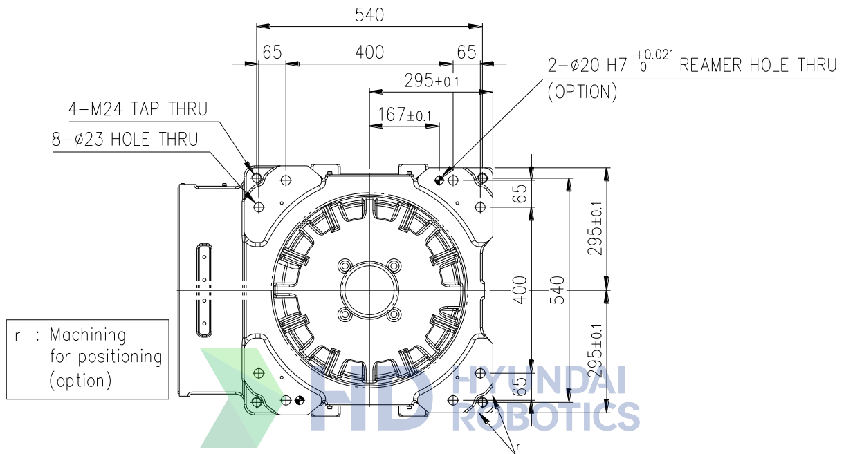
그림 3.5 로봇 본체 설치 치수
