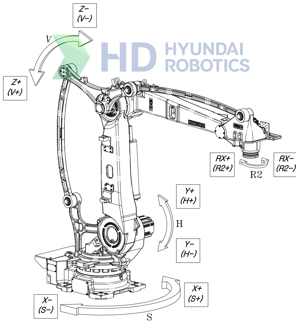
그림 2.4 본체 외관 및 동작 축
