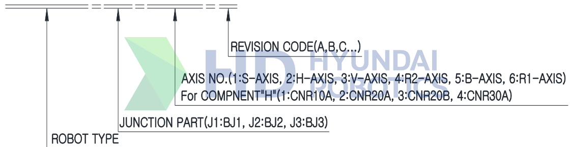
그림 5.1 본체 내 배선 기호 설명
