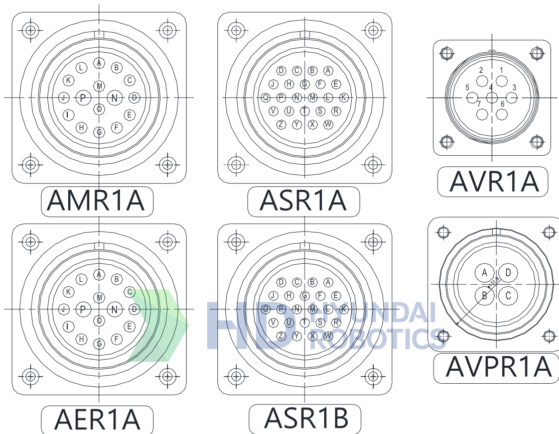
그림 2.6 어플리케이션 커넥터 상세도
