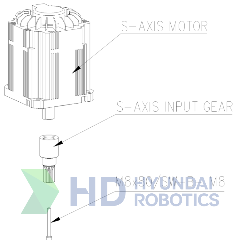
그림 6.2 S 축 모터 ASSEMBLY
