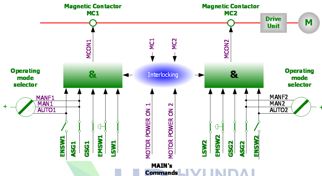
그림 1.5 안전체인 구성도
