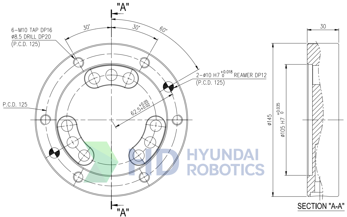
그림 2.7 손목축 취부면 상세도
