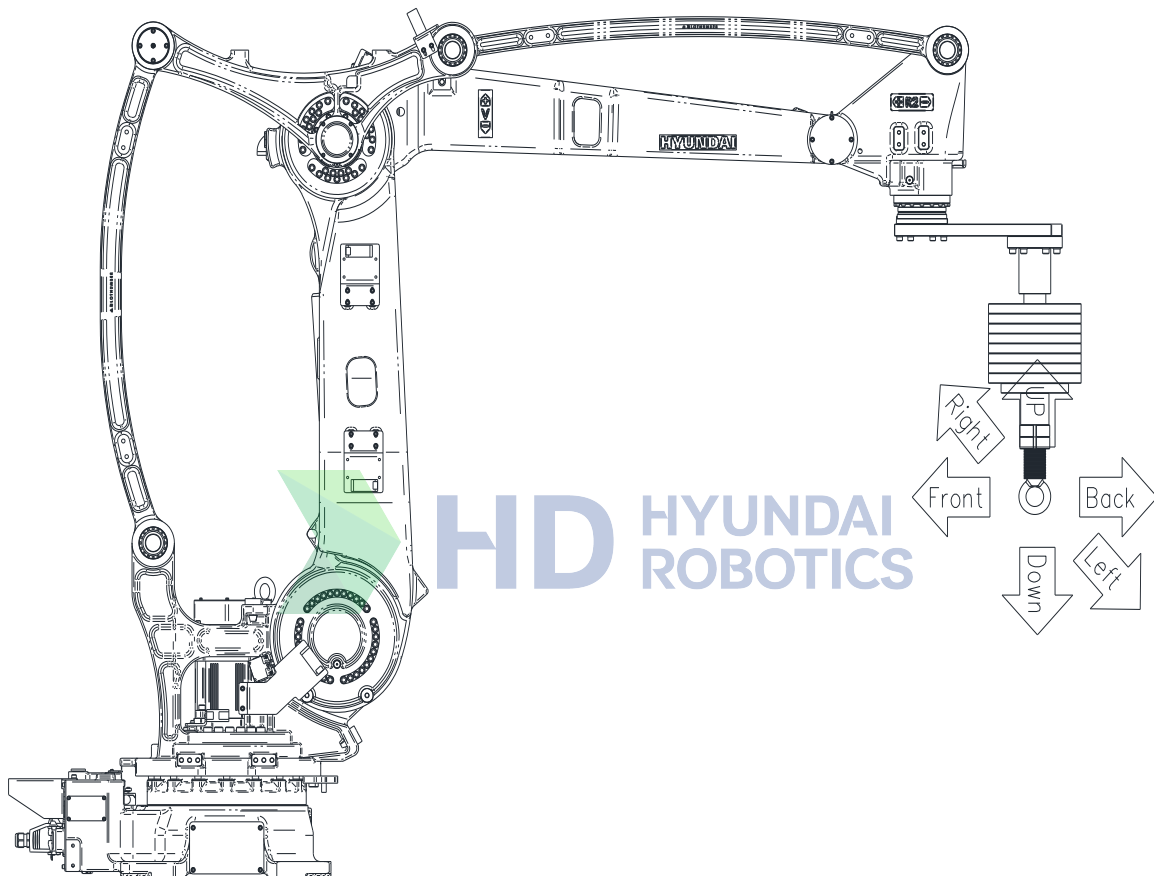
그림 4.2 유격 점검 방향
