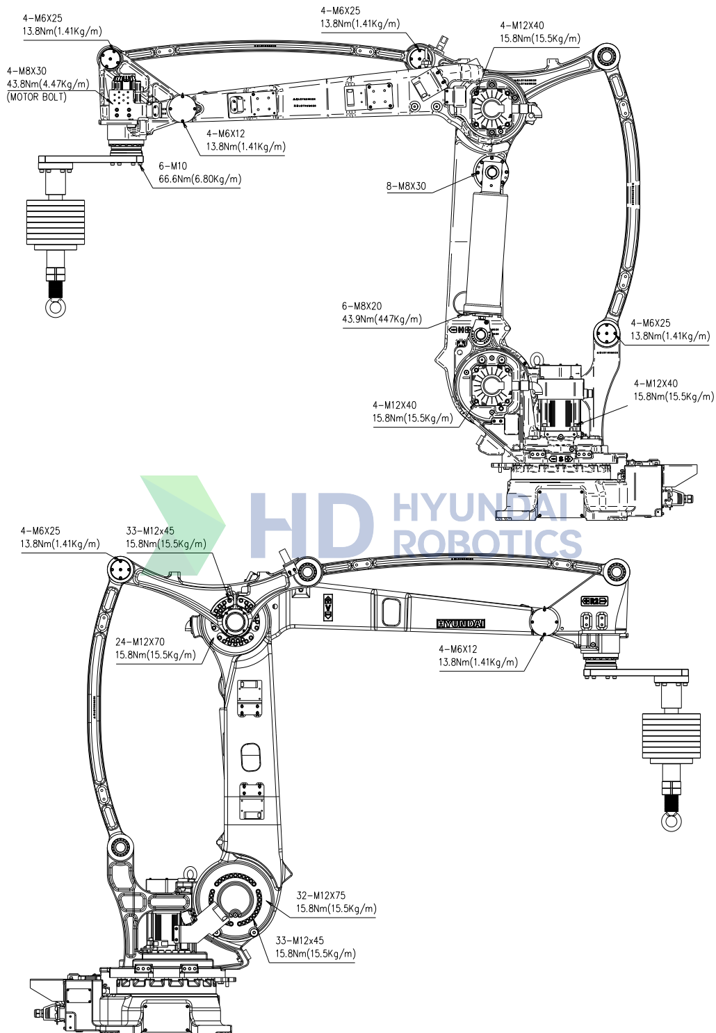
그림 4.1 주요 볼트 점검 부위
