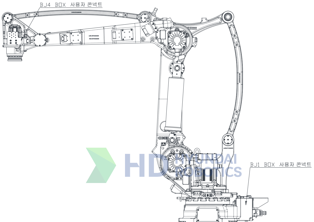
그림 9.1 본체 부품 배치
