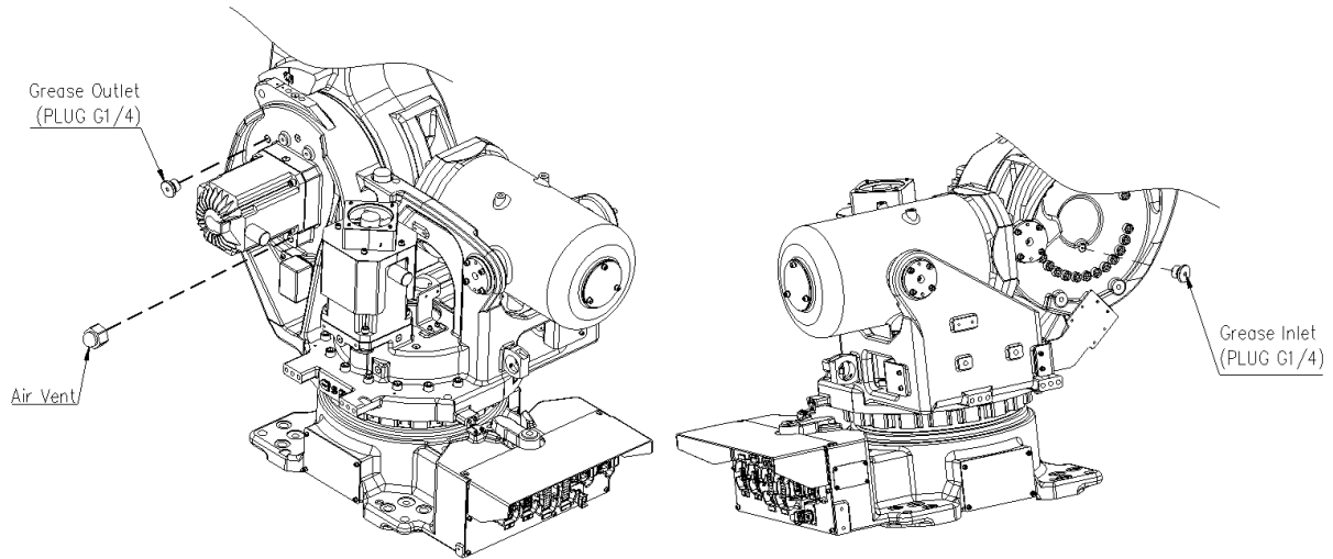
그림 5.2 H 축 감속기 그리스 주입/배출구
