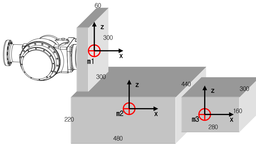
그림 3.14 3 차원 부하 모델 3D 형상
