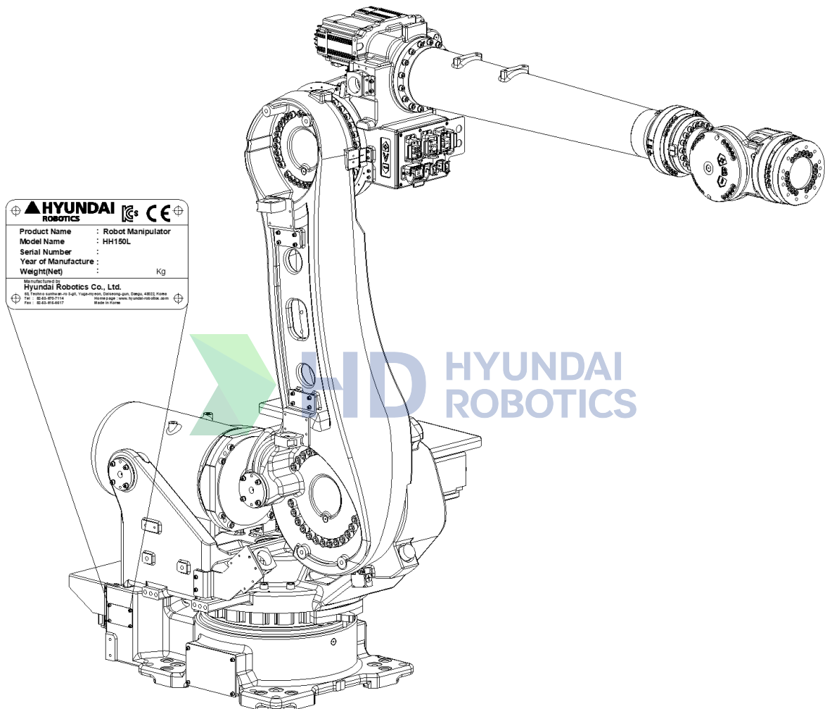
그림 2.2 로봇 명판 부착 위치
