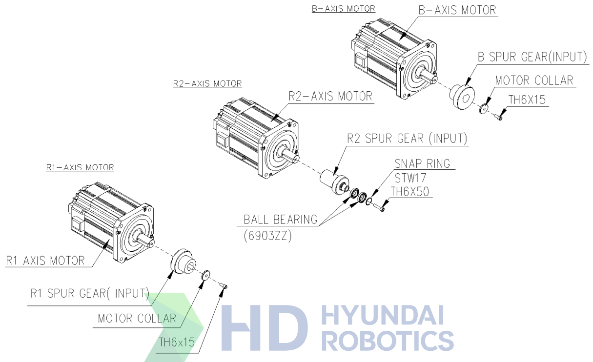
그림 6.5 손목축 모터 ASSEMBLY
