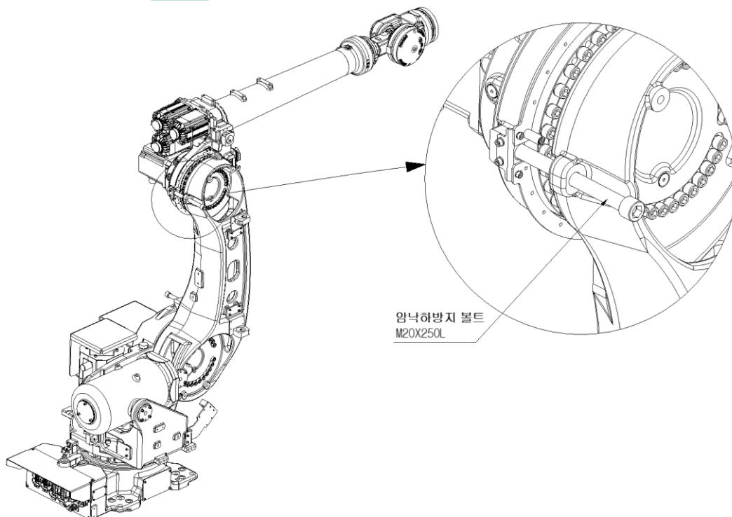
그림 6.2 암(V 축) 고정용 볼트 삽입 위치
