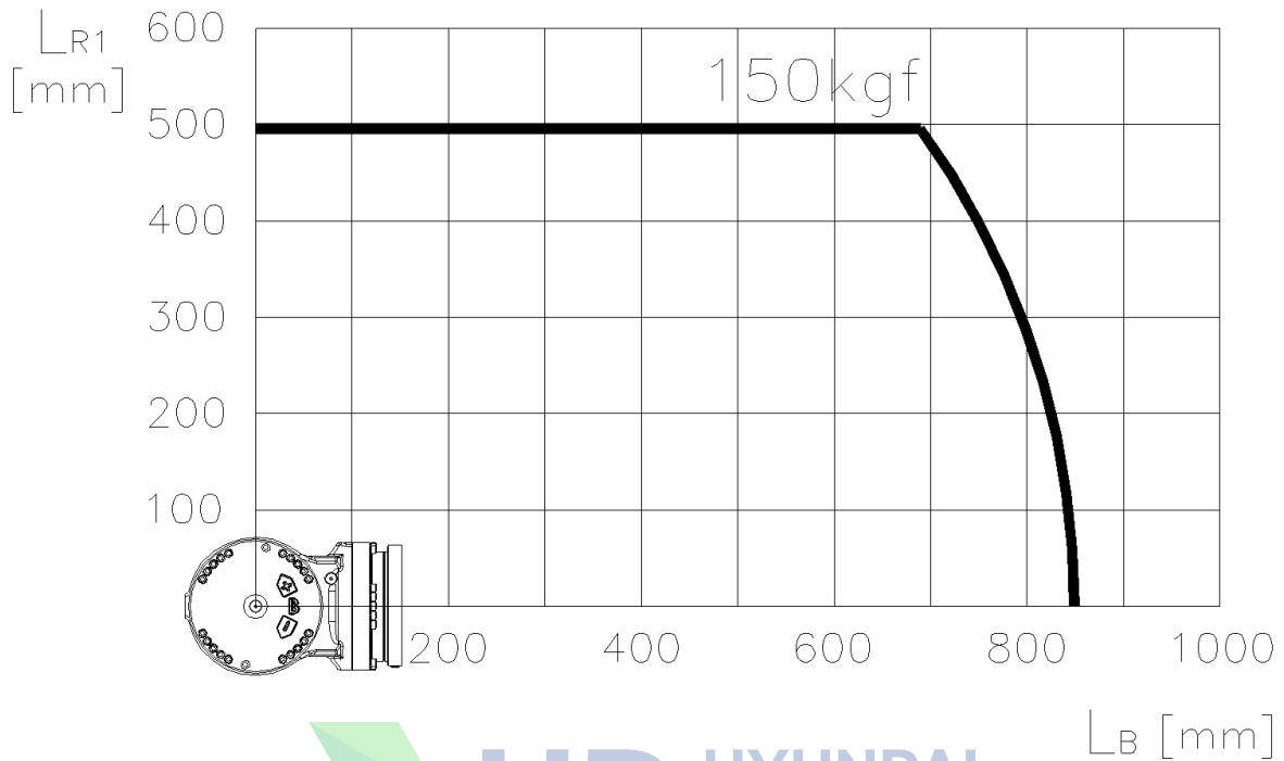
그림 3.10 손목축 토크 선도 (HH150L)
