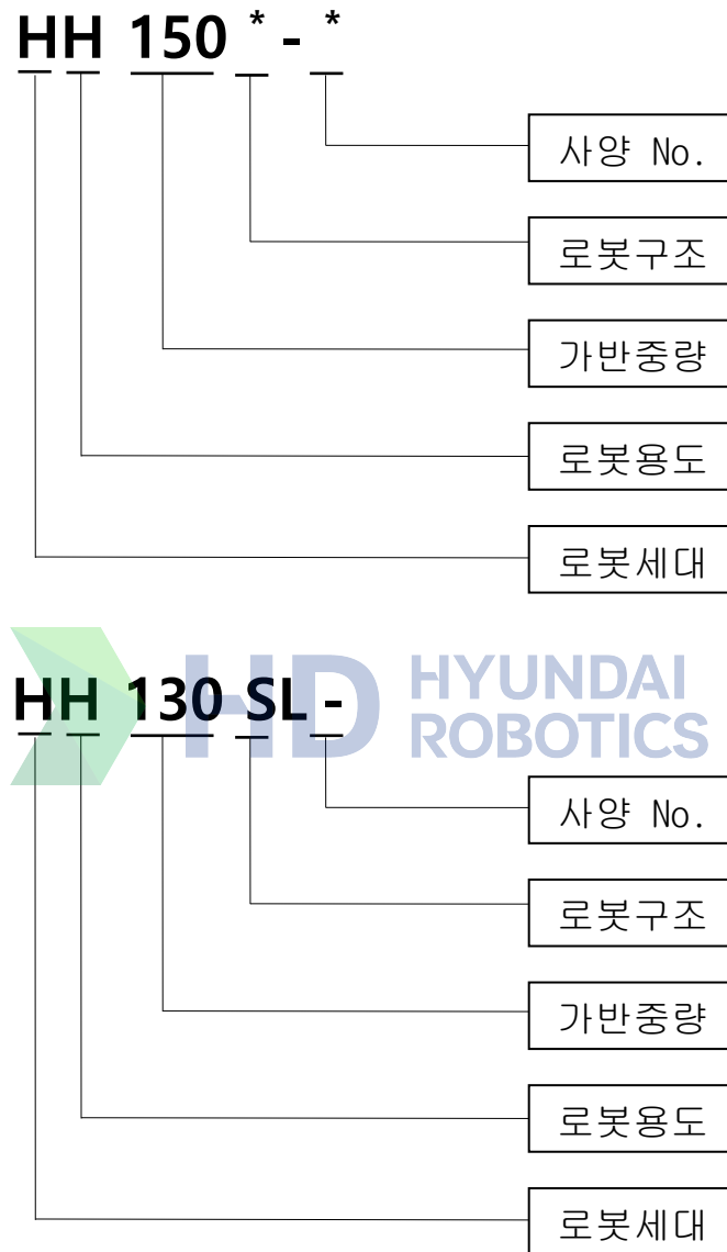
그림 2.1 로봇 기구부 형식
