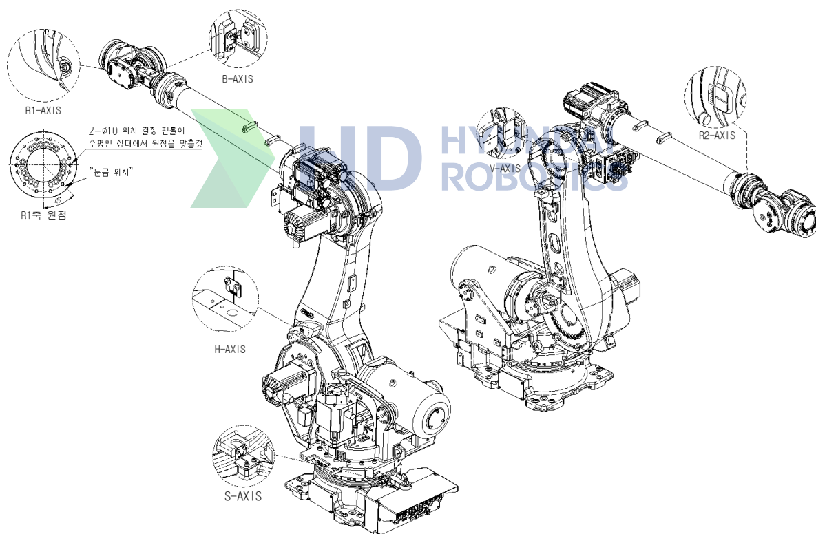
그림 6.6 원점 설정 방법
