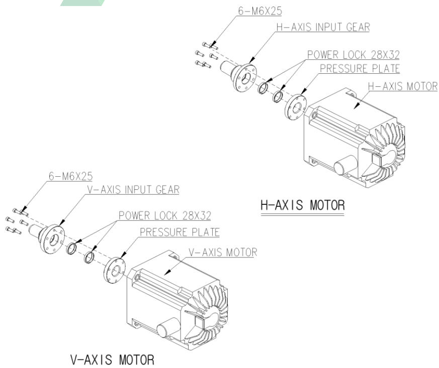
그림 6.4 H&V 축 모터 ASSEMBLY
