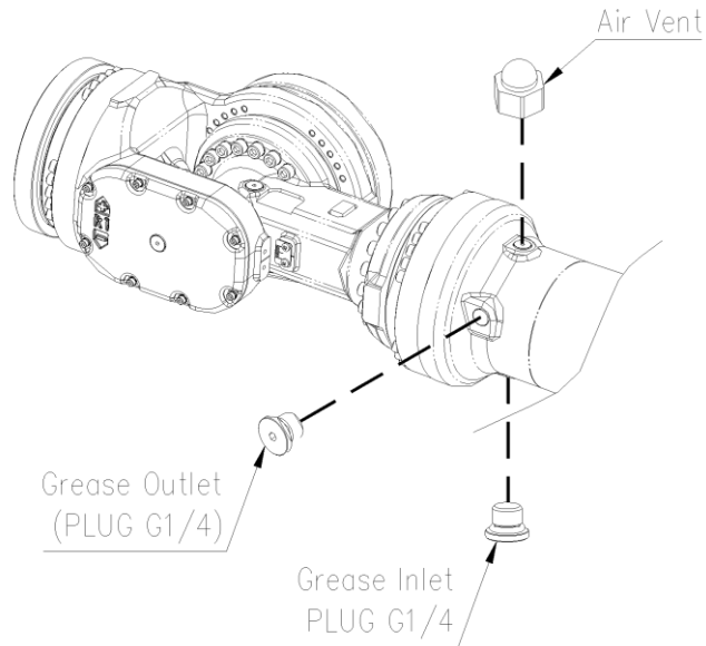
그림 5.4 R2 축 감속기 그리스 주입/배출구
