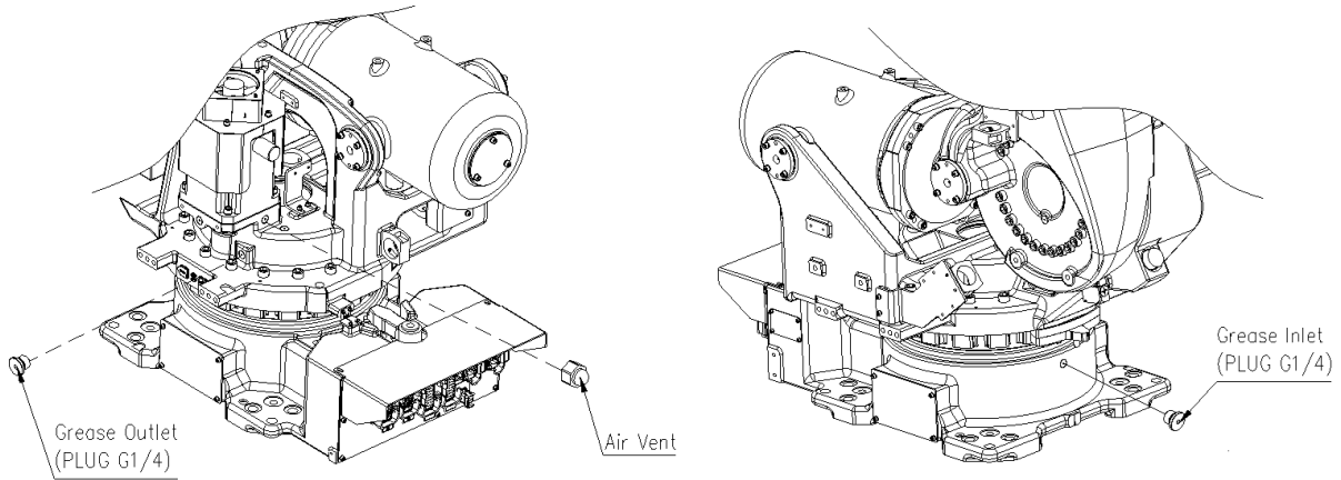
그림 5.1 S 축 감속기 그리스 주입/배출구
