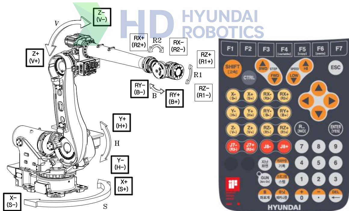
그림 2.5 본체 외관 및 동작 축
