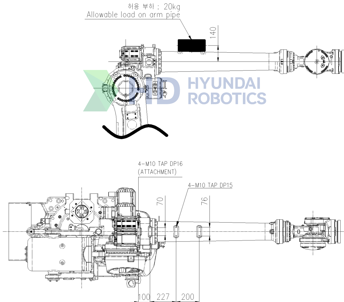
그림 2.7 ARM FRAME 상부 부착부 상세도
