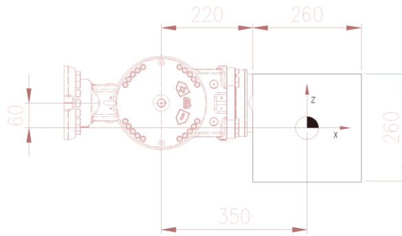
그림 3.12 2 차원 부하 모델
