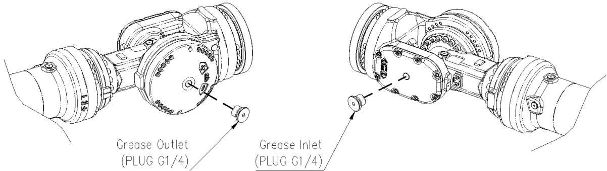
그림 5.5 B 축 감속기 그리스 주입/배출구
