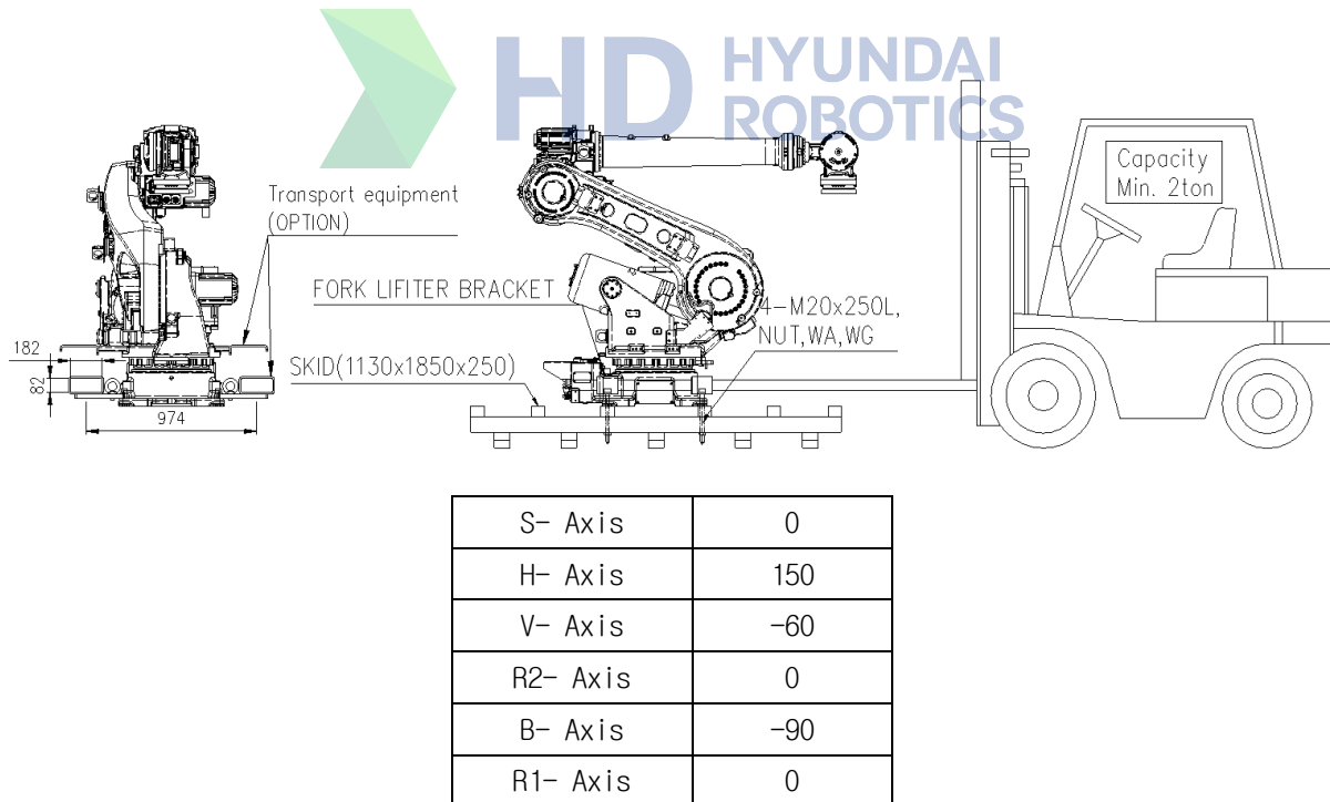
그림 3.6 운송 방법 : 지게차 이용
