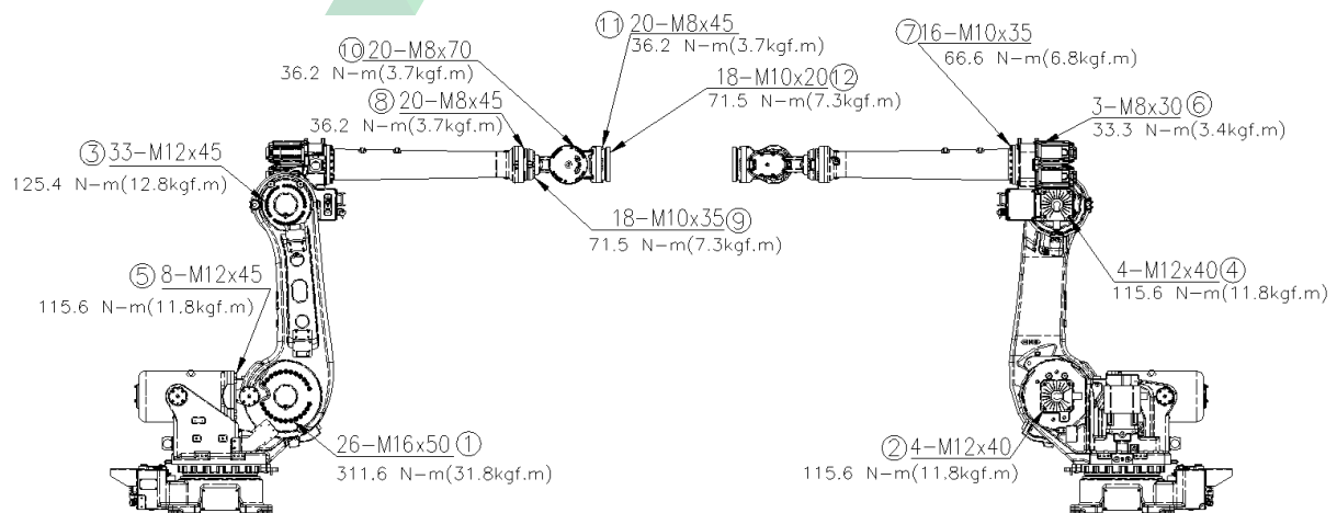
그림 4.1 주요 볼트 점검 부위
