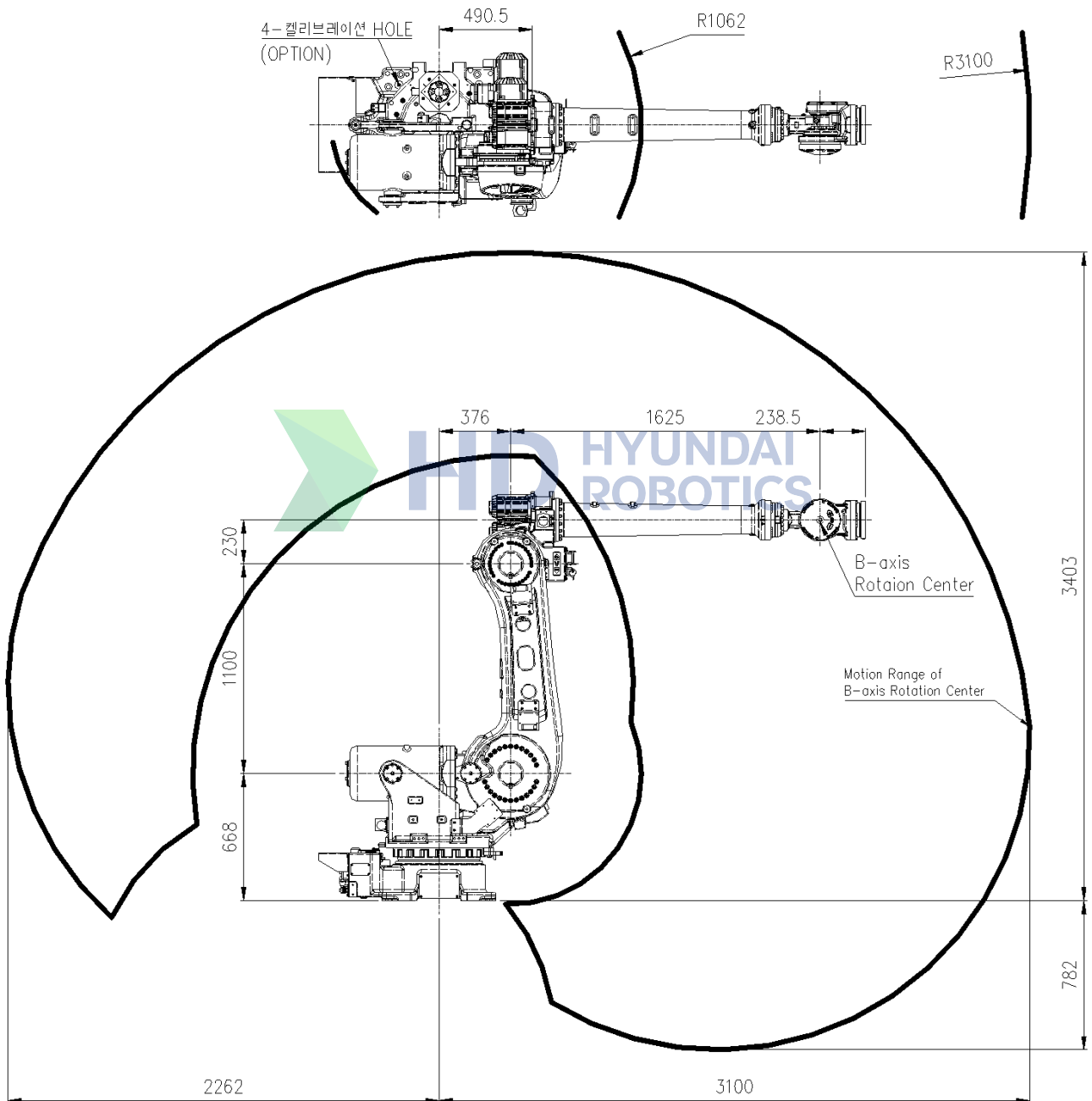
그림 2.3 로봇 본 외형 치수 및 동작 영역 (HH150L)
