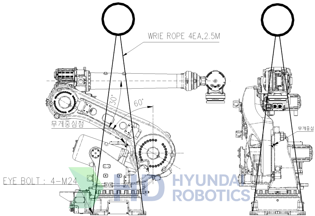
그림 3.4 운송 방법 : 크레인 이용 (HH150L)
