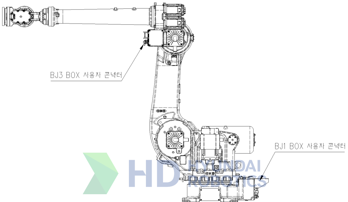
그림 9.1 본체 부품 배치
