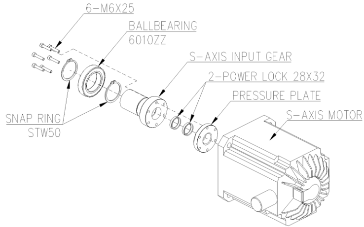
그림 6.3 S 축 모터 ASSEMBLY
