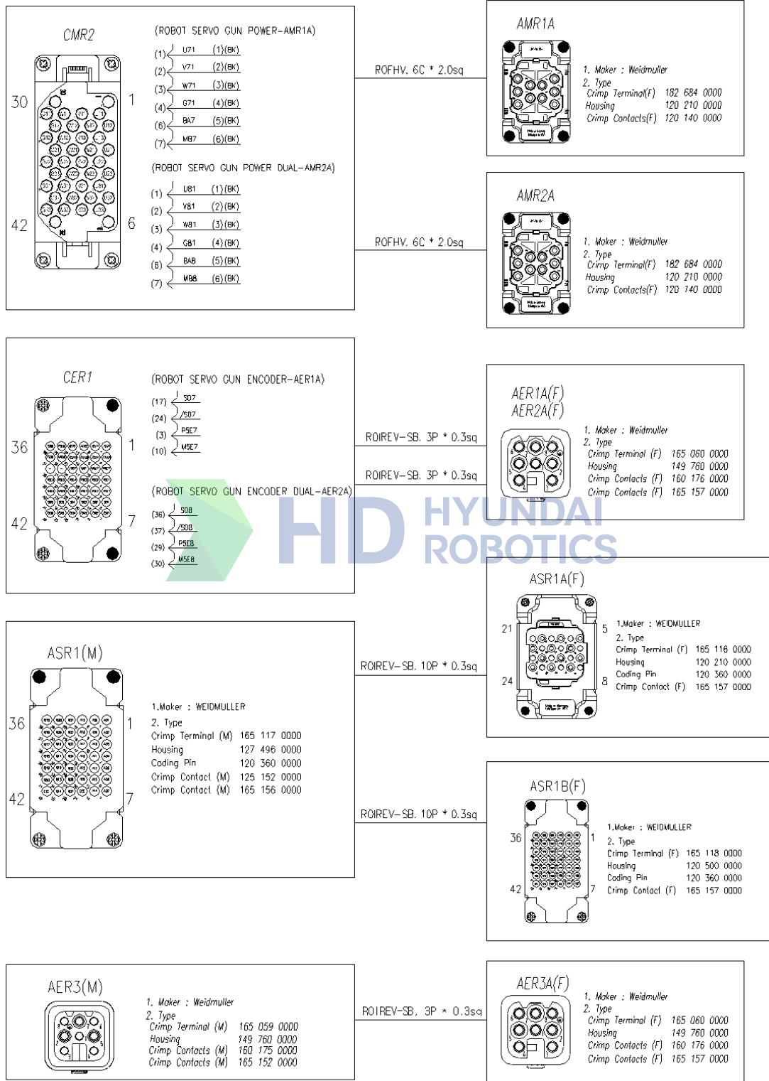
그림 2.9 어플리케이션 커넥터 상세
