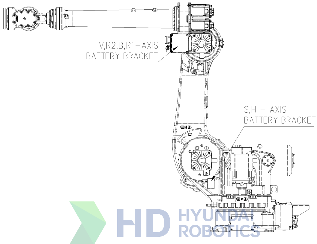
그림 5.8 배터리 교환 위치
