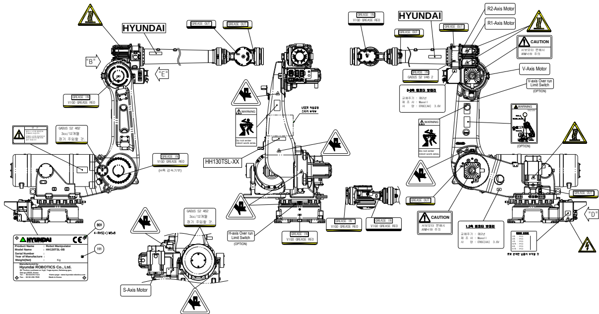
그림 3.3 안전 명판 위치 (HH130SL)
