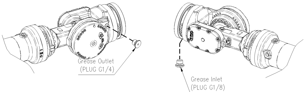
그림 5.6 R1 축 감속기 그리스 주입/배출구
