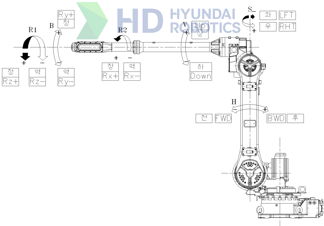
그림 2.4 본체 외관 및 동작 축 [HH020L]
