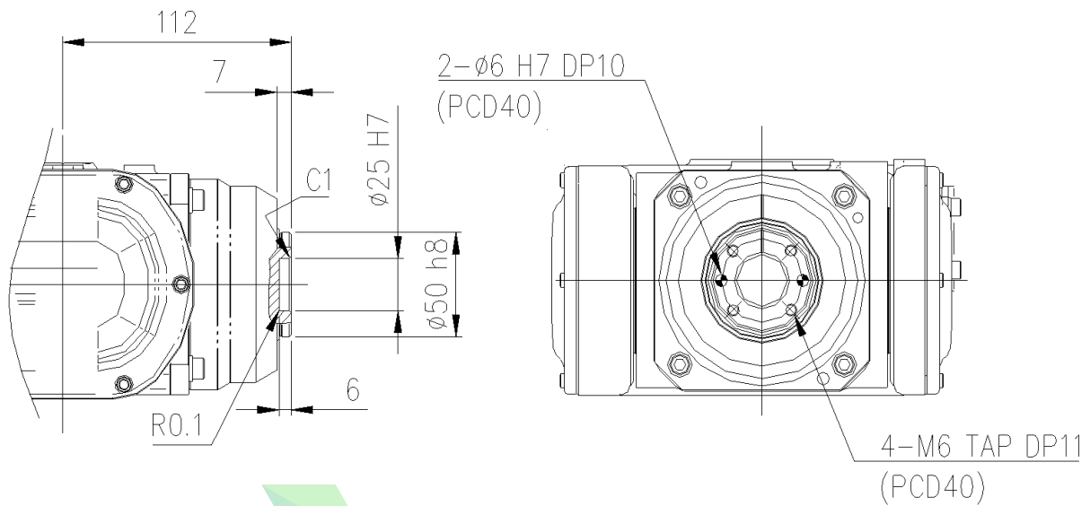
그림 2.5 손목축 취부면 상세도 [HH020L]
