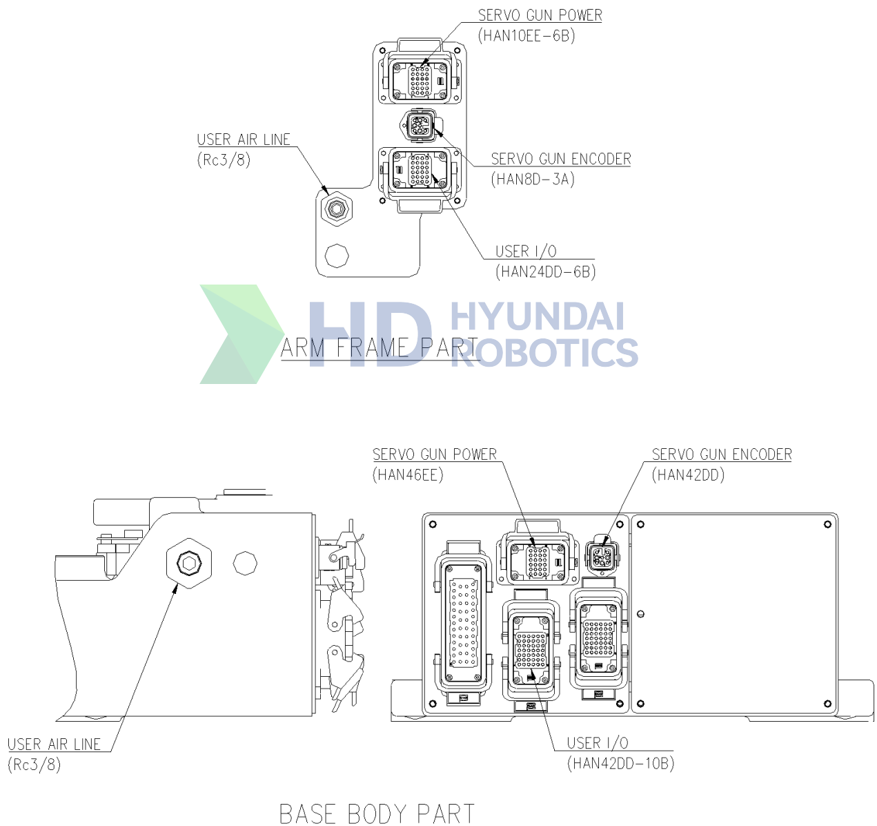
그림 2.7 어플리케이션용 배선 및 배관도 [HH020L]
