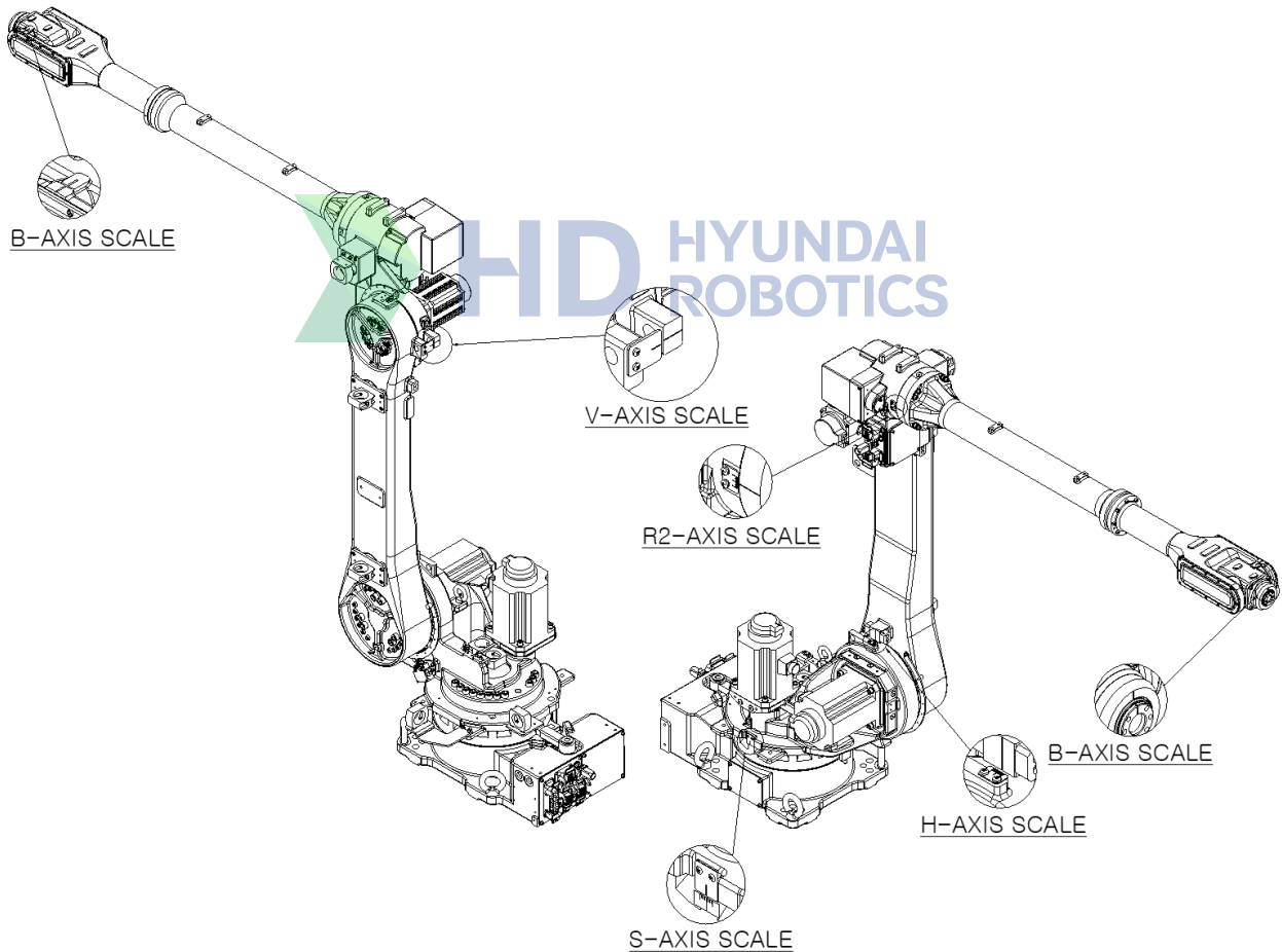
그림 6.7 원점 설정 방법 [HH020L]
