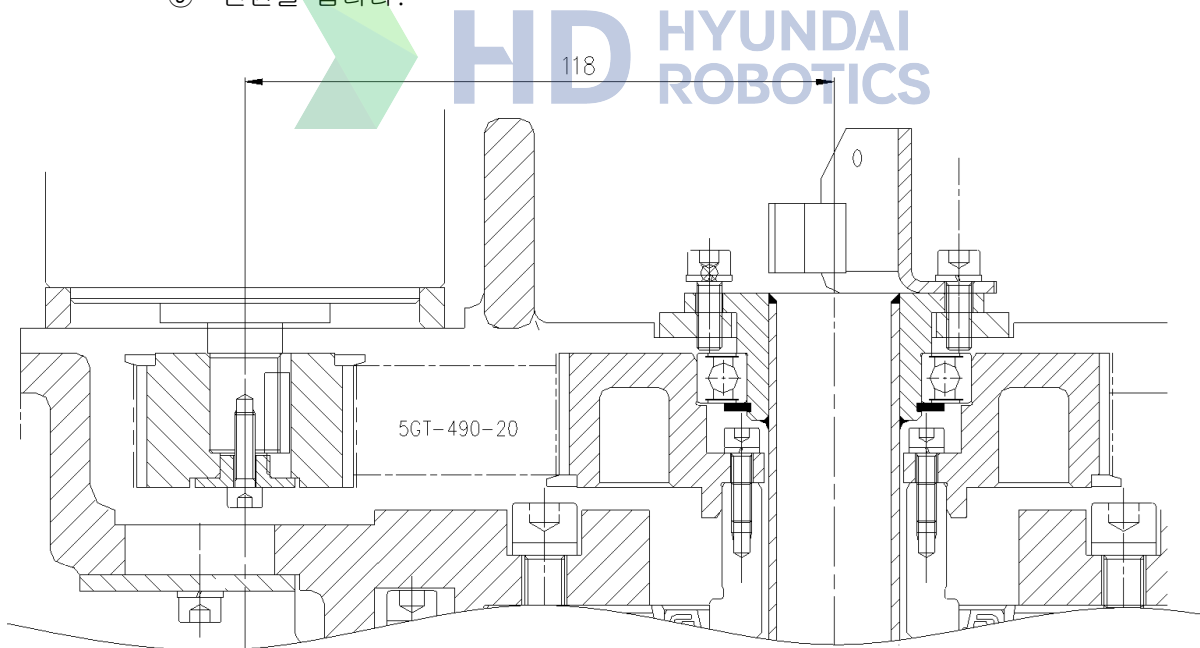
그림 4.2 R2 축 타이밍 벨트 장력 체크 부위 [HH020L]
