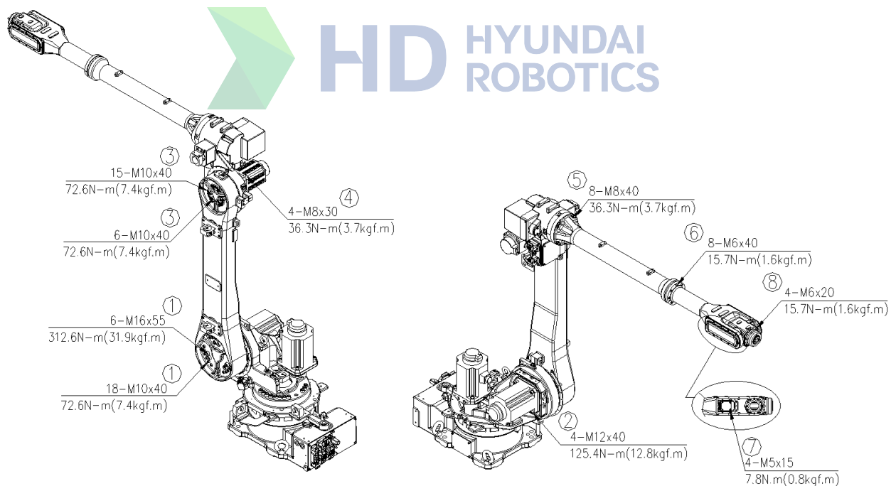
그림 4.1 주요 볼트 점검 부위 [HH020L]
