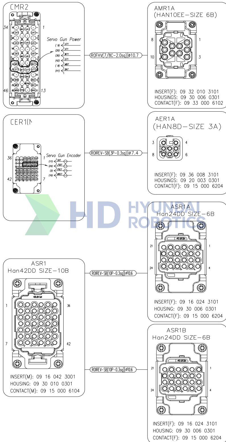
그림 2.8 어플리케이션 커넥터 상세 [HH020L]
