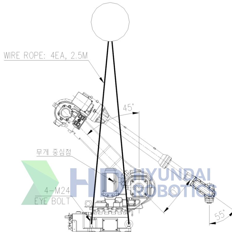
그림 3.3 운송 방법 : 크레인 이용 [HH020L]
