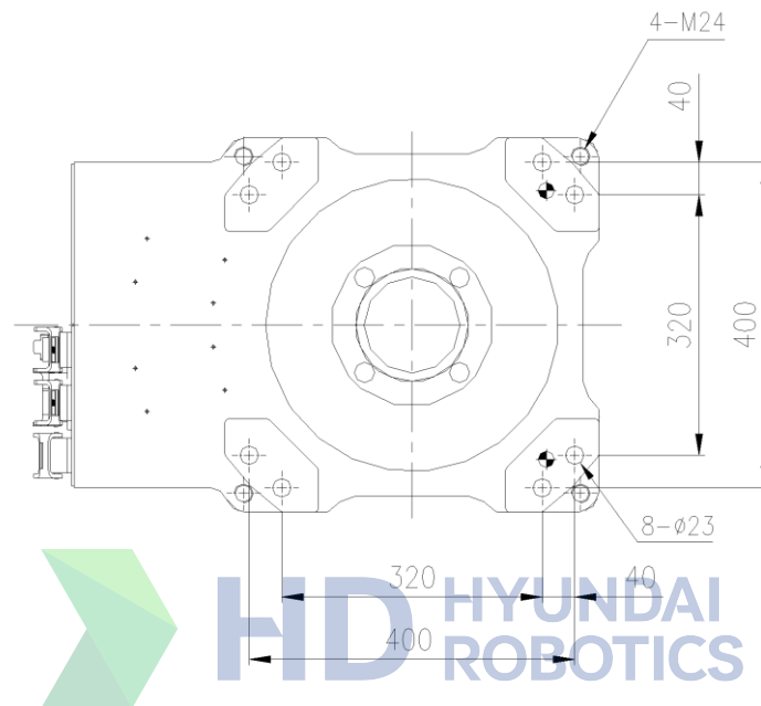
그림 3.6 로봇 설치면 치수 [HH020L]
