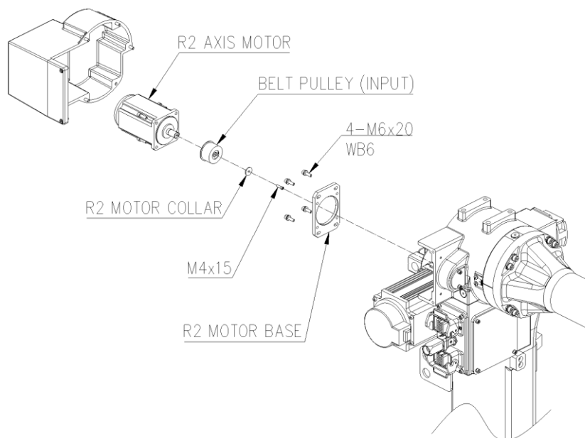
그림 6.4 R2 축 모터 ASSEMBLY
