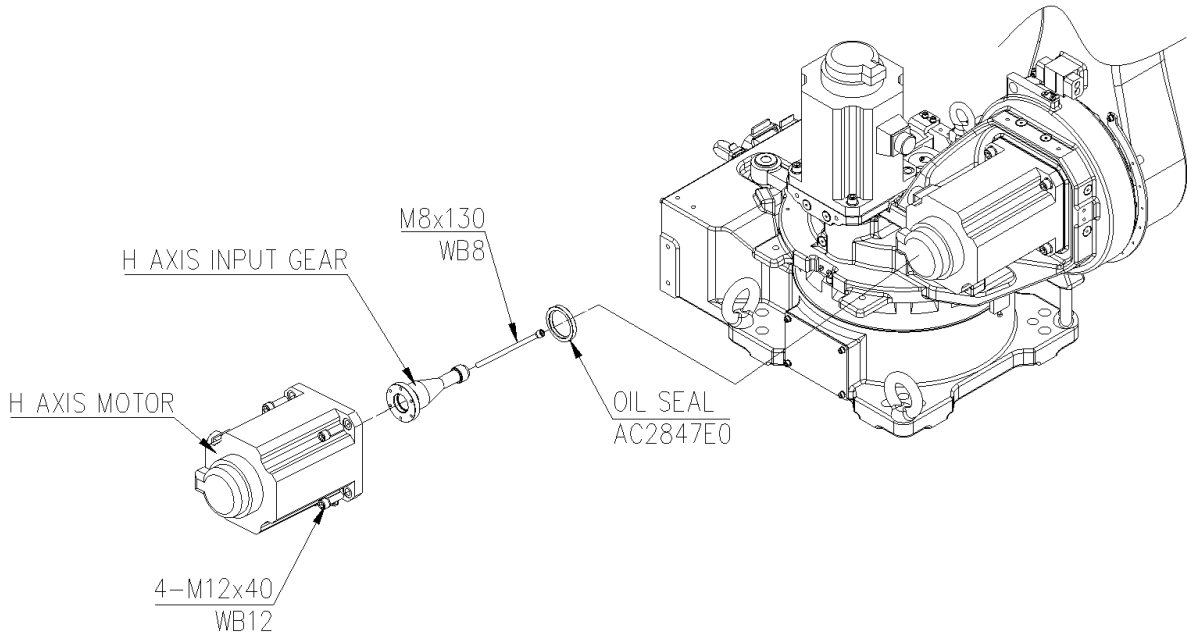
그림 6.2 H 축 모터 ASSEMBLY
