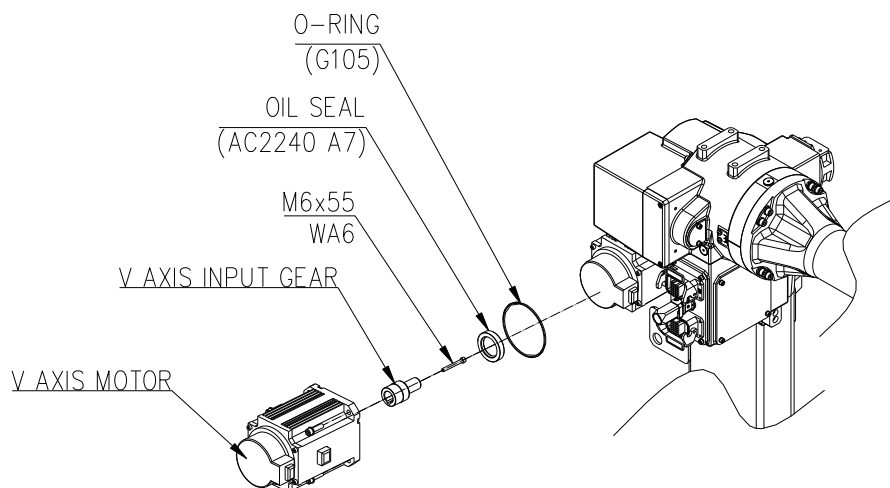
그림 6.3 V 축 모터 ASSEMBLY
