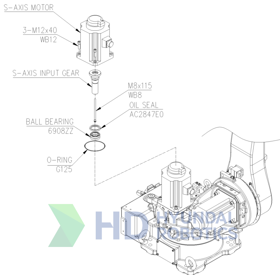
그림 6.1 S 축 모터 ASSEMBLY
