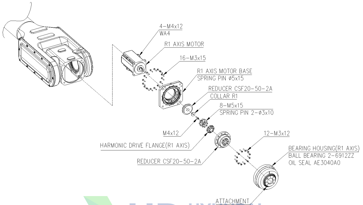
그림 6.6 R1 축 모터 ASSEMBLY
