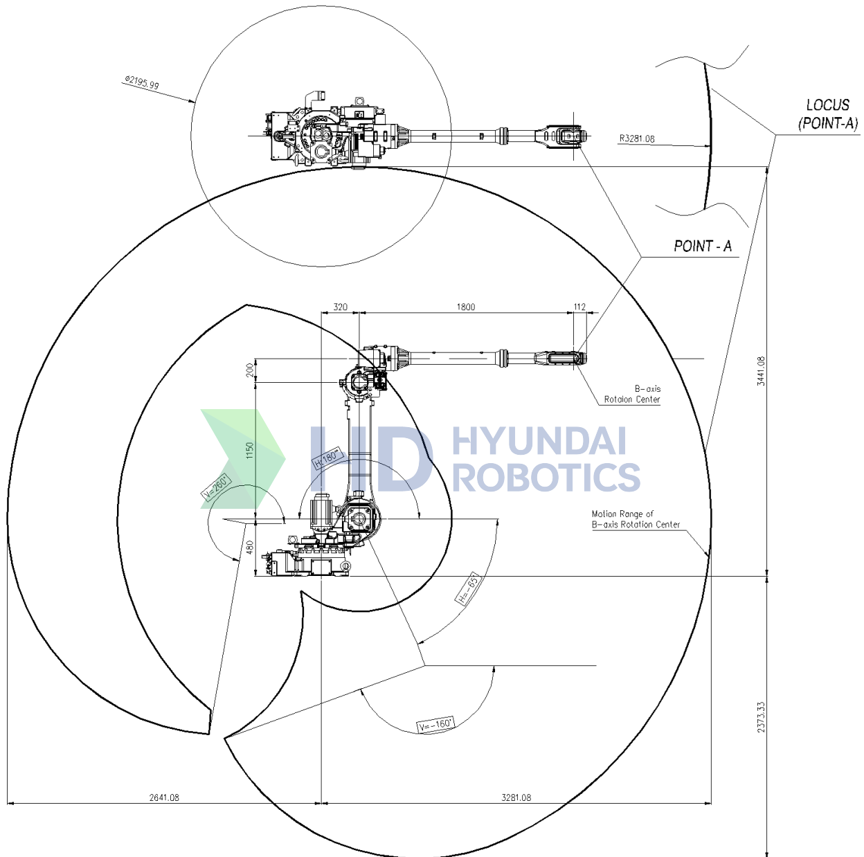
그림 2.3 로봇 본체 외형 치수 및 동작 영역 [HH020L]
