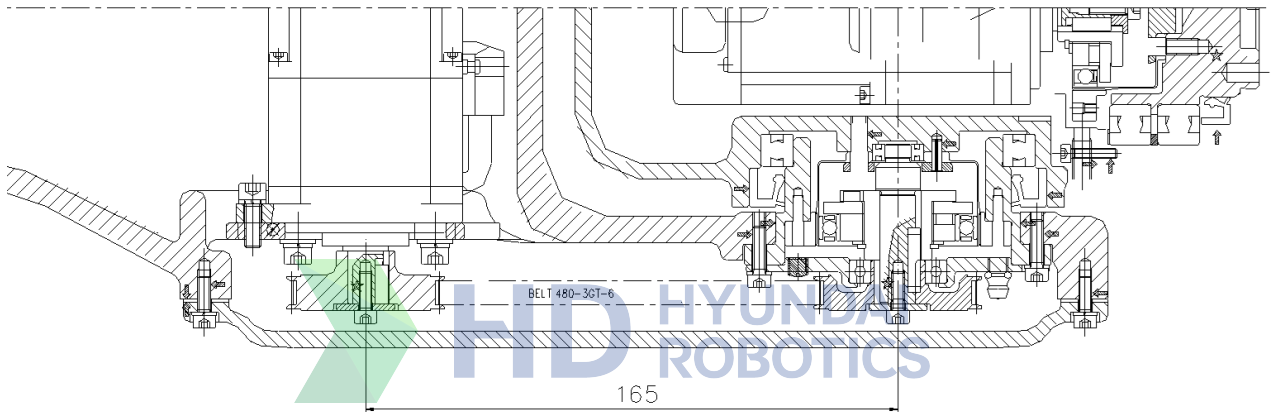
그림 4.3 B 축 타이밍 벨트 장력 체크 부위 [HH020L]
