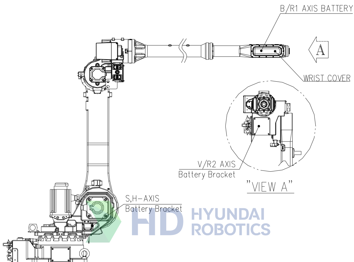
그림 5.1 배터리 교환 위치
