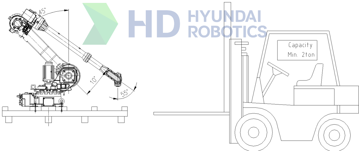
그림 3.4 운송 방법 : 지게차 이용 [HH020L]
