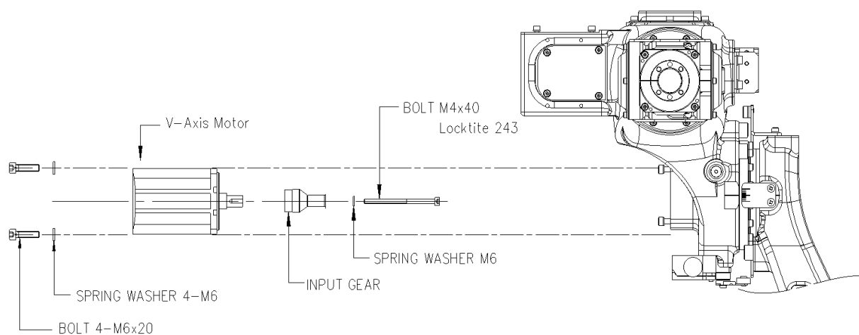
그림 6.5 V 축 모터 교체 [HH012]
