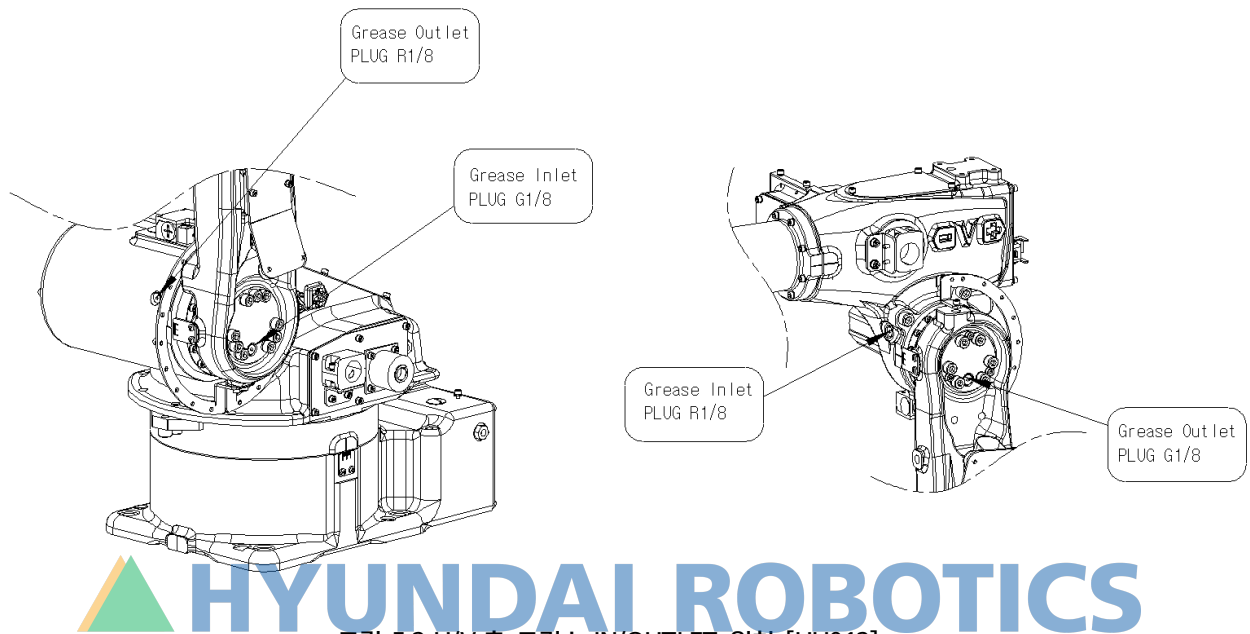
그림 5.2 H/V 축 그리스 IN/OUTLET 위치 [HH012]
