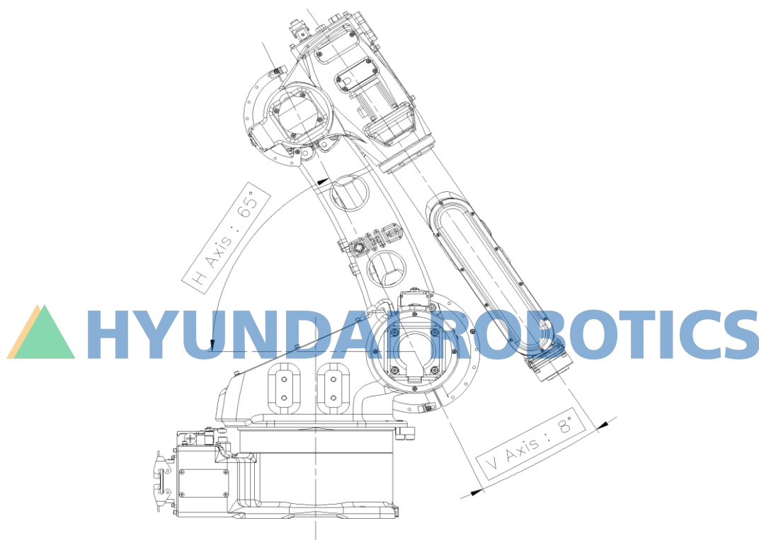
그림 6.4 V 축 모터 교체시의 로봇 자세 [HH012]
