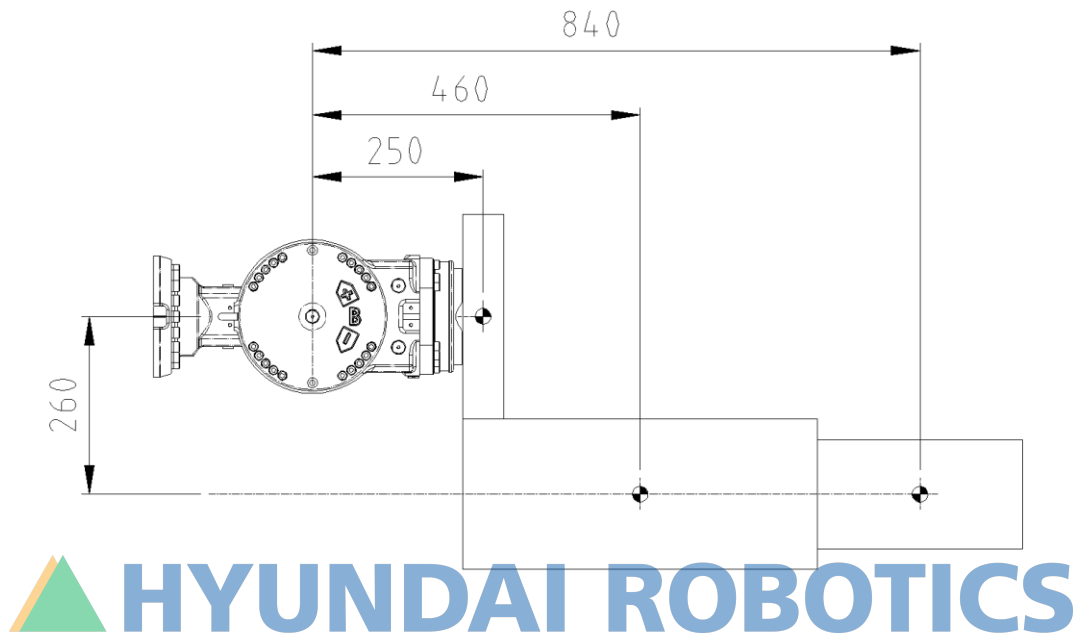
그림 3.8 3 차원 부하 모델 2D 형상
