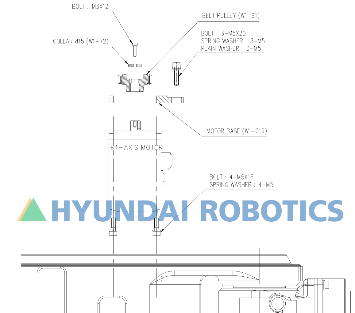
그림 6.7 B/R1 축 모터교체 (HH012)
