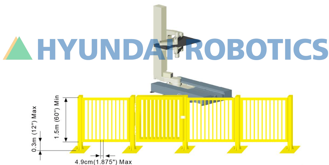
그림 1.1 권장 펜스 크기와 출입구 크기(슬롯형 출입구)
