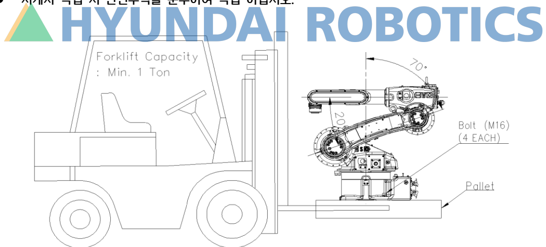
그림 3.4 운반 방법: 지게차 이용 [HH012]
