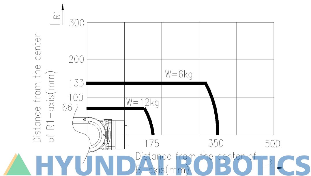
그림 3.10 손목축 토크 선도
