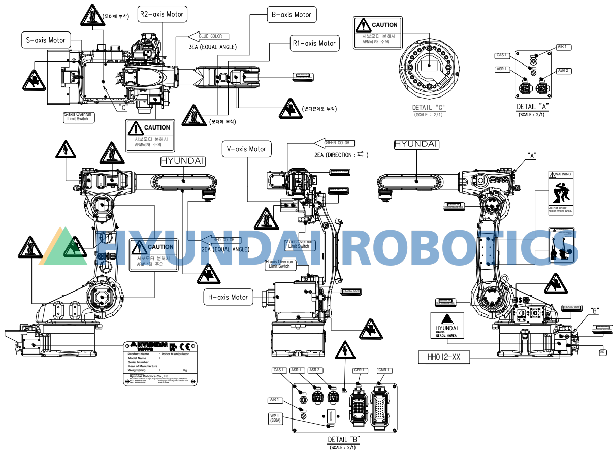
그림 3.2 안전 명판 위치 [HH012]
