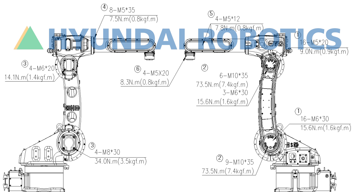
그림 4.1 주요 볼트 점검 부위 [HH012]
