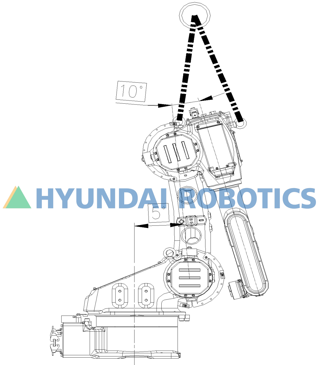
그림 6.10 H축 감속기 교체시의 로봇 자세 [HH012]
