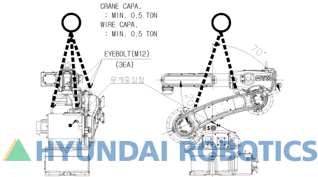
그림 3.3 운반 방법: 크레인 이용 [HH012]
