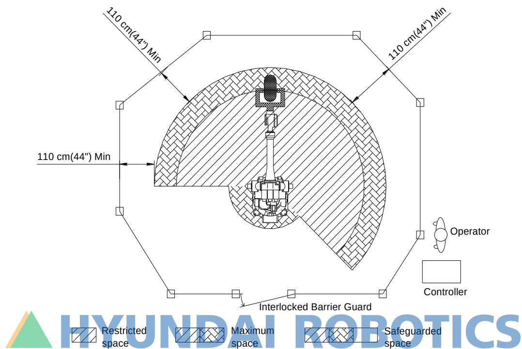
그림 1.4 산업용 로봇 주변장치와 작업자의 배치
