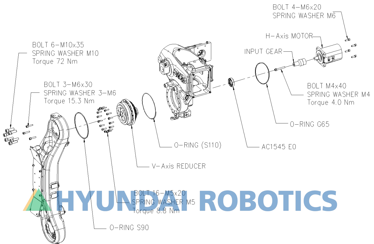
그림 6.13 V 축 감속기 분해도[HH012]
