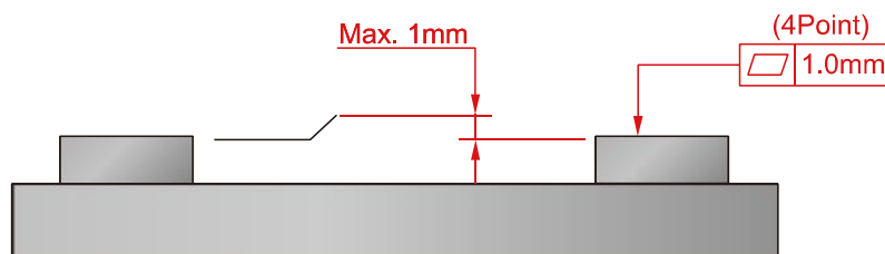
그림 3.6 로봇 설치면 정도
