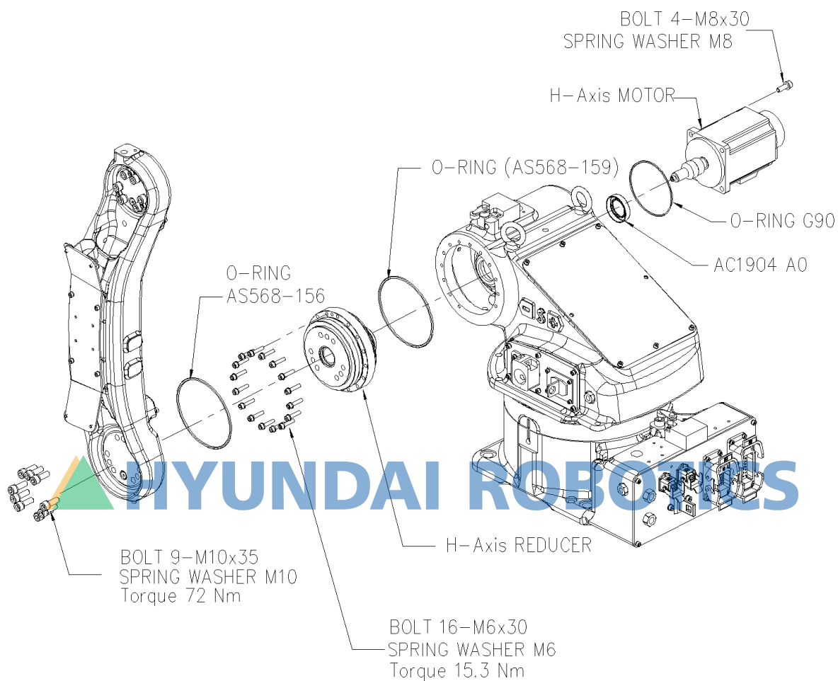
그림 6.11 H 축 감속기 분해도 [HH012]
