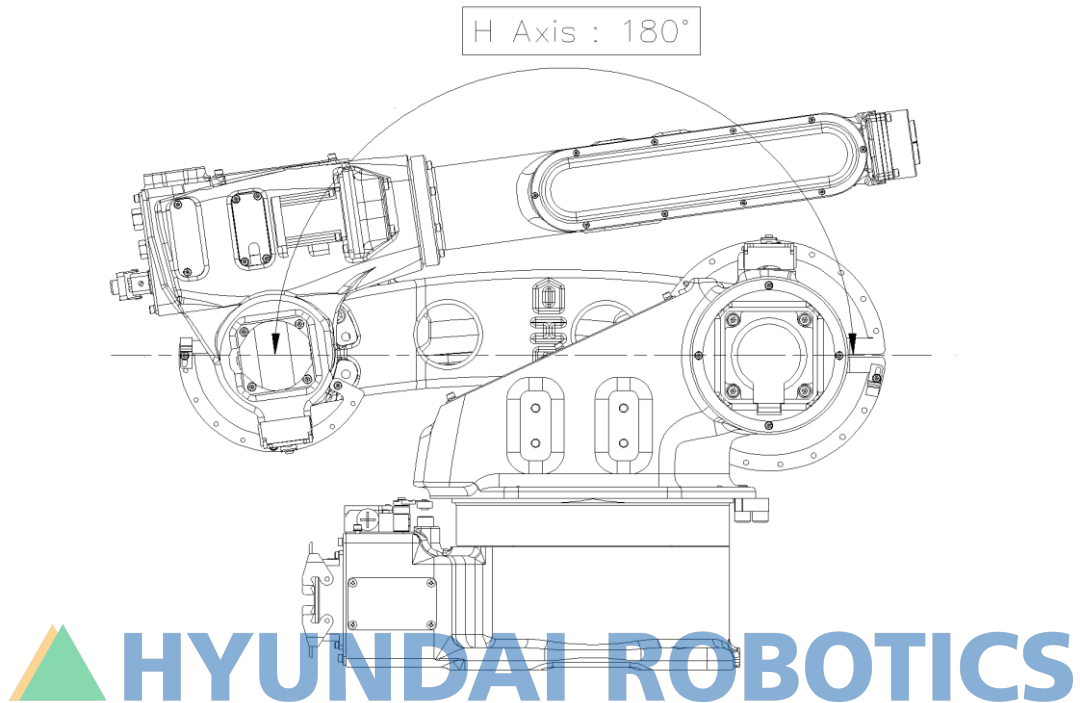
그림 6.2 H축 모터 교체시의 로봇 자세 [HH012]
