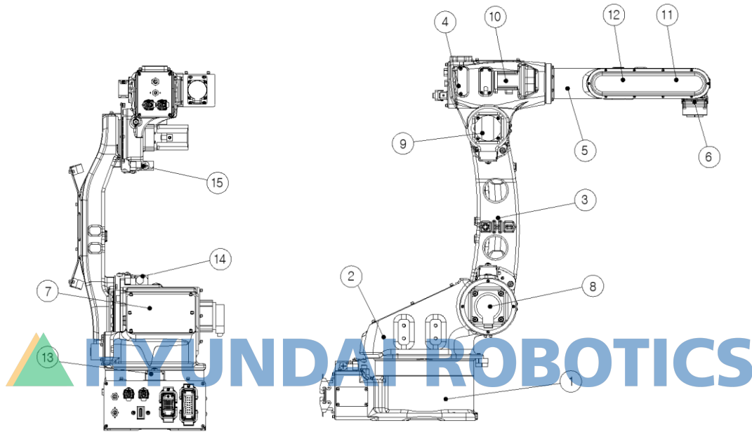
그림 3.1 본체 각 부위 명칭[HH012]
