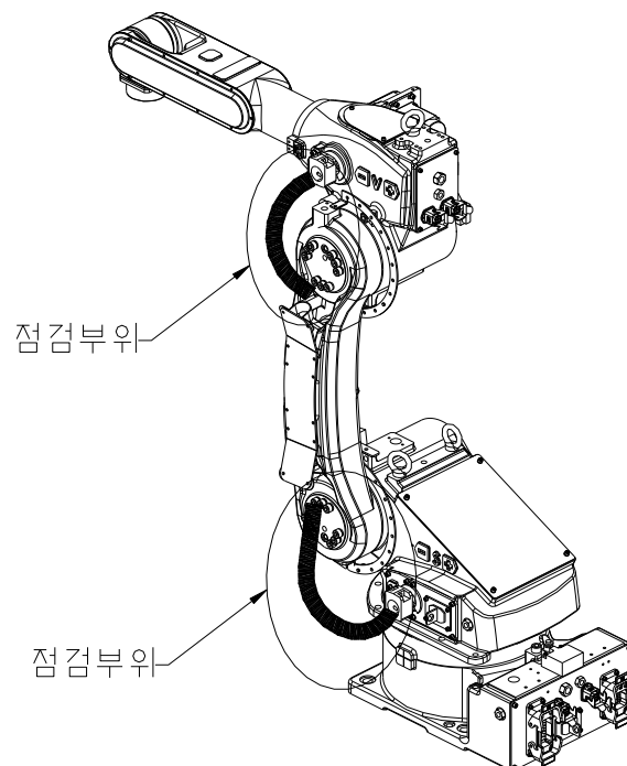
그림 4.2 케이블 점검 부위 [HH012]
