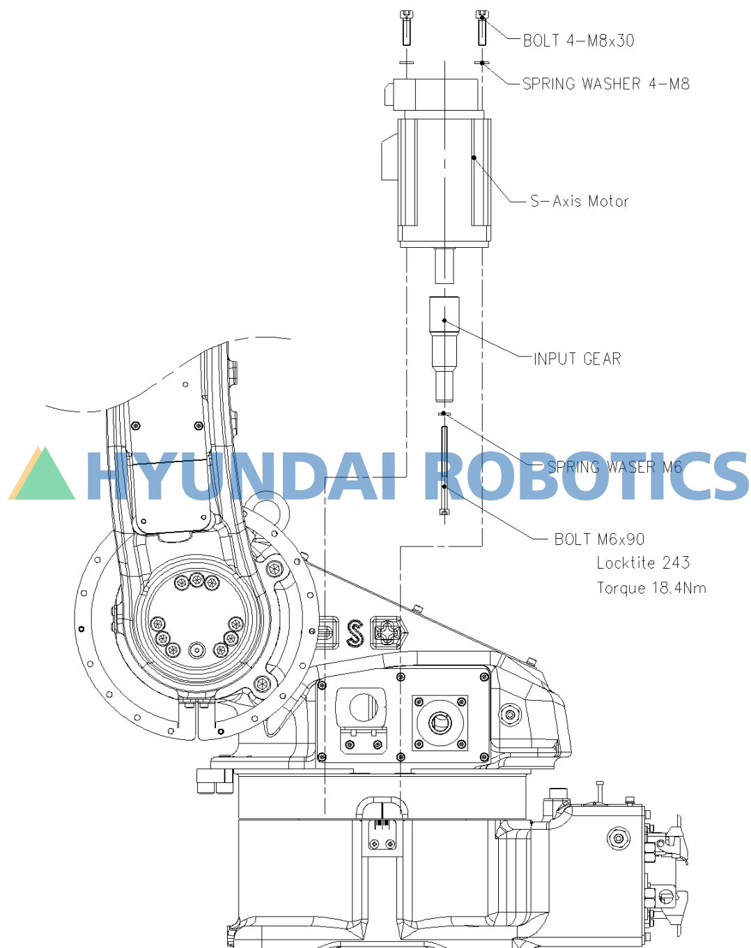
그림 6.1 S 축 모터 교체 [HH012]
