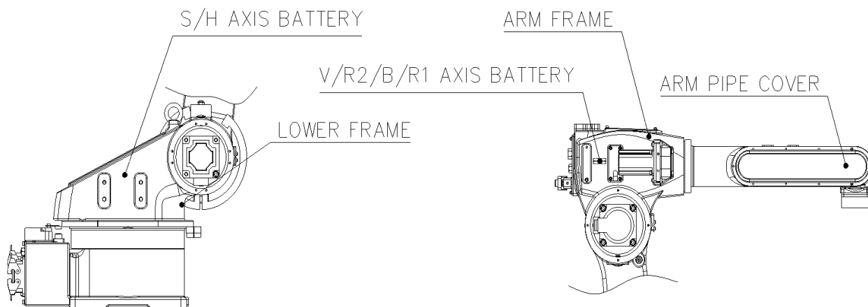
그림 5.3 배터리 교환 위치 [HH012]
