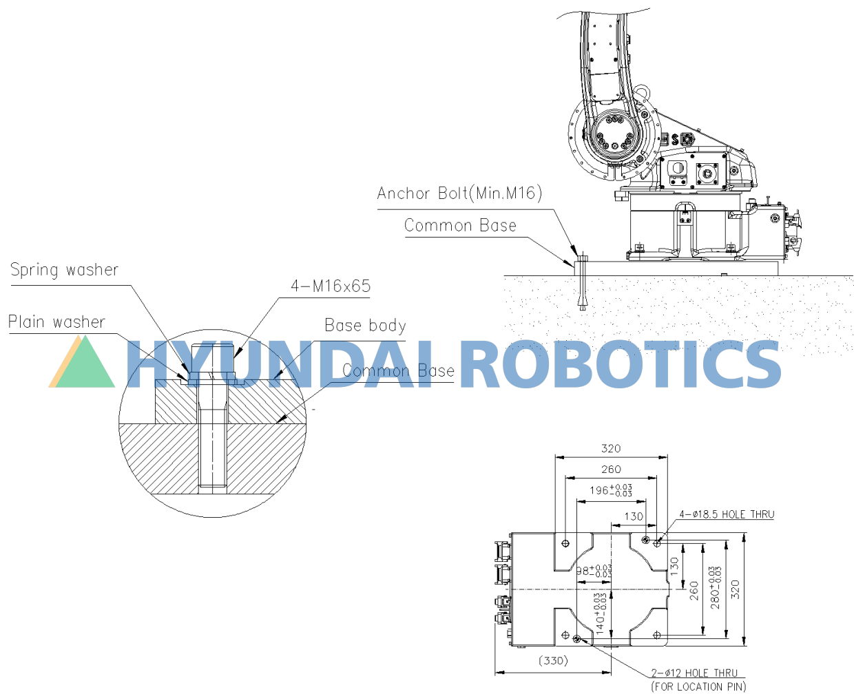
그림 3.5 로봇 설치면 치수 [HH012]
