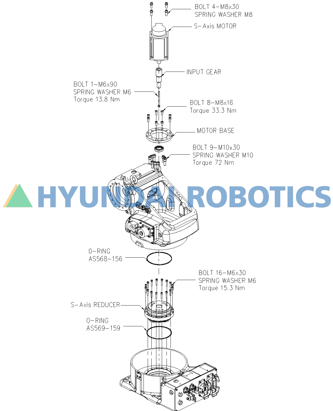
그림 6.9 S 축 감속기 분해도 [HH012]
