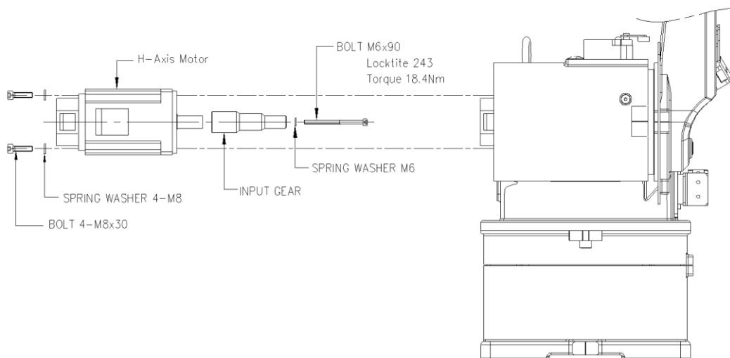
그림 6.3 H축 모터 교체 [HH012]
