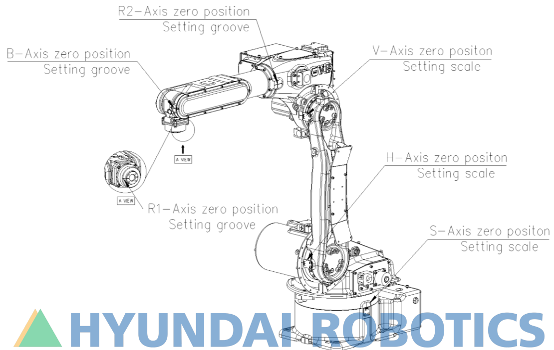
그림 6.14 원점 설정 방법 [HH012]
