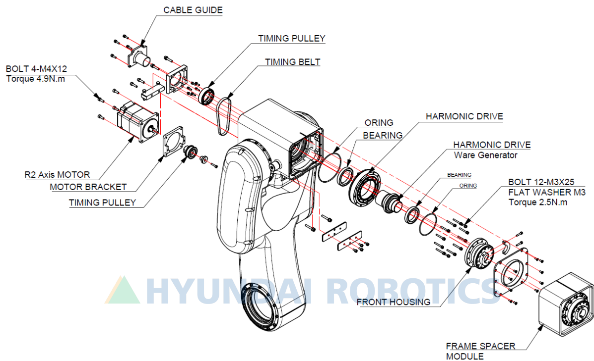
그림 6.14 R2 축 감속기 분해도 [HH007C]
