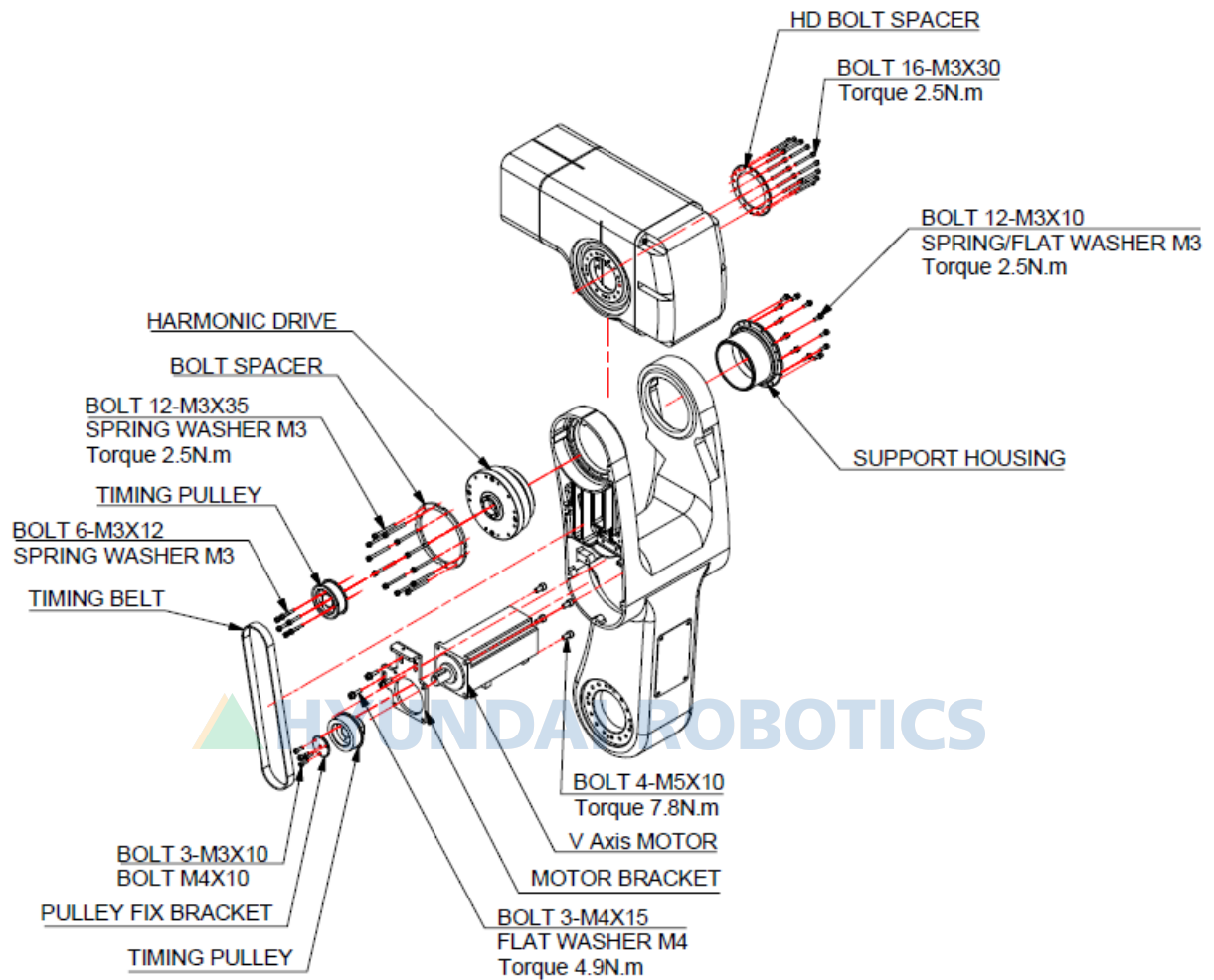
그림 6.12 V 축 감속기 분해도[HH007C]
