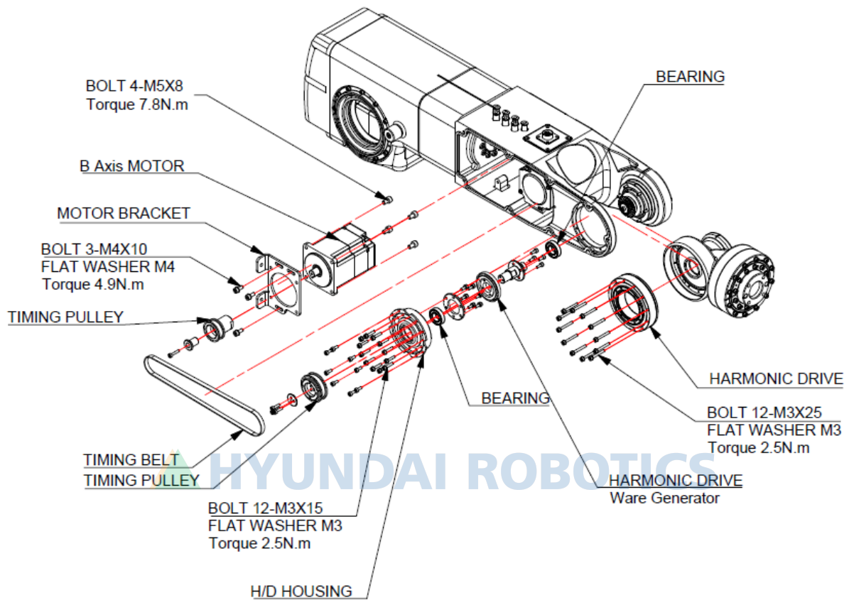
그림 6.16 B 축 감속기 분해도[HH007C]
