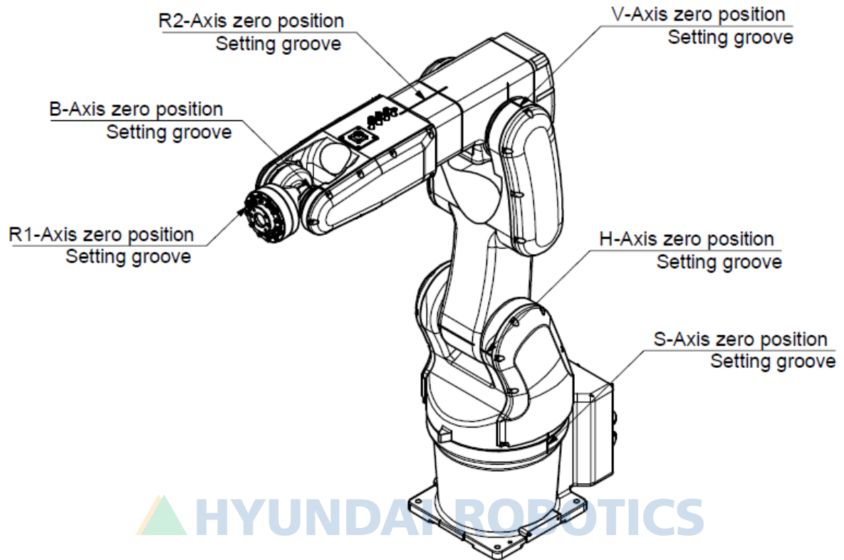
그림 6.19 원점 설정 방법 [HH007C]
