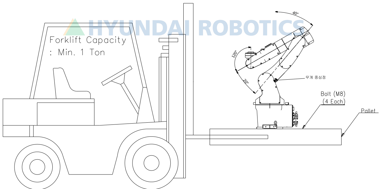
그림 3.4 운반 방법: 지게차 이용 [HH007C]
