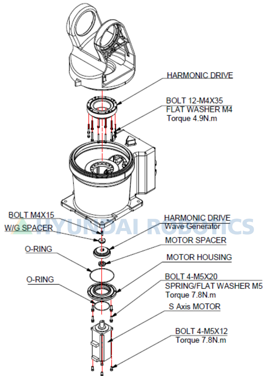
그림 6.10 S 축 감속기 분해도 [HH007C]
