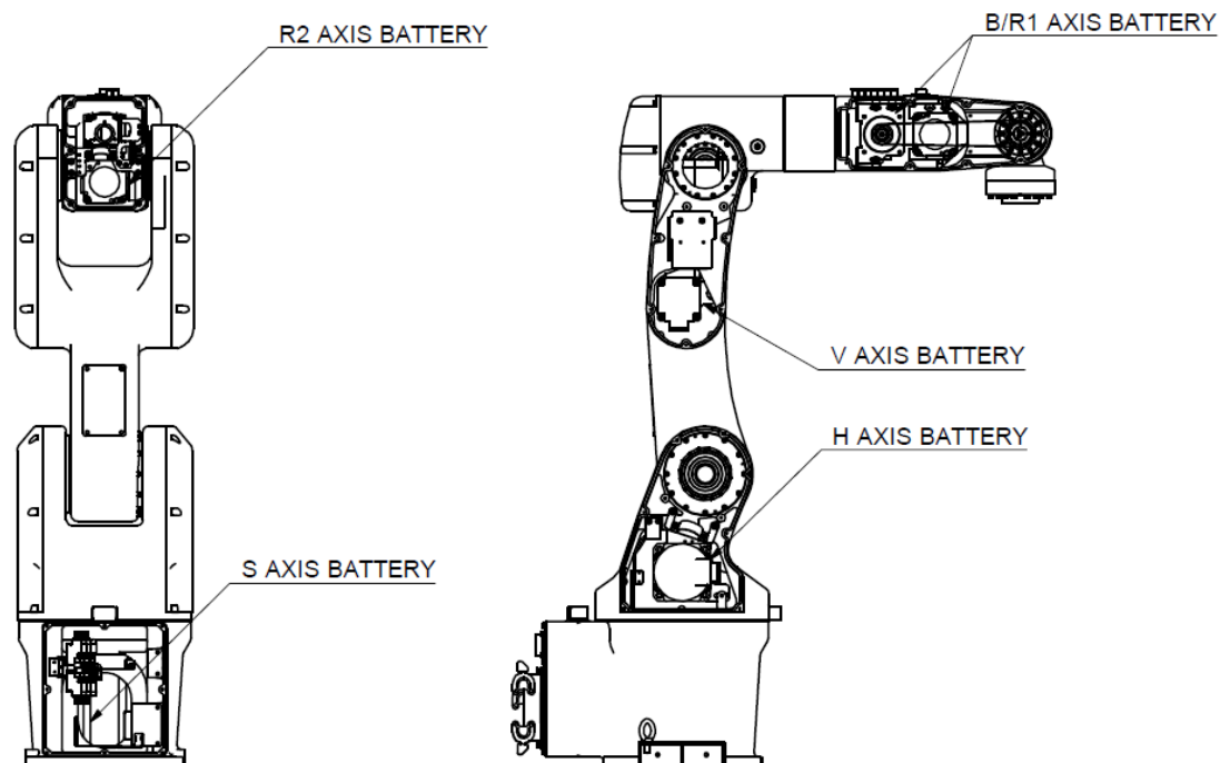
그림 5.1 배터리 교환 위치 [HH007C]
