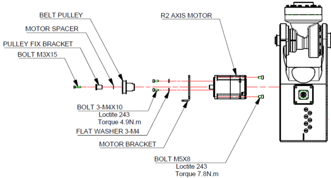
HYUNDAI ROBOTICS 그림 6.8 R1 축 모터교체 [HH007C]
