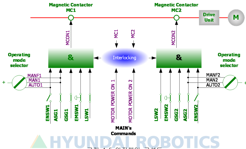
그림 1.5 안전체인 구성도
