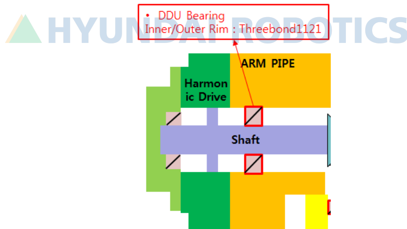
그림 6.17 R1 축 감속기 Threebond 도포 상세도[HH007C]
