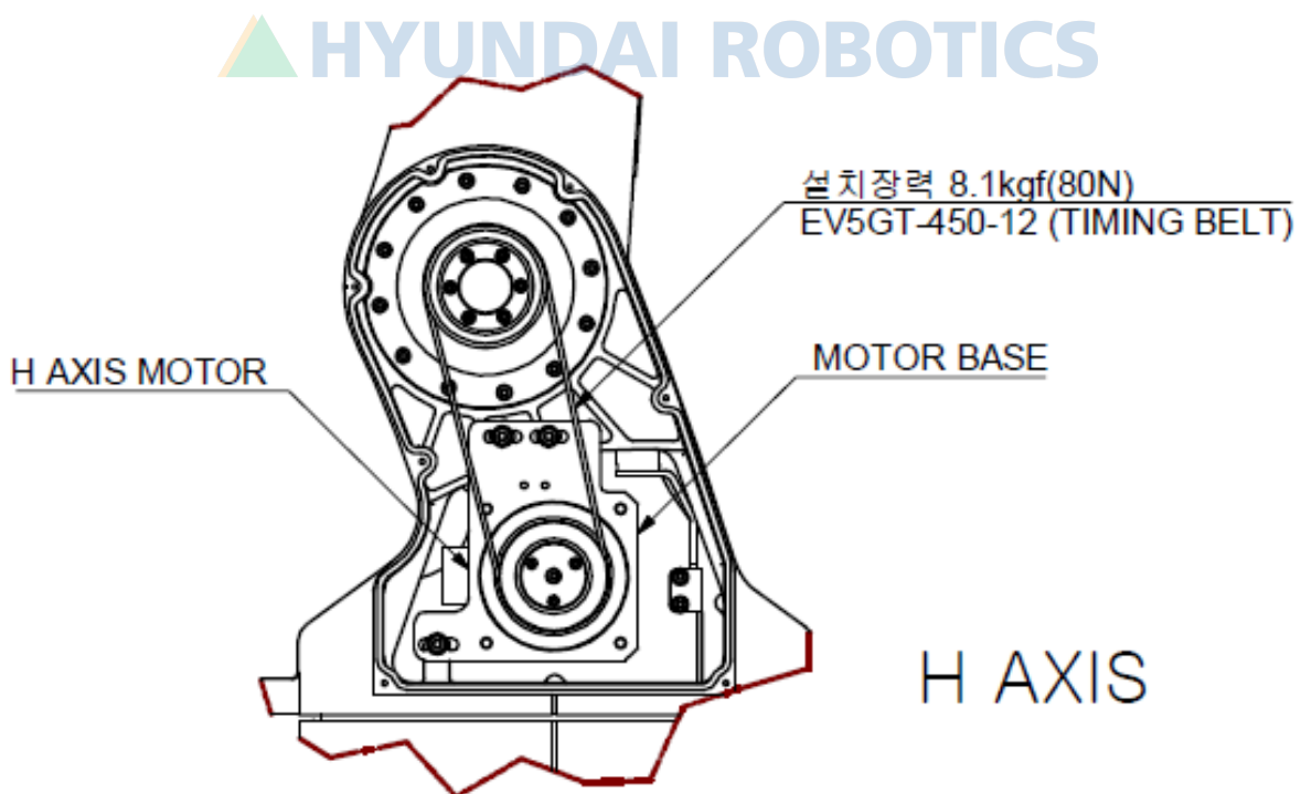
그림 4.3 H축 타이밍 벨트 장력 체크 부위[HH007C]
