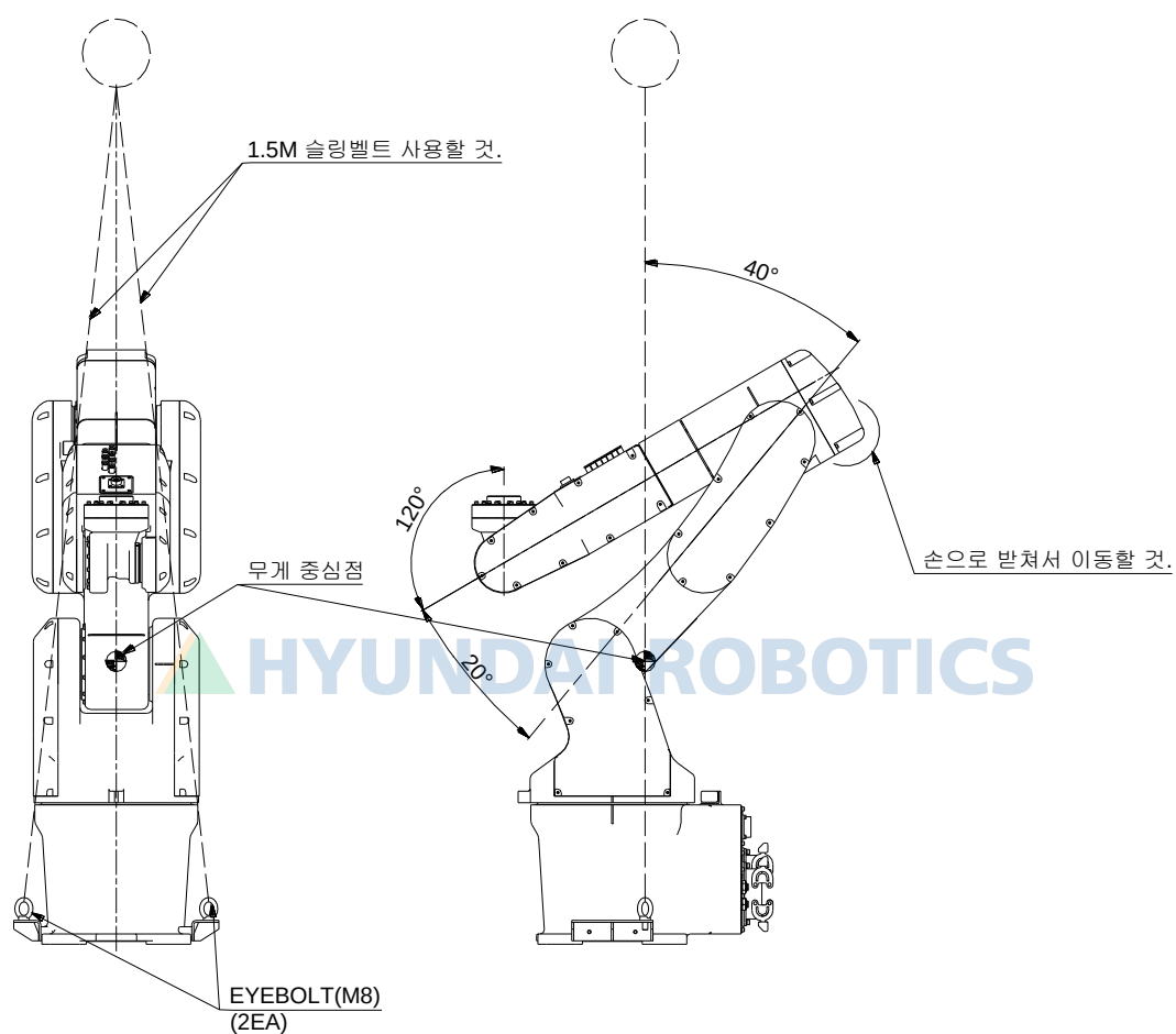
그림 3.3 운반 방법: 크레인 이용 [HH007C]
