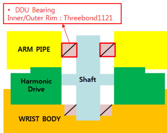
그림 6.15 B 축 감속기 Threebond 도포 상세도[HH007C]
