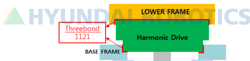
그림 6.9 S 축 감속기 Threebond 도포 상세도 [HH007C]
