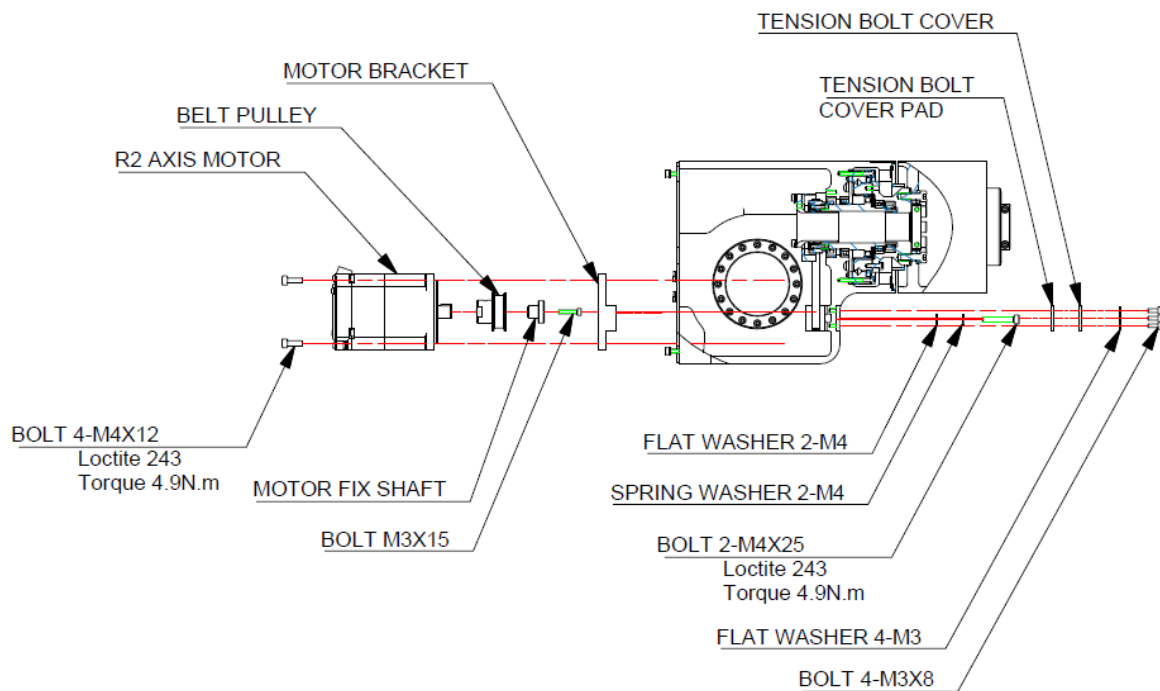
그림 6.6 R2 축 모터 교체 [HH007C]
