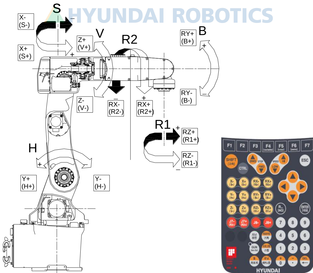
그림 2.4 본체 외관 및 동작 축
