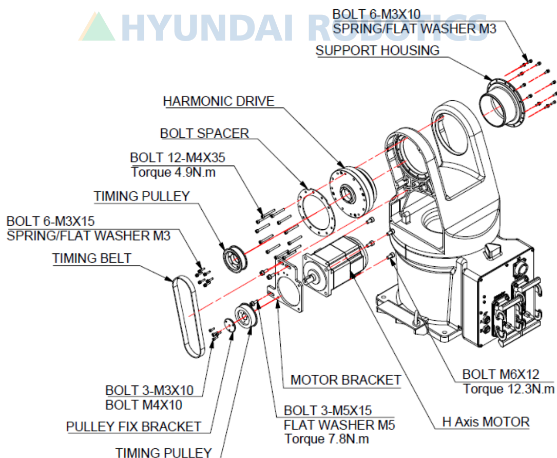
그림 6.11 H 축 감속기 분해도 [HH007C]
