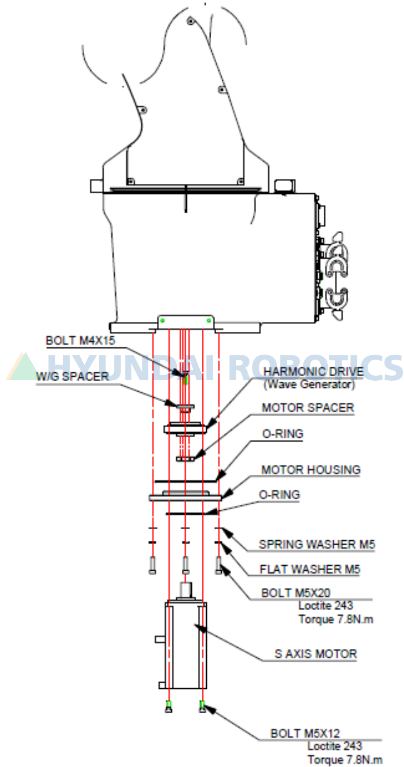
그림 6.1 S 축 모터 교체 [HH007C]
