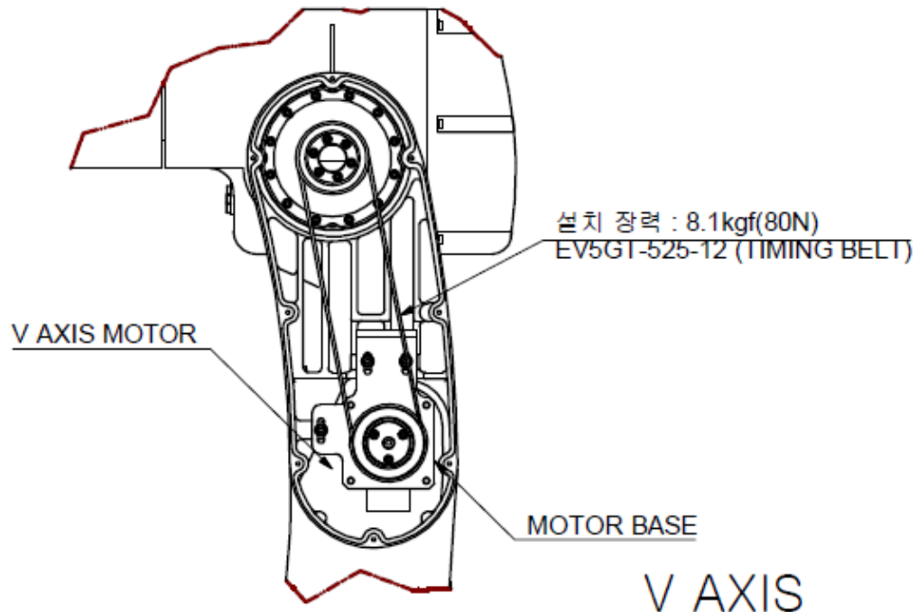
그림 4.4 V축 타이밍 벨트 장력 체크 부위[HH007C]
