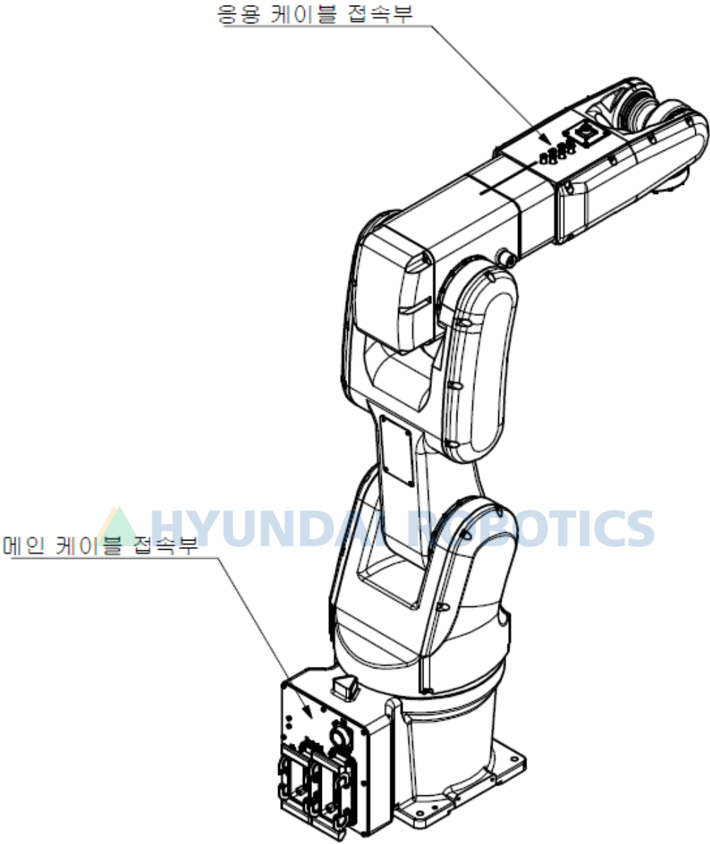
그림 9.1 본체 부품 배치 [HH007C]
