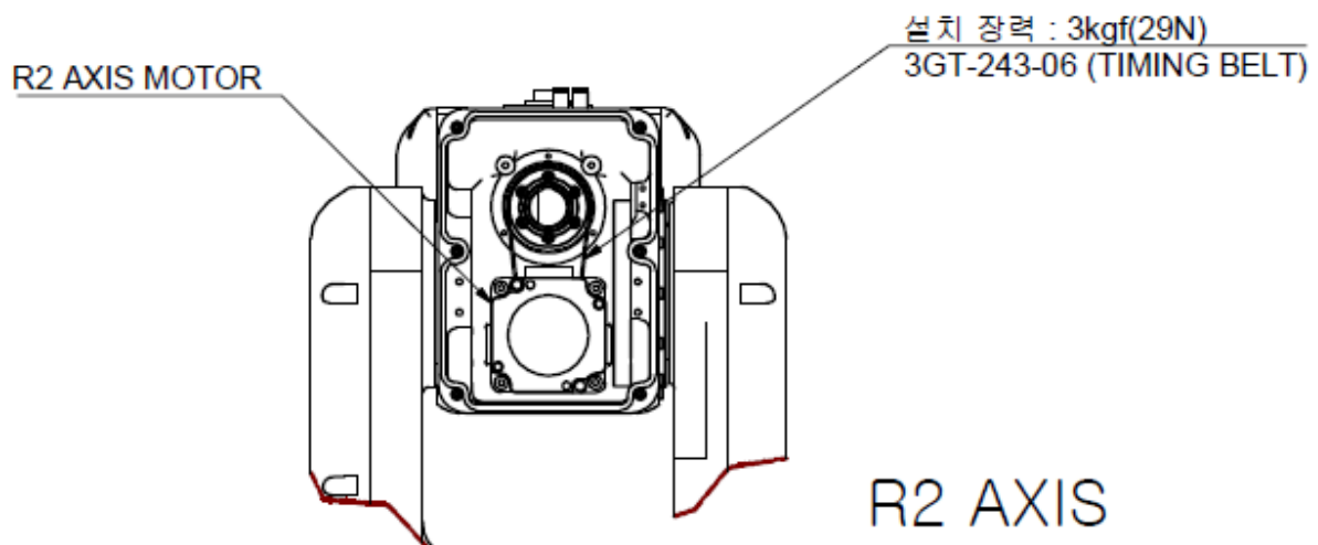
그림 4.5 V축 타이밍 벨트 장력 체크 부위[HH007C]
