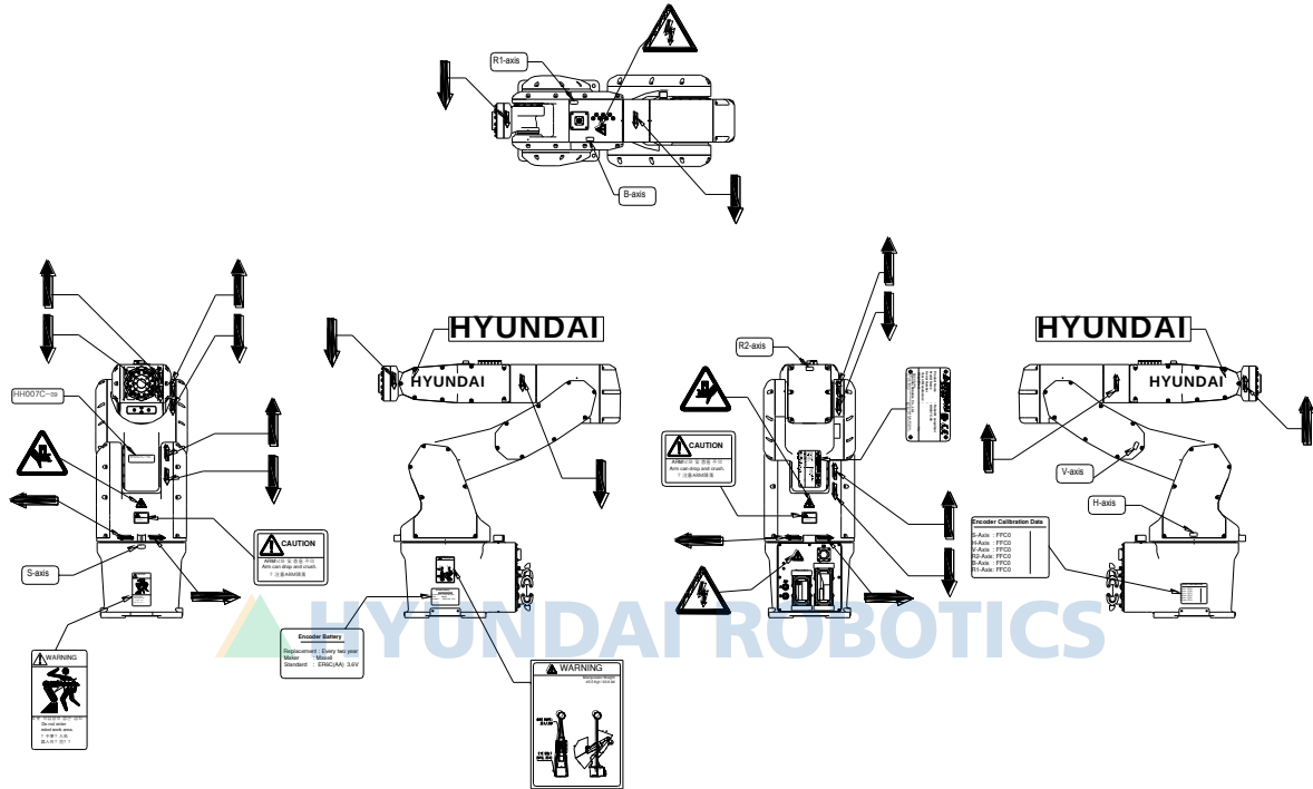
그림 3.2 안전 명판 위치 [HH007C]
