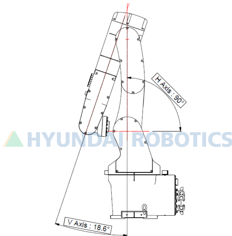
그림 6.4 V 축 모터 교체시의 로봇 자세 [HH007C]
