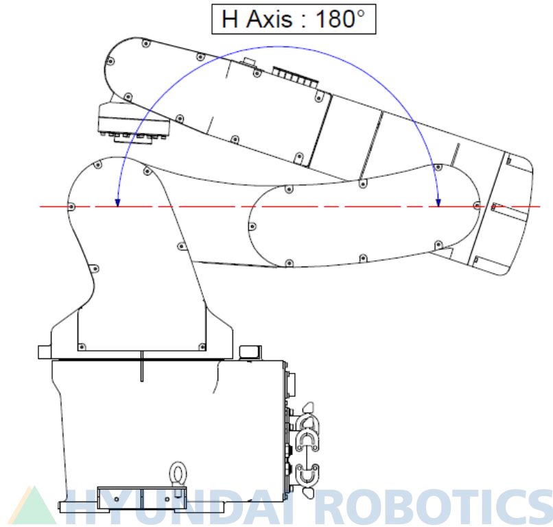
그림 6.2 H축 모터 교체시의 로봇 자세 [HH007C]
