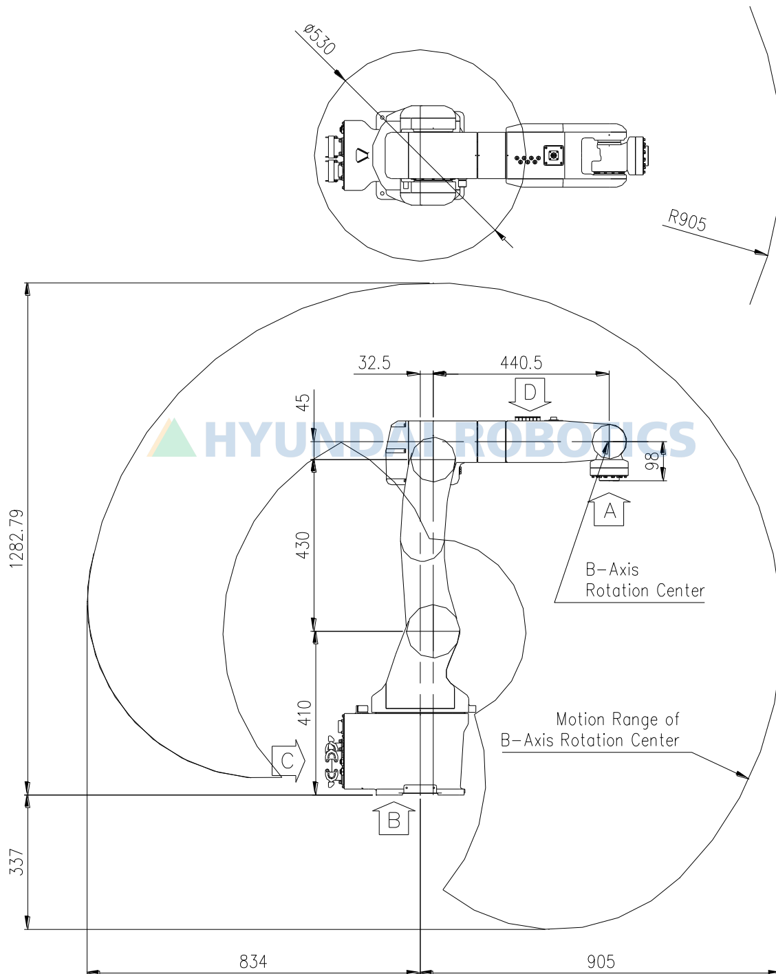
그림 2.3 로봇 본체 외형 치수 및 동작 영역: [HH007C]
