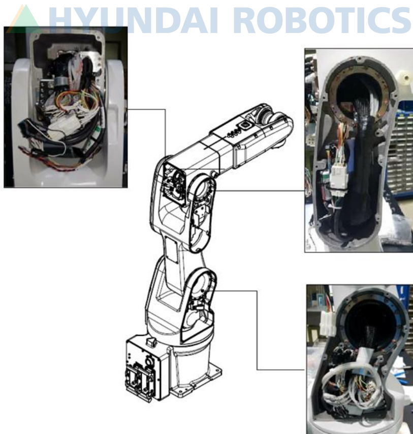
그림 4.2 케이블 점검 부위 [HH007C]
