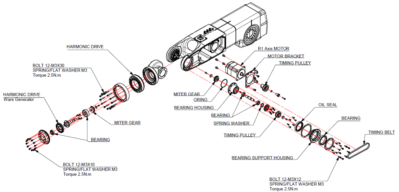
그림 6.18 R1 축 감속기 분해도[HH007C]
