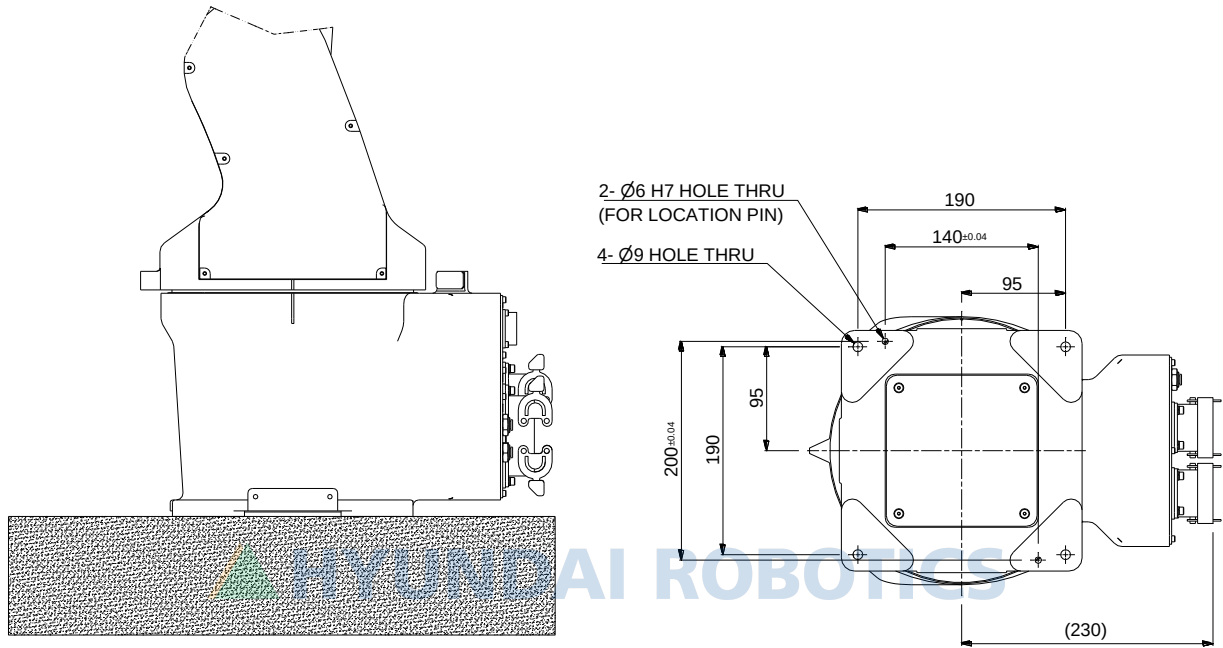
그림 3.5 로봇 설치면 치수 [HH007C]
