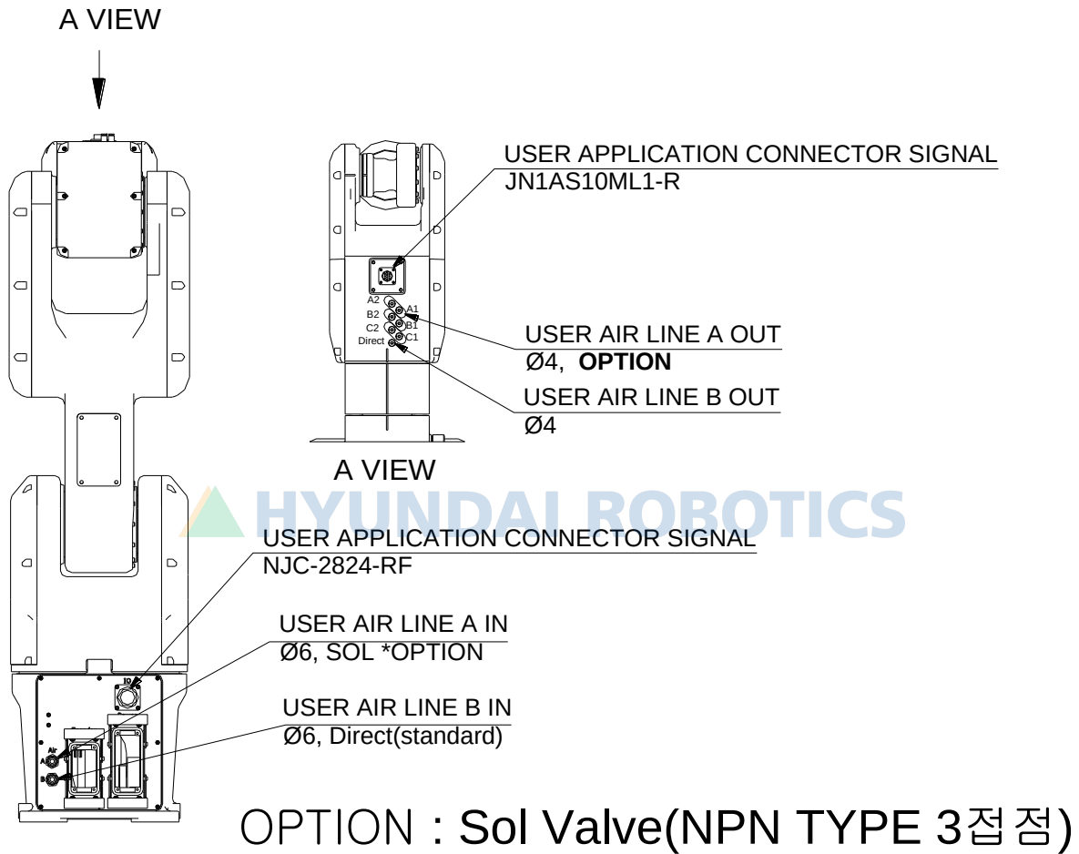
그림 2.6 어플리케이션용 배선 및 배관도: [HH007C]
