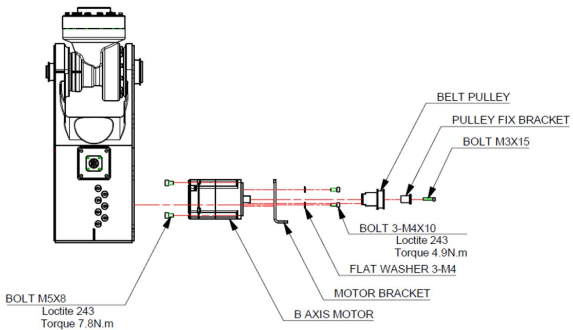
그림 6.7 B 축 모터교체 [HH007C]
