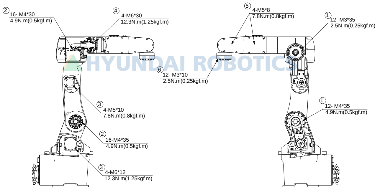
그림 4.1 주요 볼트 점검 부위 [HH007C]
