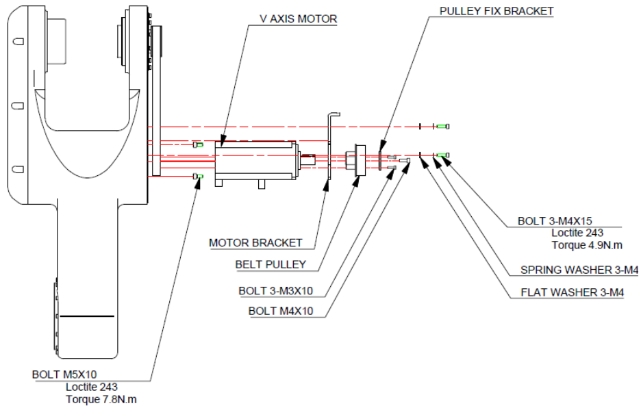
그림 6.5 V 축 모터 교체 [HH007C]
