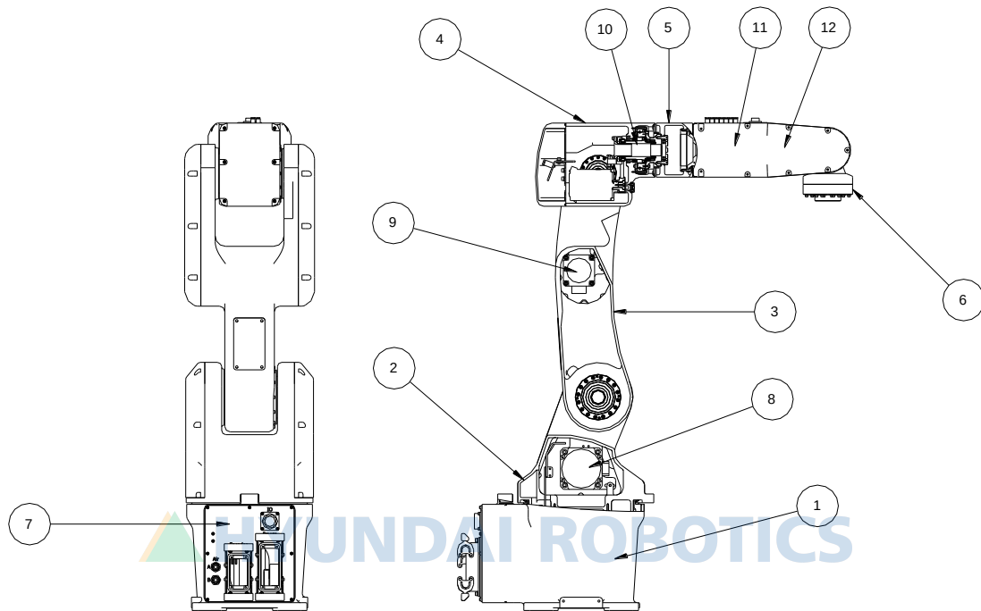
그림 3.1 본체 각 부위 명칭[HH007C]
