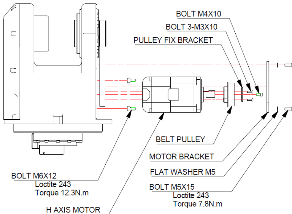
그림 6.3 H축 모터 교체 [HH007C]
