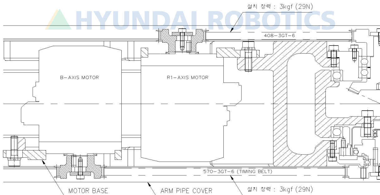
그림 4.3 B축 타이밍 벨트 장력 체크 부위
