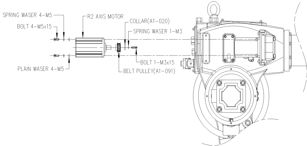
그림 6.6 R2 축 모터 교체 [HH006BL]
