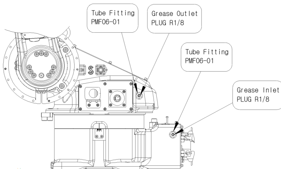
그림 5.1 S 축 그리스 IN/OUTLET 위치 [HH006BL]
