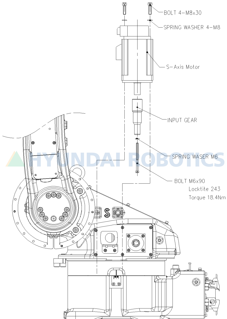
그림 6.1 S 축 모터 교체 [HH006BL]
