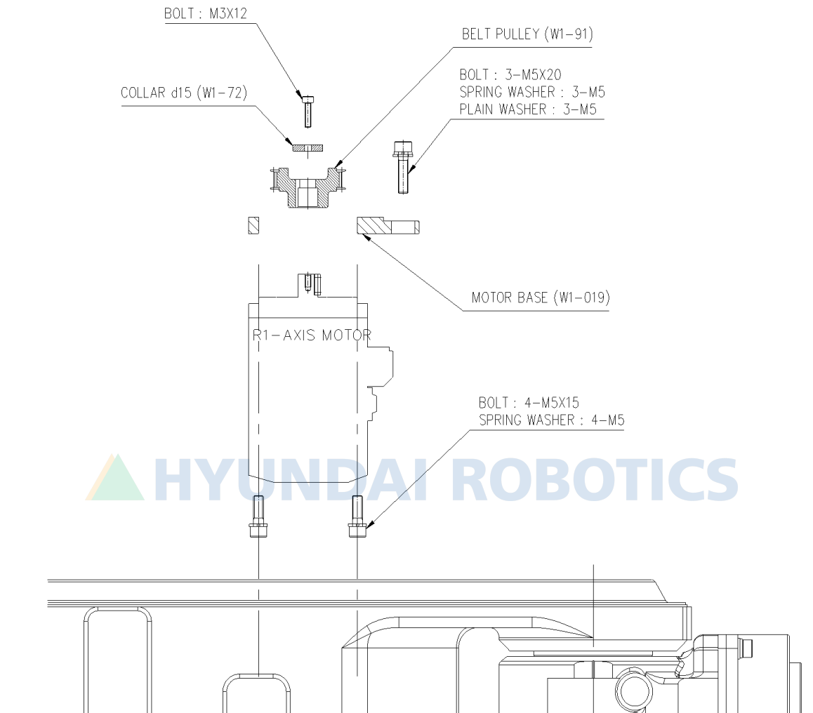
그림 6.7 B/R1 축 모터교체 (HH006BL)
