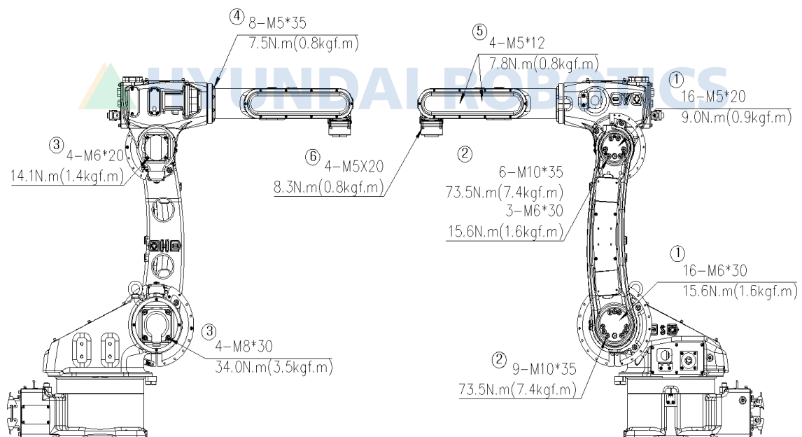
그림 4.1 주요 볼트 점검 부위 [HH006BL]
