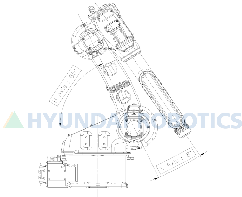
그림 6.4 V 축 모터 교체시의 로봇 자세 [HH006BL]
