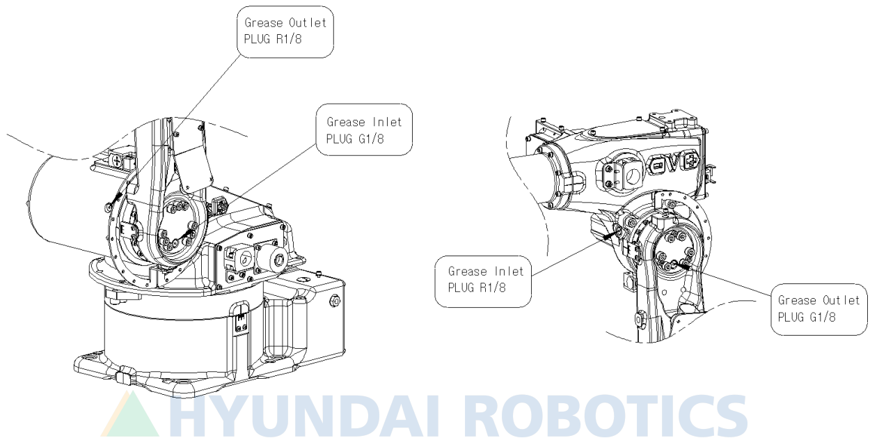
그림 5.2 H/V 축 그리스 IN/OUTLET 위치 [HH006BL]
