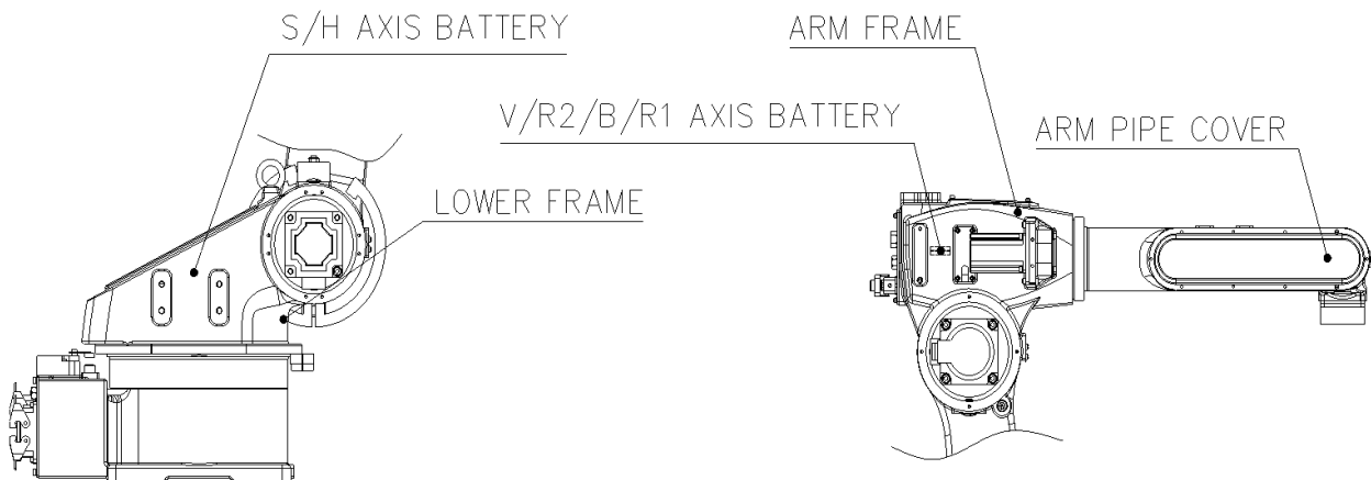
그림 5.3 배터리 교환 위치 [HH006BL]
