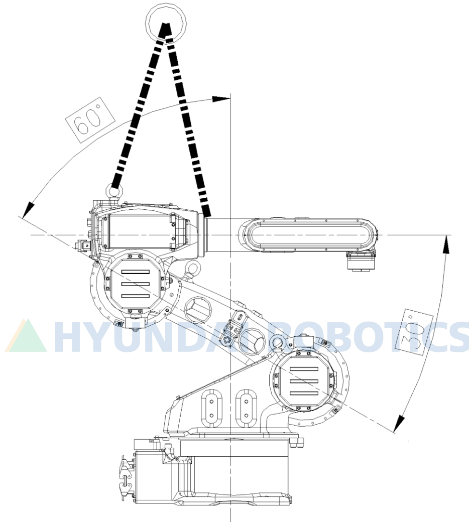
그림 6.12 V 축 감속기 교체시의 로봇 자세[HH006BL]
