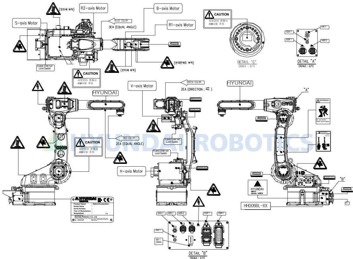
그림 3.2 안전 명판 위치 [HH006BL]
