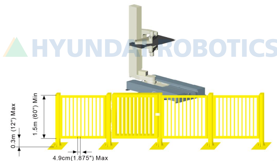
그림 1.1 권장 펜스 크기와 출입구 크기(슬롯형 출입구)
