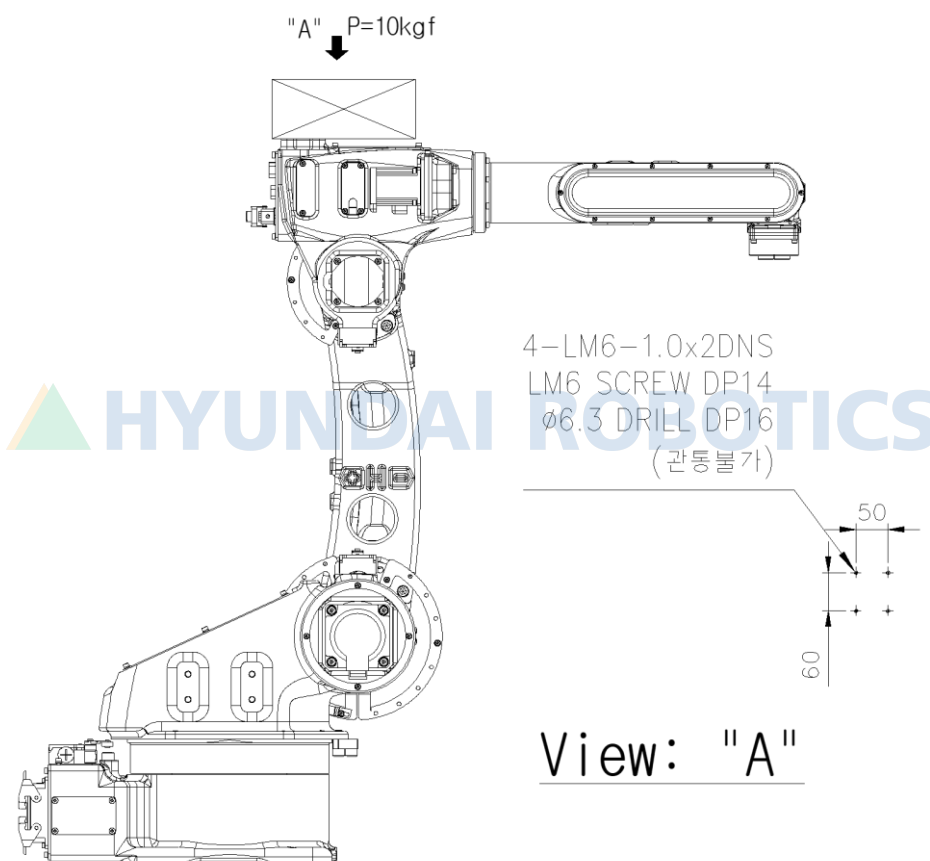
그림 2.6 제 1ARM 상부 부착부 상세도: [HH006BL]
