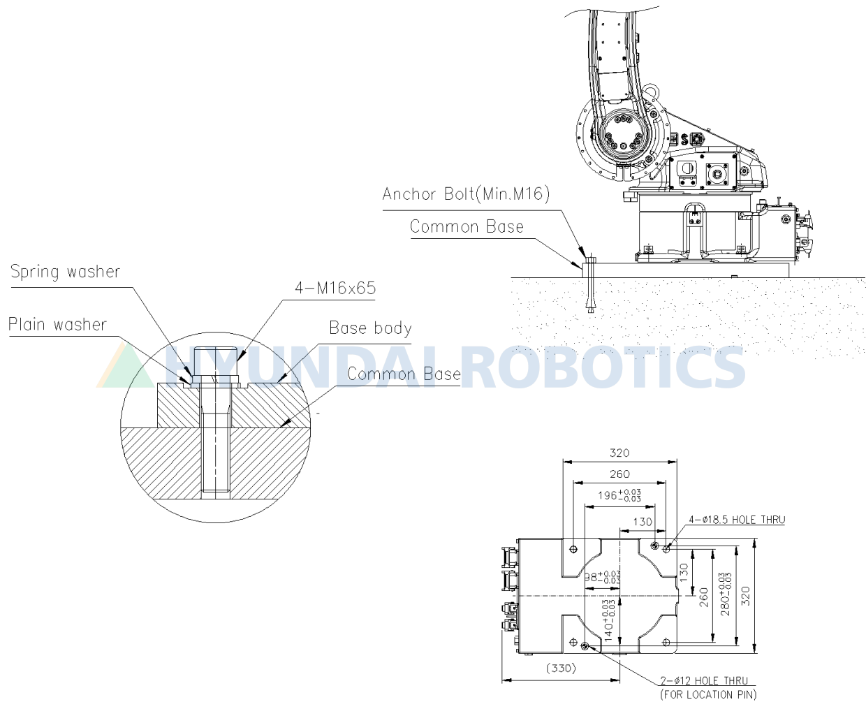
그림 3.5 로봇 설치면 치수 [HH006BL]
