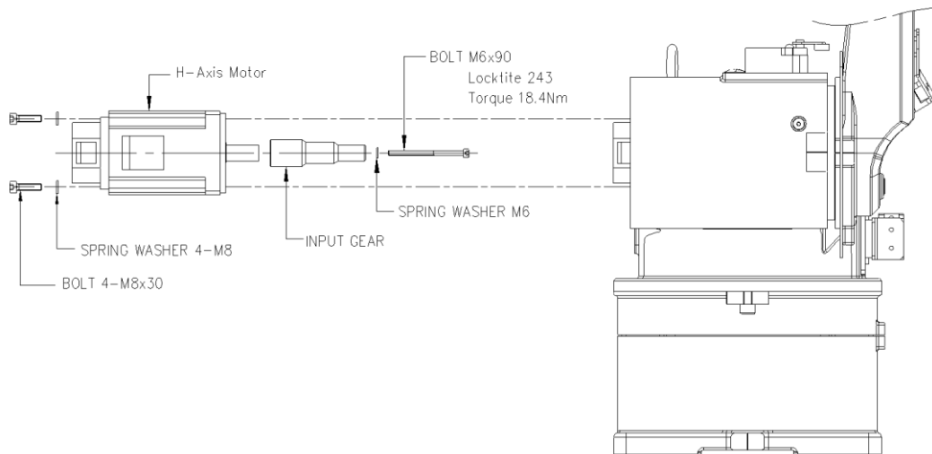
그림 6.3 H축 모터 교체 [HH006BL]
