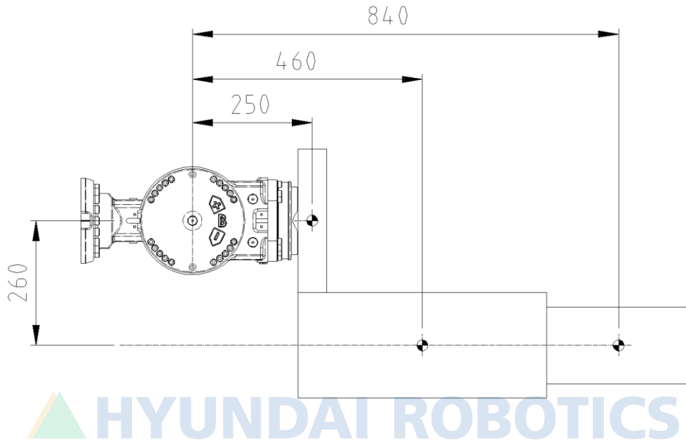
그림 3.8 3 차원 부하 모델 2D 형상
