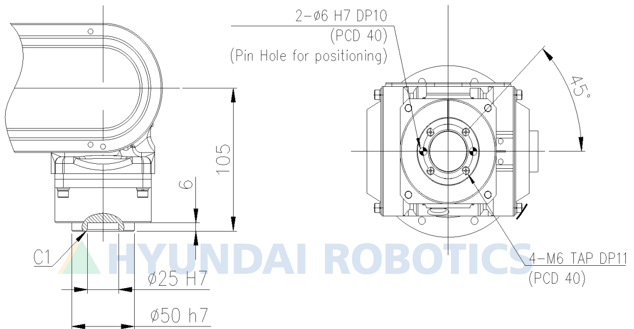
그림 2.5 손목축 취부면 상세도
