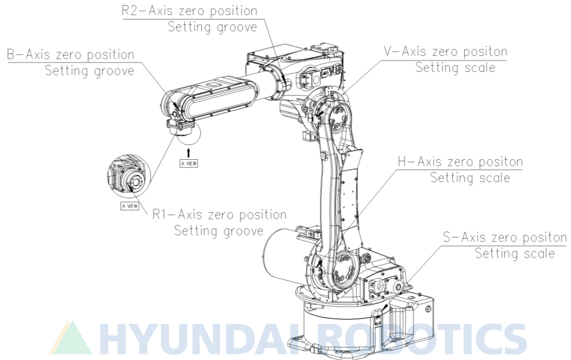
그림 6.14 원점 설정 방법 [HH006BL]
