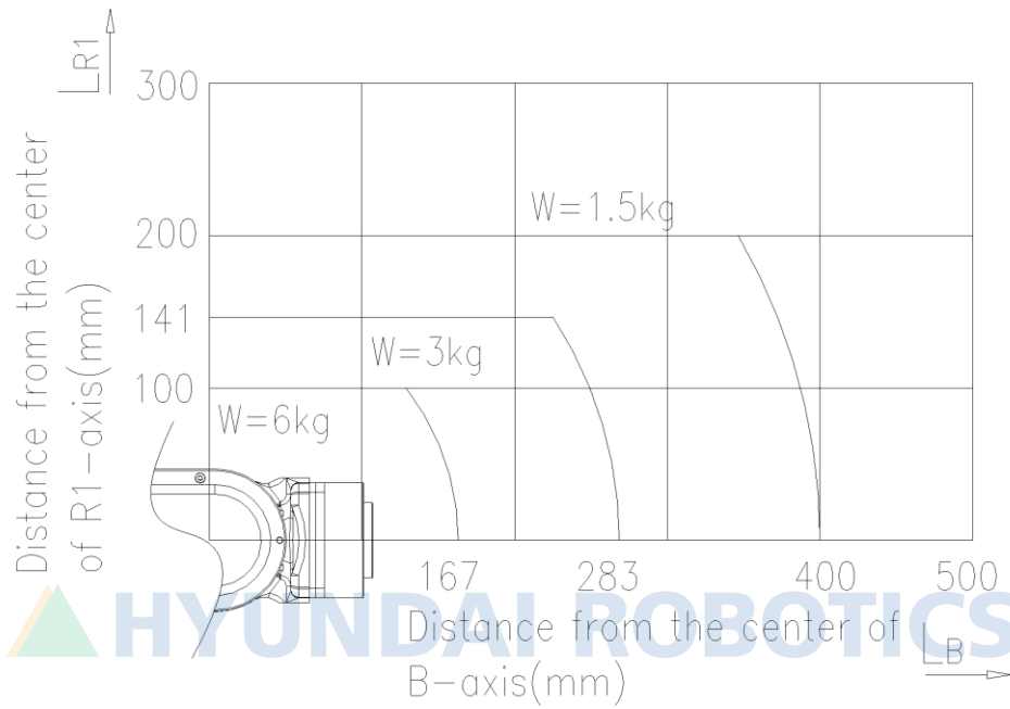
그림 3.10 손목축 토크 선도 [HH006BL]
