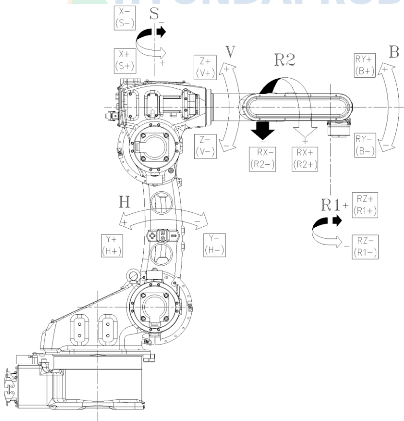
그림 2.4 본체 외관 및 동작 축
