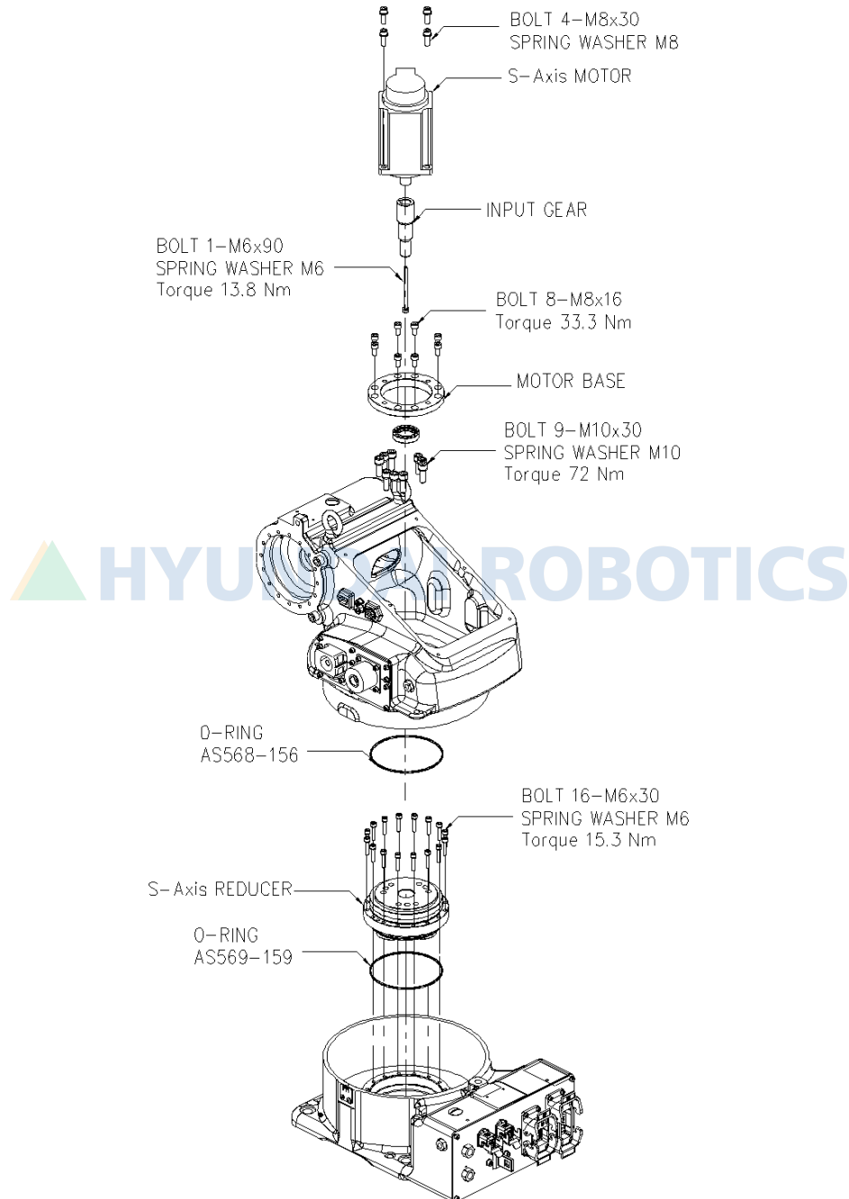
그림 6.9 S 축 감속기 분해도 [HH006BL]
