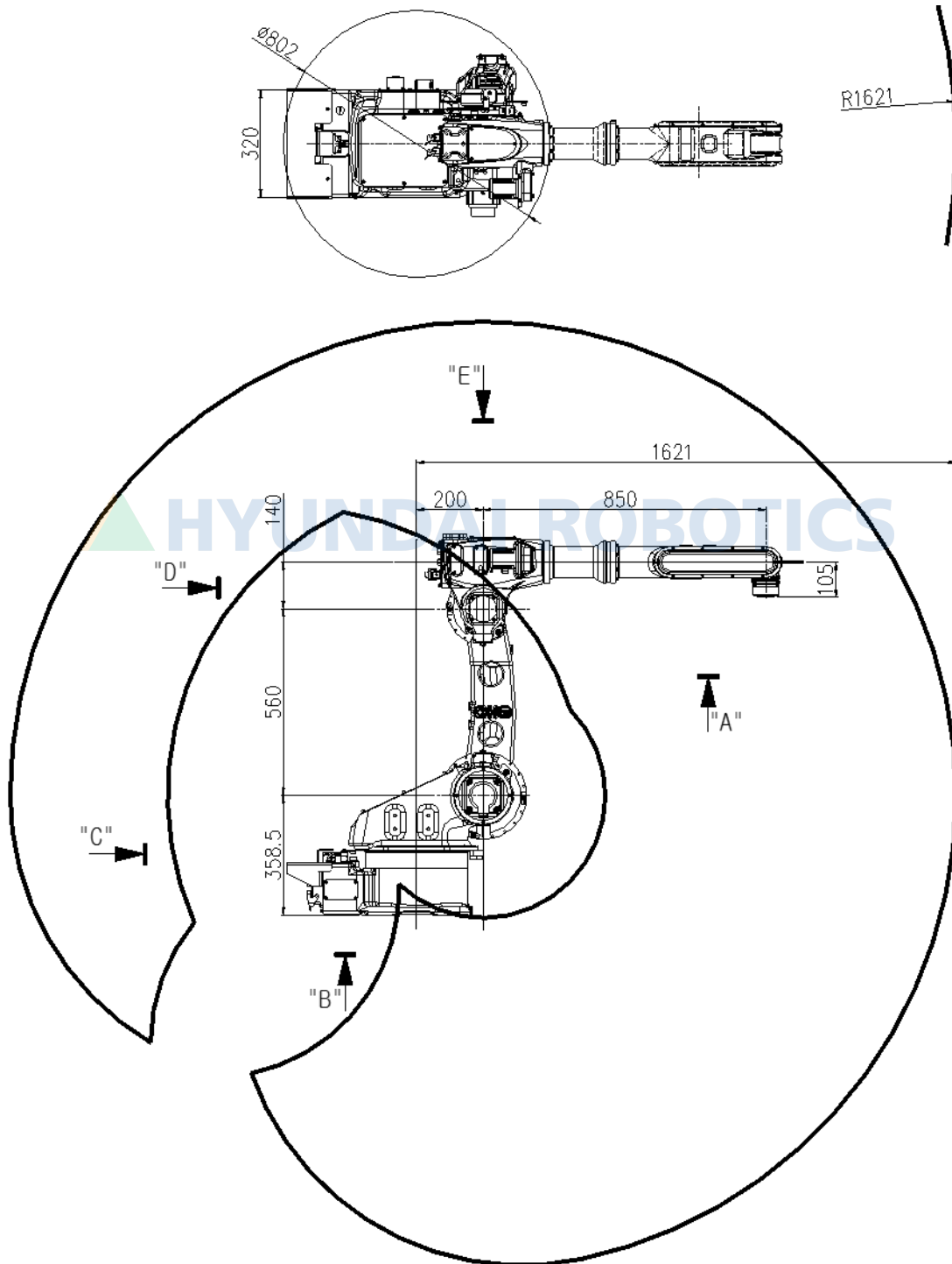
그림 2.3 로봇 본체 외형 치수 및 동작 영역: [HH006BL]
