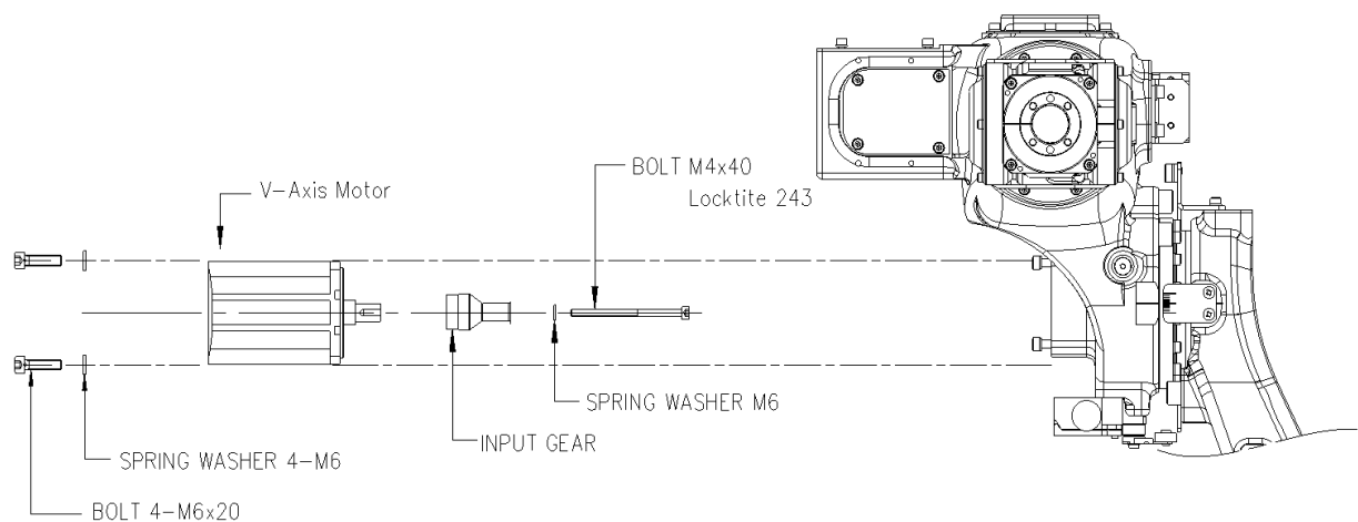
그림 6.5 V 축 모터 교체 [HH006BL]
