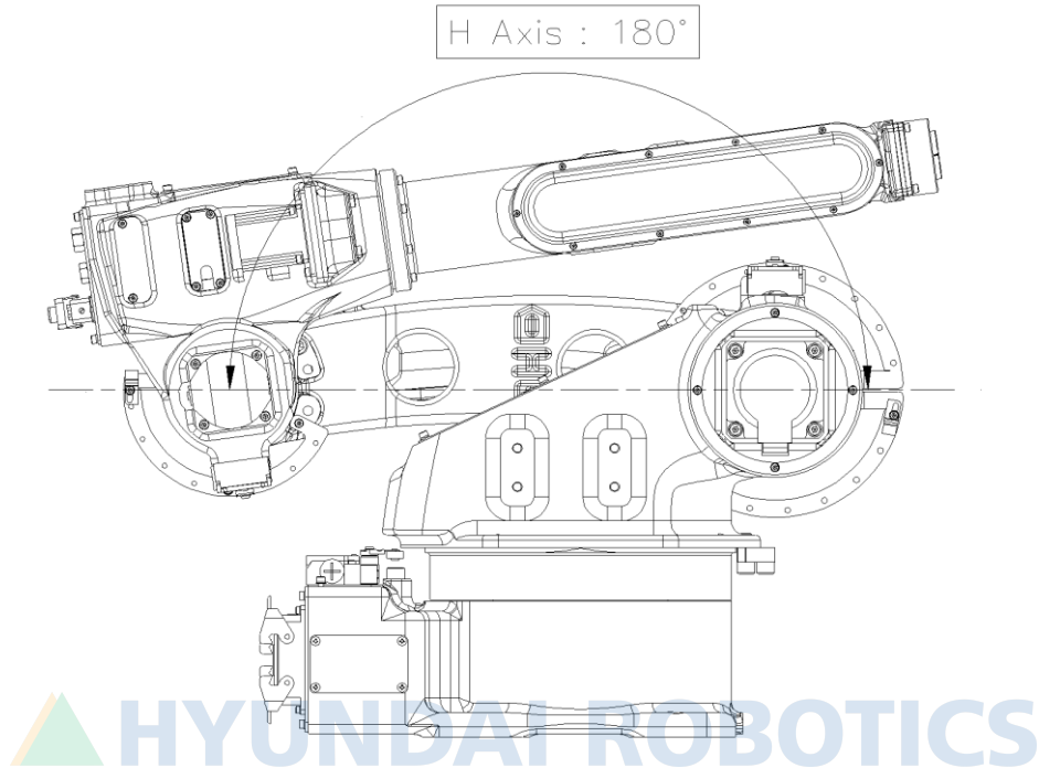
그림 6.2 H축 모터 교체시의 로봇 자세 [HH006BL]
