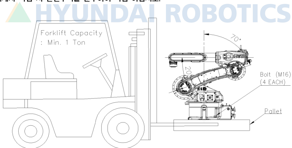
그림 3.4 운반 방법: 지게차 이용 [HH006BL]
