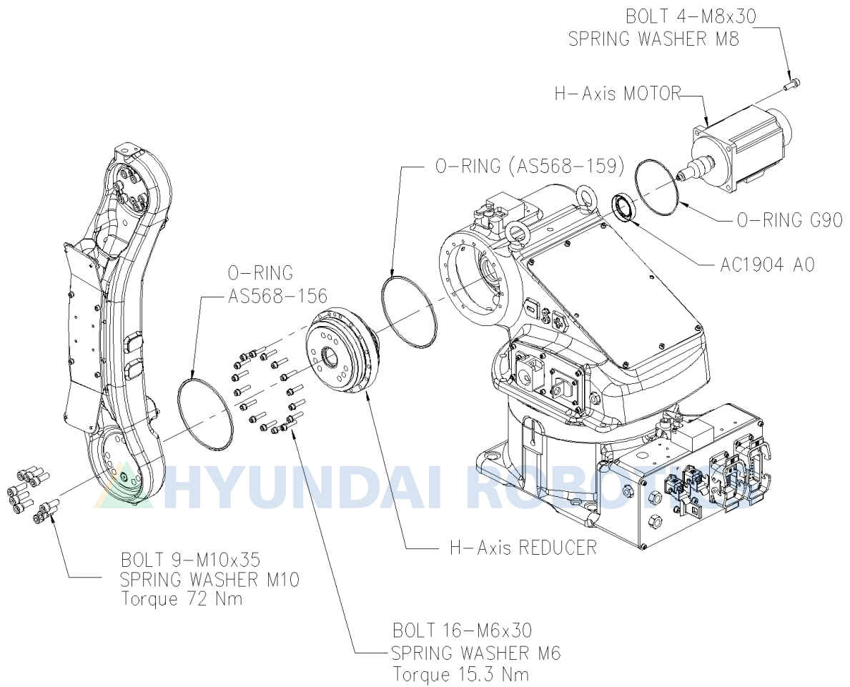
그림 6.11 H 축 감속기 분해도 [HH006BL]
