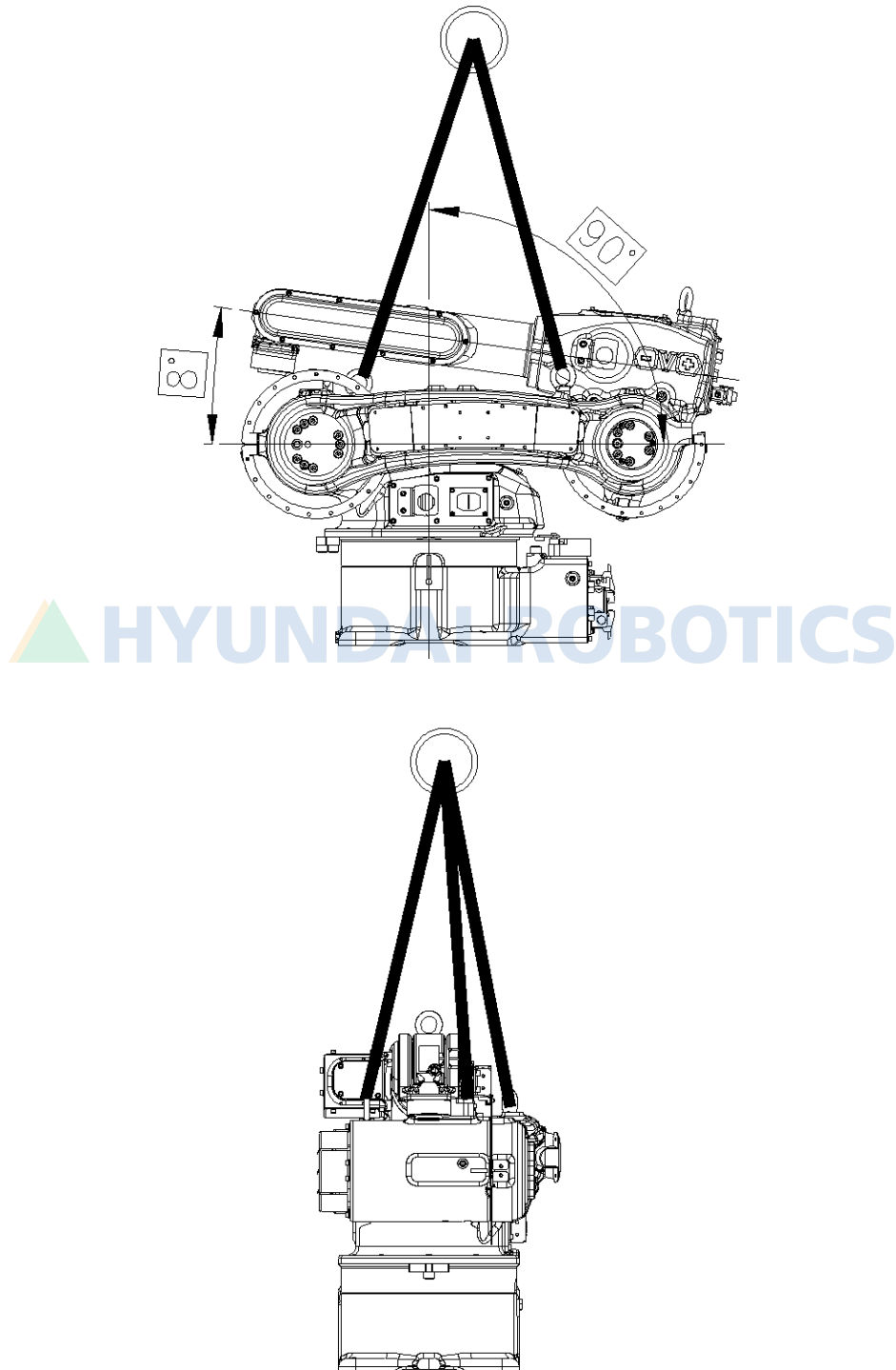
그림 6.8 S 축 감속기 교체시의 로봇 자세 [HH006BL]
