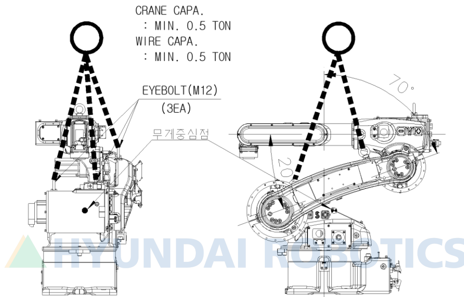
그림 3.3 운반 방법: 크레인 이용 [HH006BL]
