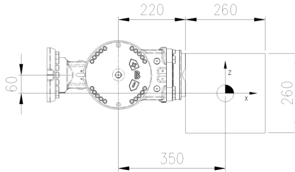
그림 3.7 2 차원 부하 모델
