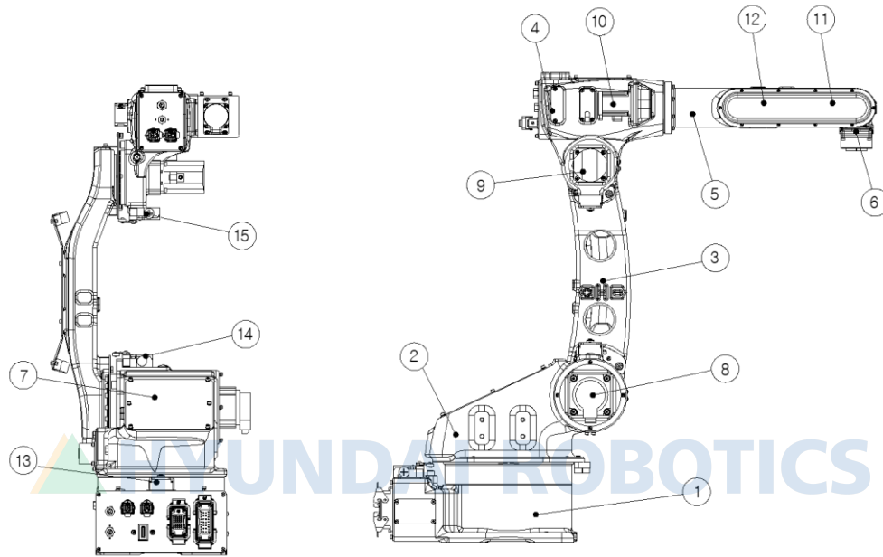
그림 3.1 본체 각 부위 명칭[HH006BL]
