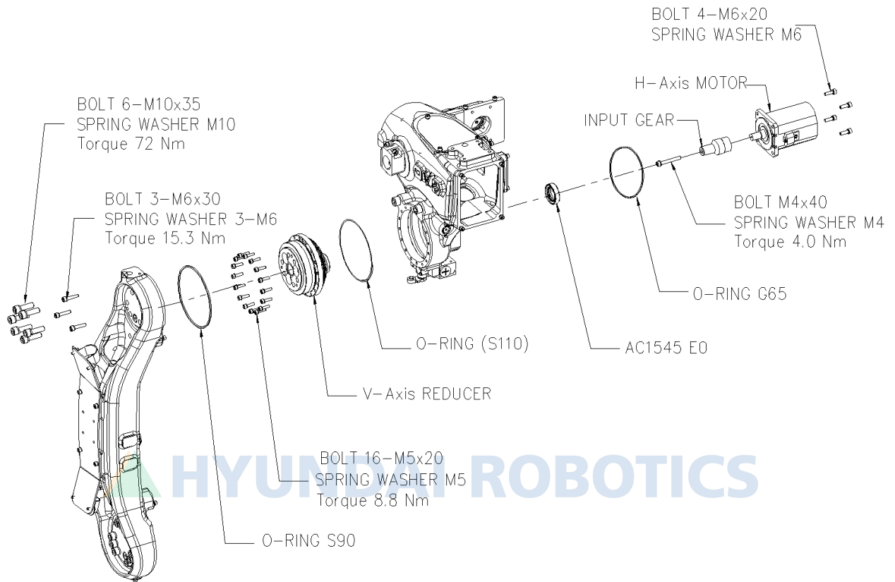
그림 6.13 V 축 감속기 분해도[HH006BL]
