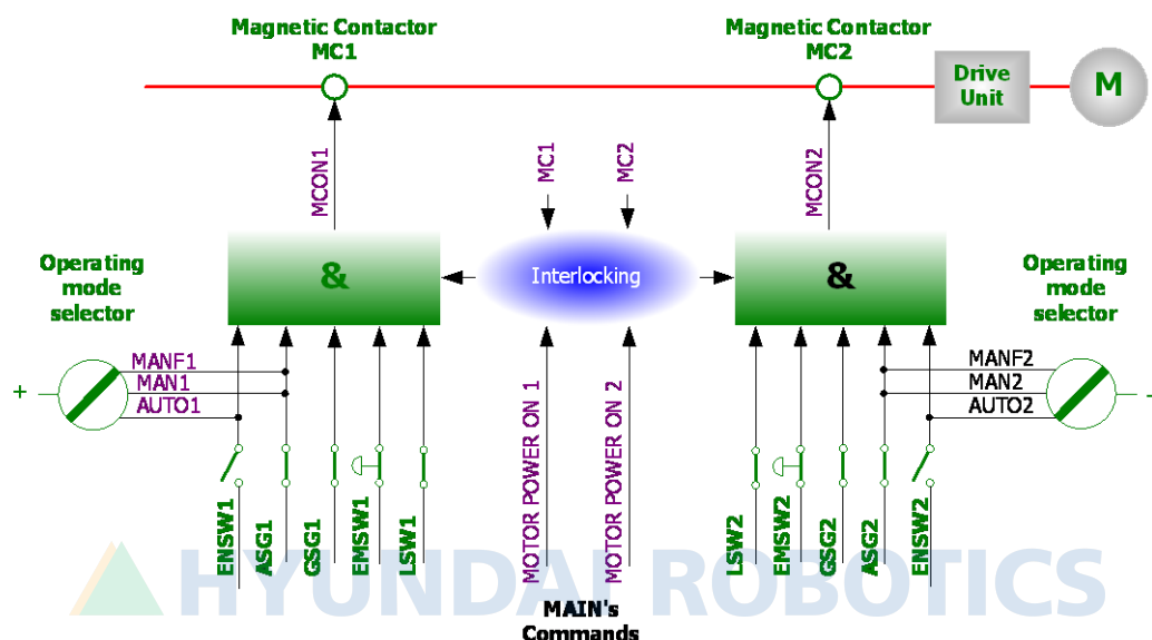
그림 1.5 안전체인 구성도
