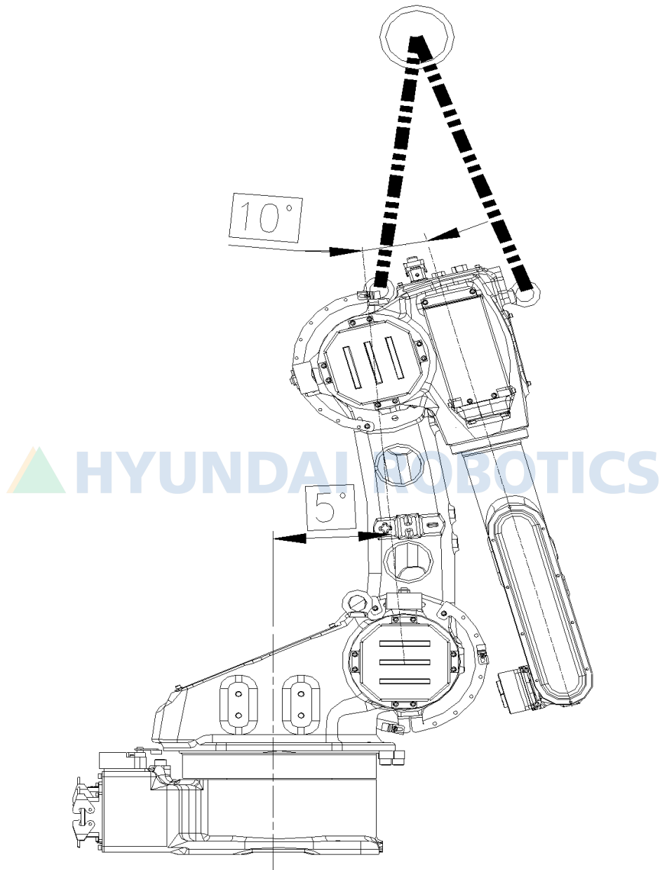
그림 6.10 H축 감속기 교체시의 로봇 자세 [HH006BL]
