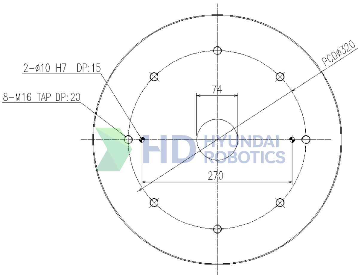
그림 1.8 Mechanical Interface 취부면 상세도
