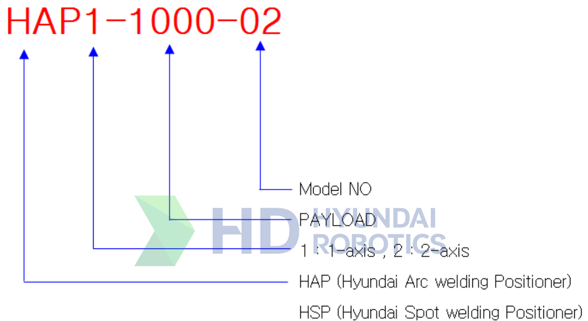
그림 1.1 POSITIONER 기구부 형식
