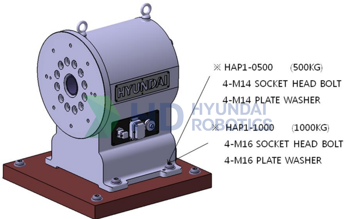
그림 2.5 설치면 치수
