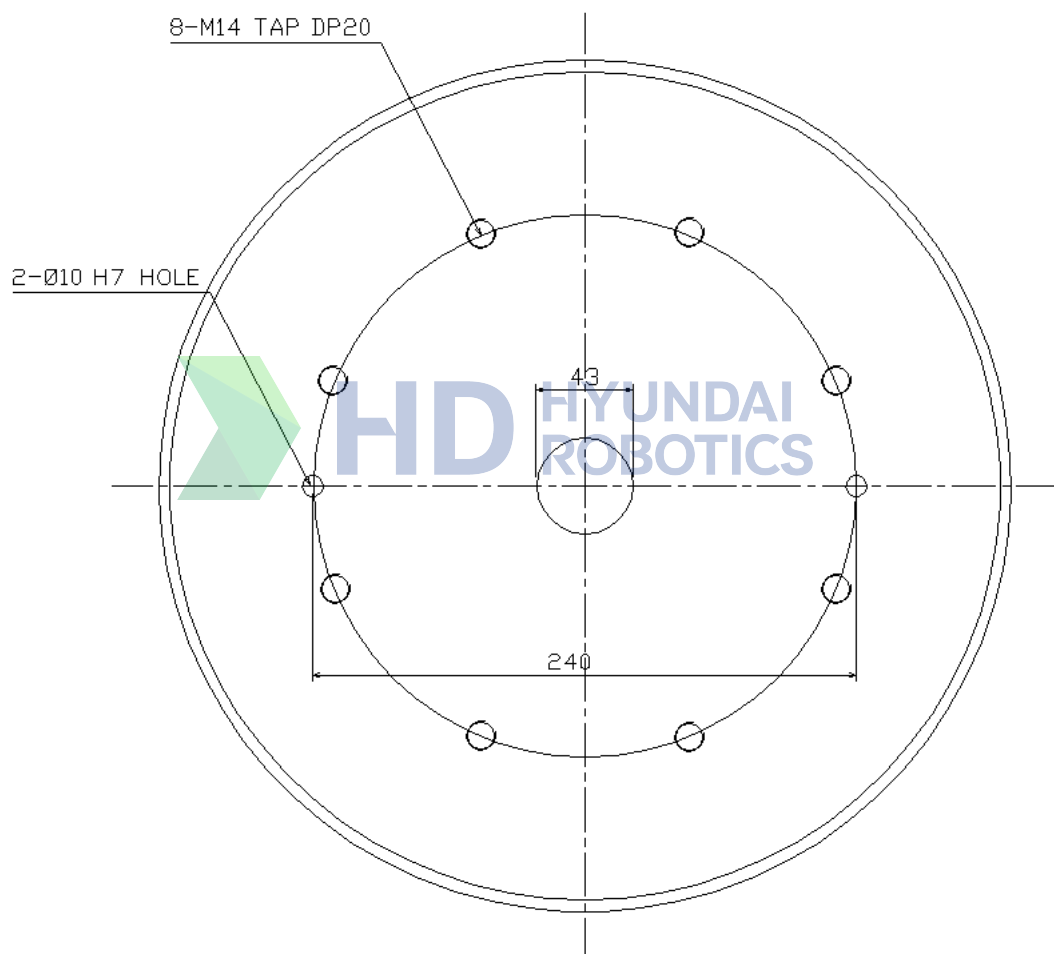
그림 1.7 Mechanical Interface 취부면 상세도
