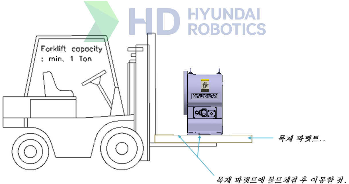
그림 2.4 운송 방법 : 지게차 이용
