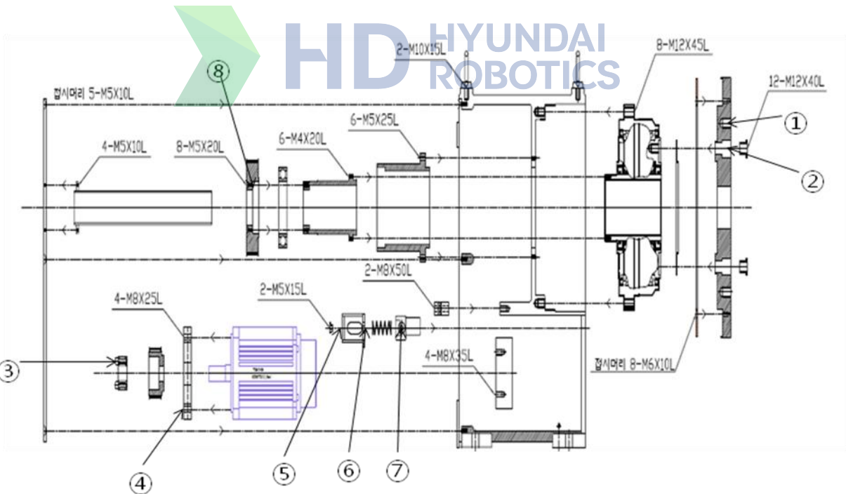
그림 3.1 주요 볼트 점검 부위
