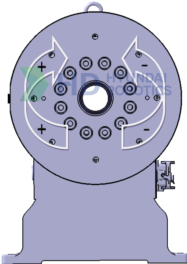
그림 1.5 본체 외관 및 동작 축
