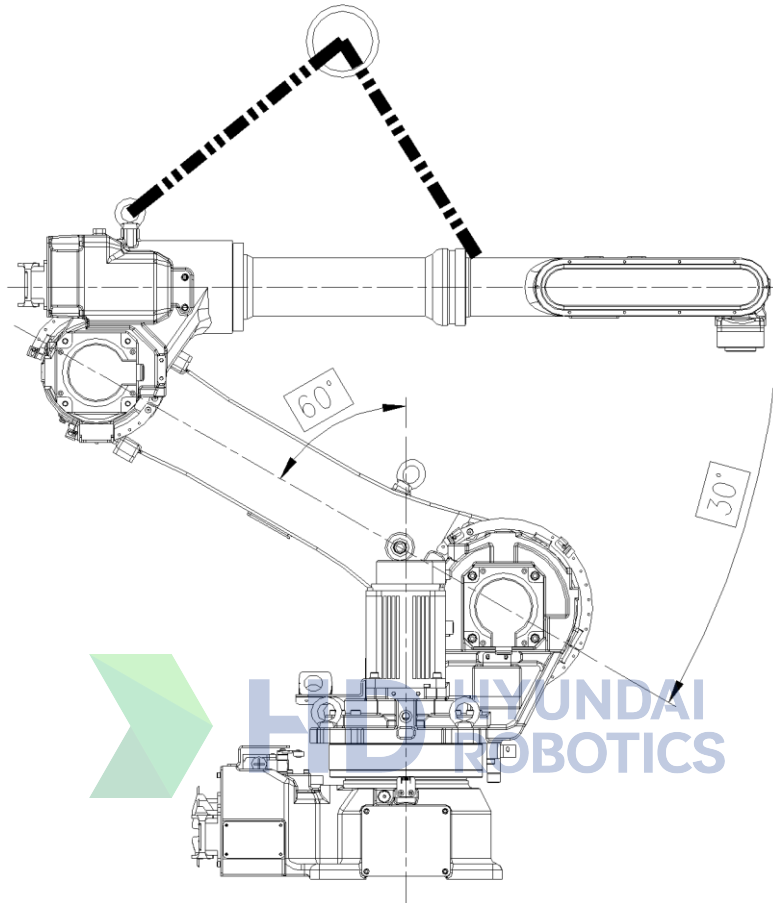
그림 6.23 V 축 감속기 교체시의 로봇 자세[HA006L]
