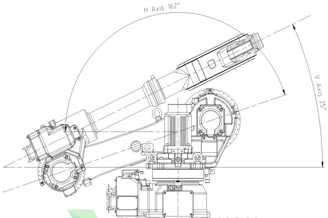
그림 6.8 H/V 축 모터 교체시의 로봇 자세 [HA006L]
