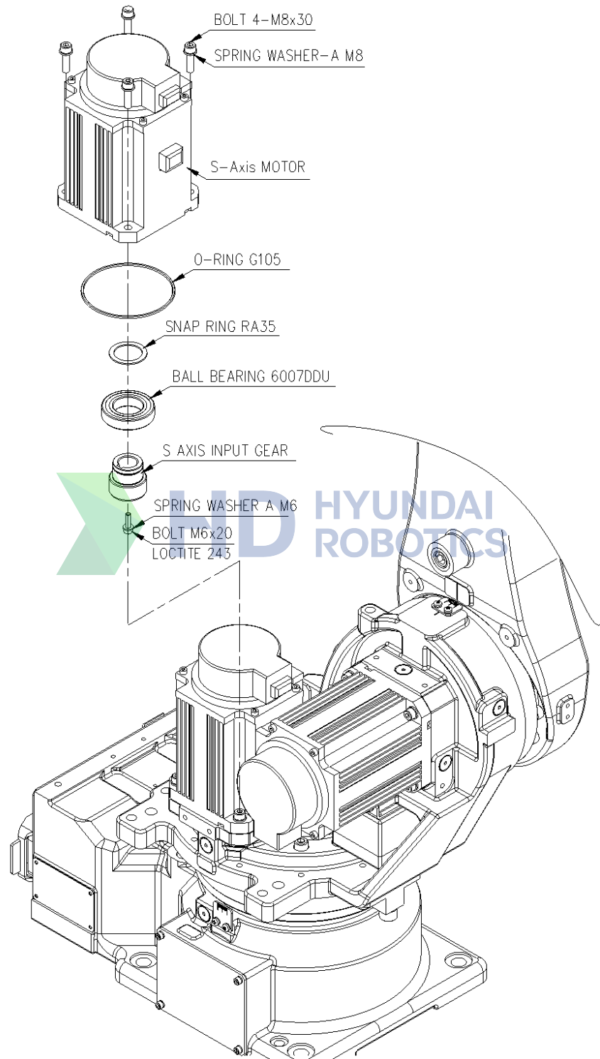
그림 6.7 S 축 모터 교체 [HA006L]
