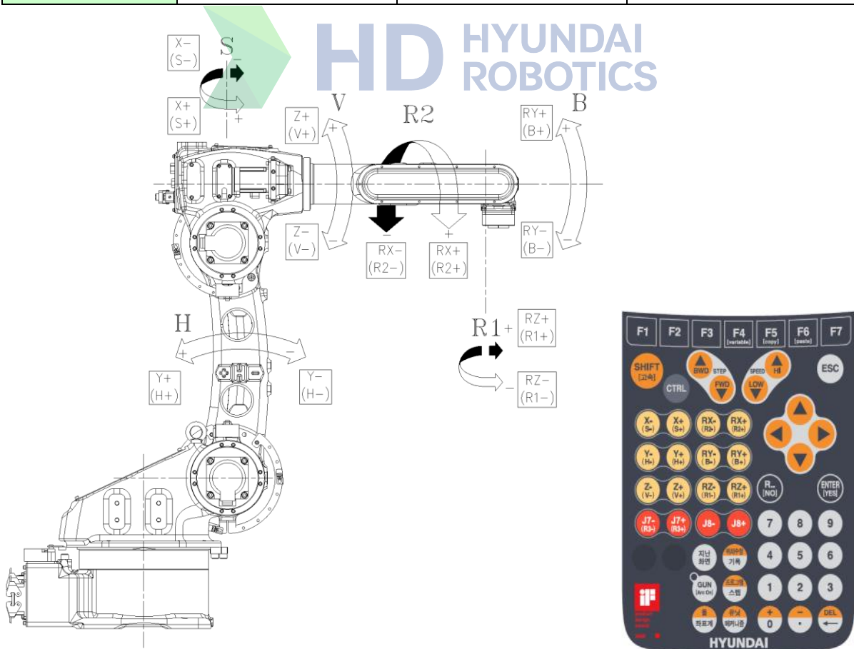
그림 2.5 본체 외관 및 동작 축
