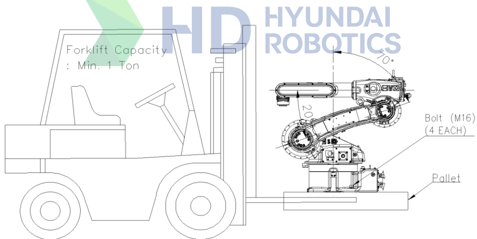
그림 3.7 운반 방법: 지게차 이용 [HA006B]
