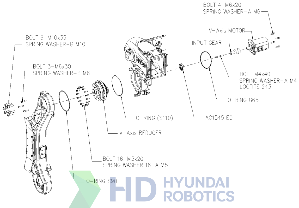
그림 6.18 V 축 감속기 분해도[HA006B]
