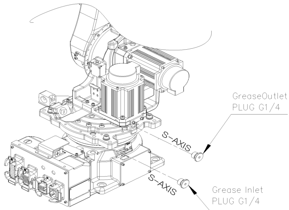
그림 5.2 S 축 그리스 IN/OUTLET 위치 [HA006L]
