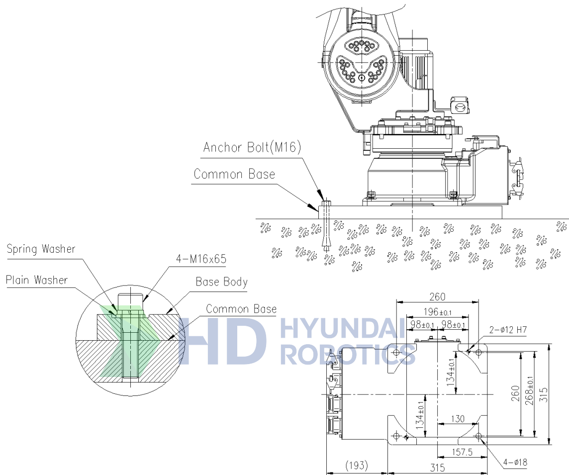
그림 3.10 로봇 설치면 치수 [HA006L]
