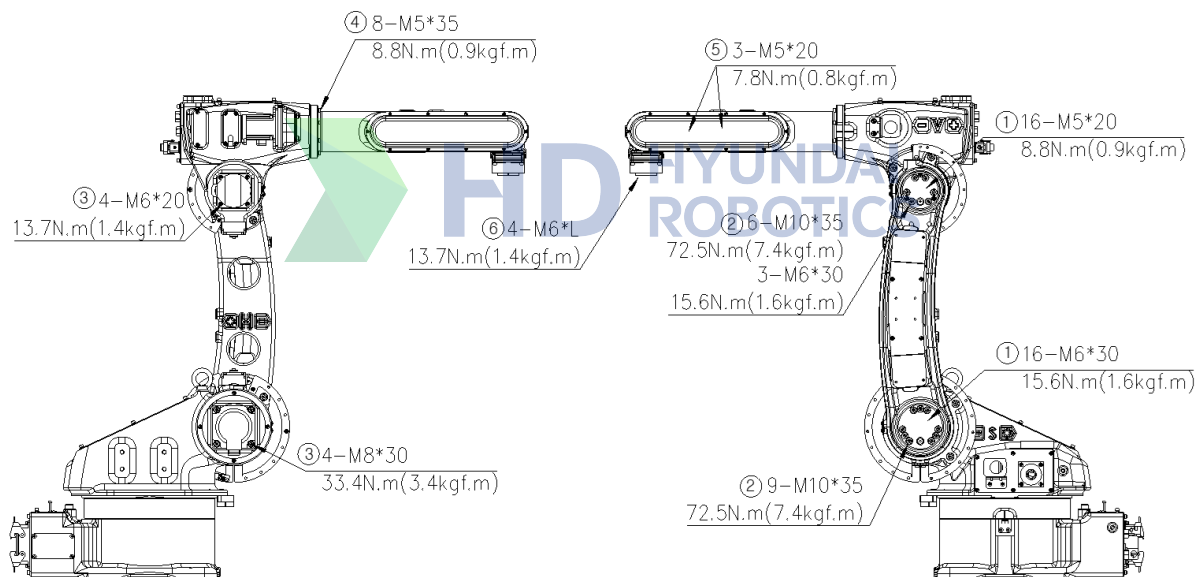
그림 4.1 주요 볼트 점검 부위 [HA006B]
