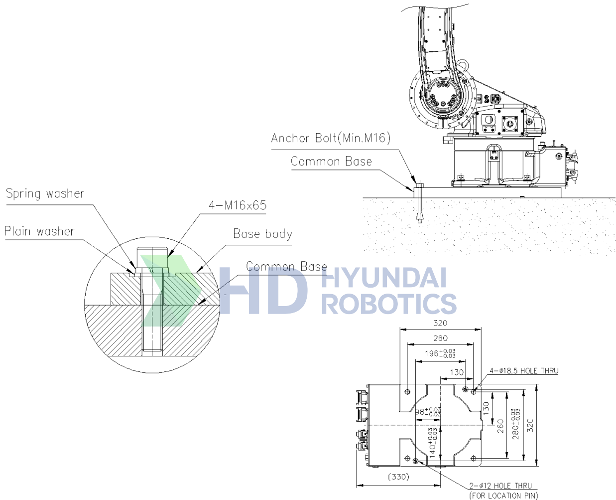
그림 3.9 로봇 설치면 치수 [HA006B]
