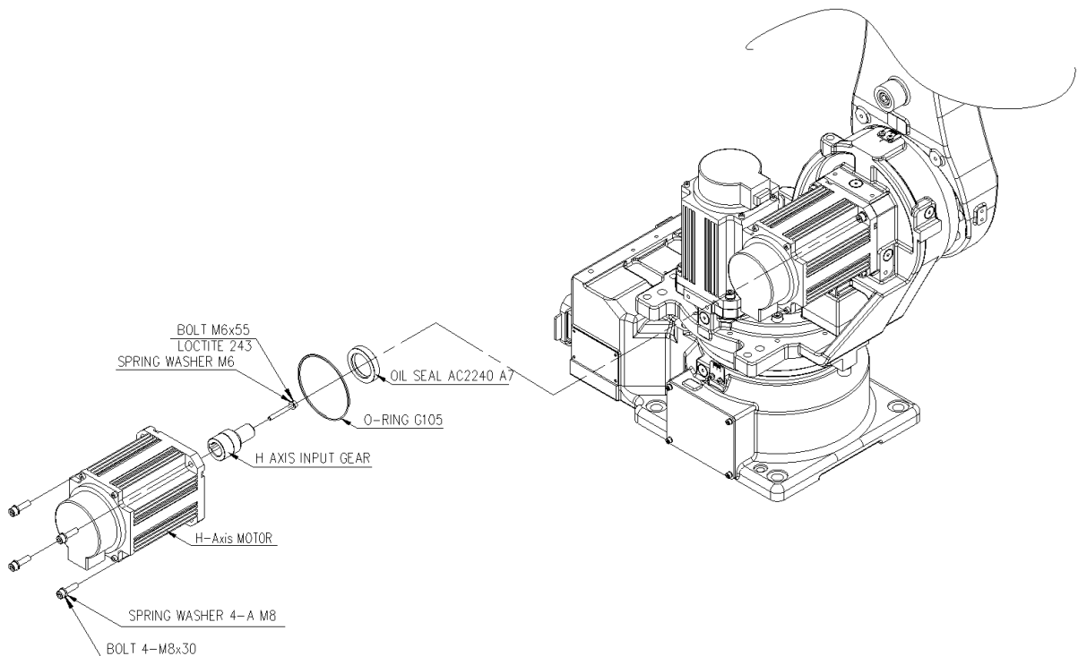
그림 6.9 H 축 모터 교체 [HA006L]
