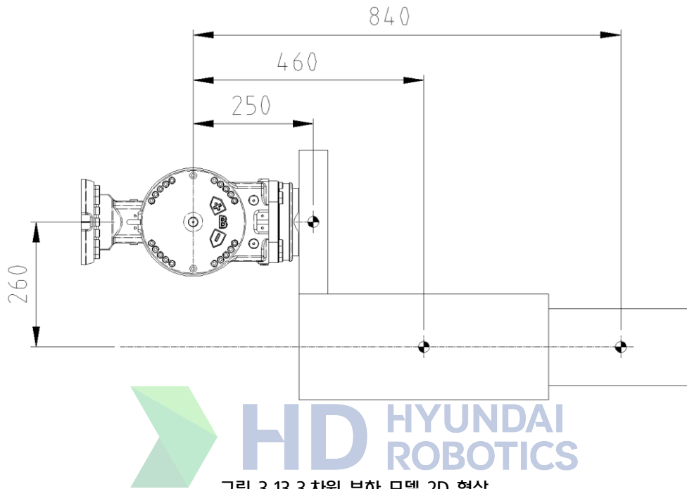
그림 3.13 3 차원 부하 모델 2D 형상
