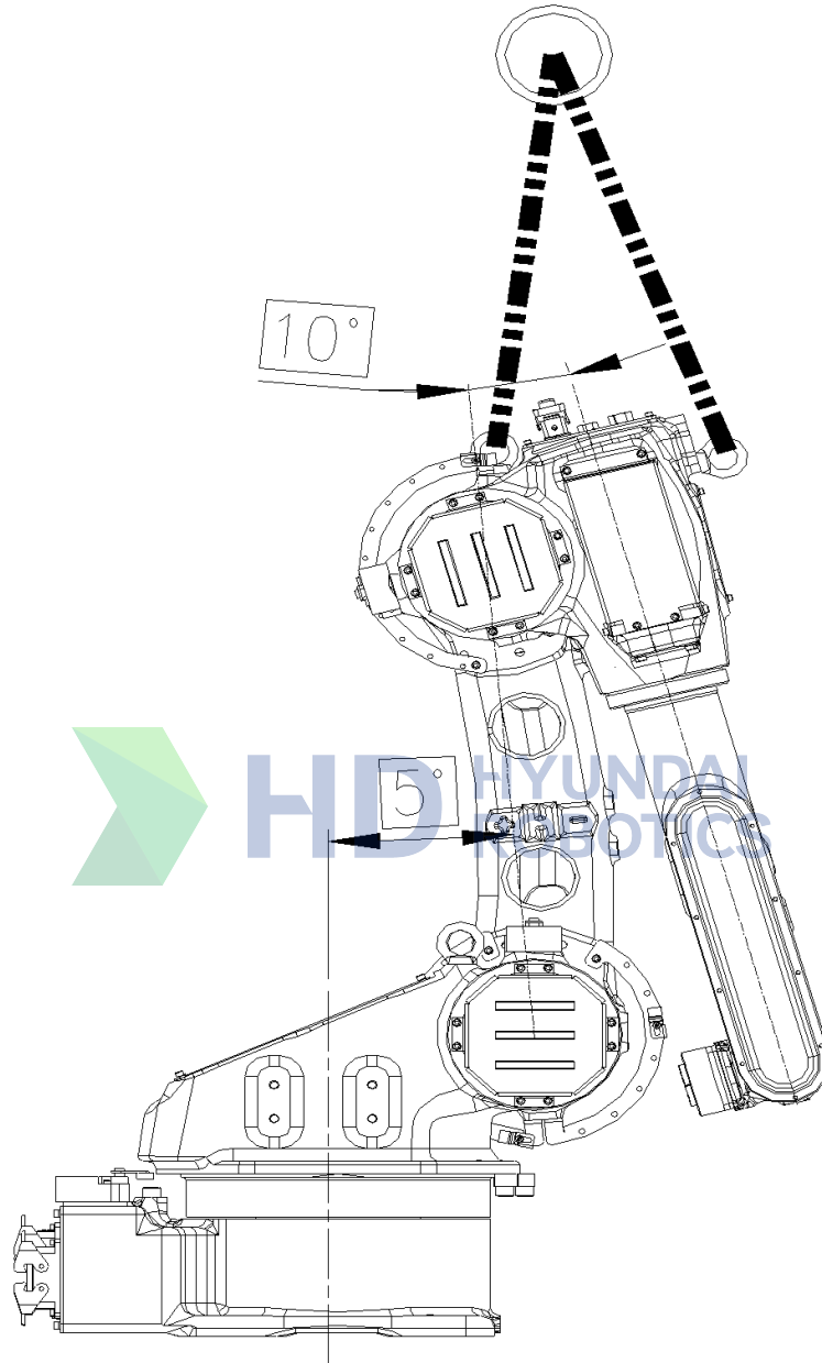
그림 6.15 H 축 감속기 교체시의 로봇 자세 [HA006B]
