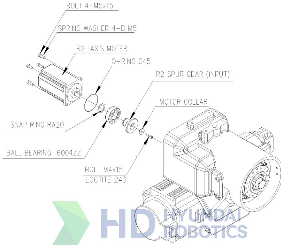
그림 6.11 R2 축 모터 교체 [HA006L]
