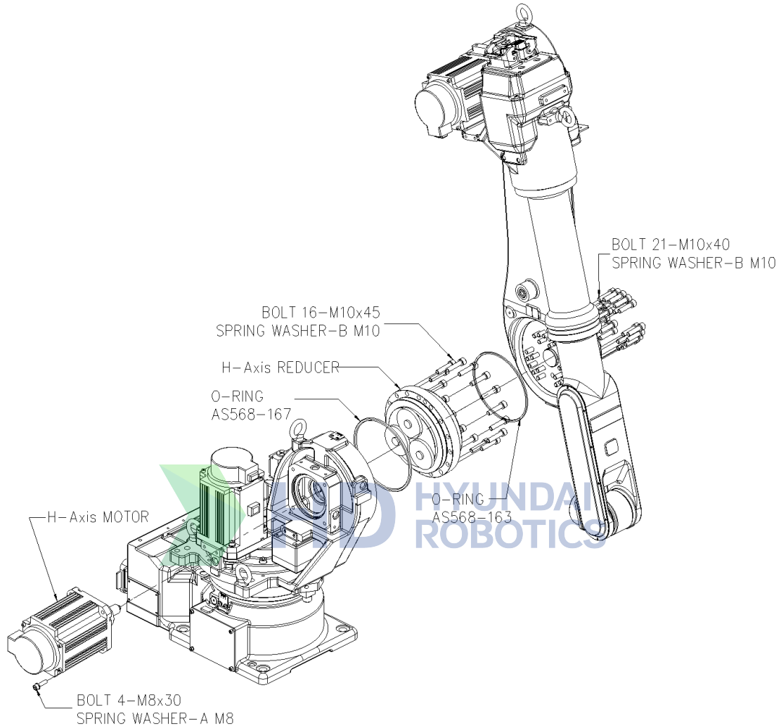
그림 6.22 H축 감속기 분해도[HA006L]
