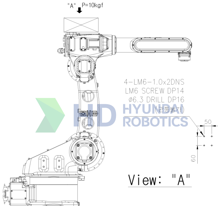
그림 2.7 제 1ARM 상부 부착부 상세도: [HA006B]
