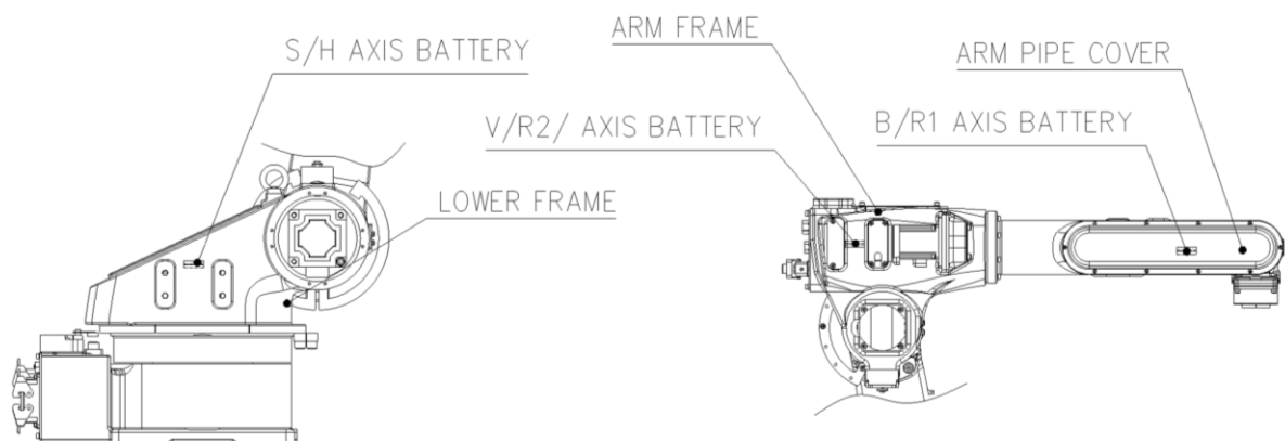
그림 5.5 배터리 교환 위치 [HA006B]
