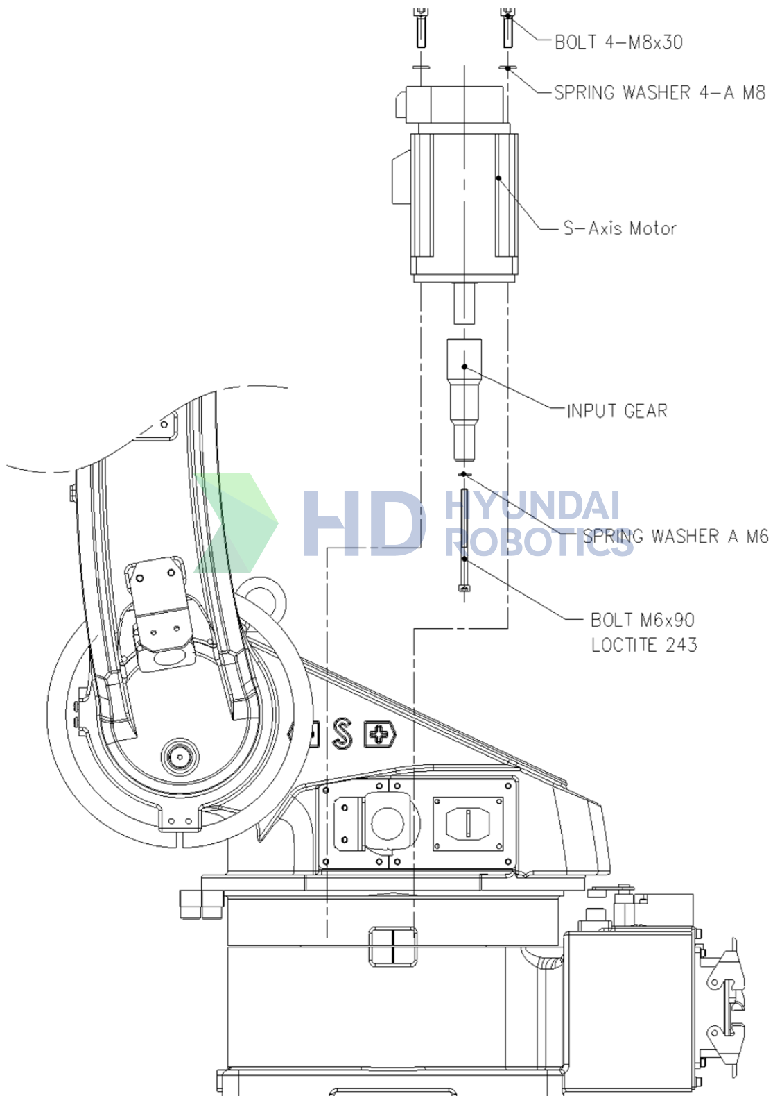
그림 6.1 S 축 모터 교체 [HA006B]
