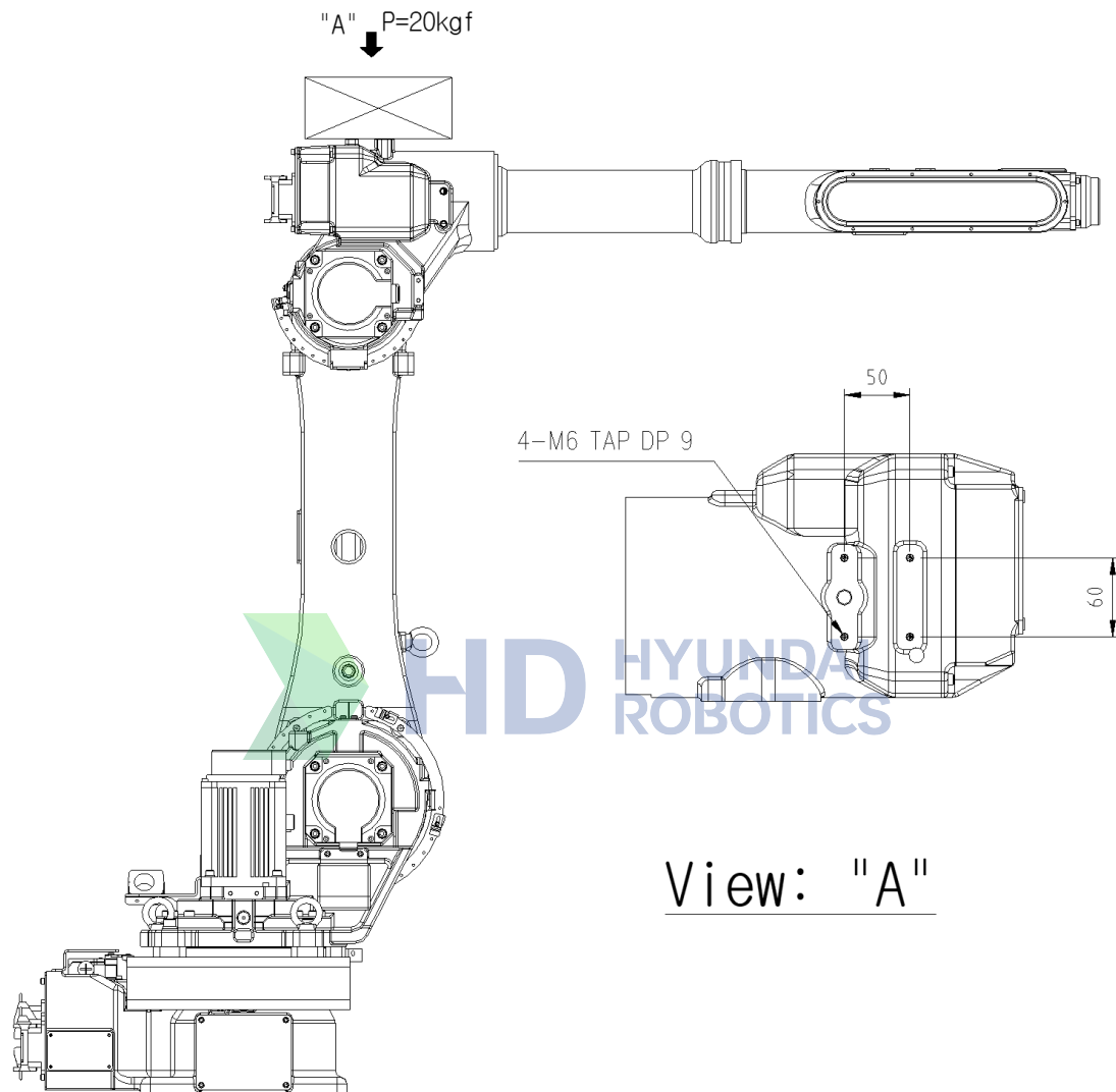
그림 2.8 제 1ARM 상부 부착부 상세도: [HA006L]
