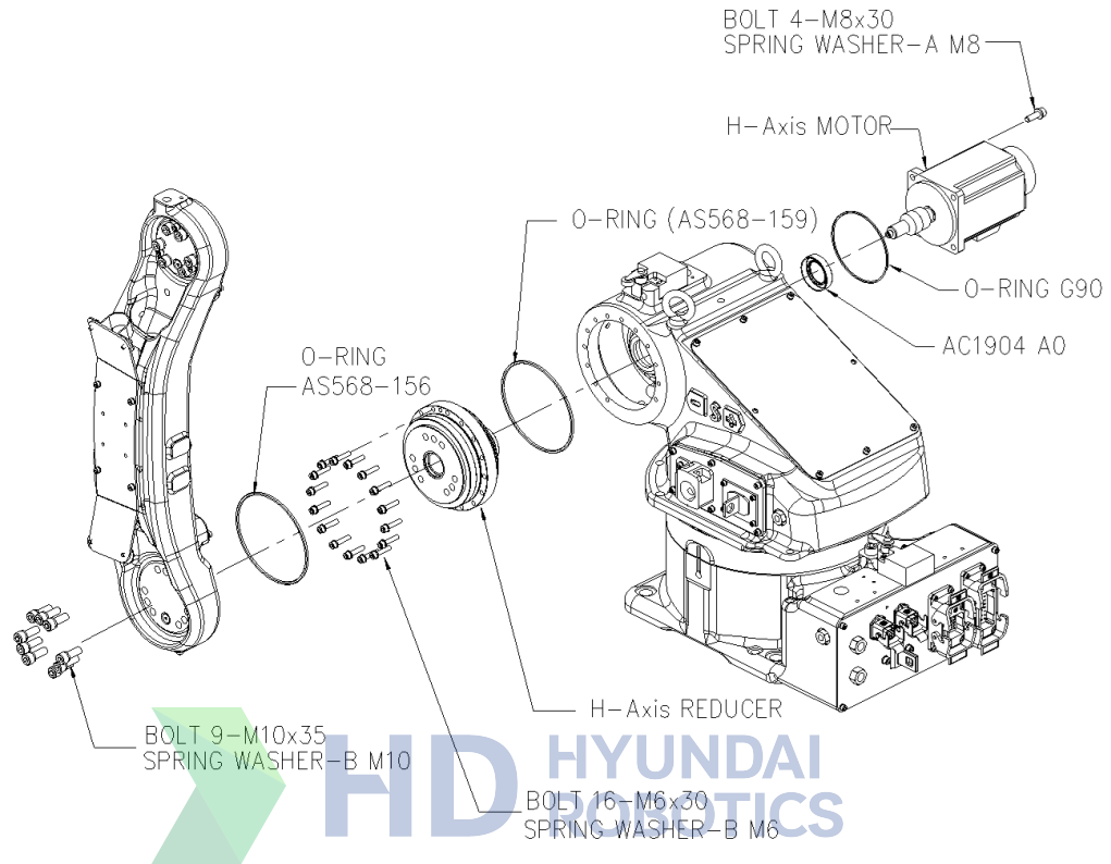
그림 6.16 H축 감속기 분해도 [HA006B]
