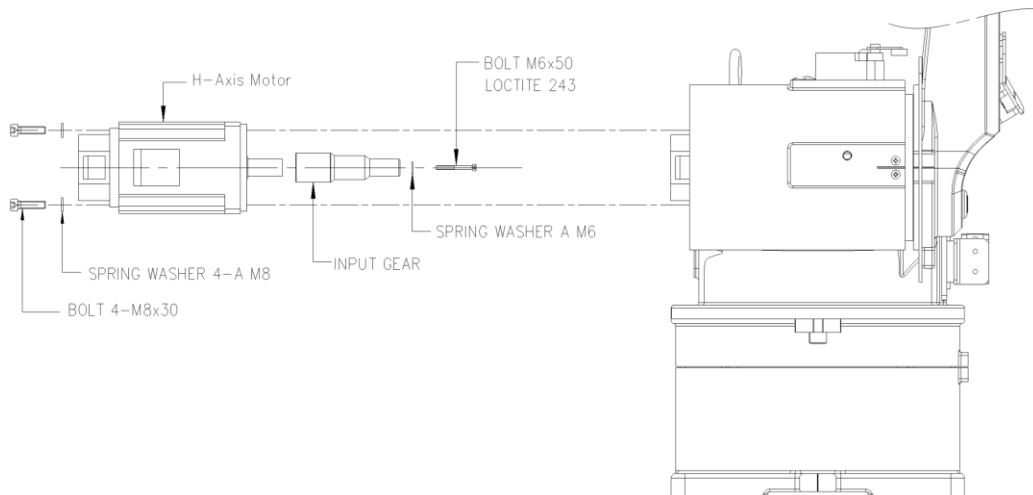
그림 6.3 H축 모터 교체 [HA006B]
