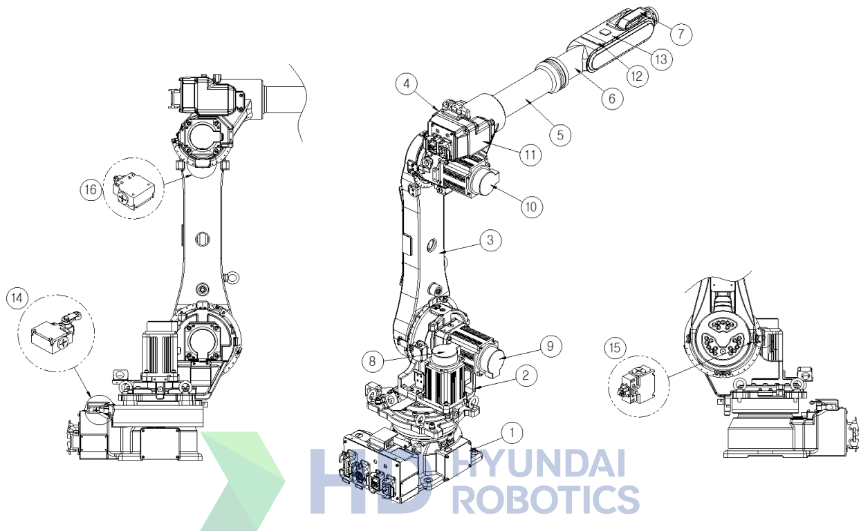
그림 3.2 본체 각 부위 명칭 [HA006L]
