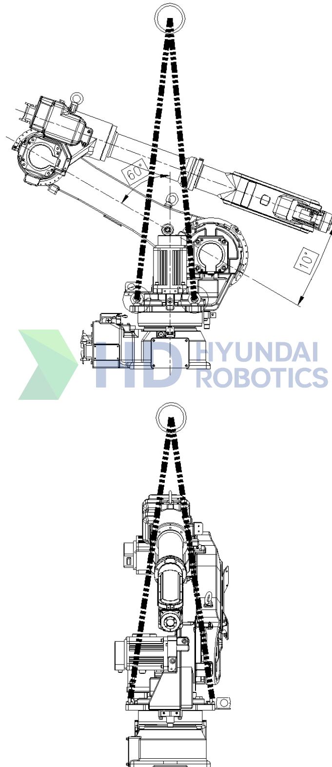
그림 6.19 S 축 감속기 교체시의 로봇 자세 [HA006L]
