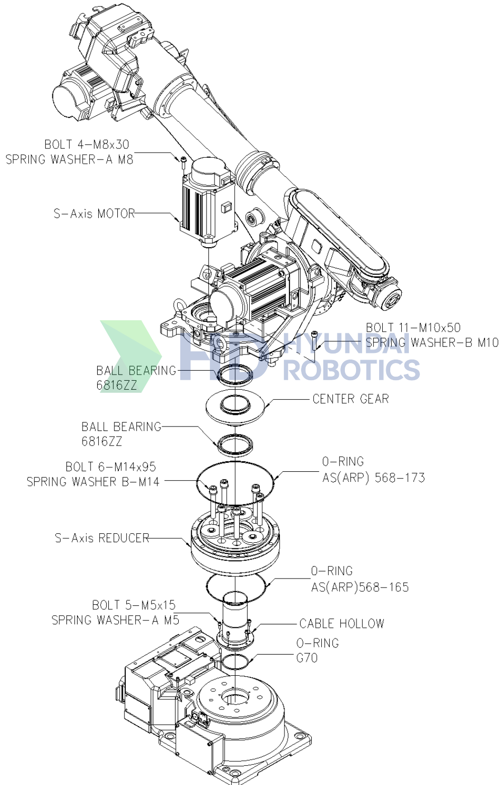
그림 6.20 S 축 감속기 분해도 [HA006L]
