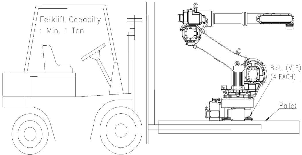
그림 3.8 운반 방법: 지게차 이용 [HA006L]
