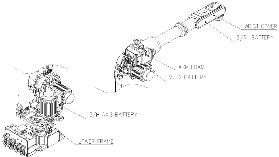
그림 5.6 배터리 교환 위치 [HA006L]
