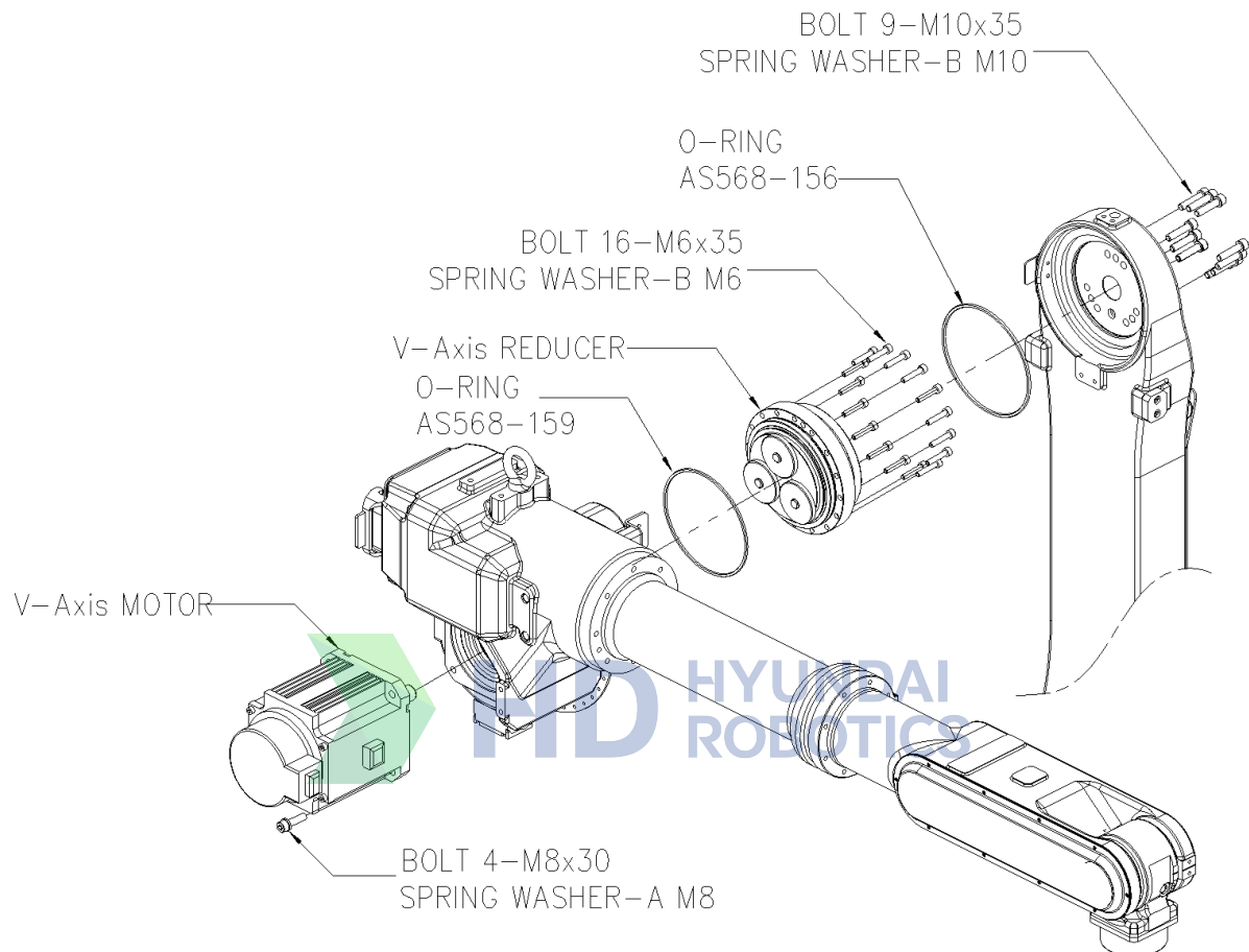
그림 6.24 V 축 감속기 분해도 [HA006L]
