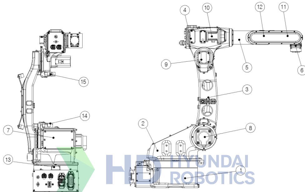
그림 3.1 본체 각 부위 명칭[HA006B]
