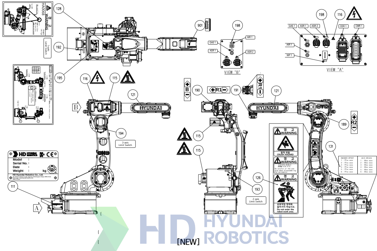
그림 3.3 안전 명판 위치 [HA006B]
