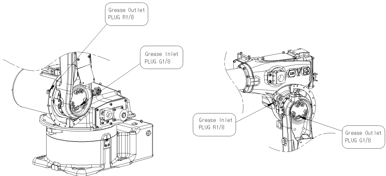
그림 5.3 H/V 축 그리스 IN/OUTLET 위치 [HA006B]
