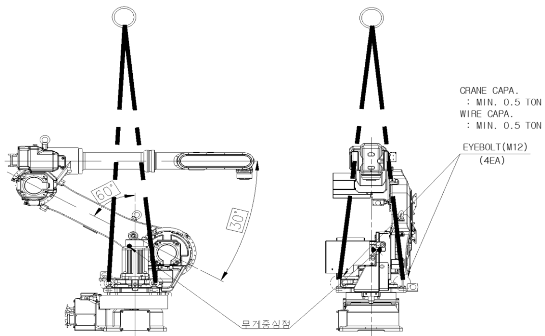
그림 3.6 운반 방법: 크레인 이용 [HA006L]
