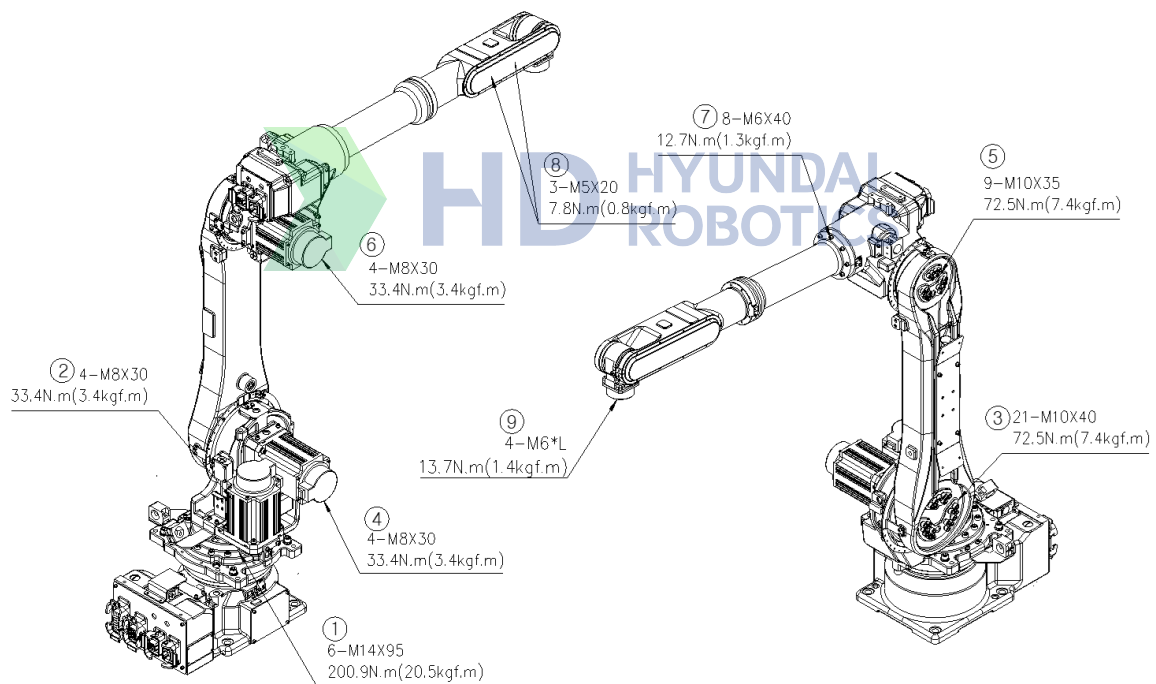
그림 4.2 주요 볼트 점검 부위 [HA006L]
