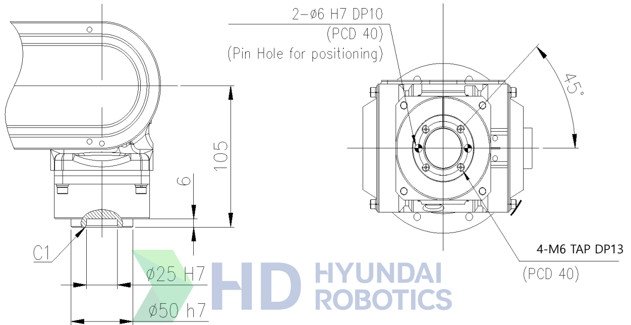
그림 2.6 손목축 취부면 상세도
