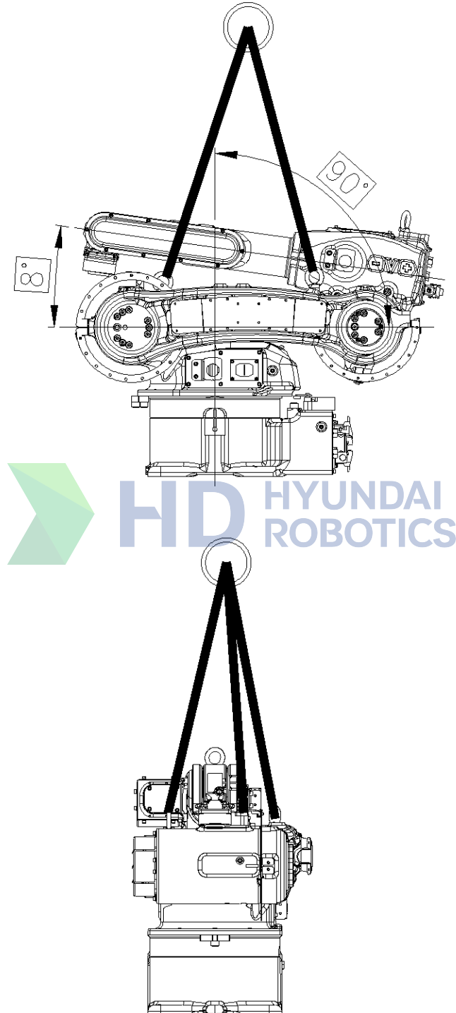
그림 6.13 S 축 감속기 교체시의 로봇 자세 [HA006B]
