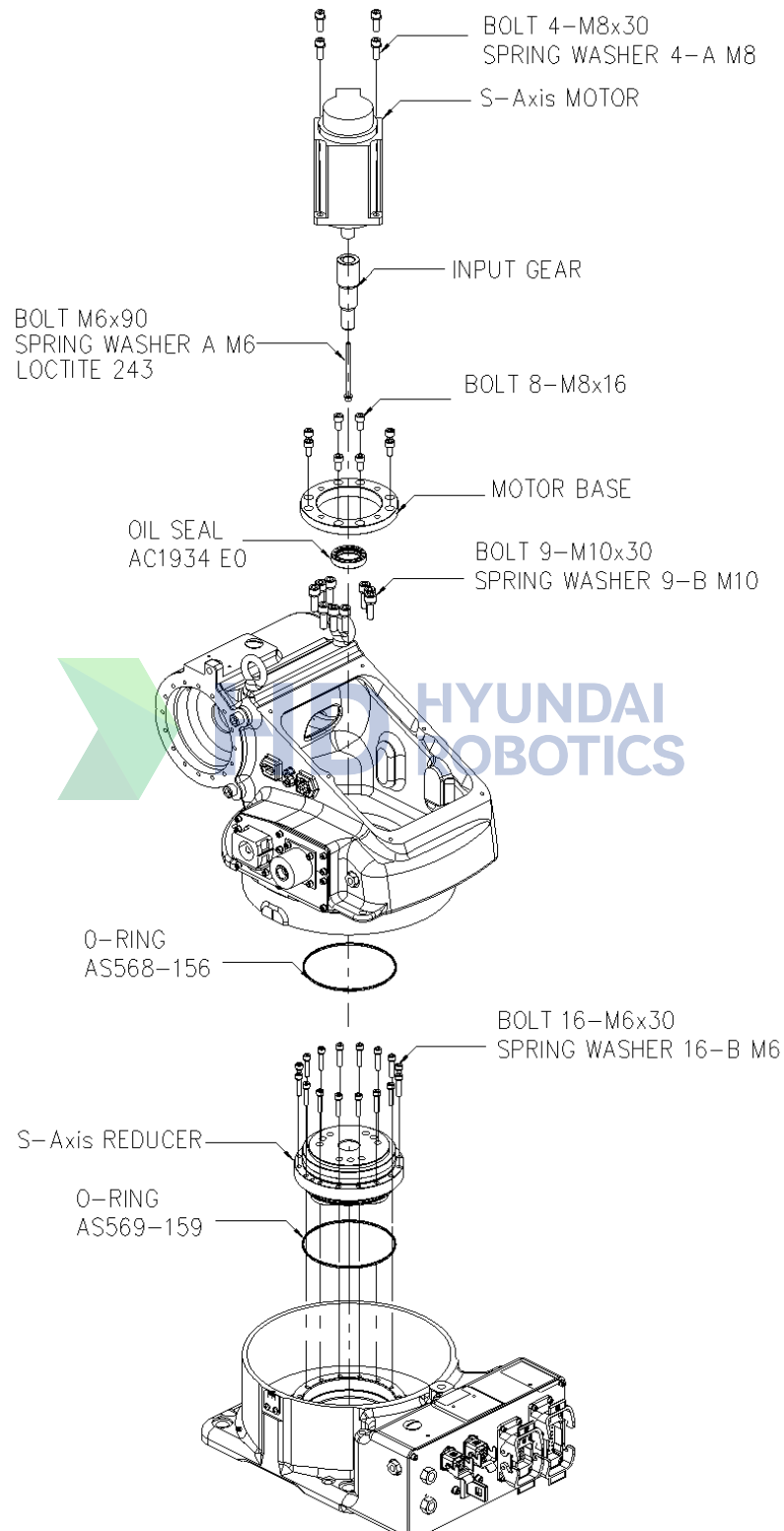
그림 6.14 S 축 감속기 분해도 [HA006B]
