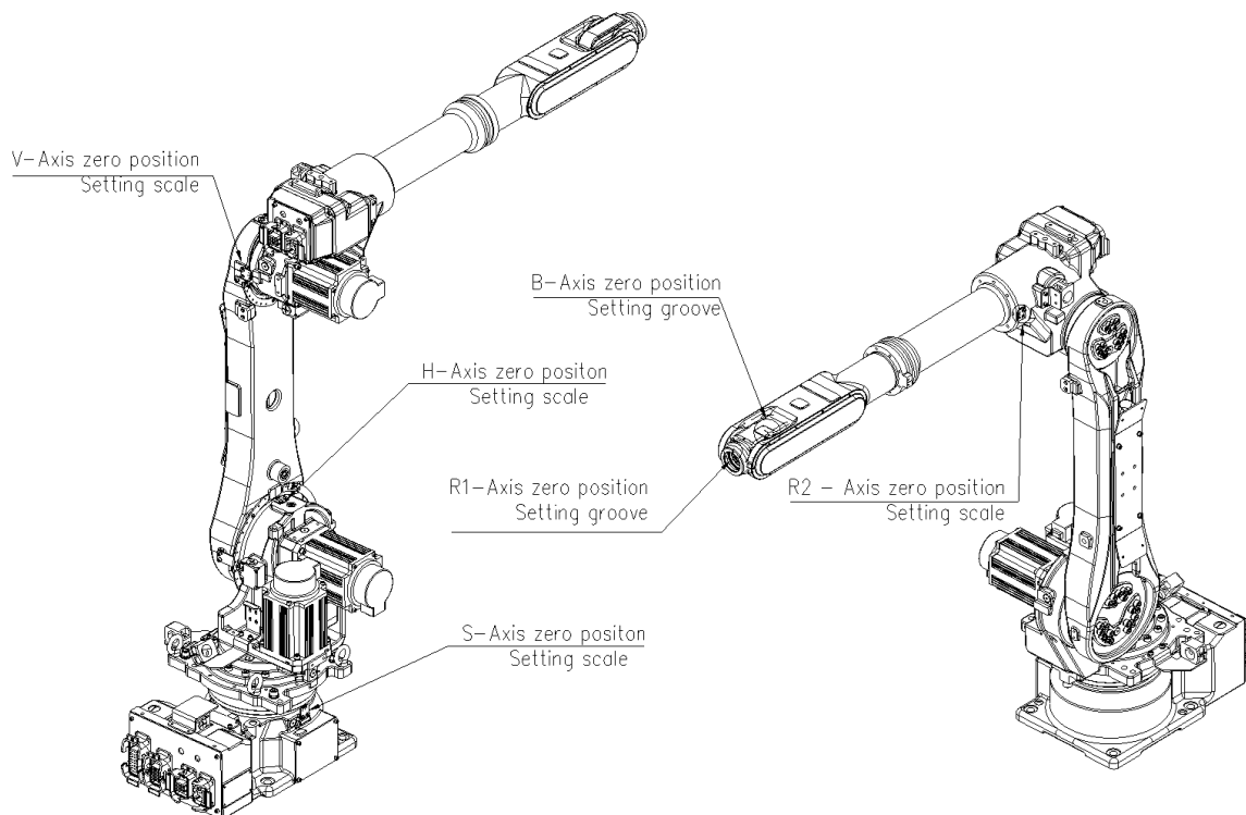
그림 6.26 원점 설정 방법 [HA006L]
