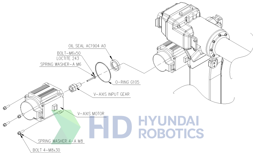
그림 6.10 V 축 모터 교체 [HA006L]
