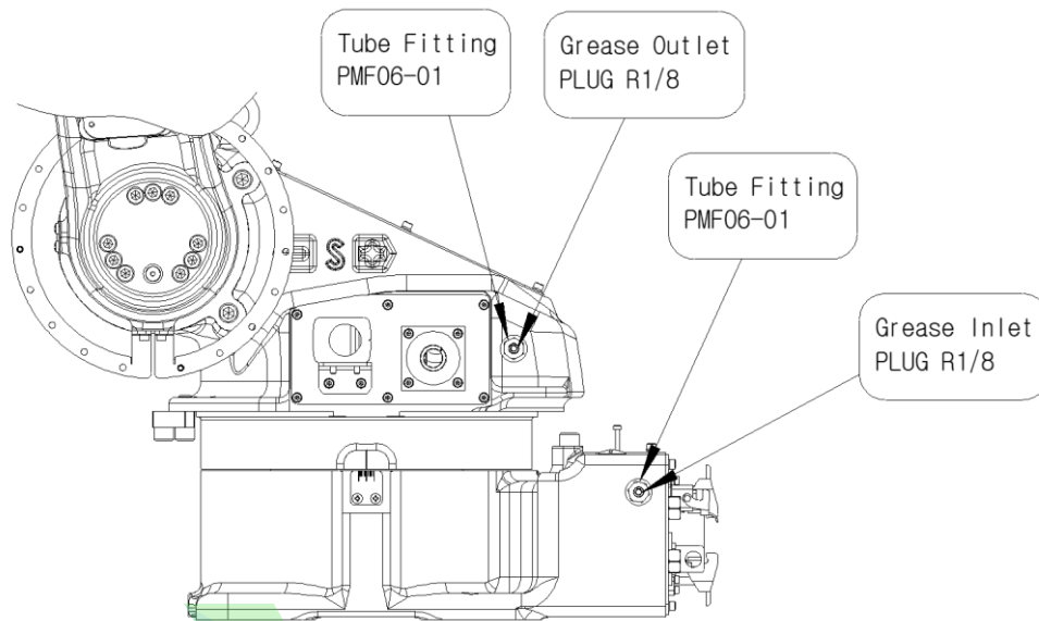
그림 5.1 S 축 그리스 IN/OUTLET 위치 [HA006B]
