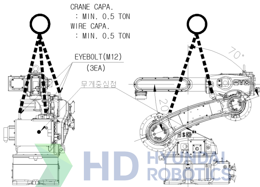
그림 3.5 운반 방법: 크레인 이용 [HA006B]
