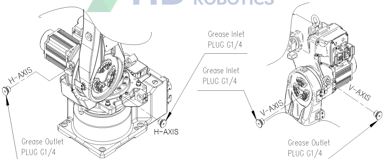
그림 5.4 H/V 축 그리스 IN/OUTLET 위치 [HA006L]
