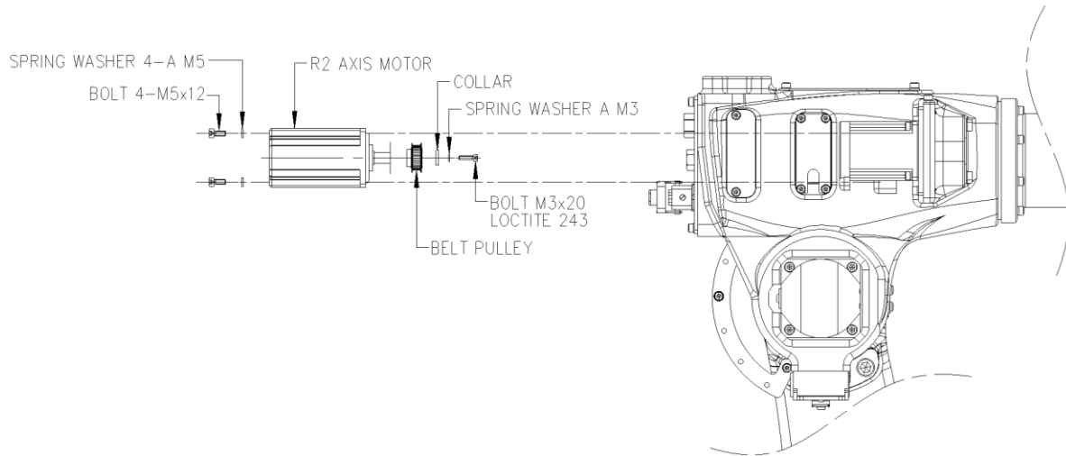
그림 6.6 R2 축 모터 교체 [HA006B]
