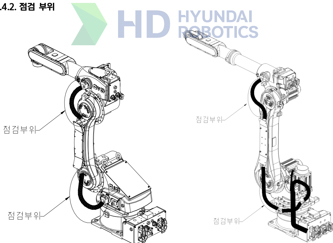
그림 4.3 케이블 점검 부위 [HA006B/HA006L]
