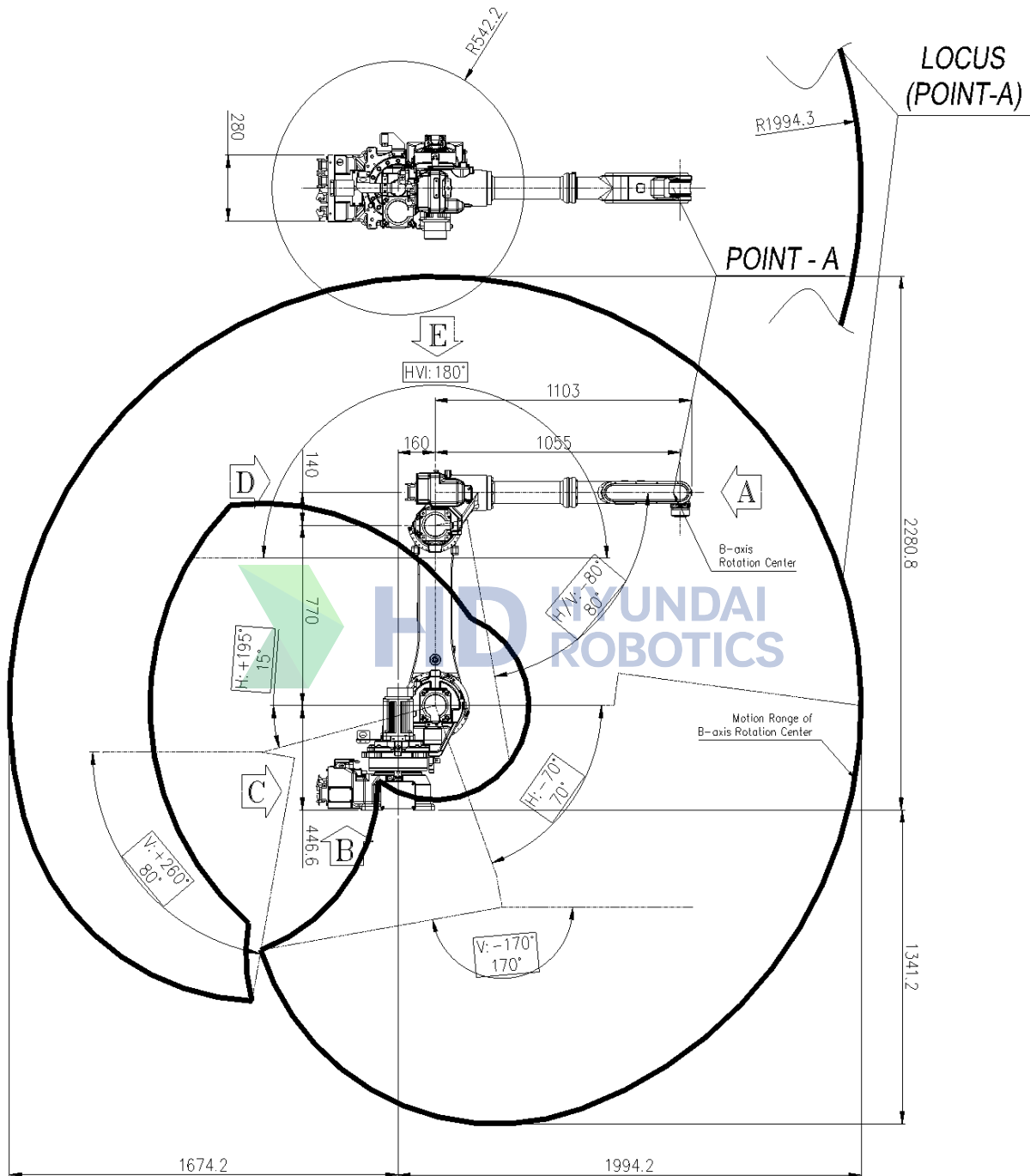
그림 2.4 로봇 본체 외형 치수 및 동작 영역: [HA006L]
