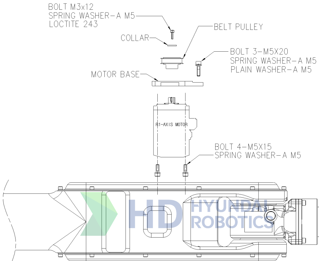
그림 6.12 B/R1 축 모터교체 (HA006B/HA006L)
