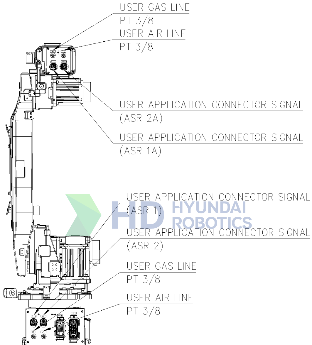
그림 2.10 어플리케이션용 배선 및 배관도: [HA006L]
