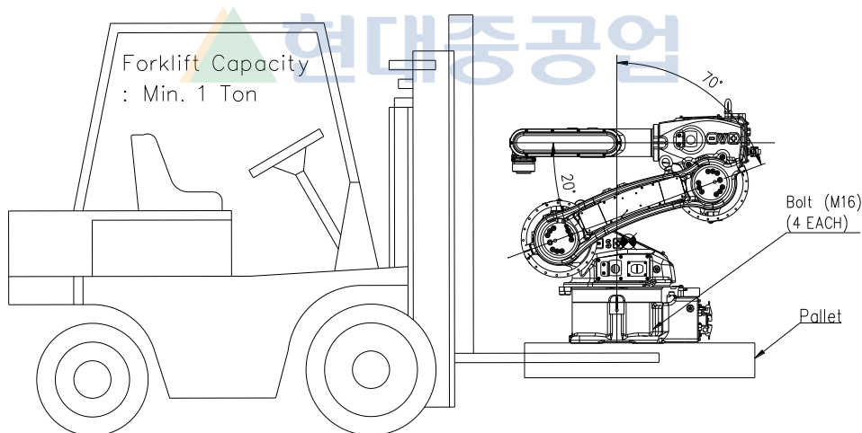
그림 3.7 운반 방법: 지게차 이용 [HA006A]
