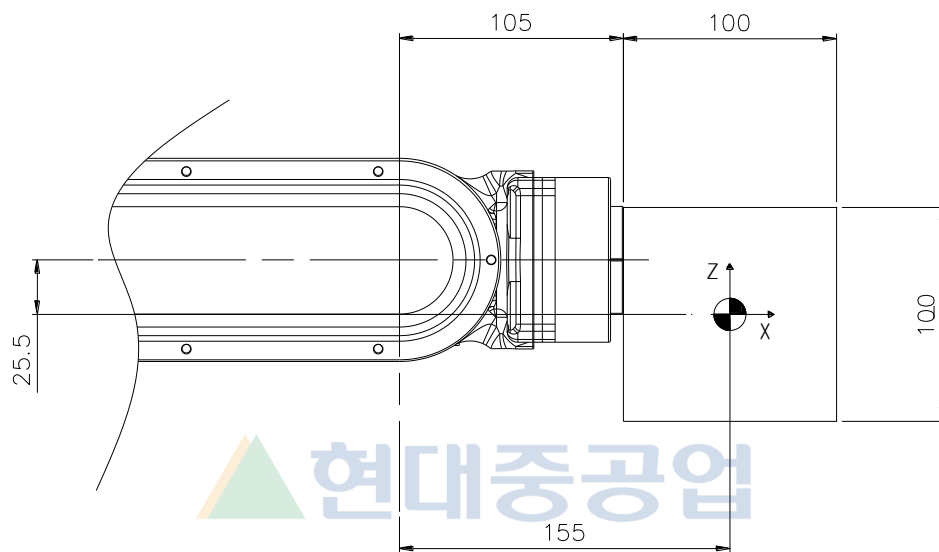
그림 3.12 2 차원 부하 모델
