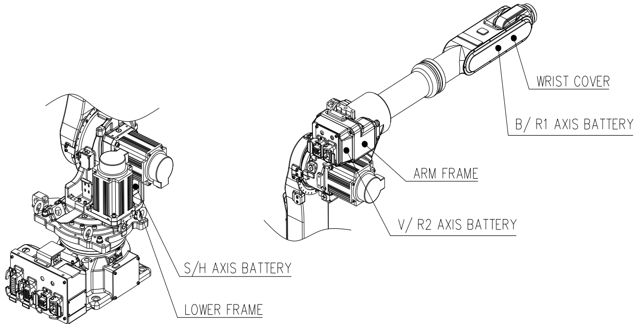
그림 5.6- 배터리 교환 위치 [HA006L]
