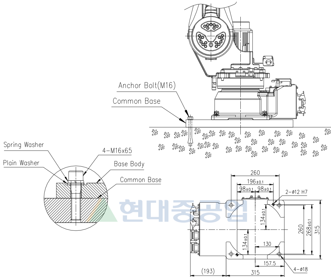
그림 3.10 로봇 설치면 치수 [HA006L]
