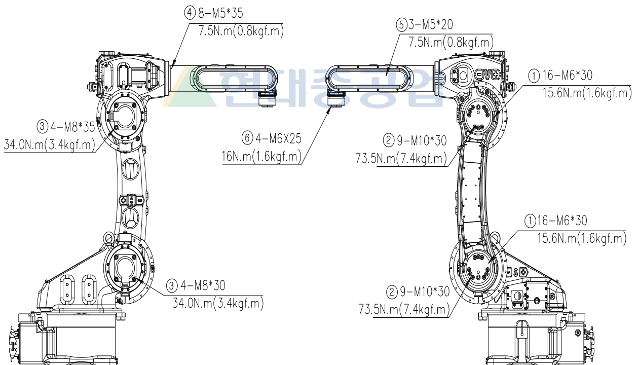
그림 4.1 주요 볼트 점검 부위 [HA006A]
