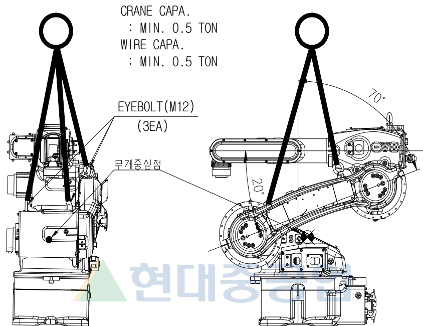
그림 3.5 운반 방법: 크레인 이용 [HA006A]
