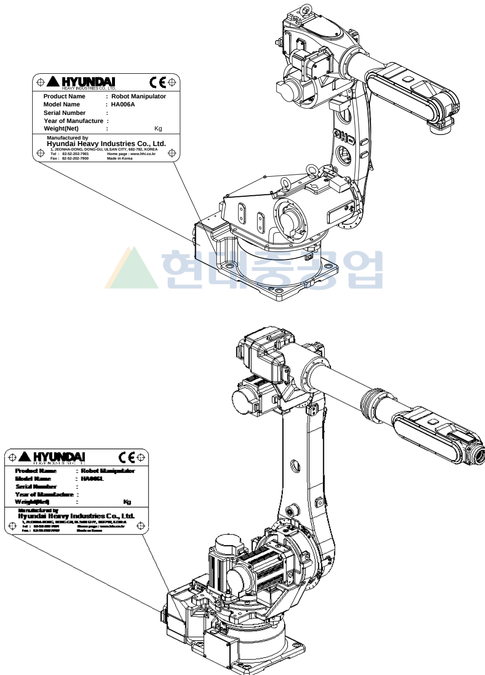
그림 2.2 로봇 명판 부착 위치 [HA006A/HA006L]
