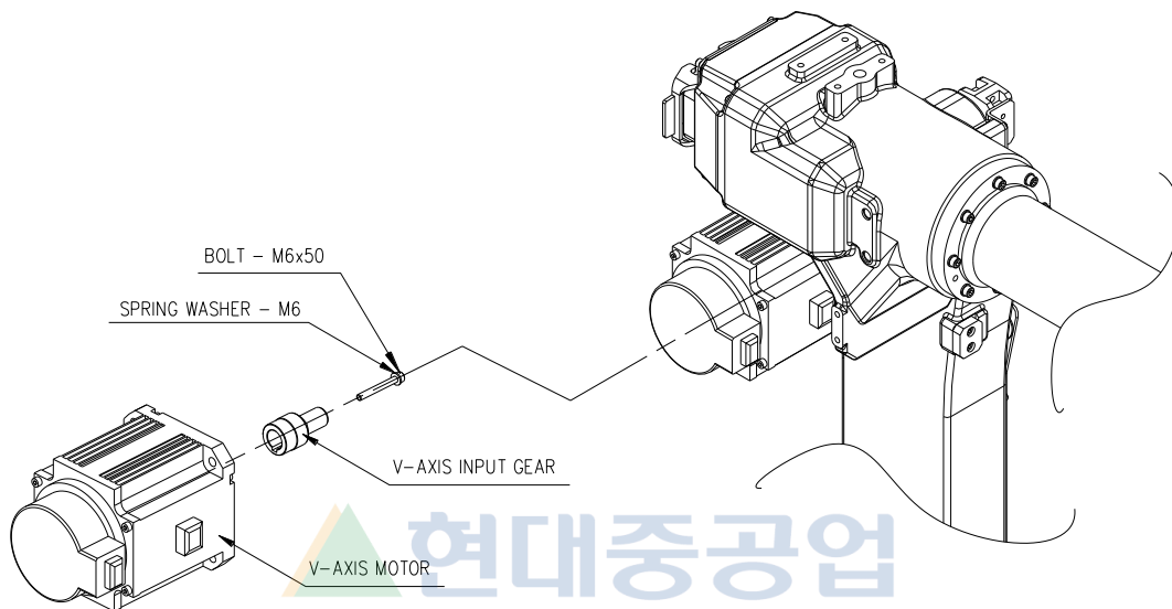
그림 6.10 V 축 모터 교체 [HA006L]
