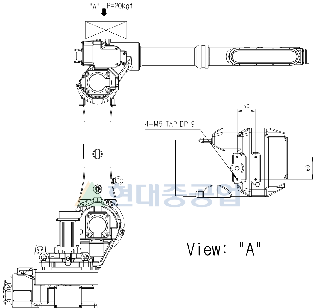
그림 2.8 제 1ARM 상부 부착부 상세도: [HA006L]
