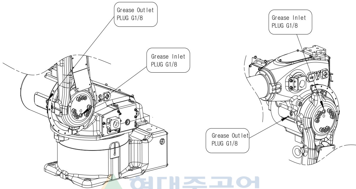
그림 5.3 H/V 축 그리스 IN/OUTLET 위치 [HA006A]
