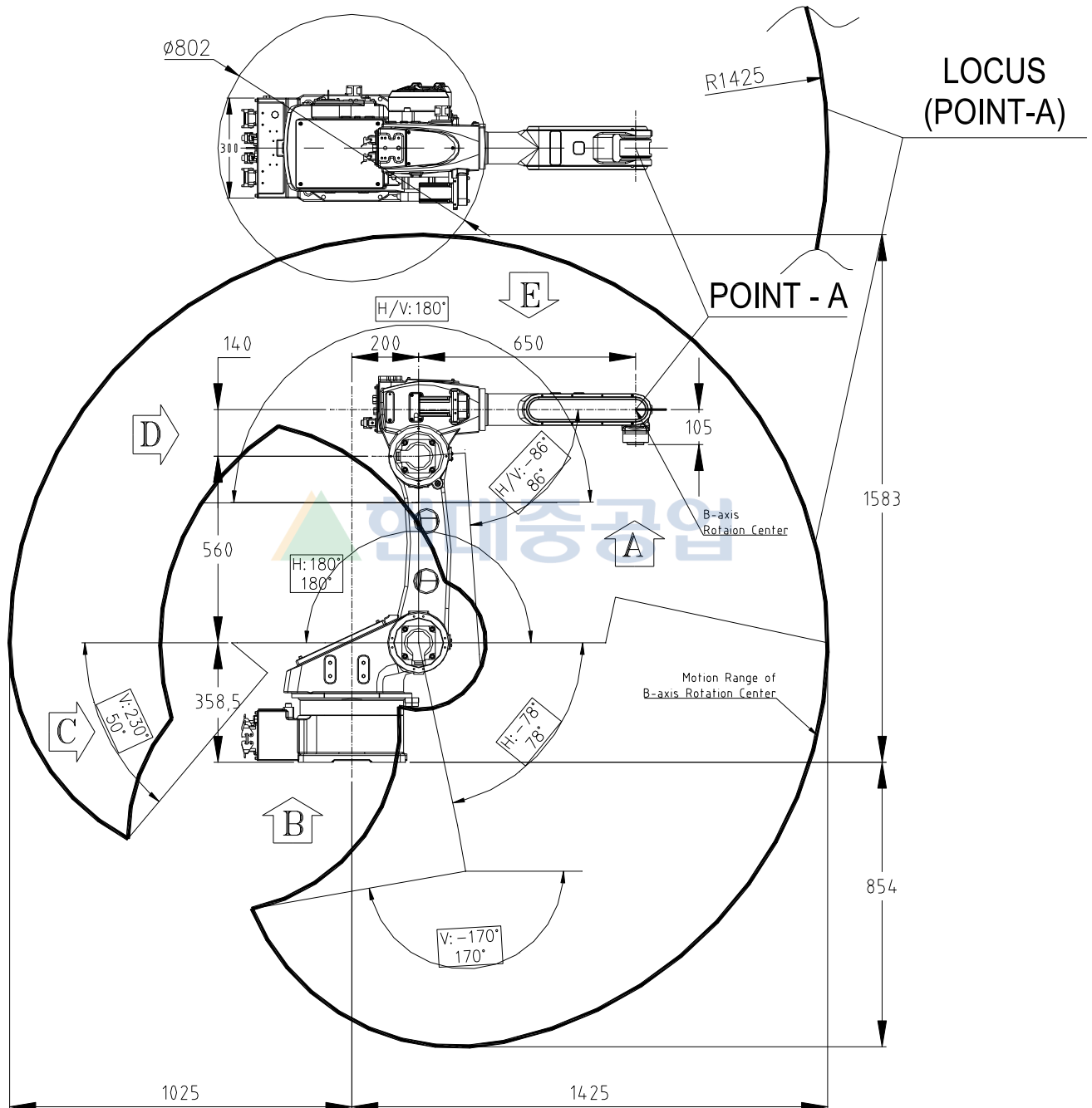
그림 2.3 로봇 본체 외형 치수 및 동작 영역: [HA006A]
