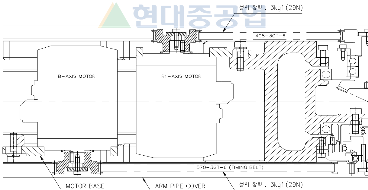
그림 4.4 B 축 타이밍 벨트 장력 체크 부위
