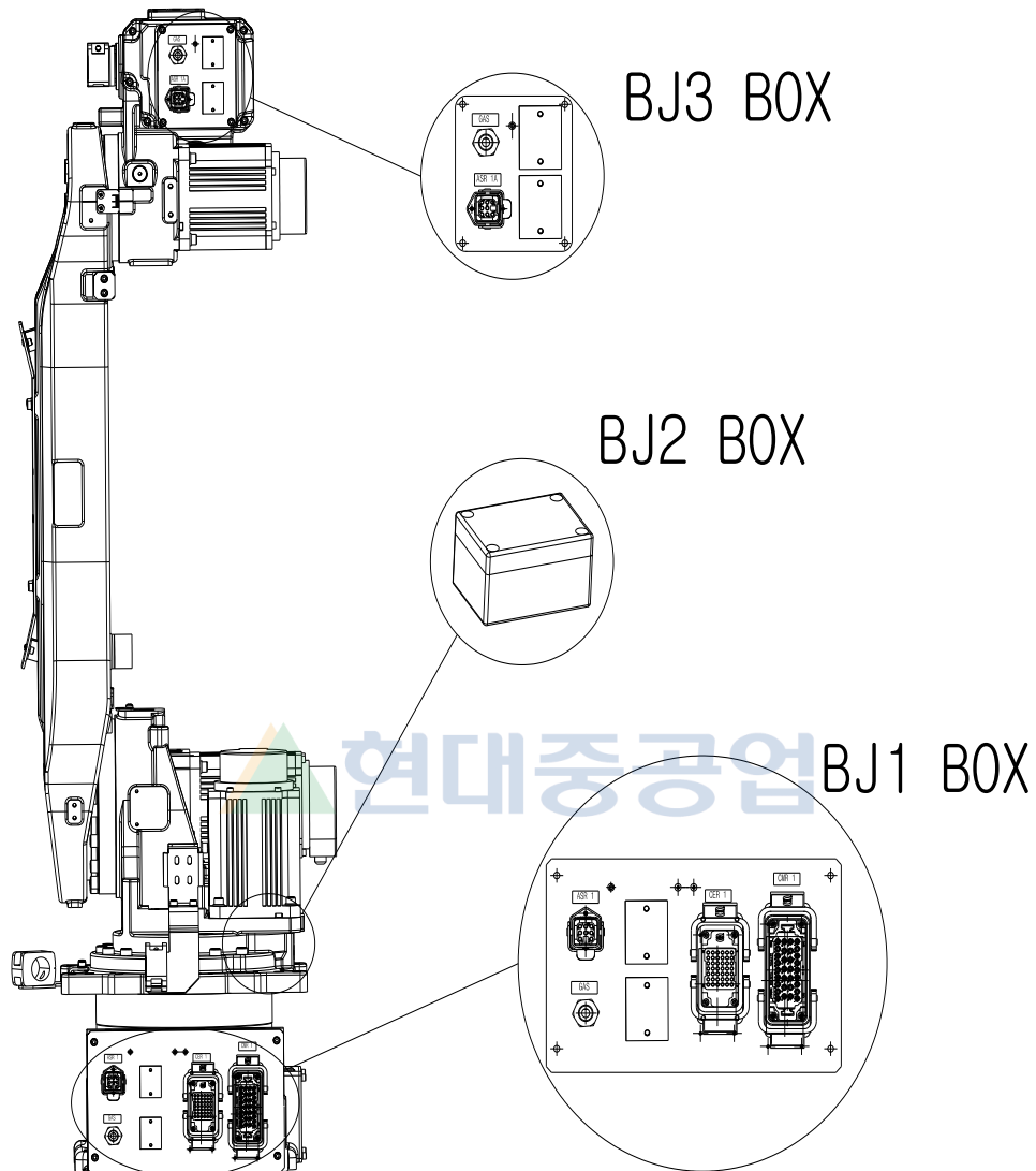
그림 8.2 본체 부품 배치 [HA006L]
