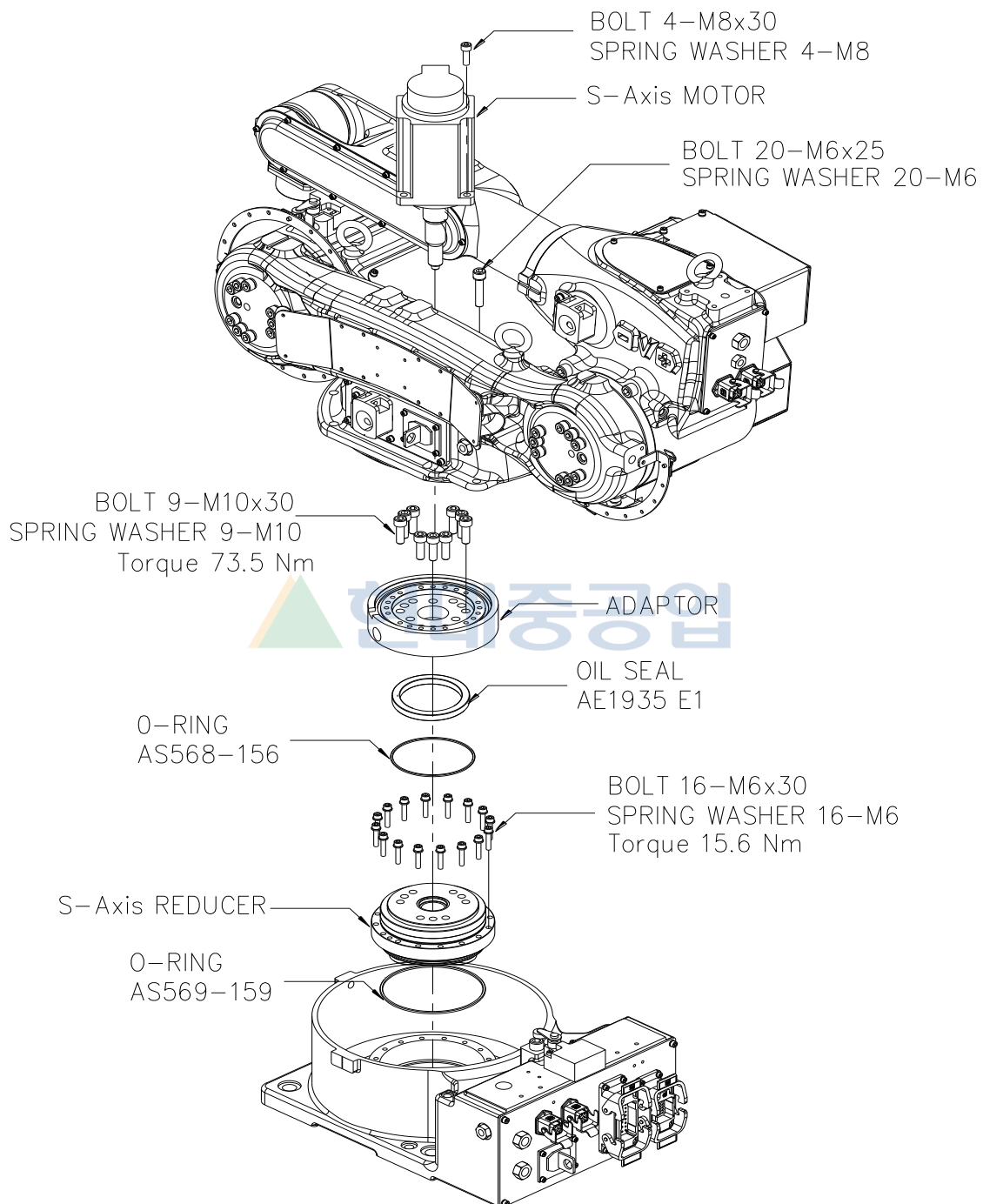
그림 6.14 S 축 감속기 분해도 [HA006A]
