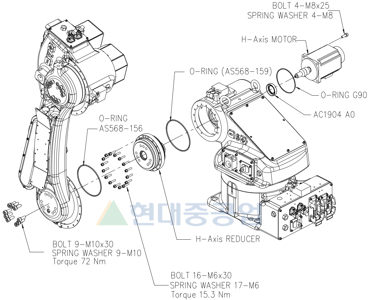
그림 6.16 H 축 감속기 분해도 [HA006A]
