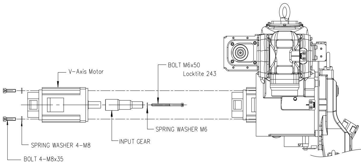
그림 6.5 V 축 모터 교체 [HA006A]
