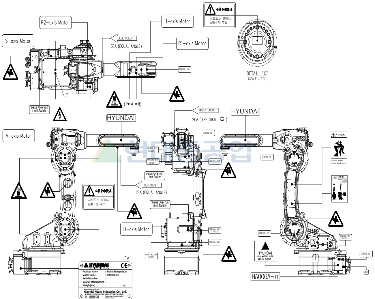
그림 3.3 안전 명판 위치 [HA006A]
