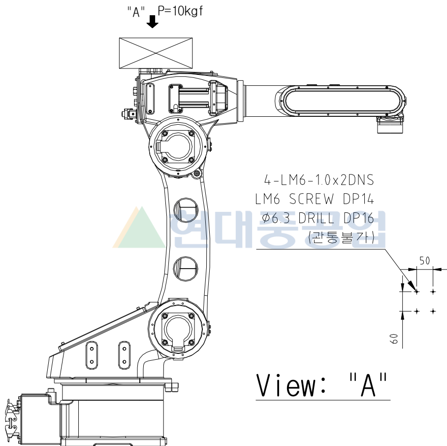
그림 2.7 제 1ARM 상부 부착부 상세도: [HA006A]
