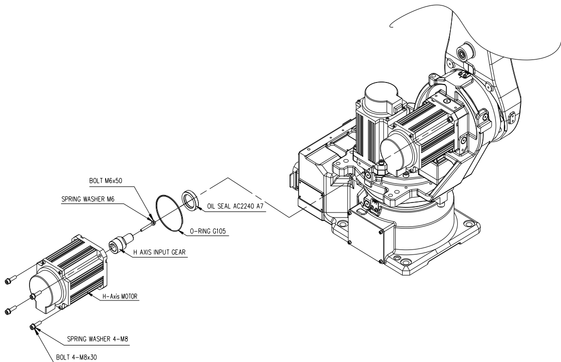
그림 6.9 H 축 모터 교체 [HA006L]
