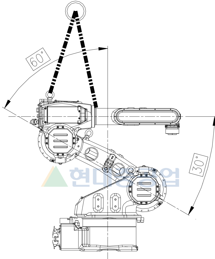
그림 6.17 V 축 감속기 교체시의 로봇 자세 [HA006A]
