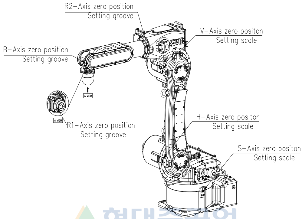
그림 6.25 원점 설정 방법 [HA006A]
