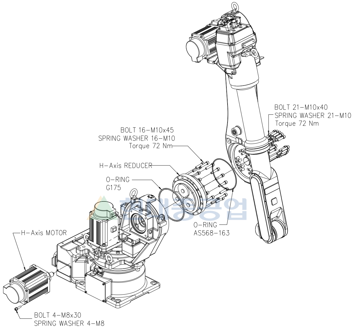
그림 6.22 H 축 감속기 분해도 [HA006L]
