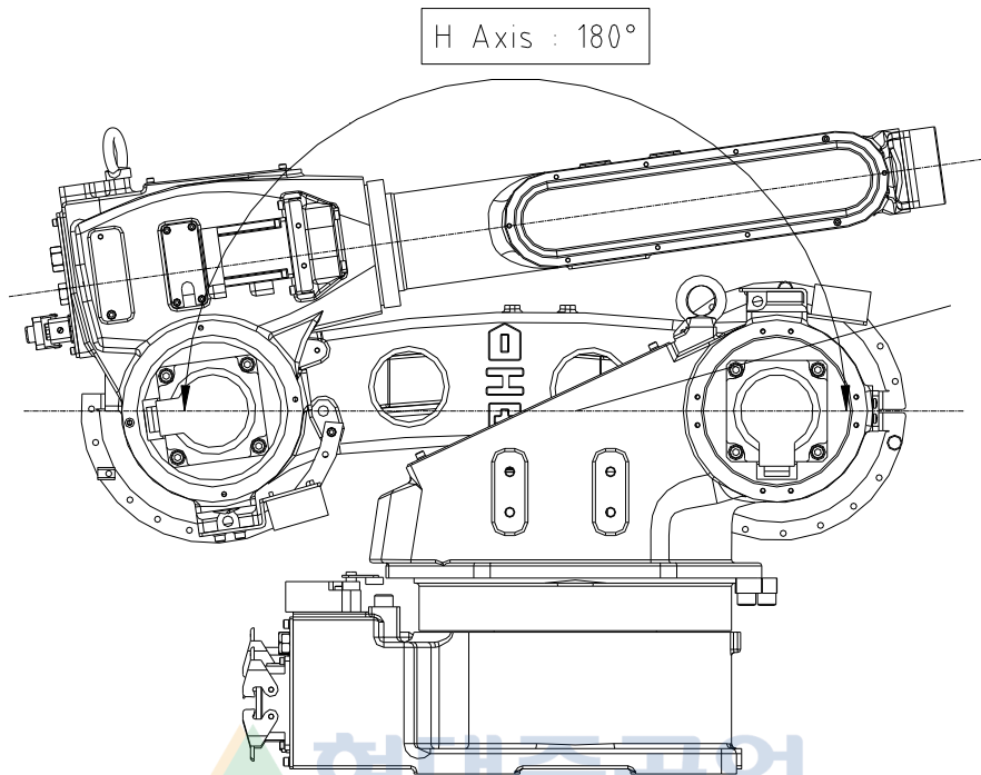
그림 6.2 H축 모터 교체시의 로봇 자세 [HA006A]
