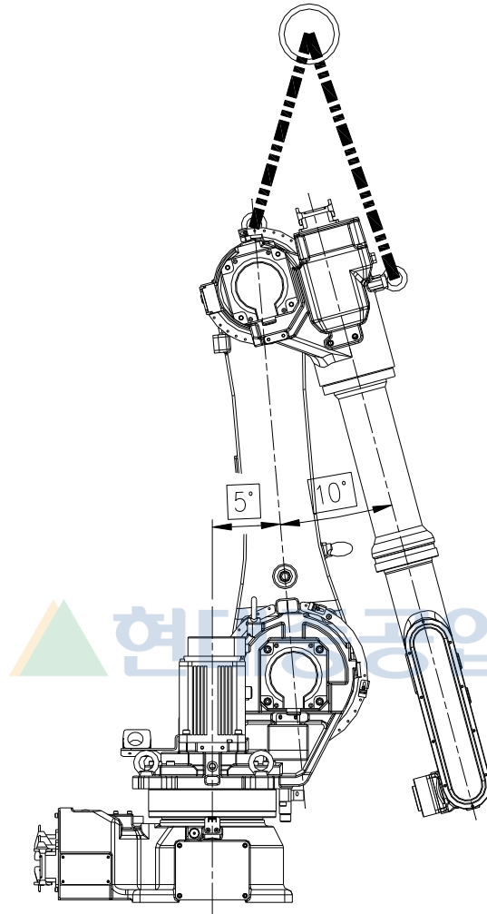
그림 6.21 H축 감속기 교체시의 로봇 자세 [HA006L]
