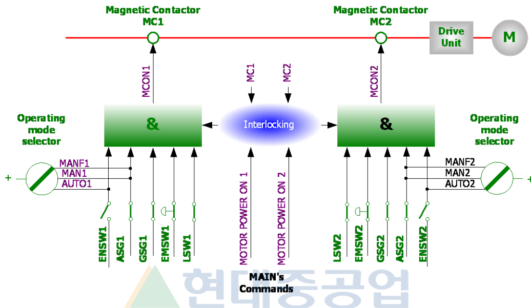
그림 1.5 안전체인 구성도
