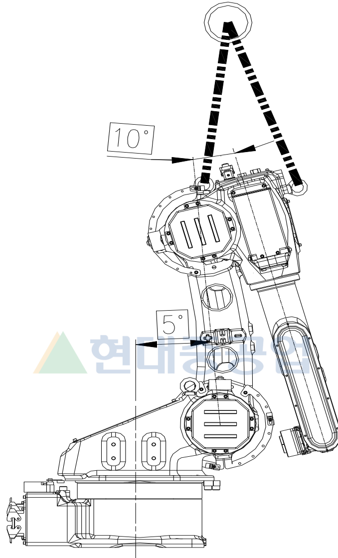
그림 6.15 H 축 감속기 교체시의 로봇 자세 [HA006A]
