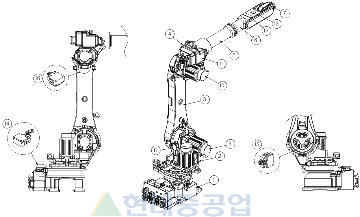
그림 3.2 본체 각 부위 명칭 [HA006L]
