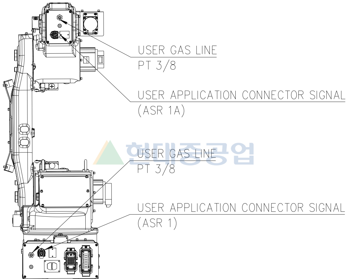
그림 2.9 어플리케이션용 배선 및 배관도: [HA006A]
