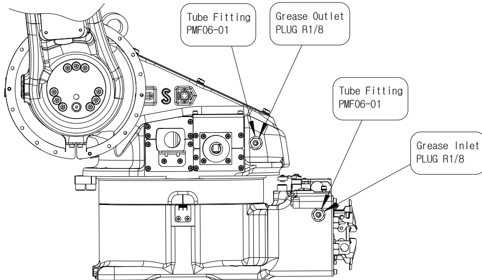
그림 5.1 S 축 그리스 IN/OUTLET 위치 [HA006A]
