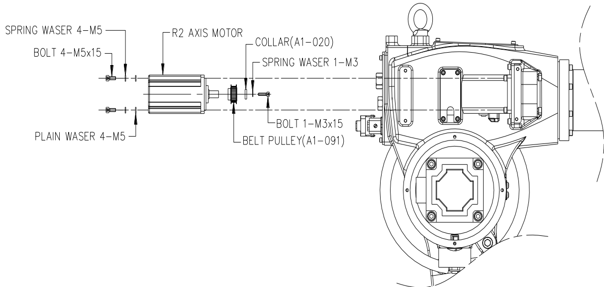
그림 6.6 R2 축 모터 교체 [HA006A]
