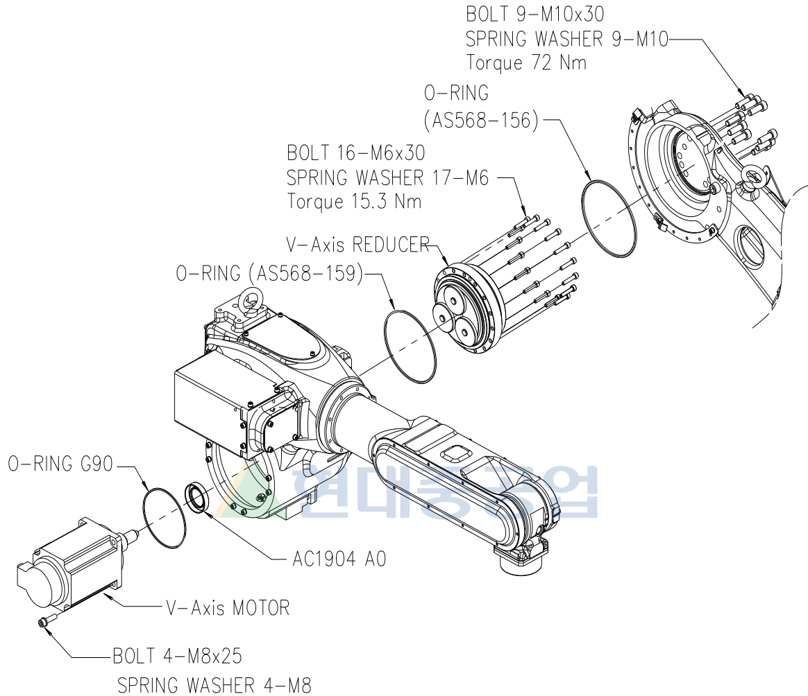
그림 6.18 V 축 감속기 분해도 [HA006A]
