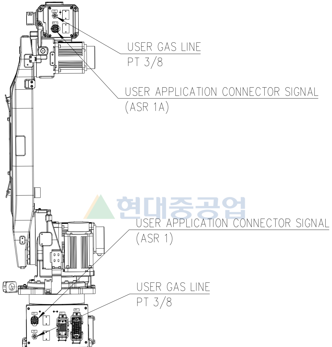
그림 2.10 어플리케이션용 배선 및 배관도: [HA006L]
