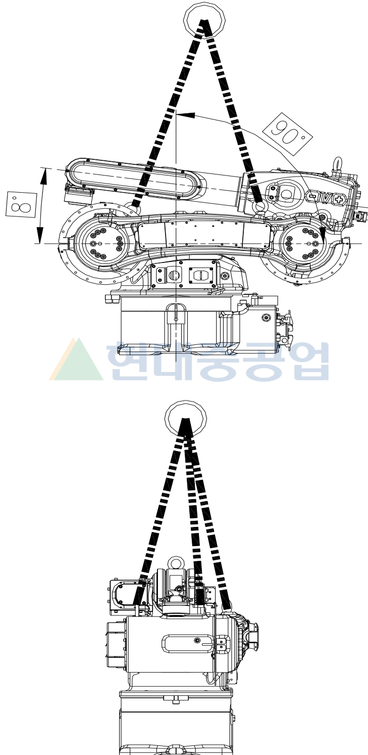
그림 6.13 S 축 감속기 교체시의 로봇 자세 [HA006A]
