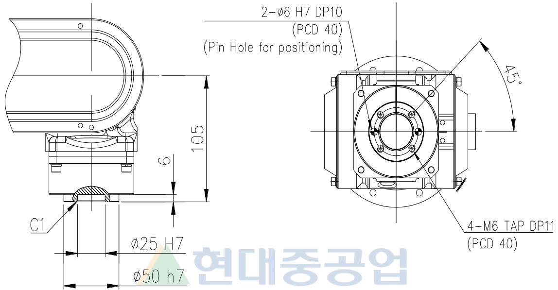
그림 2.6 손목축 취부면 상세도
