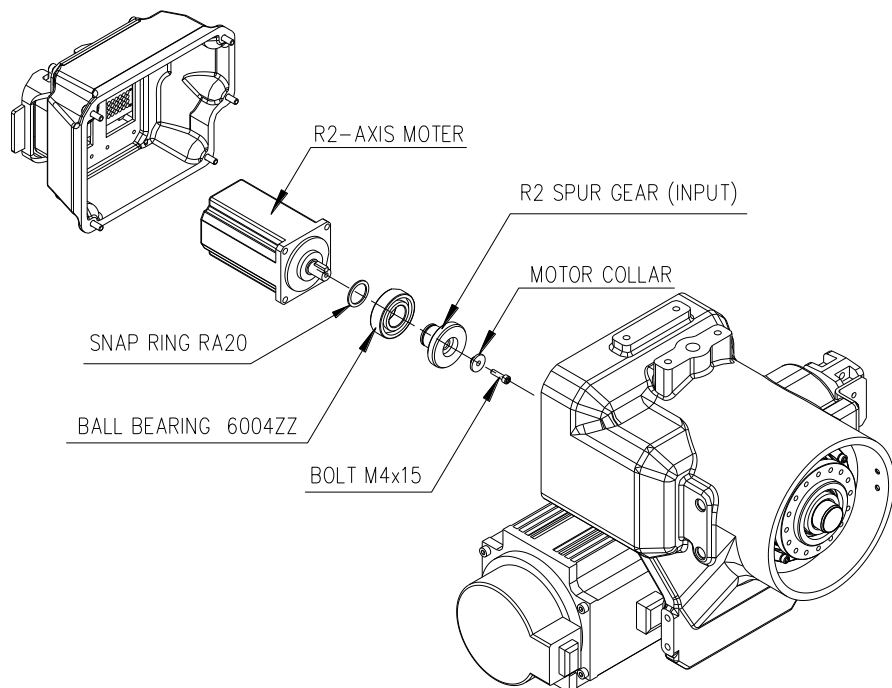
그림 6.11 R2 축 모터 교체 [HA006L]
