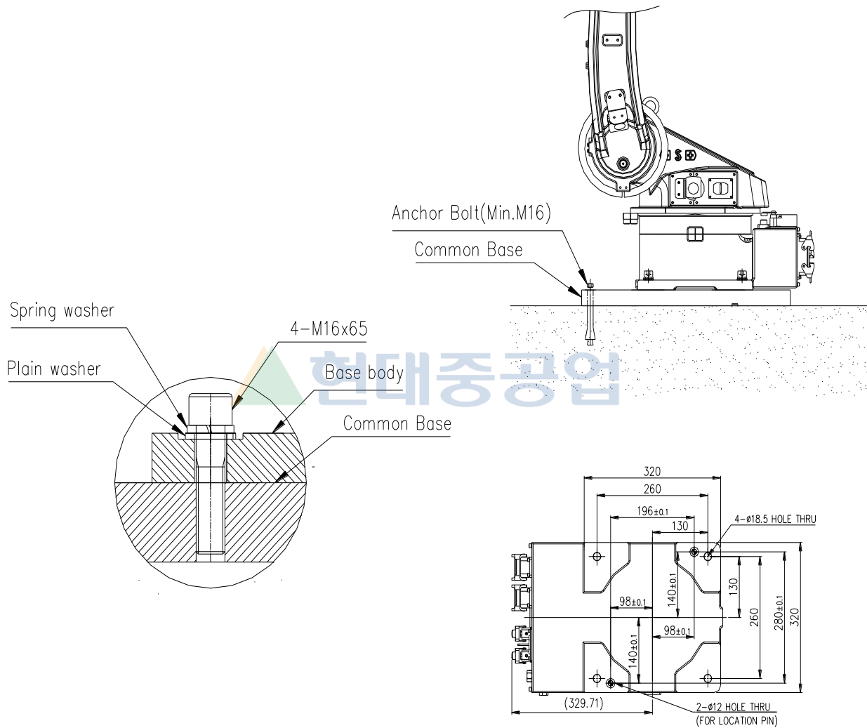
그림 3.9 로봇 설치면 치수 [HA006A]
