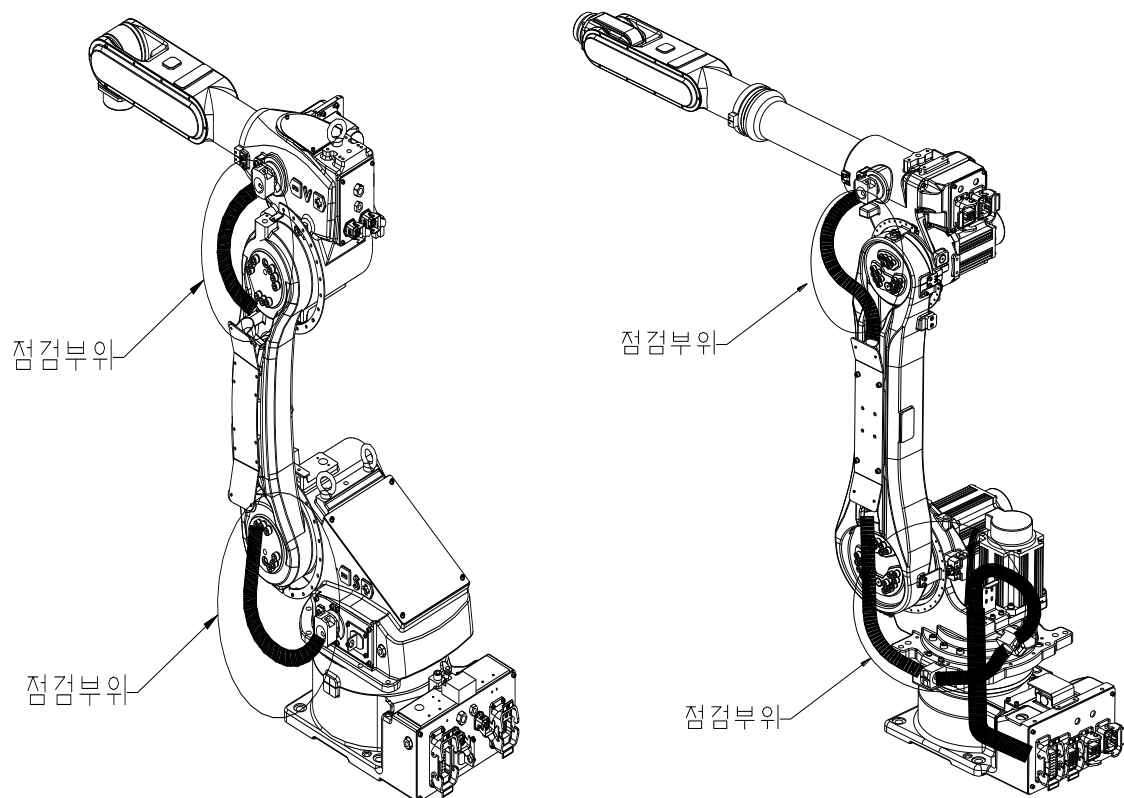
그림 4.3 케이블 점검 부위 [HA006A/HA006L]
