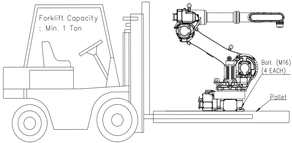
그림 3.8 운반 방법: 지게차 이용 [HA006L]
