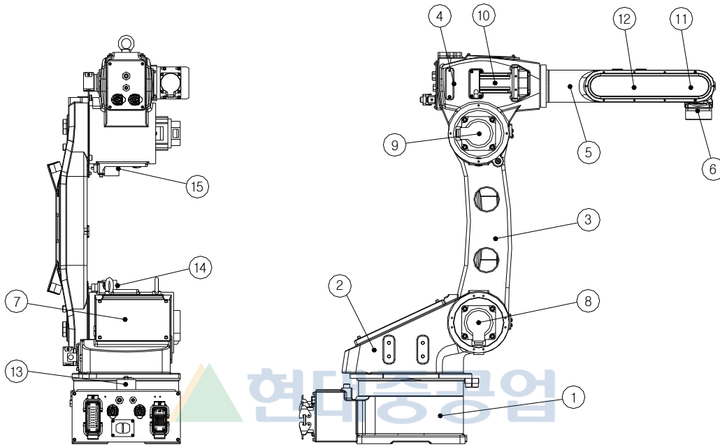
그림 3.1 본체 각 부위 명칭[HA006A]
