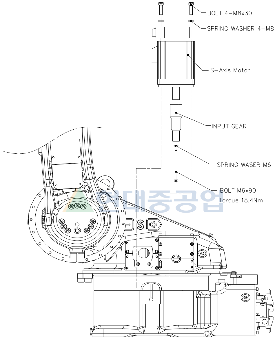
그림 6.1 S 축 모터 교체 [HA006A]
