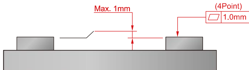
그림 3.11 로봇 설치면 정도
