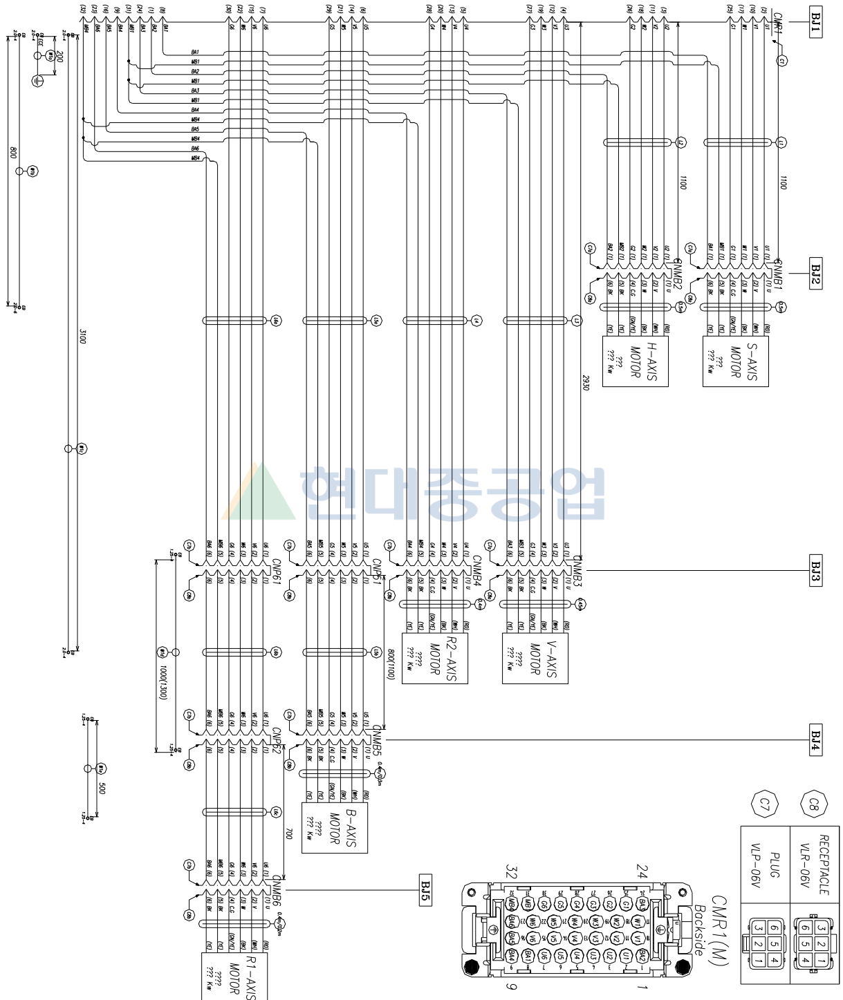
그림 8.9 MOTOR POWER CABLE [HA006L]
