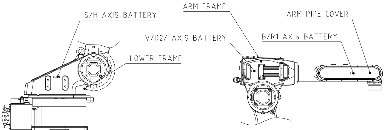
그림 5.5 배터리 교환 위치 [HA006A]
