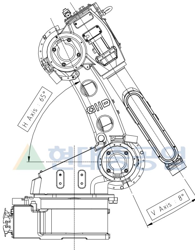
그림 6.4 V 축 모터 교체시의 로봇 자세 [HA006A]
