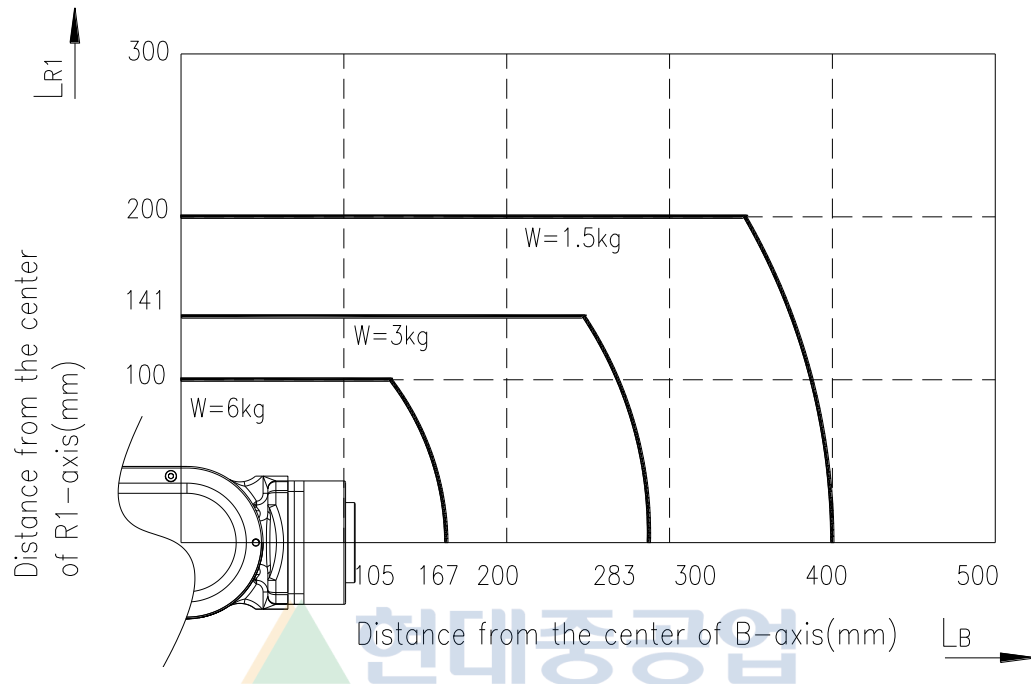
그림 3.13 손목축 토크 선도
