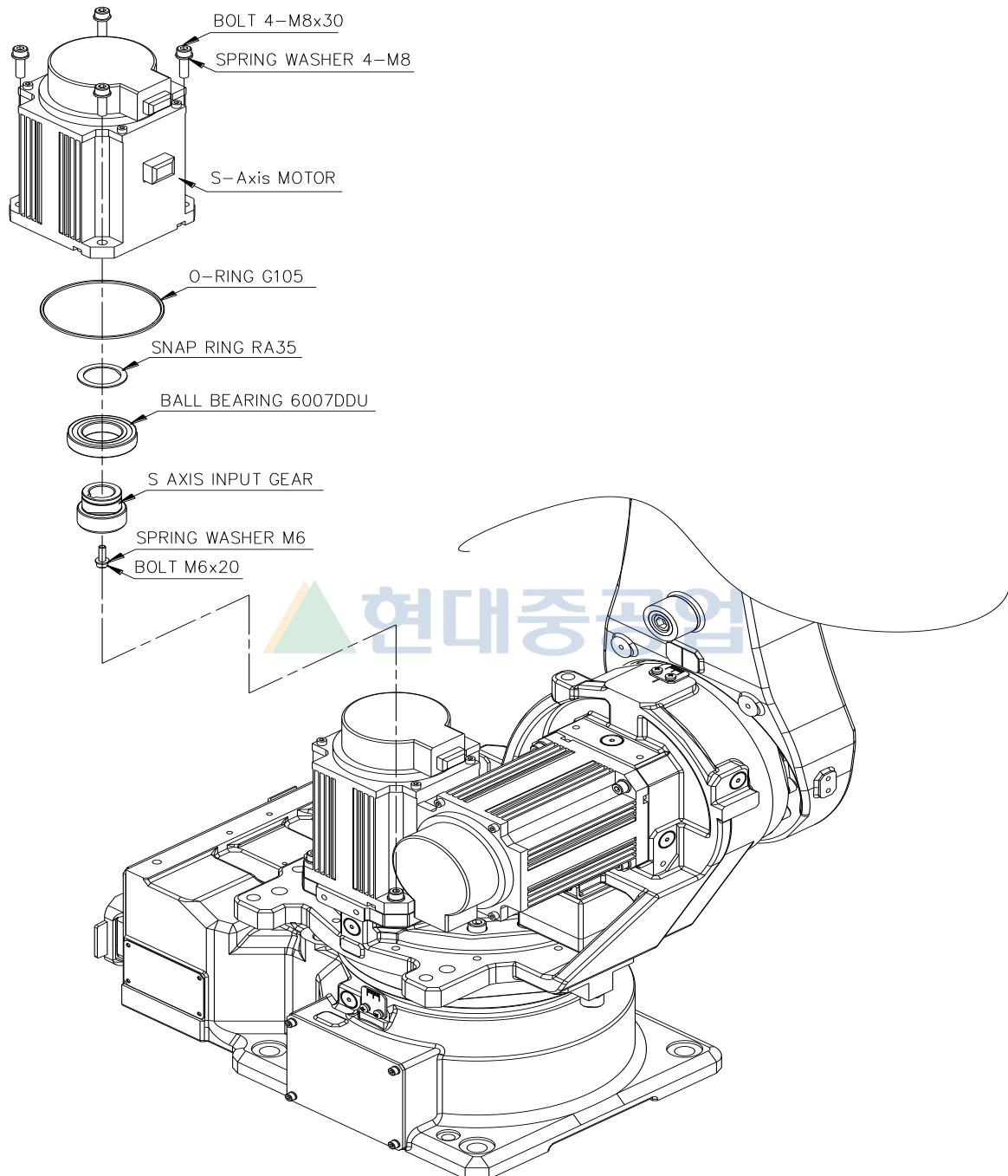
그림 6.7 S 축 모터 교체 [HA006L]
