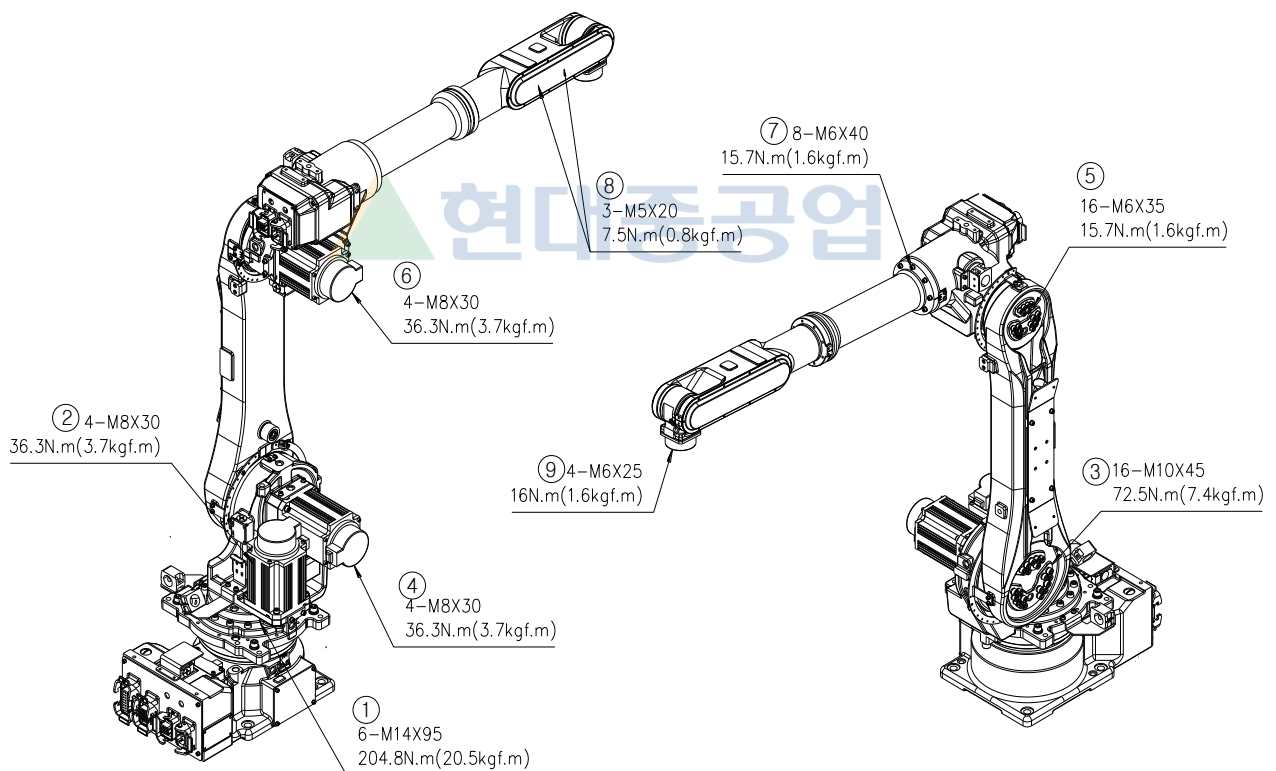
그림 4.2 주요 볼트 점검 부위 [HA006L]
