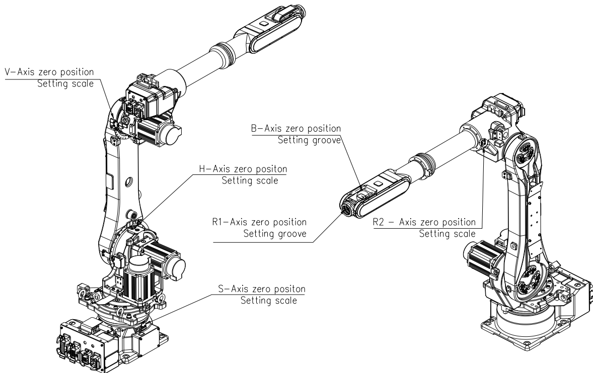
그림 6.26 원점 설정 방법 [HA006L]
