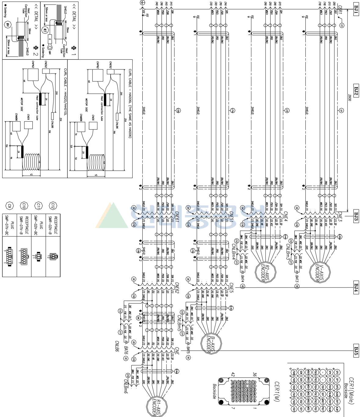
그림 8.11 ENCORDER CABLE FOR V, R2, B, R1 AXIS [HA006L]
