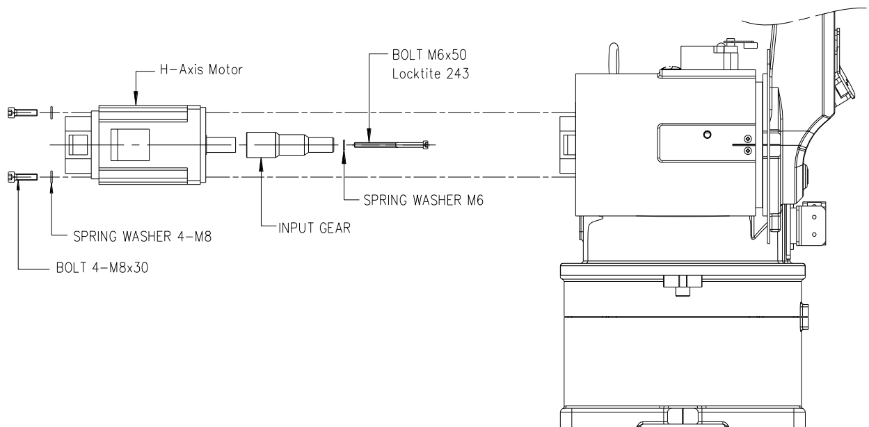
그림 6.3 H축 모터 교체 [HA006A]
