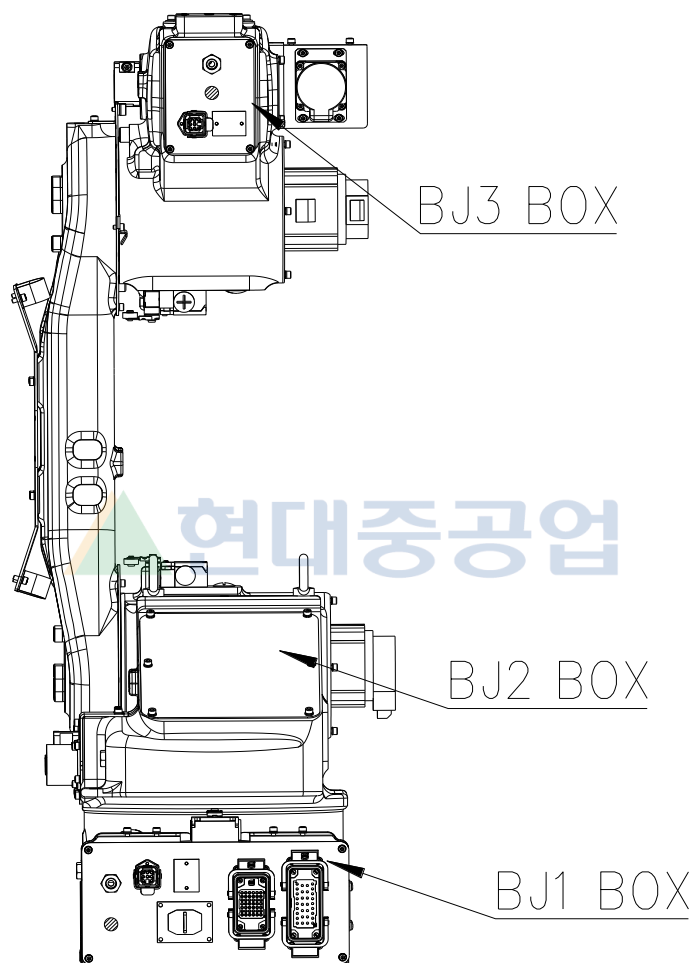
그림 8.1 본체 부품 배치 [HA006A]
