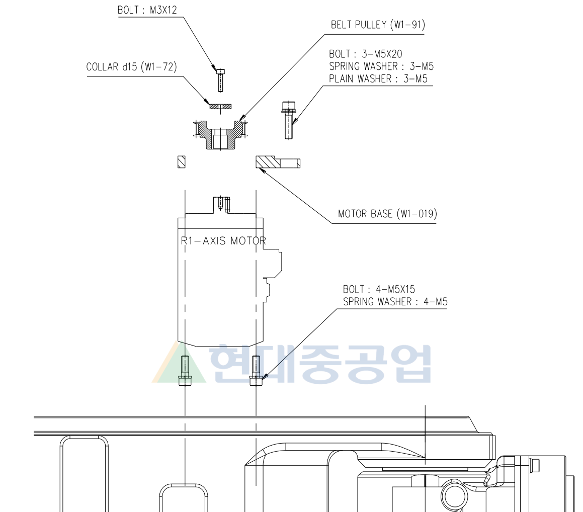
그림 6.12 B/R1 축 모터교체 (HA006A/HA006L)
