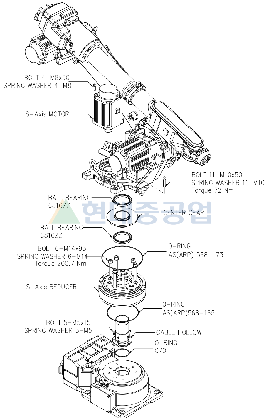
그림 6.20 S 축 감속기 분해도 [HA006L]
