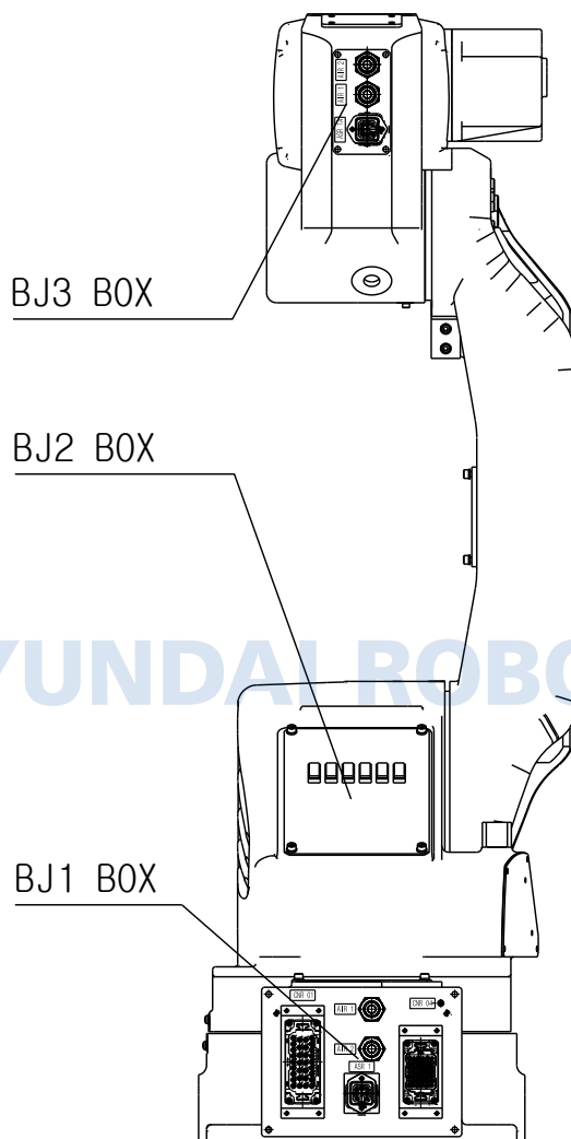
그림 8.1 본체 부품 배치
