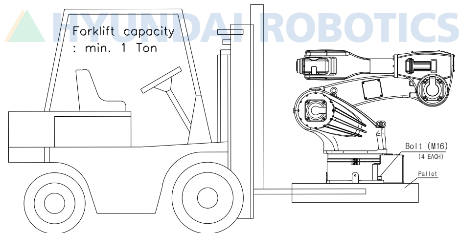
그림 3.6 운반 방법 : 지게차 이용 [HA020/HA010L]
