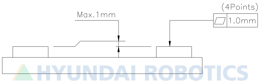
그림 3.9 로봇 설치면 정도
