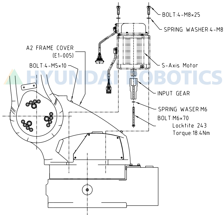
그림 6.1 S 축 모터/감속기 분해도
