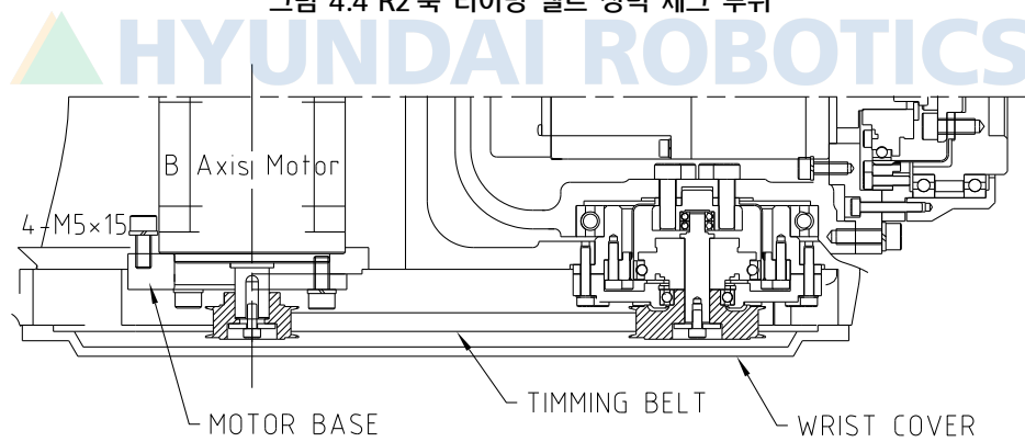
그림 4.5 B 축 타이밍 벨트 장력 체크 부위
