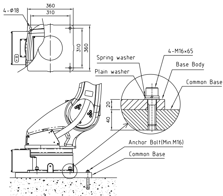
그림 3.8 로봇 설치면 치수 [HA020]
