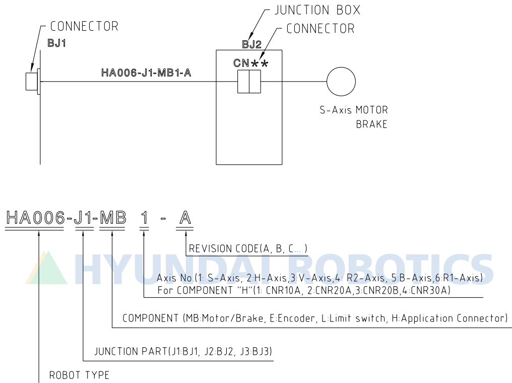
그림 5.2 본체 내 배선기호 설명
