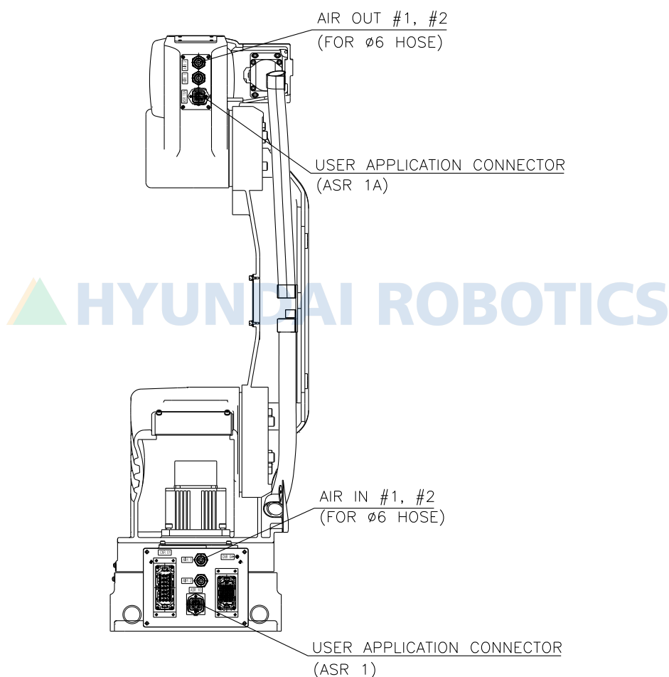
그림 2.11 어플리케이션용 배선 및 배관도 : [HA006]
