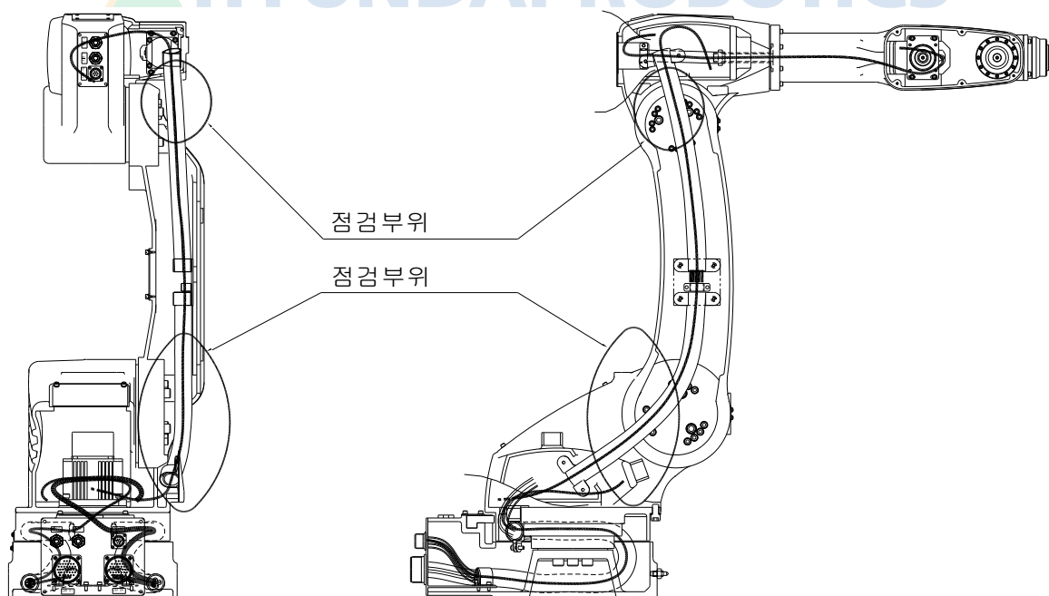
그림 4.3 케이블 점검 부위
