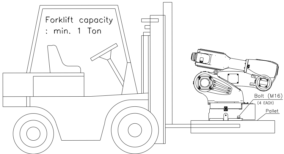
그림 3.5 운반 방법 : 지게차 이용 [HA006]
