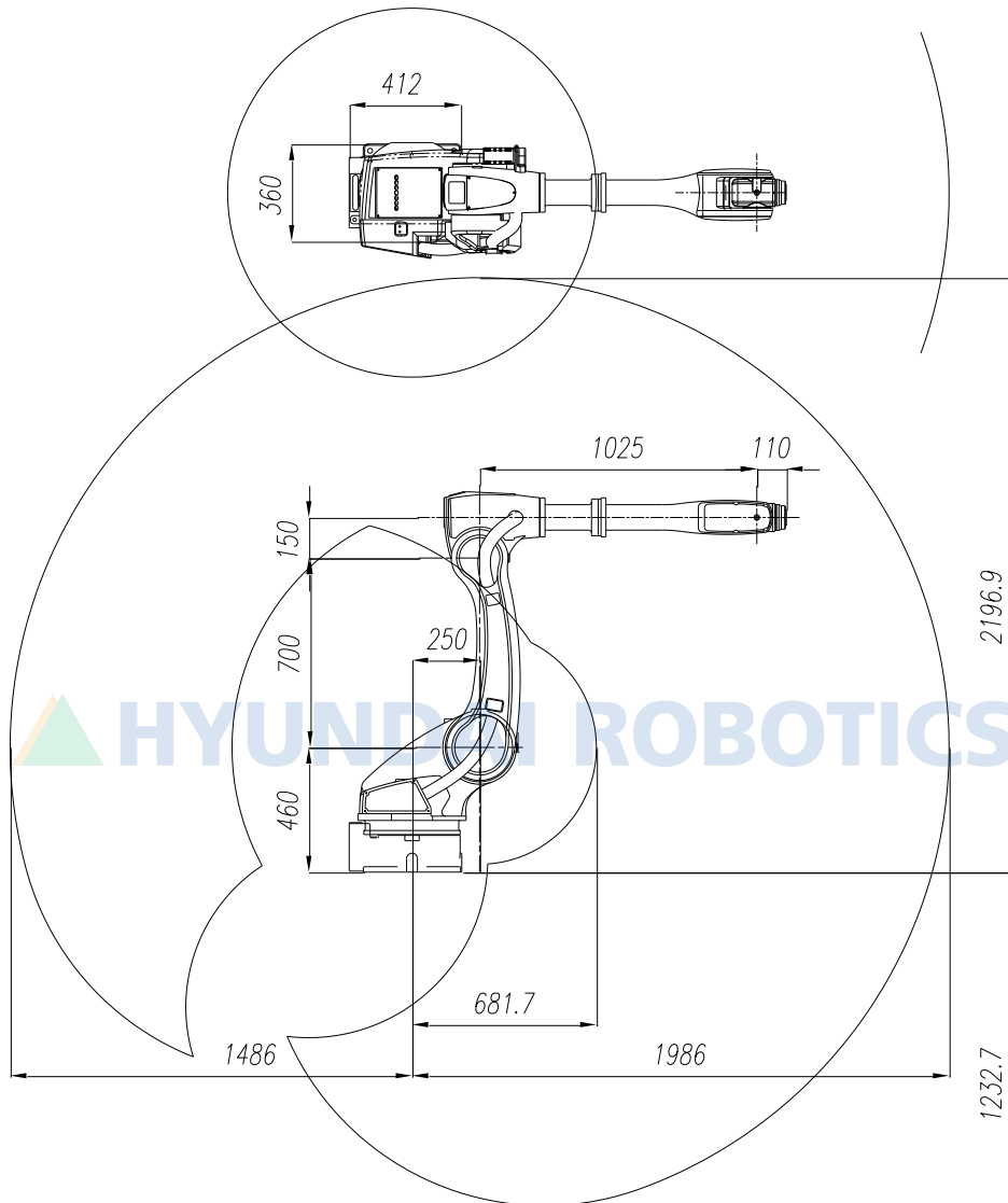
그림 2.5 본체 외형 치수 및 동작 영역 : [HA010L]
