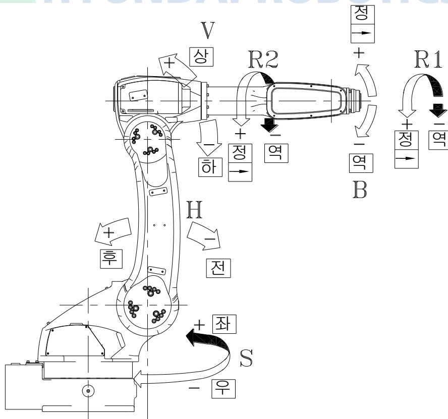
그림 2.6 본체 외관 및 동작 축
