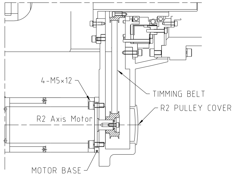
그림 4.4 R2 축 타이밍 벨트 장력 체크 부위
