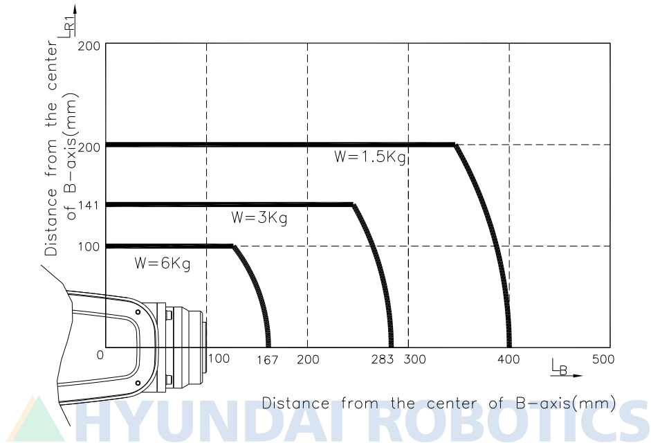
그림 3.10 손목 축 토크 선도 [HA006]
