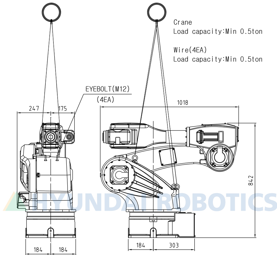
그림 3.4 운반 방법 : 크레인 이용 [HA020/HA010L]
