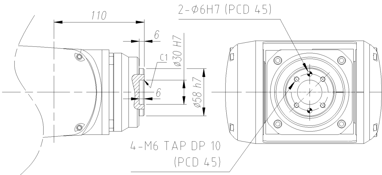
그림 2.8 손목 축 취부면 상세도 : [HA020]
