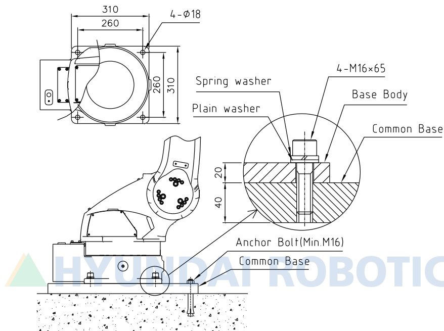
그림 3.7 로봇 설치면 치수 [HA006]
