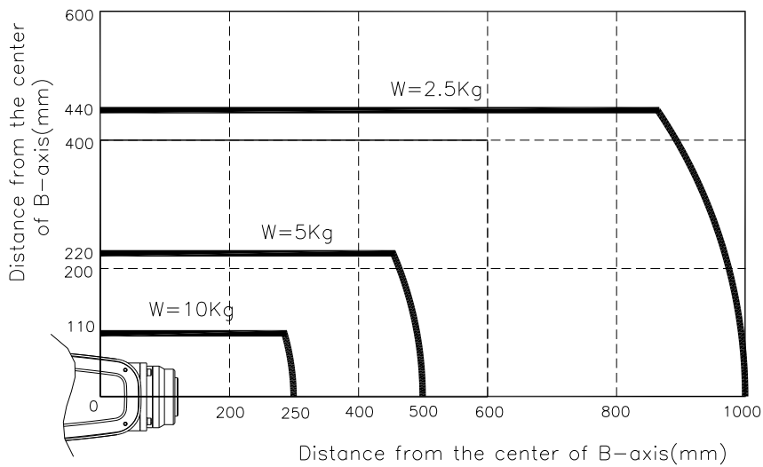
그림 3.12 손목축 토크 선도 [HA010L]
