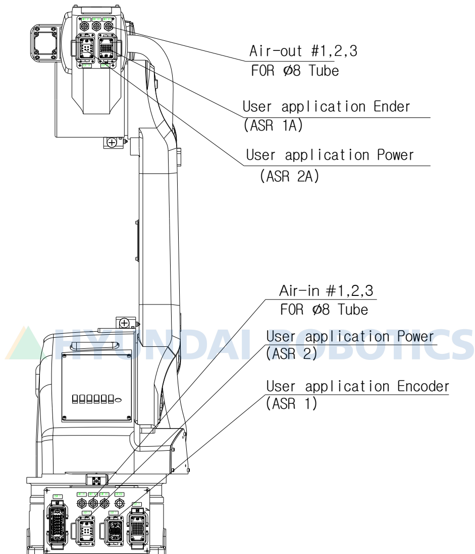
그림 2.13 어플리케이션용 배선 및 배관도 : [HA020/HA010L]
