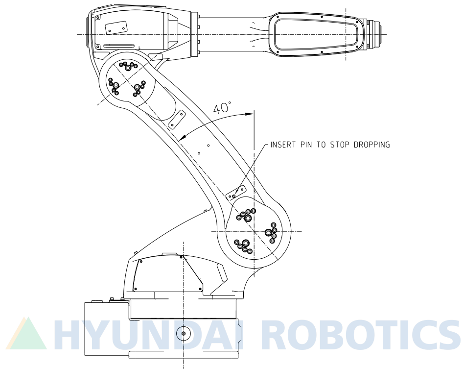
그림 6.2 H축 모터 교체시의 로봇 자세
