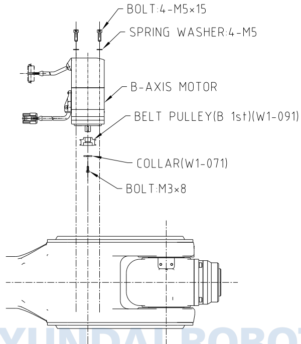
그림 6.6 B 축 모터
