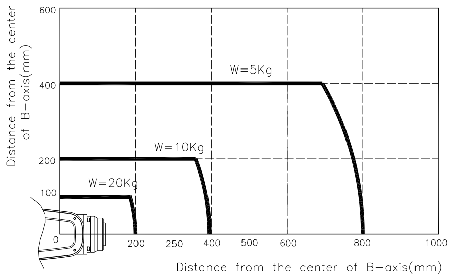
그림 3.11 손목축 토크 선도 [HA020]
