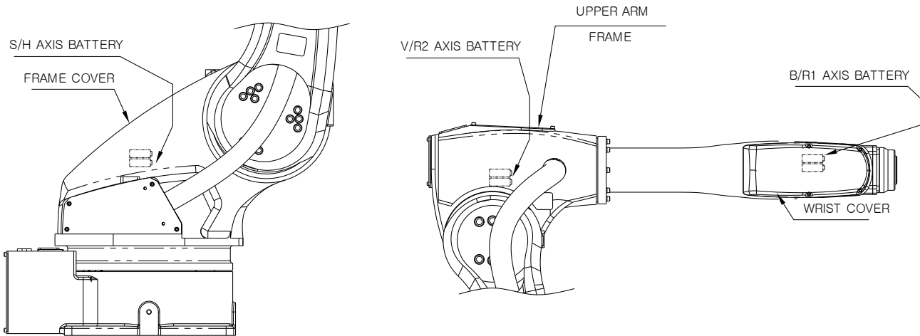
그림 5.1 배터리 교환 위치
