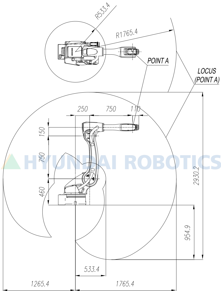
그림 2.4 본체 외형 치수 및 동작 영역 : [HA020]
