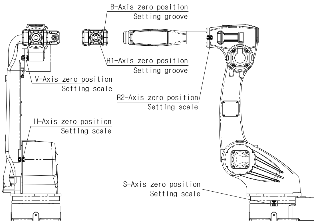
그림 6.9 원점 설정 방법 [HA020]
