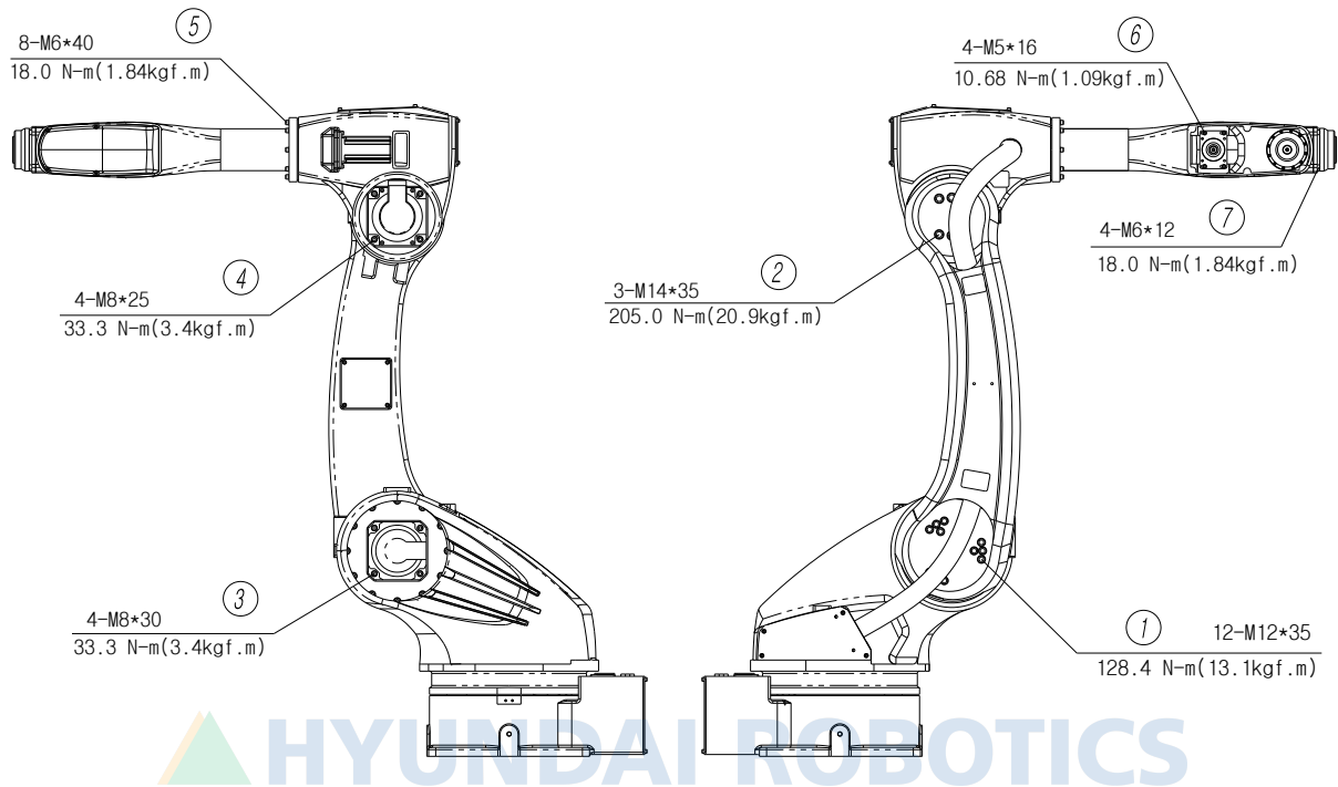
그림 4.2 주요 볼트 점검 부위 [HA020/HA010L]
