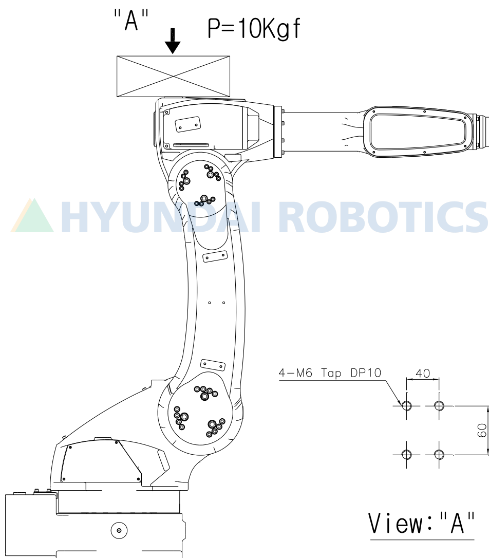
그림 2.9 제 1ARM 상부 부착부 상세도 : [HA006]
