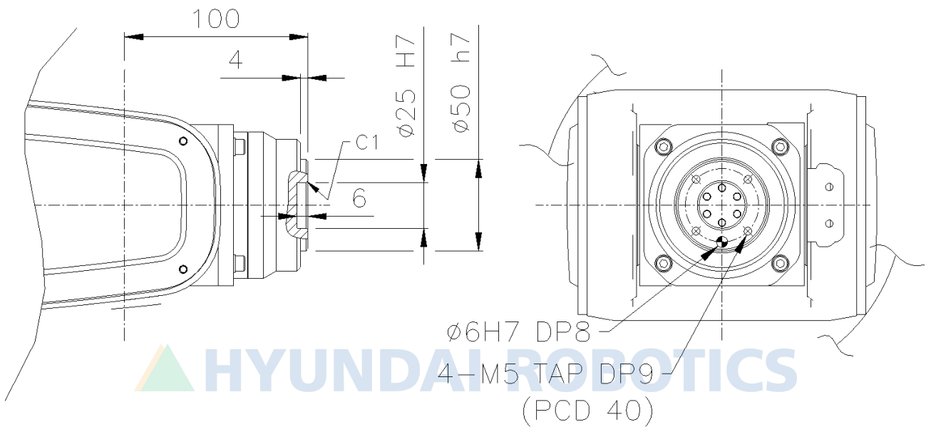
그림 2.7 손목 축 취부면 상세도 : [HA006]
