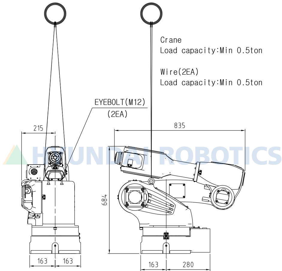
그림 3.3 운반 방법 : 크레인 이용 [HA006]
