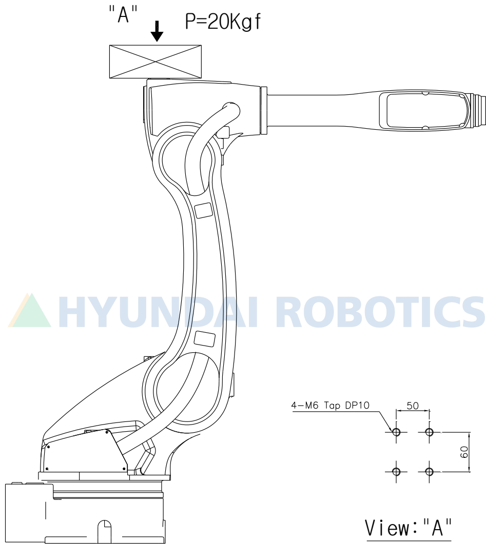
그림 2.10 제1ARM 상부 부착부 상세도 : [HA020/HA010L]
