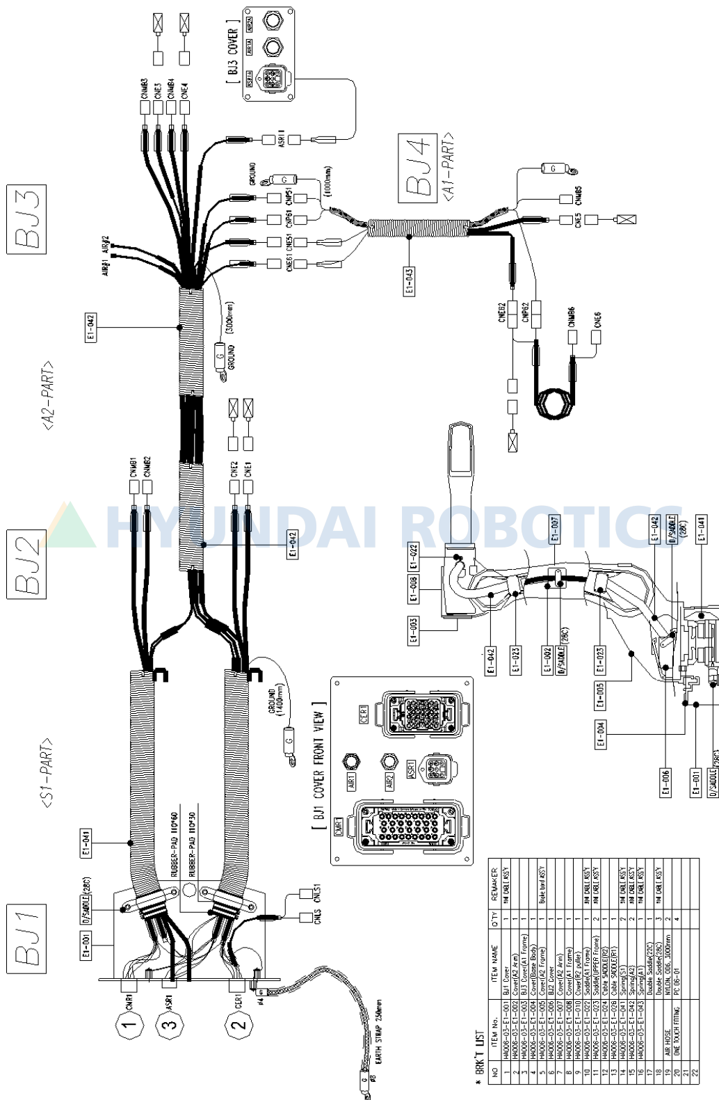
그림 8.3 CABLE ASSEMBLY [HA006]
