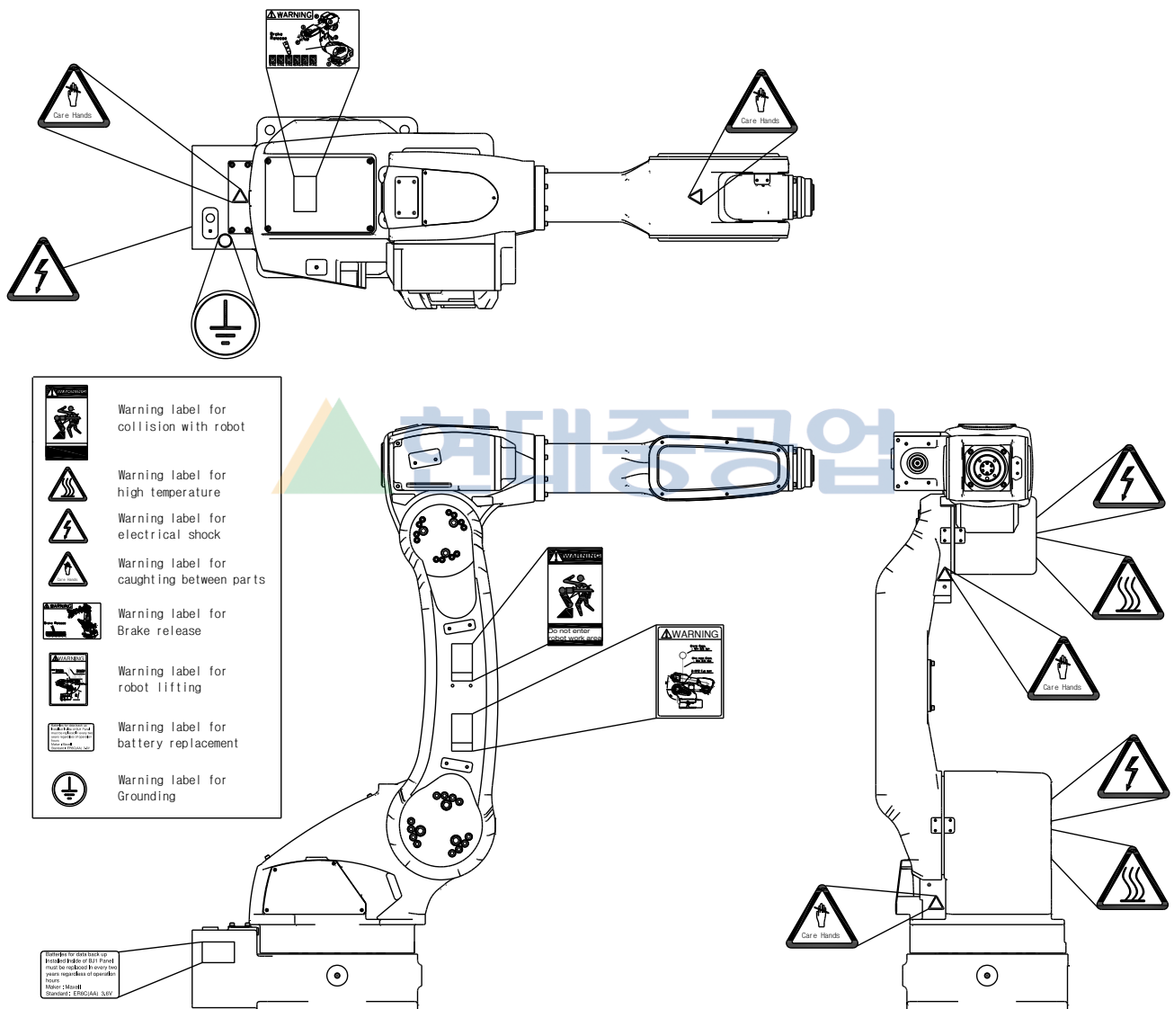
그림 3.2 안전 명판 위치
