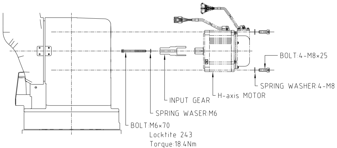
그림 6.3 H축 모터 교체
