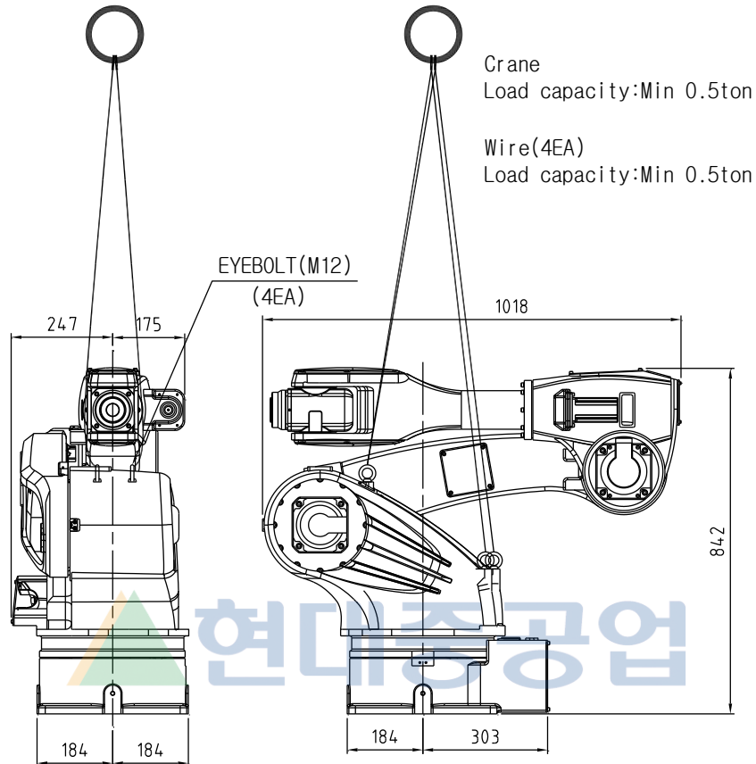
그림 3.4 운반 방법 : 크레인 이용 [HA020W]
