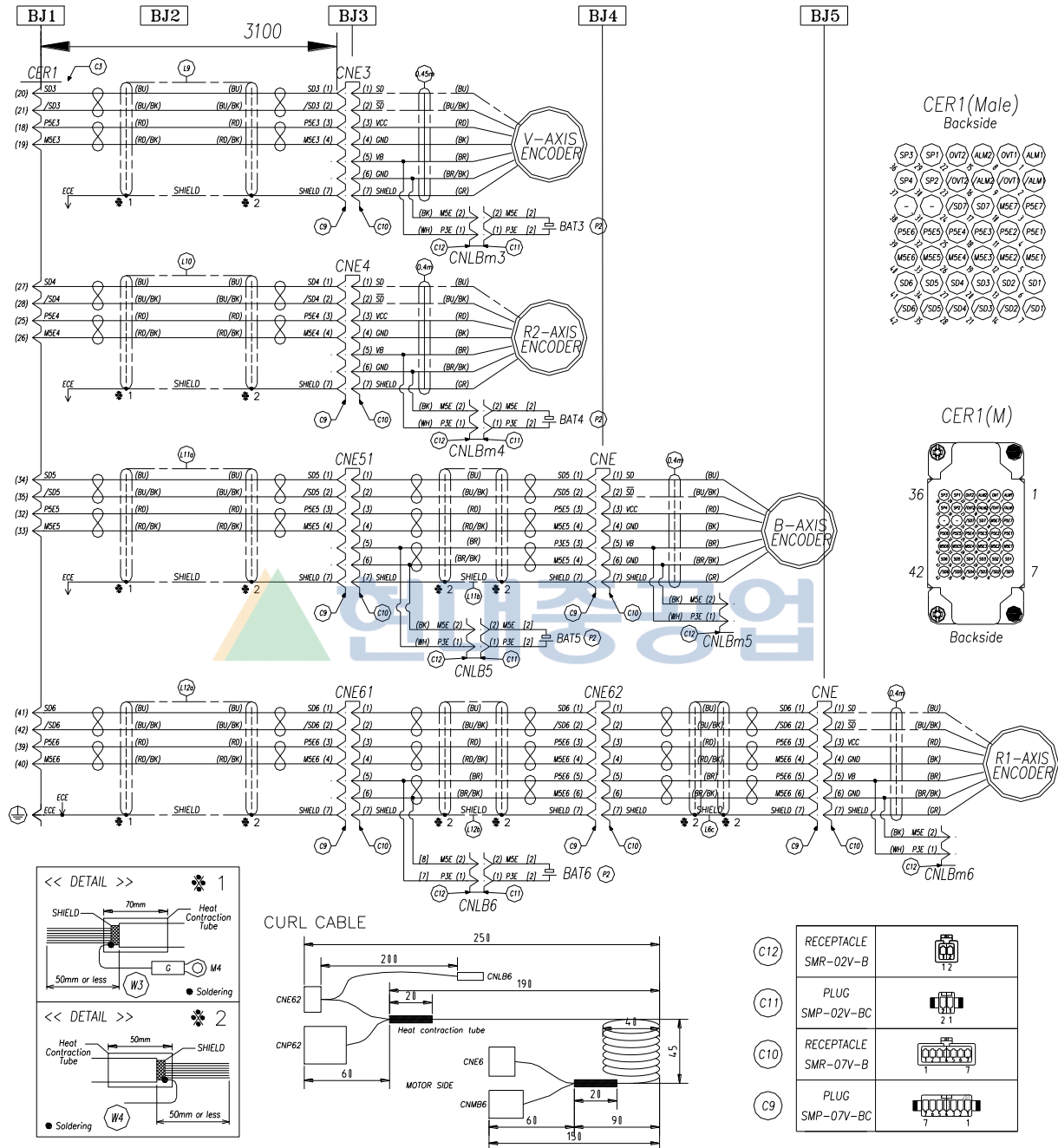
그림 8.12 ENCODER CABLE FOR V,R2,B,R1 AXIS [HA020W/HA010LW]
