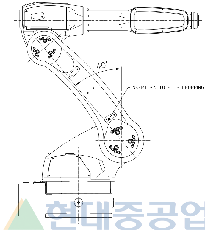
그림 6.2 H축 모터 교체시의 로봇 자세
