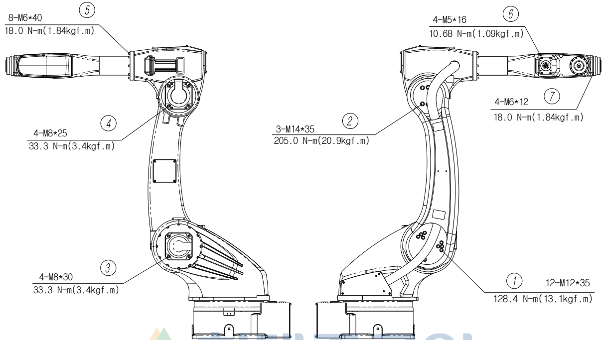
그림 4.2 주요 볼트 점검 부위 [HA020W/HA010LW]
