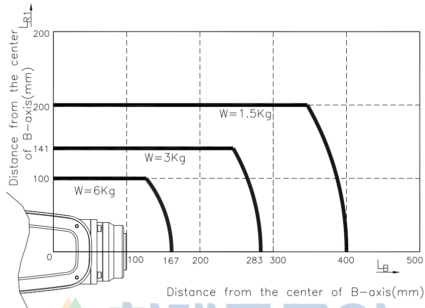
그림 3.10 손목 축 토크 선도 [HA006]
