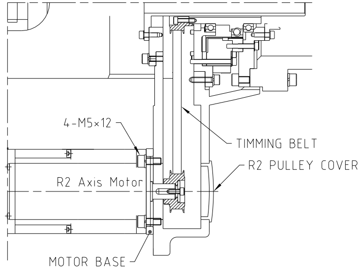
그림 4.4 R2 축 타이밍 벨트 장력 체크 부위
