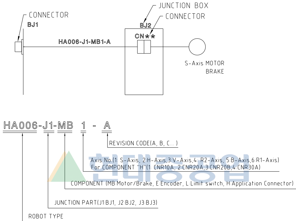
그림 5.3 본체 내 배선기호 설명
