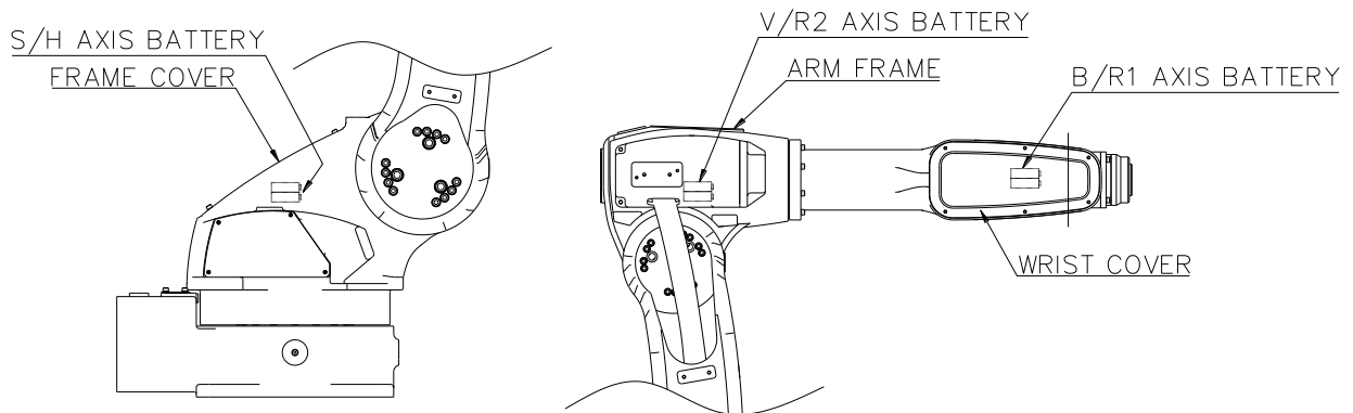
그림 5.1 배터리 교환 위치 [HA006]
