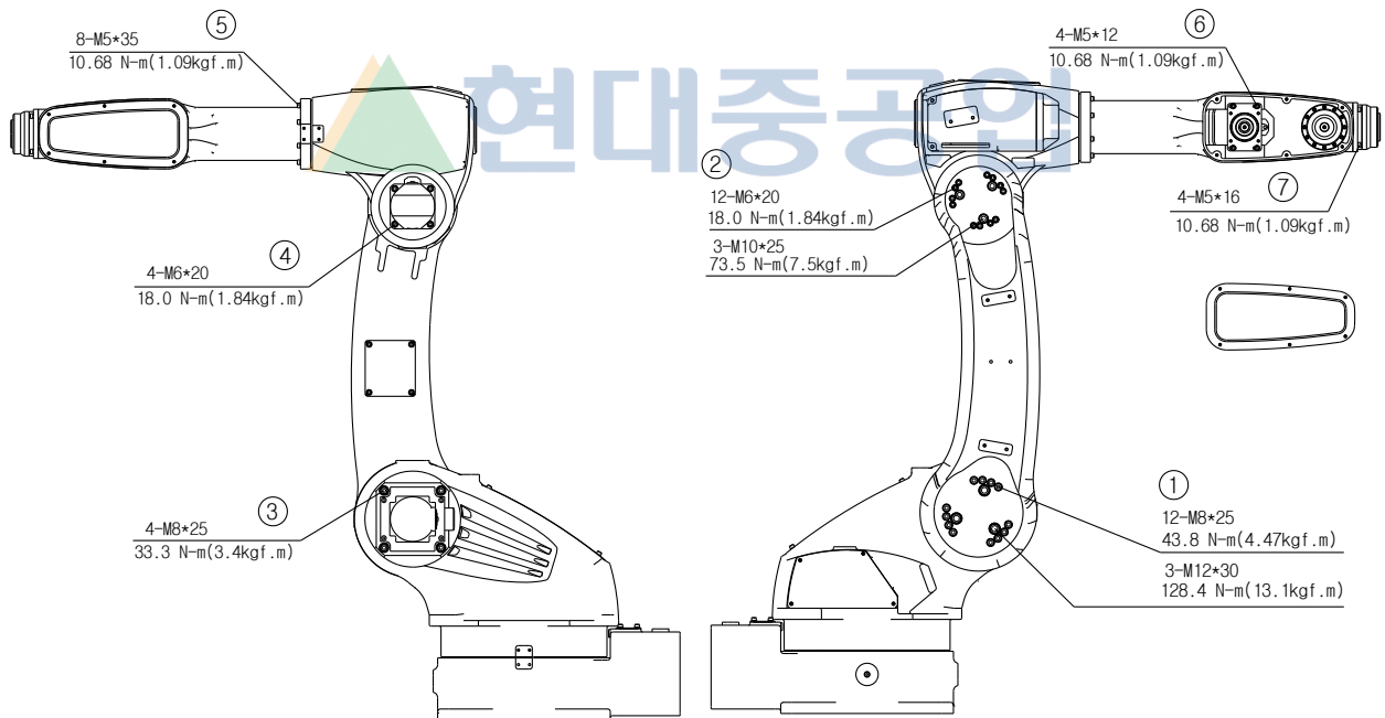
그림 4.1 주요 볼트 점검 부위 [HA006]
