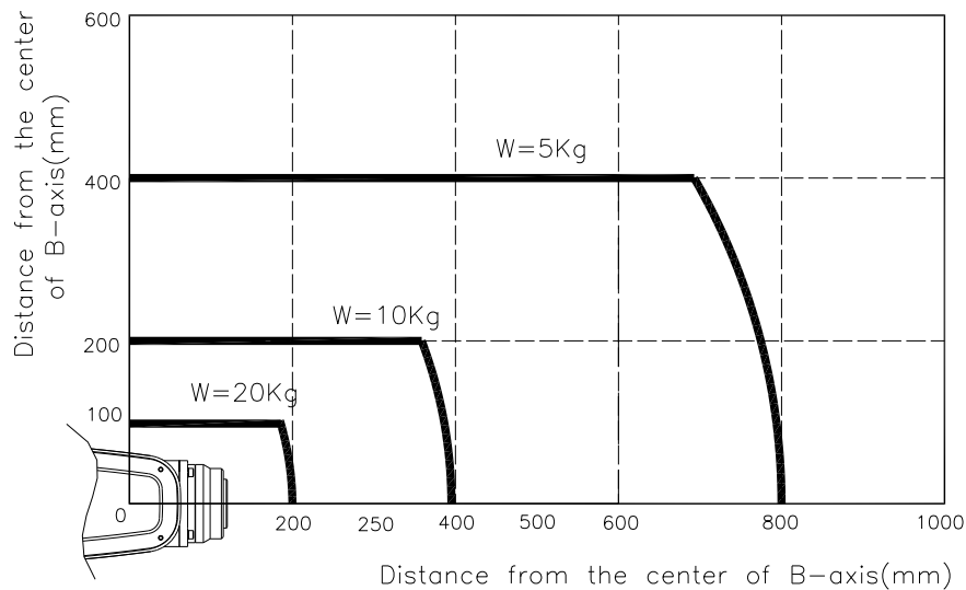
그림 3.11 손목축 토크 선도 [HA020W]
