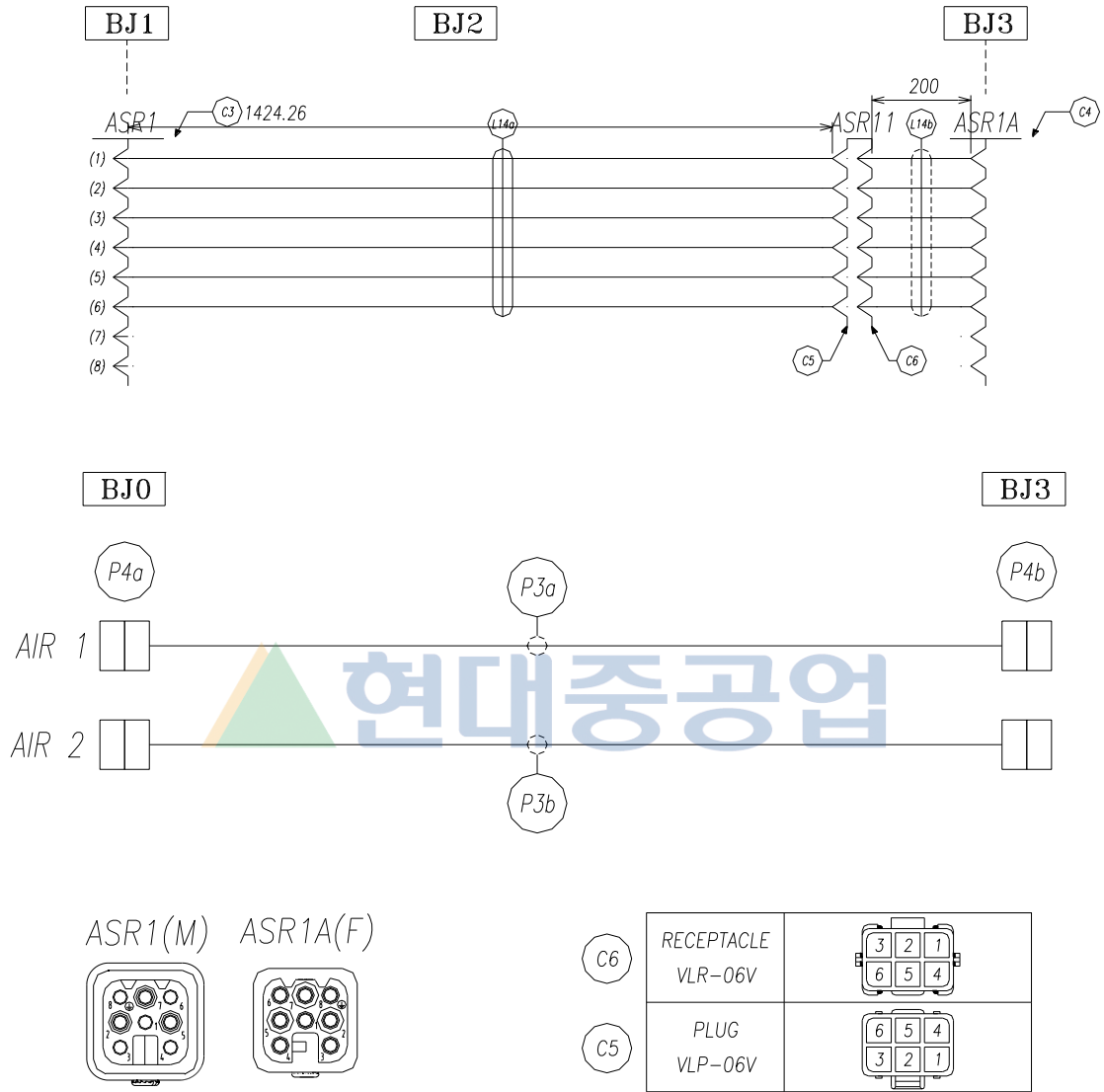
그림 8.7 APPLICATION CABLE & AIR TUBE [HA006]
