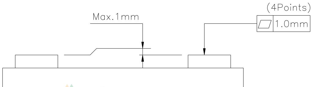
그림 3.9 로봇 설치면 정도
