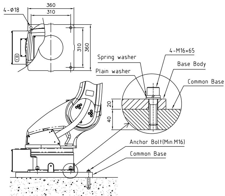
그림 3.8 로봇 설치면 치수 [HA020W]
