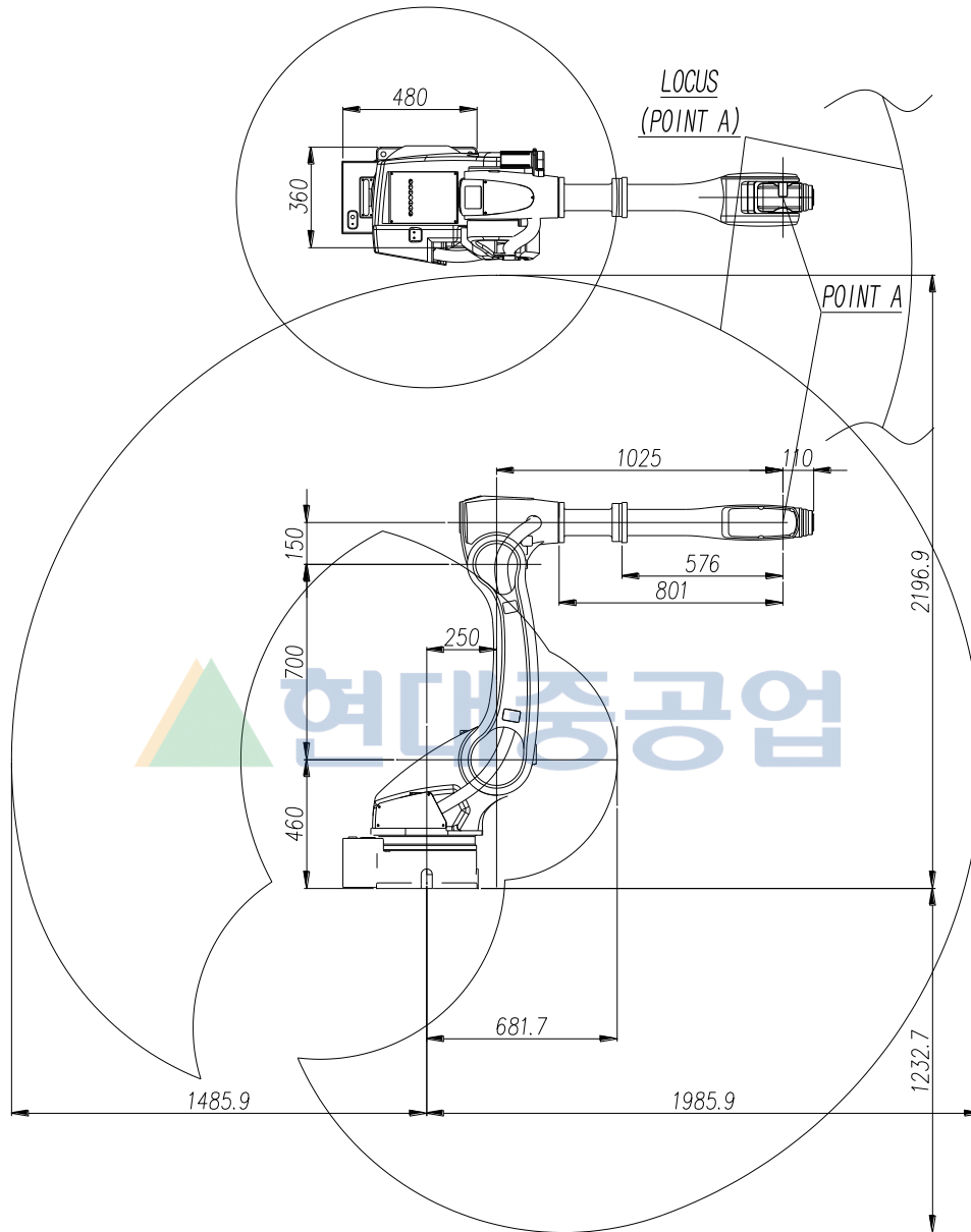
그림 2.5 본체 외형 치수 및 동작 영역 : [HA010LW]
