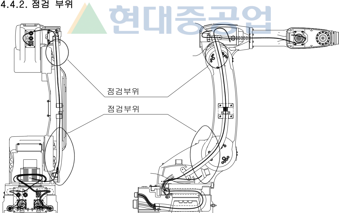
그림 4.3 케이블 점검 부위
