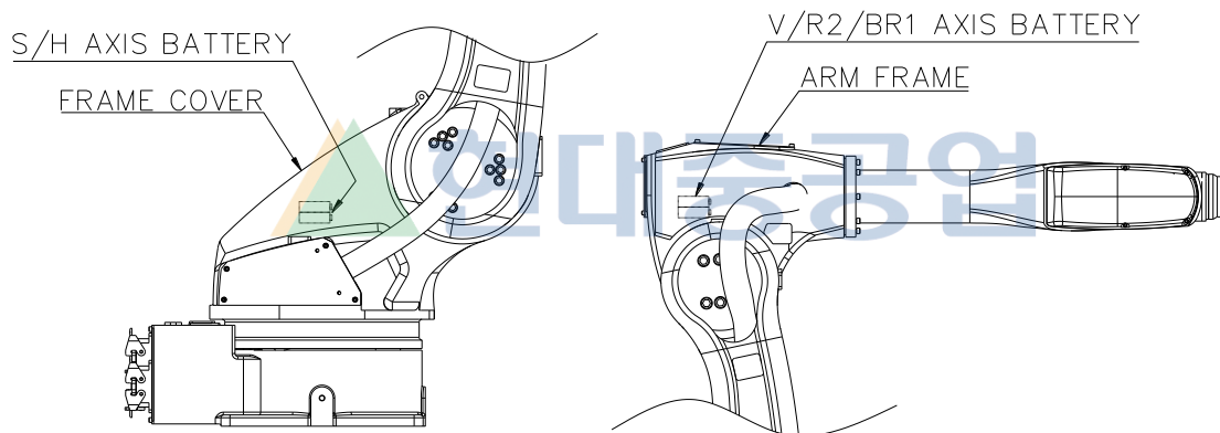
그림 5.2 배터리 교환 위치 [HA020W/HA010LW]
