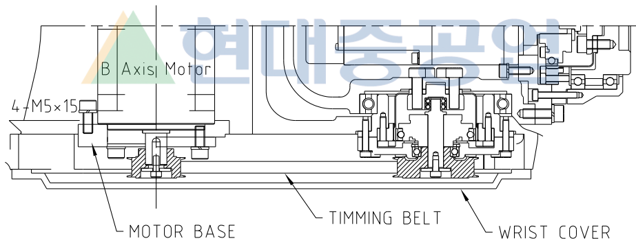
그림 4.5 B 축 타이밍 벨트 장력 체크 부위
