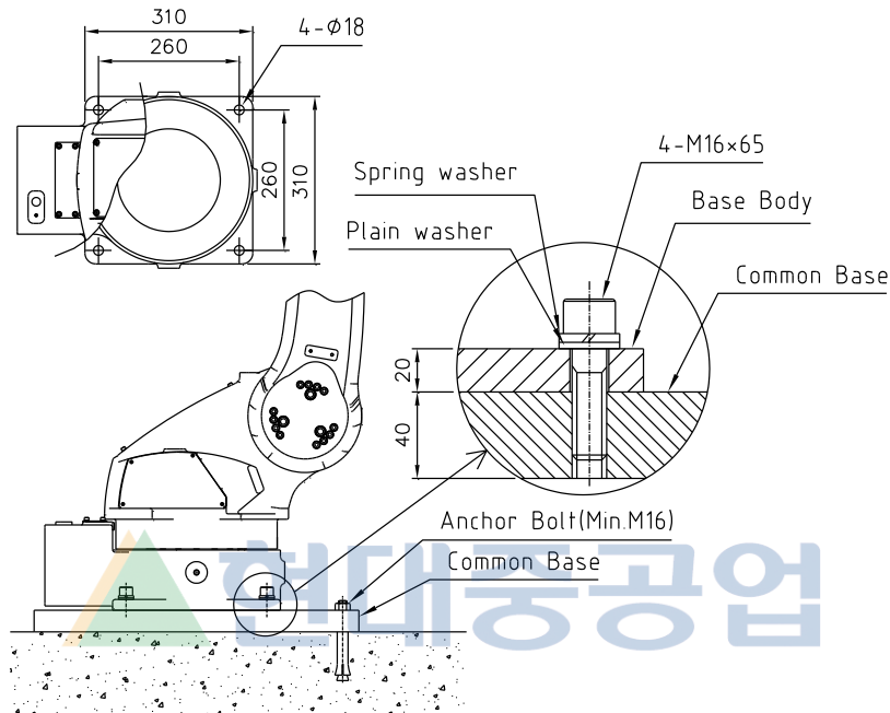
그림 3.7 로봇 설치면 치수 [HA006]
