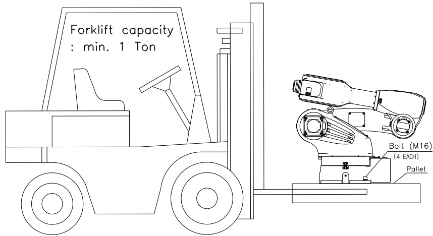
그림 3.5 운반 방법 : 지게차 이용 [HA006]
