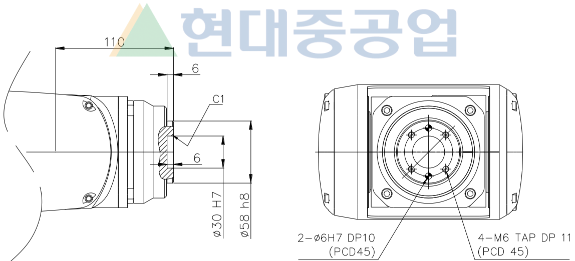
그림 2.8 손목 축 취부면 상세도 : [HA020W/HA010LW]
