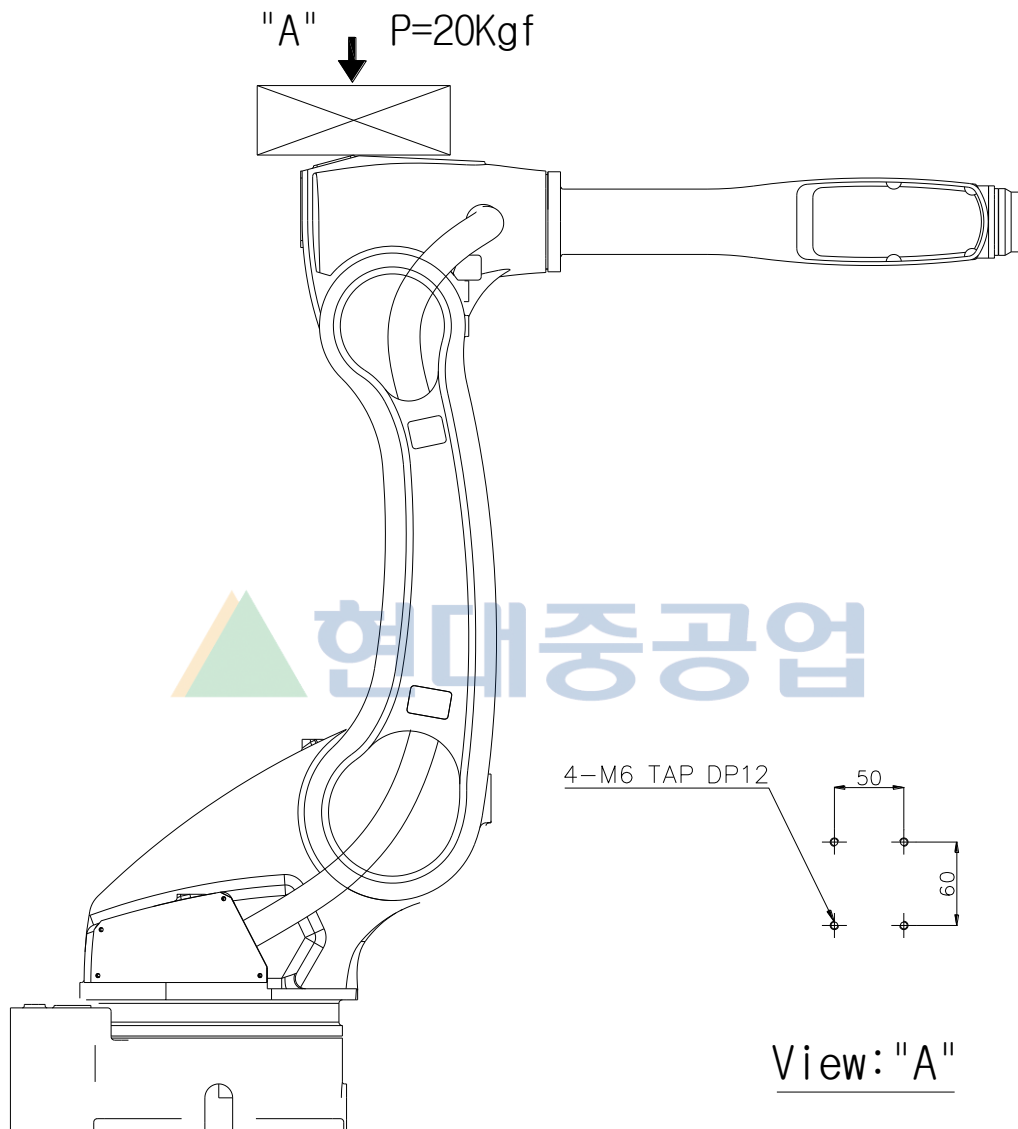
그림 2.10 제 1ARM 상부 부착부 상세도 : [HA020W/HA010LW]
