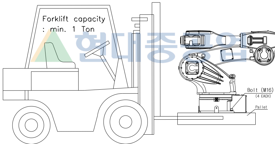
그림 3.6 운반 방법 : 지게차 이용 [HA020W/HA010LW]
