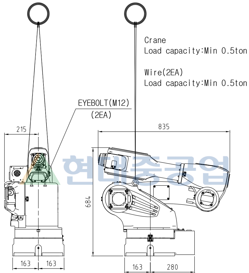
그림 3.3 운반 방법 : 크레인 이용 [HA006]
