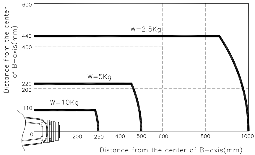
그림 3.12 손목축 토크 선도 [HA010LW]
