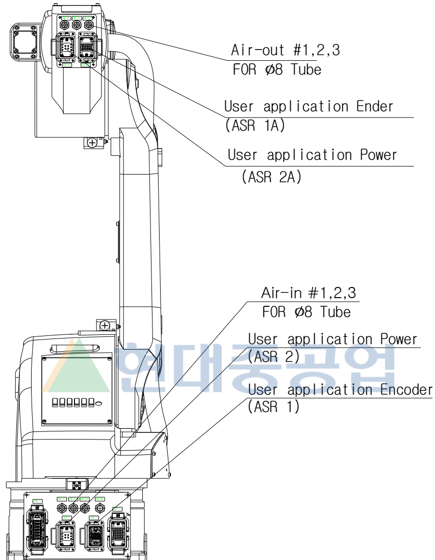
그림 2.13 어플리케이션용 배선 및 배관도 : [HA020W/HA010LW]
