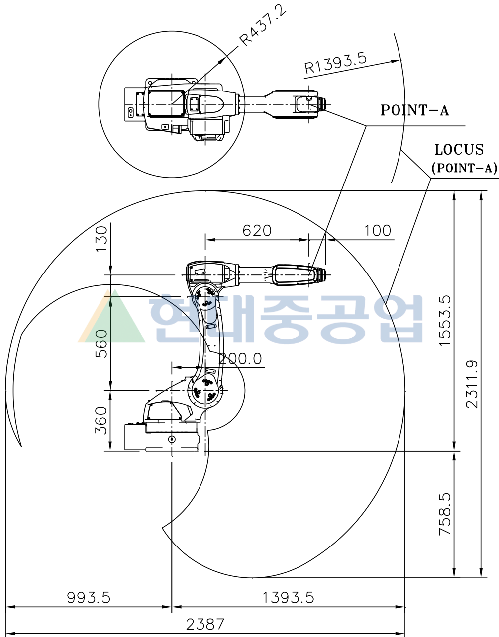
그림 2.3 로봇 본체 외형 치수 및 동작 영역 : [HA006]
