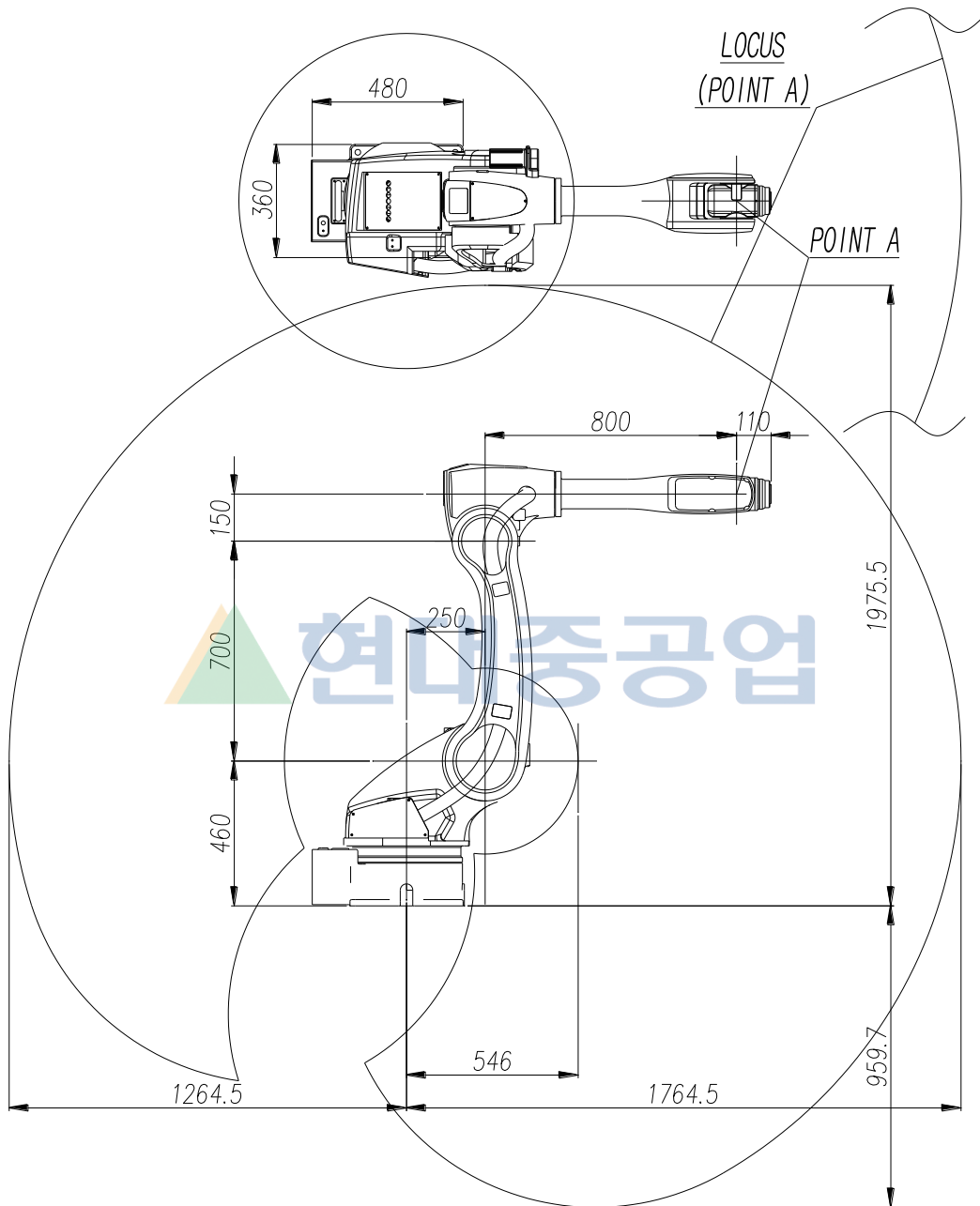
그림 2.4 본체 외형 치수 및 동작 영역 : [HA020W]
