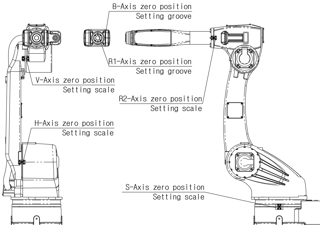
그림 6.9 원점 설정 방법 [HA020W]
