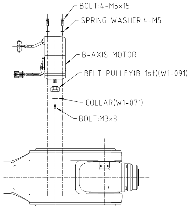
그림 6.6 B 축 모터
