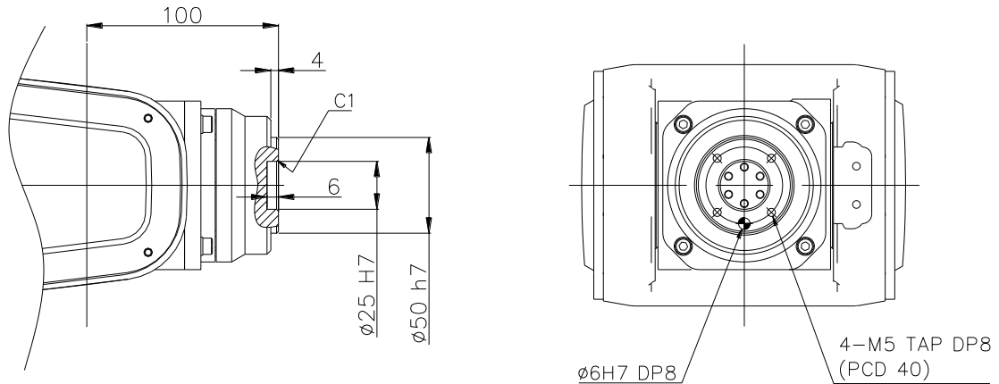
그림 2.7 손목 축 취부면 상세도 : [HA006]
