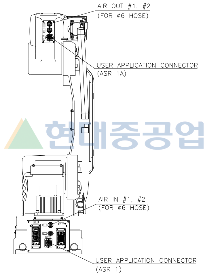
그림 2.11 어플리케이션용 배선 및 배관도 : [HA006]
