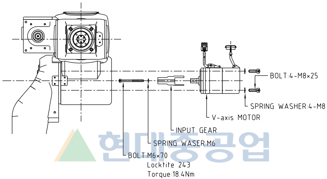
그림 6.4 V 축 모터
