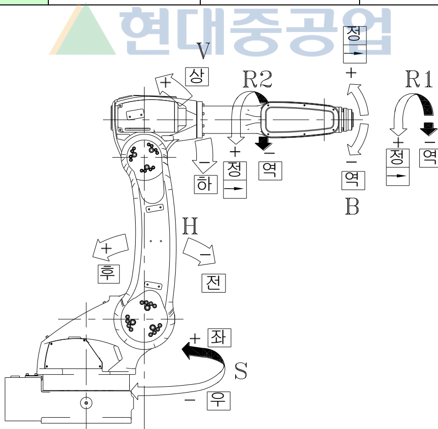
그림 2.6 본체 외관 및 동작 축
