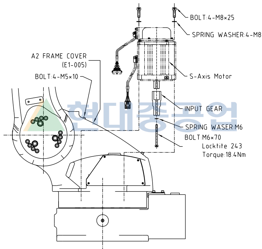
그림 6.1 S 축 모터/감속기 분해도
