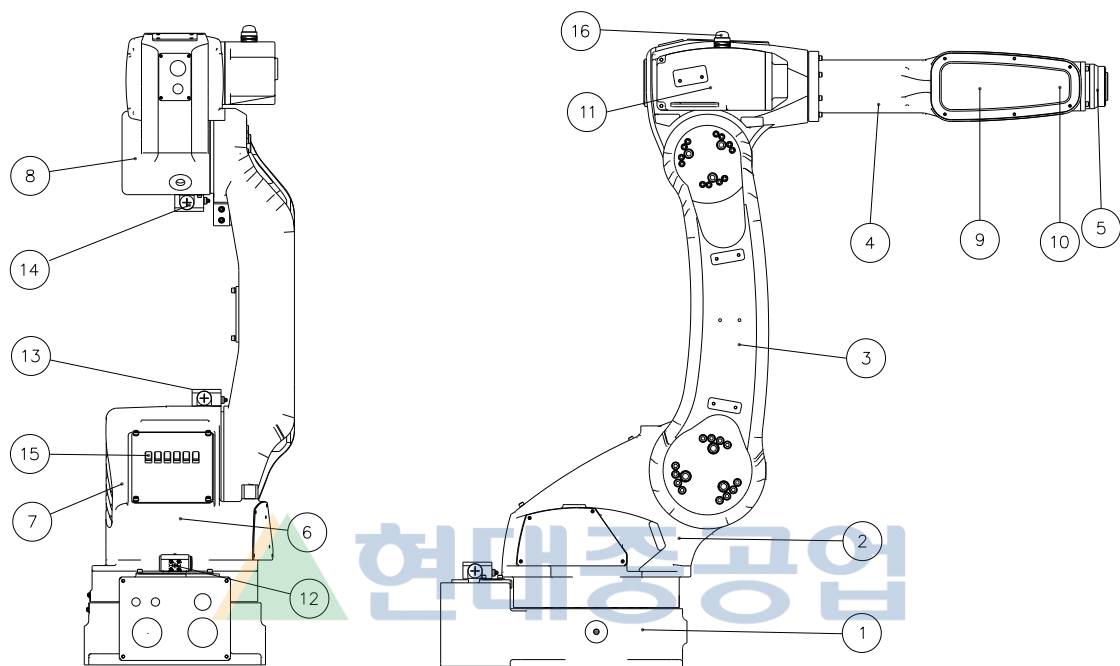
그림 3.1 본체 각 부위 명칭
