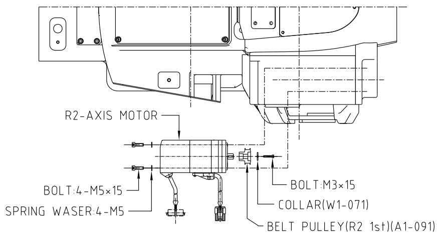
그림 6.5 R2 축 모터
