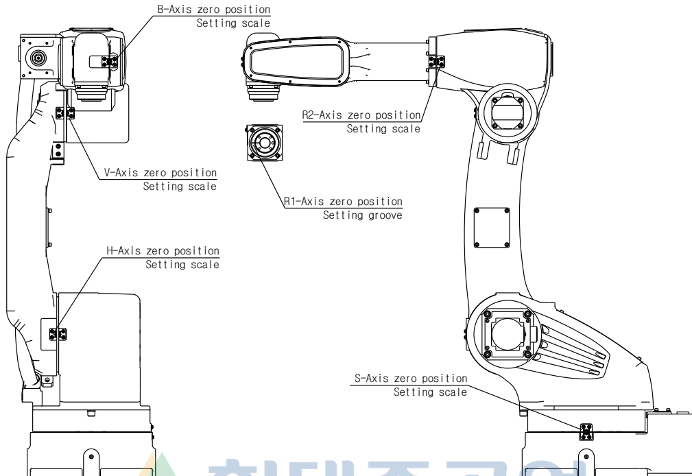
그림 6.8 원점 설정 방법 [HA006]
