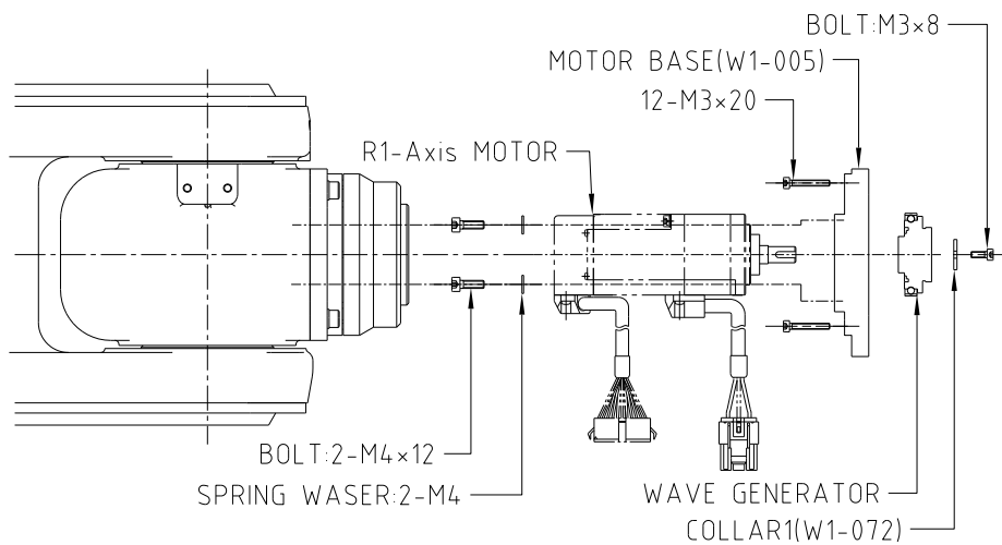
그림 6.7 R1 축 모터
