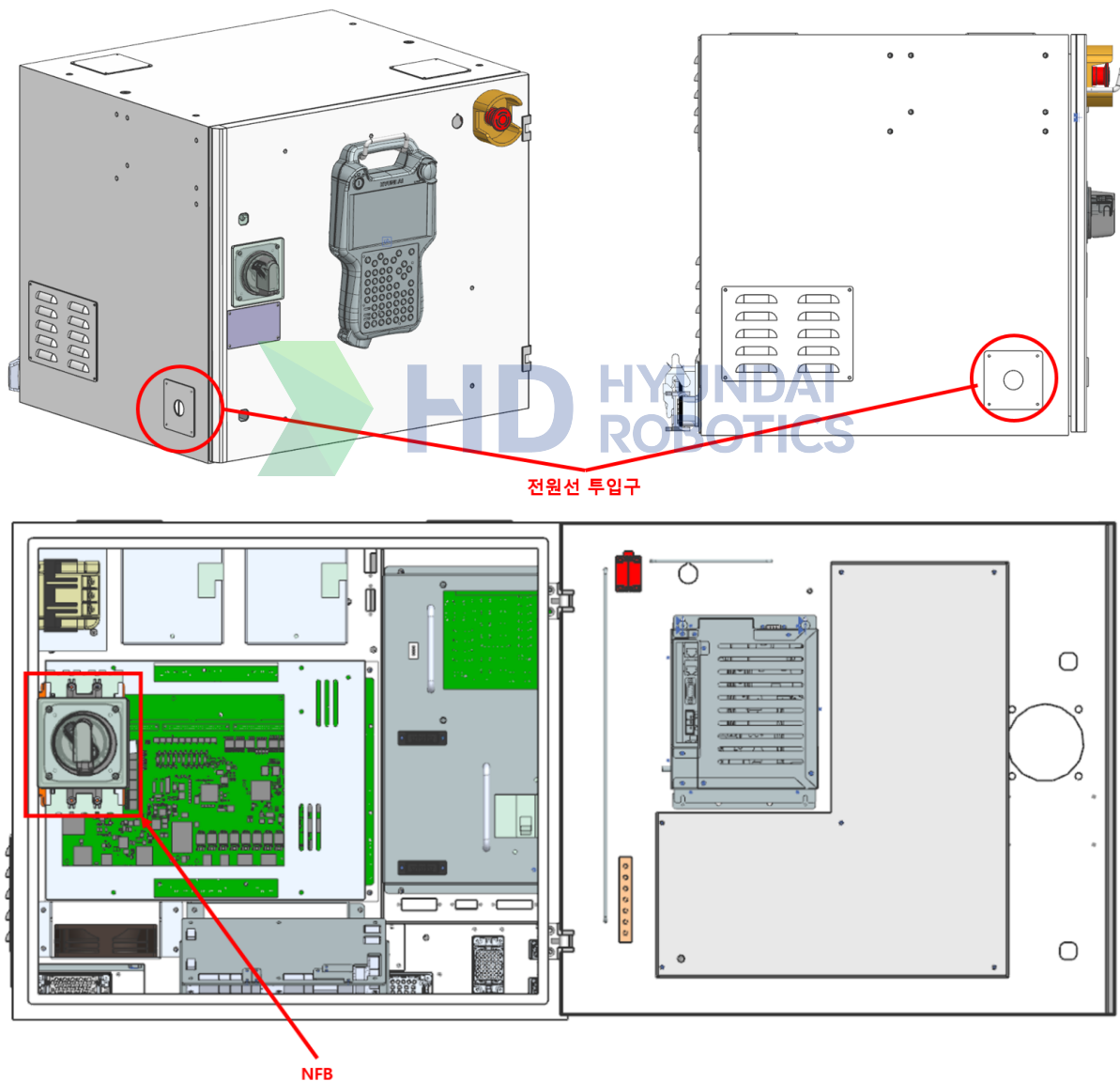
그림 3.7 Hi6-N**(U) 제어기에 1차 전원 접속부
