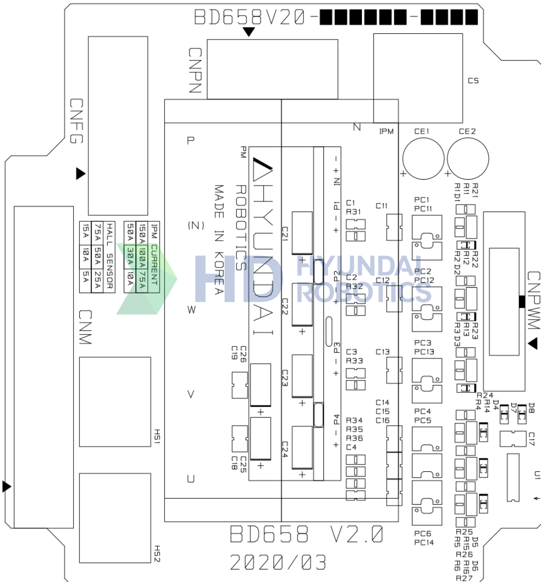
그림 4.24 H6D1X 용 BD658 부품 배치도
