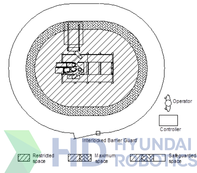
그림 1.5 LCD 핸들링 로봇의 빔형 안전펜스
