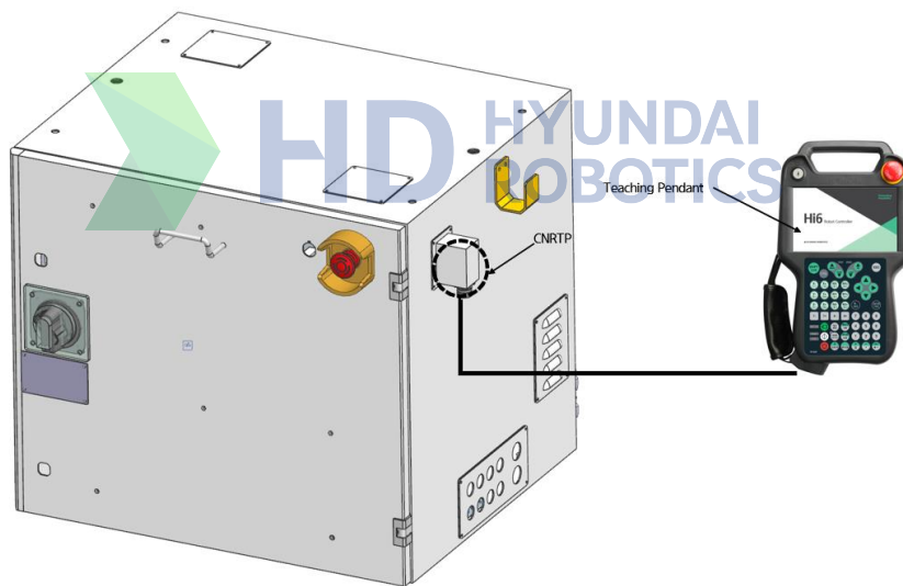
그림 3.5 Hi6-N**(U) 티칭펜던트의 접속
