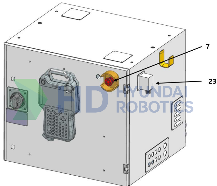
그림 4.3 Hi6-N00(U)/N30(U)/N80(U) 제어기 전면 외부의 부품배치
