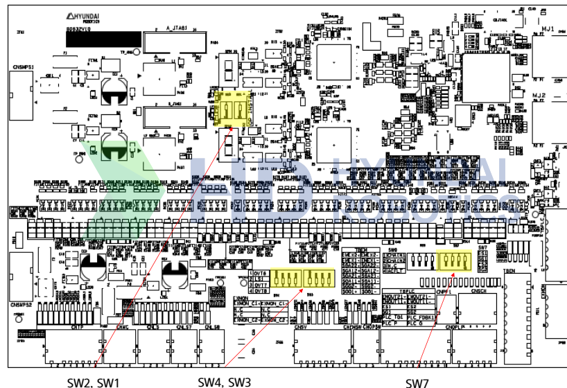
그림 4.11 BD632(Safety IO Board)의 설정장치 설명
