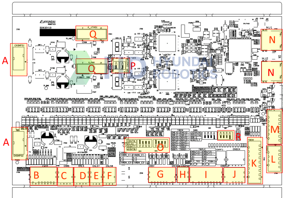
그림 4.7 BD632(Safety IO Board)의 커넥터 및 스위치 배치
