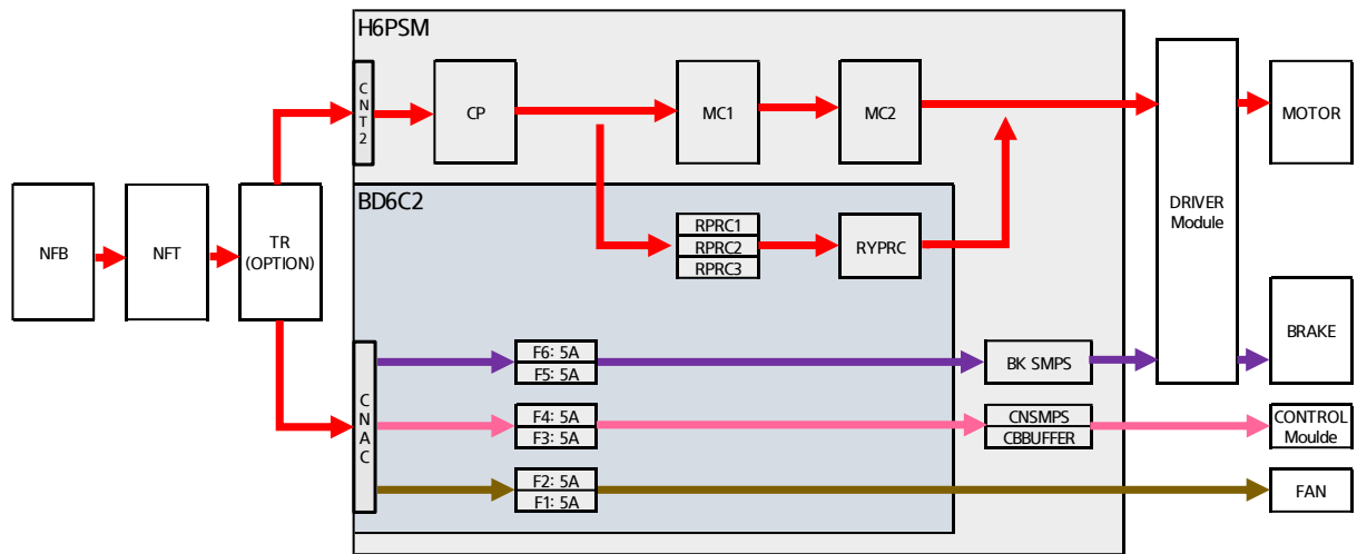
그림 4.27 Hi6-N 제어기의 전원계통
