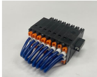
그림 4.8 BD632(Safety IO Board) TBEM
