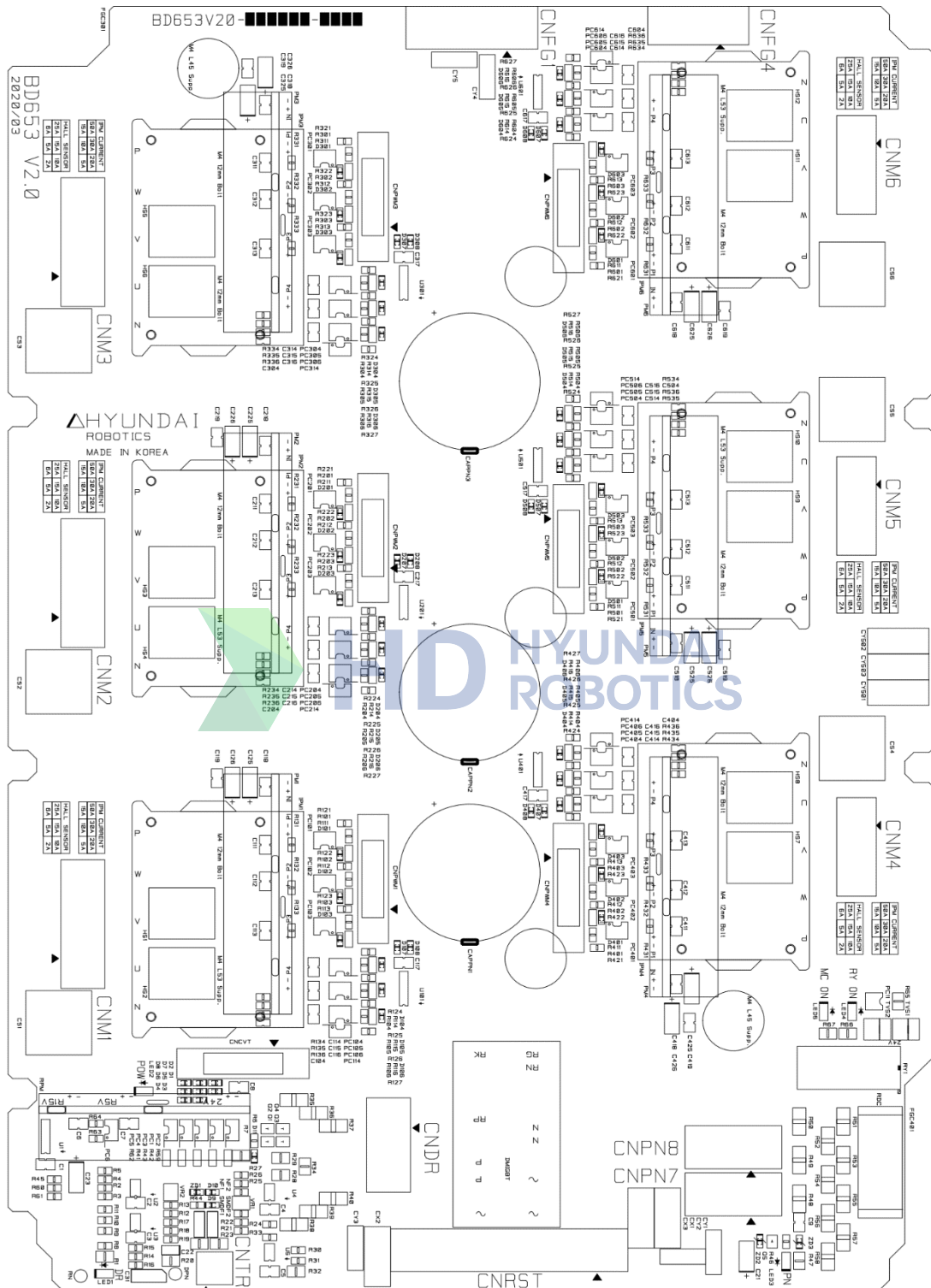
그림 4.22 BD653 부품 배치도
