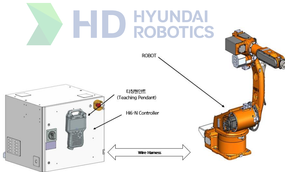
그림 3.1 산업용 로봇 설치의 기본 구성
