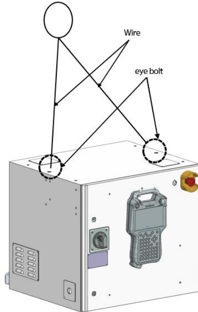
그림 3.3 제어기 와이어 연결 위치
