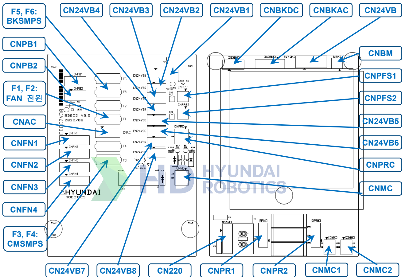
그림 4.28 전장보드(BD6C2)의 커넥터
