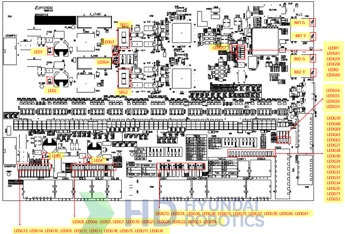
그림 4.10 BD632(Safety IO Board)의 표시장치
