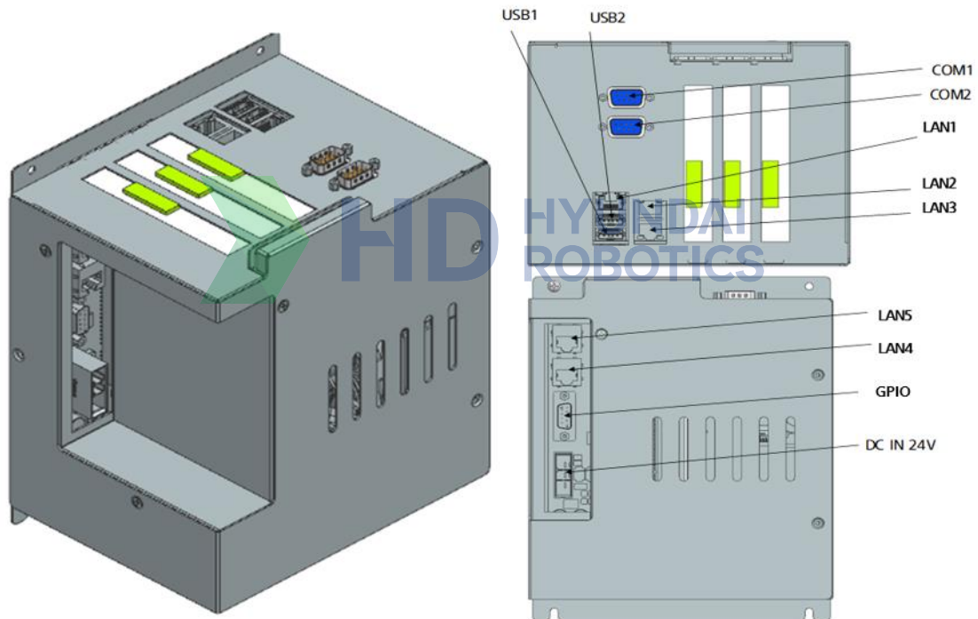
그림 4.6 H6COM-T
