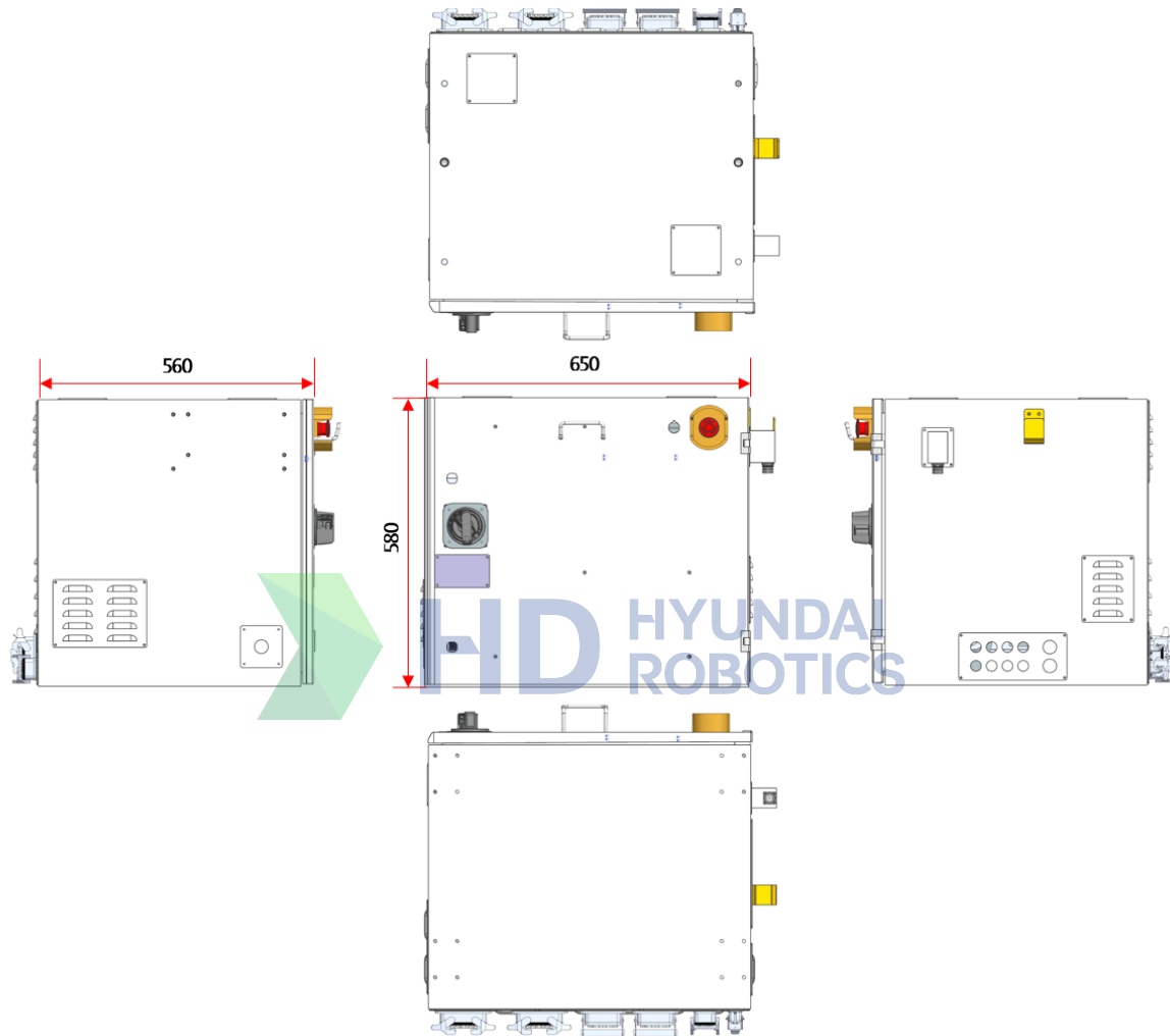
그림 2.1 제어기 전면 외관도
