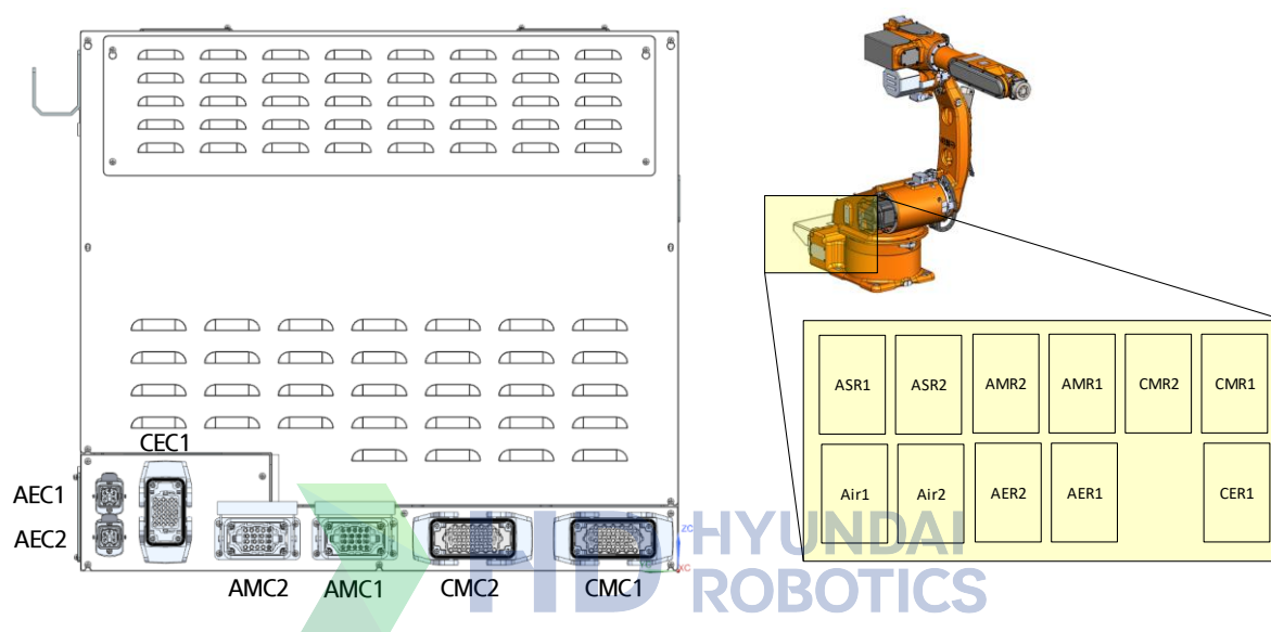
Wire Harness 결선도
