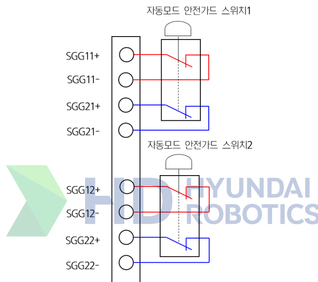
그림 4.16 터미널블록 TBEM 에 접점입력 자동 안전가드를 연결하는 방법
