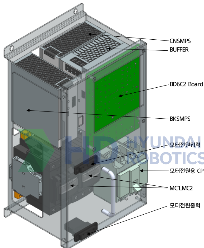
그림 4.26 H6PSM(Hi6-N 제어기 전원공급모듈) 외부
