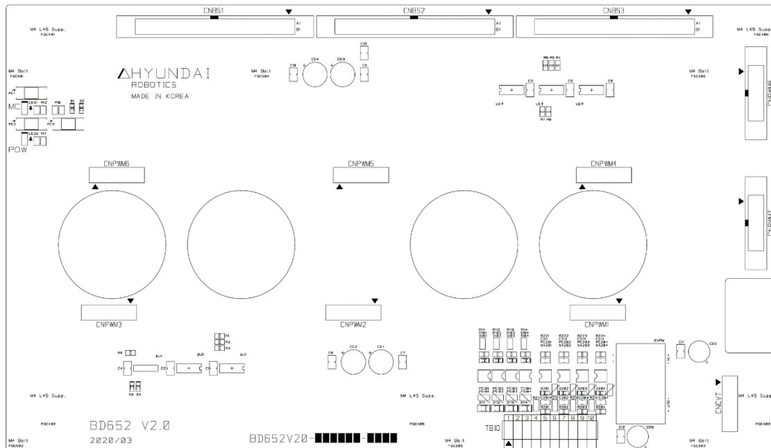
그림 4.21 BD652 부품 배치도
