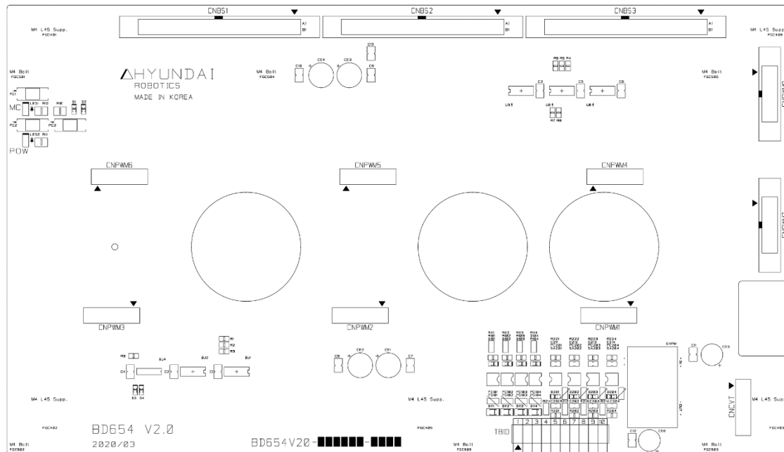
그림 4.23 BD654 부품 배치도
