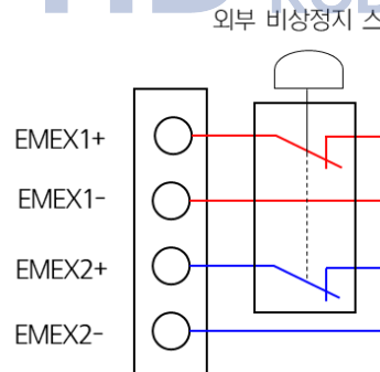
그림 4.12 터미널블록 TBEM 에 외부비상정지 스위치를 연결하는 방법
