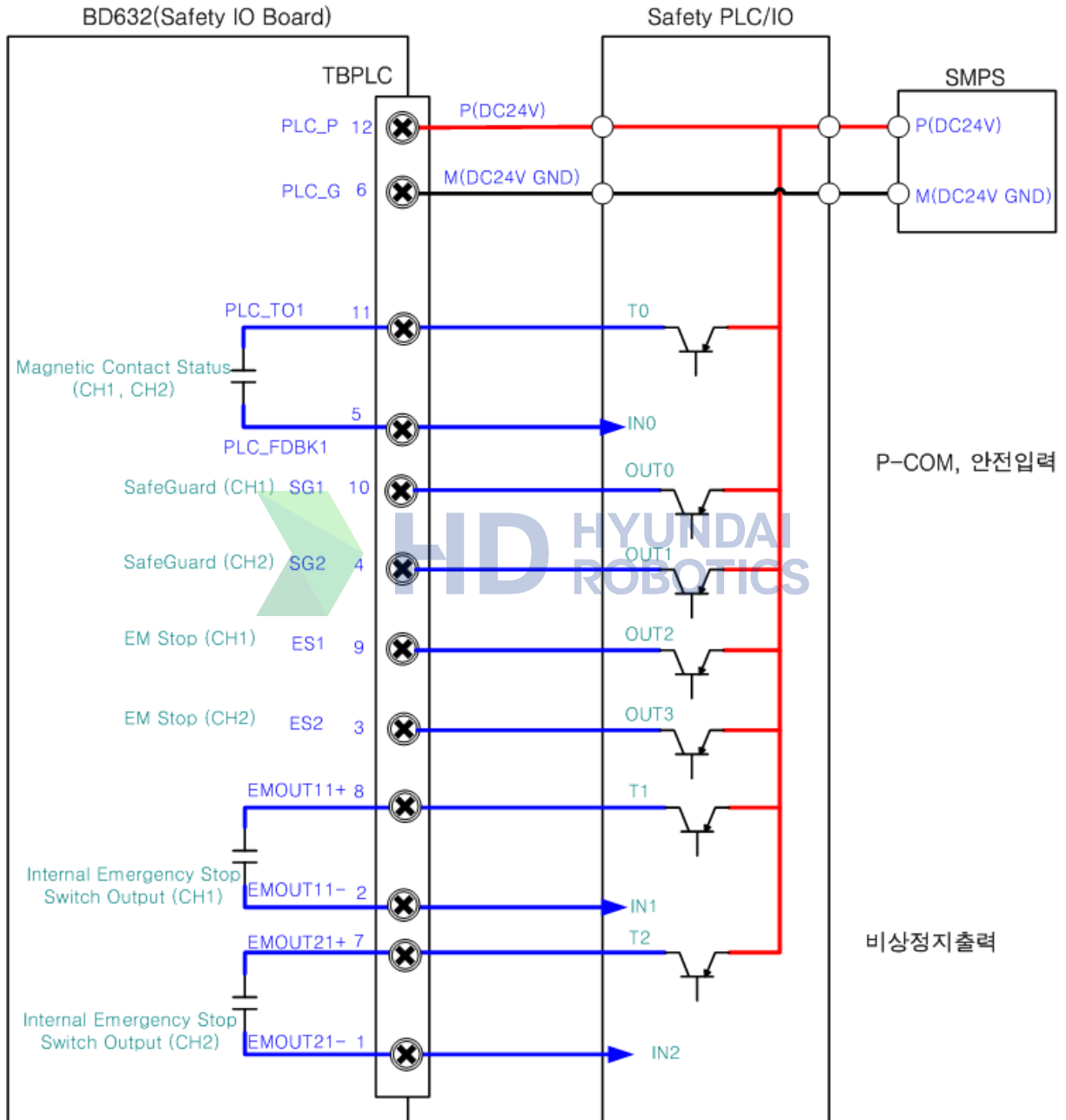
그림 4.18 Safety PLC/IO의 연결방법
