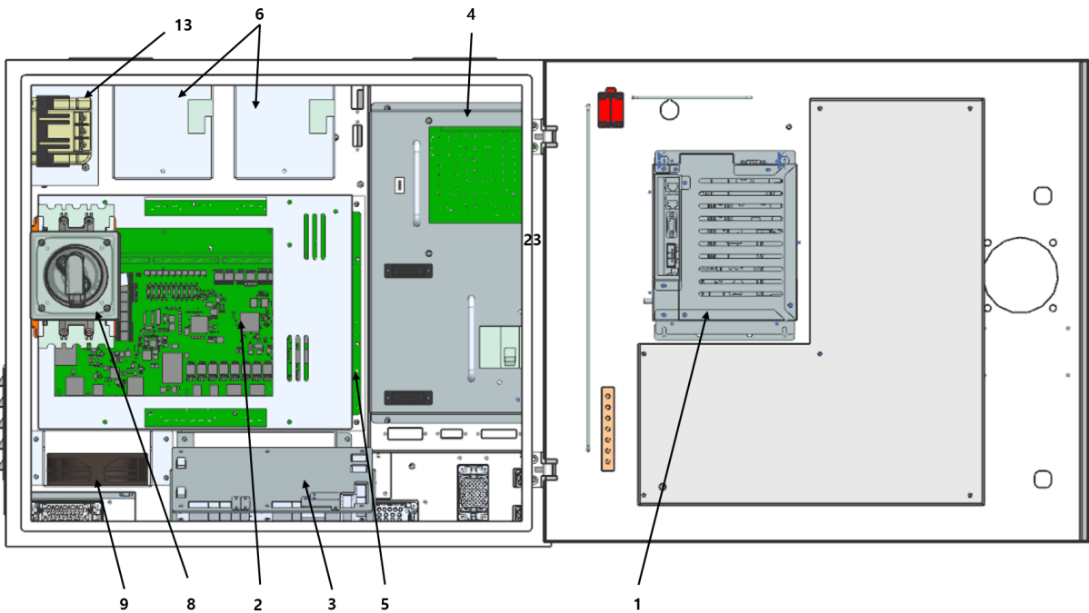
그림 4.4 Hi6-N00(U)/N30(U)/N80(U) 제어기 전면 내부의 부품배치
