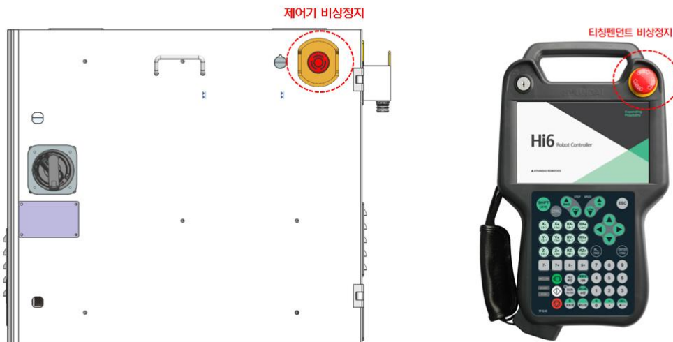
그림 1.2 제어기, 티칭펜던트 비상정지 스위치
