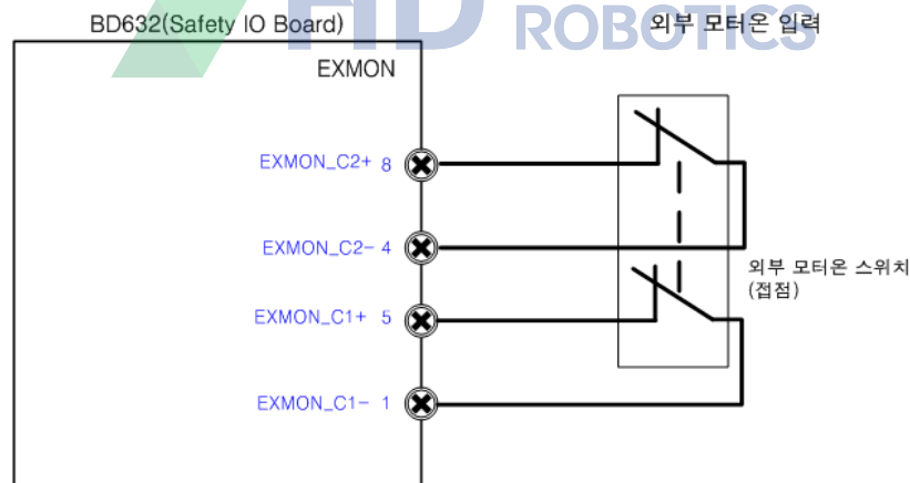
그림 4.19 외부 모터온 신호의 연결방법
