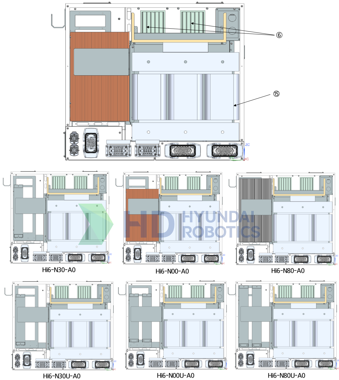
그림 4.5 Hi6-N00(U)/N30(U)/N80(U) 제어기 후면 부품배치
