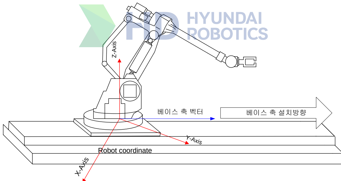
그림 7.99 베이스 축 캘리브레이션
