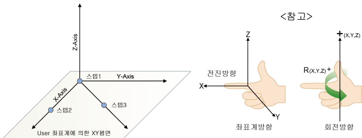
그림 10.7 사용자 좌표계
