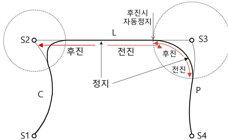
그림 2.25 End 재생 전/후진 경로
