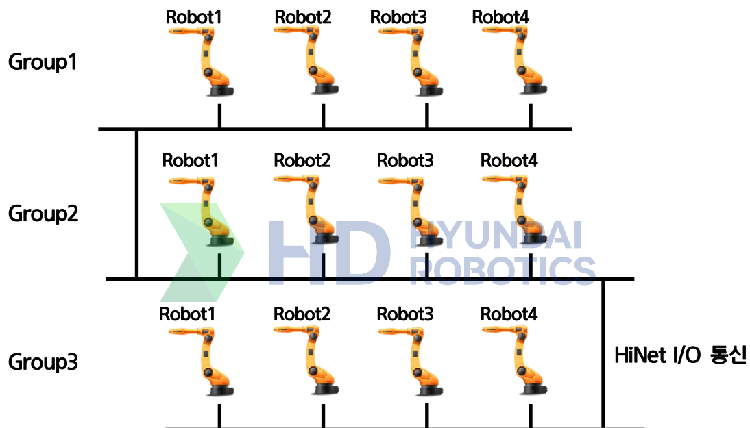
그림 10.4 협조 그룹/로봇과 HiNet I/O
