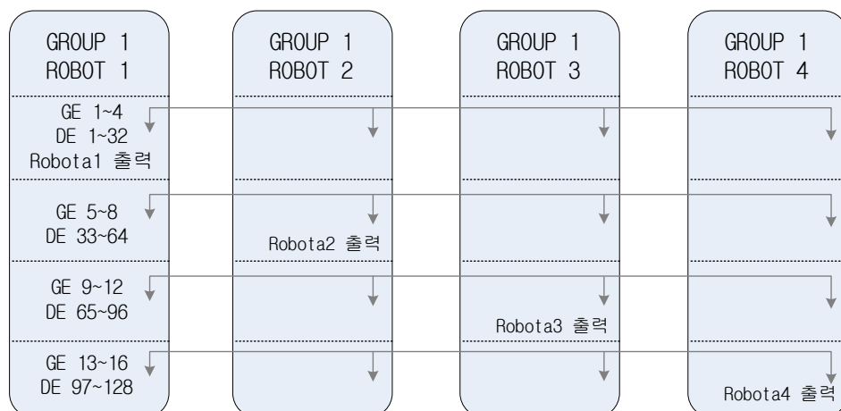
그림 10.5 HiNet I/O 사용 예시(그룹 1 번 – 로봇 4 대)
