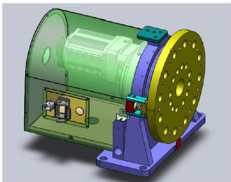
1 축 포지셔너
