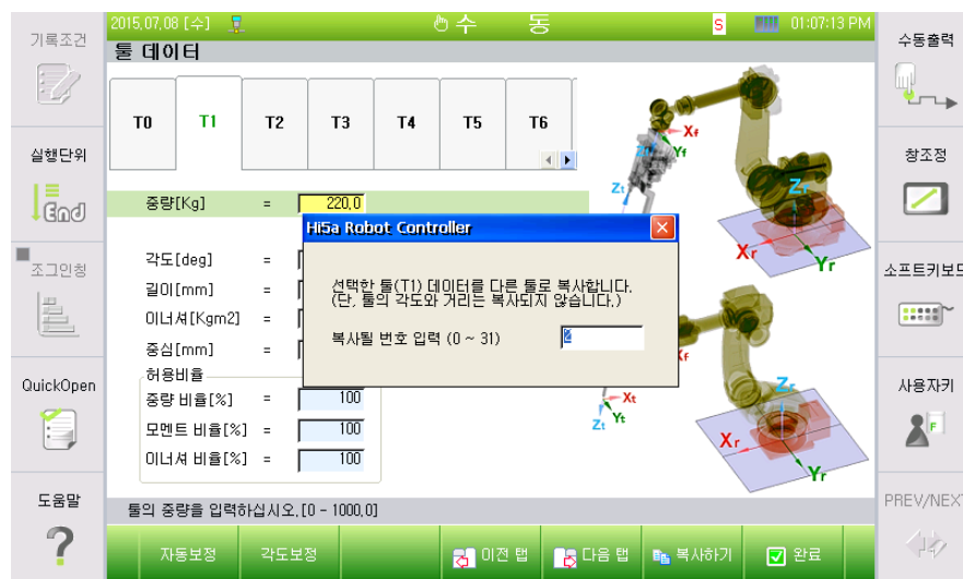
그림 7.60 툴각도 보정 화면
