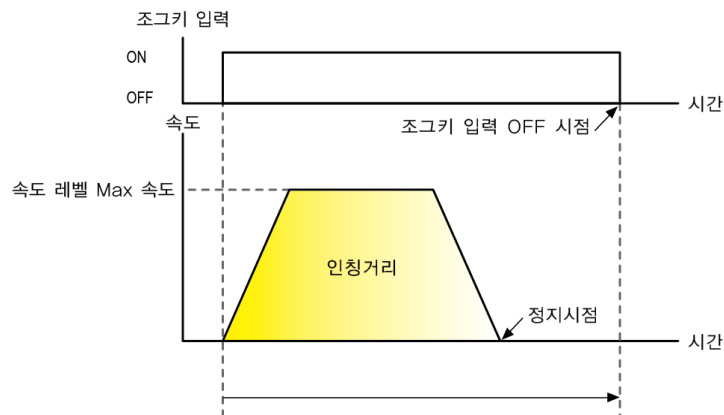
그림 7.75 인칭거리 도달후 키를 뗀 경우 로봇의 동작
