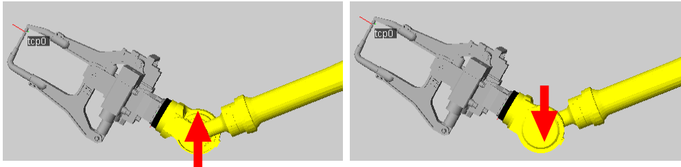
그림 2.41 Flip(좌)/Non-flip(우) 자세
