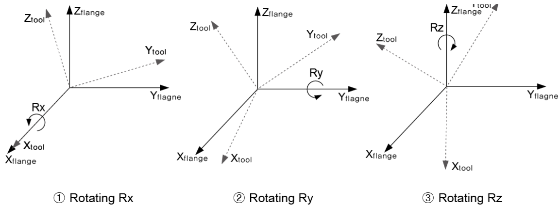
그림 7.56 툴 각도
