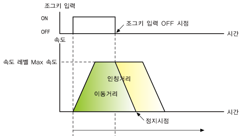
그림 7.76 인칭거리 도달전 키를 뗀 경우 로봇의 동작
