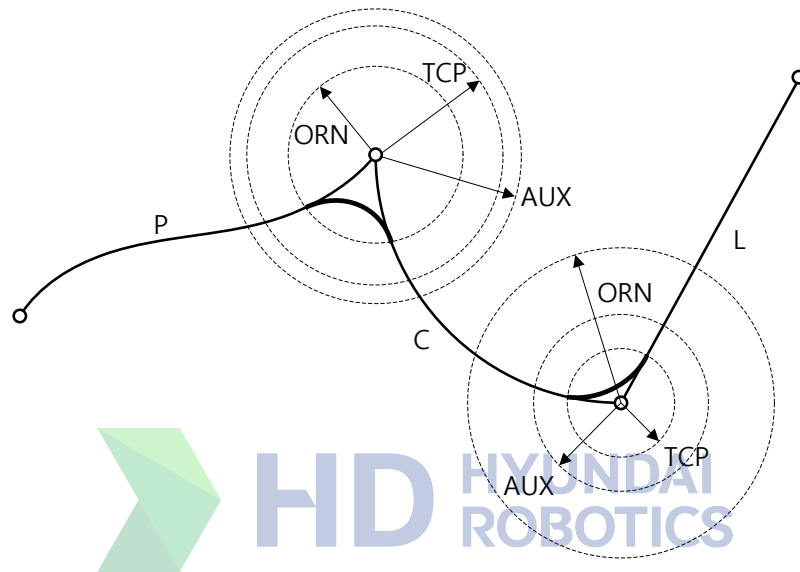
그림 2.36 Accuracy level 의 값에 따른 코너링 경로
