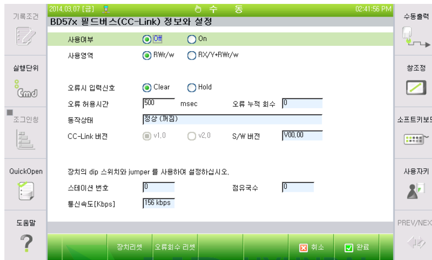
그림 7.24 BD57X 필드버스(CC-Link) 정보와 설정 메뉴
