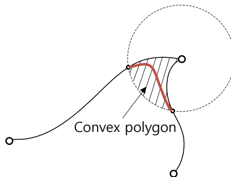
그림 2.37 코너링 경로의 모든 점이 convex polygon (빗금친 부분) 안에 존재함
