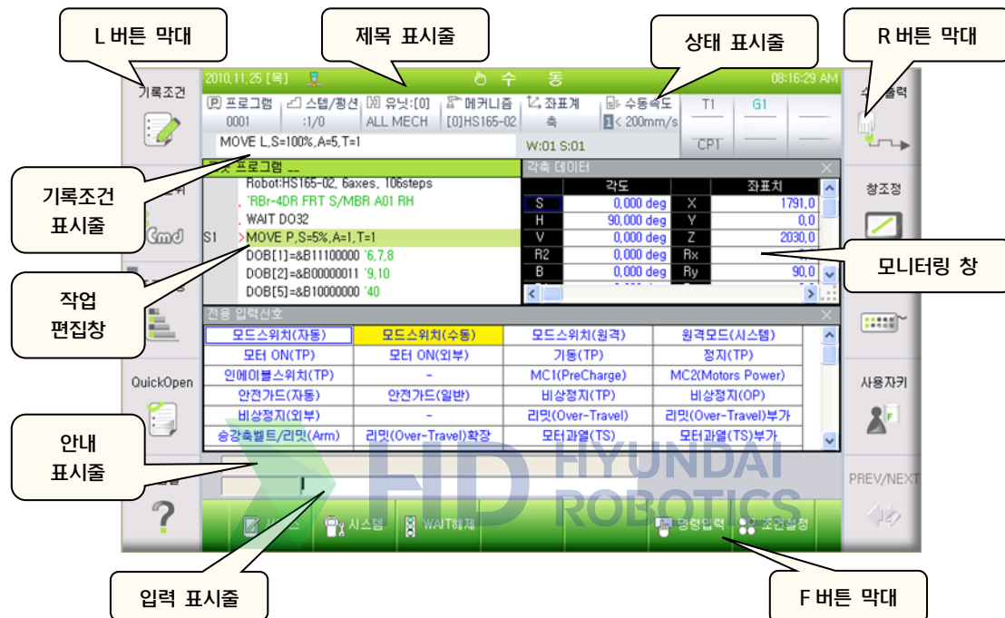
그림 2.6 티치펜던트 화면
