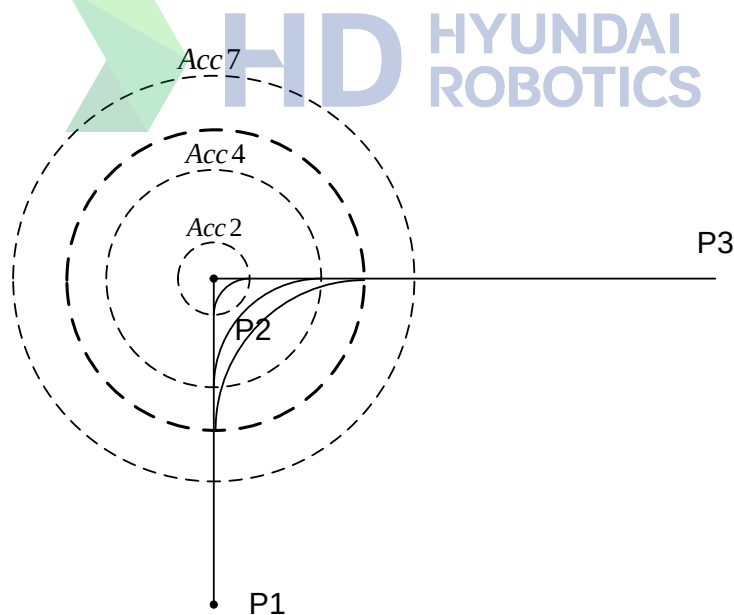
그림 2.35 P2 의 Accuracy 에 따른 경로변화
