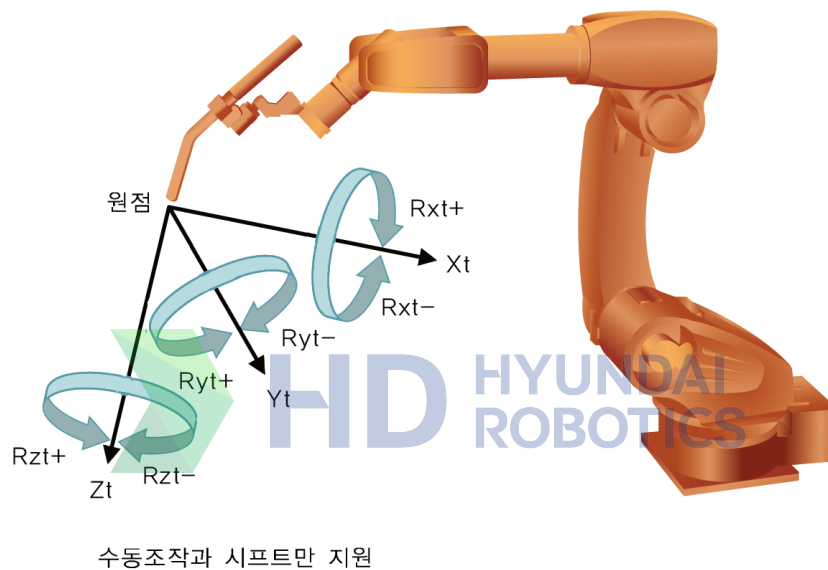
그림 2.53 툴 좌표계 (토치 부착인 경우)
