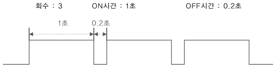
그림 7.13 펄스출력 사용 예
