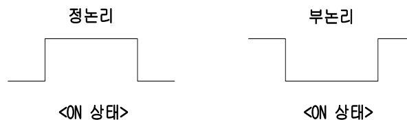
그림 7.10 범용입력 신호의 정논리, 부논리
