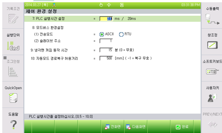
그림 7.7 제어 환경 설정 메뉴 (2)
