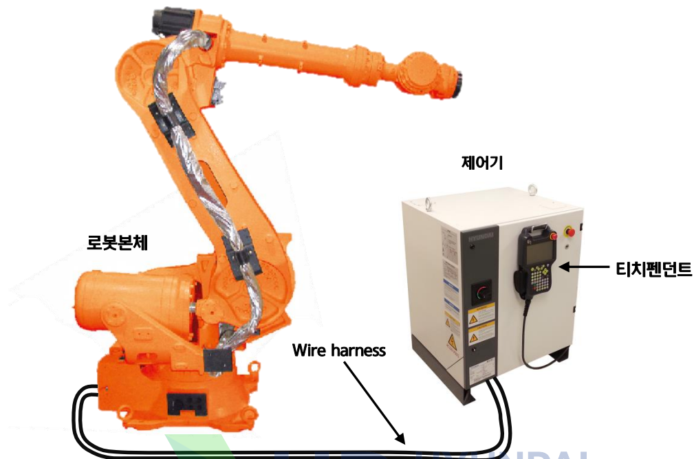
그림 2.3 로봇 시스템의 기본 구성도 (수직 다관절 로봇)
