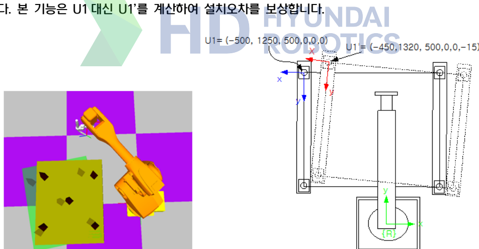
그림 7.103 OLP 를 위한 좌표계 보정 방법 예
