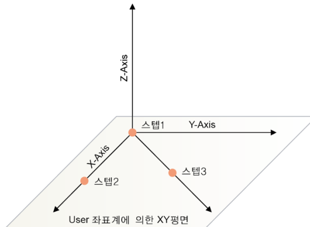
그림 7.37 사용자 좌표계 정의를 위한 3 개의 기준 스텝의 티칭방법
