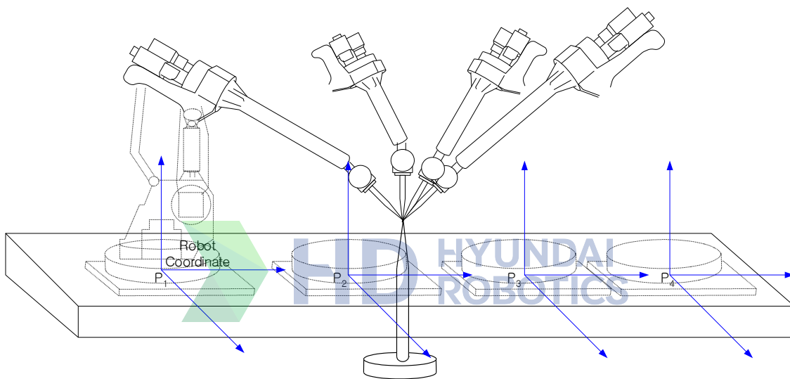
그림 7.100 베이스축 캘리브레이션 프로그램 티칭
