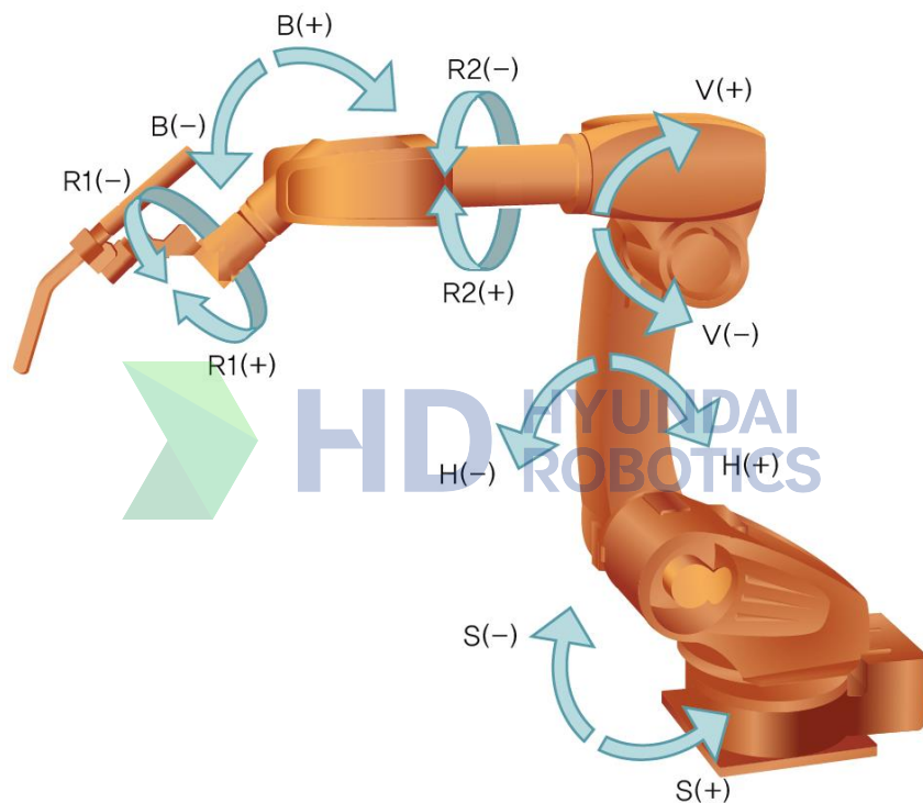
그림 2.49 축 좌표계
