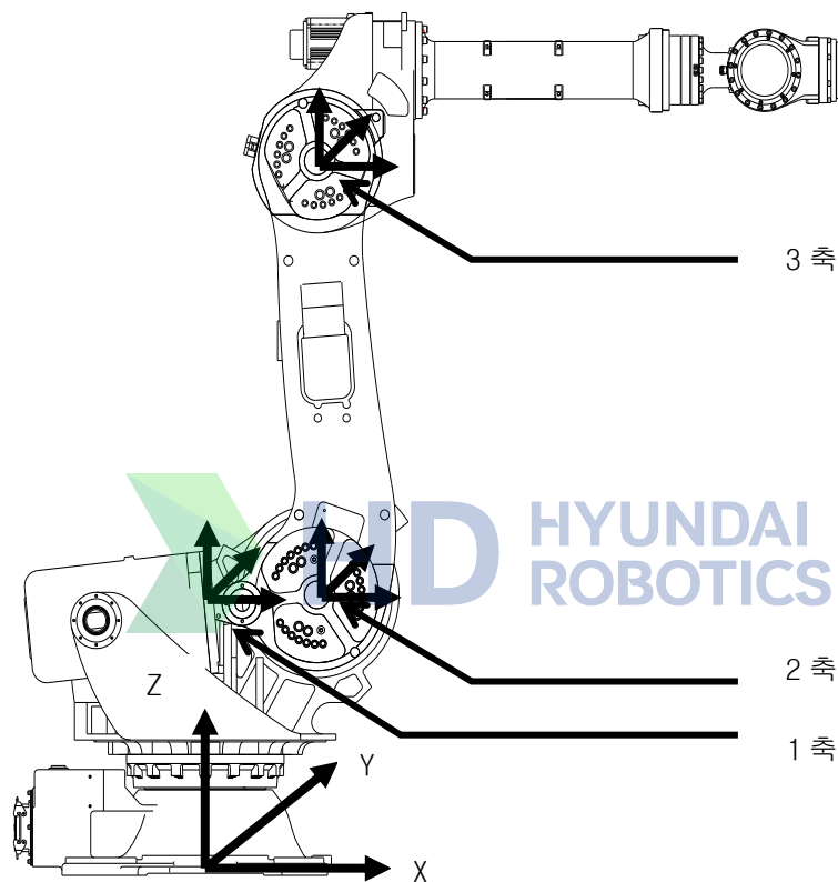
그림 7.68 각 축에 대한 좌표계 원점
