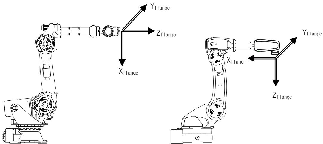
그림 7.55 로봇 형태별 플랜지 좌표계
