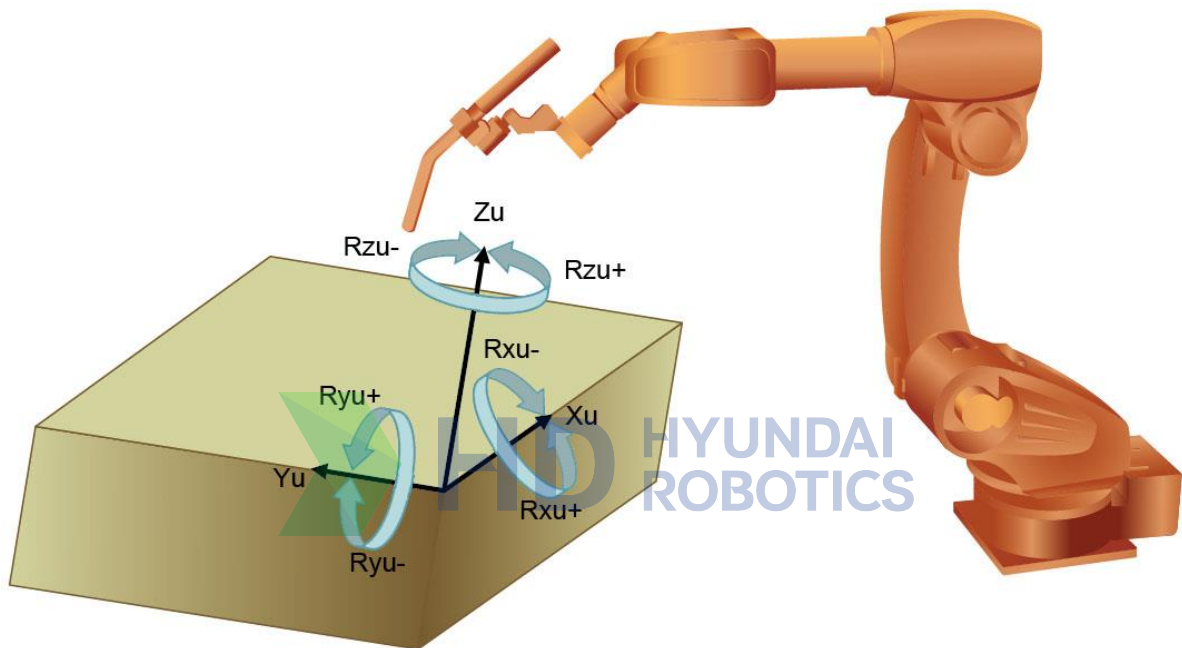
그림 2.52 사용자 좌표계
