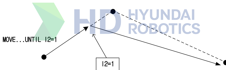
그림 2.38 정지 조건의 예
