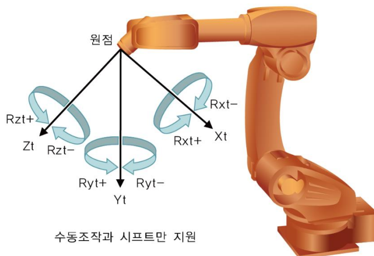
그림 2.54 툴 좌표계 (툴이 없는 경우)
