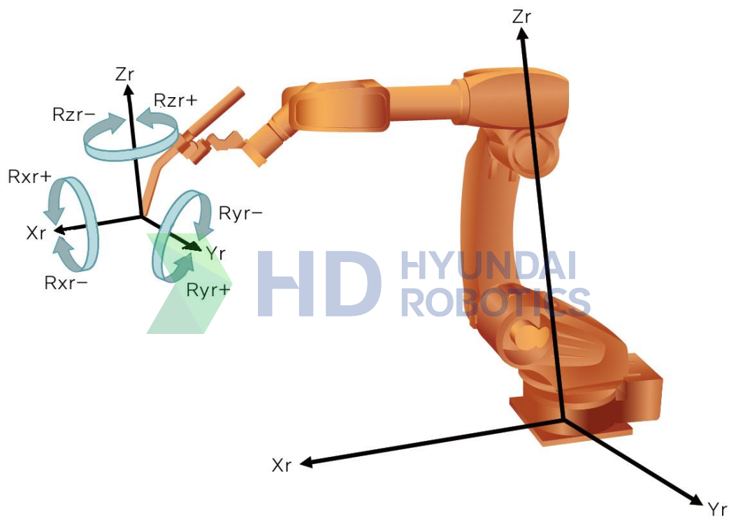
그림 2.50 로봇 좌표계
