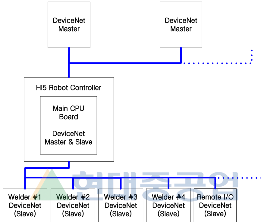
그림 1.2 Hi5 제어기 기반의 통합 용접 시스템 구성 예
