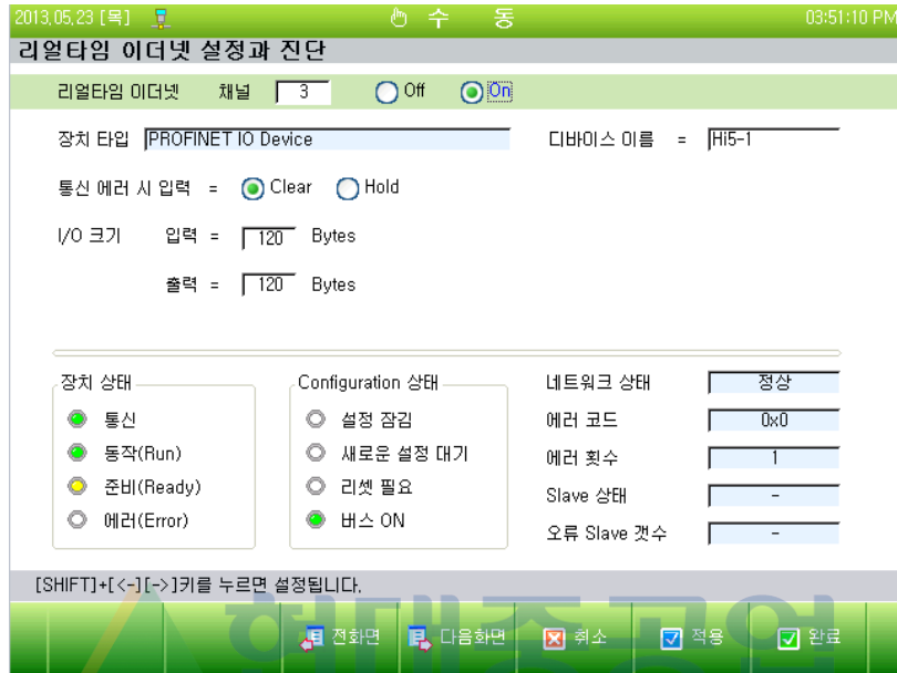
그림 3.2 PROFINET IO-Device 설정 화면
