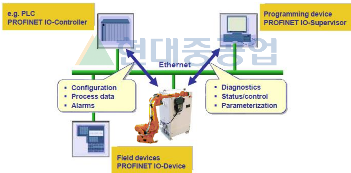
그림 1.1 PROFINET IO 통신 연결
