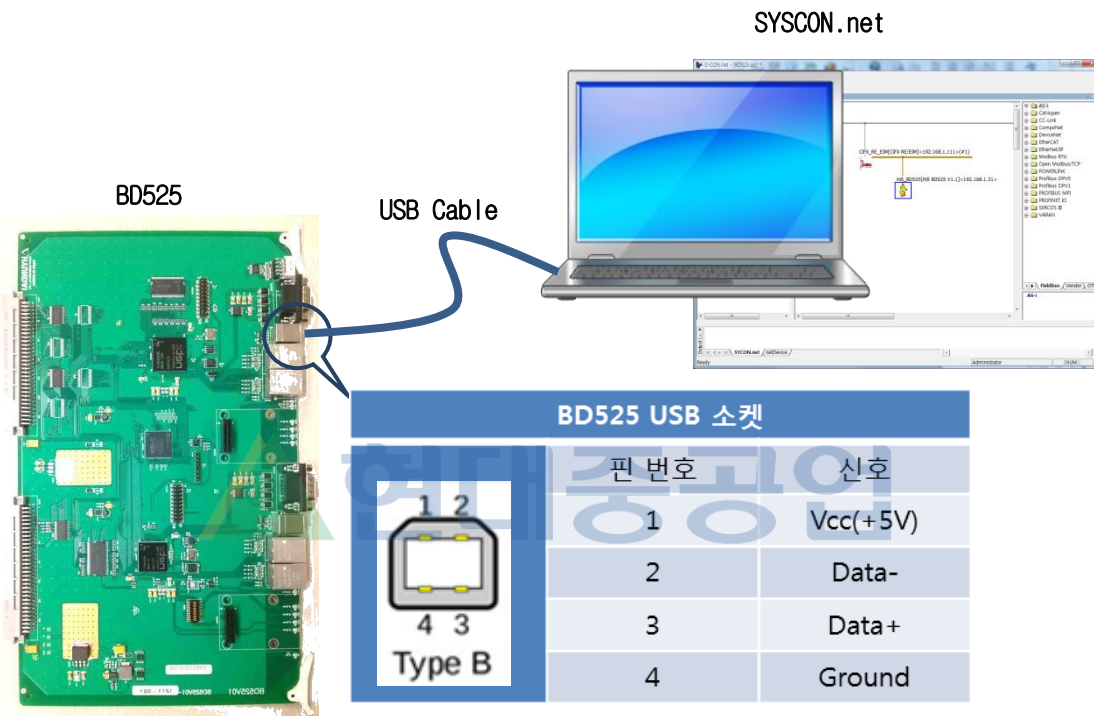
그림 4.1 SYCON.net 과 BD525 USB 연결
