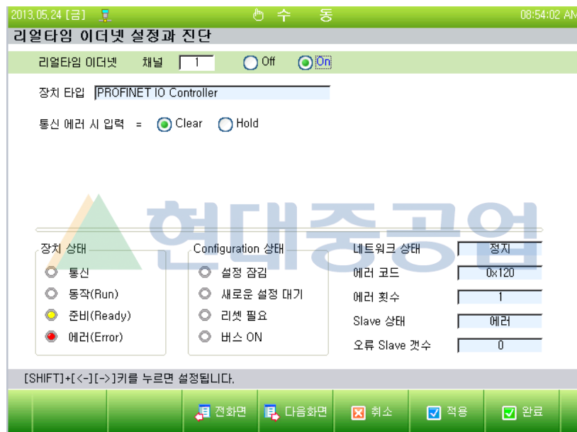
그림 4.4 PROFINET IO-Controller 진단 화면
