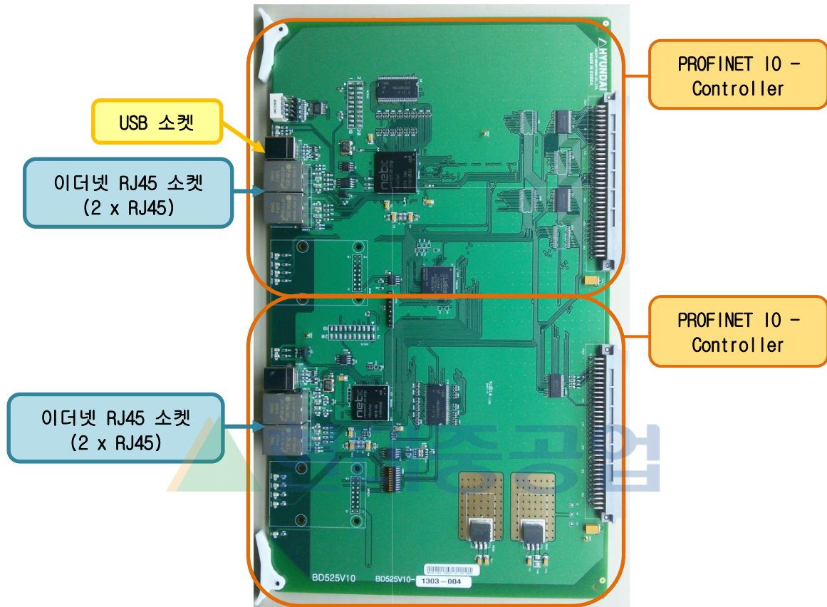
그림 1.2 BD525 PROFINET IO 통신 보드
