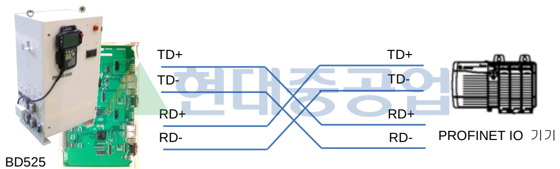
그림 2.5 Direct 케이블 연결
