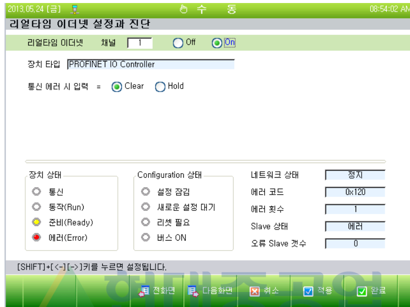
그림 4.3 PROFINET IO-Controller 설정 화면
