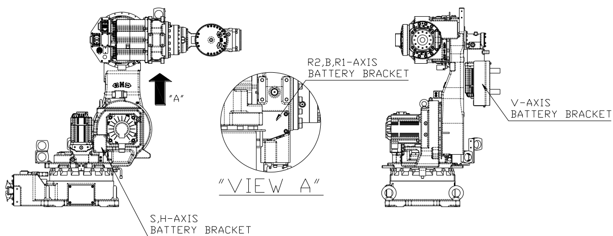
图 5.8 电池的位置
