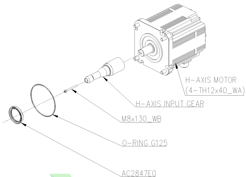
图 6.2 H 轴电机安装
