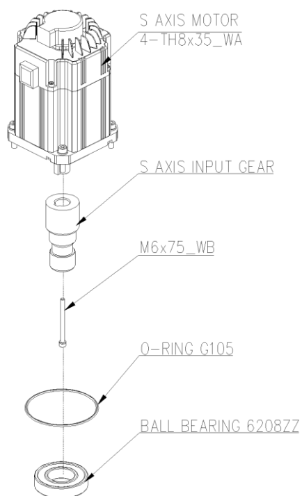
图 6.1 S 轴电机安装
