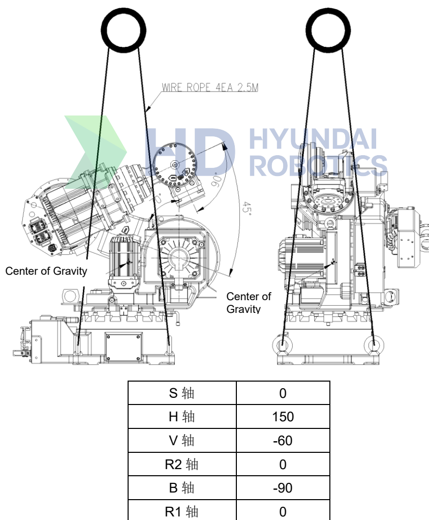
图 3.4 运送方法：使用吊车
