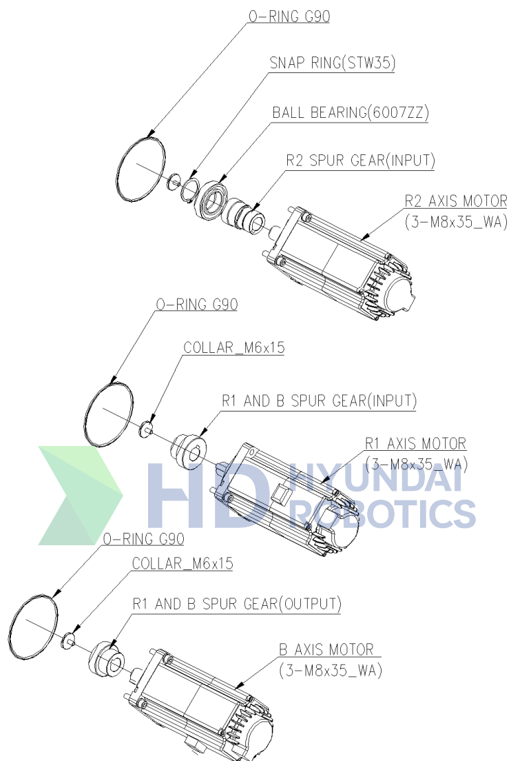
图 6.4 R2/B/R1 轴电机安装
