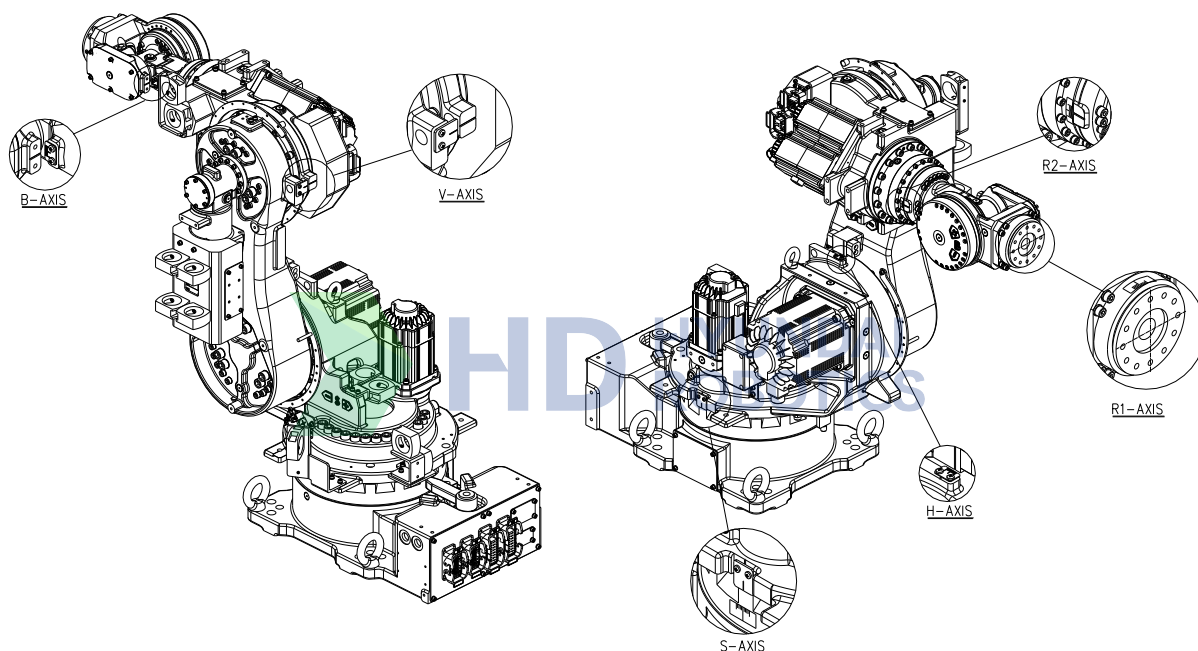
图 6.5 归零设定的方法(YS140D)
