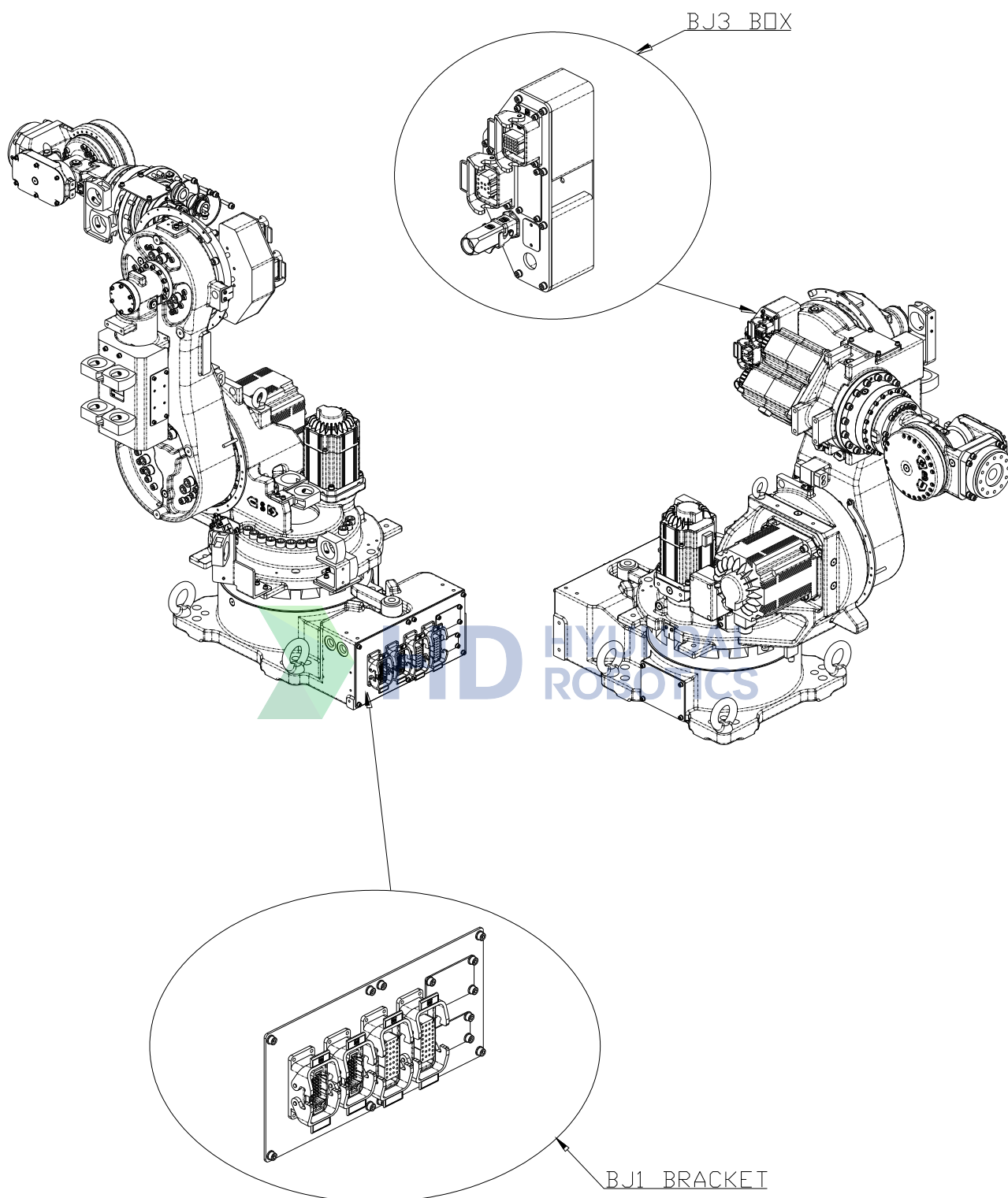
图 9.1 机械手配置 (YS140D)
