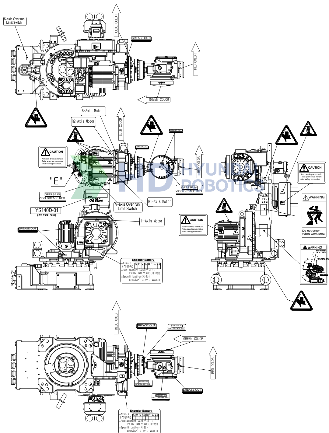
图 3.2 安全标识牌位置 (YS140D)
