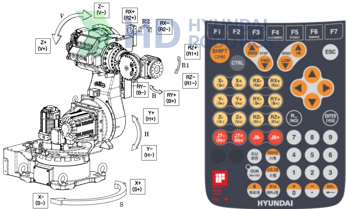
图 2.4 机器人尺寸和轴(YS140D)
