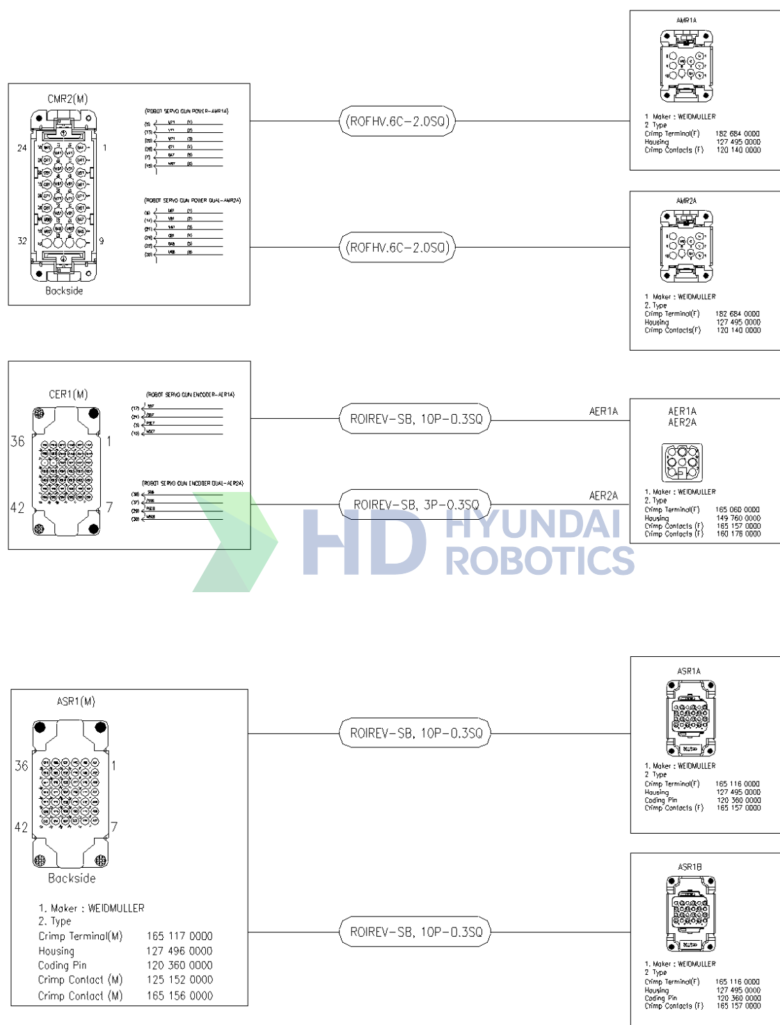
图 2.8 应用连接器细节 (YS140D)
