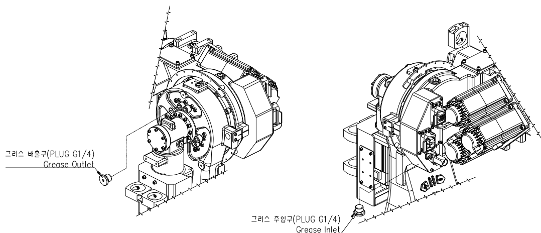
图 5.3 V 轴减速机润滑油加注/排油口
