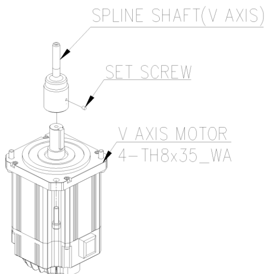
图 6.3 V 轴电机安装
