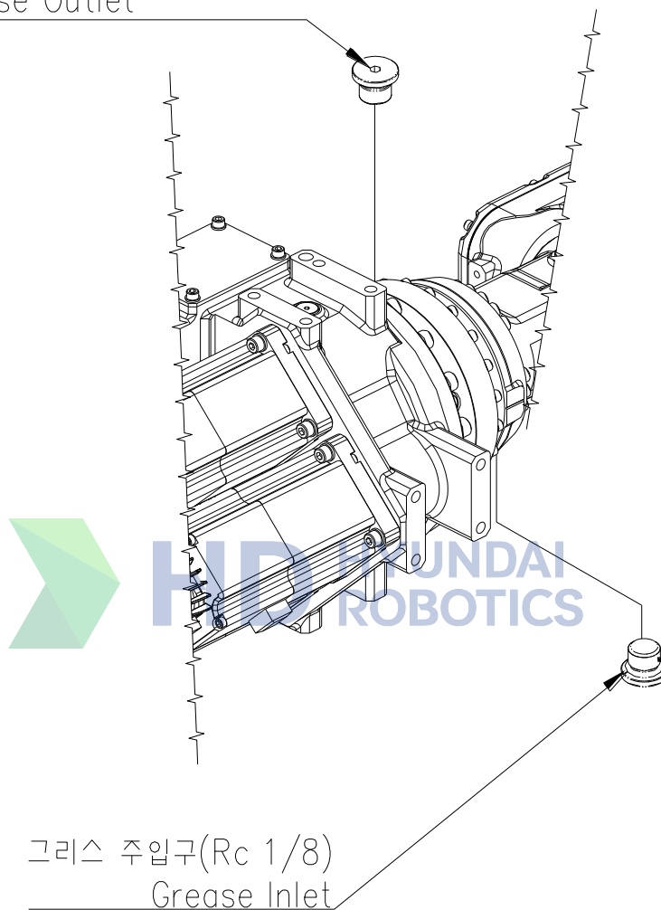
图 5.4 R2 轴减速机润滑油加注/排油口
