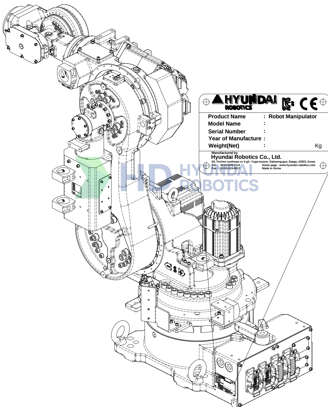
图 2.2 机器人识别铭牌的位置
