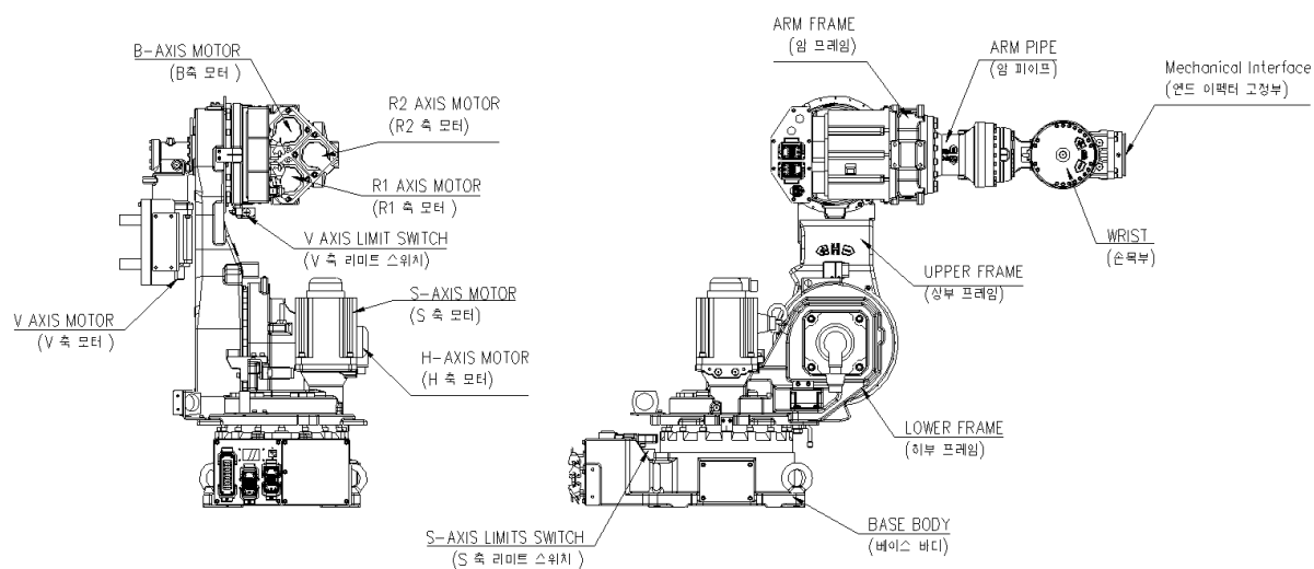
图 3.1 机器人零件名称 (YS140D)
