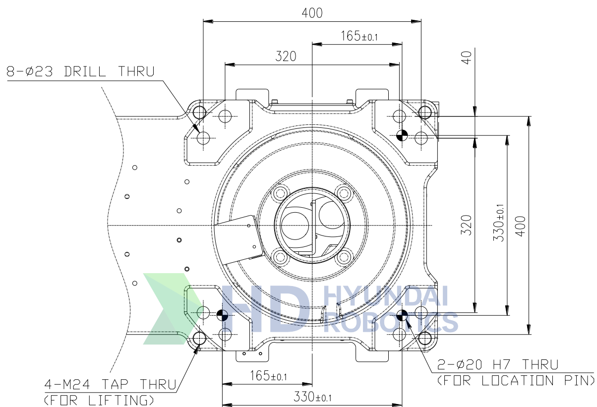
图 3.7 机器人安装尺寸 (YS140D)
