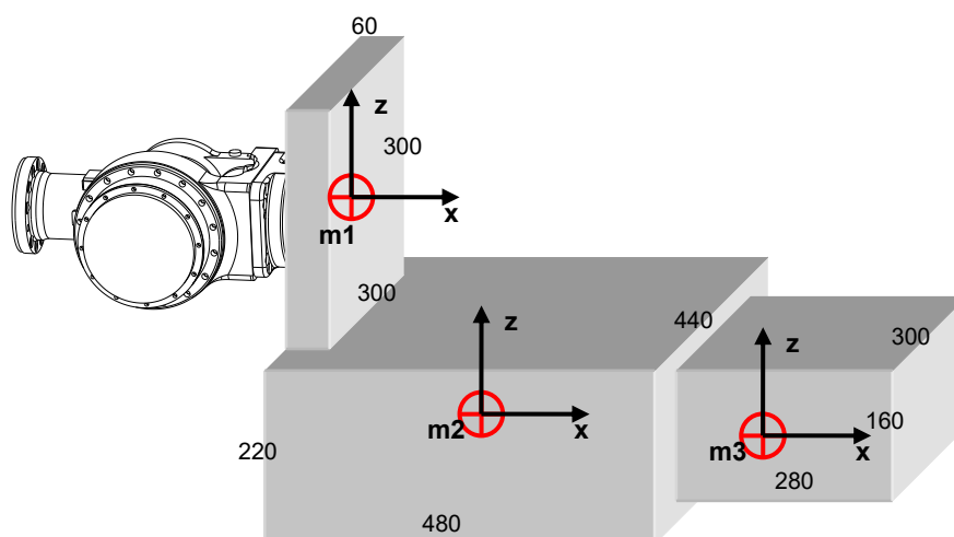
图 3.13 3-D 负载模型 3-D 形状
