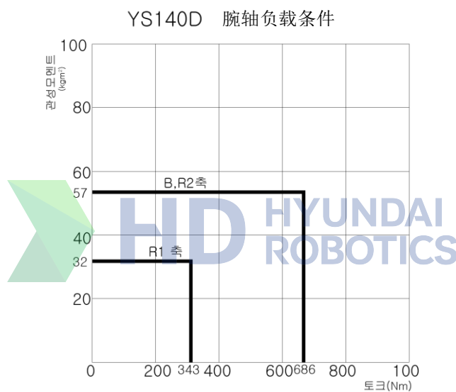
图 3.10 腕轴负载条件 (YS140D)
