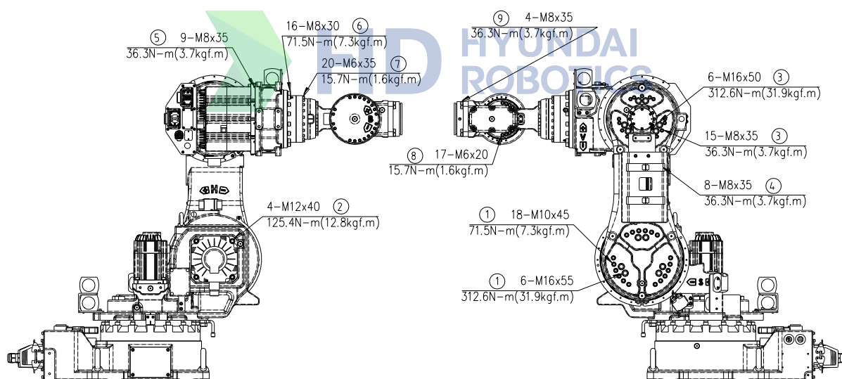
图 4.1 主要螺栓的检查部位 (YS140D)
