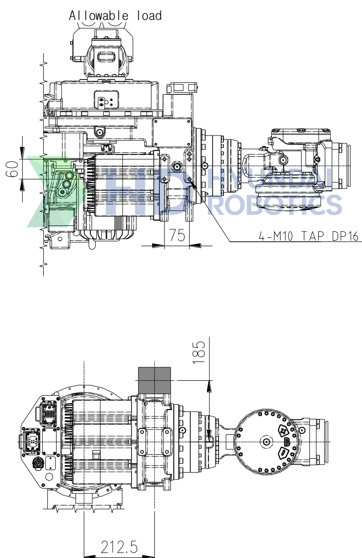
图 2.6 上机械臂支撑连接面细节 (YS140D)
