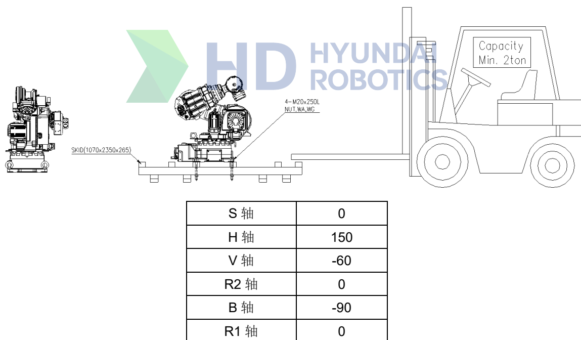
图 3.5 运送方法：利用叉车
