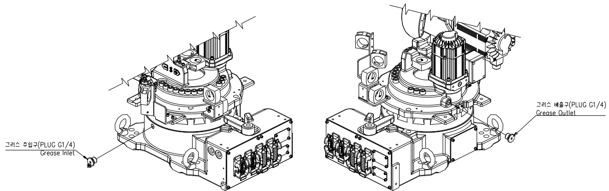
图 5.1 S 轴减速机润滑油加注/排油口
