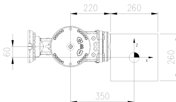
图 3.11 2-D 负载模型
