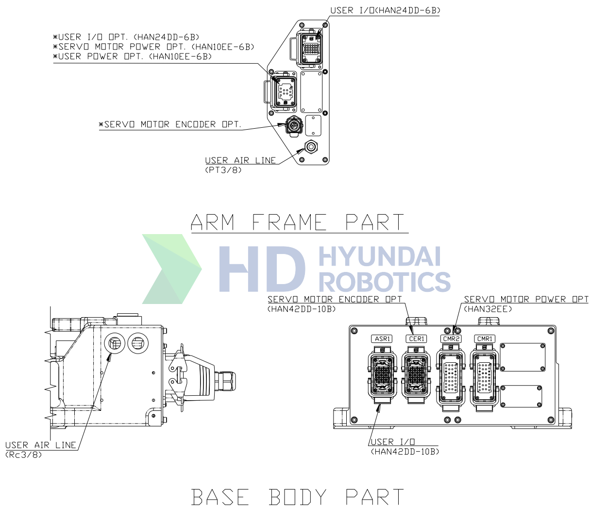
图 2.7 工作线路和检查线路图 (YS140D)
