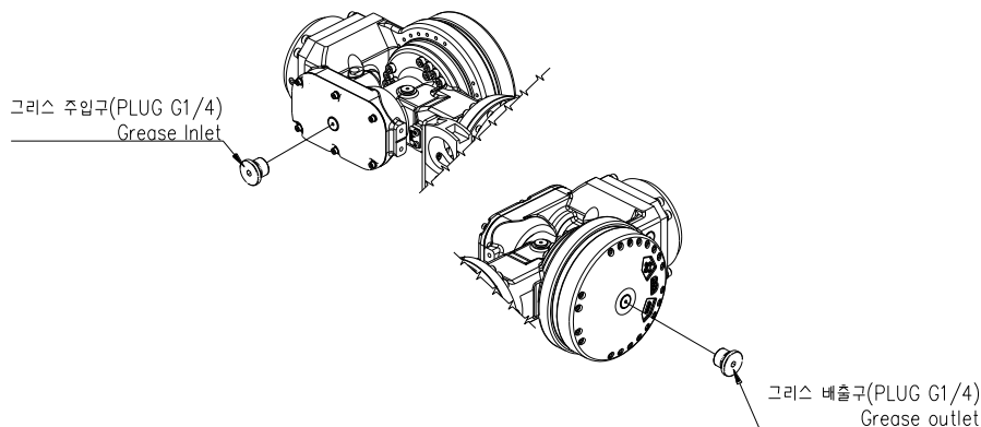
图 5.5 B 轴减速机润滑油加注/排油口 (YS140D)
