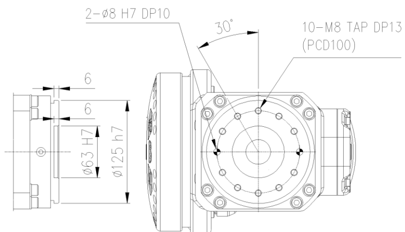
图 2.5 机械腕轴连接面细节 (YS140D)
