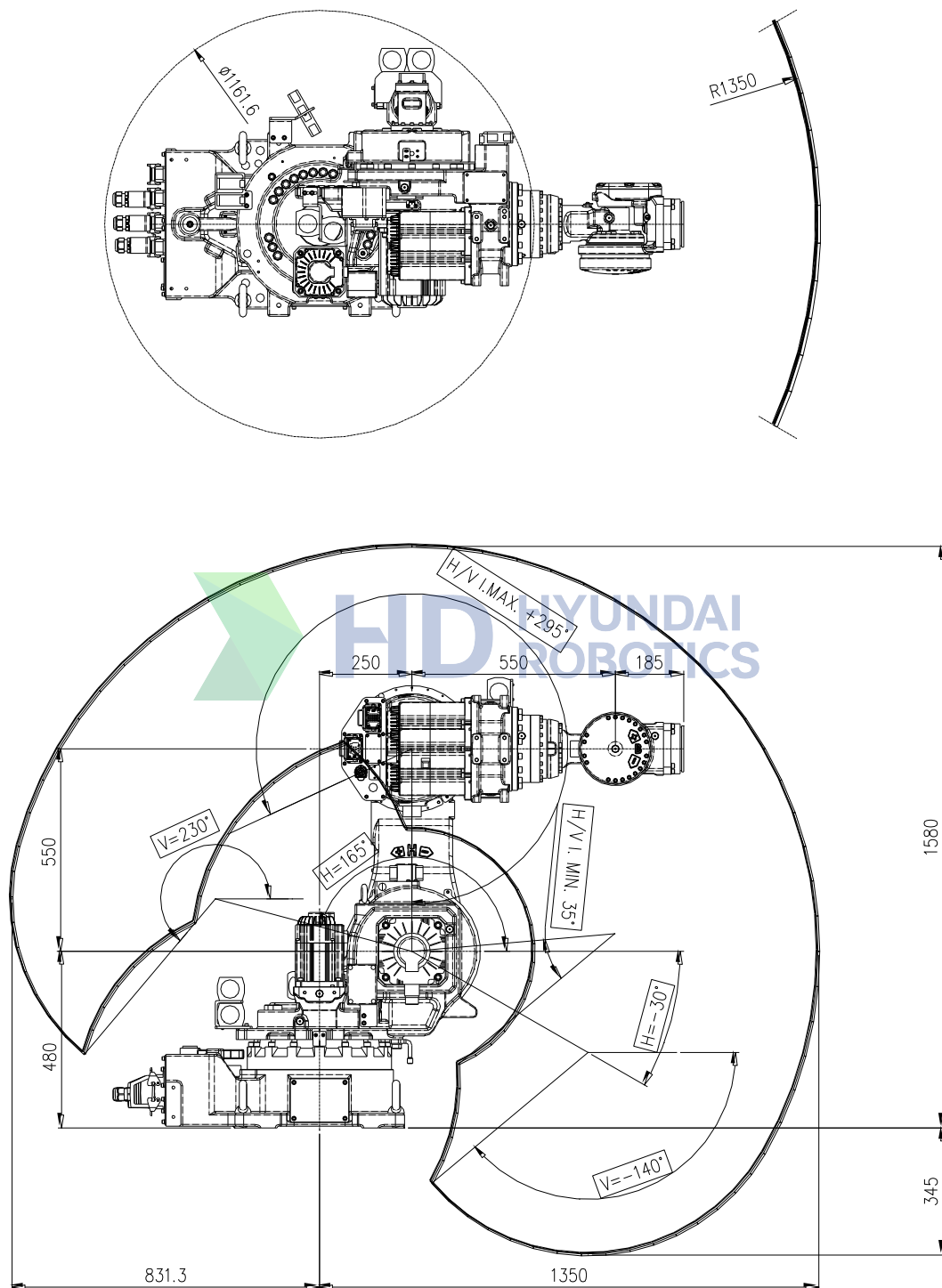
图 2.3 机器人尺寸和工作区间 (YS140D)
