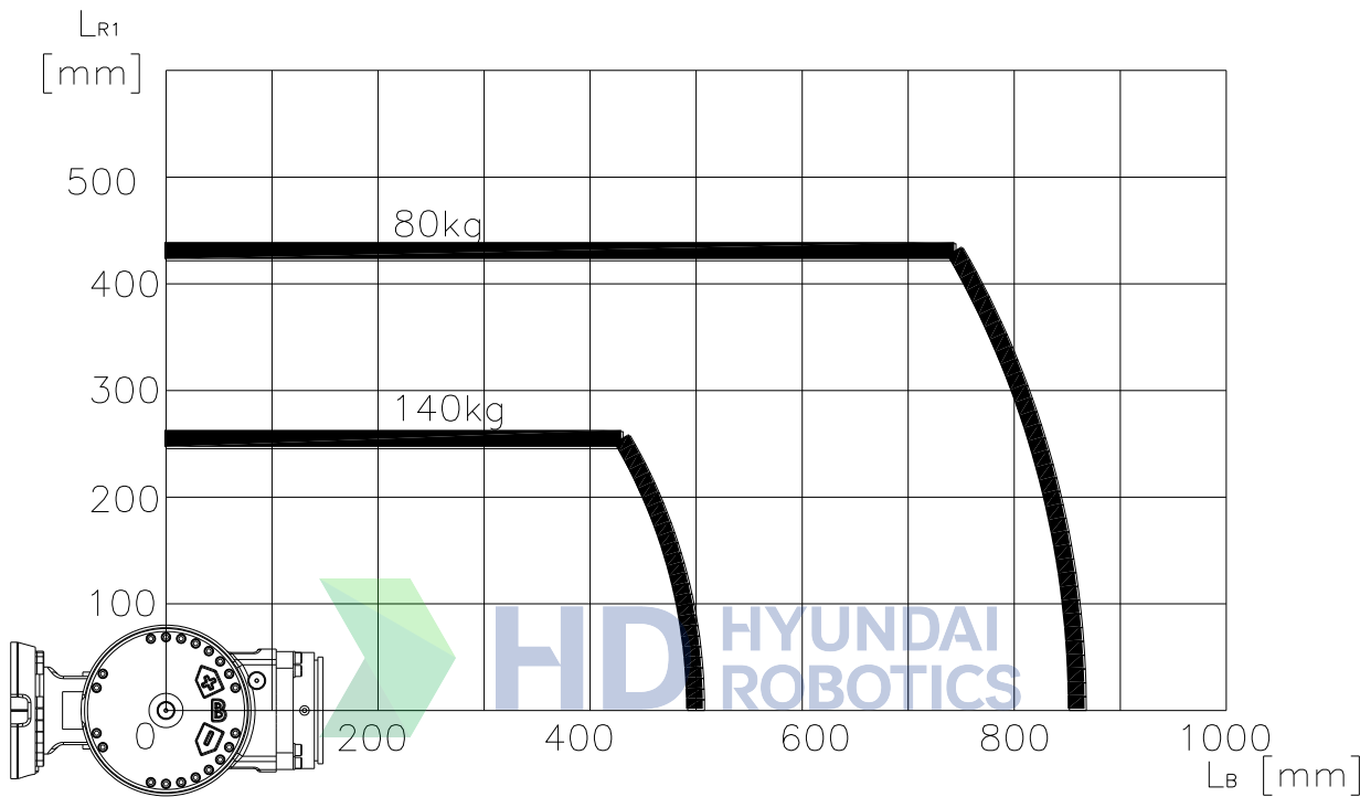
图 3.9 腕轴转矩图 (YS140D)
