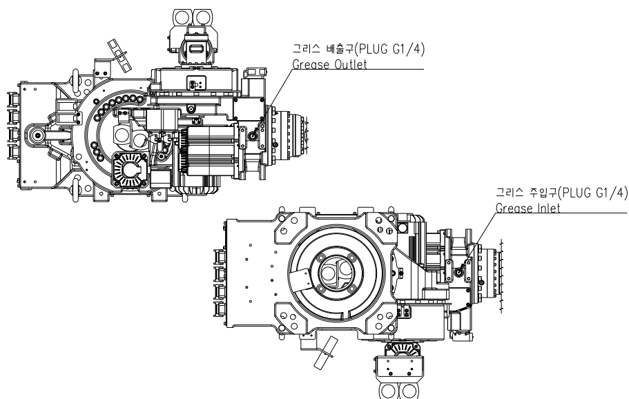
图 5.7 Arm Frame 润滑油注入/排油口
