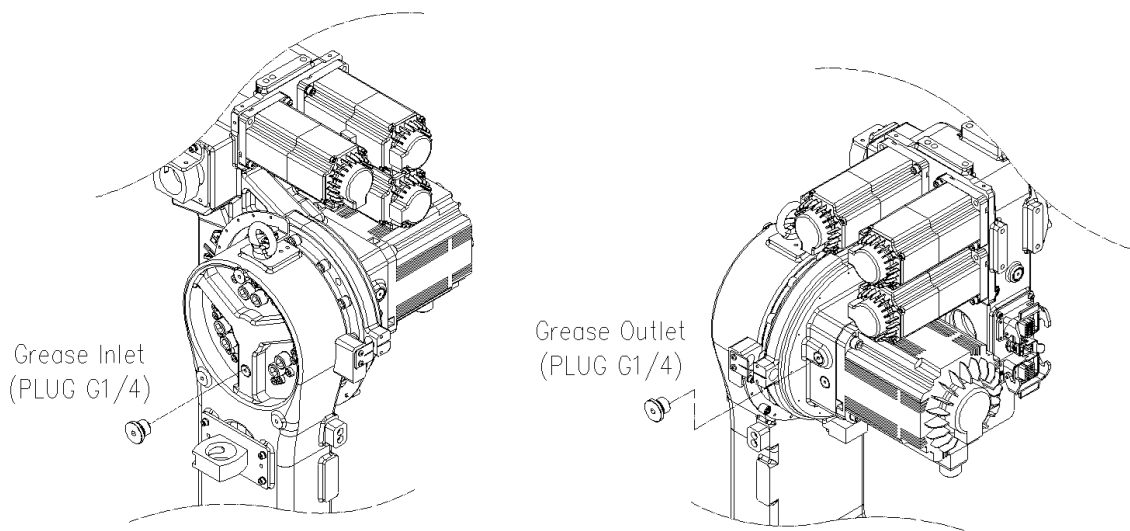
图 5.3 V 轴减速机润滑脂注入/排油口
