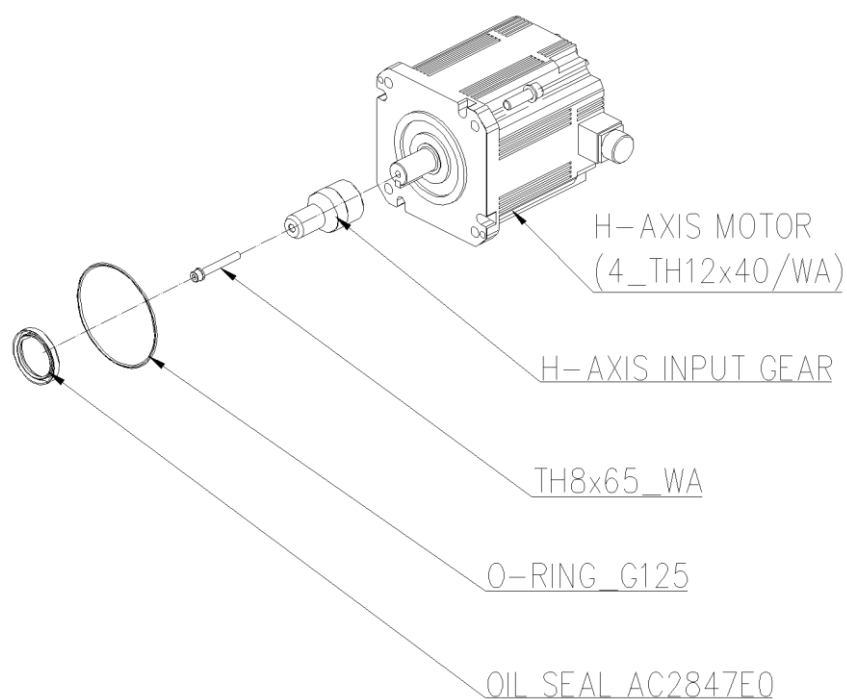
图 6.2 H 轴电机安装
