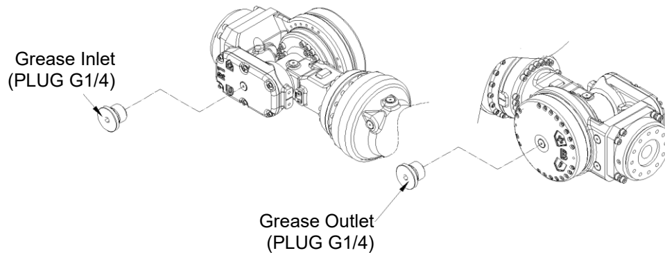
图 5.6 B 轴减速机润滑油注入/排油口(YS140)
