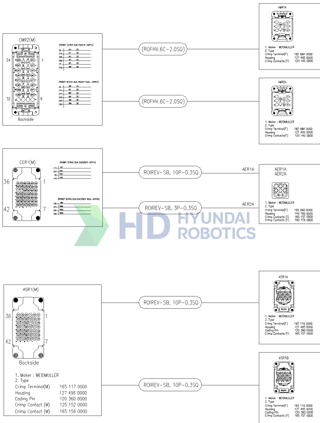
图 2.11 应用连接器细节: [YS080L/YS140]
