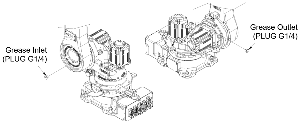
图 5.2 H 轴减速机润滑油加注/排油口
