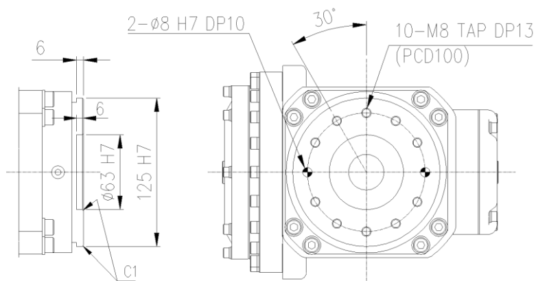
图 2.6 机械腕轴连接面细节: [YS080L]
