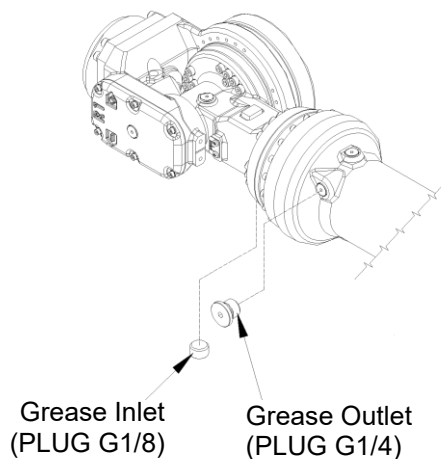
图 5.4 R2 轴减速机润滑油注入/排油口
