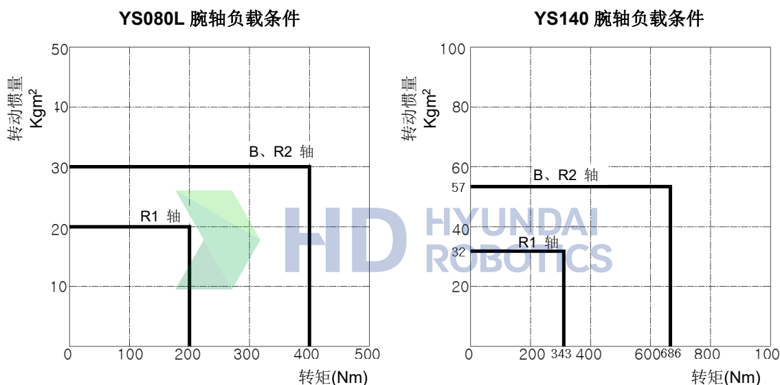
图 3.10 腕轴负载条件: [YS080L/YS140]
