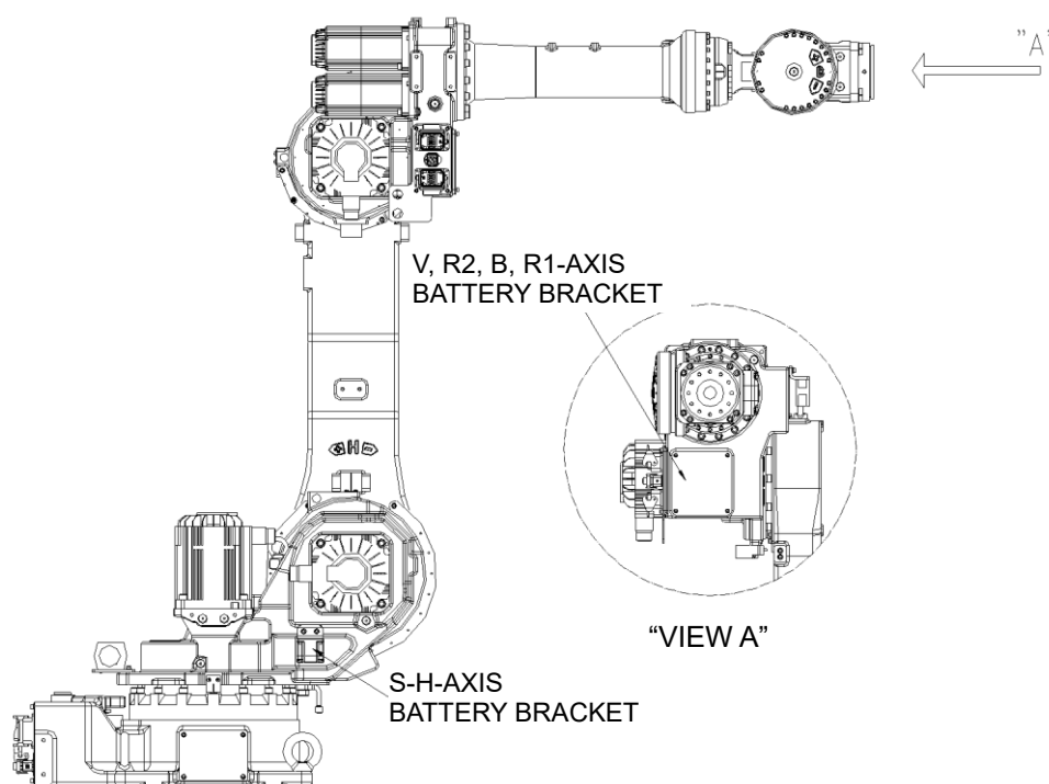
图 5.9 电池的位置
