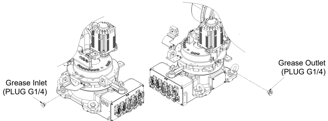
图 5.1 S 轴减速机润滑油加注/排油口
