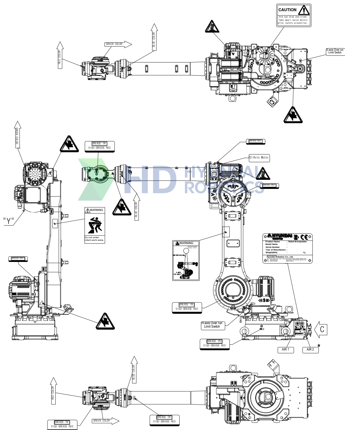
图 3.2 安全标识牌位置 [YS080L/YS140]
