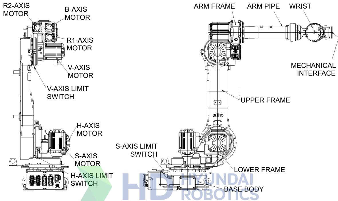
图 3.1 机器人零件名称 [YS080L/YS140]
