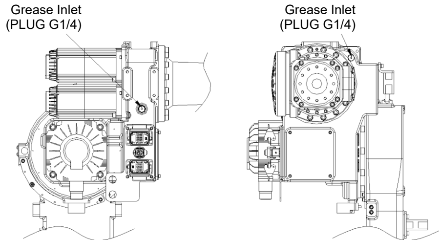
图 5.8 Arm Frame 润滑油注入/排油口
