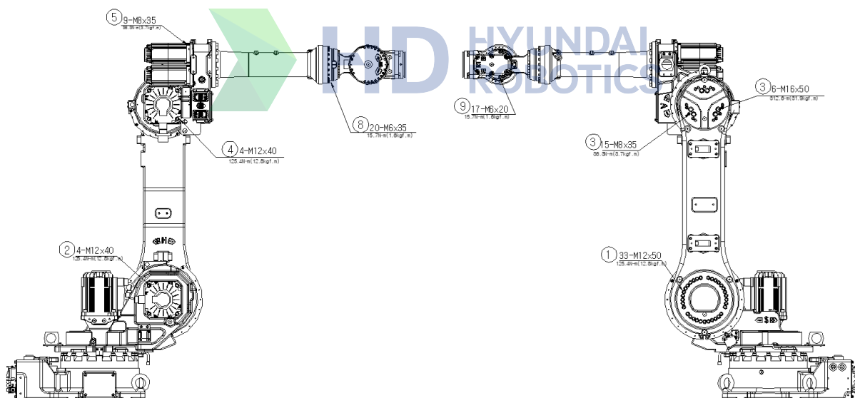
图 4.1 主要螺栓的检查部位 [YS080L/YS140]
