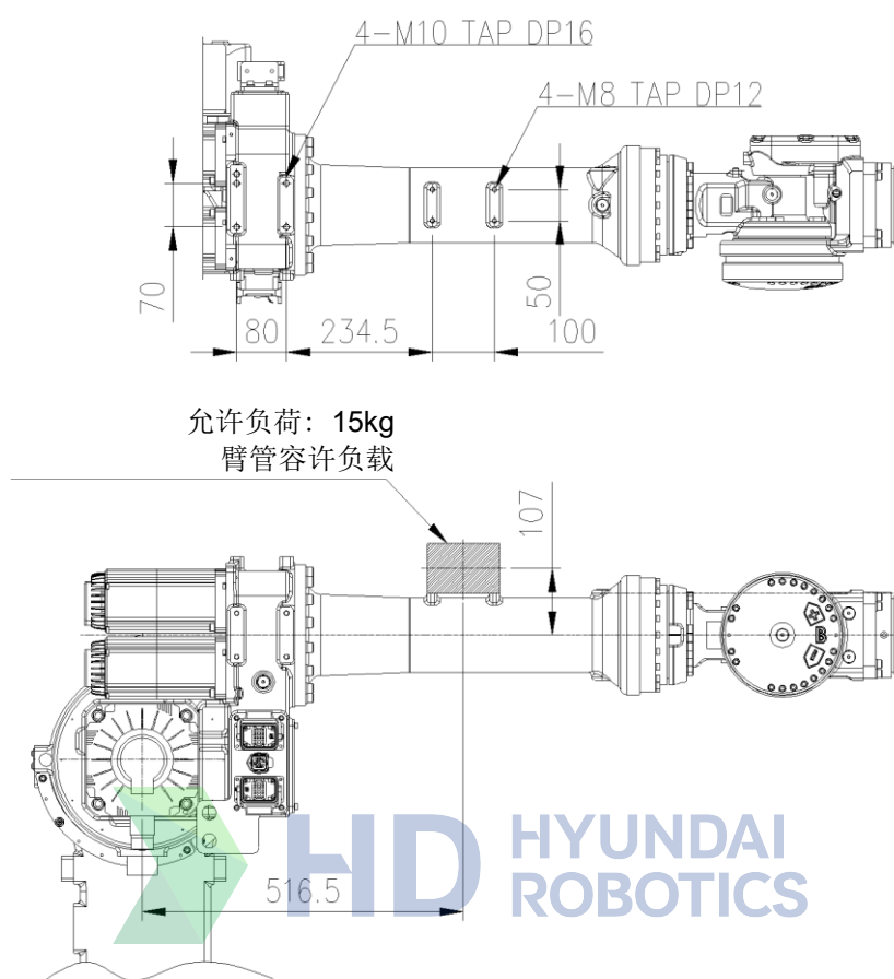
图 2.9 上机械臂支撑连接面细节: [YS140]
