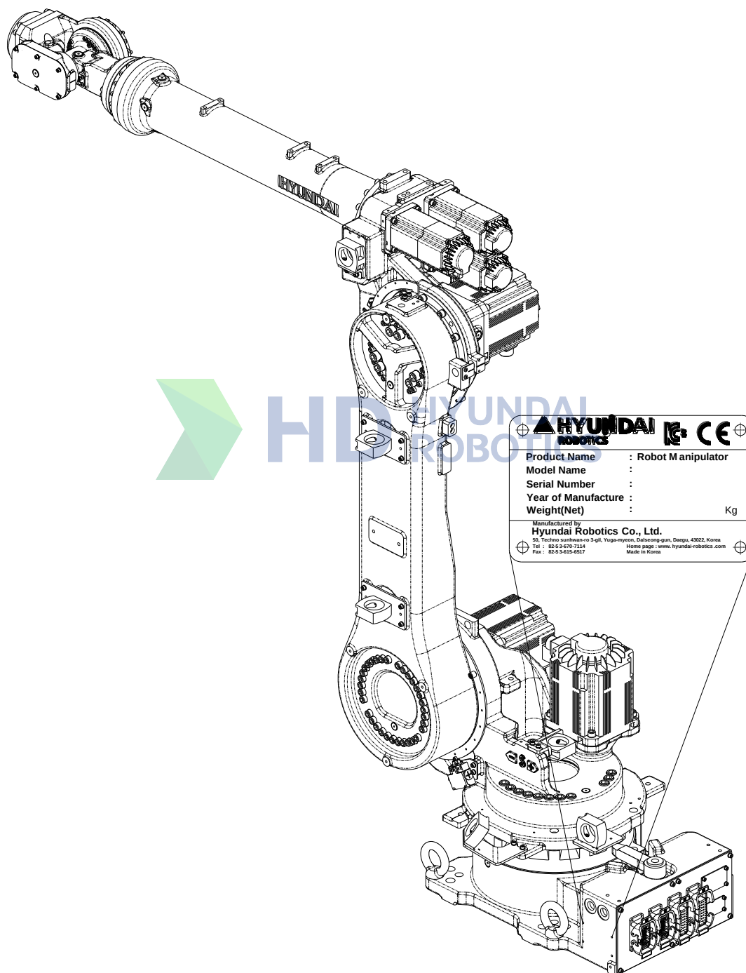
图 2.2 机器人识别铭牌的位置
