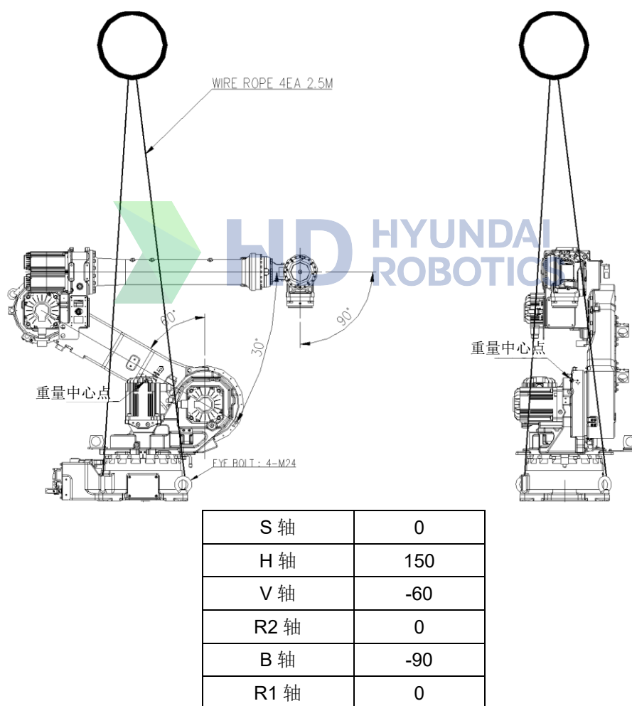
图 3.4 运送方法: 使用吊车
