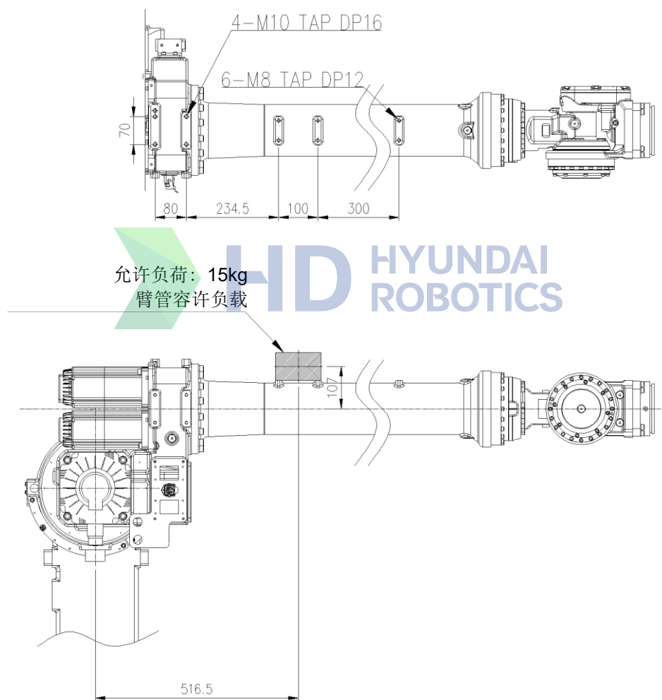
图 2.8 上机械臂支撑连接面细节: [YS080L]
