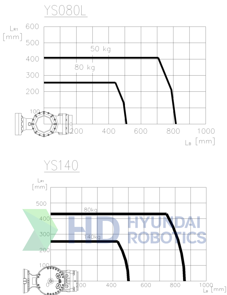
图 3.9 腕轴转矩图: [YS080L/YS140]
