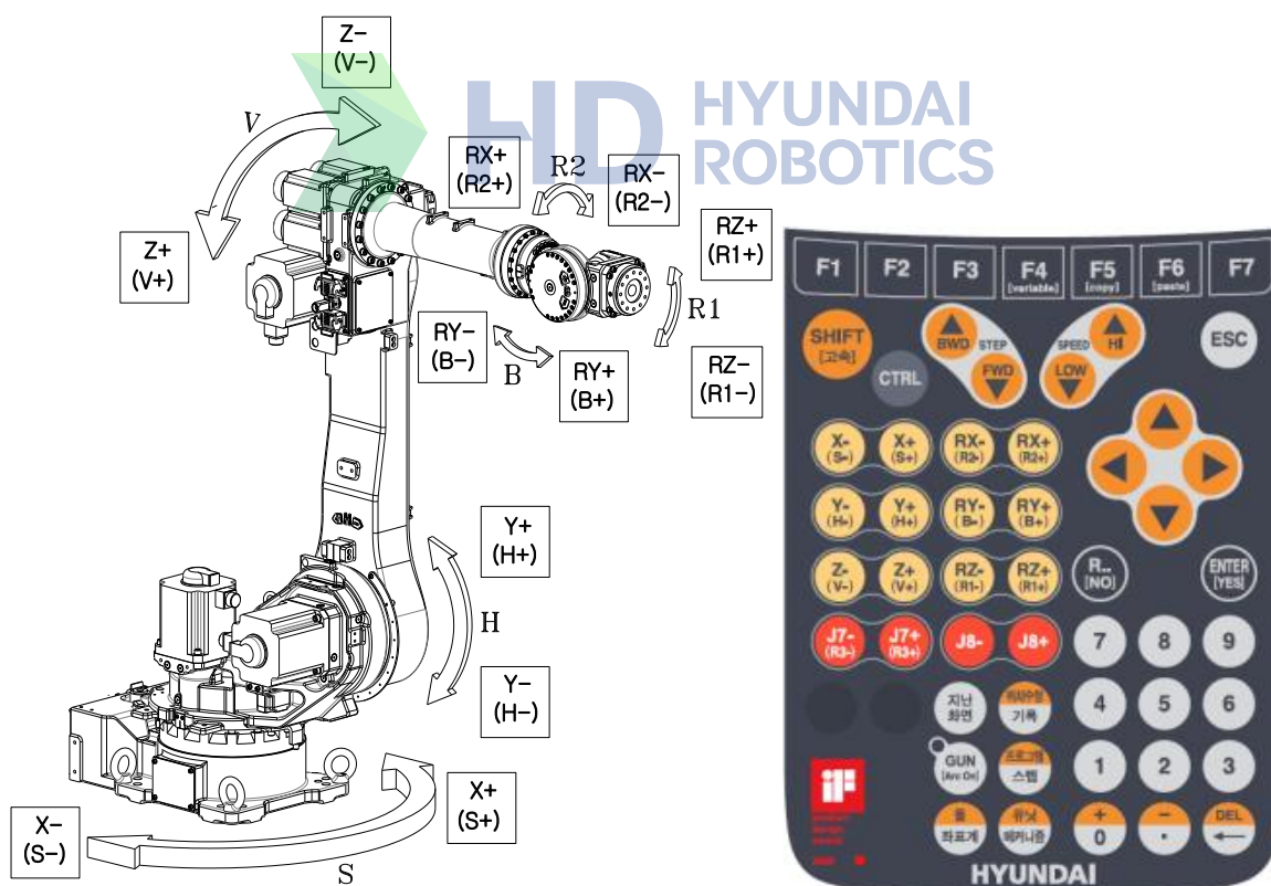
图 2.5 机器人尺寸和轴 [YS080L/YS140]
