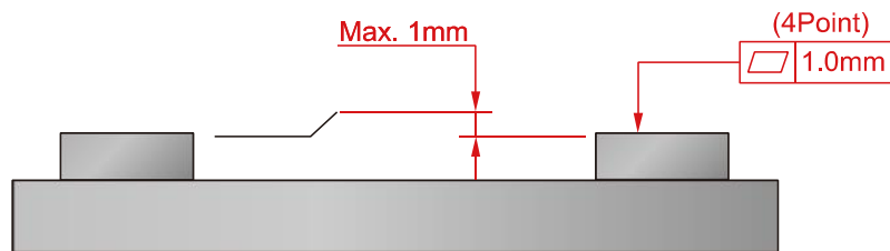
图 3.6 安装面精确度
