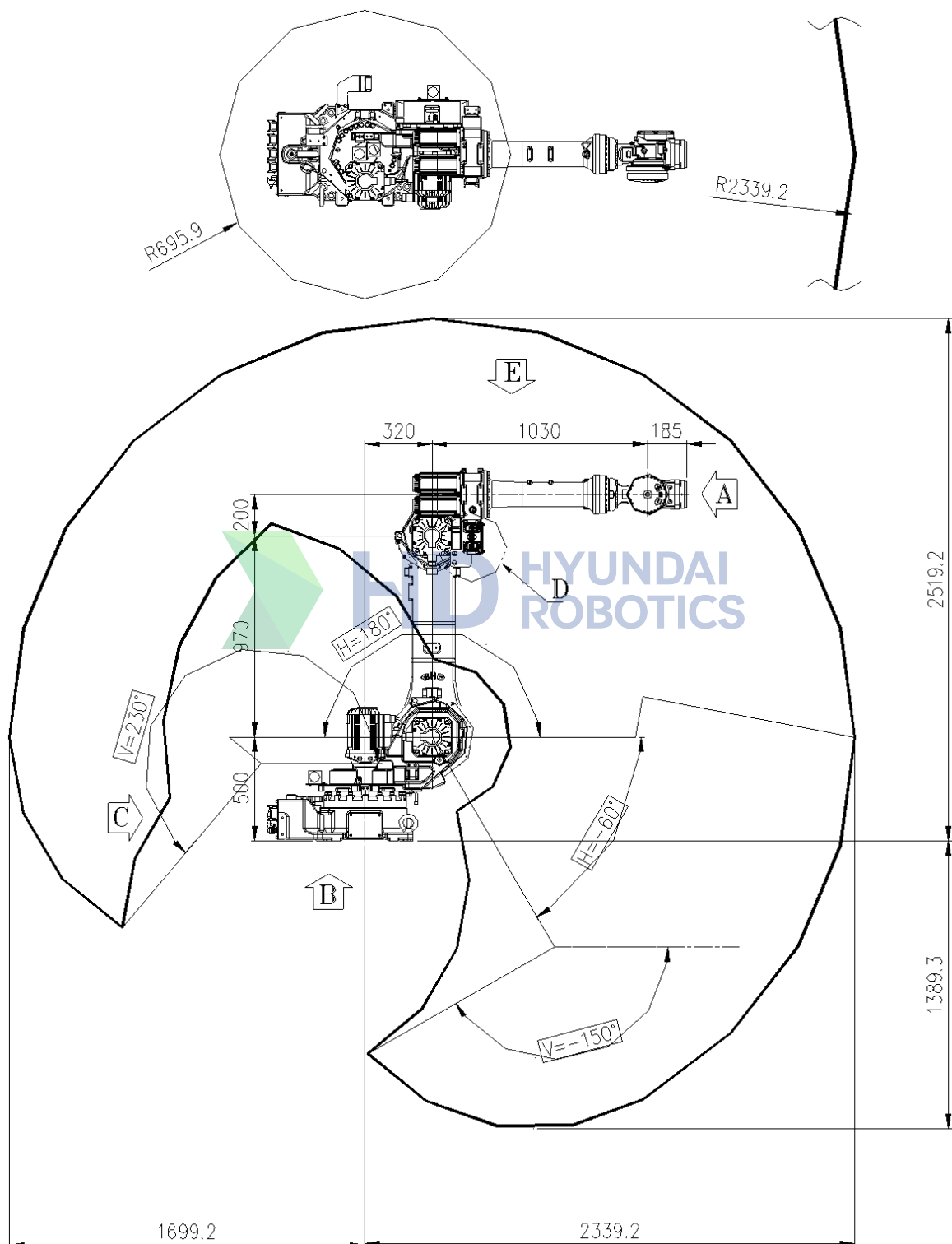
图 2.3 机器人尺寸和工作区间 [YS080L]
