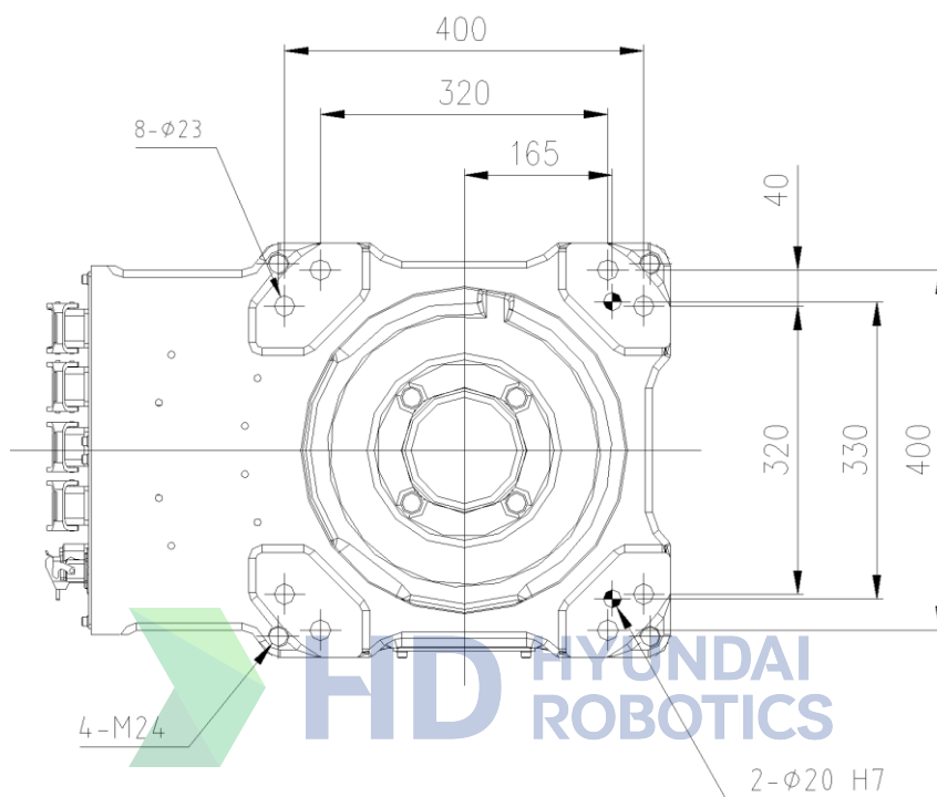
图 3.7 机器人安装尺寸[YS080L/YS140]
