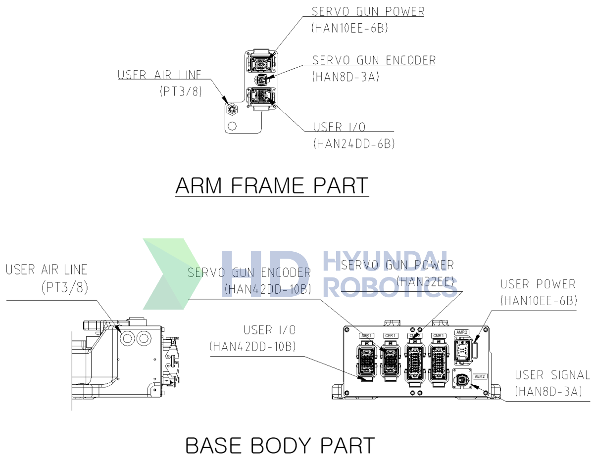
图 2.10 工作线路和检查线路图: [YS080L/YS140]
