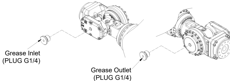
图 5.5 B 轴减速机润滑油注入/排油口(YS080L)
