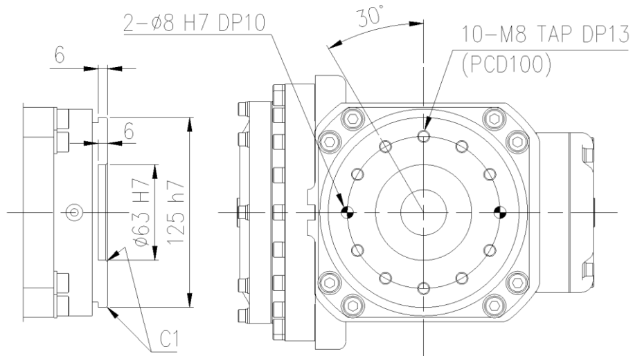
图 2.9 机械腕轴连接面细节: [YS080/YS100A/HH050/HH030L/HH050T]
