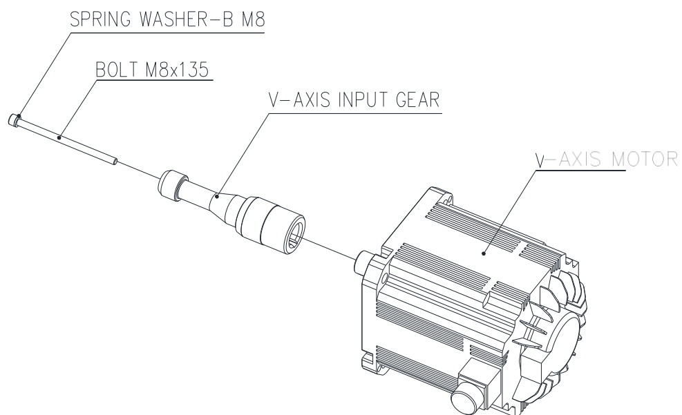
图 6.6 V 轴电机安装
