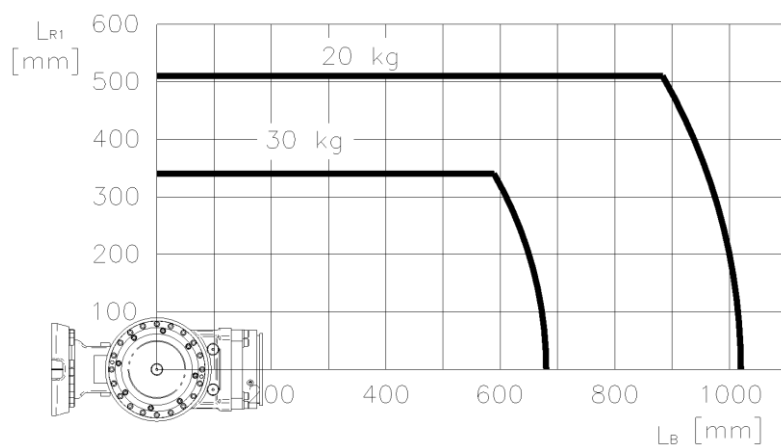
图 3.11 腕轴转矩图: [HH030L]
