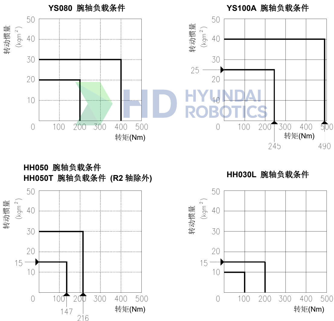
图 3.12 腕轴负载条件: [YS080/YS100A/HH050/HH030L/HH050T]
