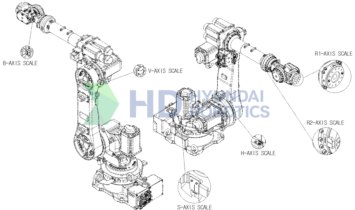
图 6.8 归零设定的方法 [YS080/YS100A/HH050/HH030L] - [HH050T-R2 轴除外]
