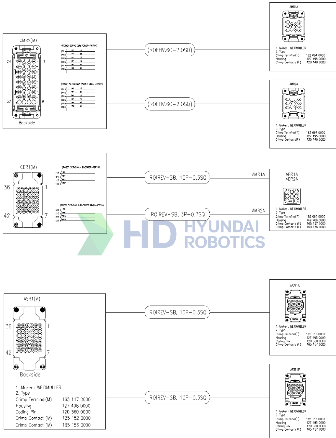
图 2.15 应用连接器细节: [YS080-11/YS100A-11/HH050-11/HH030L-11/HH050T-11]
