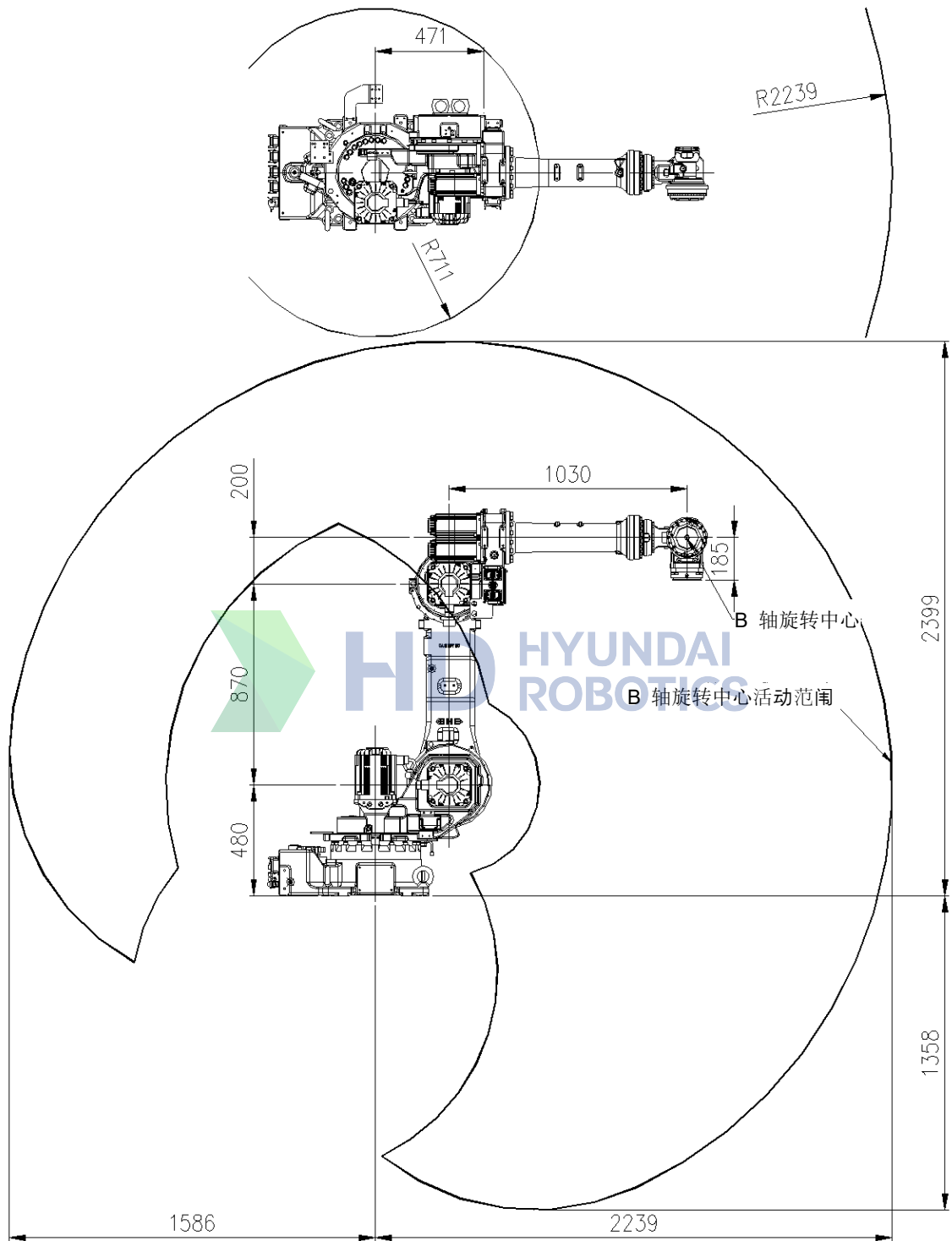
图 2.7 机器人尺寸和工作区间 [HH050T-11]
