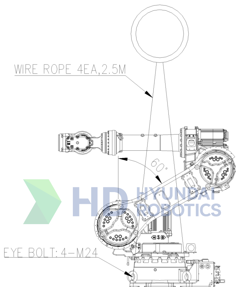
图 3.3 运送方法: 使用吊车 [YS080/YS100A/HH050/HH030L/HH050T]
