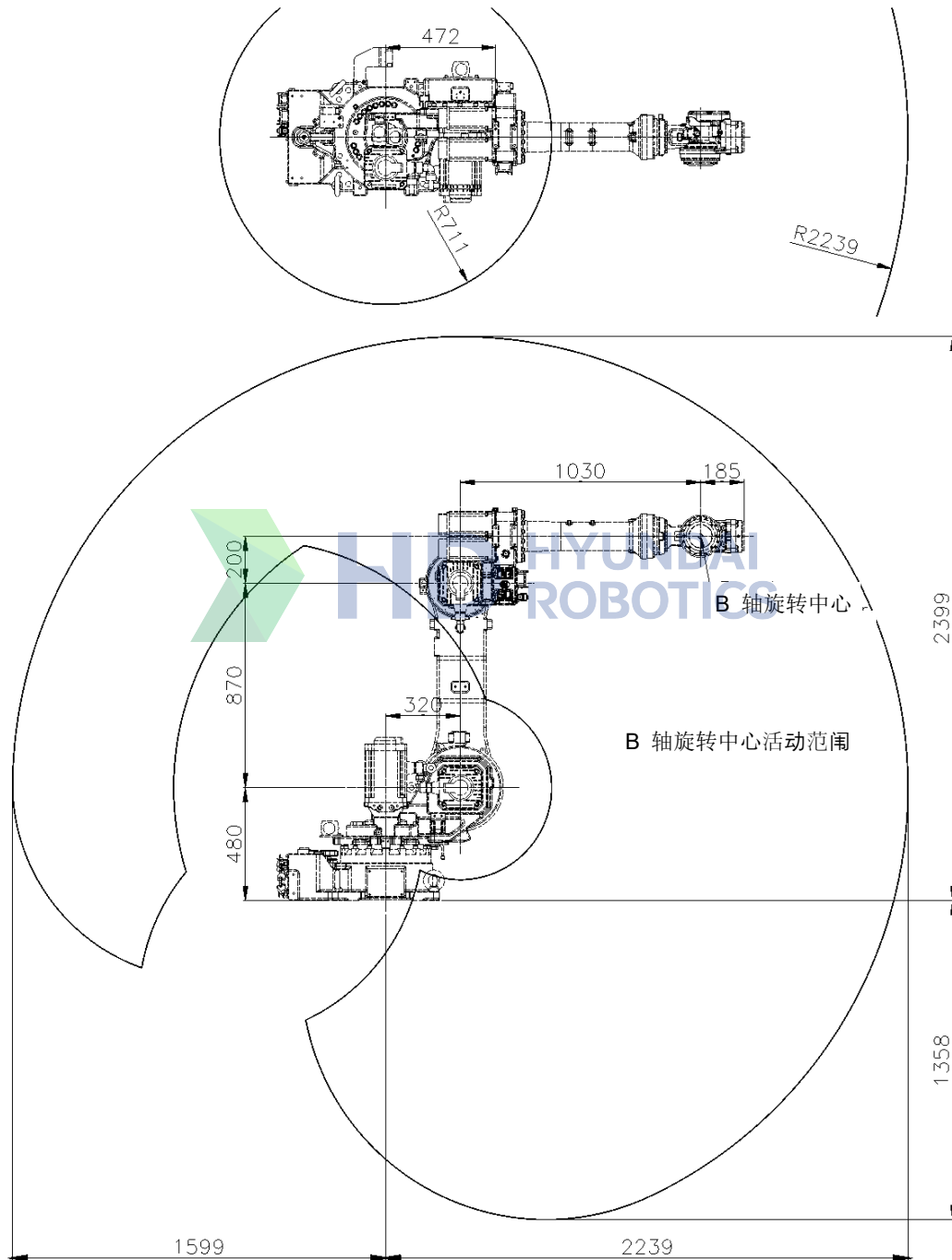
图 2.3 机器人尺寸和工作区间: [YS080/YS100A/HH050]
