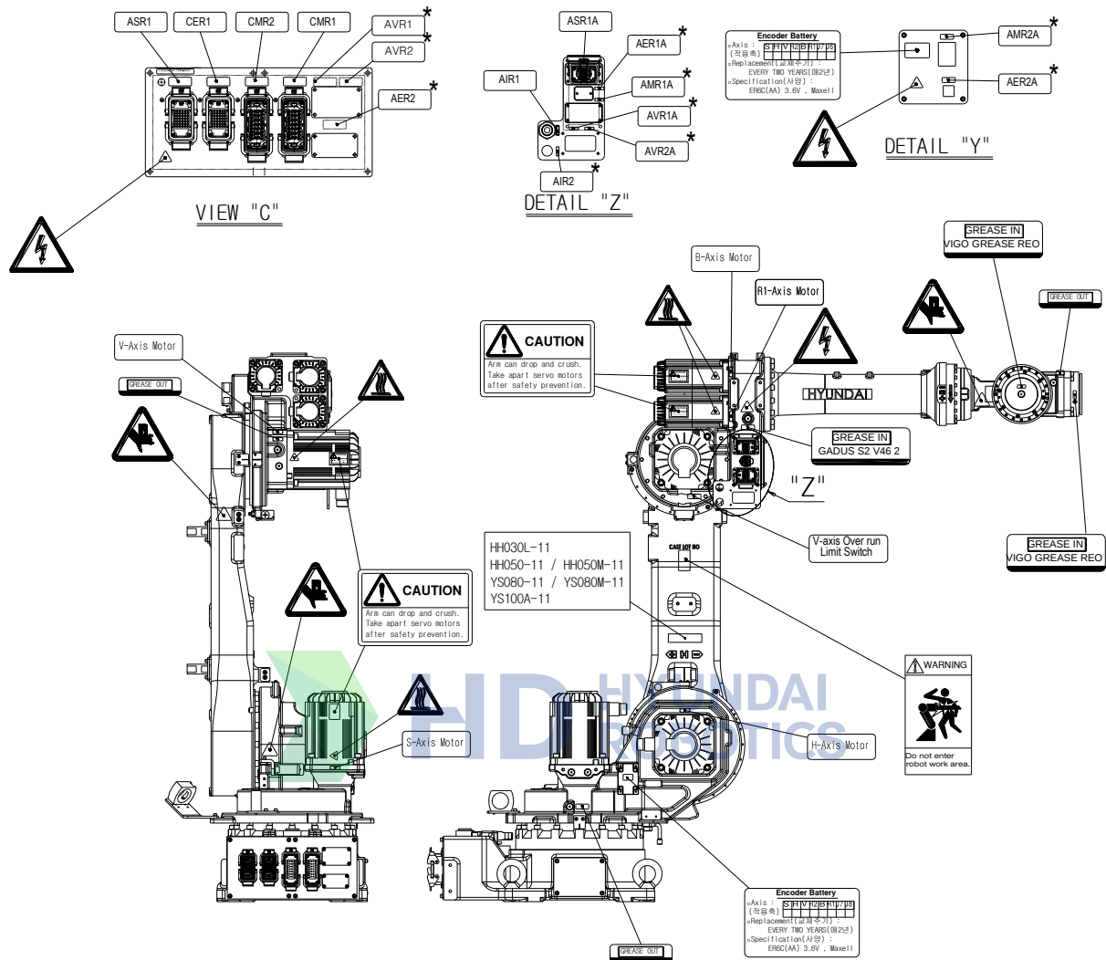
图 3.2 安全标识牌位置
