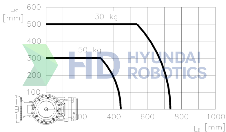
图 3.10 腕轴转矩图: [HH050/HH050T]
