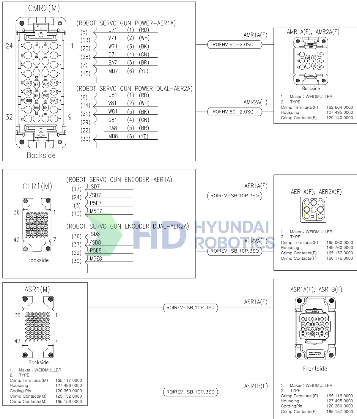
图 2.13 应用连接器细节: [YS080/YS100A/HH050/HH030L]
