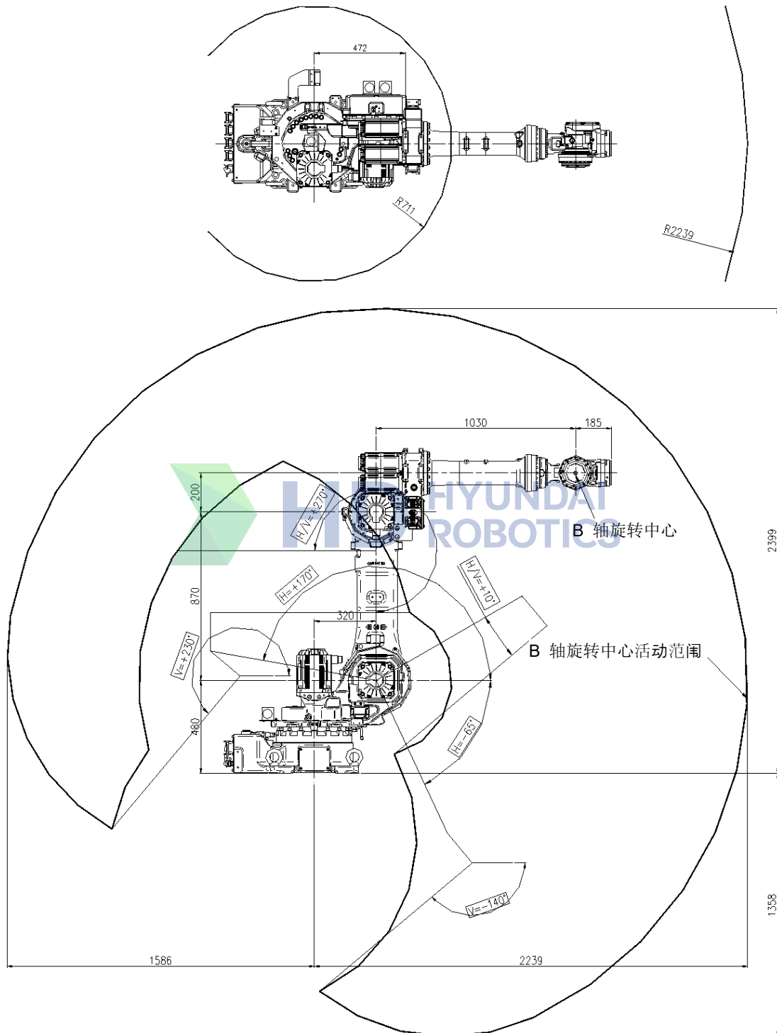
图 2.5 机器人尺寸和工作区间 [YS080-11/YS100A-11/HH050-11]
