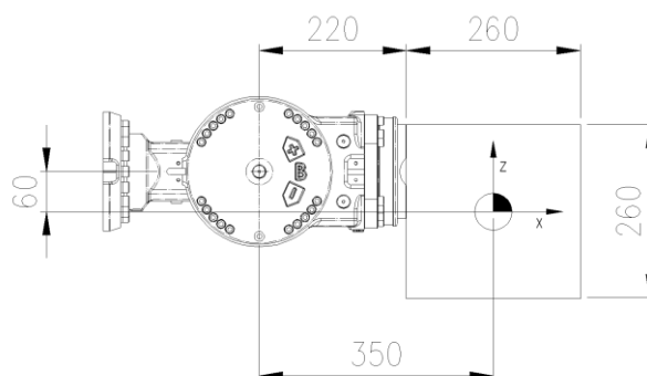
图 3.13 2-D 负载模型
