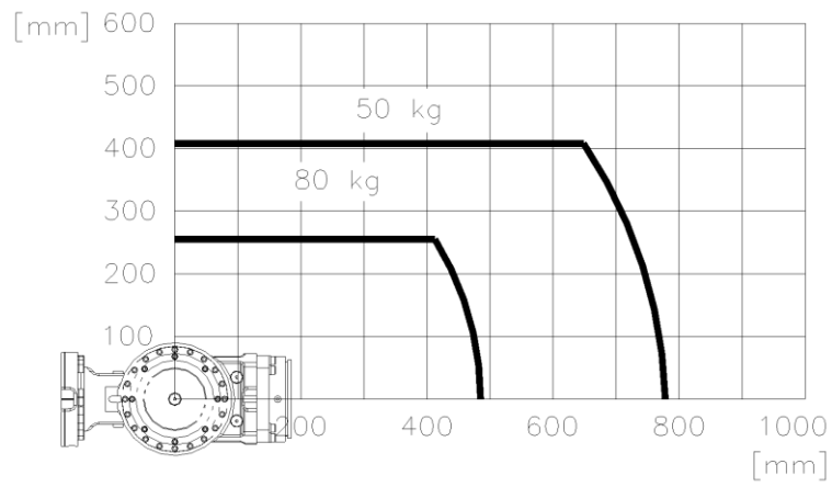
图 3.8 腕轴转矩图: [YS080]
