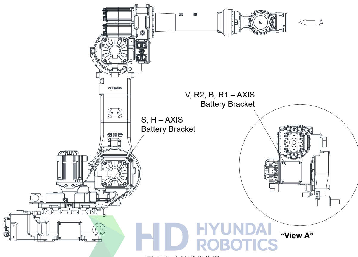
图 5.1 电池替换位置
