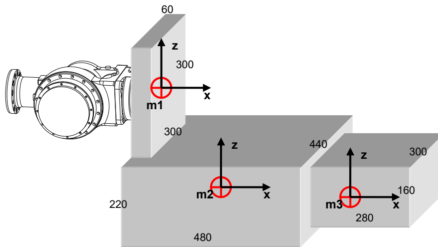
图 3.15 3-D 负载模型 3-D 形状
