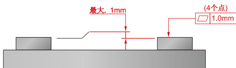
图 3.5 机器人安装面程度
