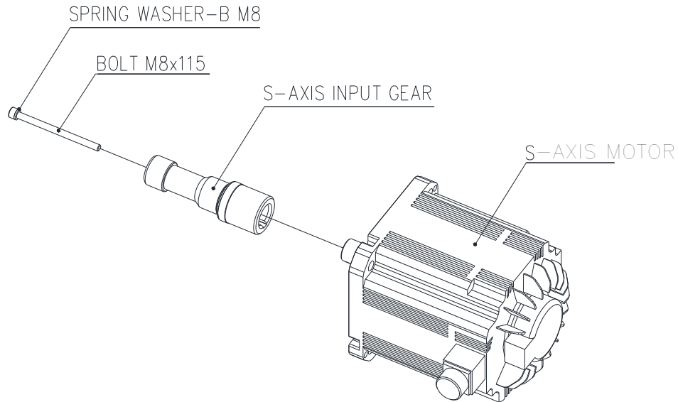
图 6.4 S 轴电机安装
