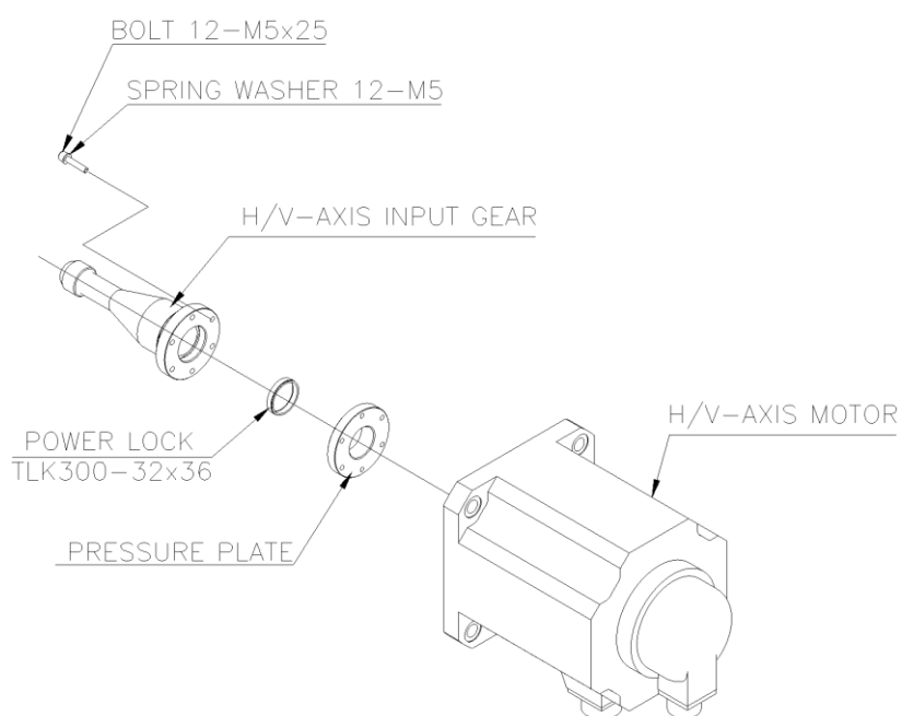
图 6.3 H&amp;V 轴电机安装
