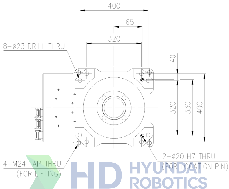
图 3.6 机器人安装尺寸: [YS080/YS100A/HH050/HH030L/HH050T]
