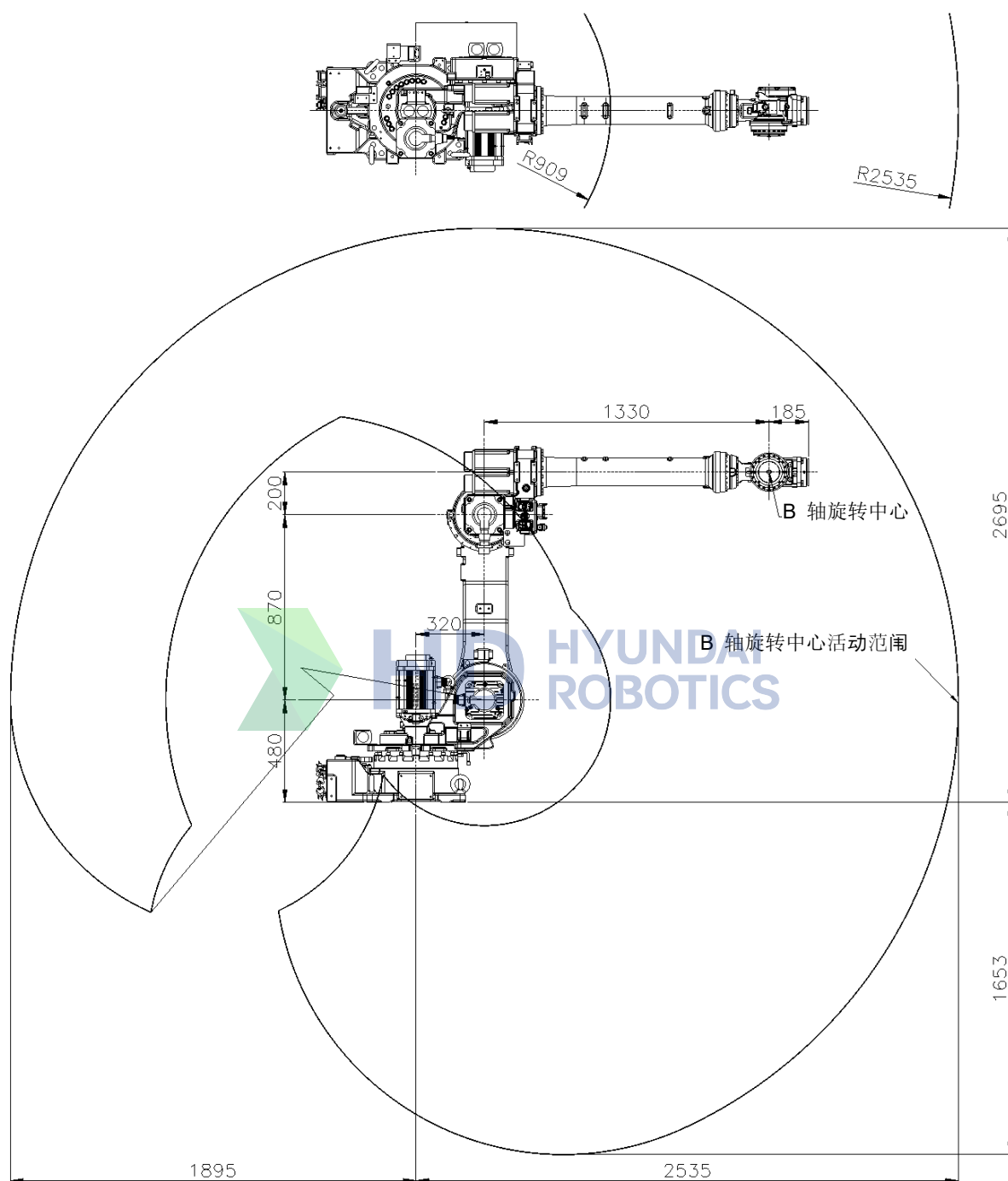
图 2.4 机器人尺寸和工作区间: [HH030L]
