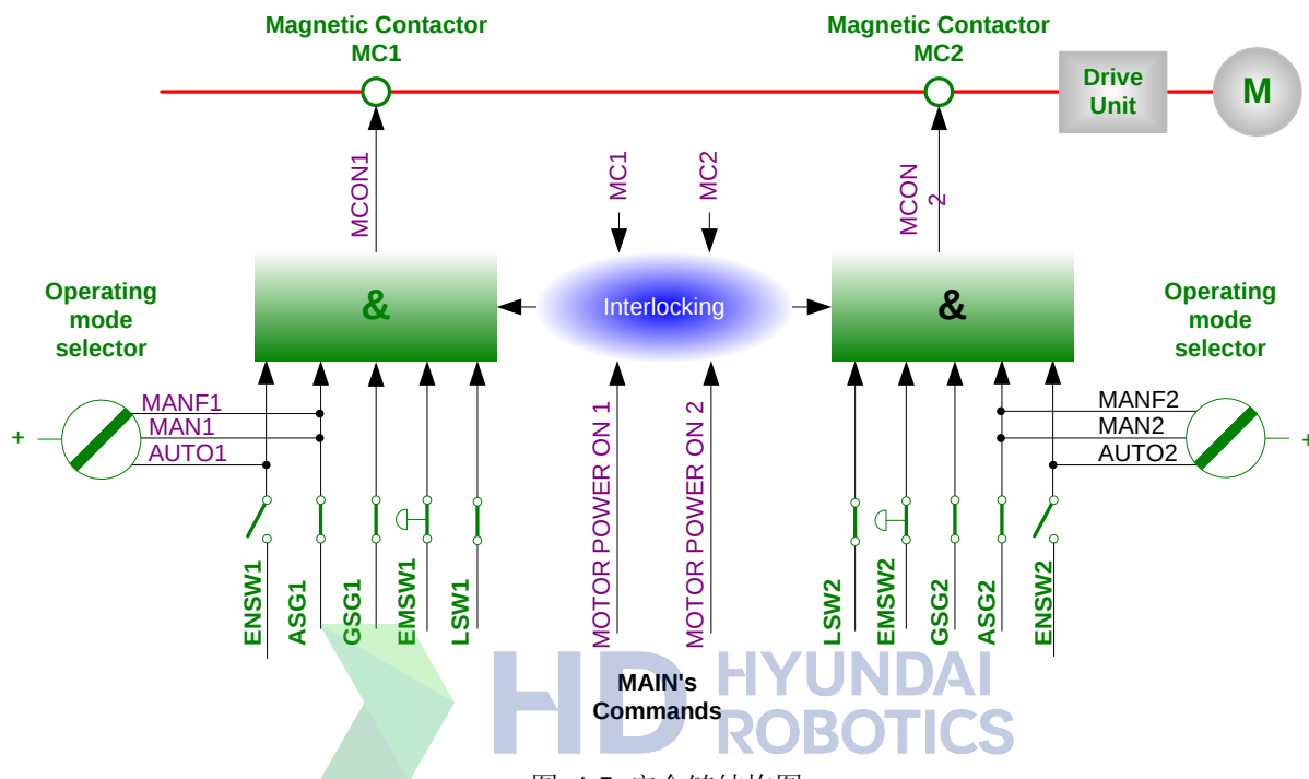
图 1.5 安全链结构图
