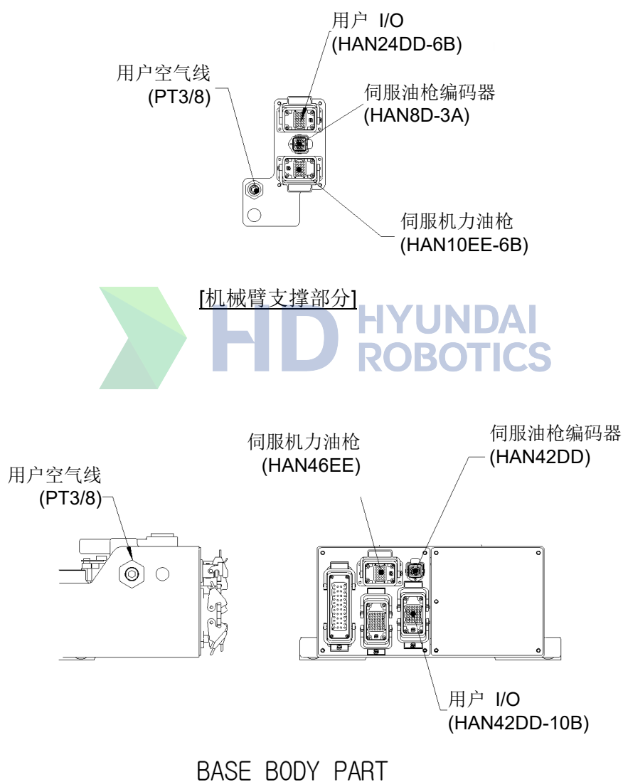
图 2.12 工作线路和检查线路图: [YS080/YS100A/HH050/HH030L]
