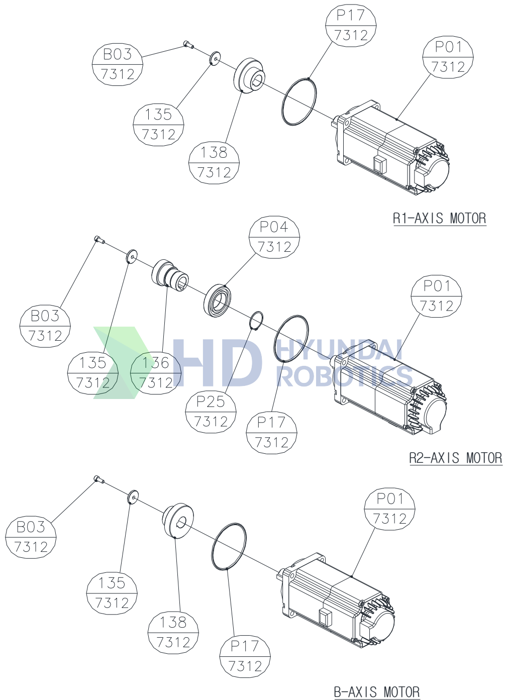
图 6.7 腕轴电机安装-R2 轴电机除外(HH050T)
