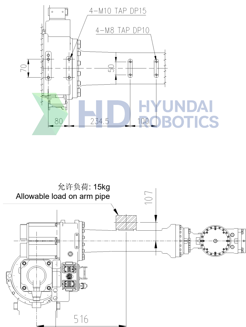
图 2.10 上机械臂支撑连接面细节: [YS080/YS100A/HH050/HH050T]
