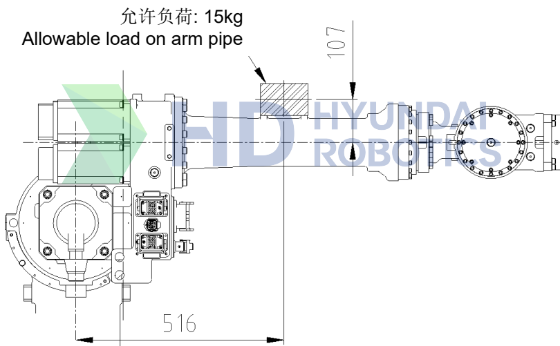
图 2.11 上机械臂支撑连接面细节: [HH030L]
