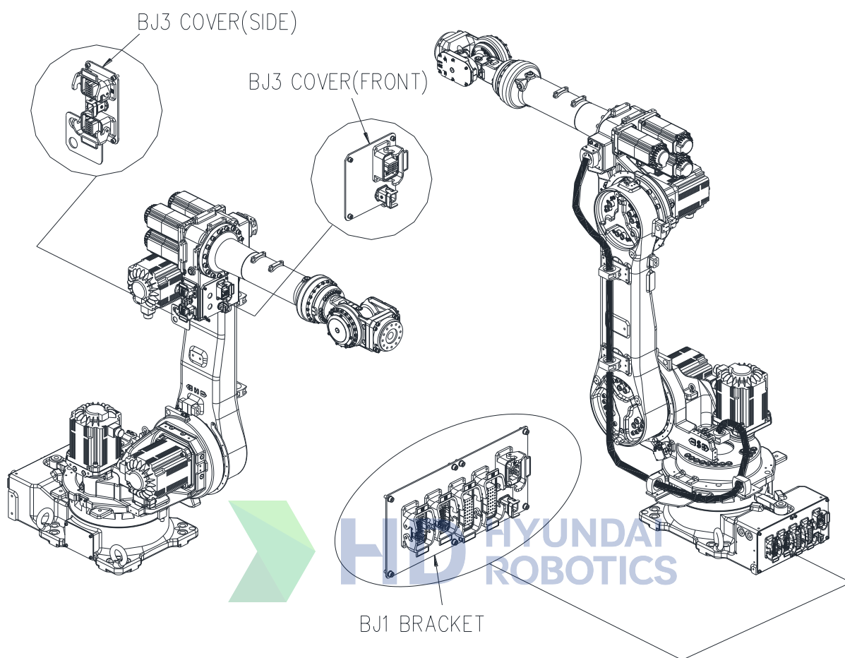
图 9.1 机体配件布置
