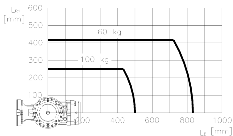
图 3.9 腕轴转矩图: [YS100A]
