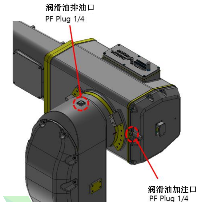
图 5.3 V 轴润滑油加注/排油口
