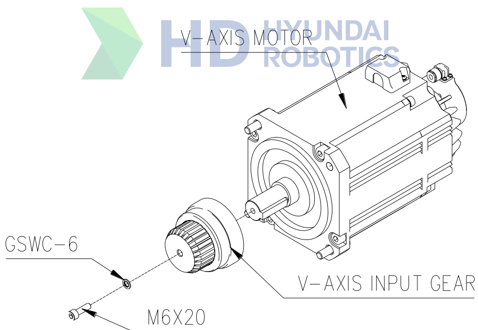
图 6.4 V 轴电机安装
