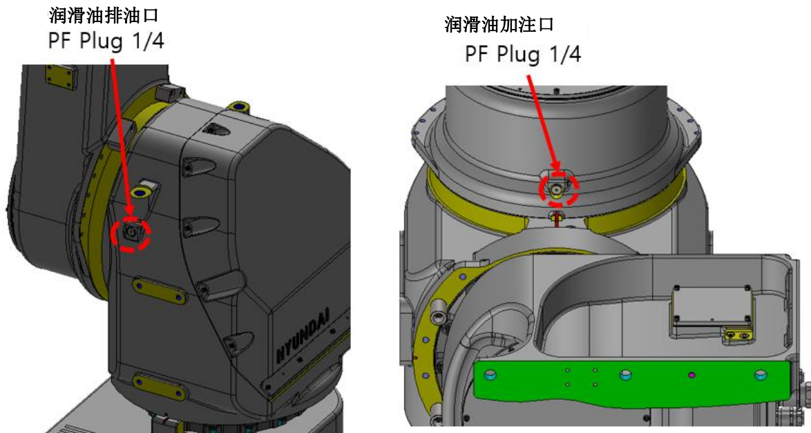
图 5.2 H 轴润滑油加注/排油口
