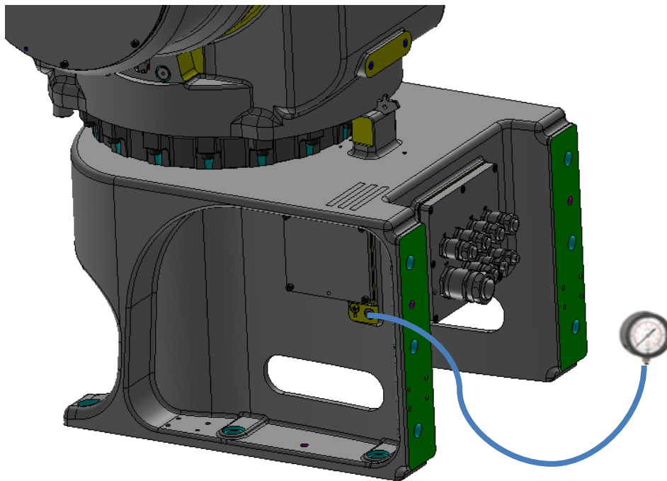
图 6.1 试验用端口
