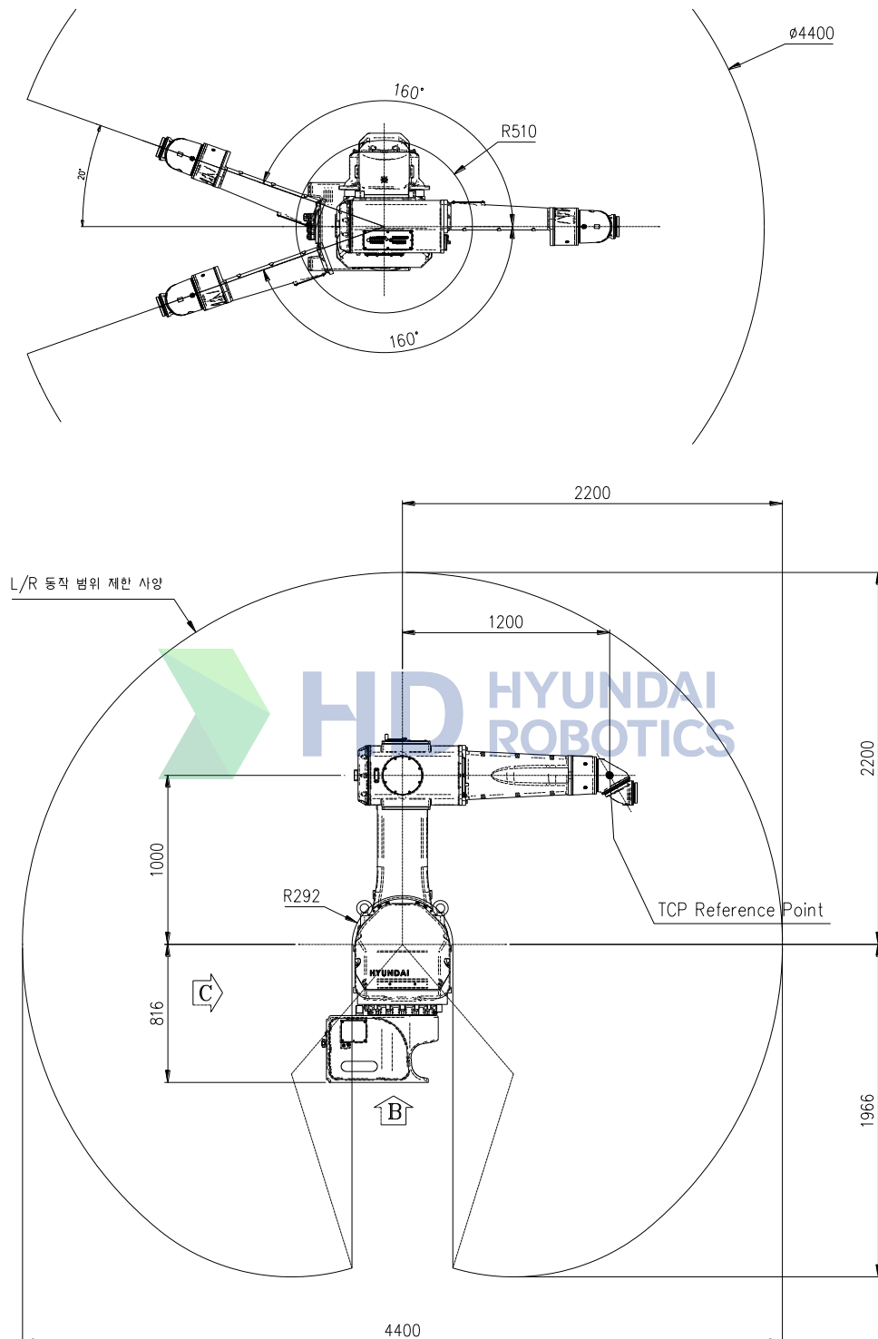
图 2.4 机器人尺寸和工作区间 (YP015A-22)
