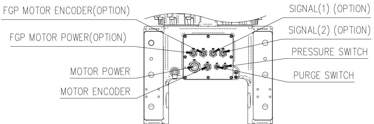
图 2.13 气压及电源接线: [Standard]
