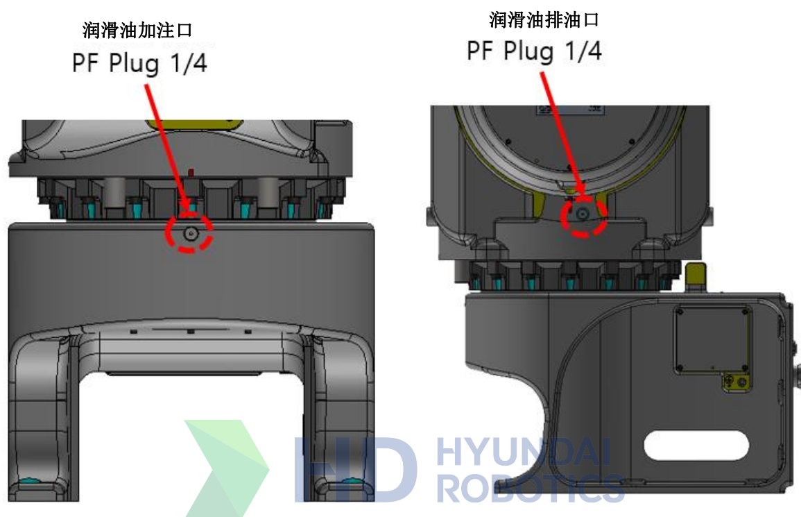
图 5.1 S 轴润滑油加注/排油口
