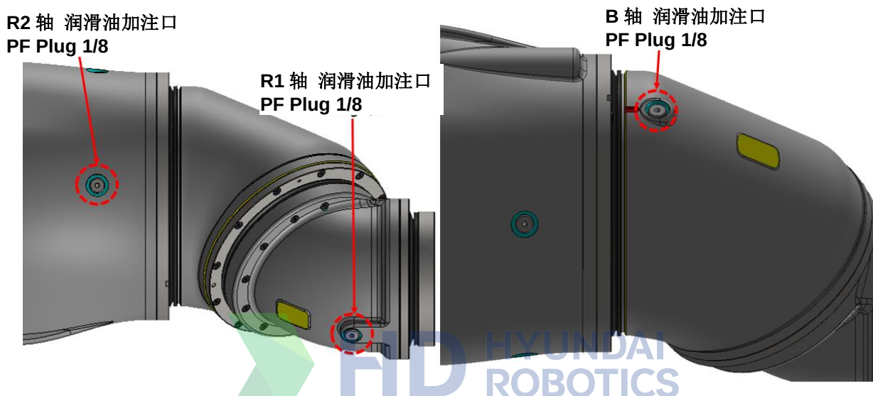
图 5.4 R2, B, R1 轴润滑脂注入口/排出口位置
