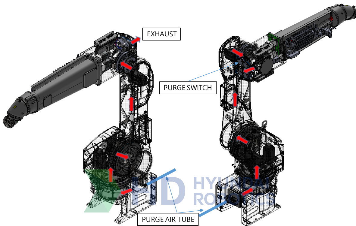
图 2.8 吹扫流程详图
