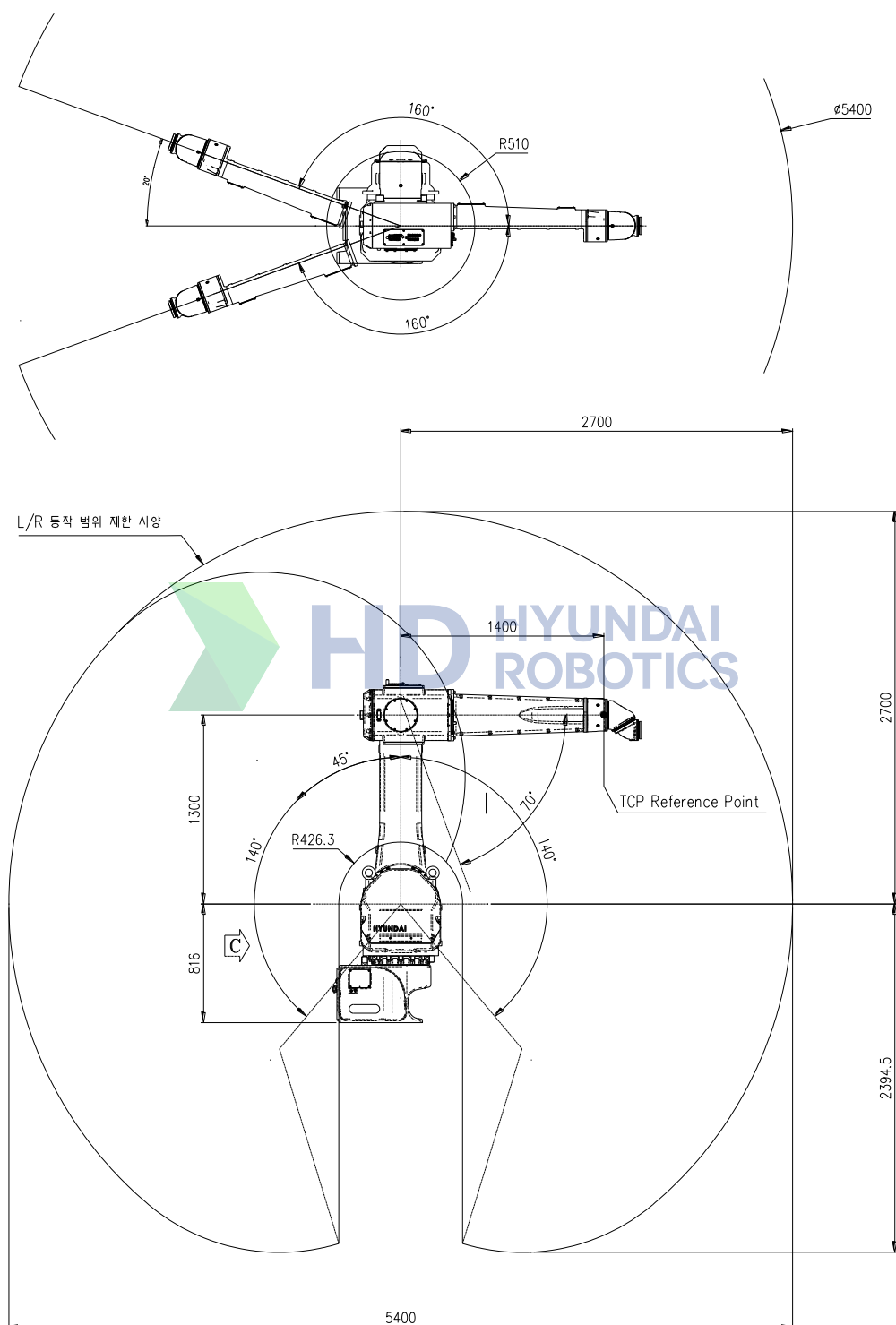
图 2.3 机器人尺寸和工作区间 (YP015A-28)
