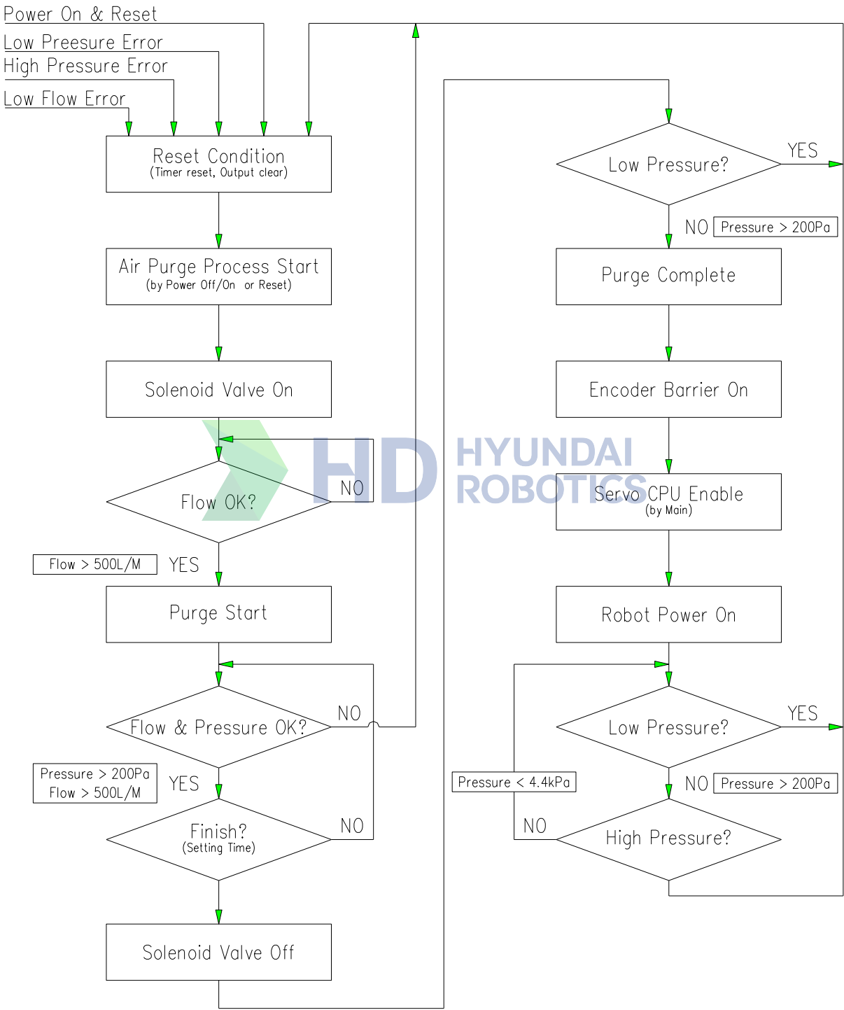
图 2.11 吹扫流程图
