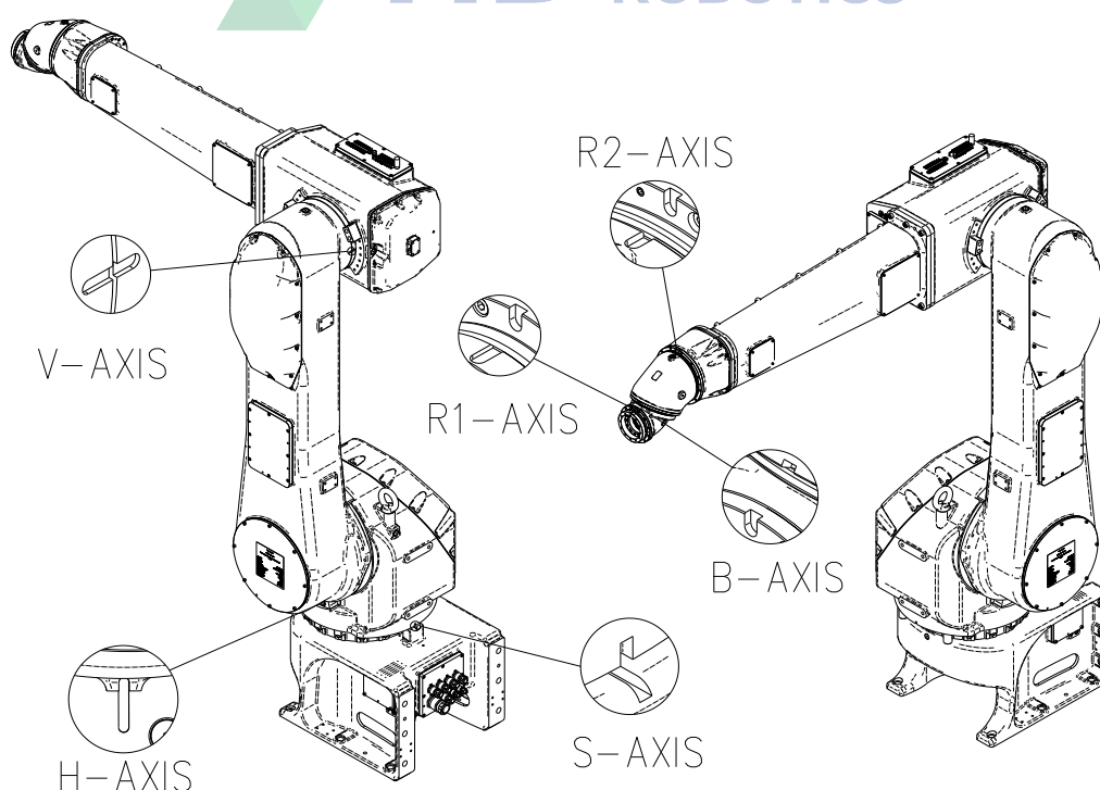
图 6.6 归零设定的 位置
