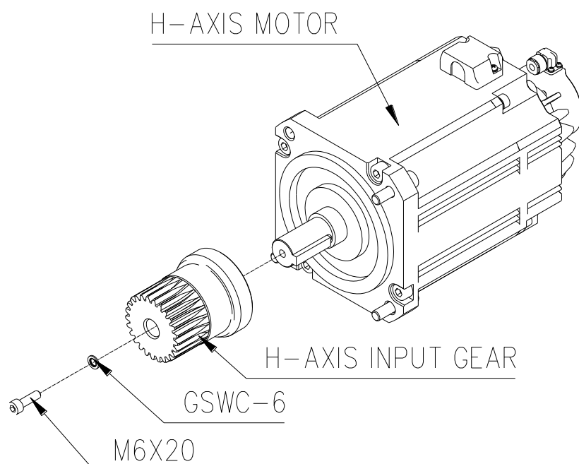
图 6.3 H 轴电机安装
