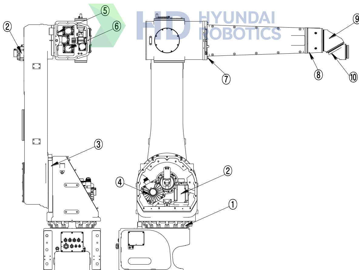
图 4.1 主要螺栓的检查部位
