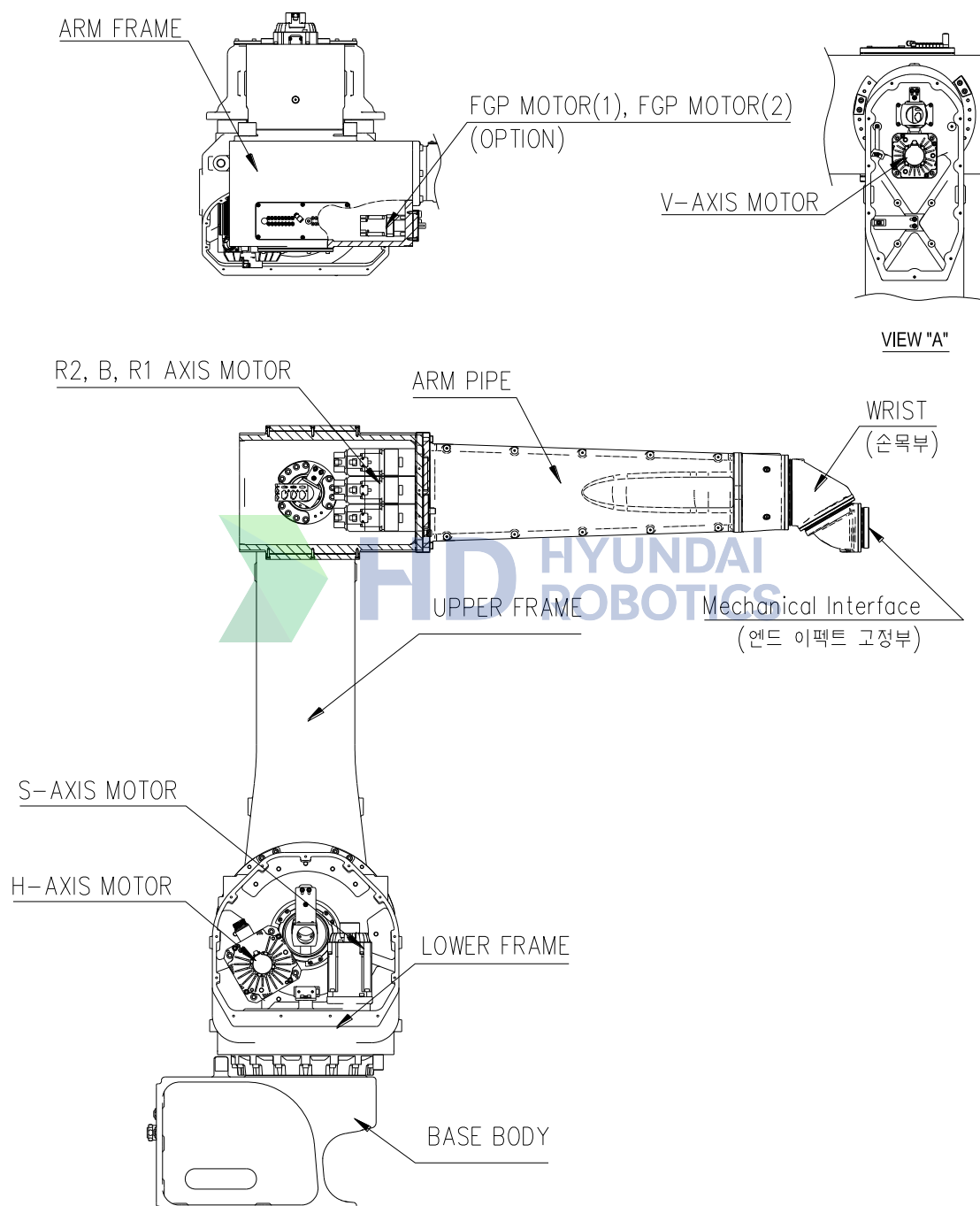
图 3.1 机器人零件名称
