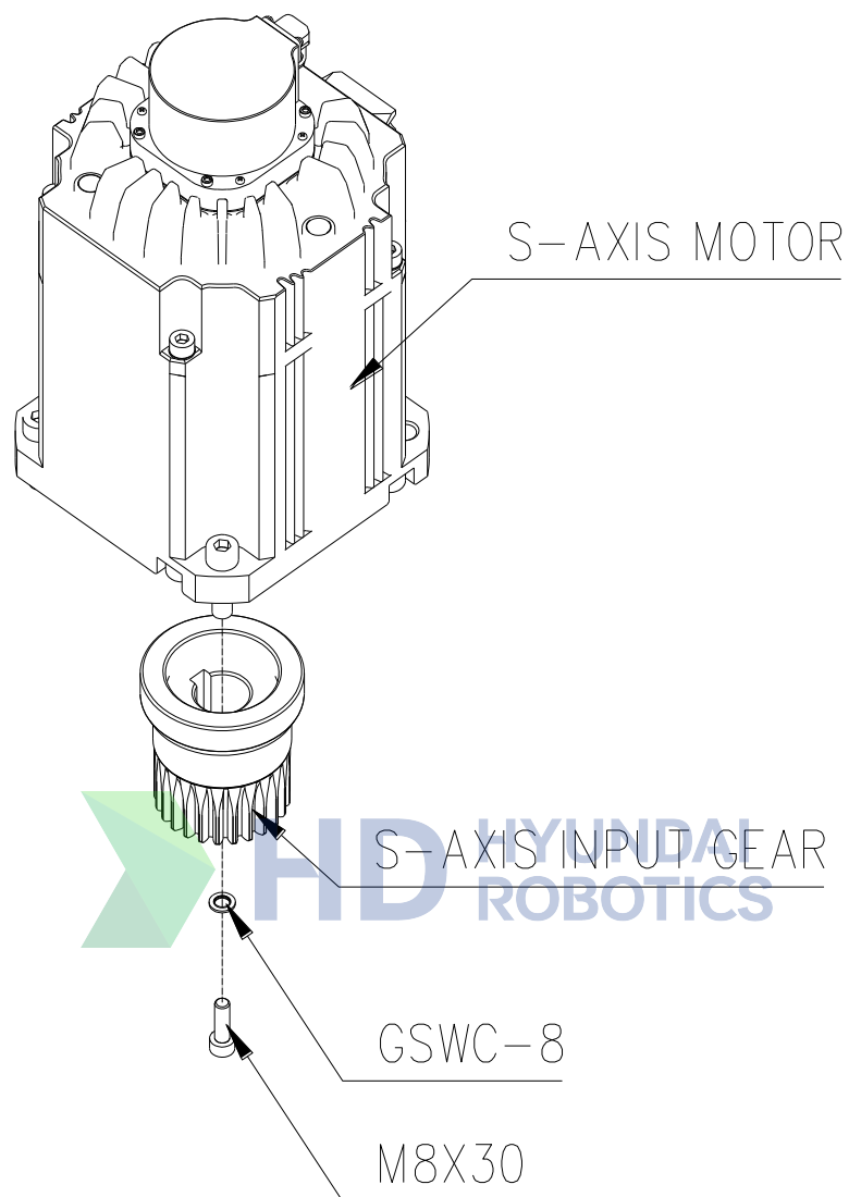
图 6.2 S 轴电机安装
