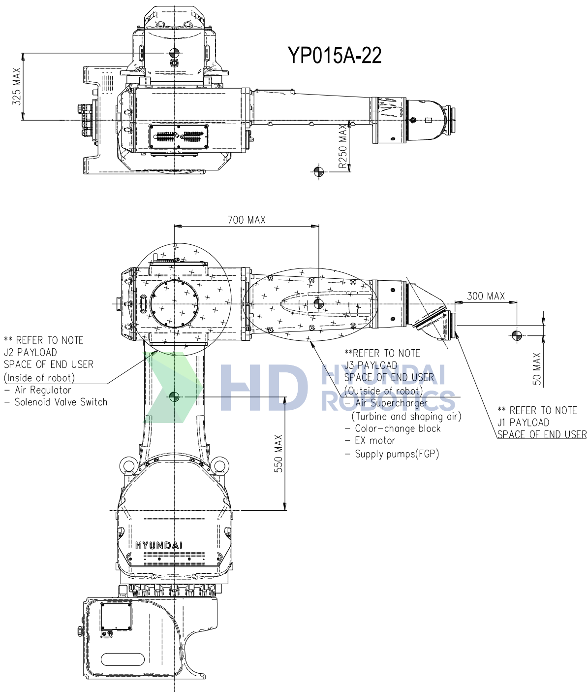
图 2.7 机械臂附着部详图
