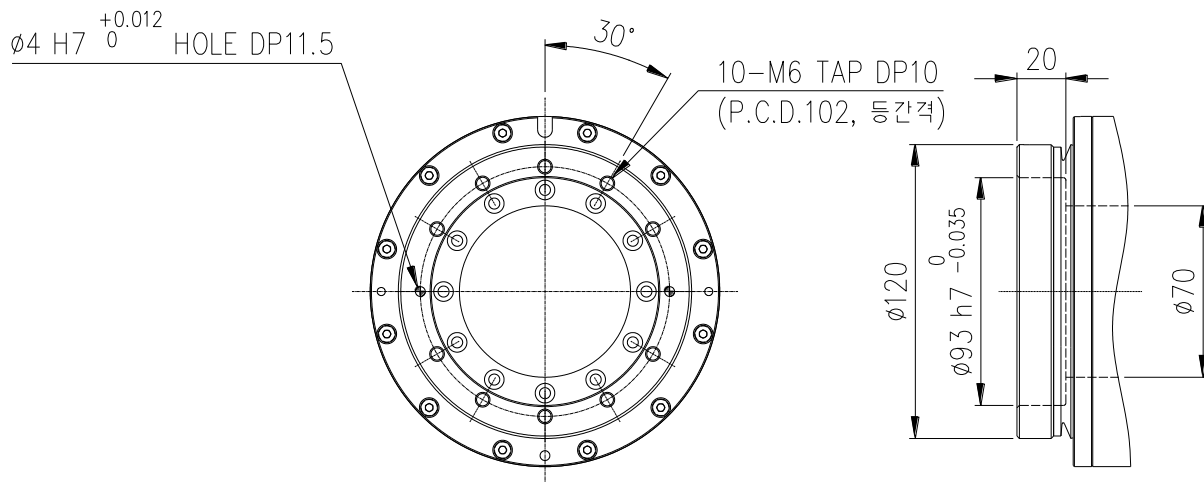
图 2.6 机械腕轴连接面细节
