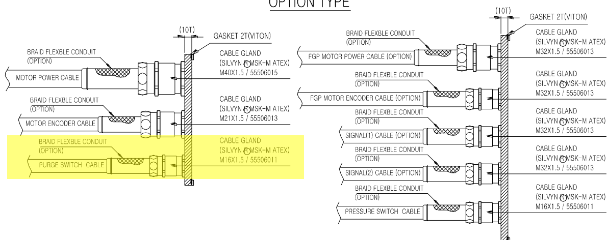
图 2.15 气压及电源
