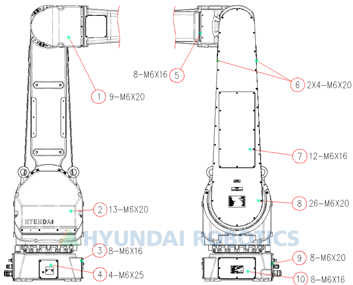
图 4.2 每个盖子部件的螺栓位置
