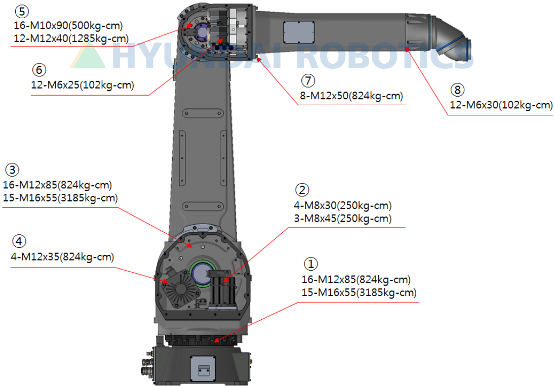
图 4.1 主要螺栓的检查部位
