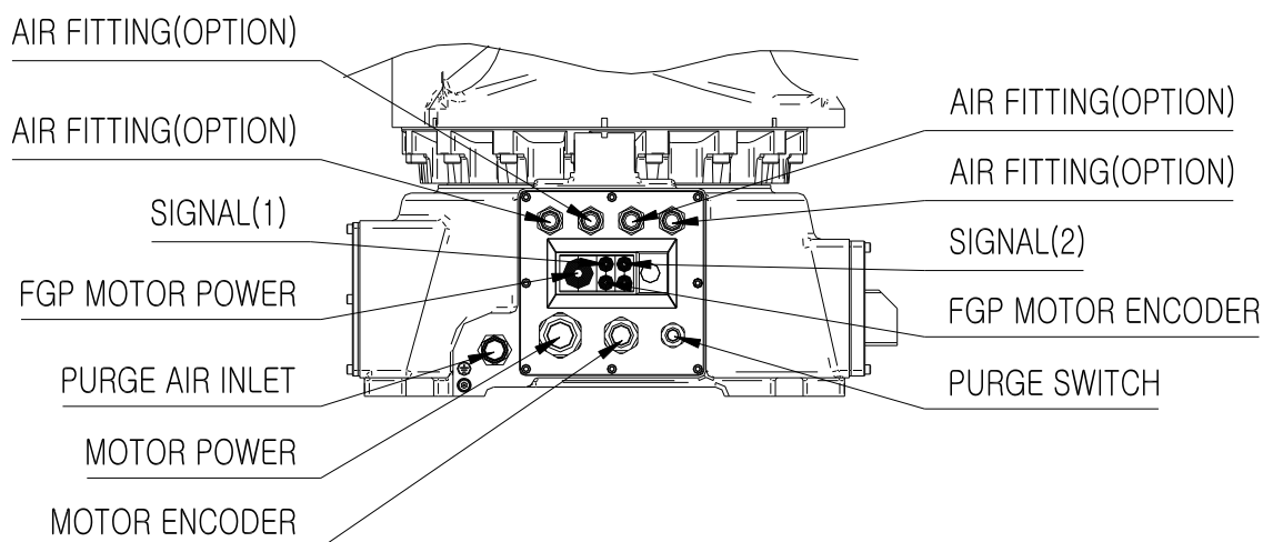
图 2.13 气压及电源接线: [Option]
