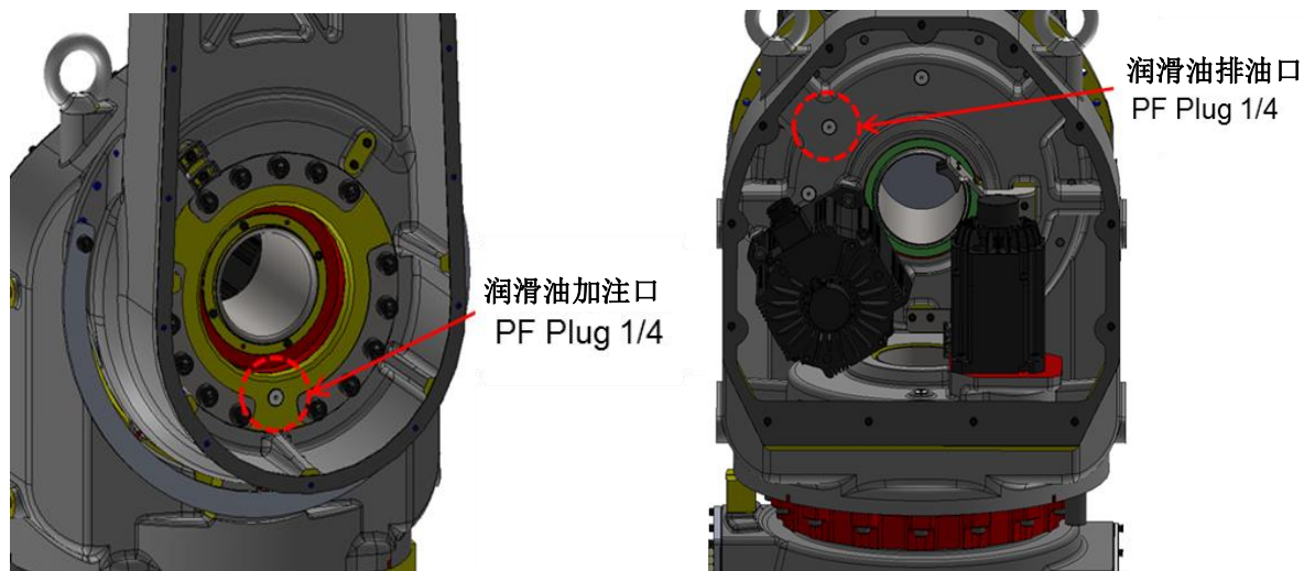
图 5.2 H 轴润滑油加注/排油口
