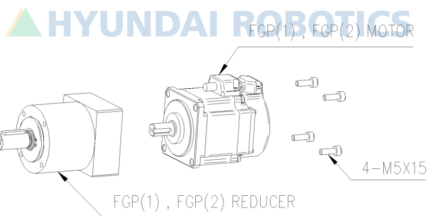
图 6.5 FGP 电机安装 (OPTION)
