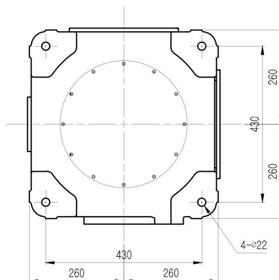
图 3.6 机器人安装尺寸:
