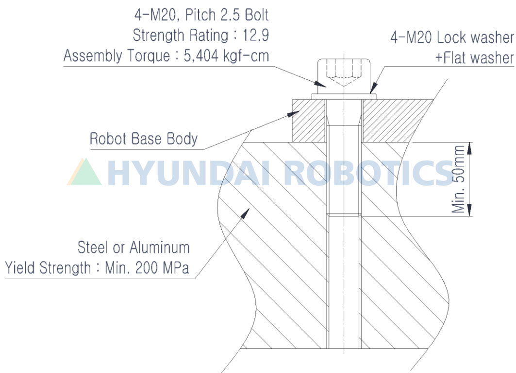
图 3.5 机器人安装断面图（地面、墙壁、天花板）
