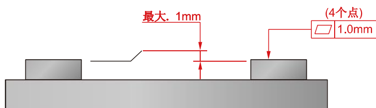
图 3.7 安装面精确度
