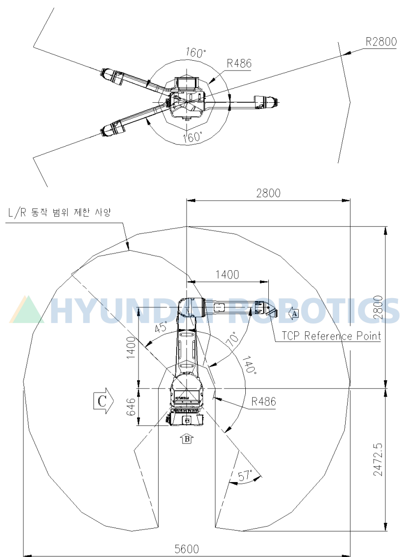
图 2.3 机器人尺寸和工作区间
