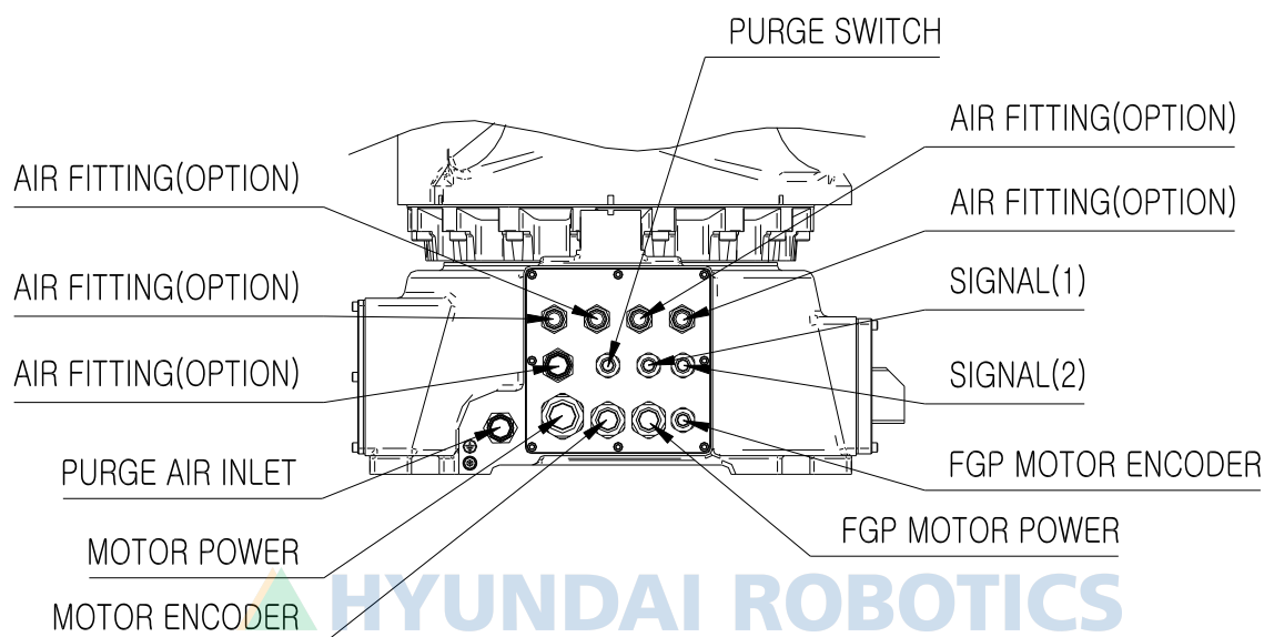
图 2.12 气压及电源接线: [Standard]
