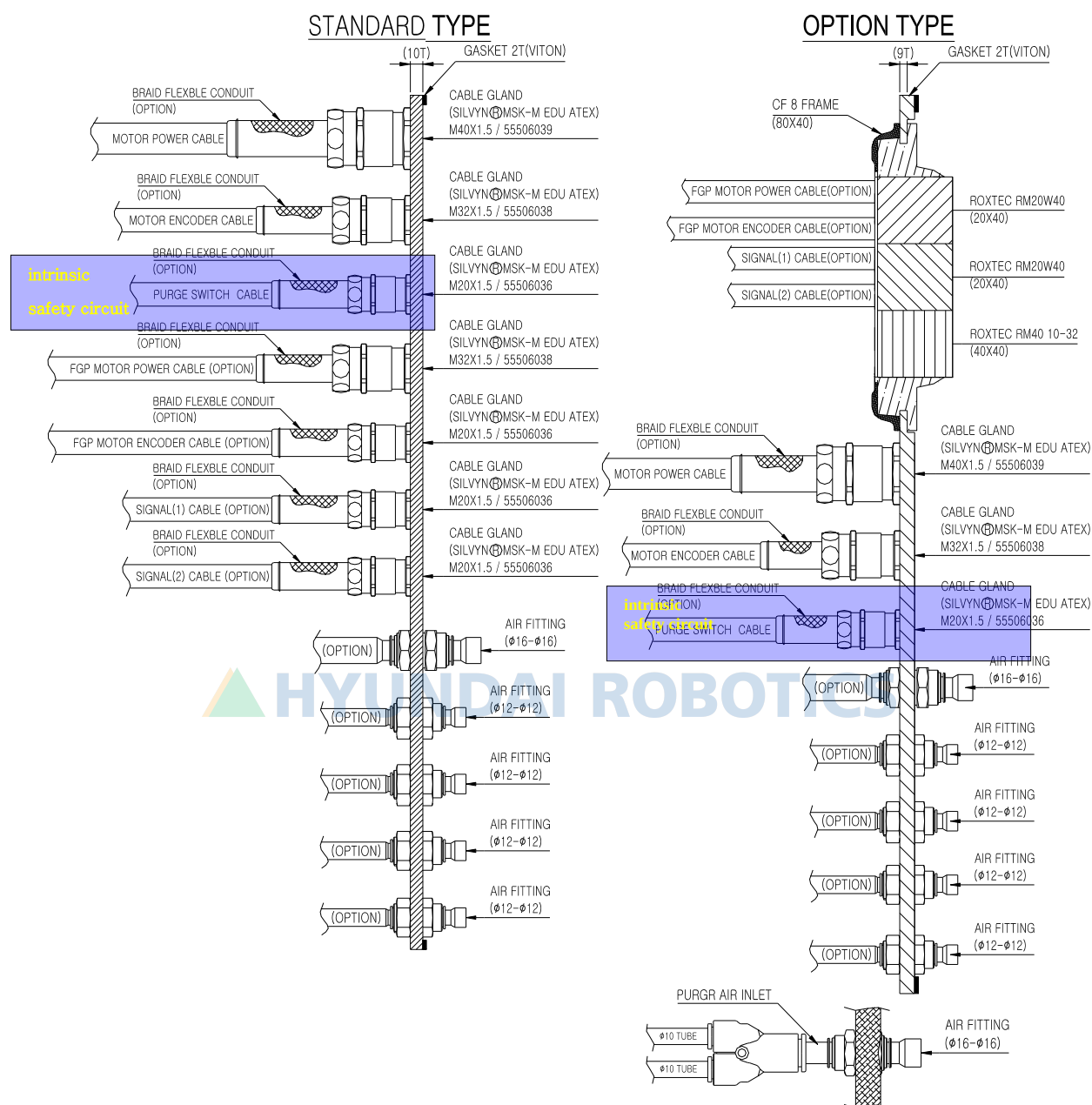
图 2.14 气压及电源: [Floor Type]
