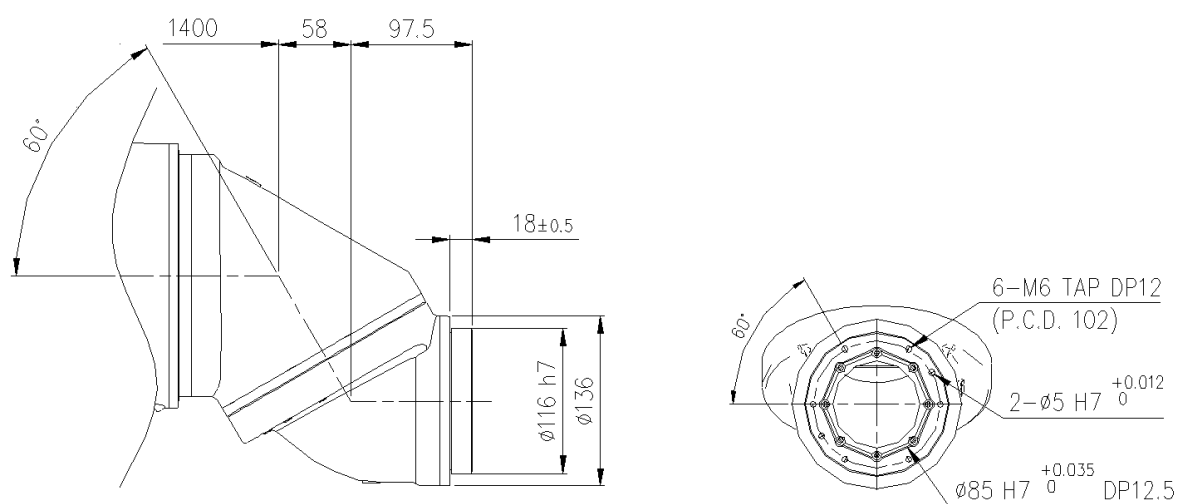
图 2.5 机械腕轴连接面细节
