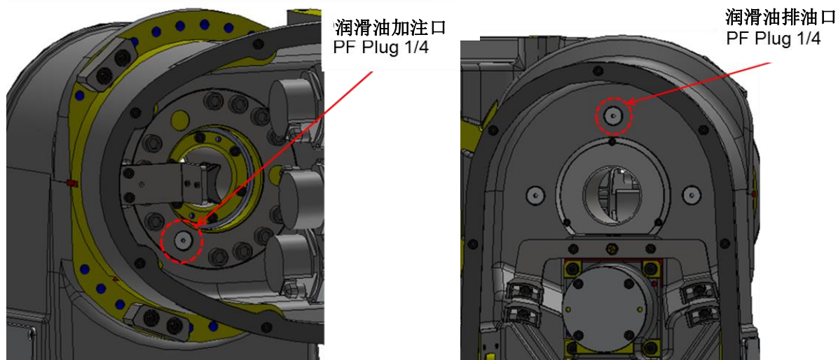
图 5.3 V 轴润滑油加注/排油口
