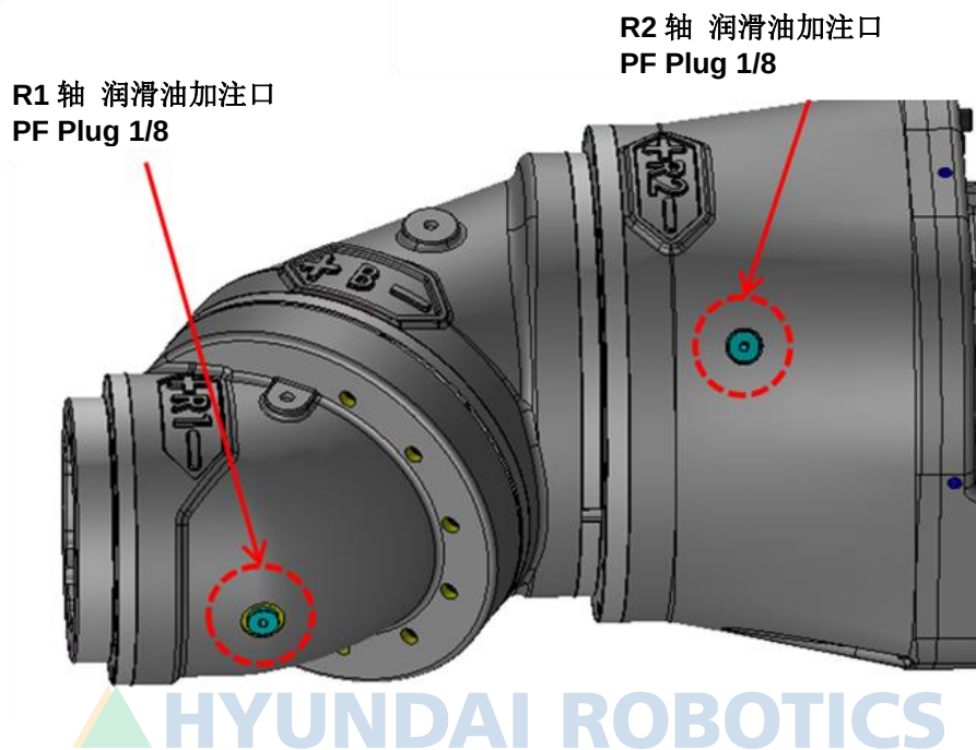
图 5.4 R2, R1 轴润滑脂注入口/排出口位置
