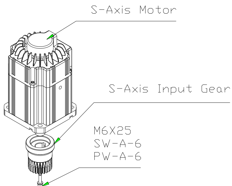
图 6.2 S 轴电机安装
