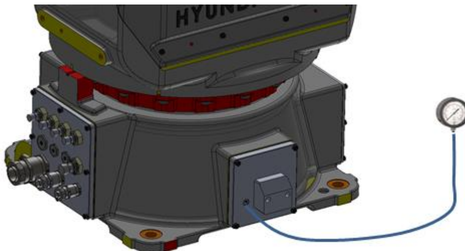
图 6.1 试验用端口
