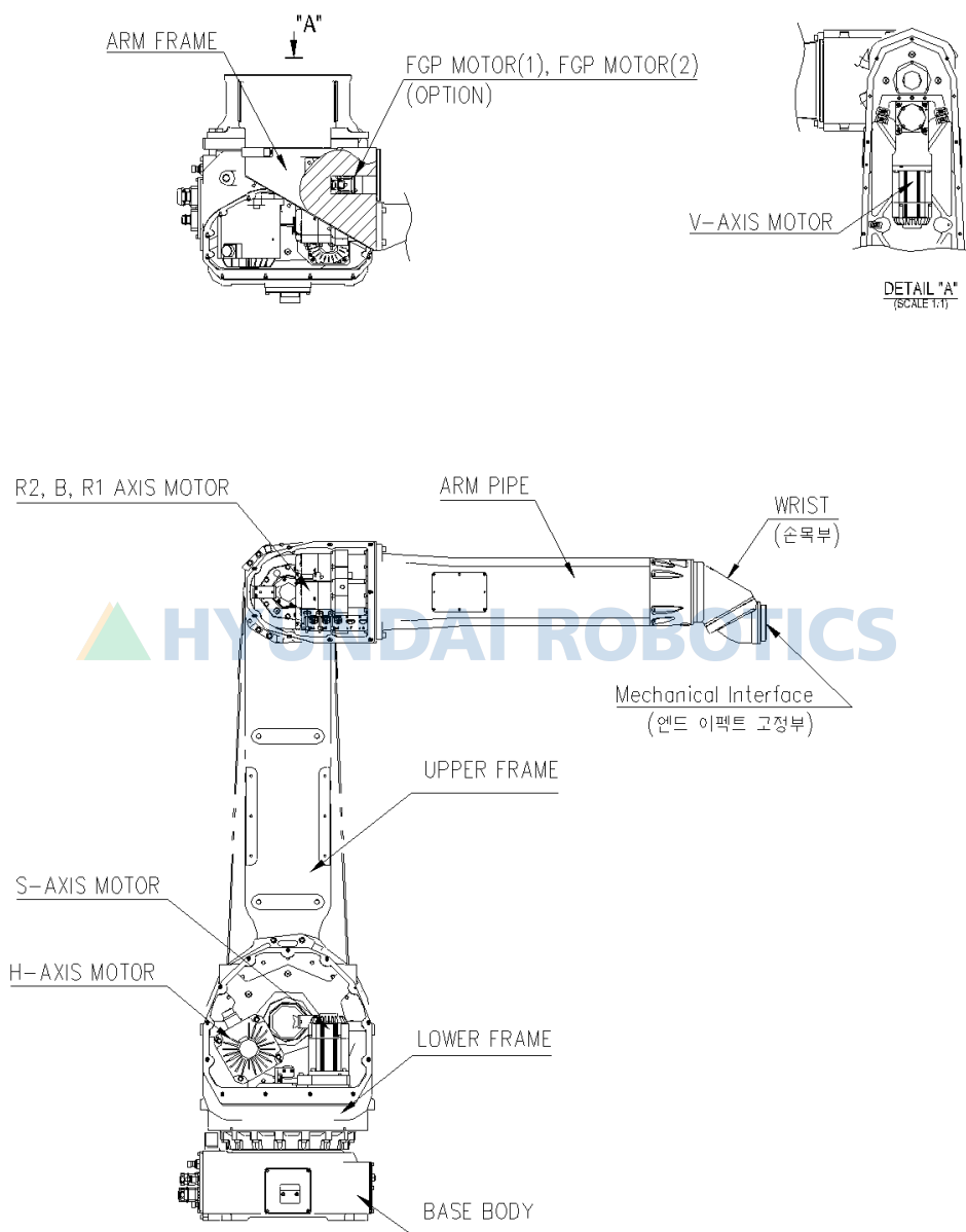
图 3.1 机器人零件名称
