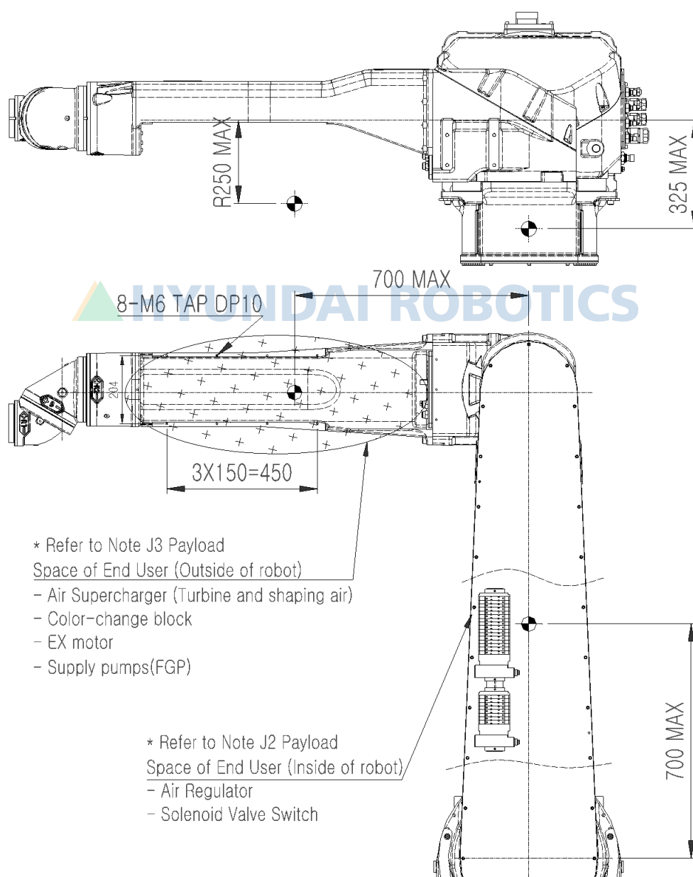
图 2.6 机械臂附着部详图
