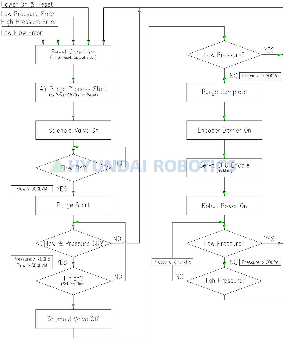
图 2.10 吹扫流程图
