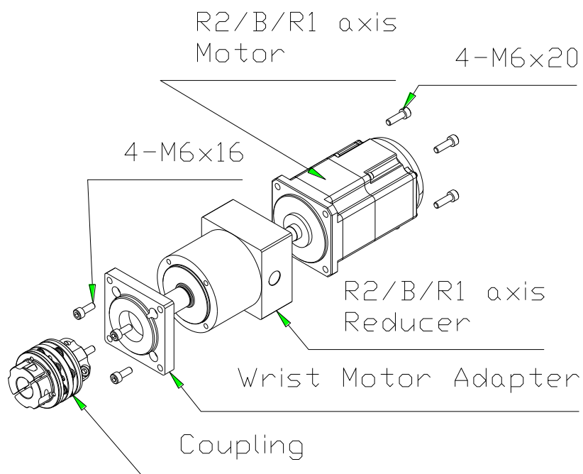
图 6.4 腕轴电机安装
