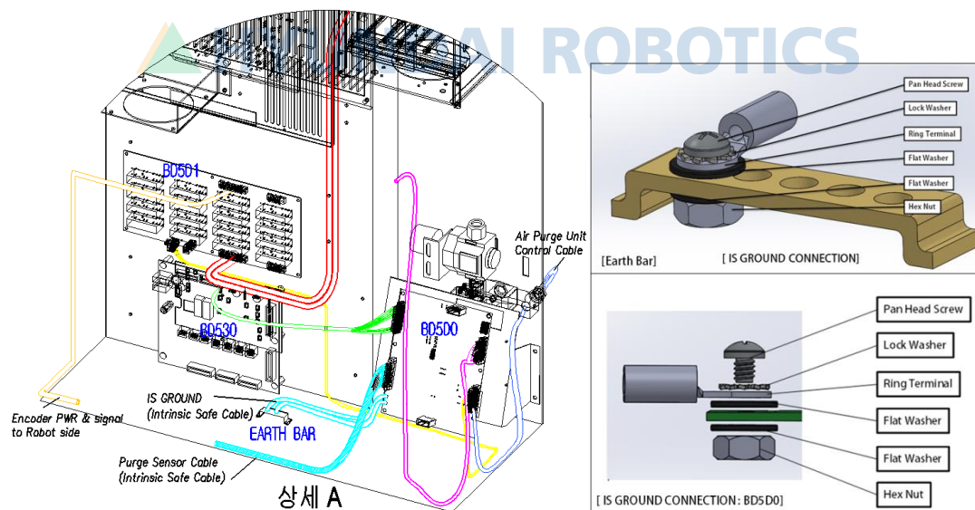
图 2.16 控制器内部接线
