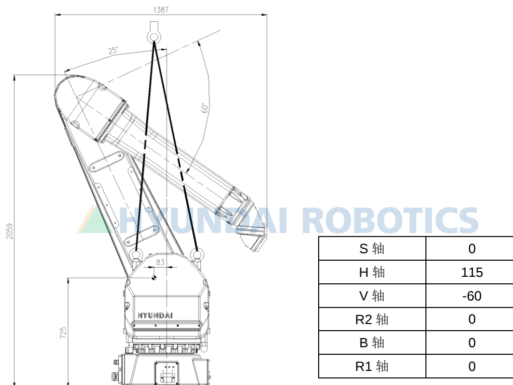
图 3.3 运送方法：使用吊车
