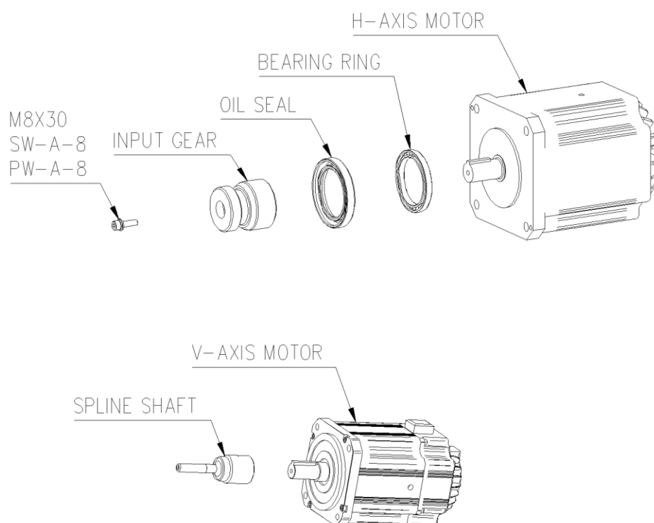
图 6.3 H&amp;V 轴电机安装
