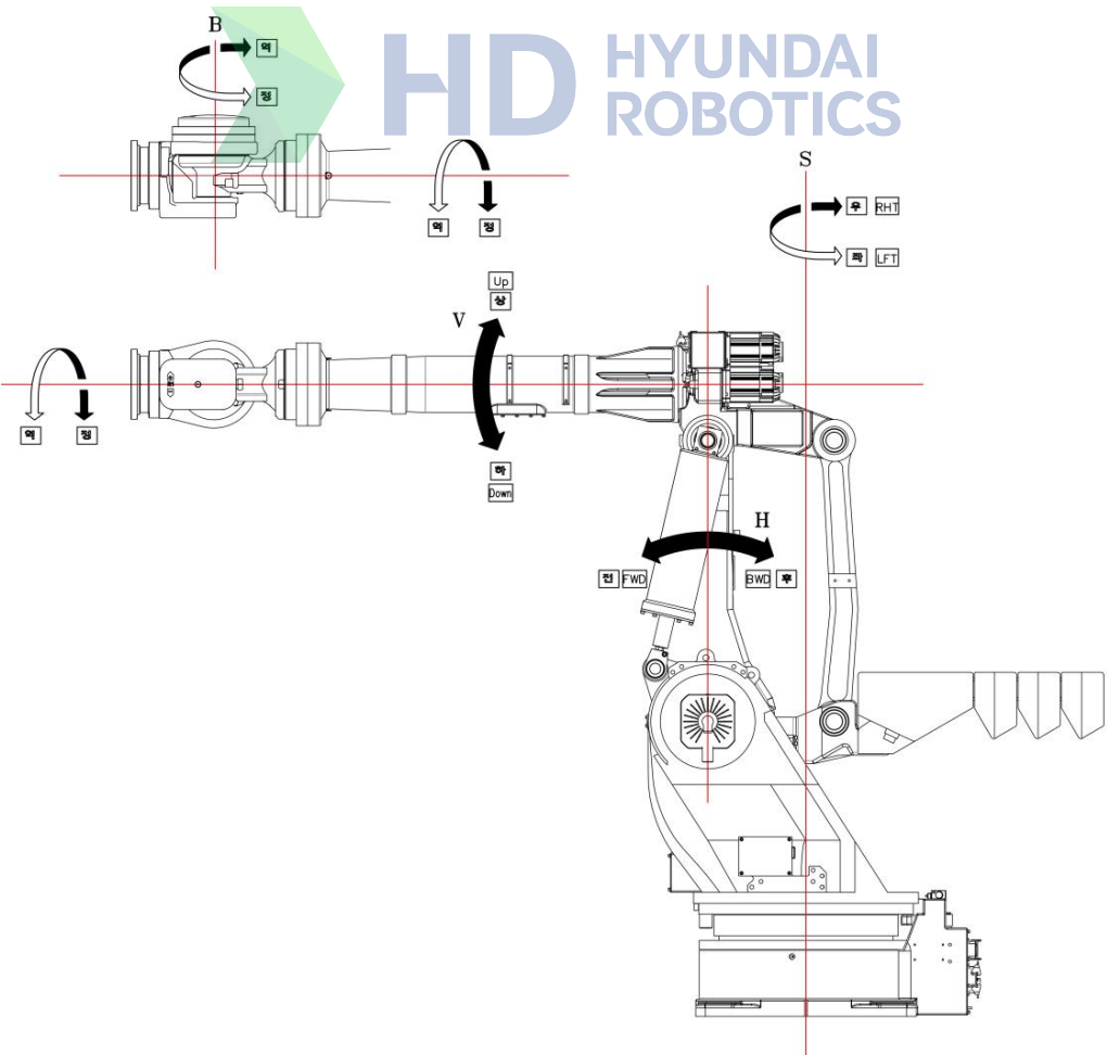
图 2.4 机器人尺寸和轴 [HX500S]
