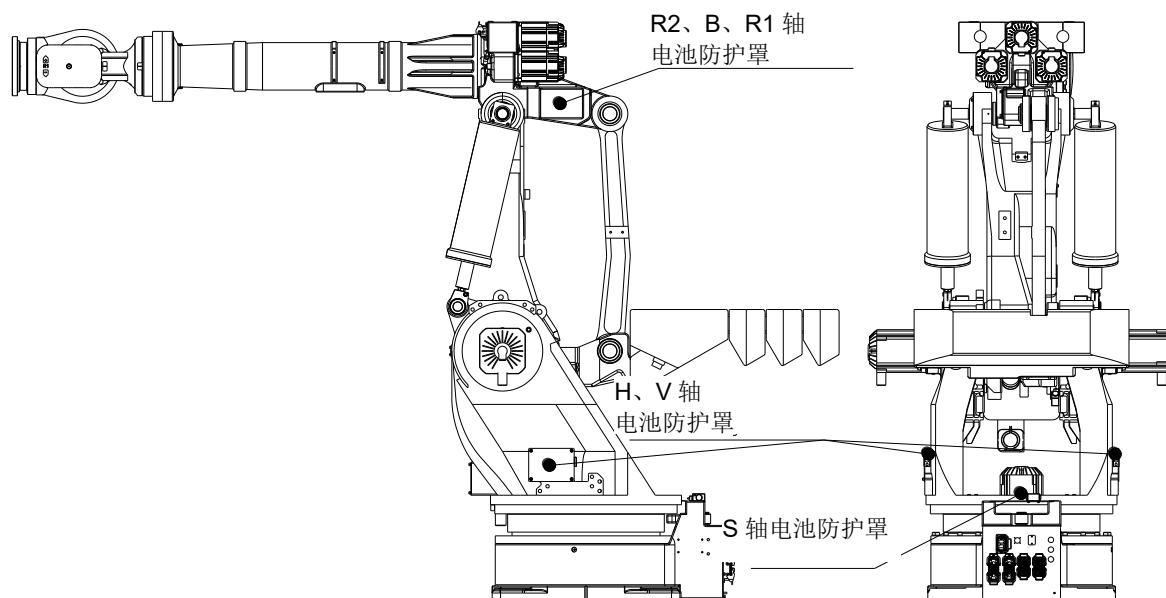
图 5.1 电池的位置
