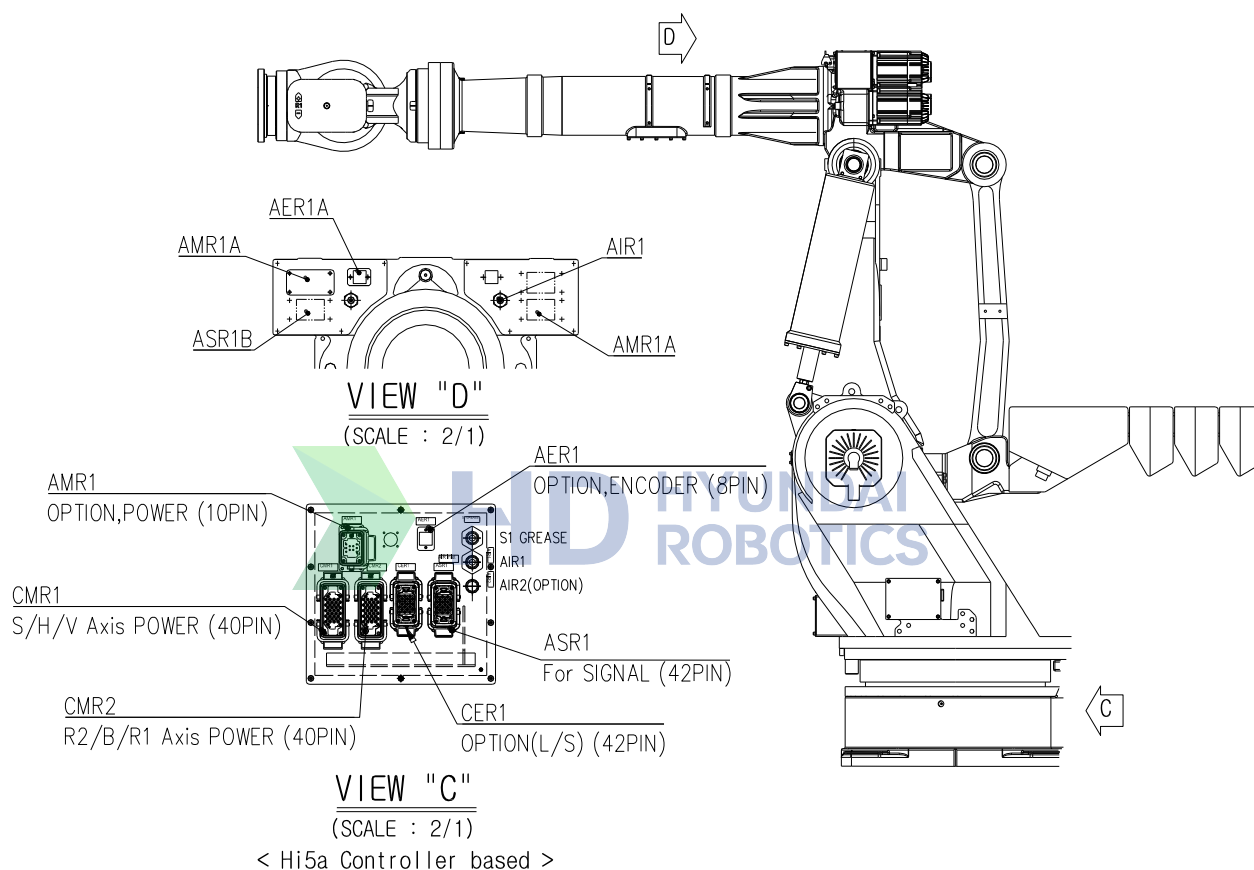
图 2.7 工作线路和检查线路图: [HX500S]
