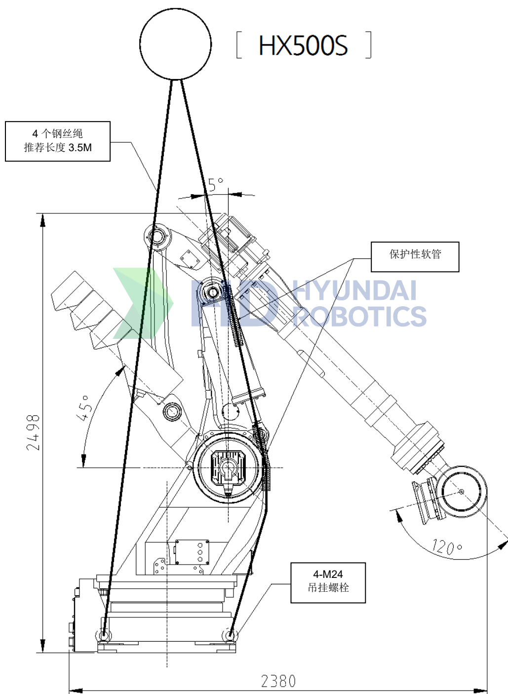
图 3.3 运送方法：使用吊车 [HX500S]
