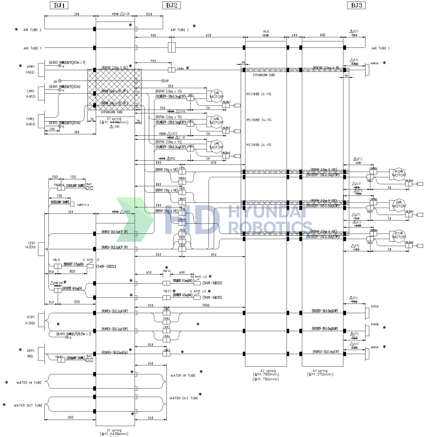
图 5.3 内部接线的连接图
