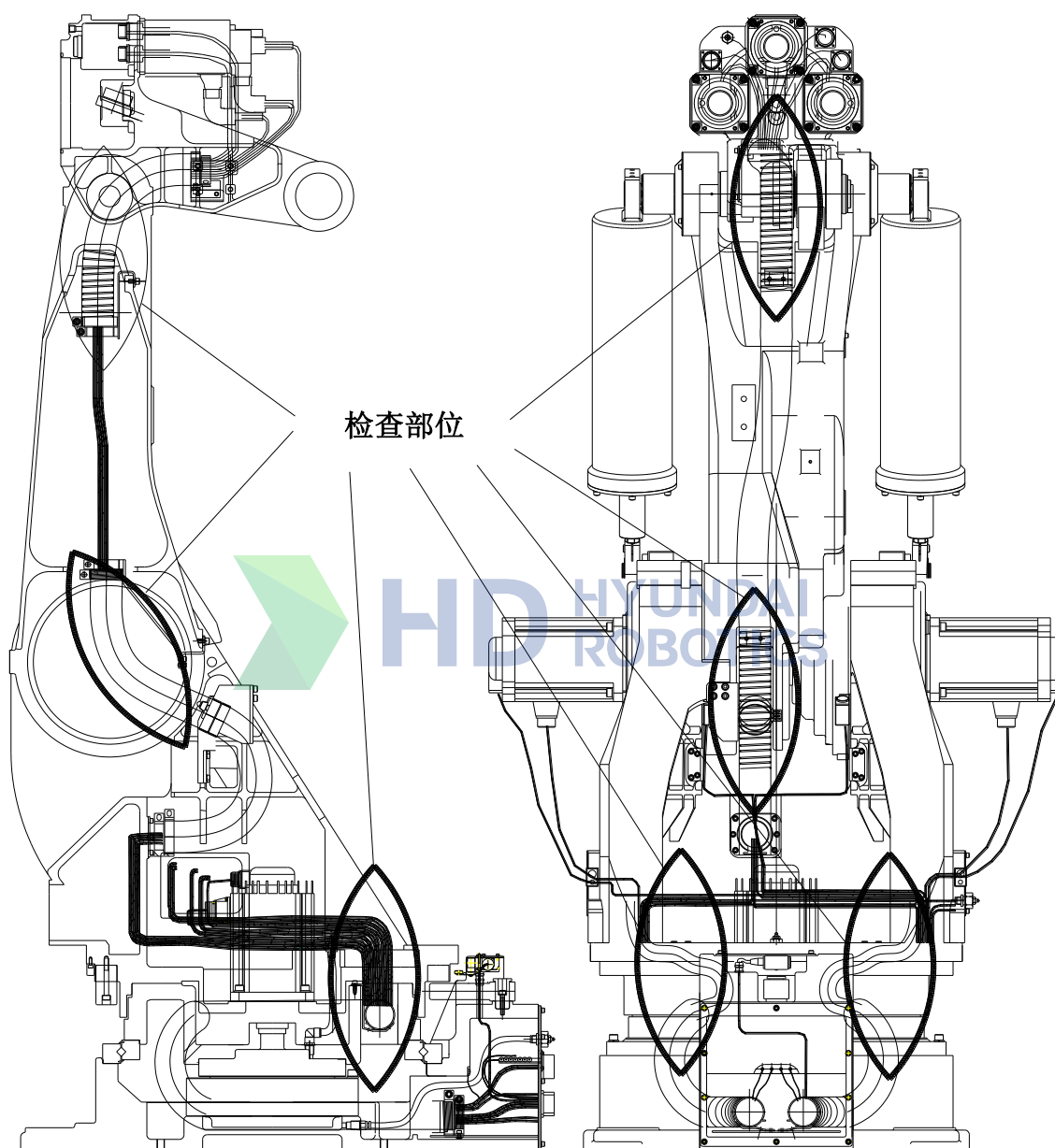
图 4.3 电缆检查部位
