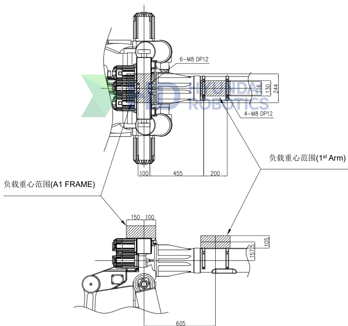
图 2.6 1 st Arm 第一臂部上部连接图 : [HX500S]
