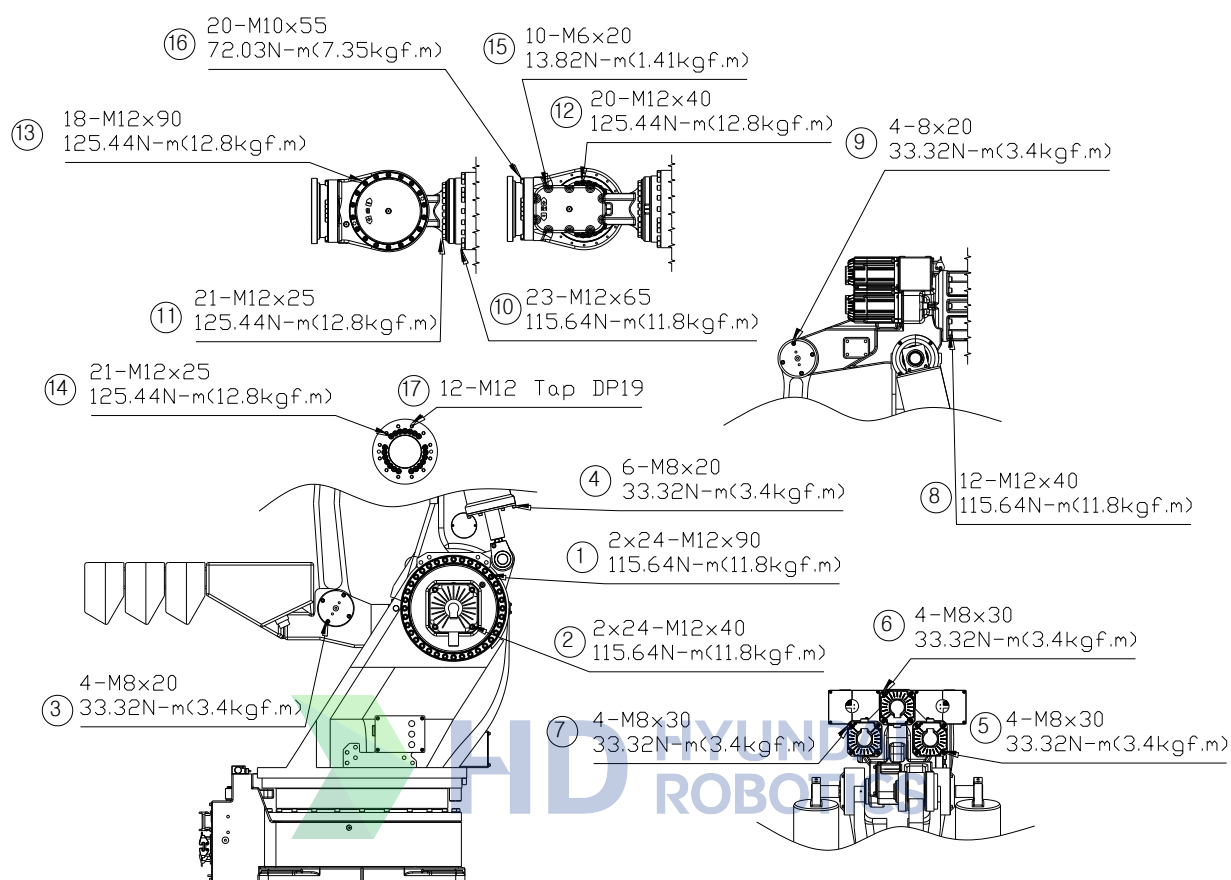
图 4.1 主要螺栓的检查部位 [HX500S]
