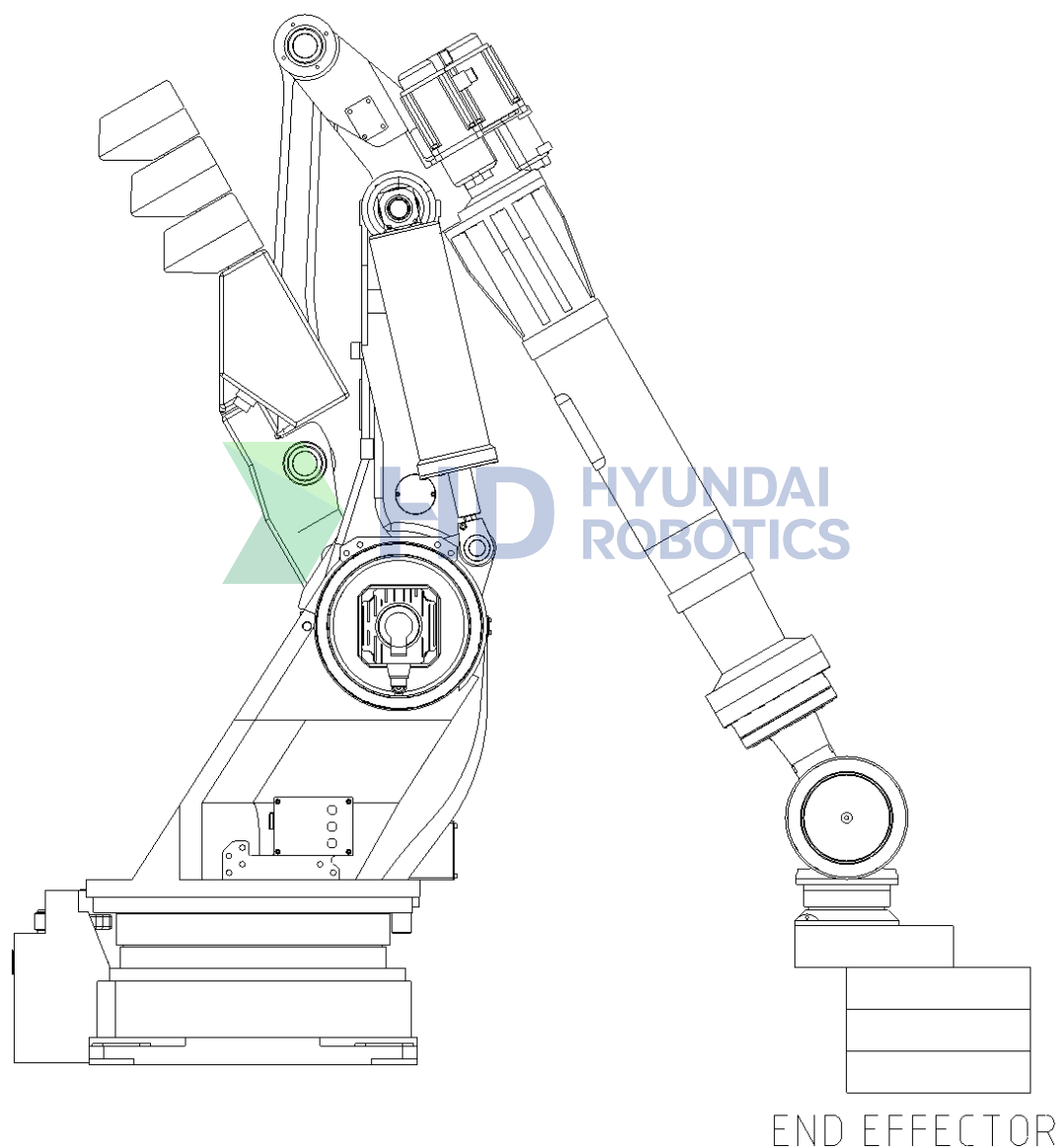
图 3.8 推荐等待姿势
