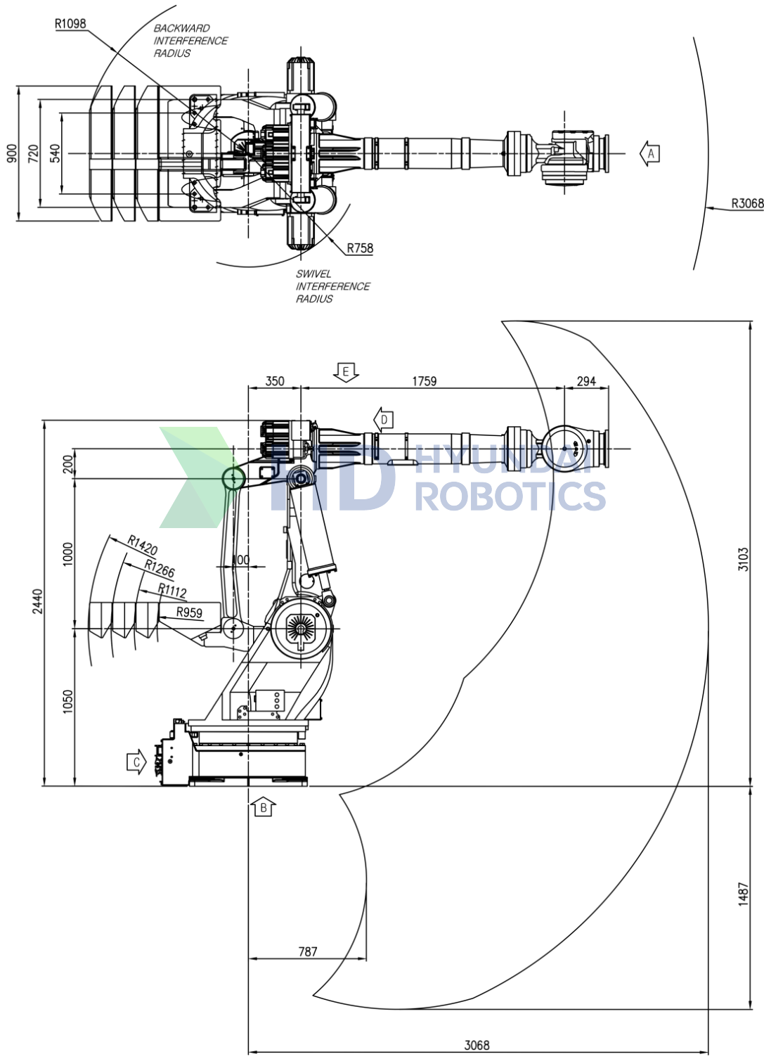
图 2.3 机器人尺寸和工作区间 : [HX500S]
