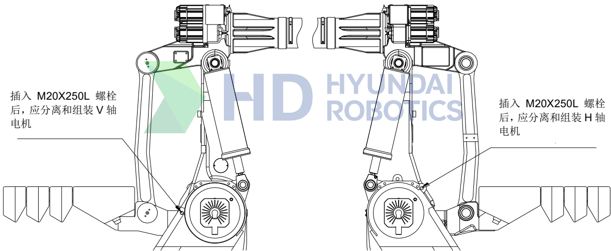
图 6.1 H, V 轴 Arm 降落防止方法
