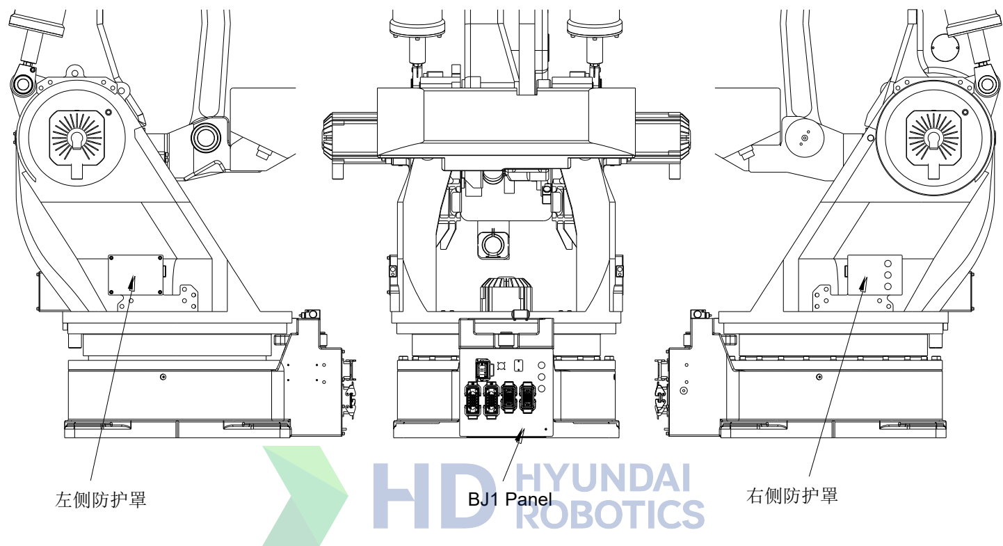
图 9.1 机械手配置
