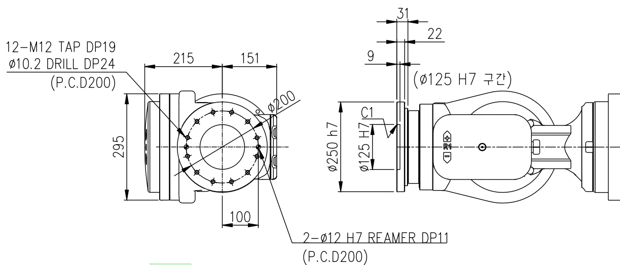
图 2.5 机械腕轴连接面细节 : [HX500S]
