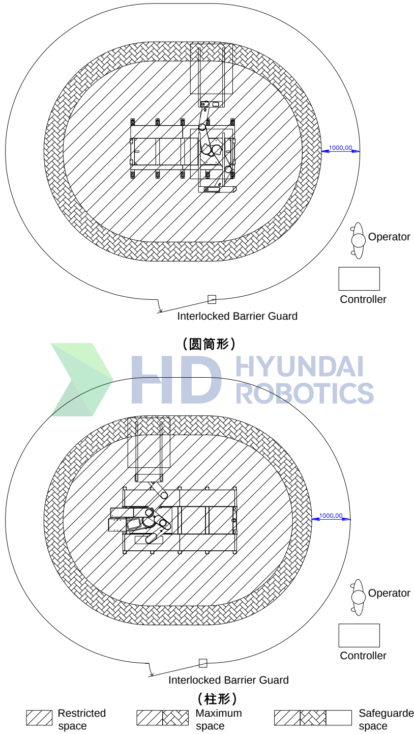
图 1.3 LCD 用机器人周边装置与工作人员的布置
