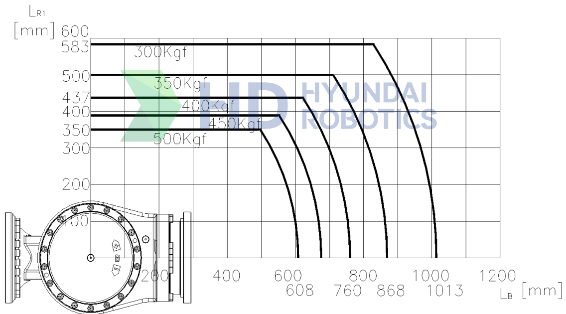
图 3.7 腕轴转矩图 [HX500S]
