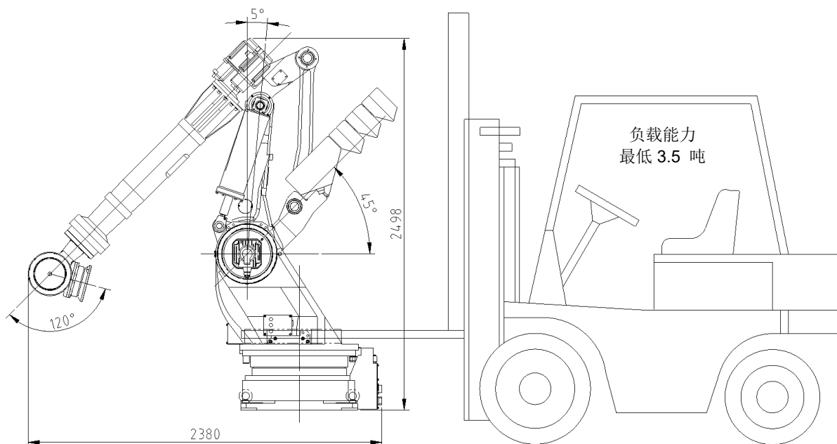
图 3.4 运送方法：利用叉车 [HX500S]
