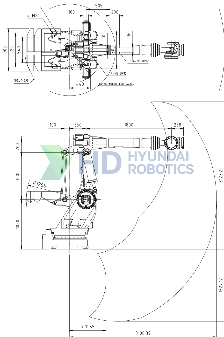
图 2.3 机器人尺寸和工作区间 : [HX400S]
