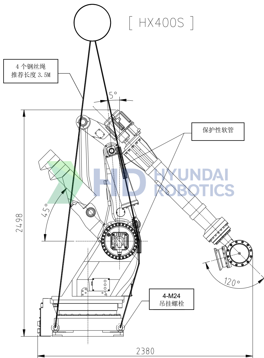
图 3.3 运送方法：使用吊车 [HX400S]
