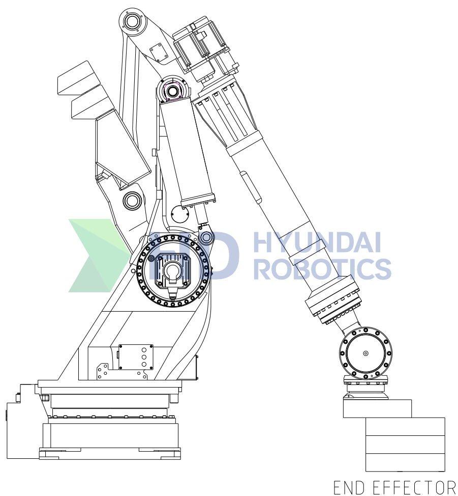
图 3.10 推荐等待姿势
