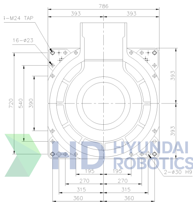
图 3.6 机器人安装尺寸
