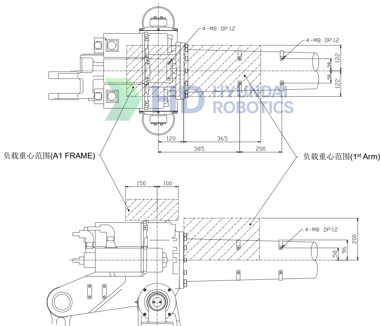
图 2.6 1 st Arm 第一臂部上部连接图 : [HX400S]
