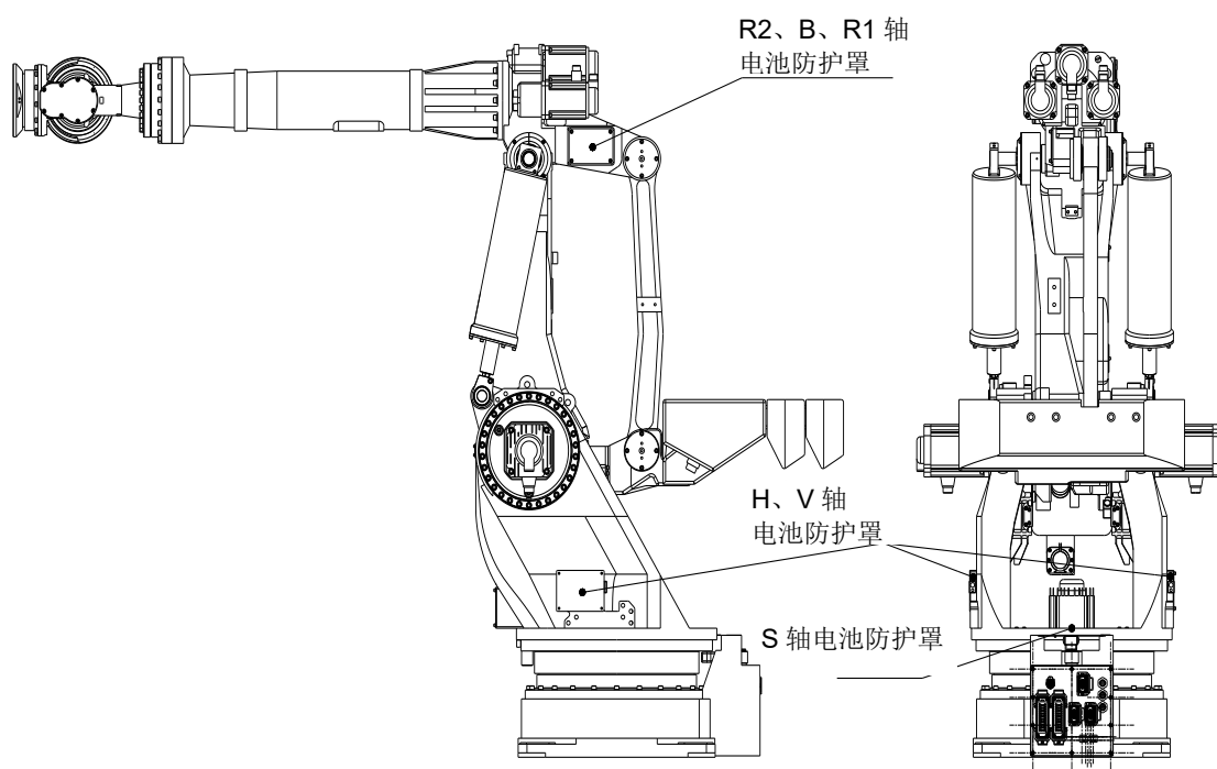
图 5.1 电池的位置
