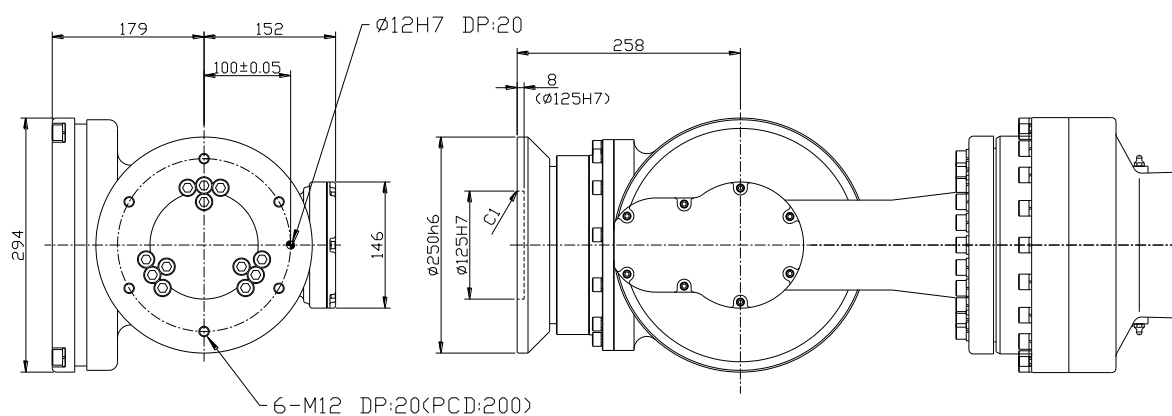
图 2.5 机械腕轴连接面细节：[HX400S]
