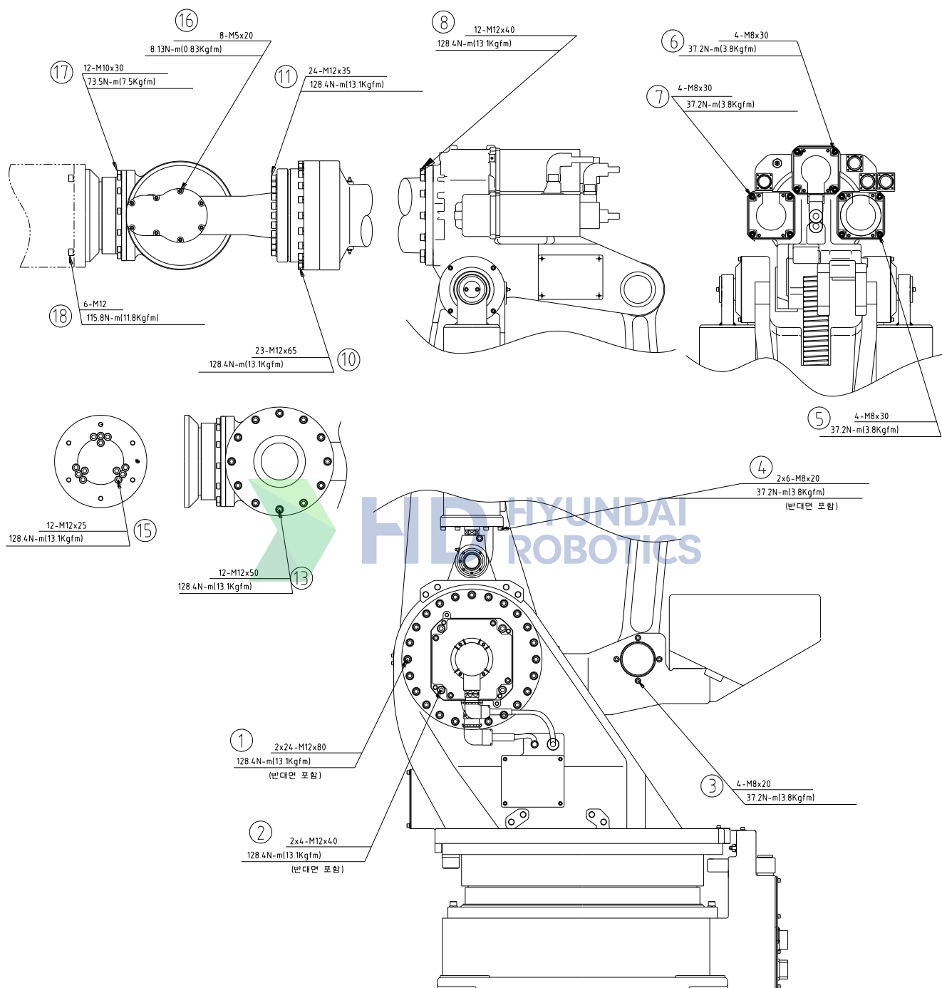
图 4.1 主要螺栓的检查部位 [HX400S]
