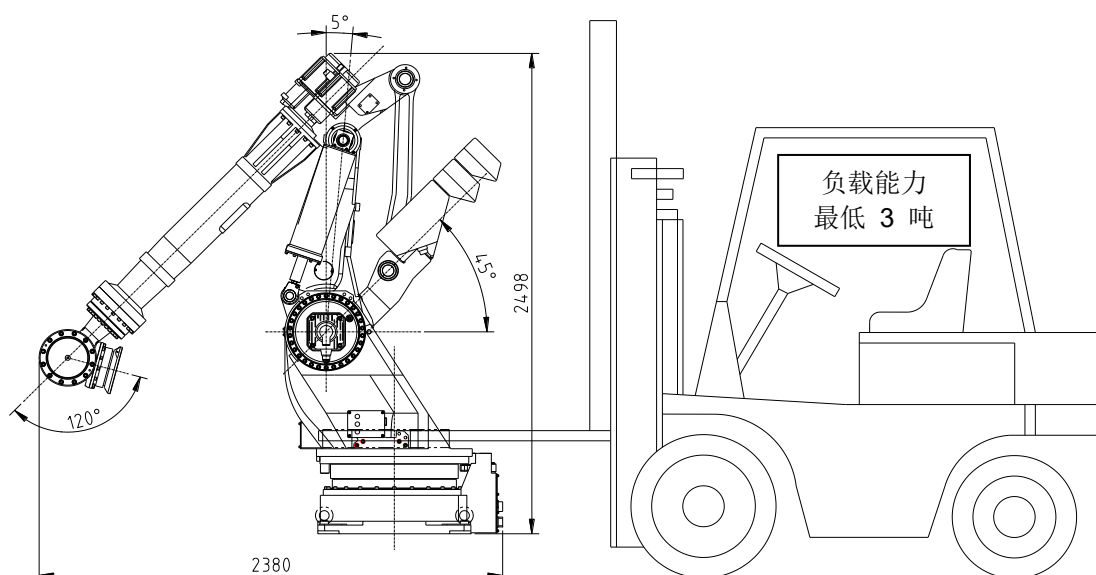
图 3.4 运送方法：利用叉车
