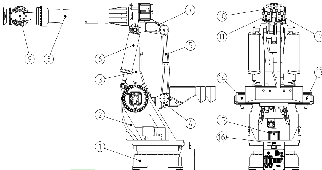
图 3.1 机器人零件名称
