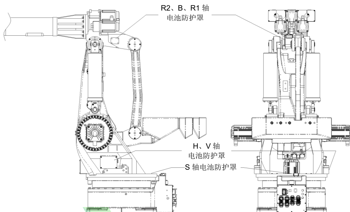
图 5.1 电池的位置
