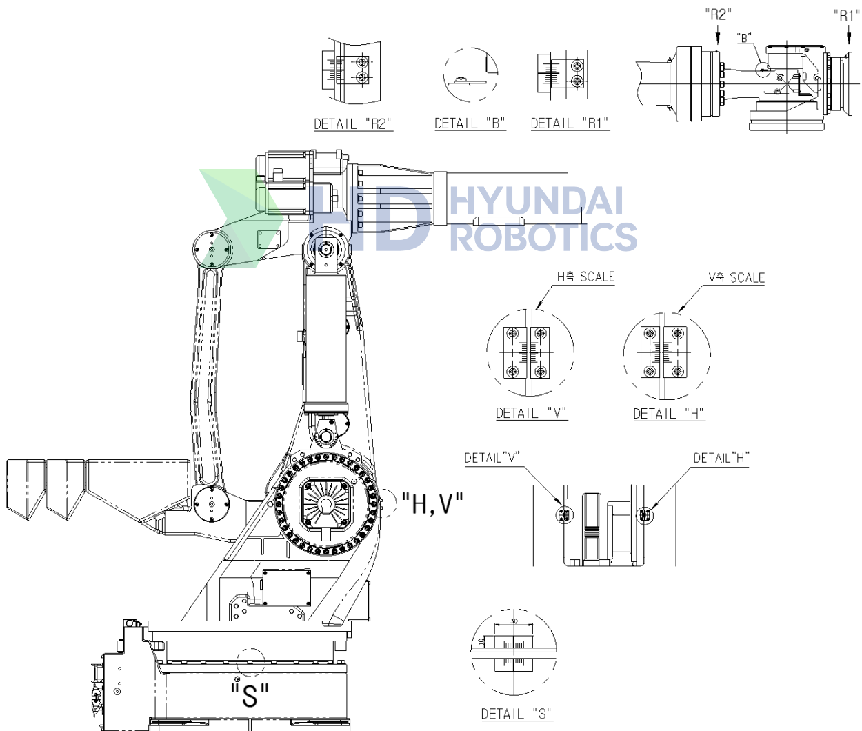
图 6.2 原点设置方法
