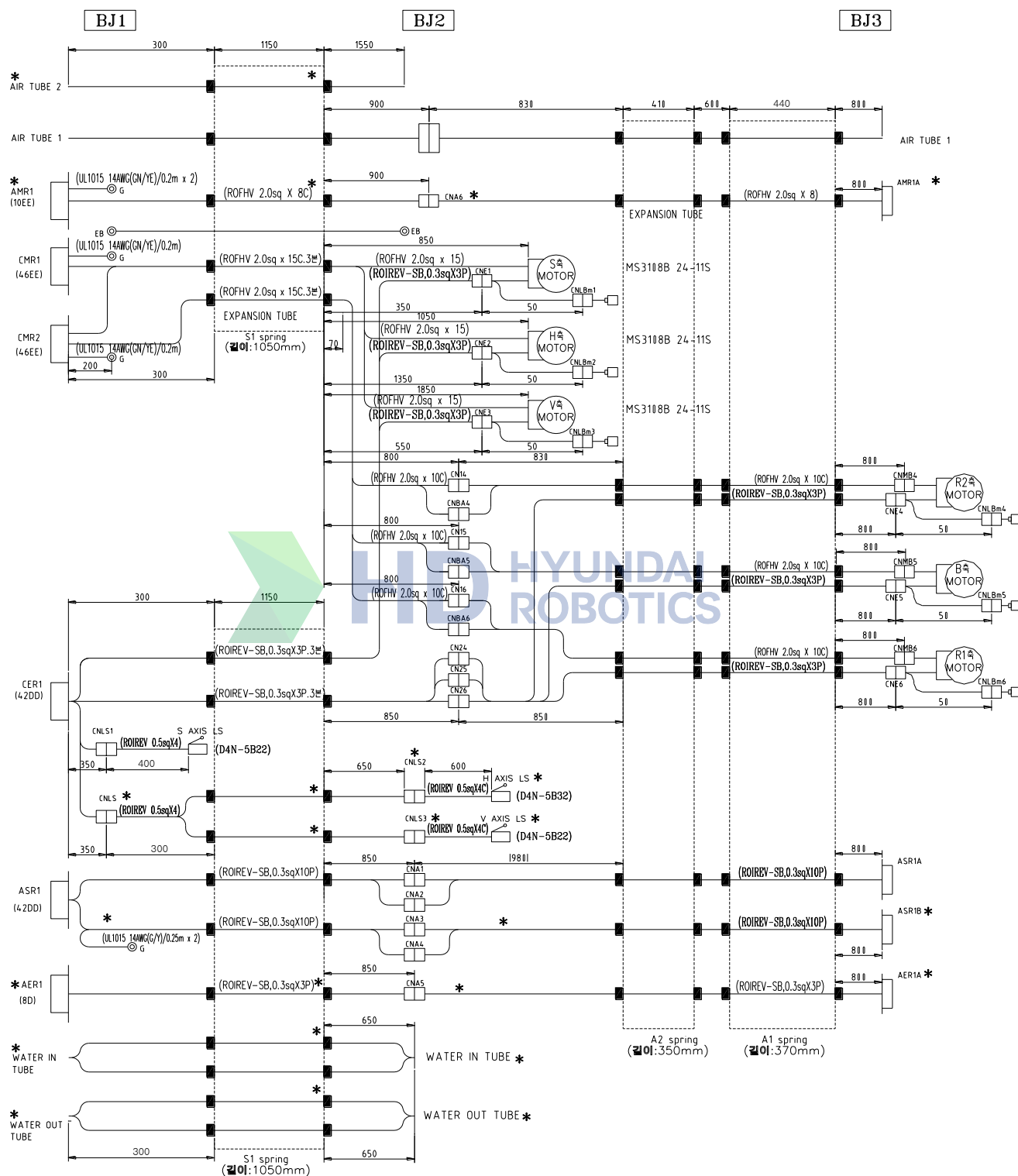
图 5.3 内部接线的连接图
