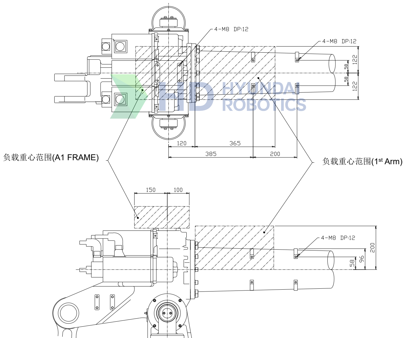
图 2.6 上部机械臂附着部详图
