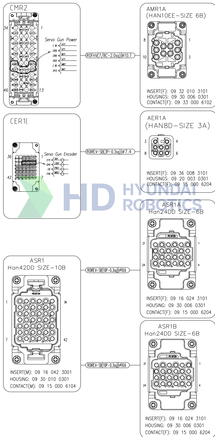
图 2.8 应用连接器细节
