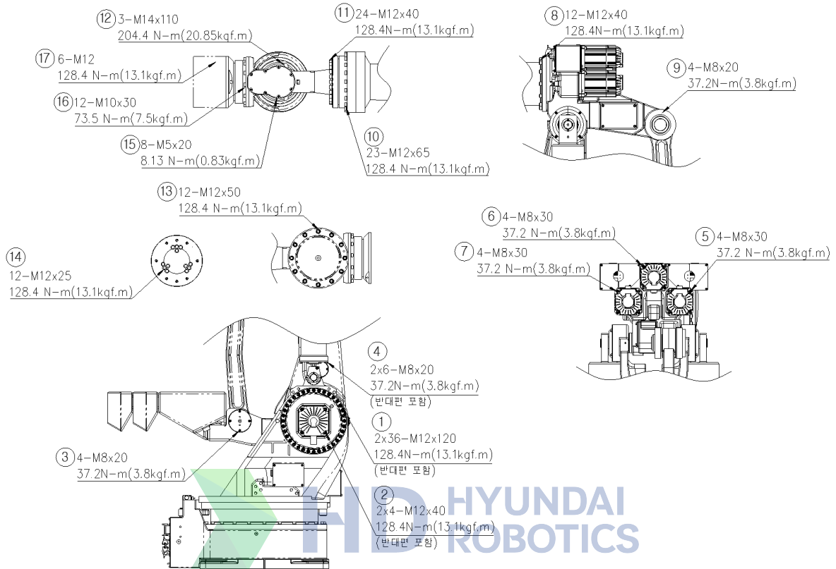
图 4.1 主要螺栓的检查部位
