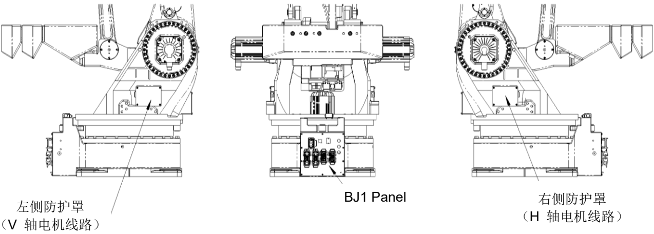
图 9.1 机械手配置
