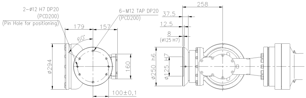
图 2.5 机械腕轴连接面细节
