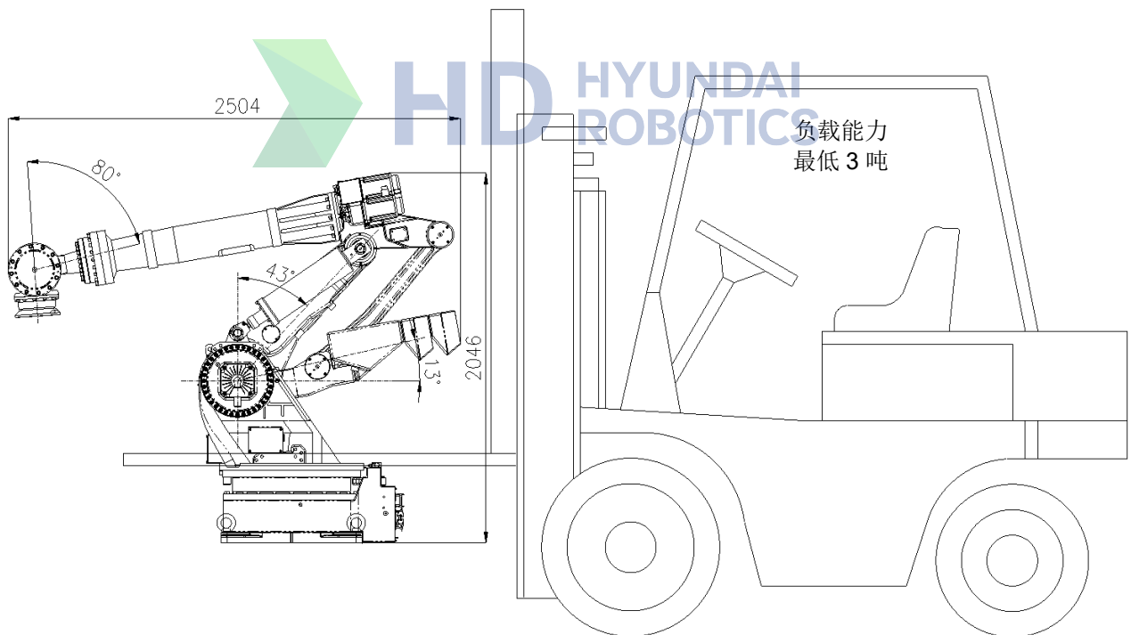
图 3.4 运送方法：利用叉车
