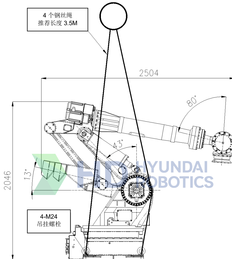
图 3.3 运送方法：使用吊车
