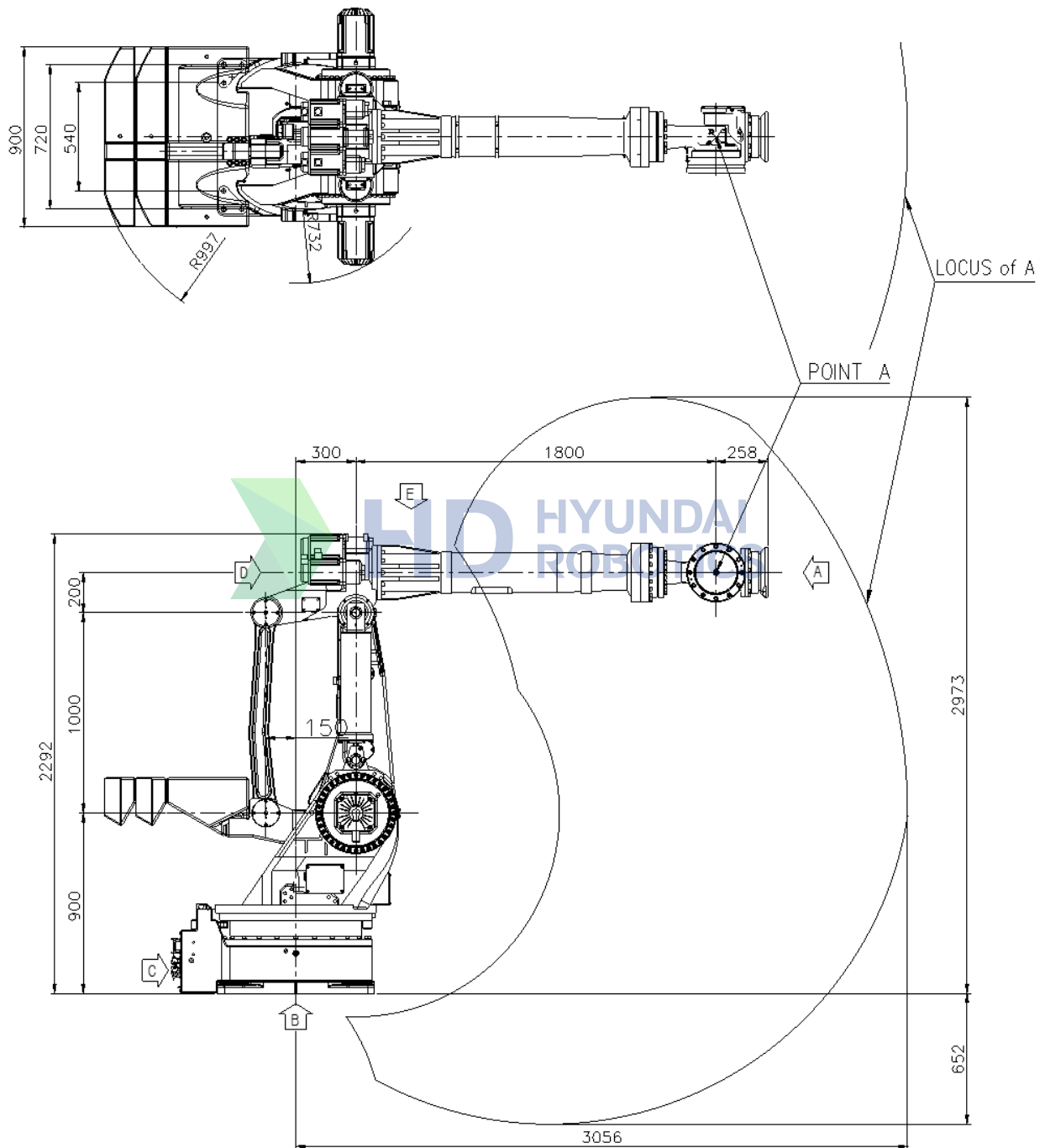
图 2.3 机器人尺寸和工作区间
