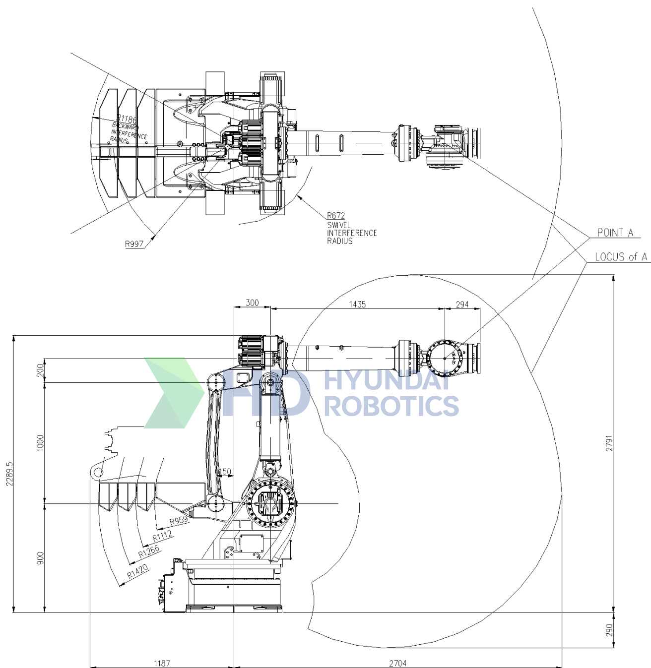
图 2.8 机器人尺寸和工作区间：[HX500]
