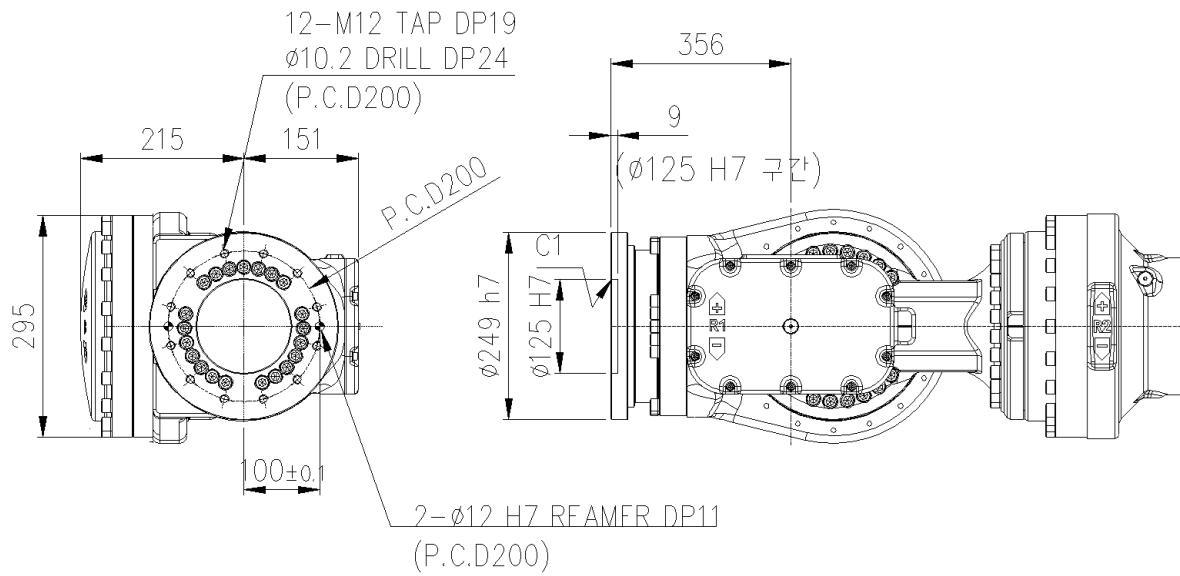
图 2.12 机械腕轴连接面细节 : [HX500]
