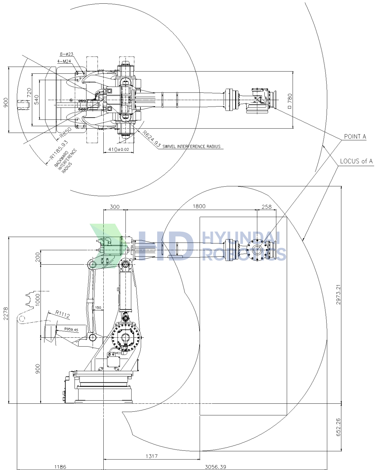
图 2.7 机器人尺寸和工作区间：[HX300L]
