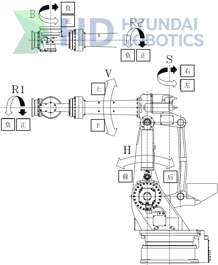
图 2.9 机器人尺寸和轴
