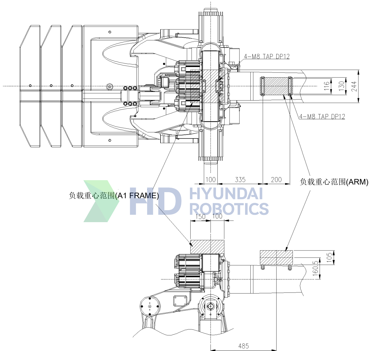
图 2.14 第一臂部上部连接图 [HX500]
