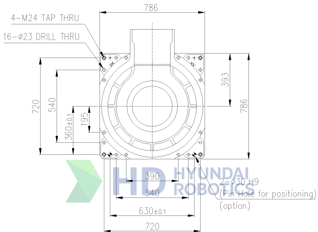
图 3.7 机器人安装尺寸
