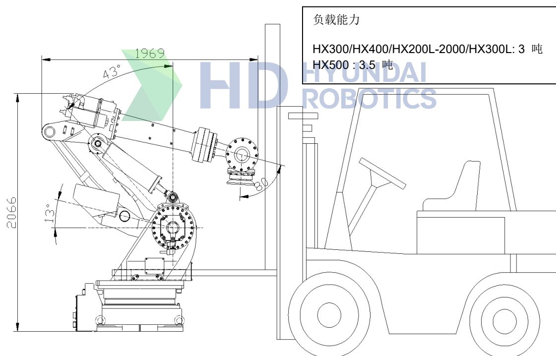
图 3.5 运送方法：利用叉车
