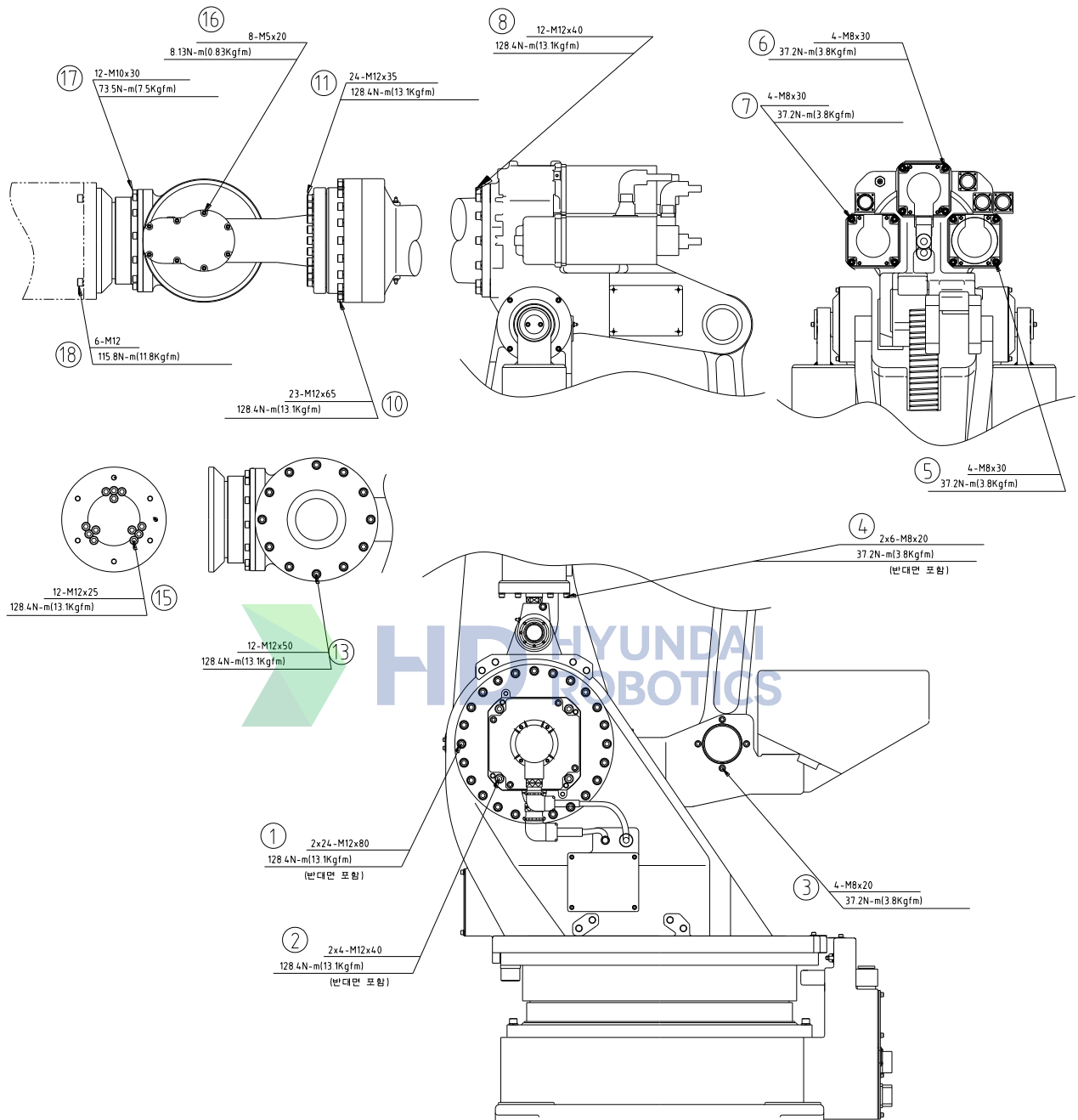
图 4.1 主要螺栓的检查部位 [HX300/HX400/HX300L]
