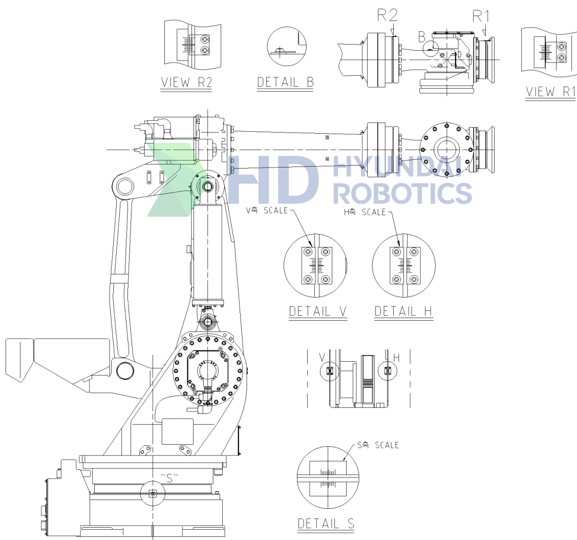
图 6.2 原点设置方法 (HX200L/HX200L-2000/HX300/HX300L/HX400)
