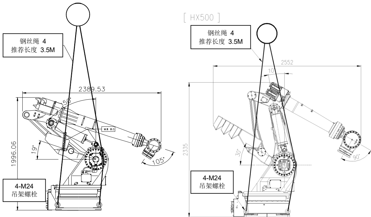
图 3.4 运送方法：使用吊车 [HX200L/HX300L/HX500]
