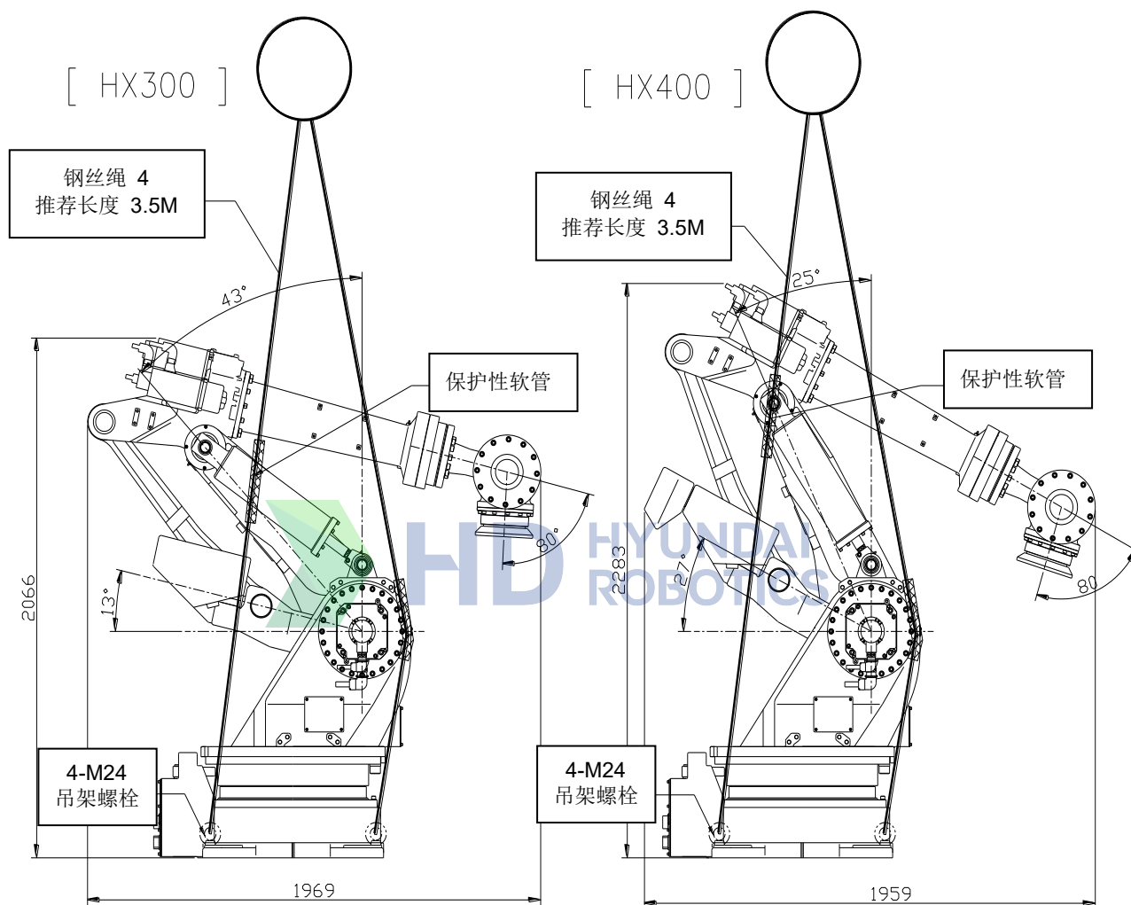
图 3.3 运送方法：使用吊车 [HX300/HX400]
