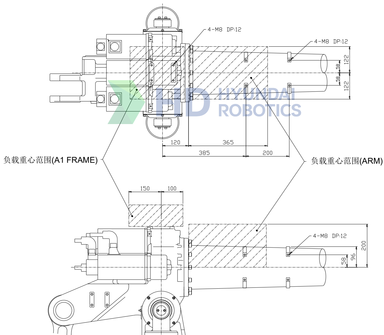
图 2.13 第一臂部上部连接图
