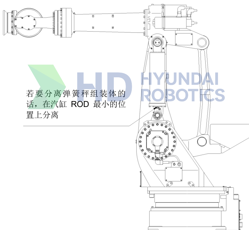
图 8.1 弹簧秤分离姿势
