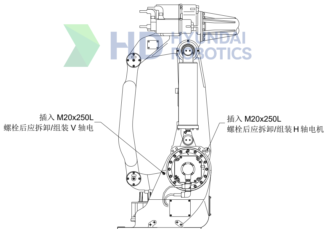
图 6.1 H,V 轴 ARM 降落防止方法
