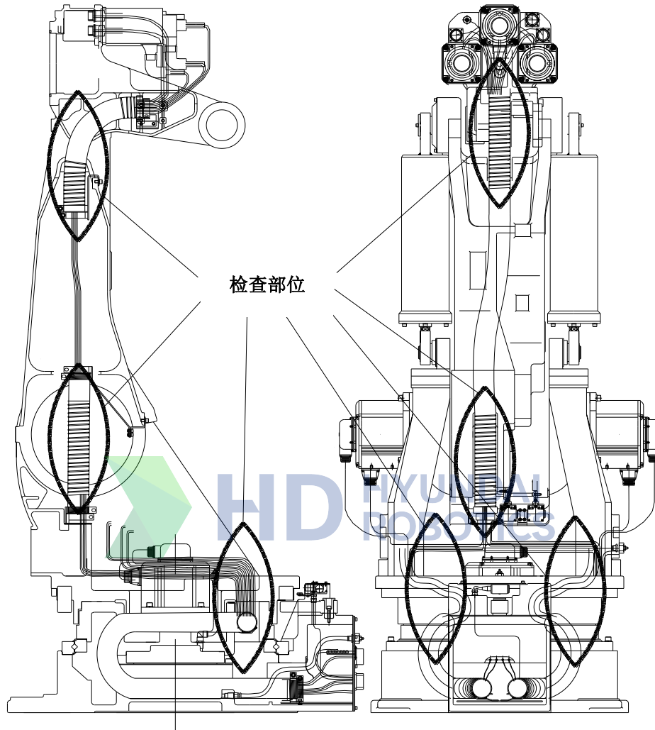
图 4.4 电缆检查部位
