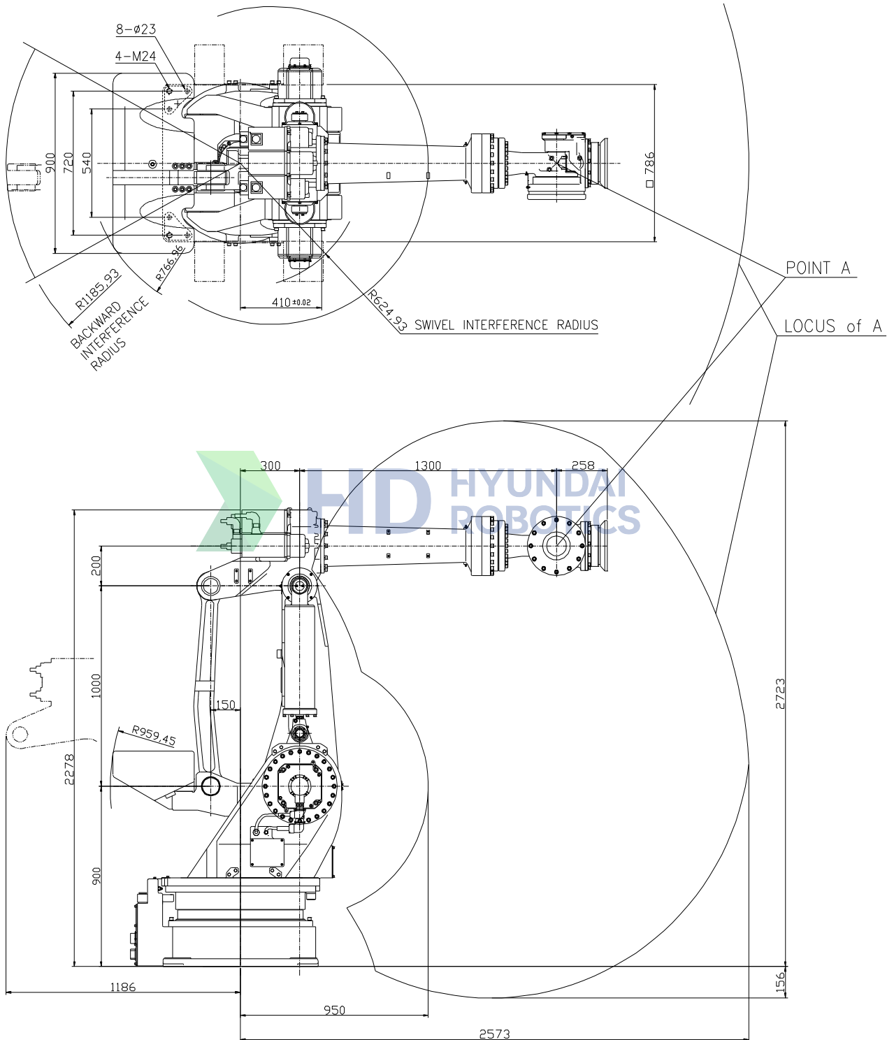
图 2.3 机器人尺寸和工作区间：[HX300]
