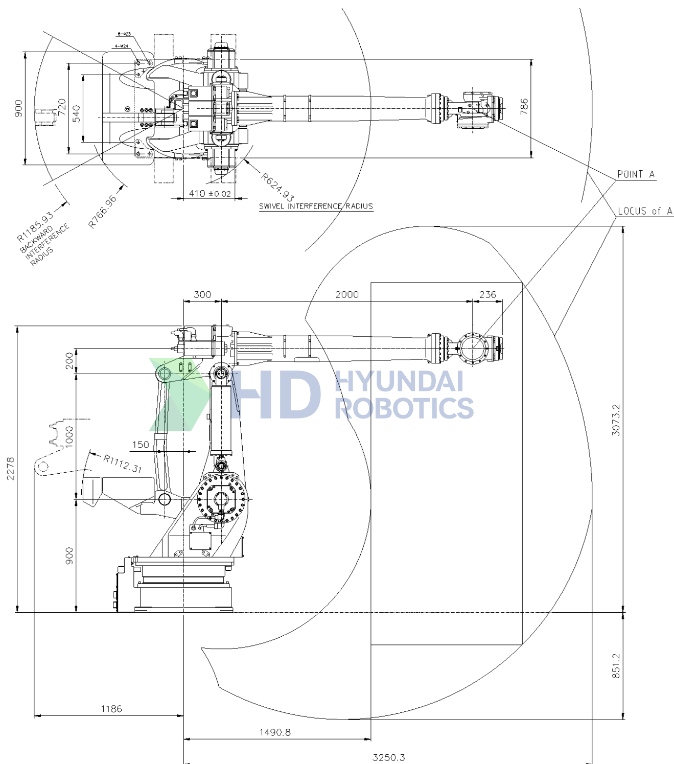
图 2.6 机器人尺寸和工作区间：[HX200L-2000]
