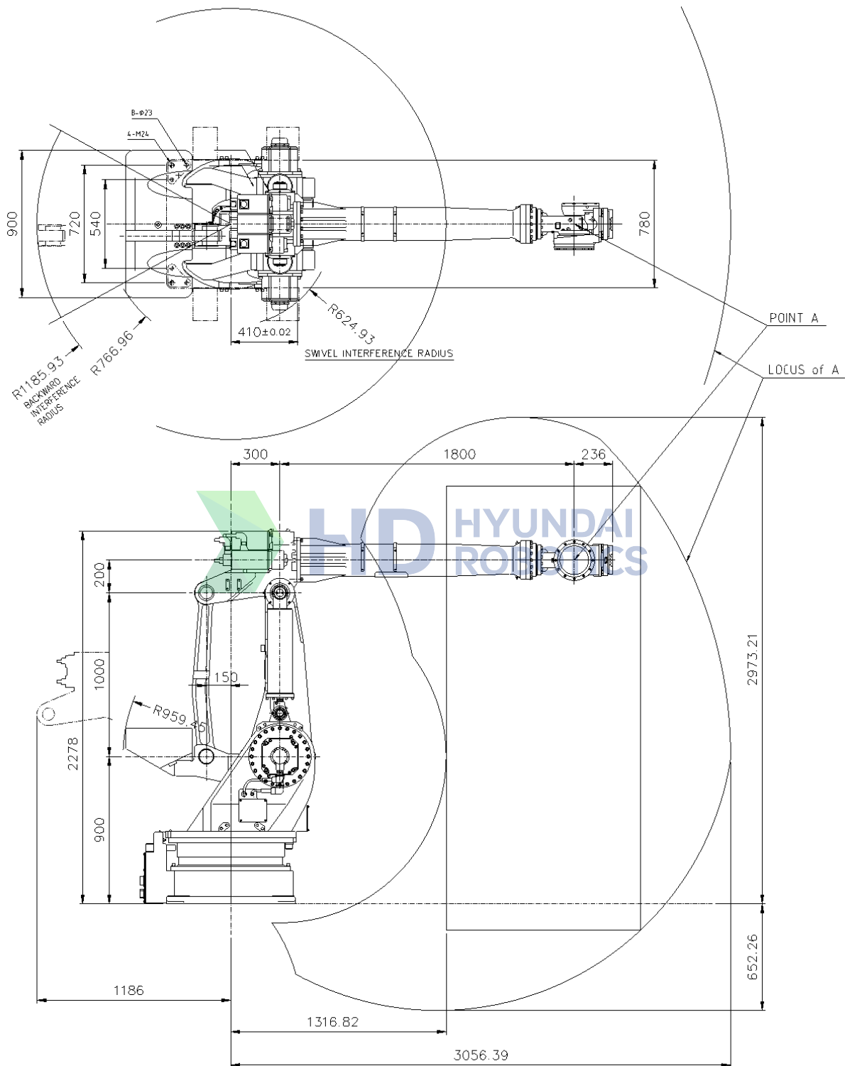
图 2.5 机器人尺寸和工作区间：[HX200L]
