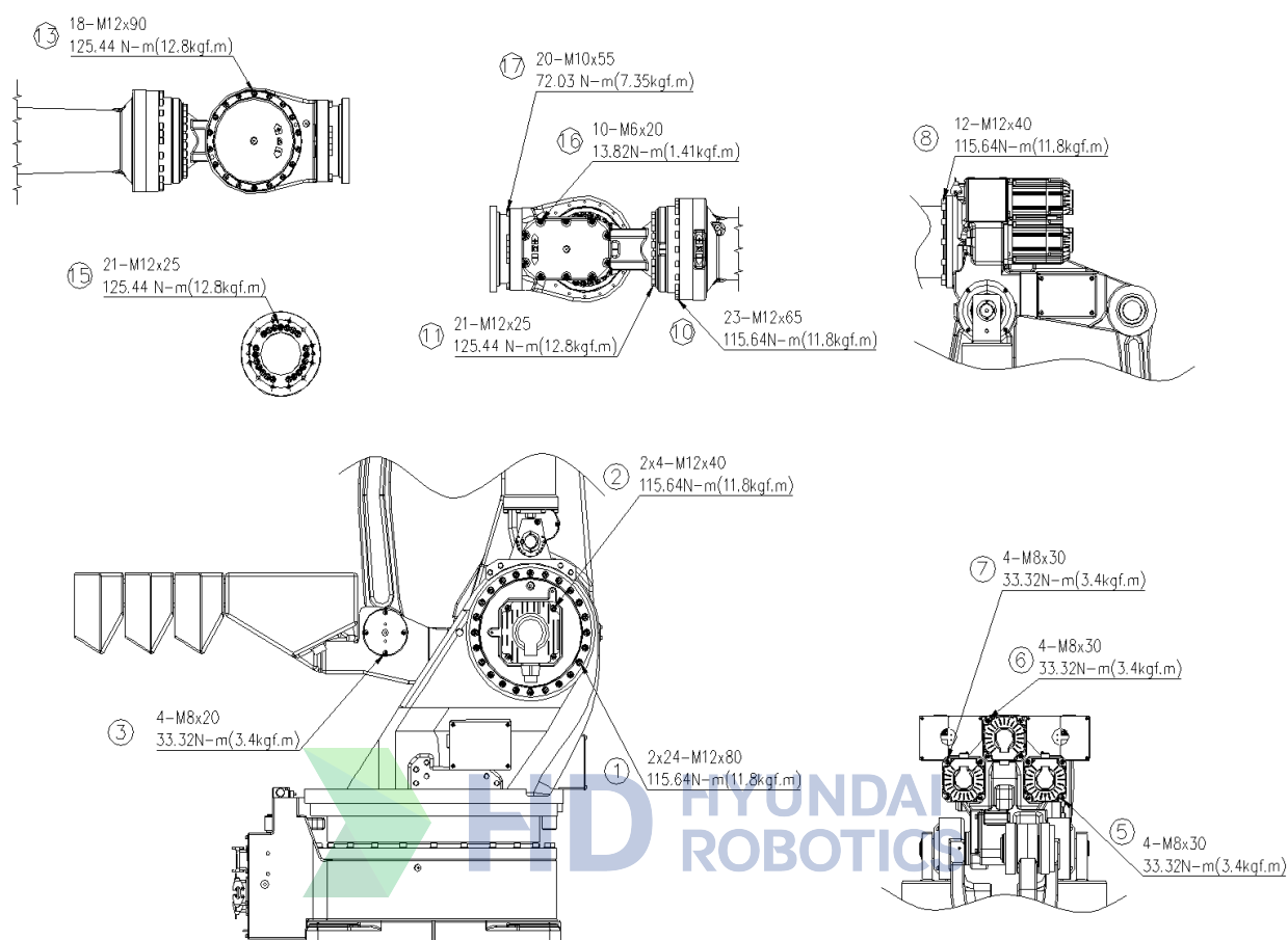
图 4.2 主要螺栓的检查部位 [HX500]
