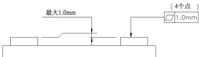
图 3.6 安装面精确度
