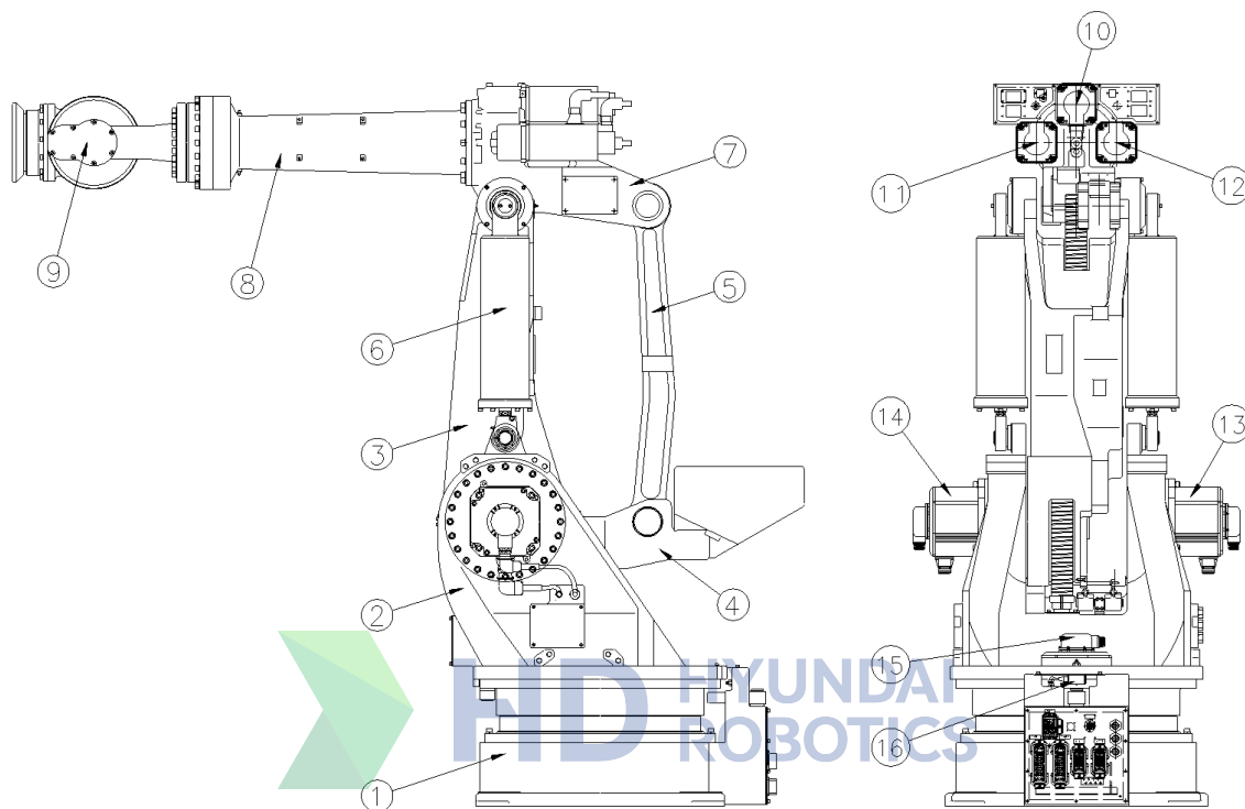
图 3.1 机器人零件名称
