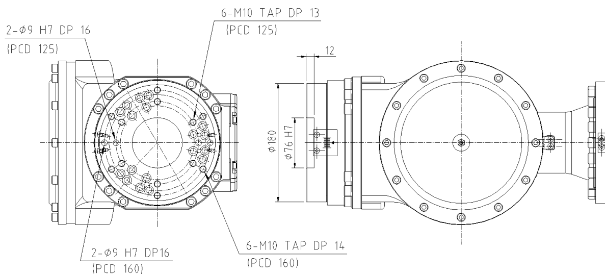
图 2.11 机械腕轴连接面细节：[HX200L]
