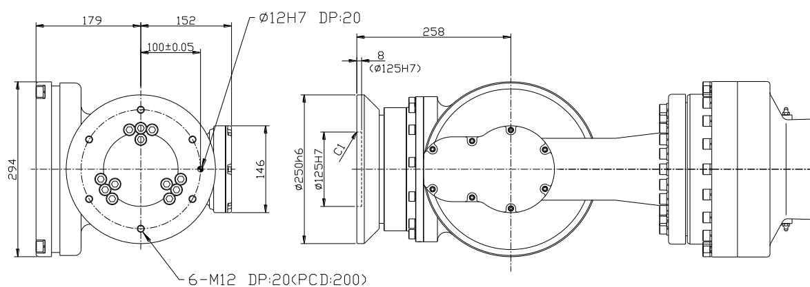
图 2.10 机械腕轴连接面细节：[HX300/HX400/HX300L]
