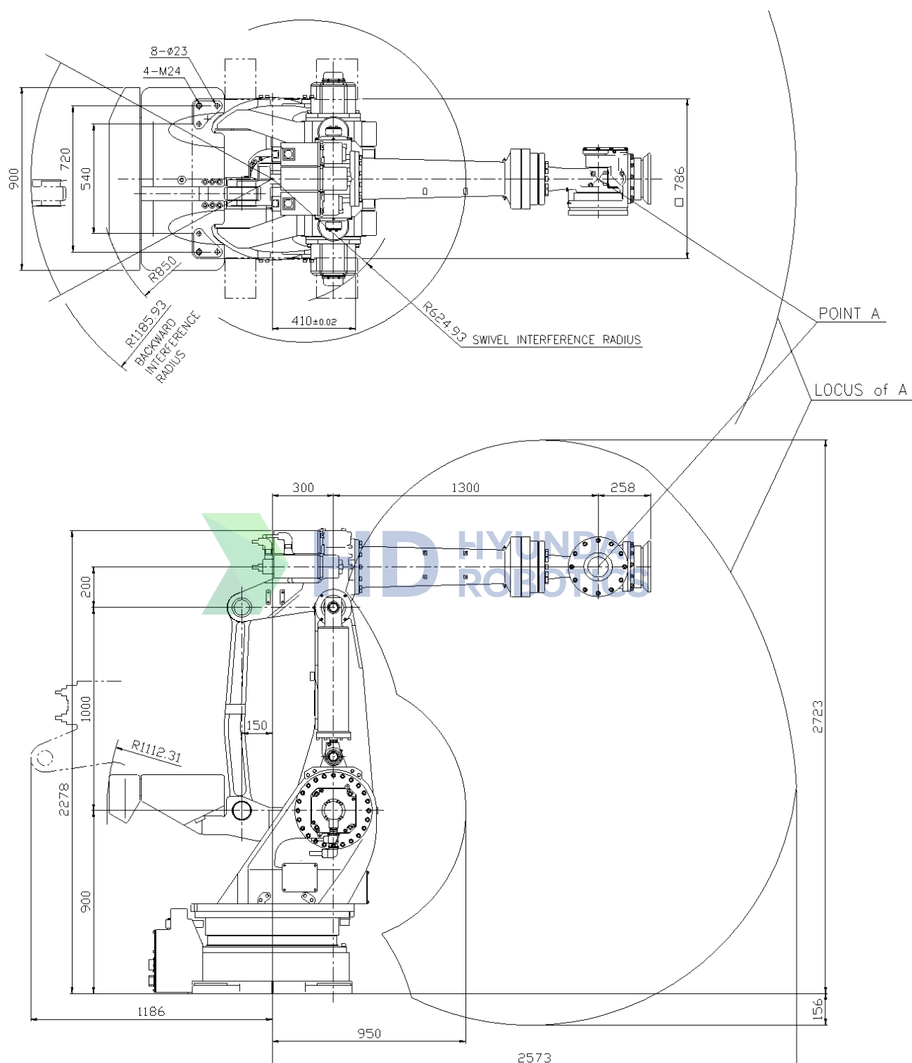
图 2.4 机器人尺寸和工作区间：[HX400]
