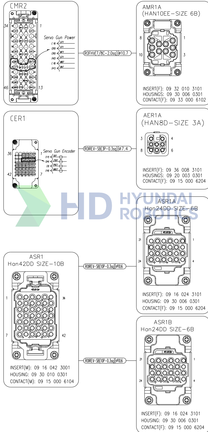
图 2.16 应用连接器细节
