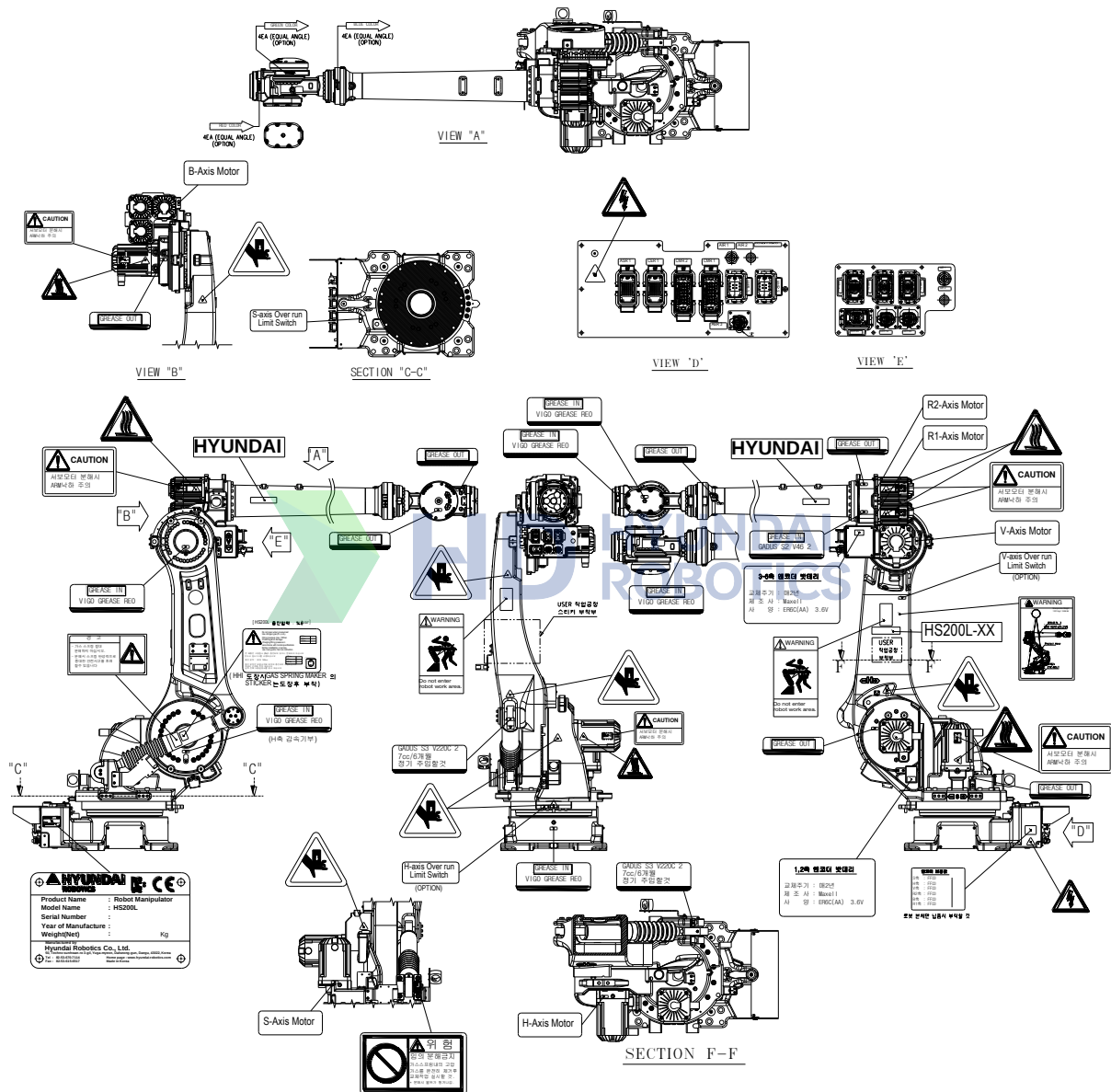
图 3.3 安全标识牌位置 [HS200L]
