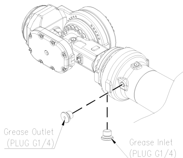
图 5.4 R2 轴减速机润滑油加注/排油口 (HS200L)
