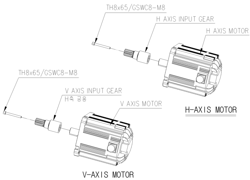
图 6.4 H&amp;V 轴电机安装
