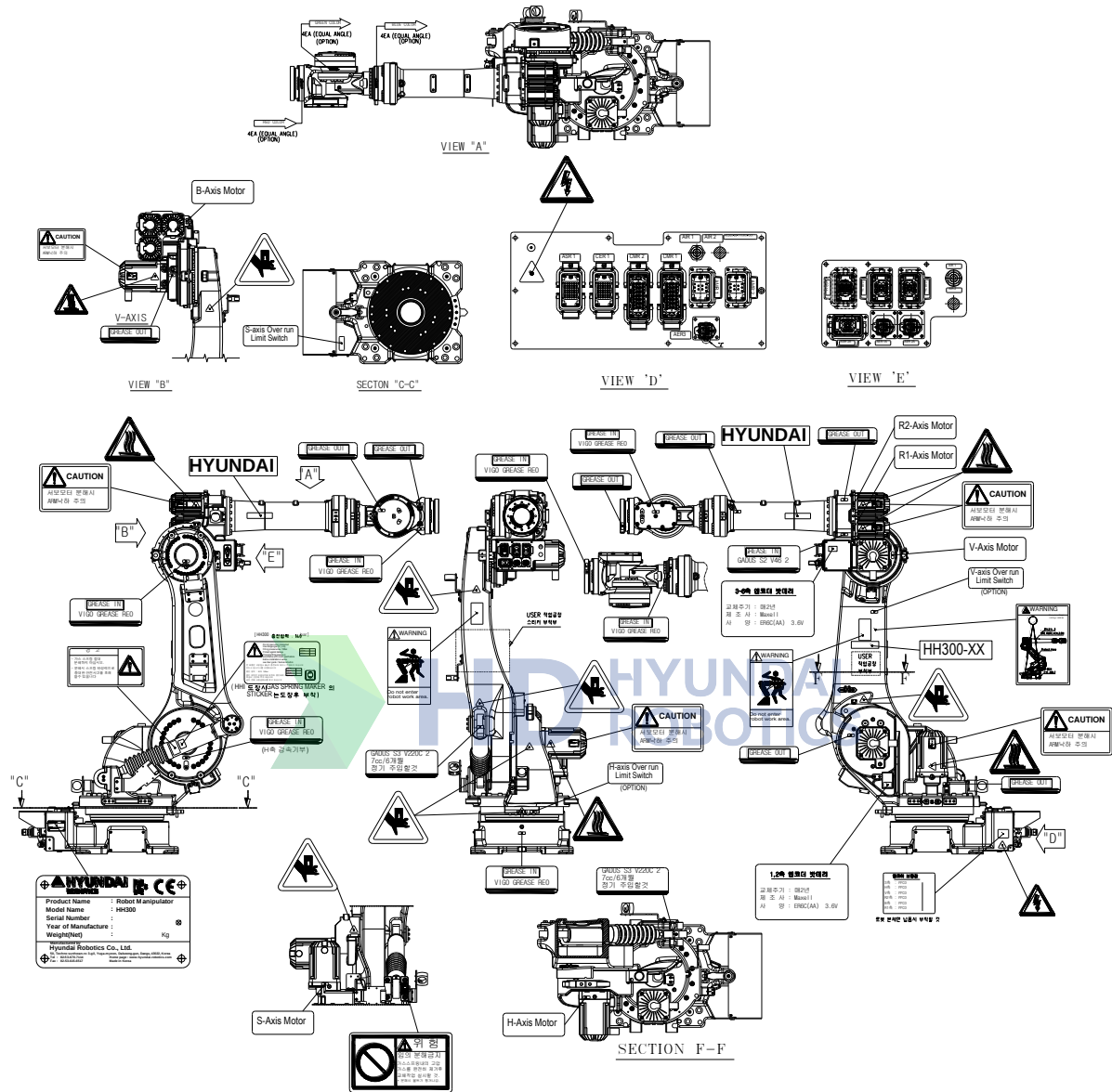
图 3.4 安全标识牌位置 [HS260/HH300]
