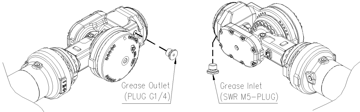
图 5.6 R1 轴减速机润滑油加注/排油口 (HS200L)
