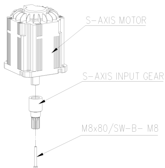
图 6.3 S 轴电机安装
