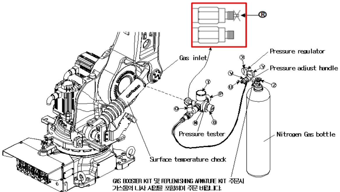
图 9.2 气弹簧充气
