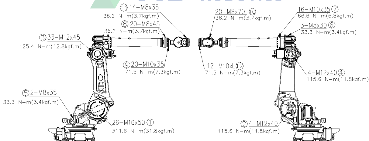
图 4.1 主要螺栓的检查部位 (HS200L)
