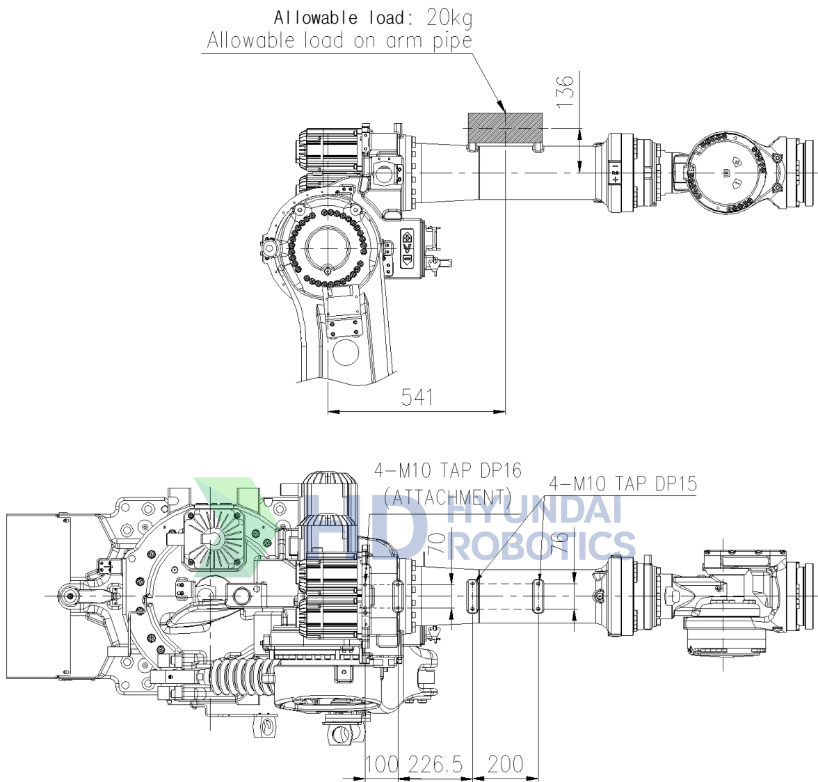
图 2.9 上机械臂支撑连接面细节 [HS260/HH300]
