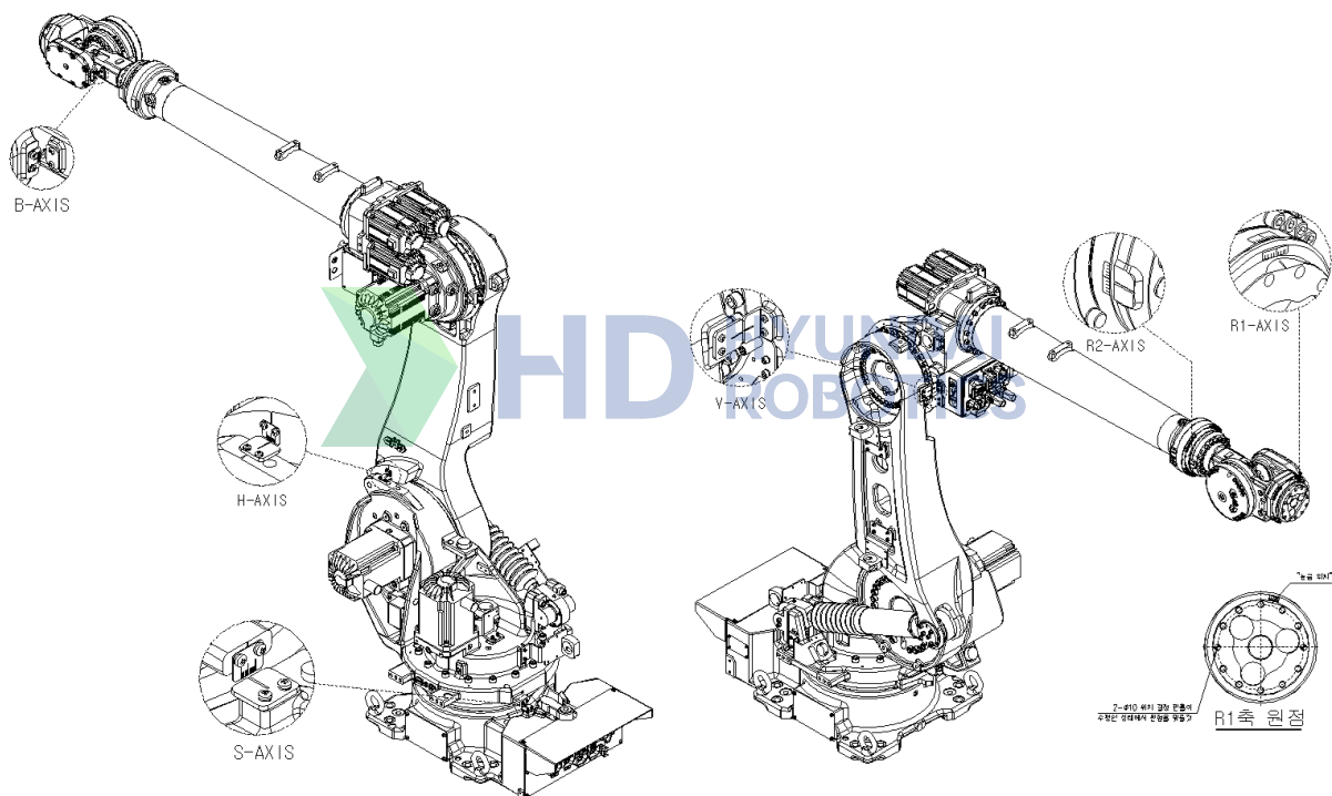
图 6.6 归零设定的方法 (HS200L)
