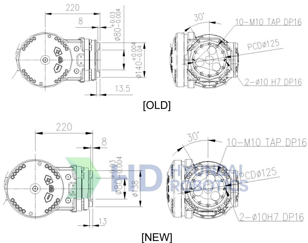
图 2.6 机械腕轴连接面细节: [HS200L]
