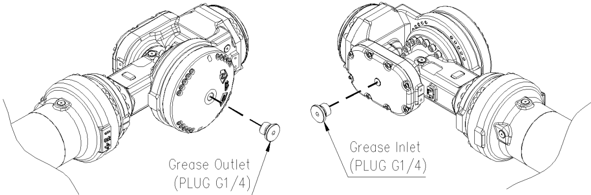
图 5.5 B 轴减速机润滑油加注/排油口 (HS200L)
