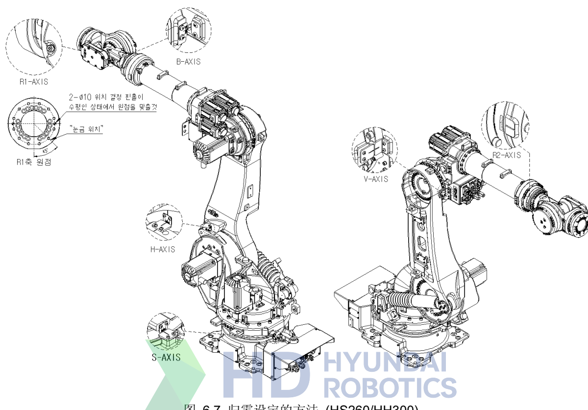
图 6.7 归零设定的方法 (HS260/HH300)
