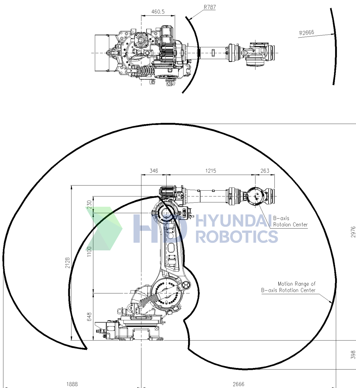
图 2.4 机器人尺寸和工作区间: [HS260/HH300]
