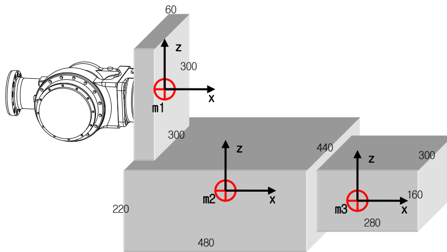
图 3.16 3-D 负载模型 3-D 形状
