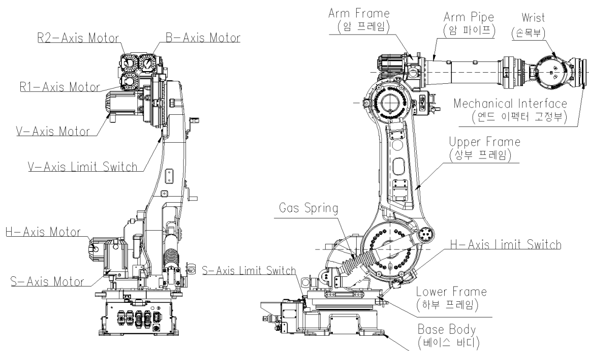
图 3.2 机器人零件名称 [HS260/HH300]
