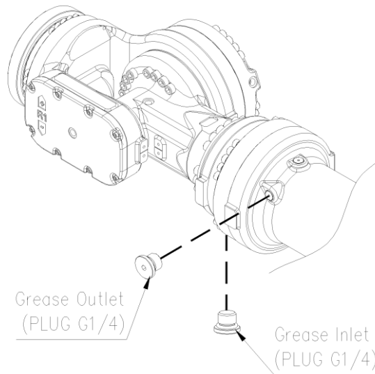
图 5.7 R2 轴减速机润滑油加注/排油口 (HS260/HH300)
