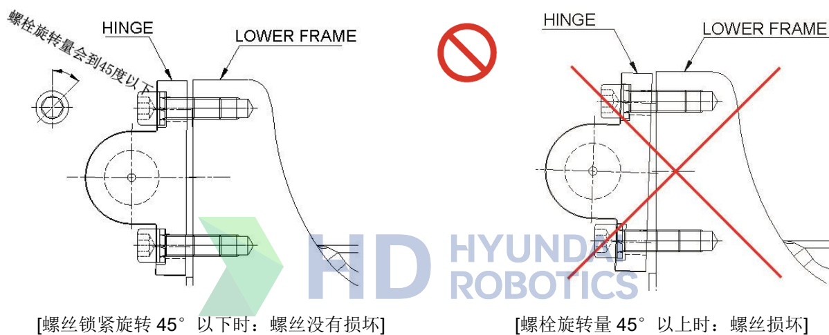
图 9.7 安装/拆卸气弹簧 HINGE 螺栓时的注意事项
