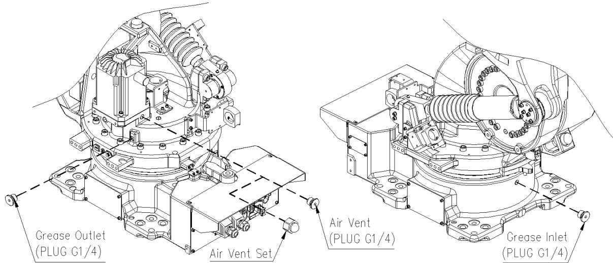
图 5.1 S 轴减速机润滑油加注/排油口
