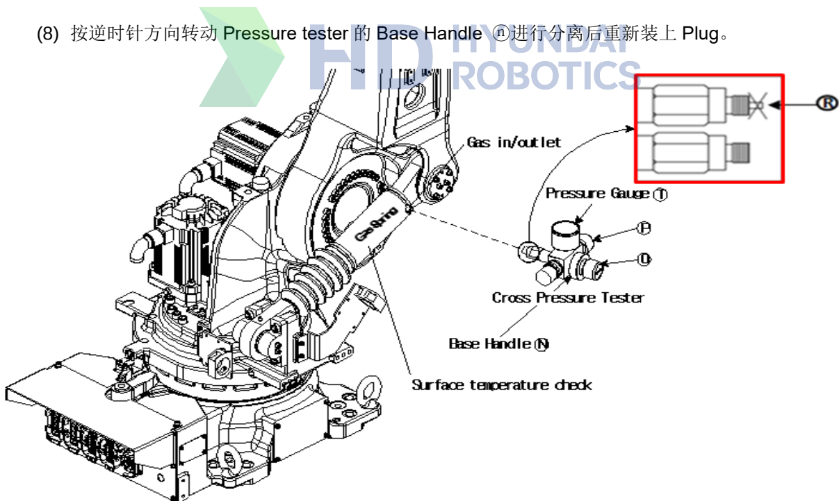
图 9.1 确认气弹簧压力
