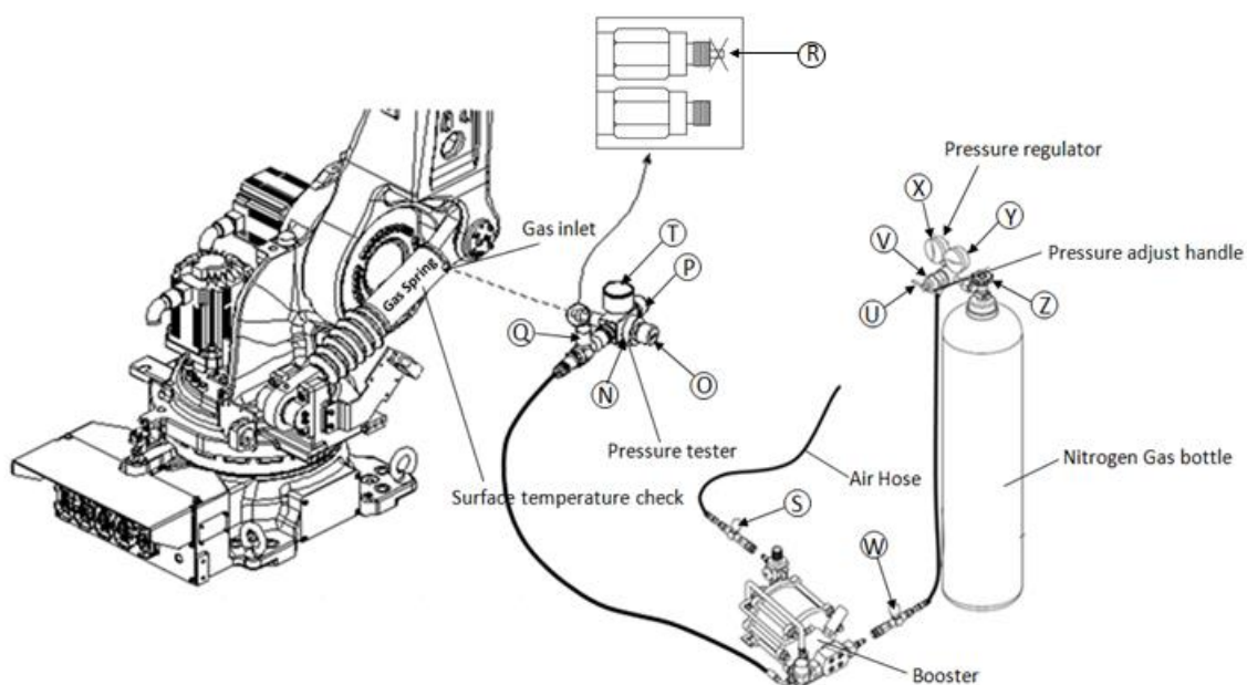
图 9.3 增压机(booster)气弹簧加气
