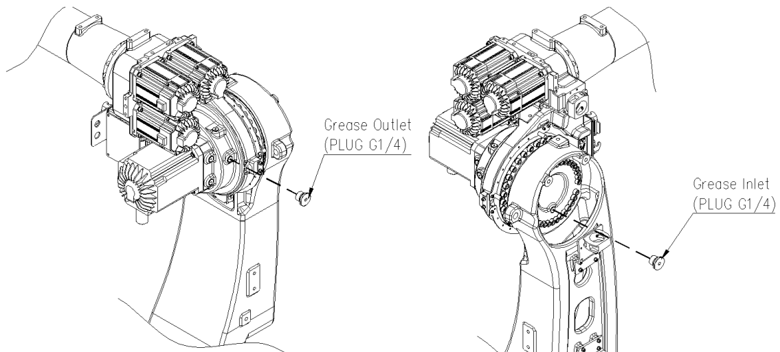
图 5.3 V 轴减速机润滑油加注/排油口
