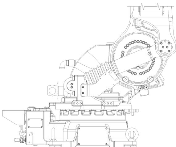
图 9.6 气弹簧组装姿势
