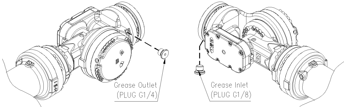
图 5.9 R1 轴减速机润滑油加注/排油口 (HS260/HH300)
