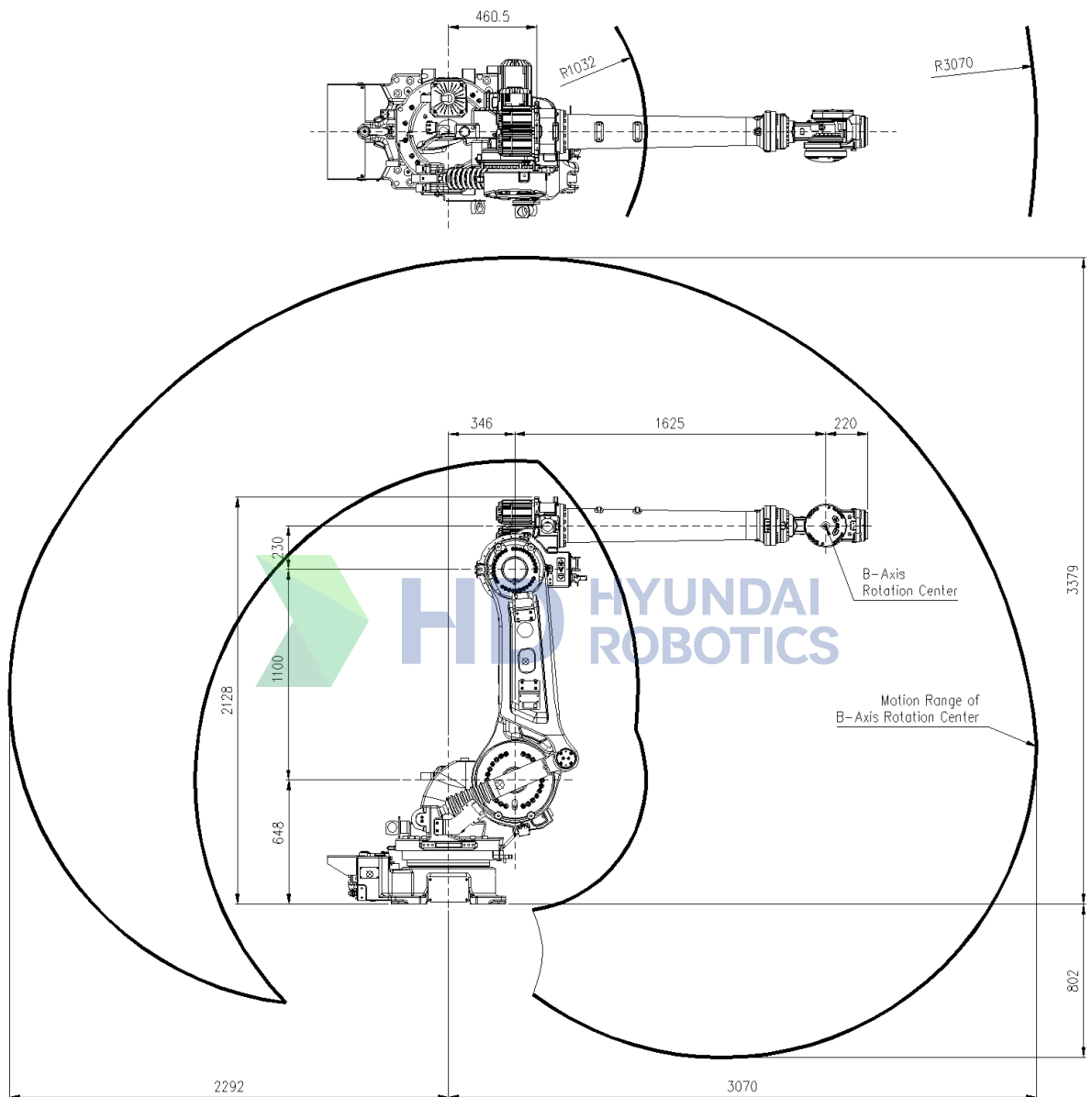
图 2.3 机器人尺寸和工作区间: [HS200L]
