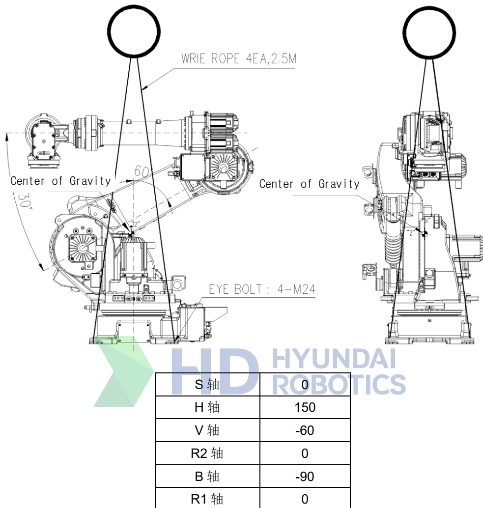
图 3.6 使用吊车 [HS260/HH300]
