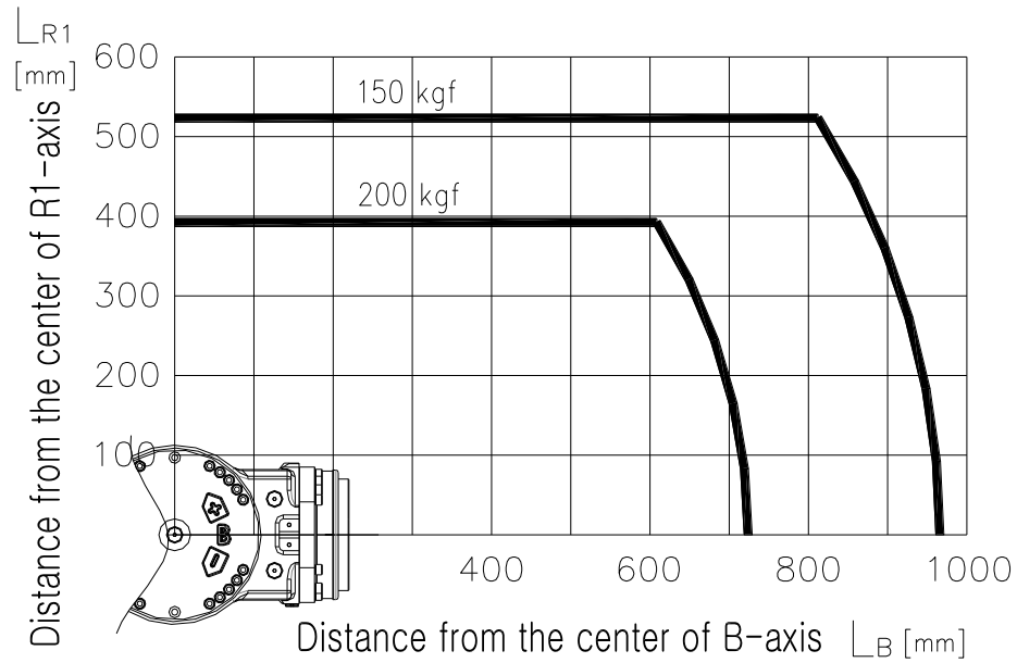
图 3.11 腕轴转矩图: [HS200L]
