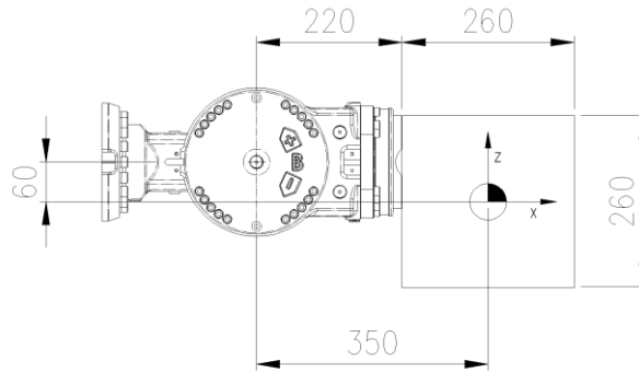
图 3.14 2-D 负载模型
