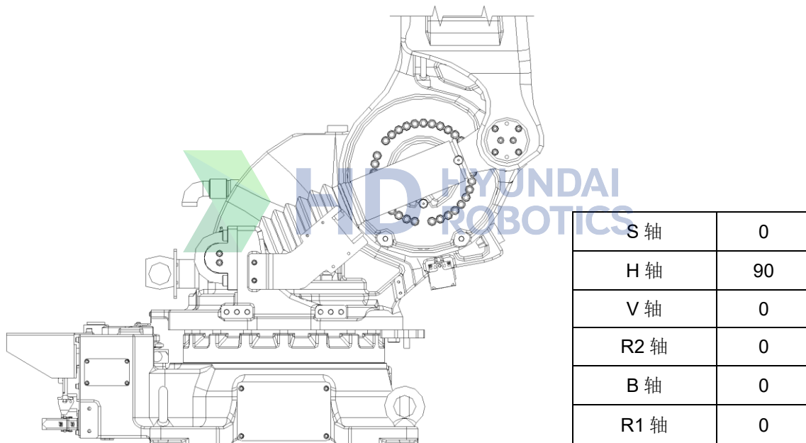
图 8.1 气弹簧分离姿势
