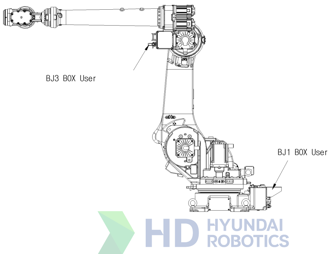
图 10.1 机械手配置
