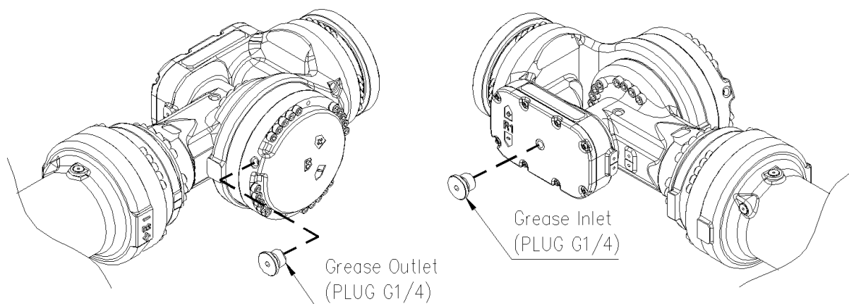
图 5.8 B 轴减速机润滑油加注/排油口 (HS260/HH300)
