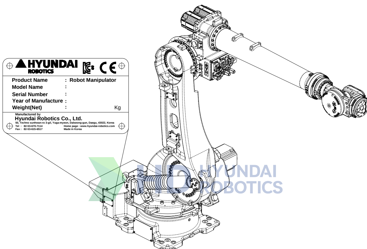
图 2.2 机器人识别铭牌的位置
