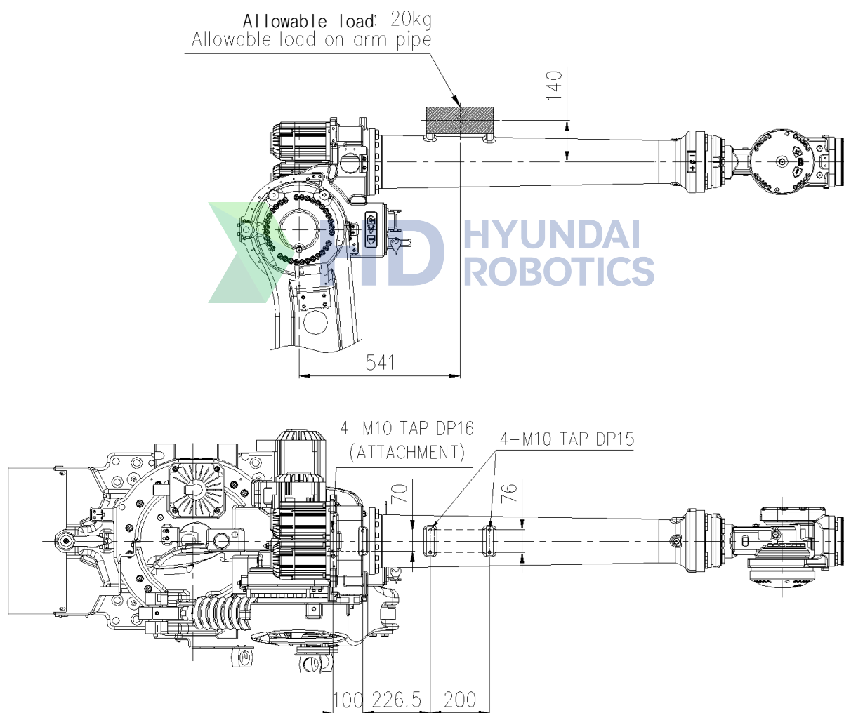
图 2.8 上机械臂支撑连接面细节 [HS200L]
