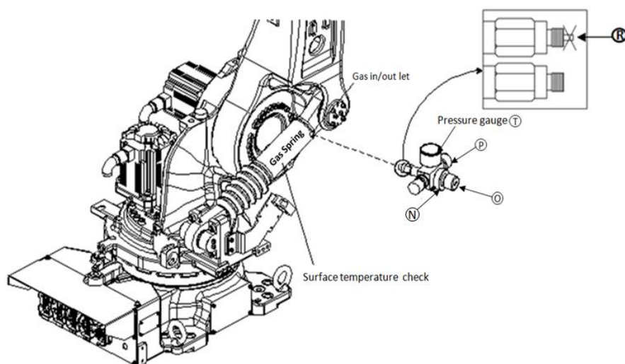
图 9.4 气弹簧放气
