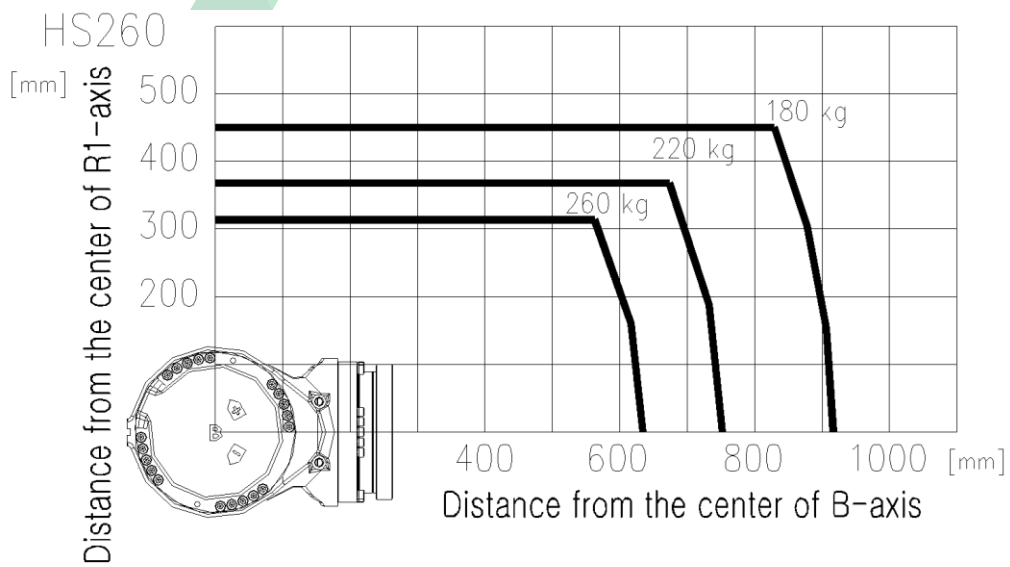
图 3.12 腕轴转矩图: [HS260]
