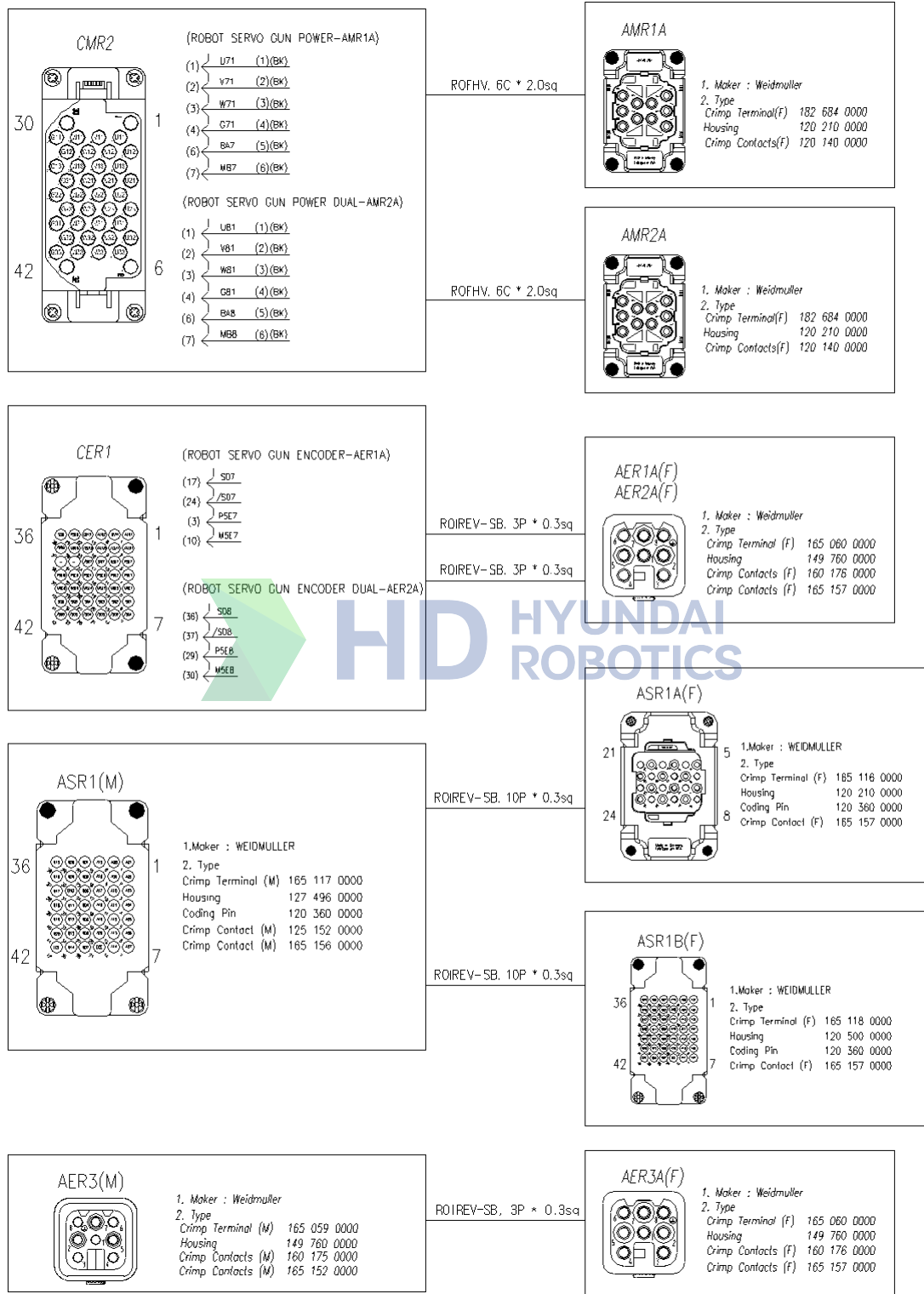
图 2.11 工作线路和检查线路图
