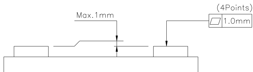
图 3.8 安装面精确度
