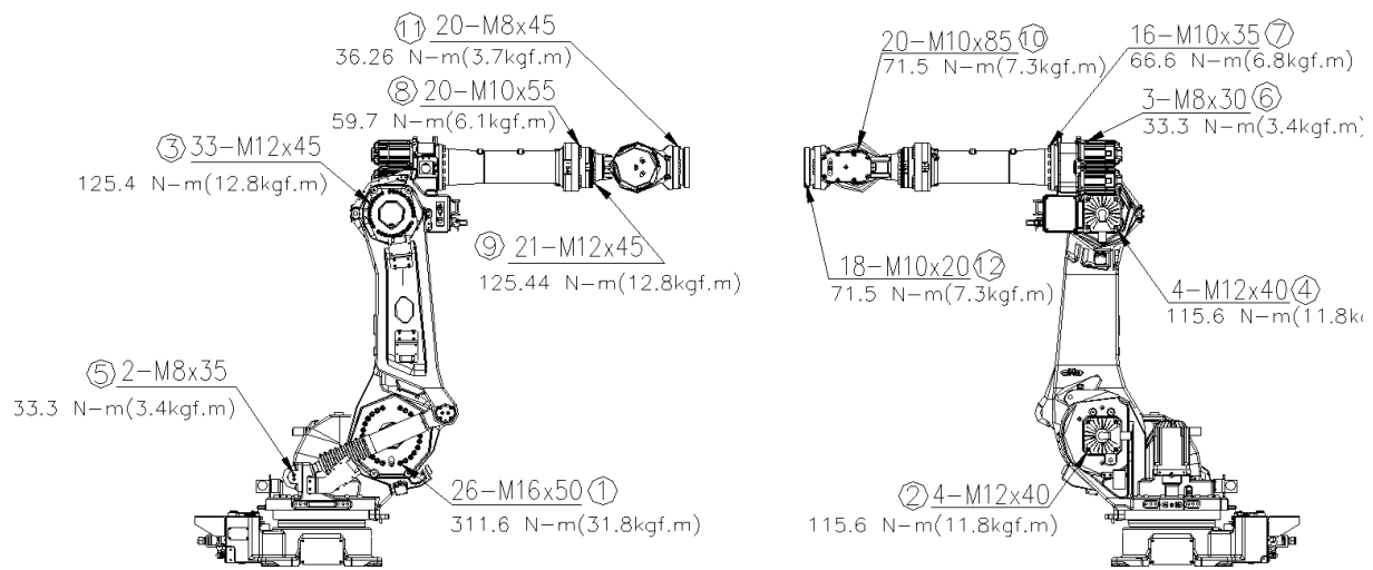
图 4.2 主要螺栓的检查部位 (HS260/HH300)
