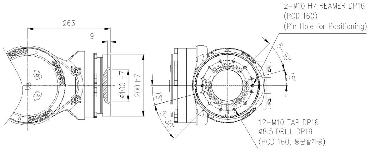
图 2.7 机械腕轴连接面细节: [HS260/HH300]
