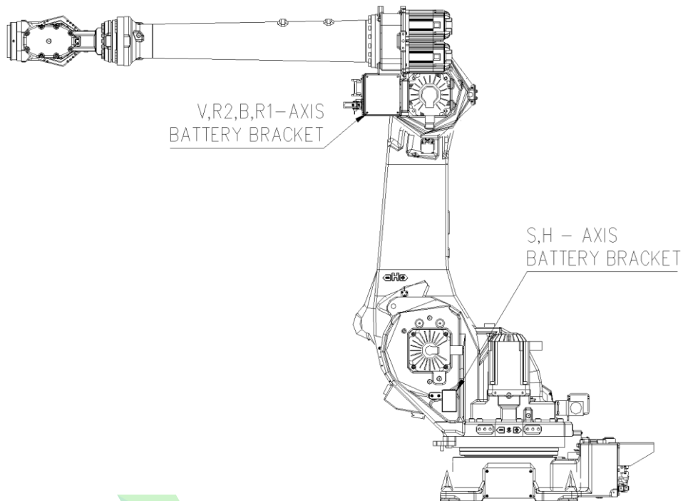
图 5.12 电池的位置
