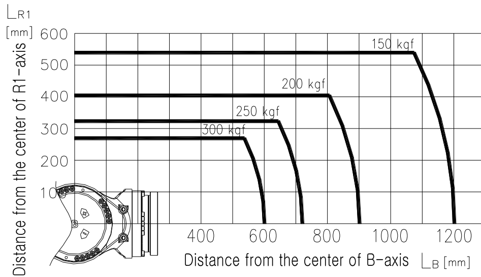
图 3.13 腕轴转矩图 [HH300]
