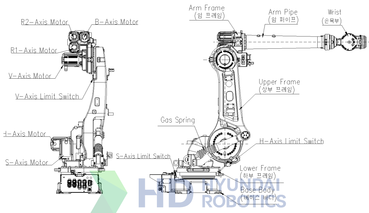
图 3.1 机器人零件名称 [HS200L]
