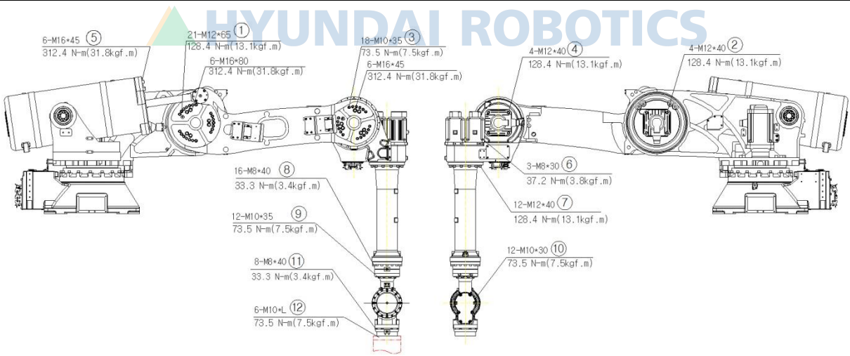
图 4.1 主要螺栓的检查部位 [HS165S]
