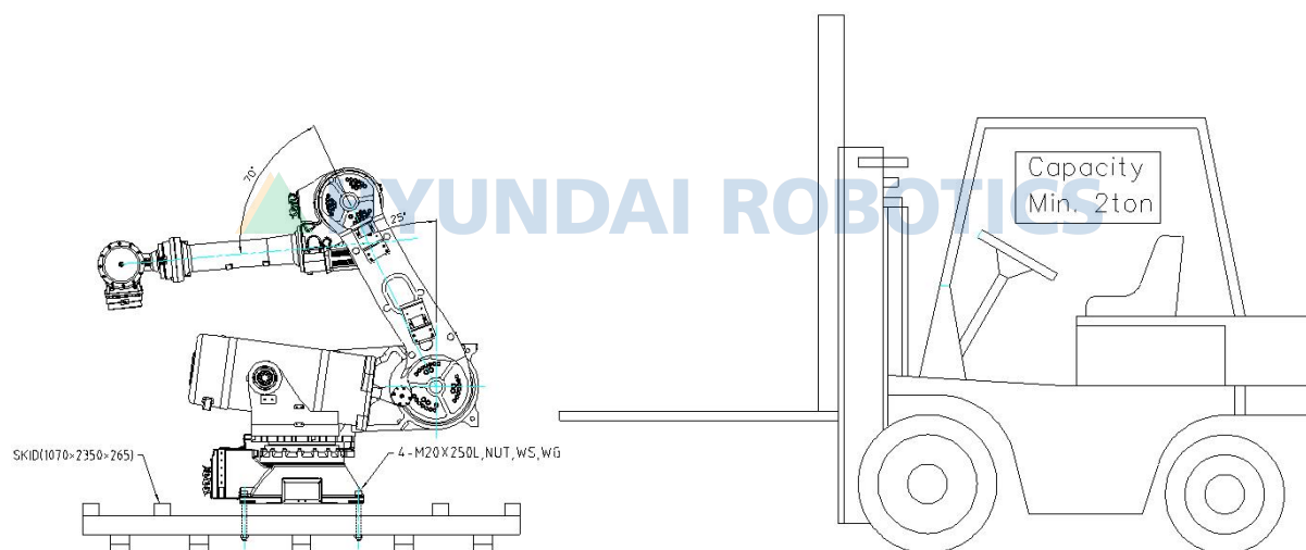
图 3.4 运送方法：利用叉车 [HS165S/HS200S]
