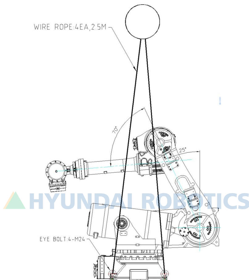
图 3.3 运送方法：使用吊车 [HS165S/HS200S]
