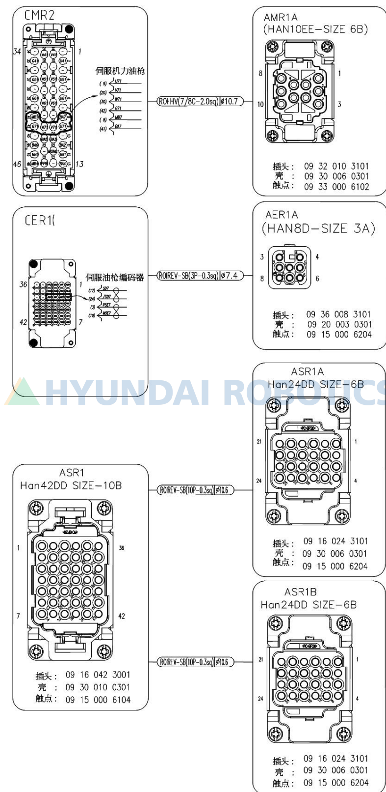
图 2.9 应用连接器细节 : [HS165S/HS200S]
