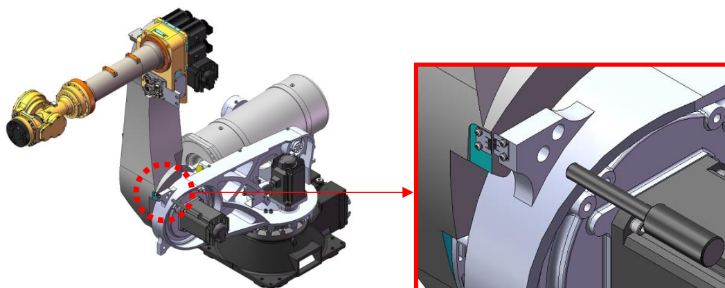
图 6.1 第 1 手臂(H 轴)固定用 Pin 的插入位置
