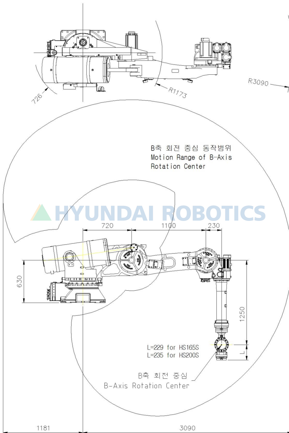
图 2.3 机器人尺寸和工作区间: [HS165S/HS200S]
