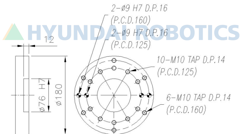
图 2.6 机械腕轴连接面细节: [HS200S]
