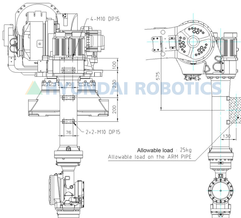
图 2.7 上机械臂支撑连接面细节: [HS165S/HS200S]
