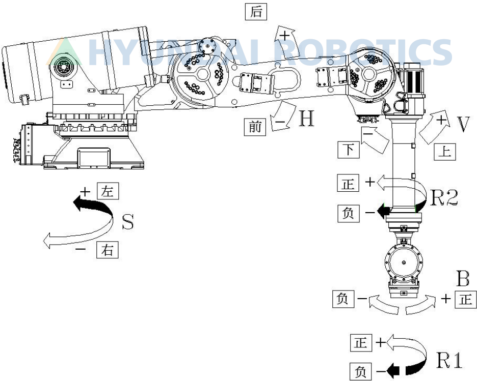
图 2.4 机器人尺寸和轴 [HS165S/HS200S]
