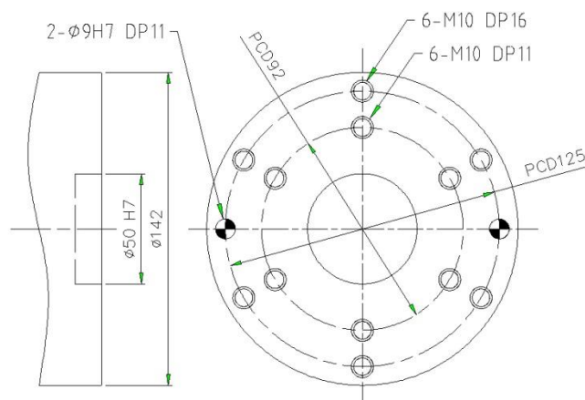
图 2.5 机械腕轴连接面细节: [HS165S]
