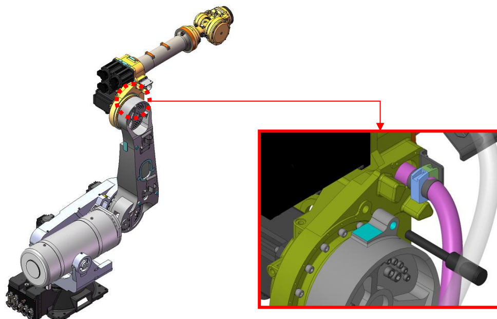
图 6.2 第 2 手臂(V 轴)固定用 Pin 的插入位置
