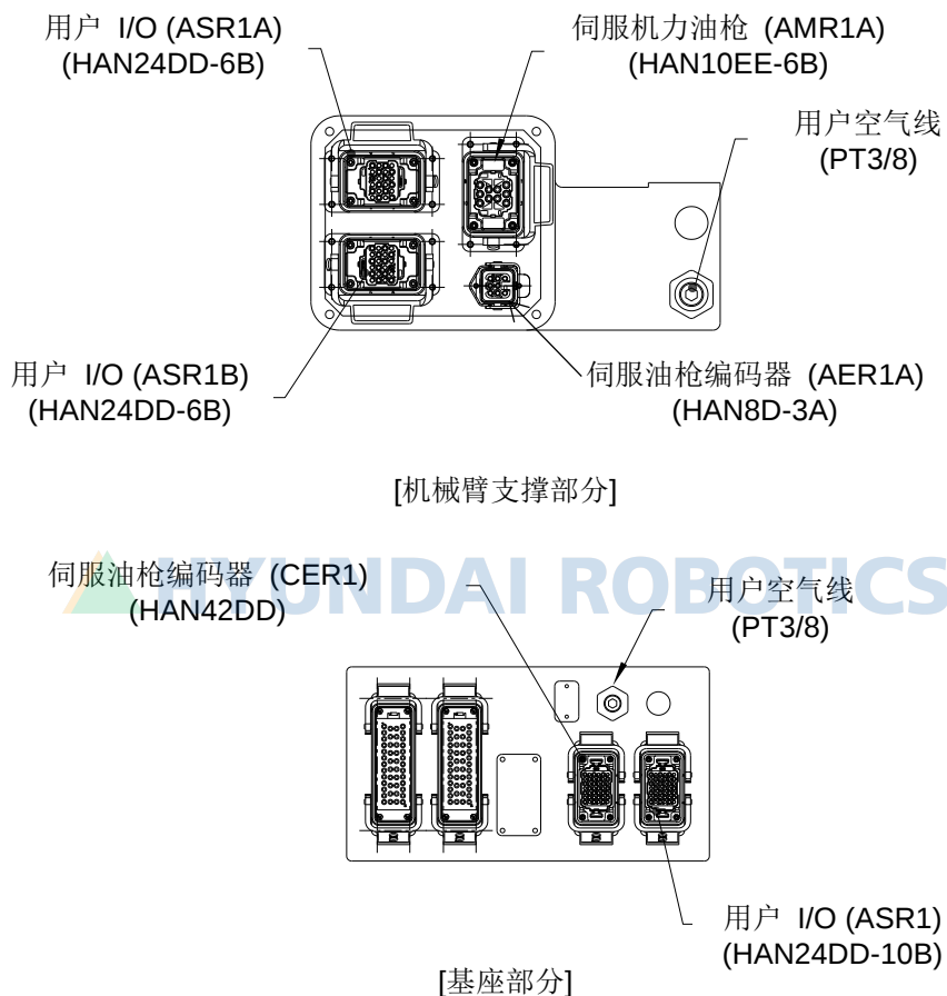
图 2.8 工作线路和检查线路图 : [HS165S/HS200S]
