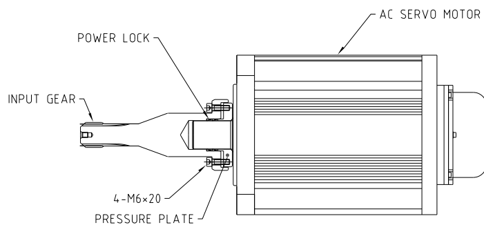
图 6.4 H&amp;V 轴电机安装
