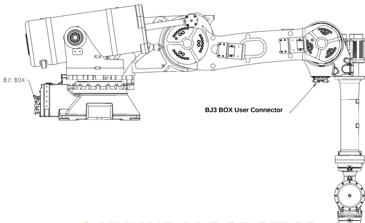
图 9.1 机械手配置
