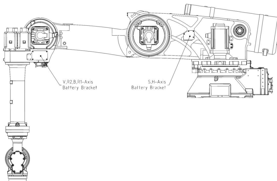
图 5.1 电池的位置
