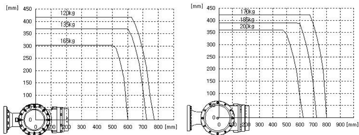
图 3.7 腕轴转矩图:[HS165S], [HS200S]
