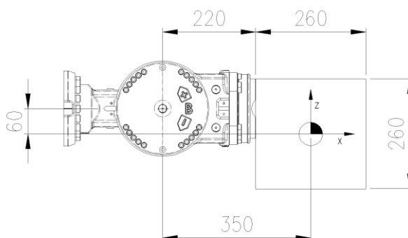
图 3.8 2-D 负载模型
