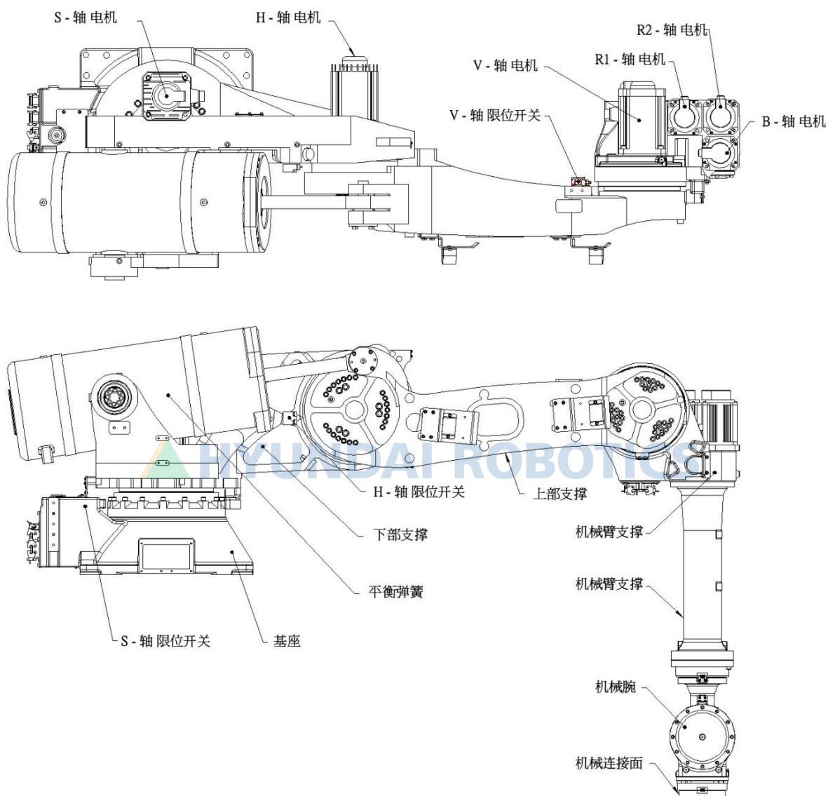
图 3.1 机器人零件名称
