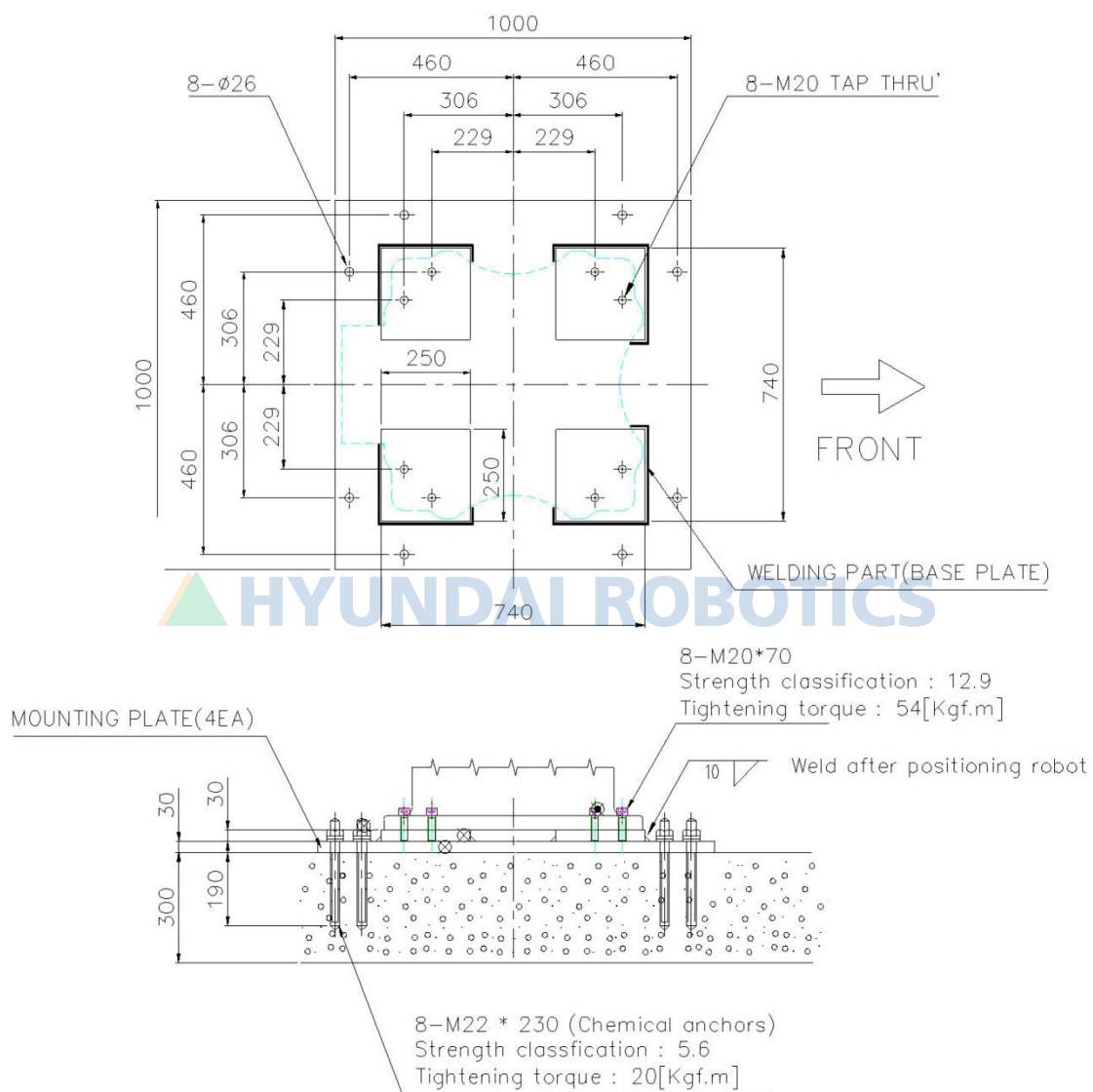
图 3.6 机器人安装尺寸 : [HS165S/HS200S]
