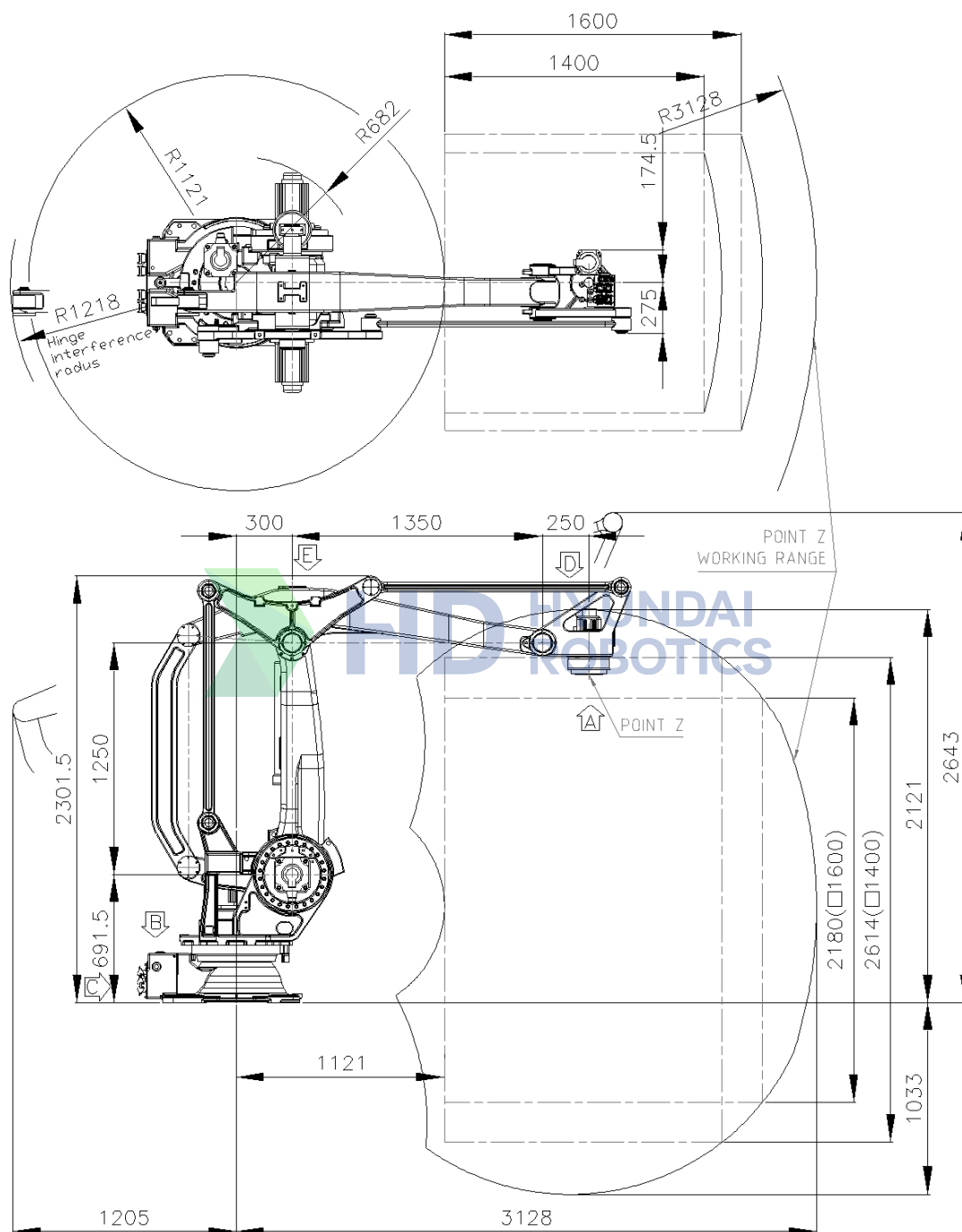
图 2.3 机器人外形尺寸及工作区域
