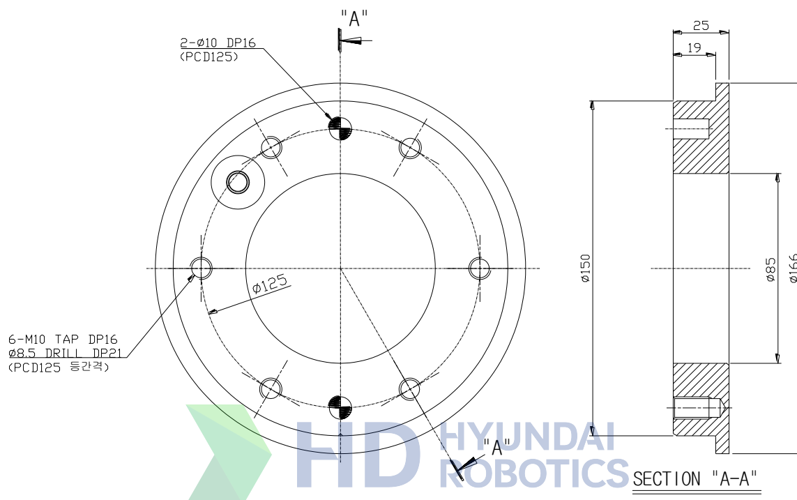
图 2.7 手腕轴接合部详图
