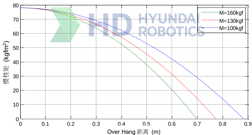
图 3.8 手腕轴负荷条件
