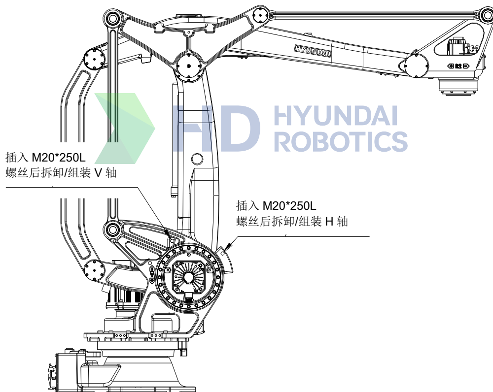
图 6.1 H、V 轴 ARM 降落防止方法(HP160)
