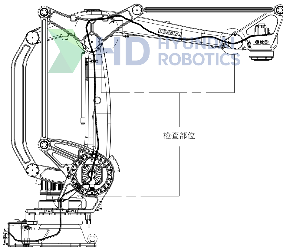
图 4.3 电缆检查部位
