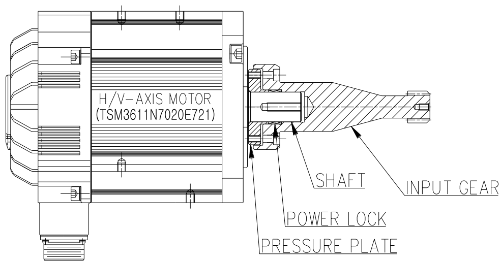
图 6.3 H &amp; V 轴电机总成
