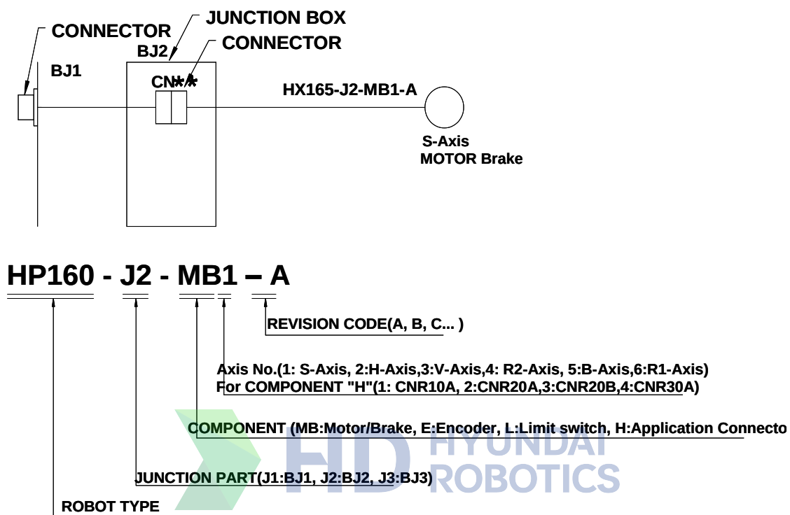
图 5.1 机体内配线符号说明
