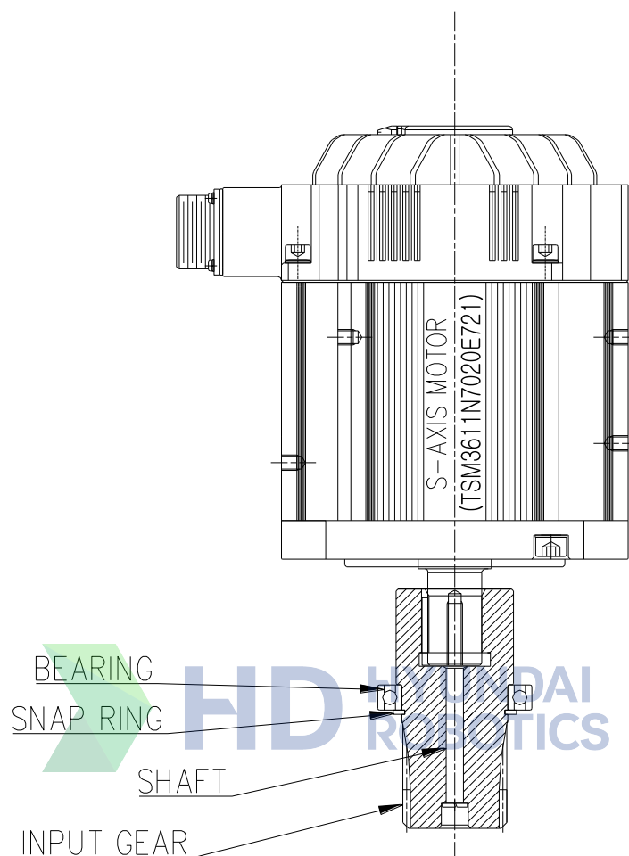
图 6.2 S 轴电机总成
