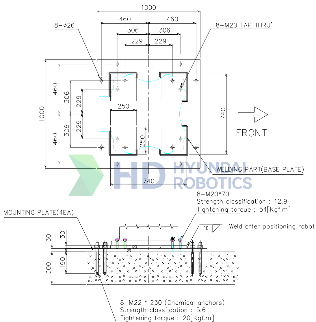
图 3.6 机器人机体安装尺寸
