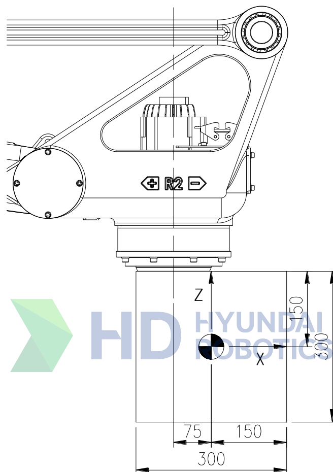
图 3.9 二维负荷型号
