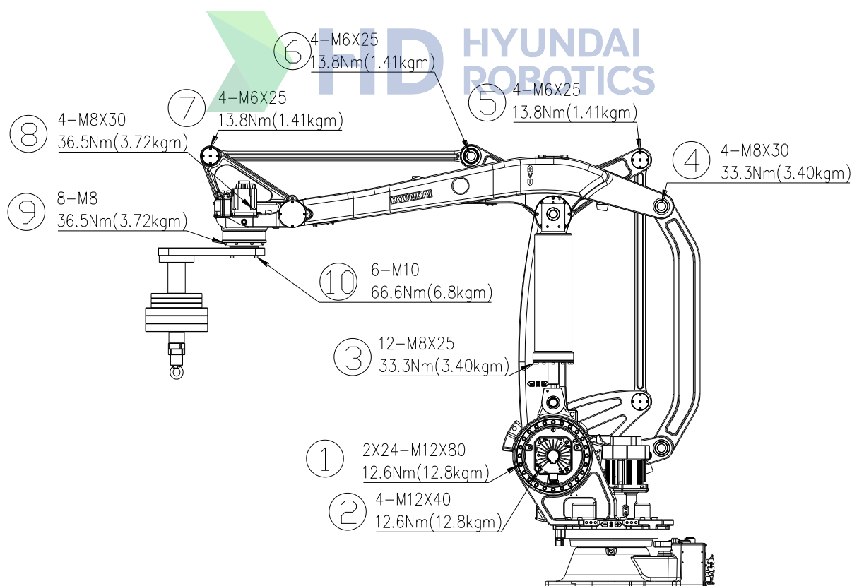
图 4.1 主要螺丝检查部位
