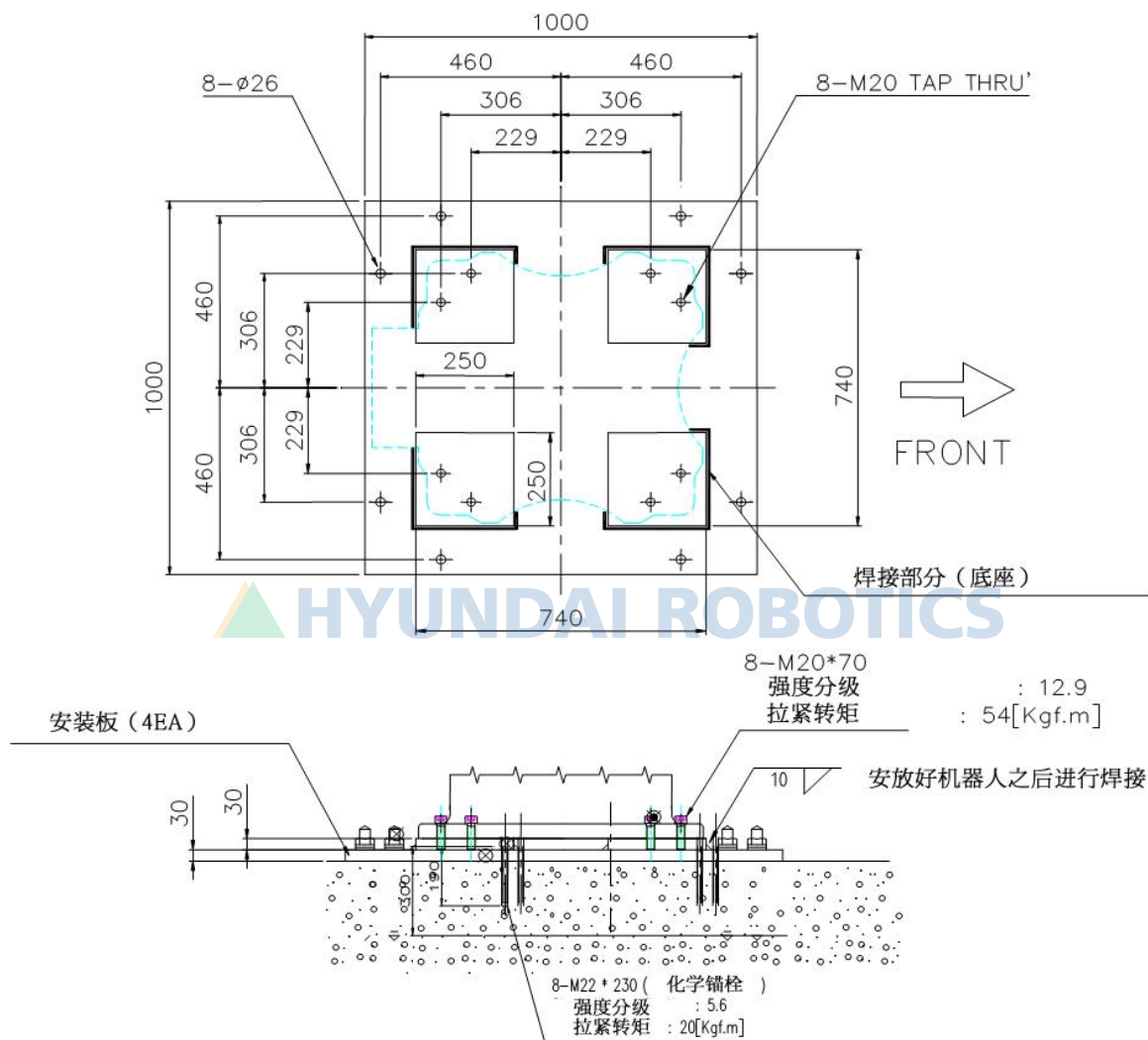
图 3.6 机器人安装尺寸 : [HH100SL]
