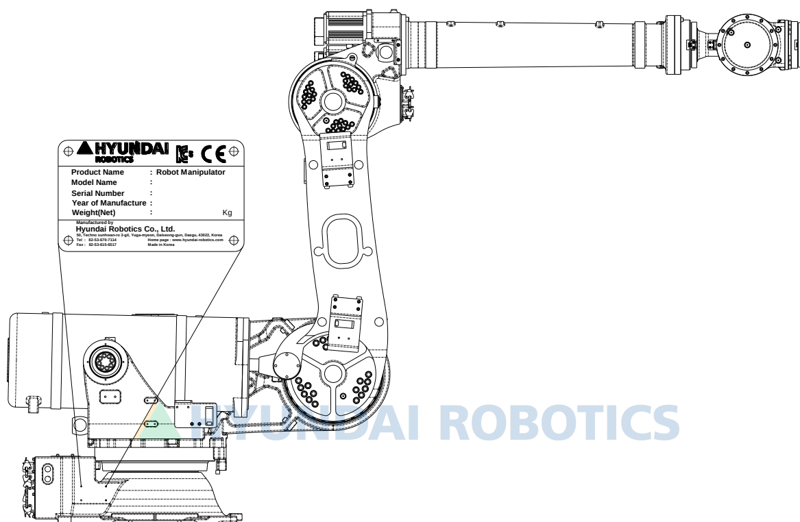
图 2.2 机器人识别铭牌的位置
