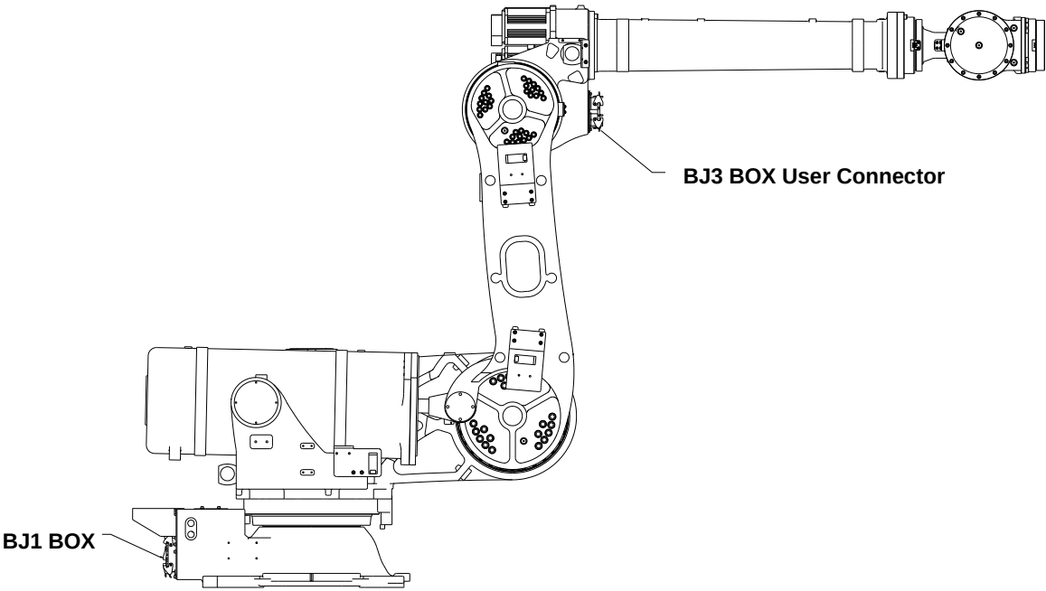
图 9.1 机械手配置
