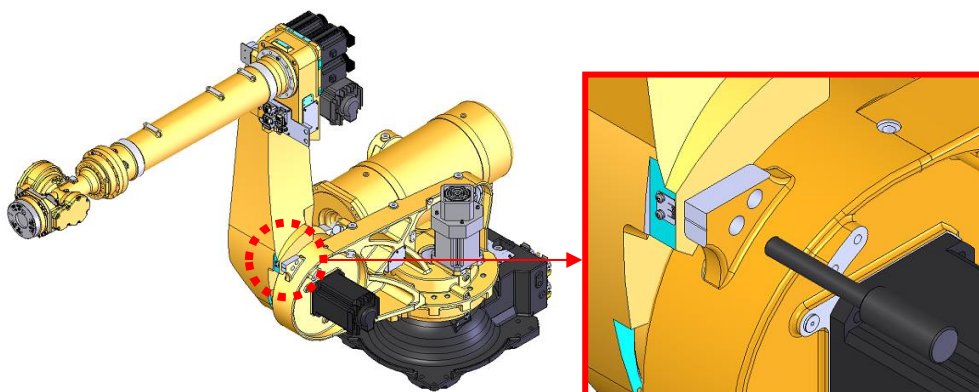
图 6.1 第 1 臂 (H 轴) 固定销的插入位置
