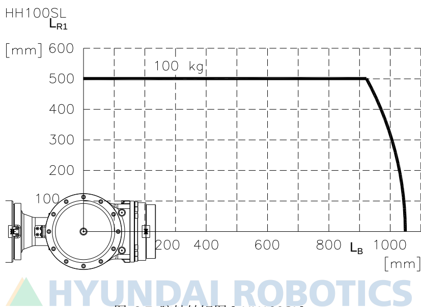
图 3.7 腕轴转矩图:[ HH100SL]
