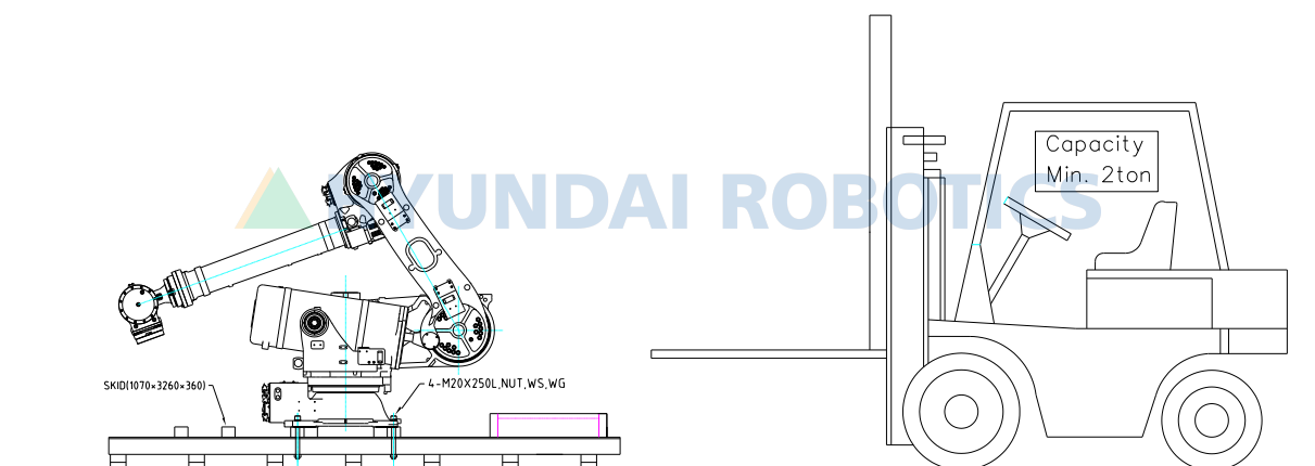
图 3.4 运送方法：利用叉车 [HH100SL]
