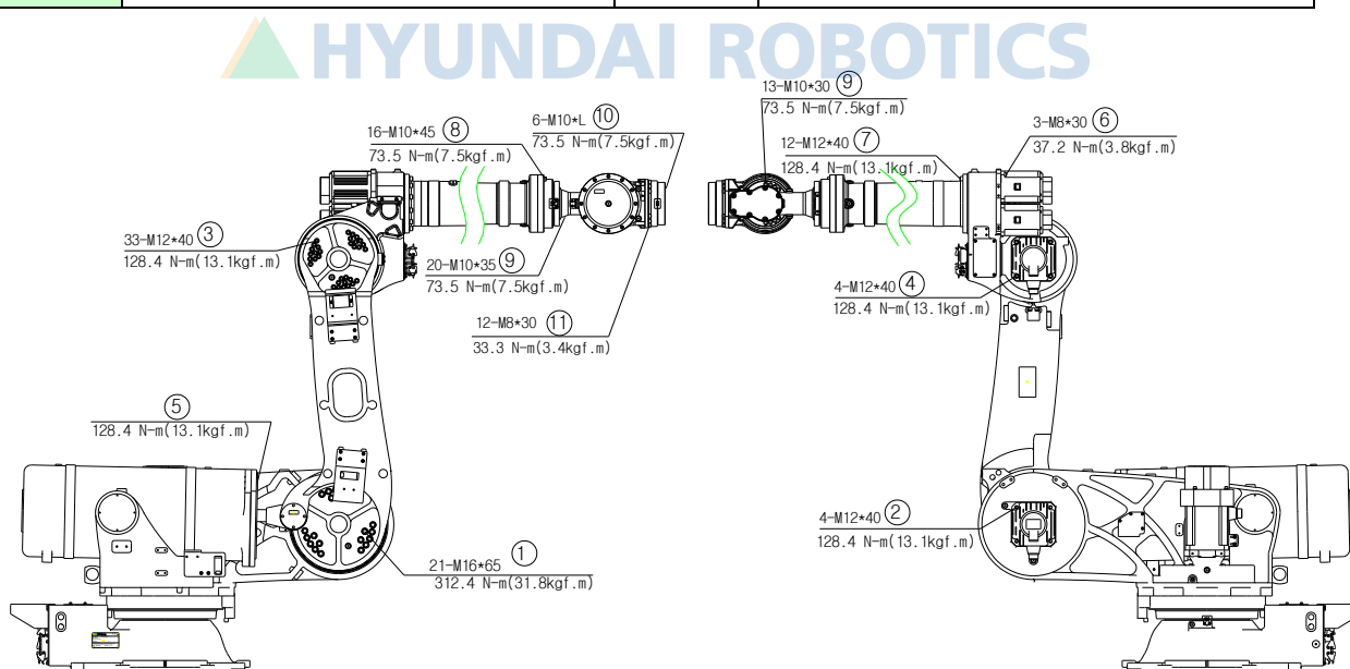
图 4.1 主要螺栓的检查部位
