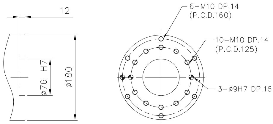
图 2.5 机械腕轴连接面细节
