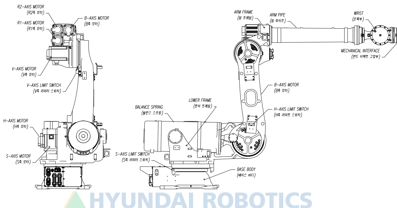
图 3.1 机器人零件名称
