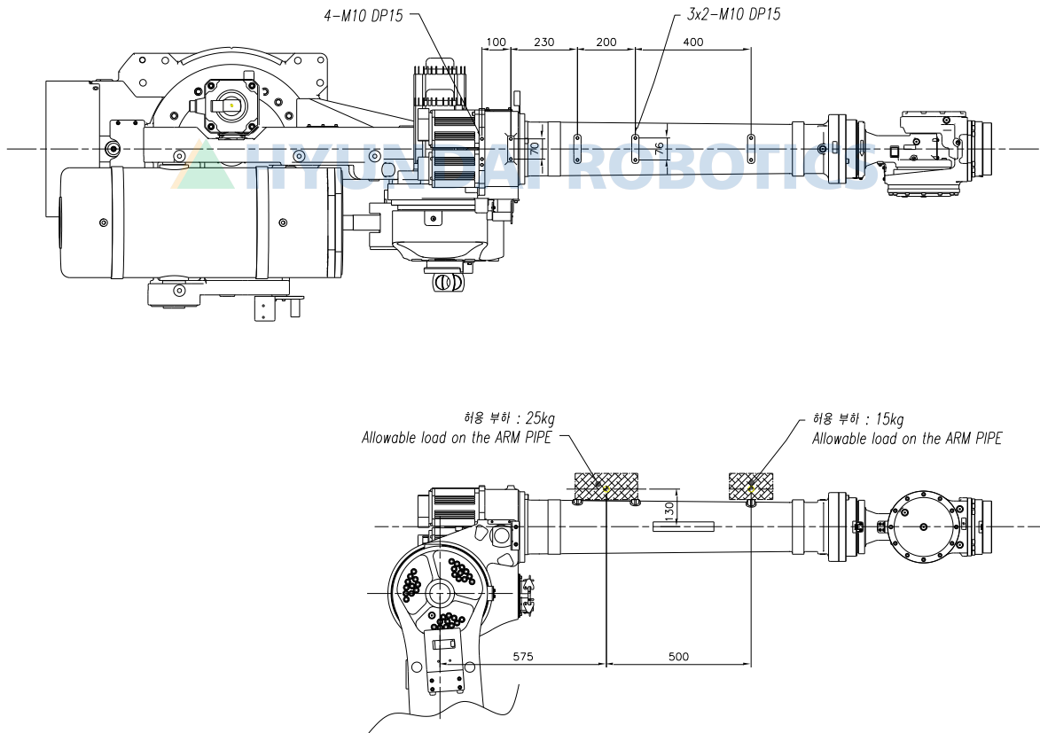
图 2.6 上机械臂支撑连接面细节
