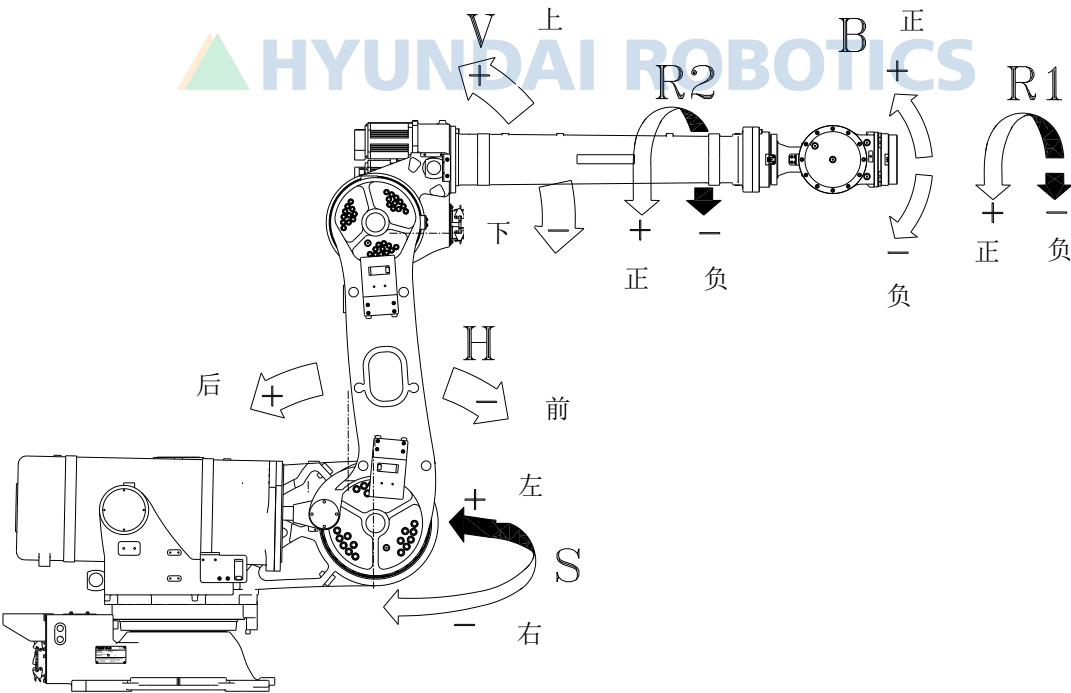
图 2.4 机器人尺寸和轴
