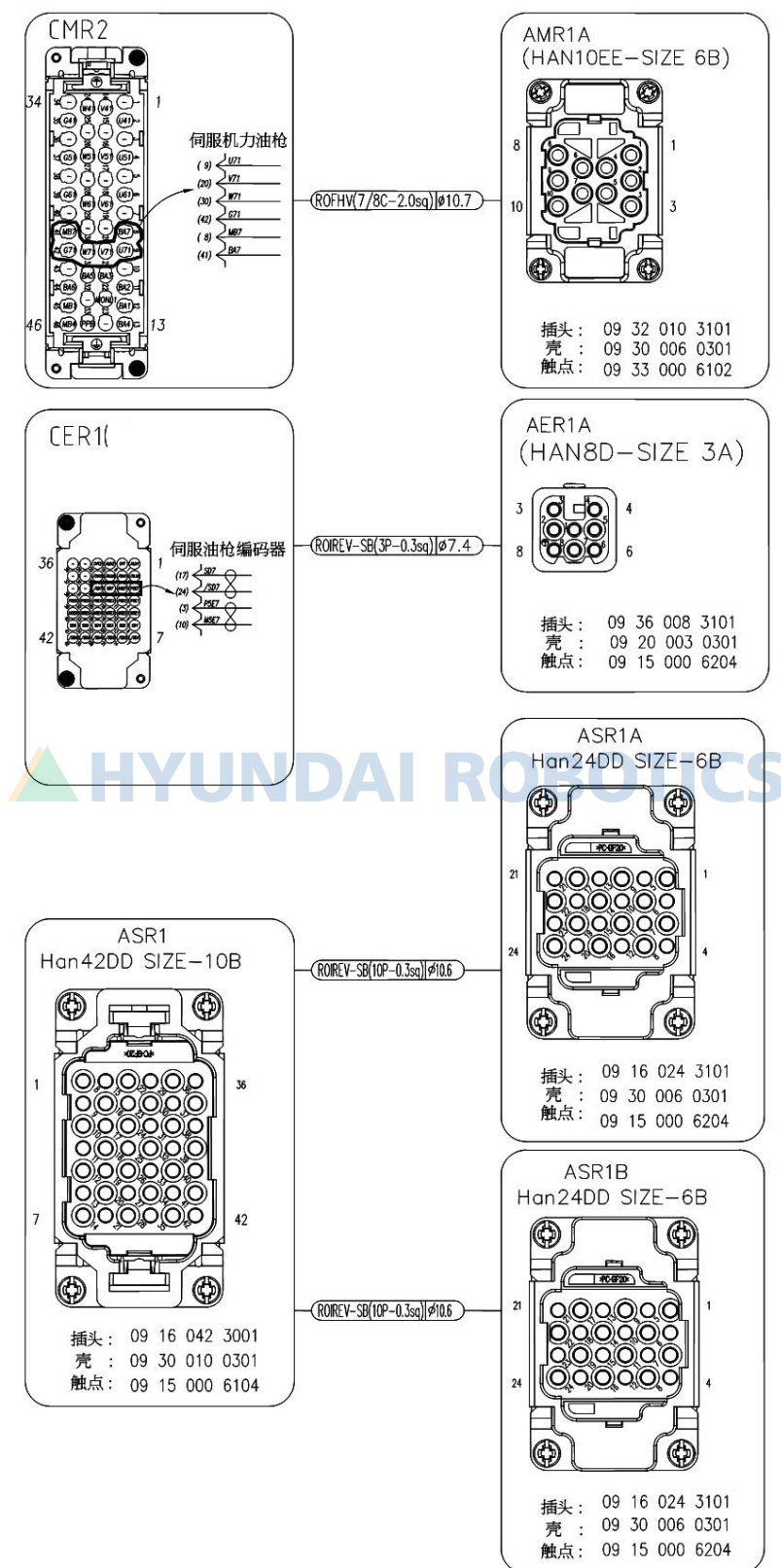
图 2.8 应用连接器细节
