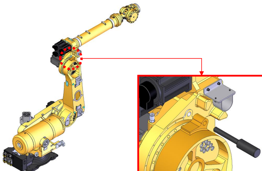
图 6.2 第 2 臂 (V 轴) 固定销的插入位置
