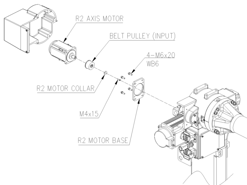
图 6.4 R2 轴电机安装
