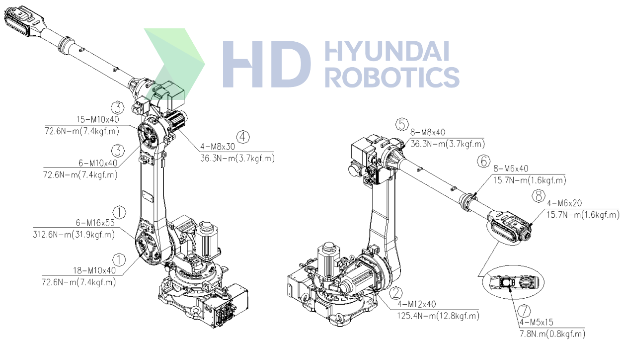
图 4.1 主要螺栓的检查部位 [HH020L]
