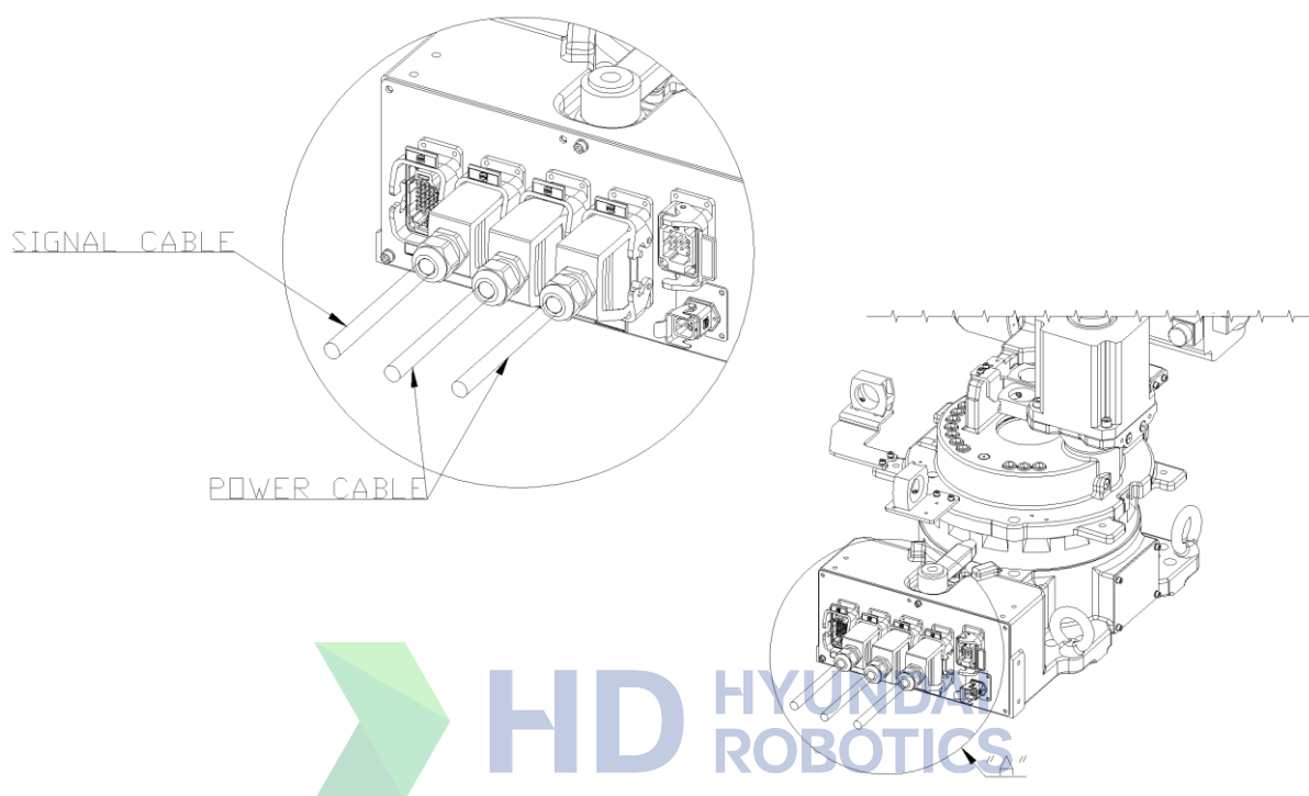
图 3.7 机器人 Cable 连接
