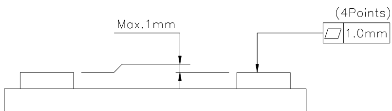
图 3.5 安装面精确度
