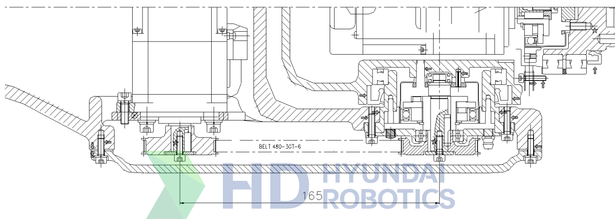
图 4.3 B 轴 Timing Belt 张力检查部位 [HH020L]
