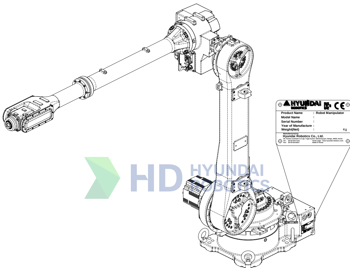
图 2.2 机器人识别铭牌的位置
