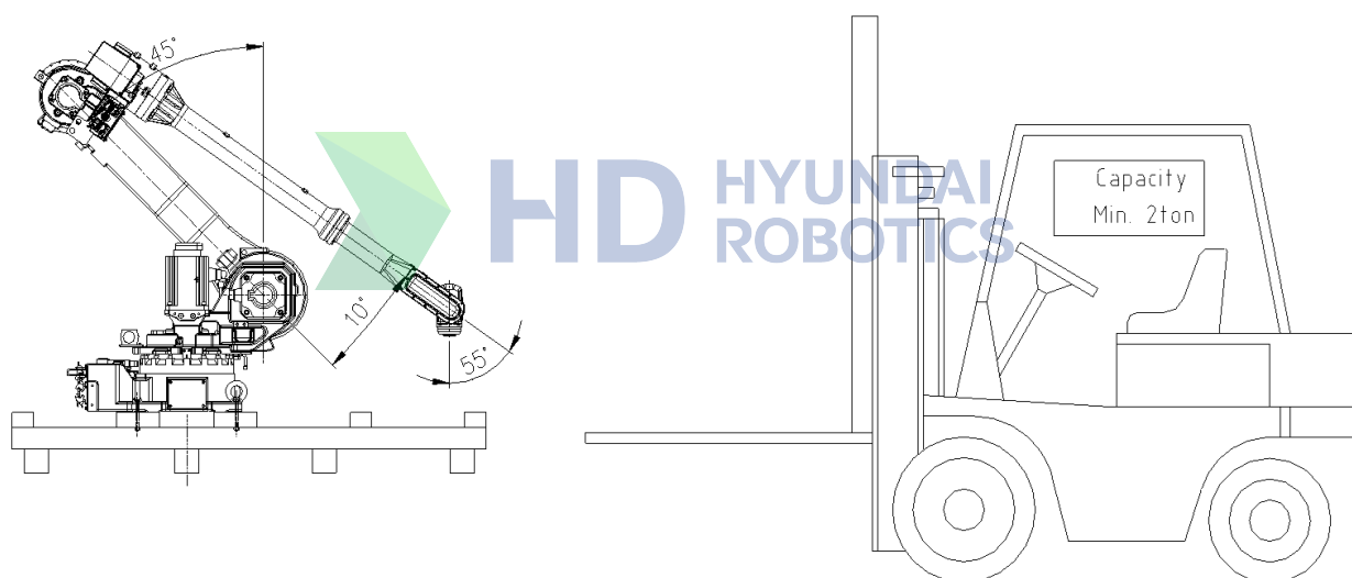
图 3.4 运送方法：利用叉车 [HH020L]
