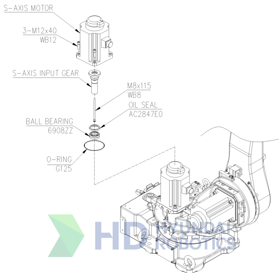
图 6.1 S 轴电机安装
