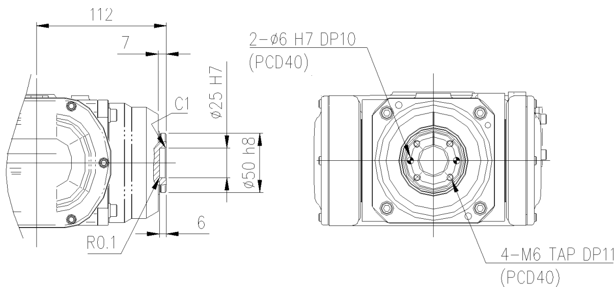
图 2.5 机械腕轴连接面细节 [HH020L]
