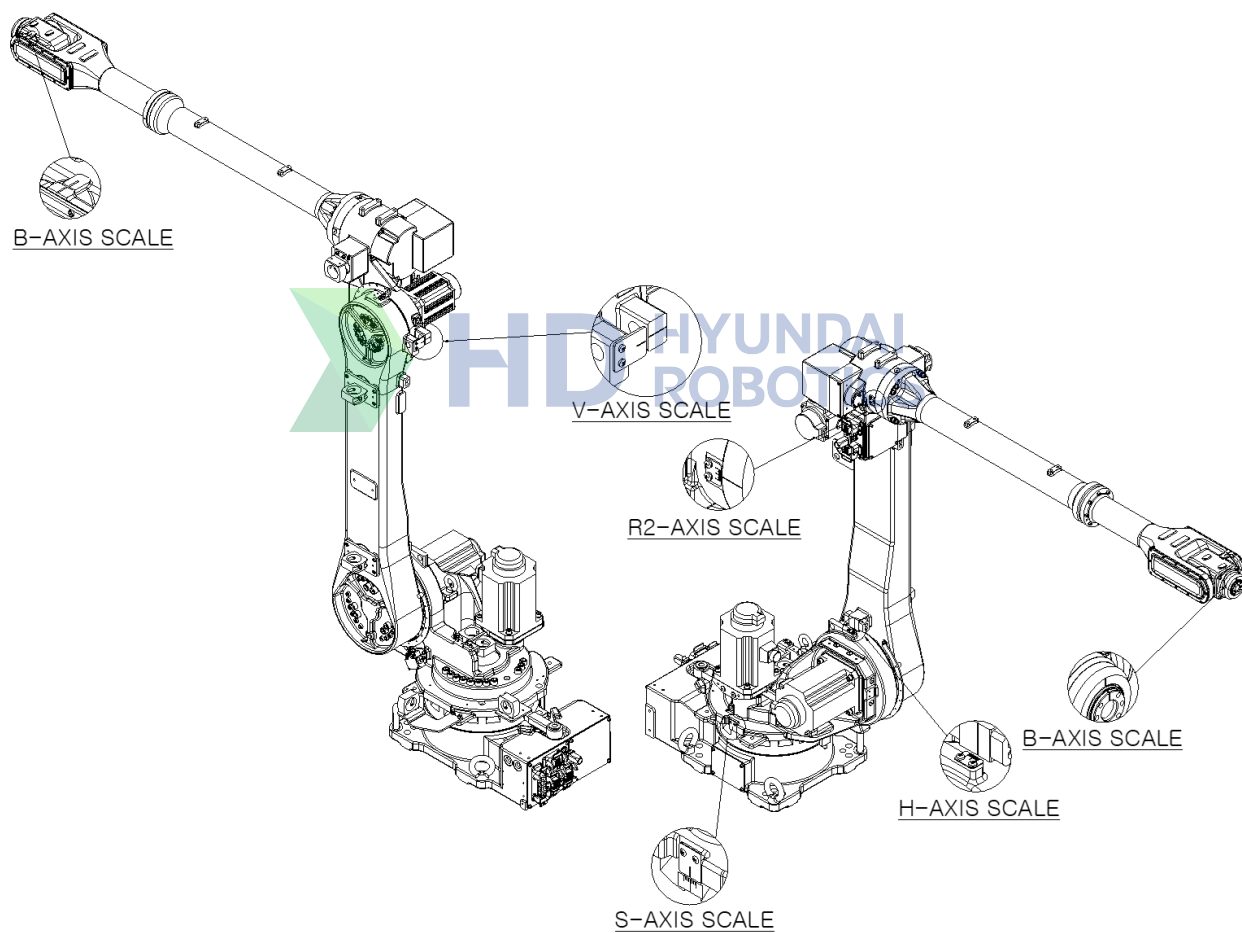
图 6.7 归零设定的方法 [HH020L]
