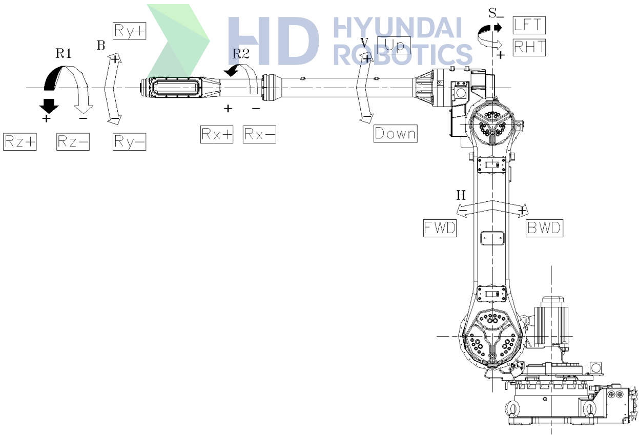
图 2.4 机器人尺寸和轴 [HH020L]
