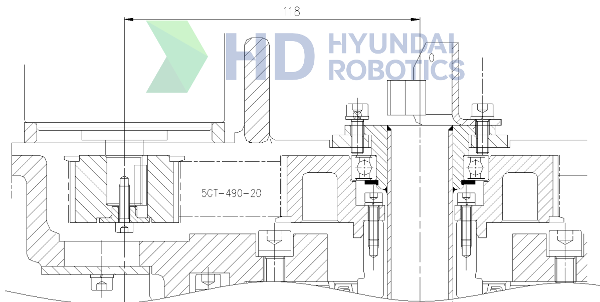
图 4.2 R2 轴 Timing Belt 张力检查部位 [HH020L]
