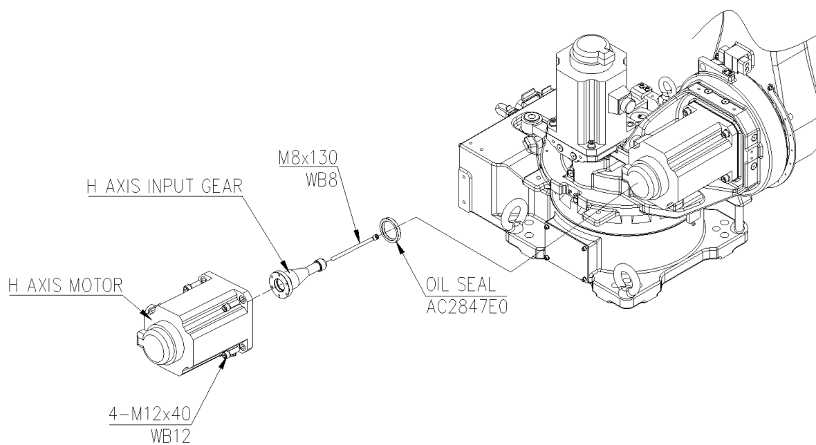
图 6.2 H 轴电机安装
