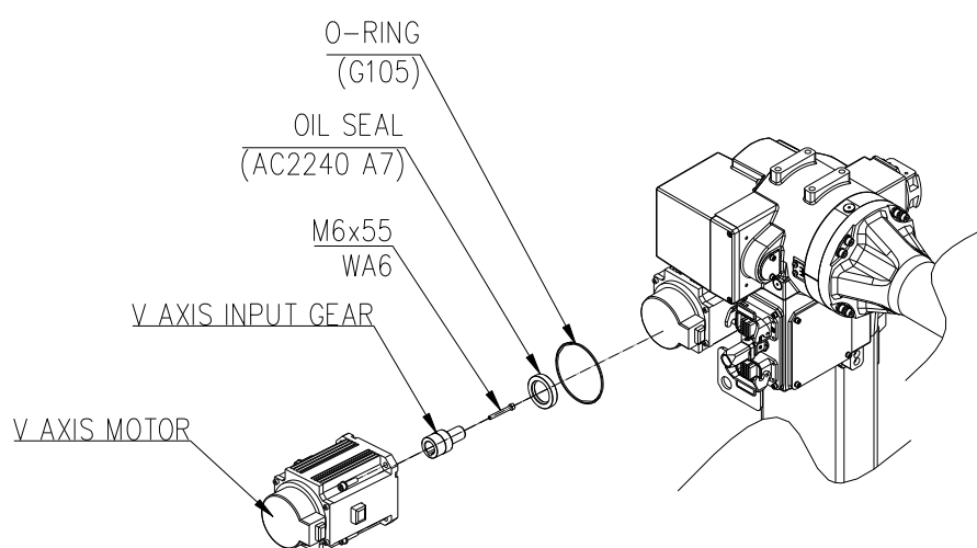
图 6.3 V 轴电机安装
