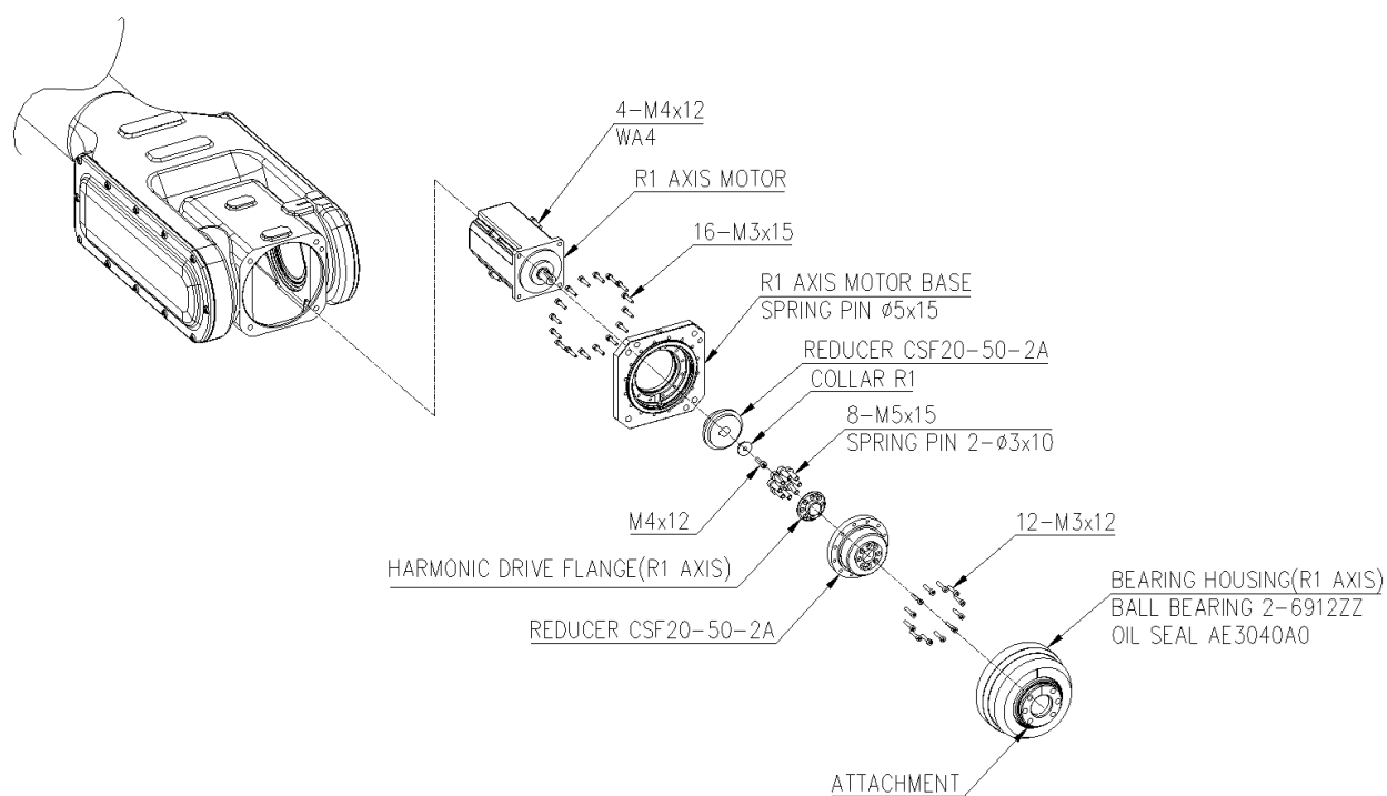
图 6.6 R1 轴电机安装
