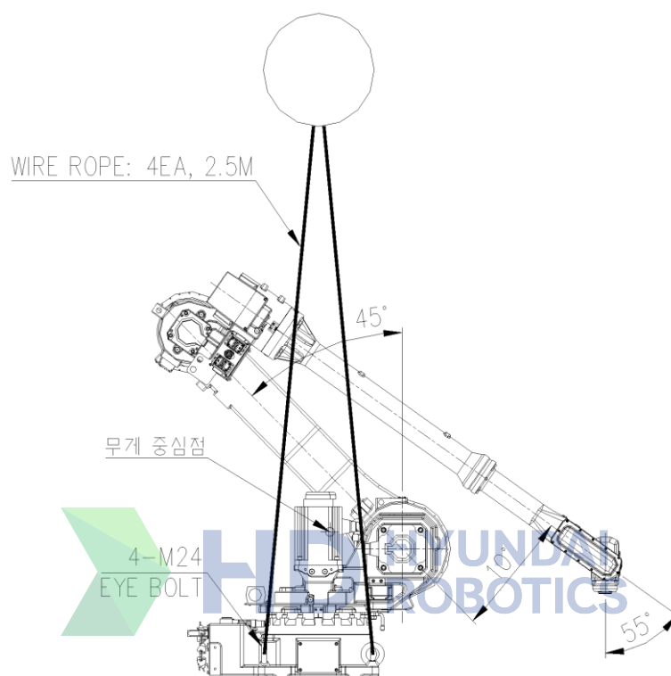
图 3.3 运送方法：使用吊车 [HH020L]
