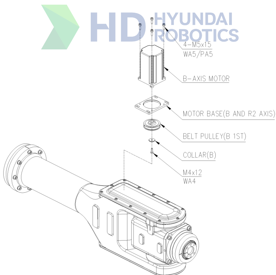
图 6.5 B 轴电机安装
