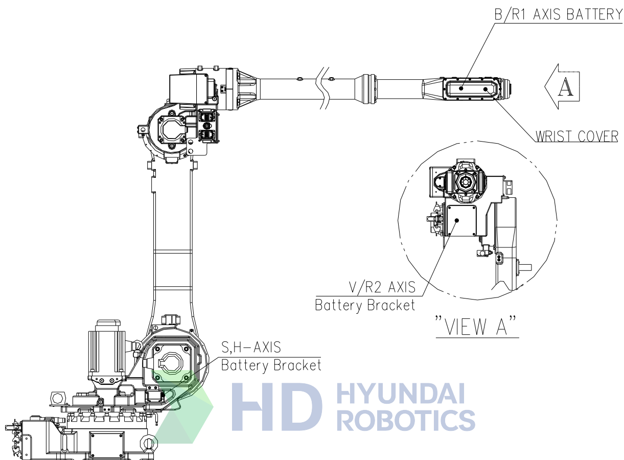
图 5.1 电池的位置
