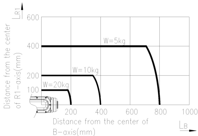
图 3.8 腕轴转矩图: [HH020L]
