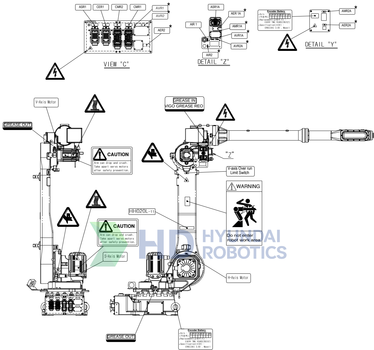
图 3.2 安全标识牌位置
