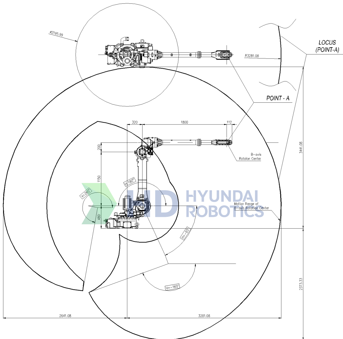
图 2.3 机器人尺寸和工作区间 [HH020L]
