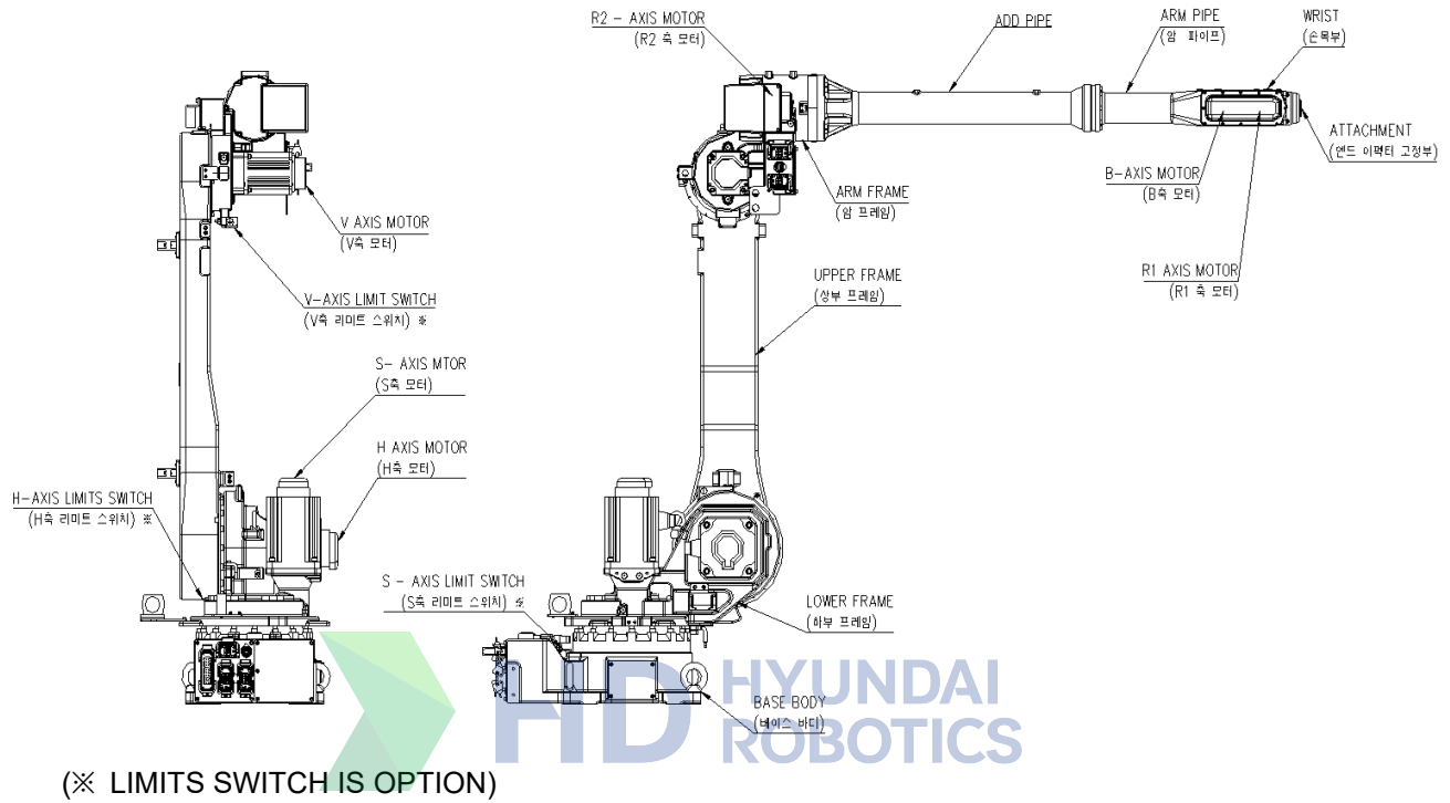
图 3.1 机器人零件名称
