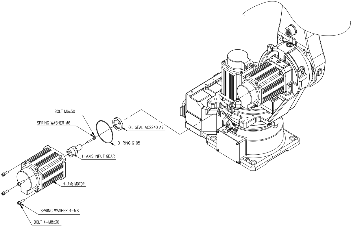
图 6.9 替换 H 轴电机 [HA006L]
