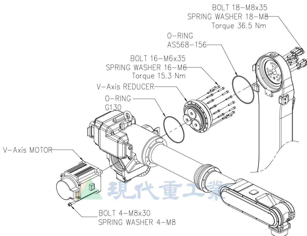
图 6.24 V 轴减速器分解 [HA006L]
