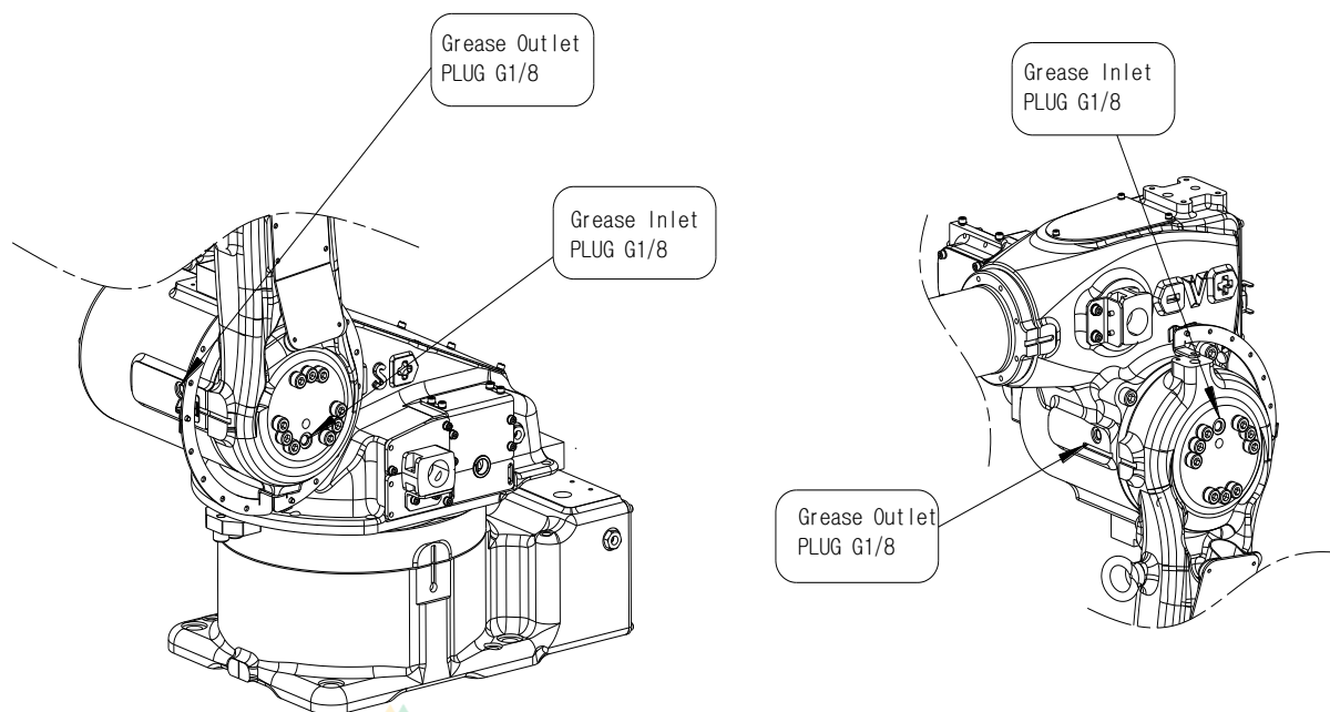
图 5.3 H/V 轴润滑油 IN/OUTLET 位置 [HA006A]
