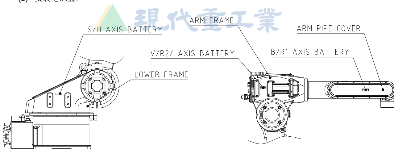
图 5.5 电池替换位置 [HA006A]
