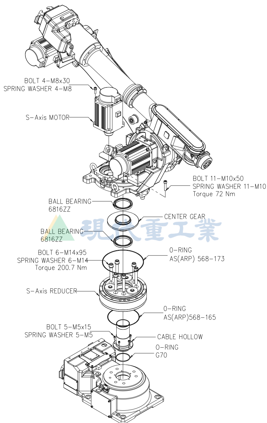
图 6.20 S 轴减速器分解图 [HA006L]
