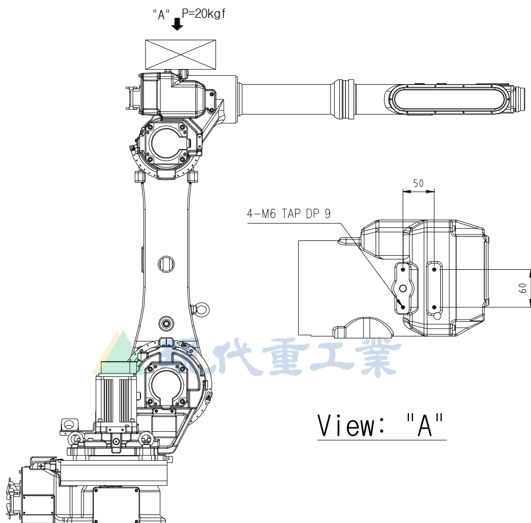
图 2.8 第 1 臂部上部接合部详图: [HA006L]
