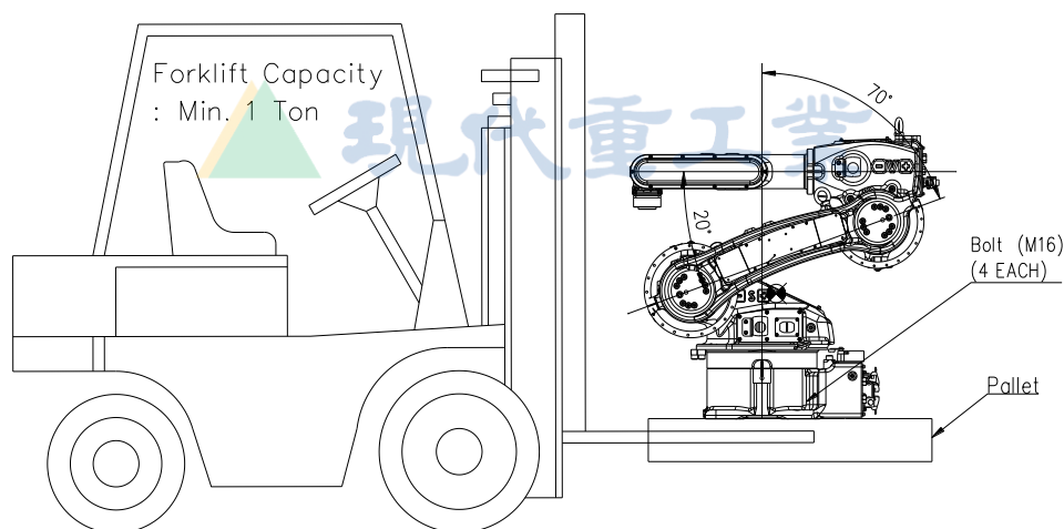
图 3.7 搬运方法: 利用叉车 [HA006A]
