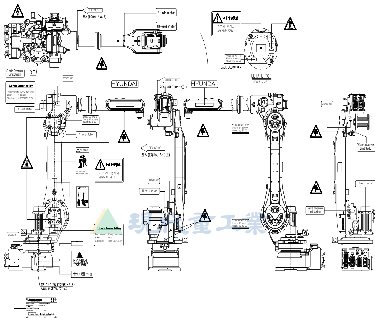
图 3.4 安全铭牌位置[HA006L]
