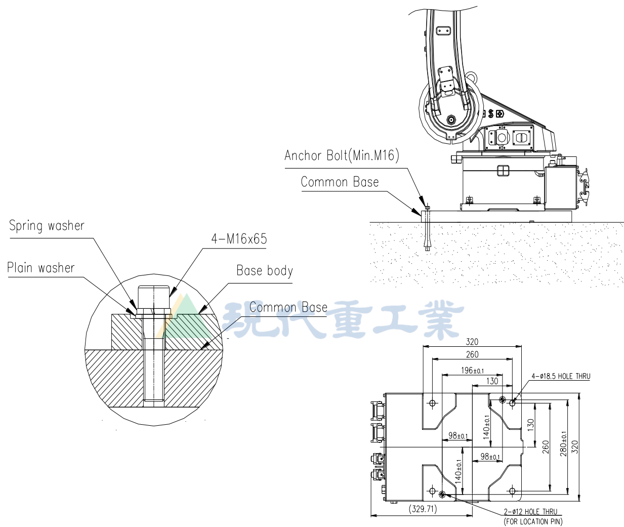
图 3.9 机器人安装面尺寸 [HA006A]
