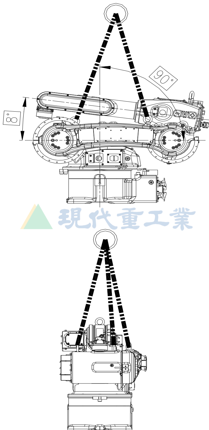
图 6.13 替换 S 轴减速器时的机器人姿势 [HA006A]
