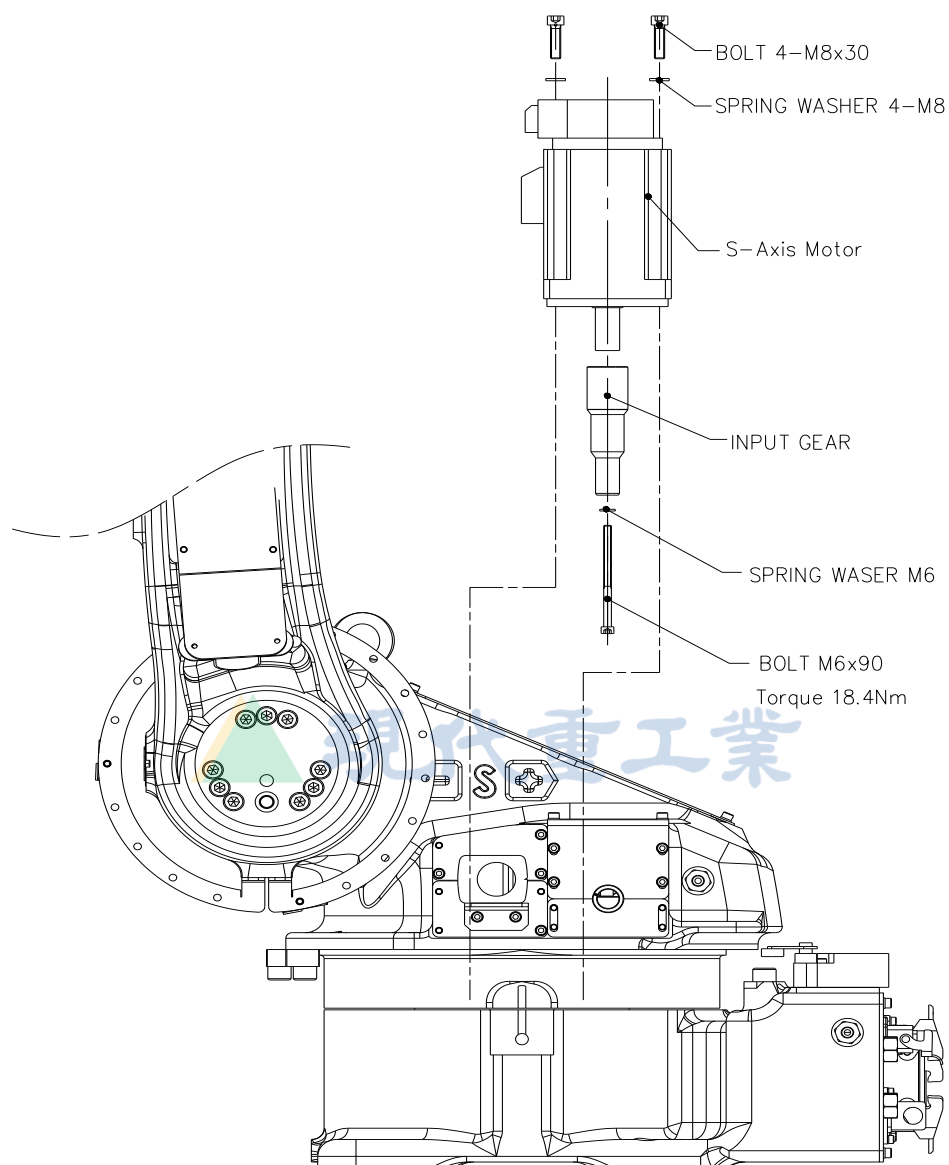
图 6.1 替换 S 轴电机 [HA006A]
