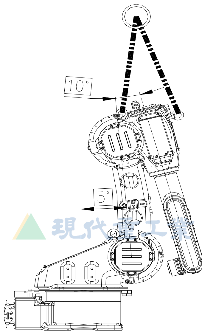
图 6.15 替换 H 轴减速器时的机器人姿势 [HA006A]
