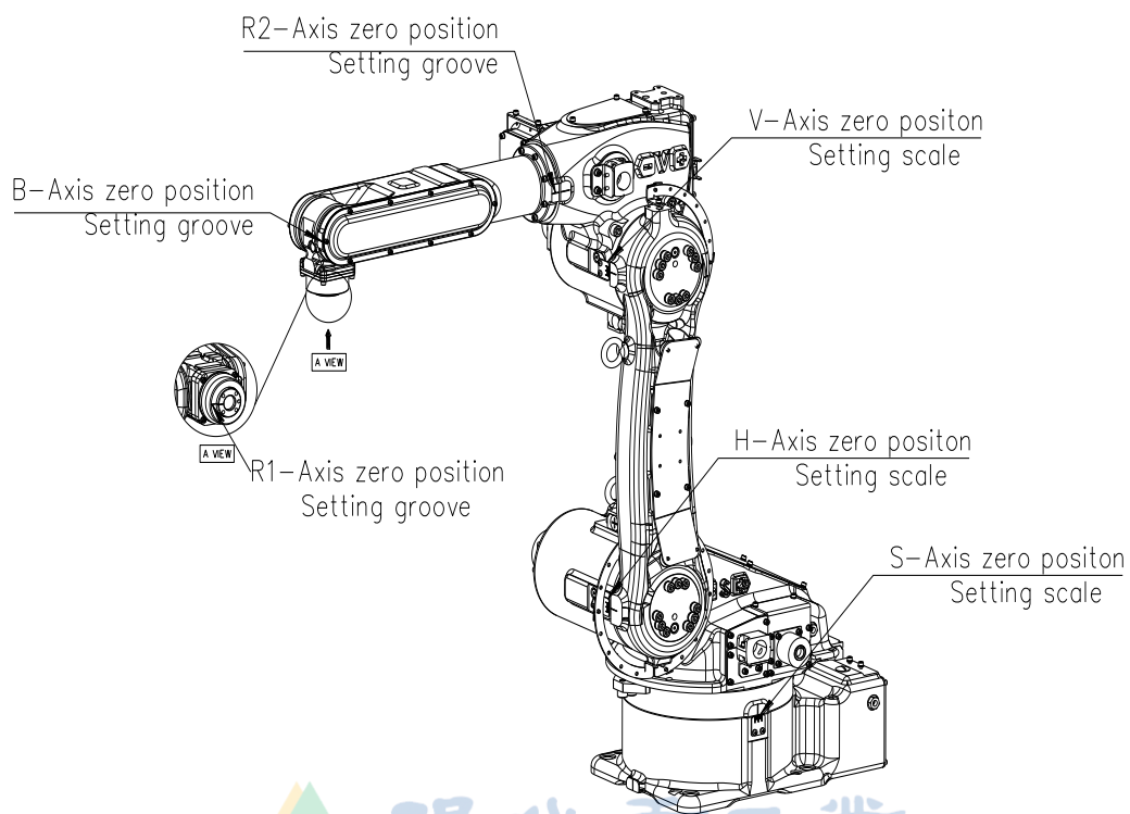
图 6.25 原点设置方法 [HA006A]
