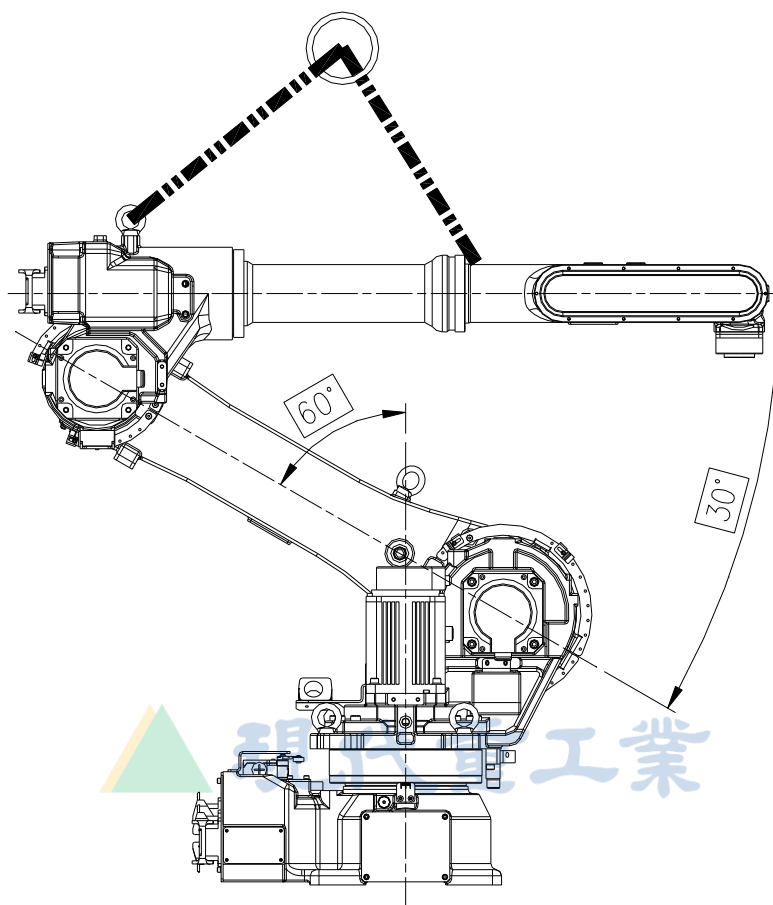
图 6.23 替换 V 轴减速器时的机器人姿势 [HA006L]
