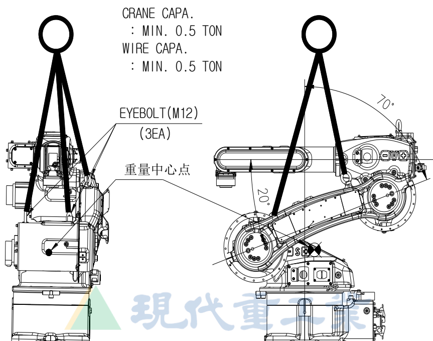
图 3.5 搬运方法: 利用起吊机 [HA006A]
