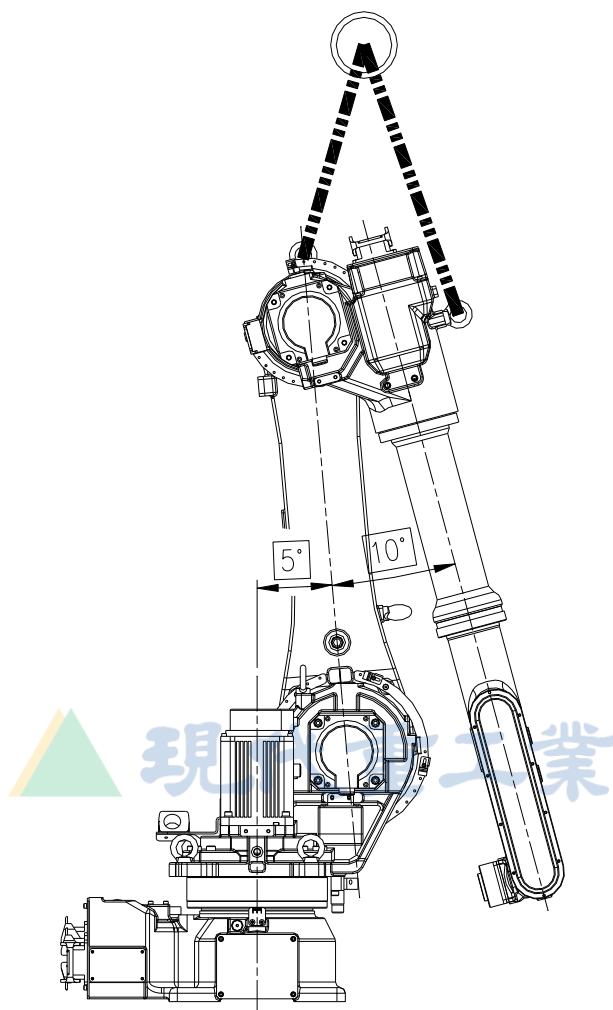
图 6.21 替换 H 轴减速器时的机器人姿势 [HA006L]
