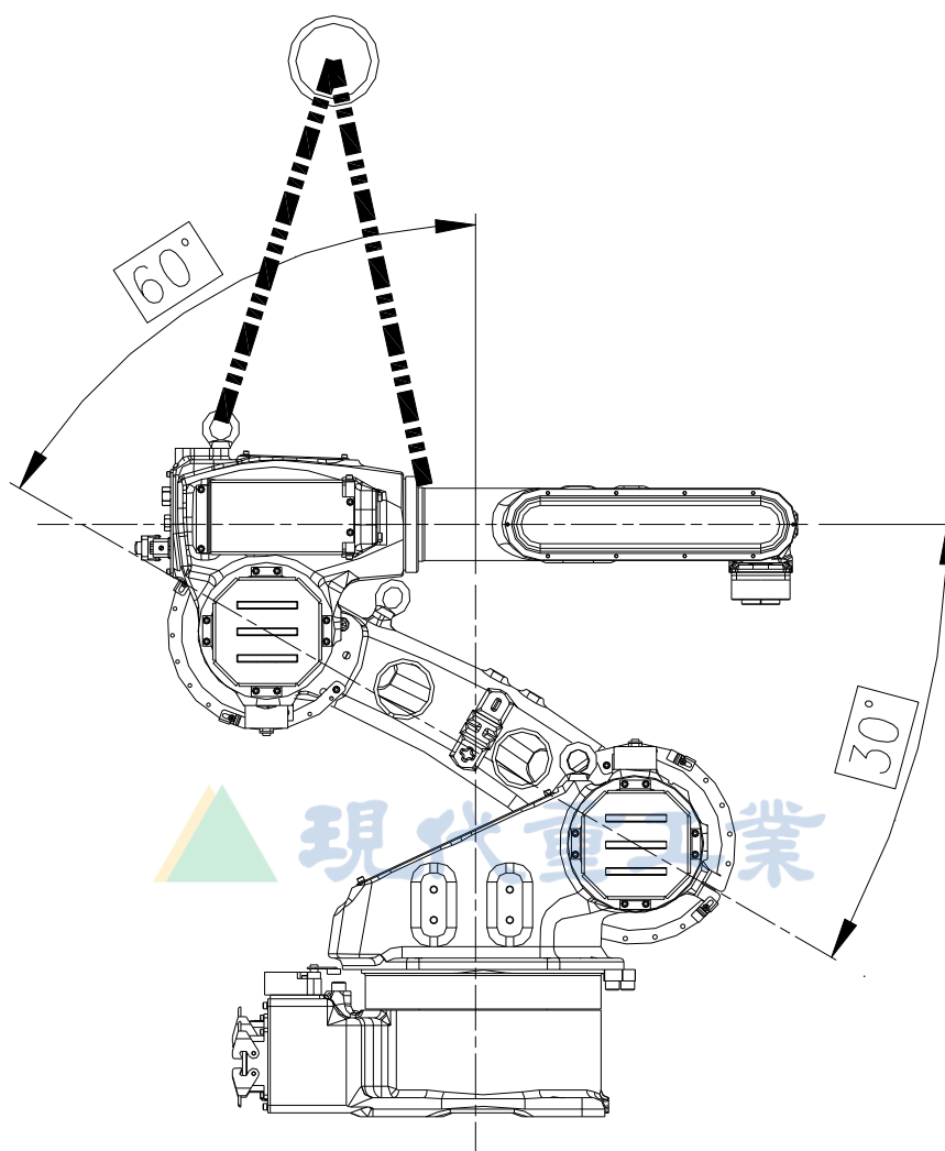
图 6.17 替换 V 轴减速器时的机器人姿势 [HA006A]
