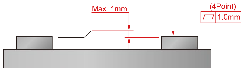
图 3.11 机器人安装面程度
