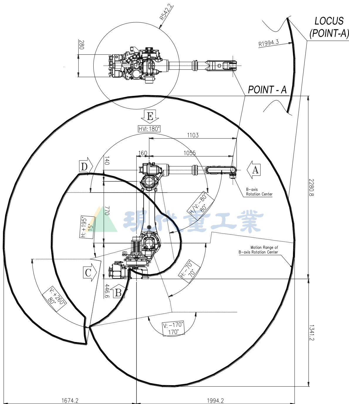
图 2.4 机器人外形尺寸及工作区域: [HA006L]
