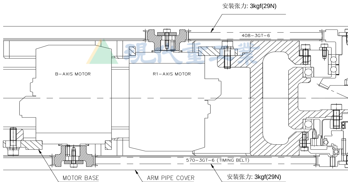
图 4.4 B 轴 Timing Belt 张力检查部位
