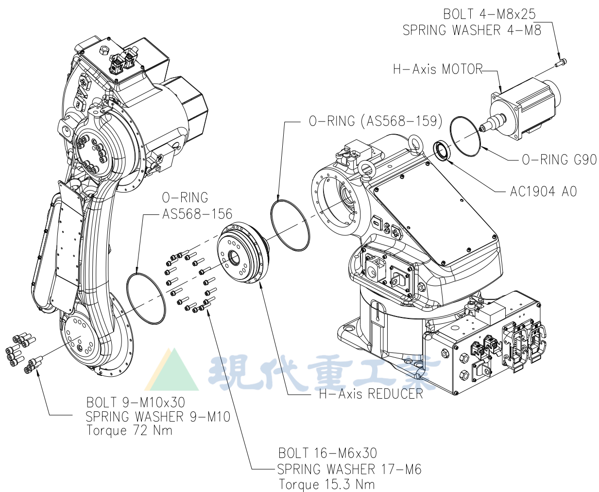
图 6.16 H 轴减速器分解图 [HA006A]
