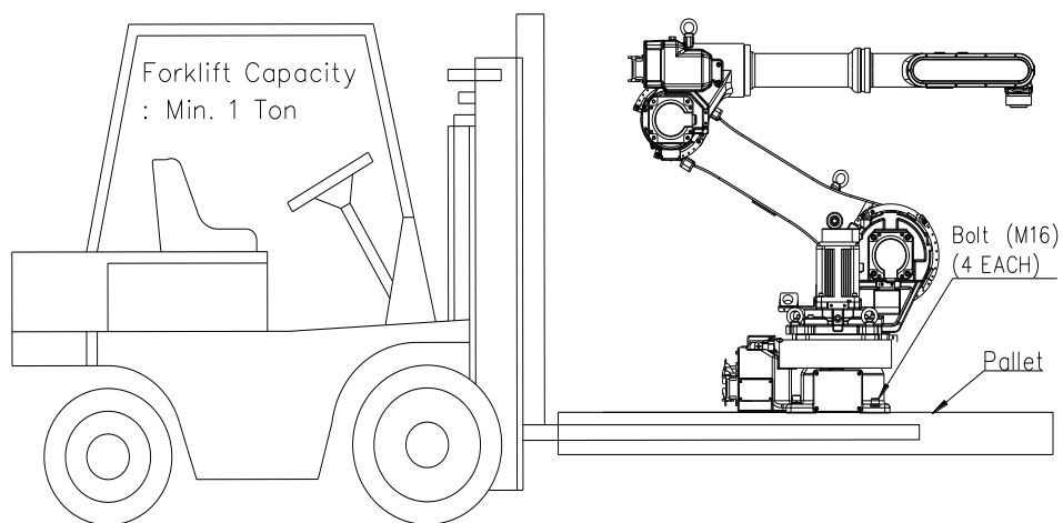
图 3.8 搬运方法: 利用叉车 [HA006L]
