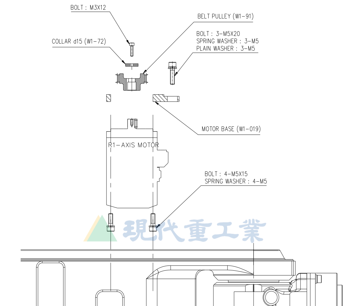
图 6.12 替换 B/R1 轴电机 [HA006A/HA006L]
