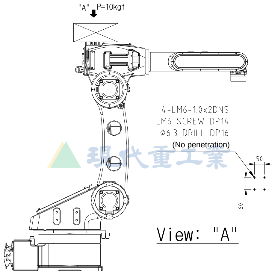
图 2.7 第 1 臂部上部接合部详图: [HA006A]
