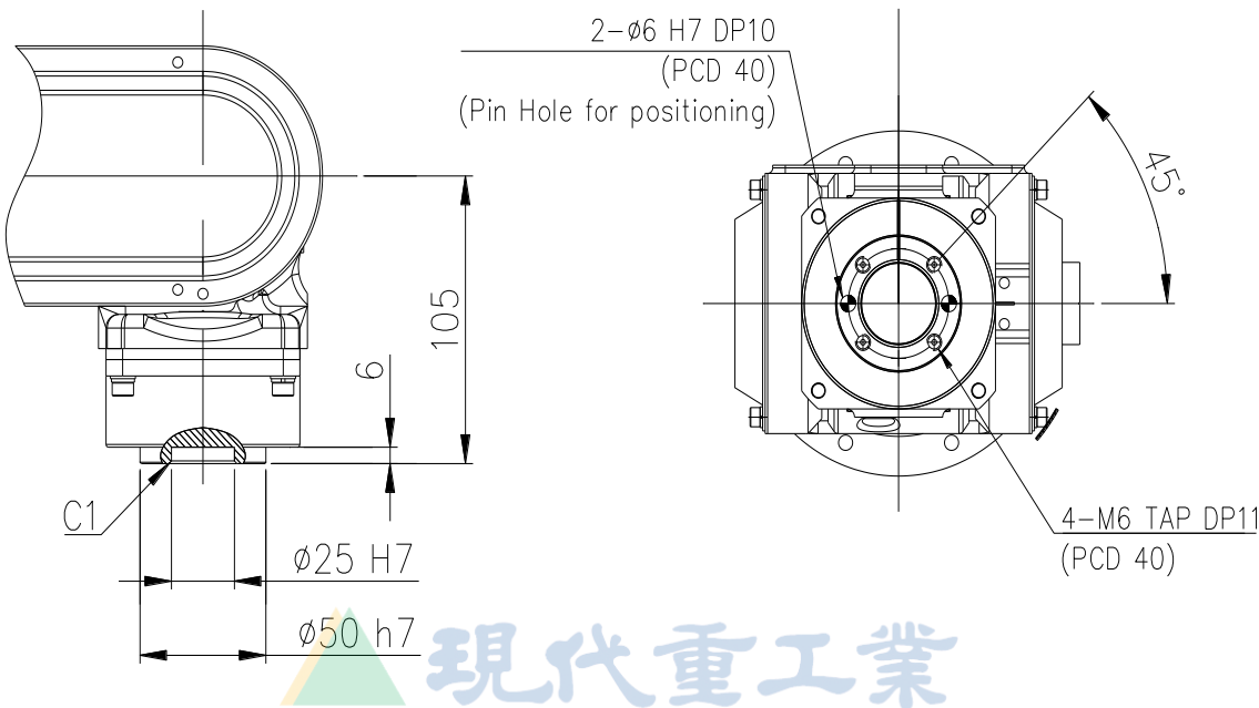
图 2.6 手腕轴贴附面详图
