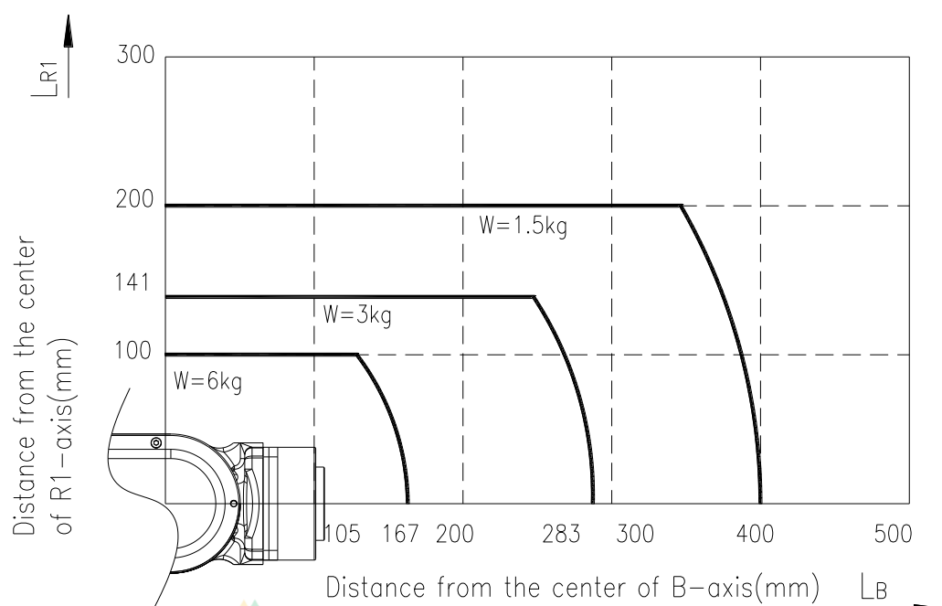
图 3.13 手腕轴扭矩线图
