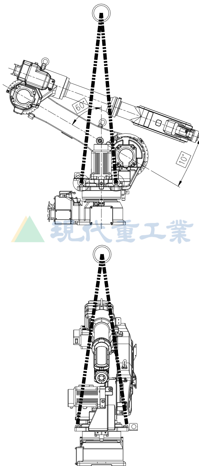
图 6.19 替换 S 轴减速器时的机器人姿势 [HA006L]
