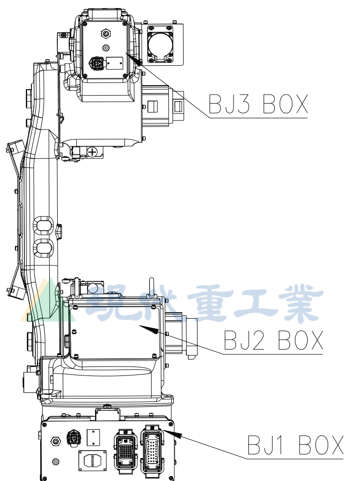
图 8.1 机体配件布置 [HA006A]
