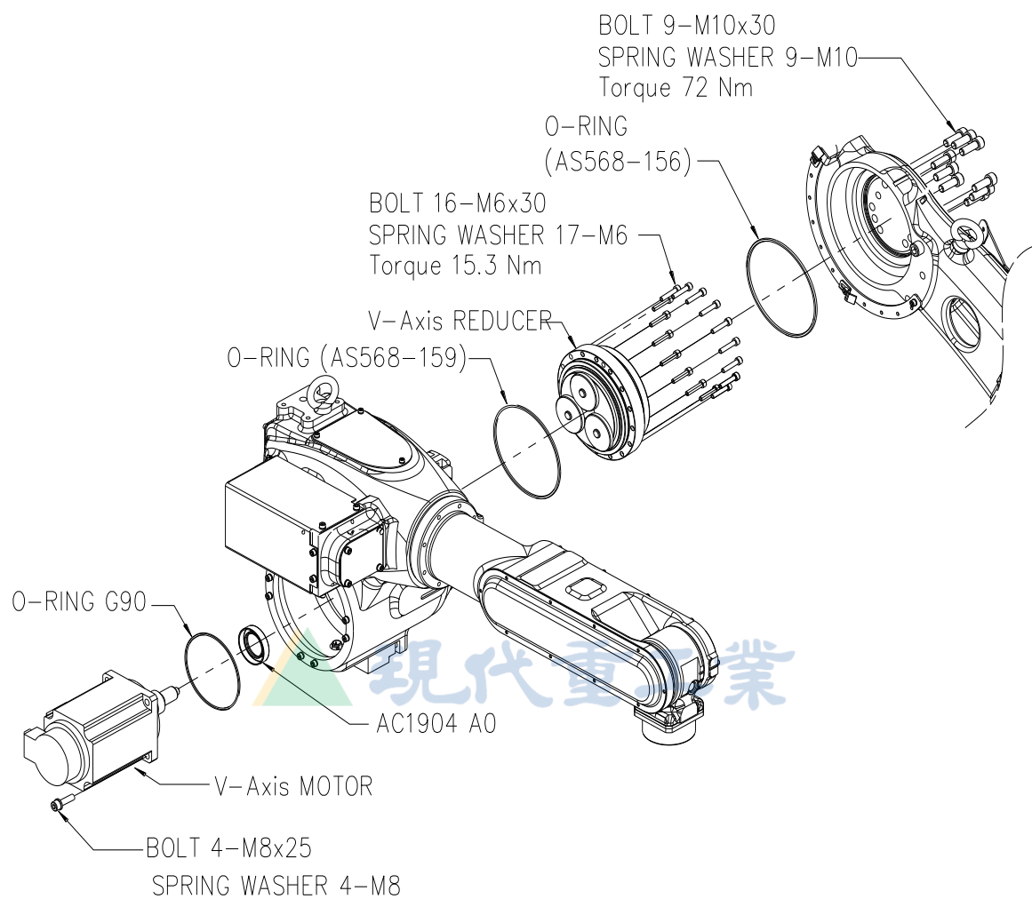
图 6.18 V 轴减速器分解图 [HA006A]
