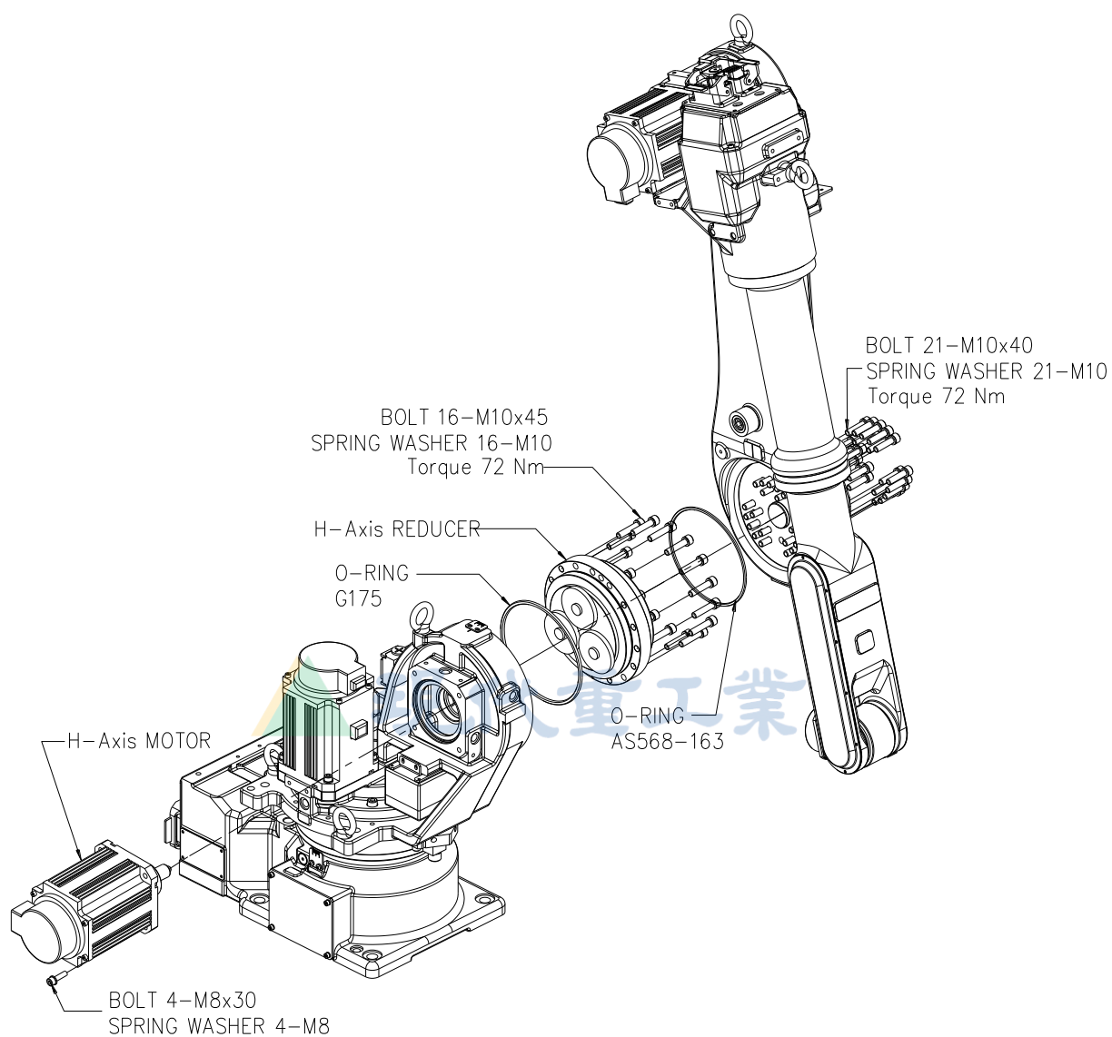
图 6.22 H 轴减速器分解 [HA006L]
