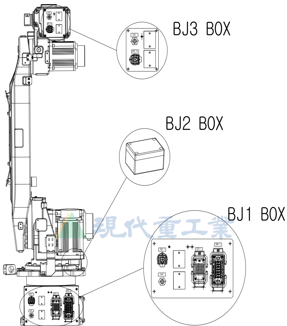
图 8.2 机体配件布置 [HA006L]
