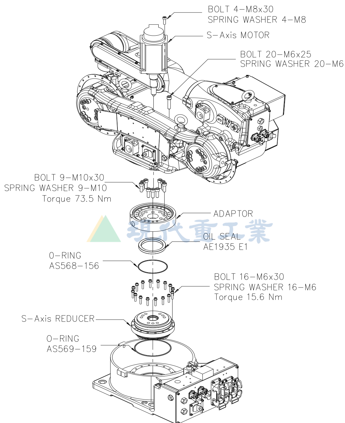
图 6.14 S 轴减速器分解图 [HA006A]
