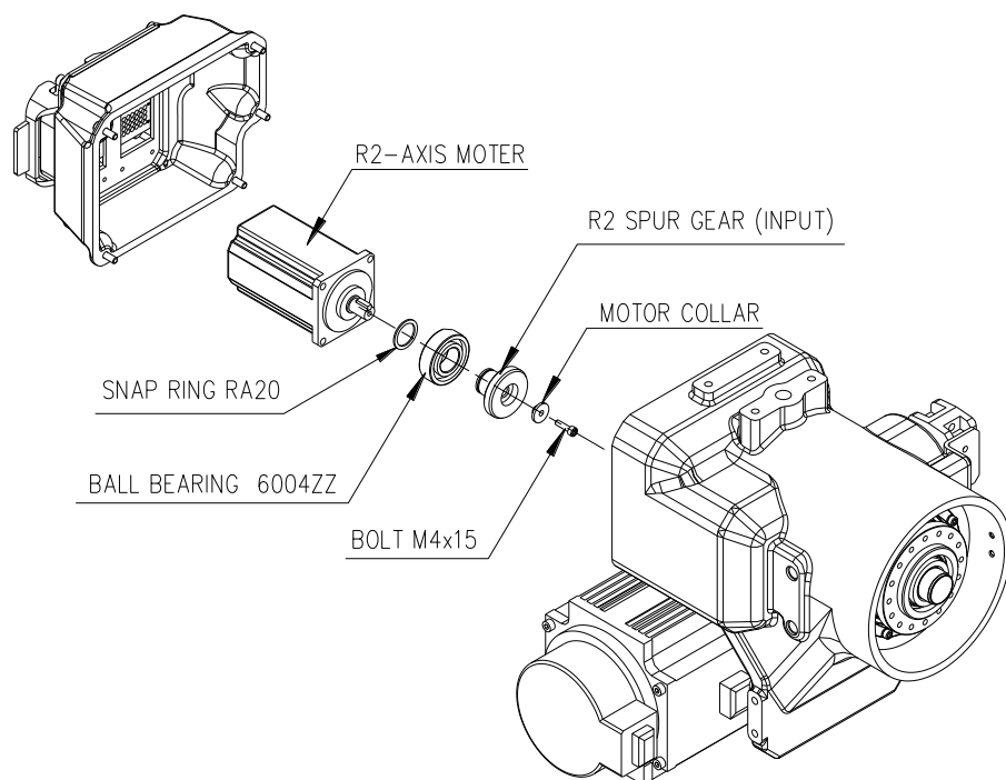
图 6.11 替换 R2 轴电机 [HA006L]
