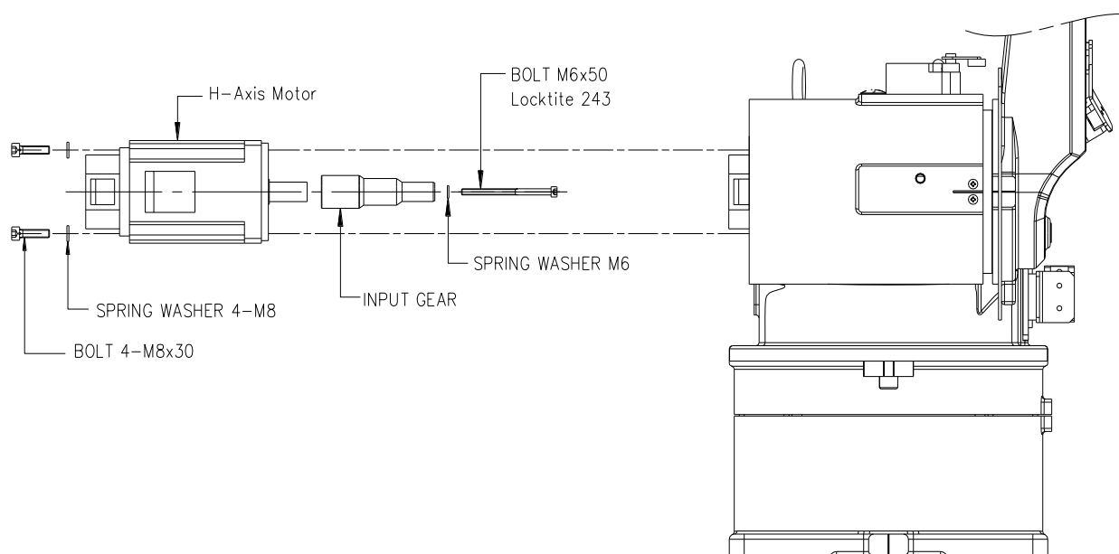
图 6.3 替换 H 轴电机 [HA006A]
