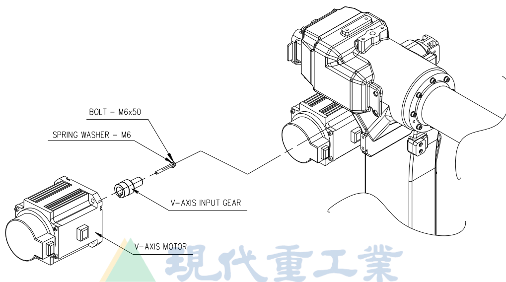
图 6.10 替换 V 轴电机 [HA006L]
