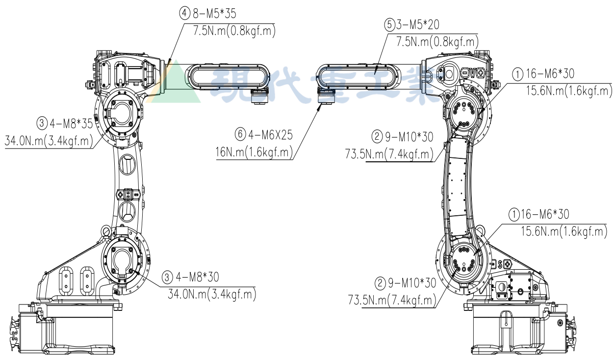
图 4.1 主要螺丝检查部位 [HA006A]
