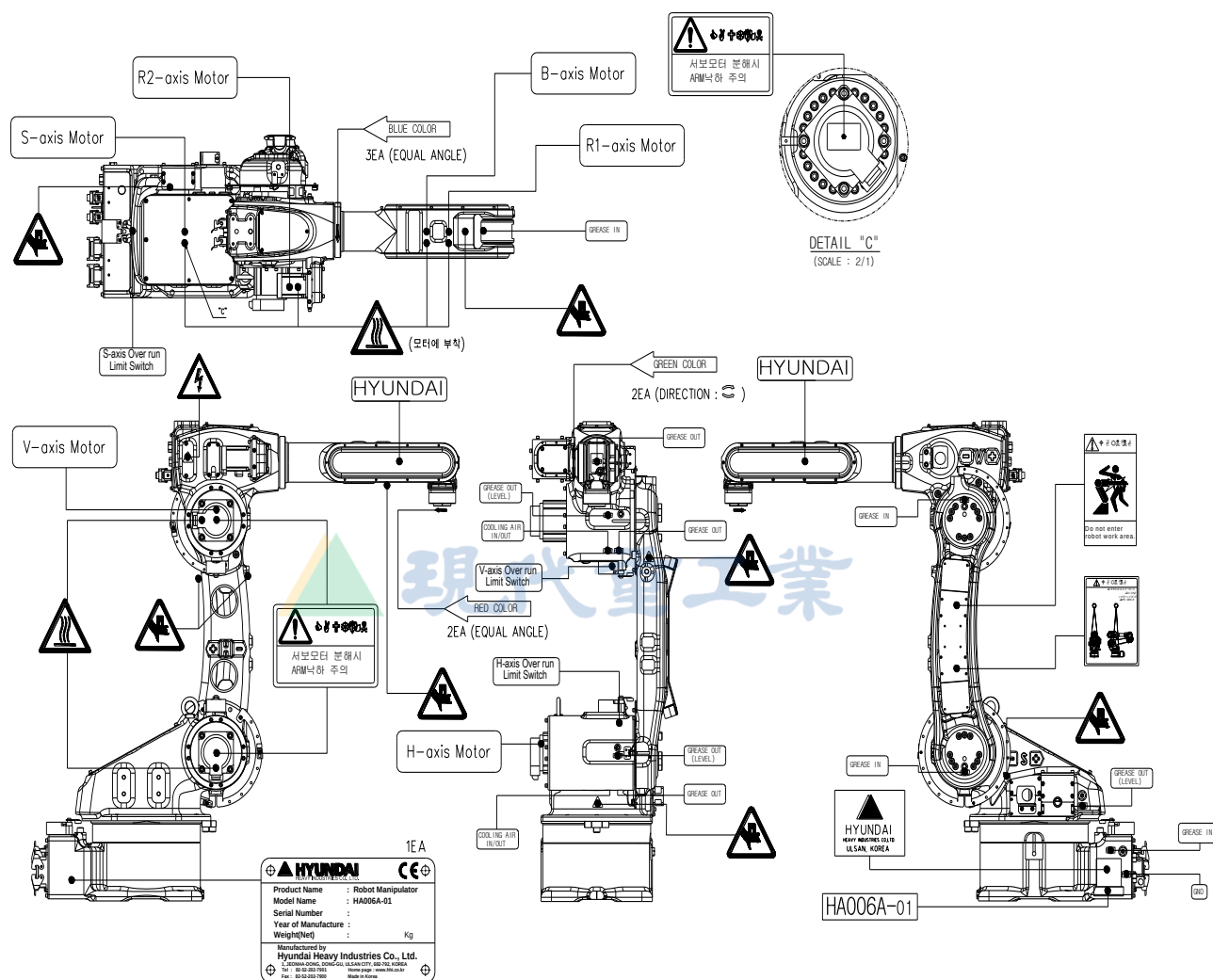
图 3.3 安全铭牌位置[HA006A]
