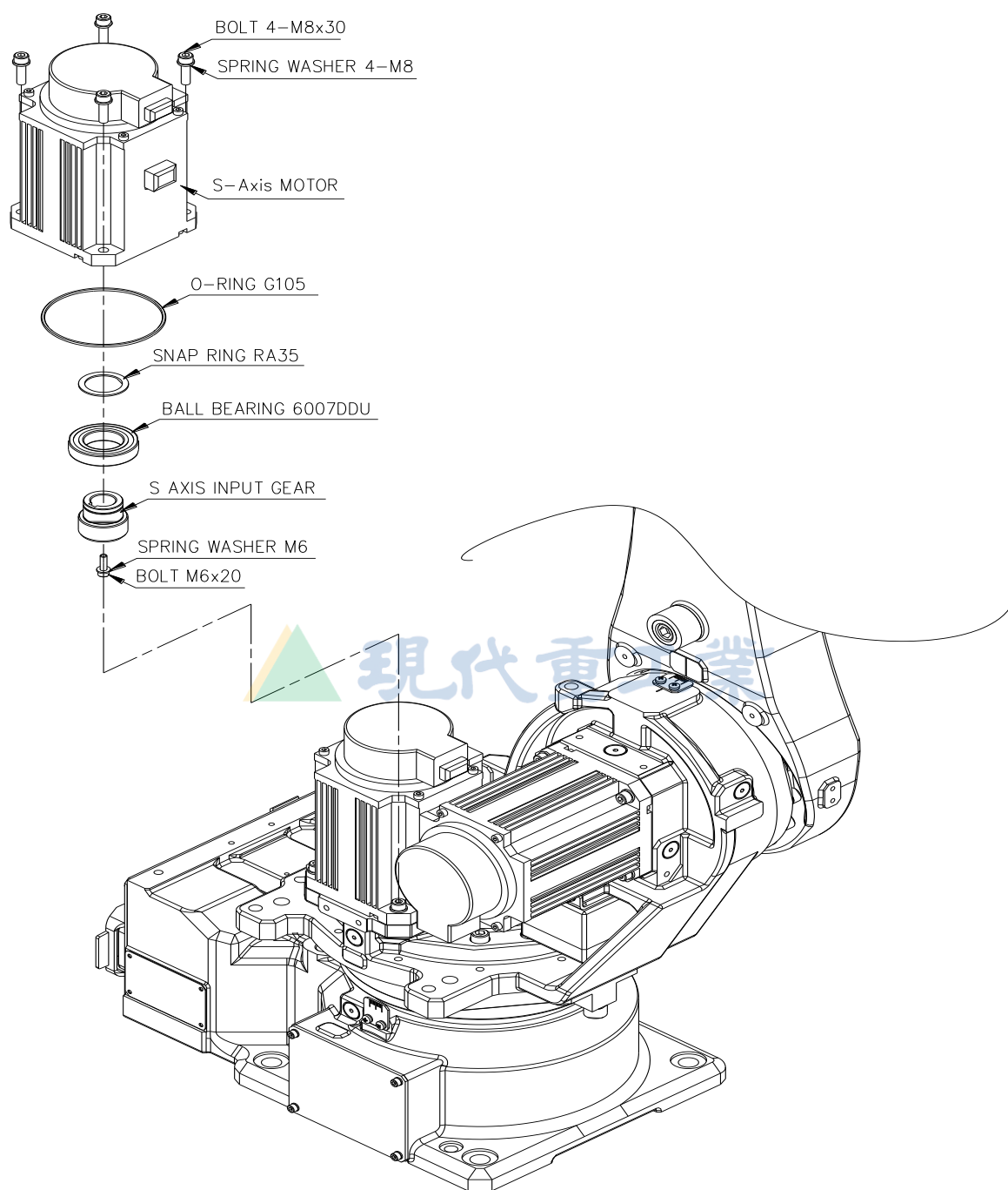
图 6.7 替换 S 轴电机 [HA006L]
