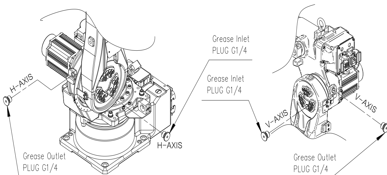
图 5.4 H/V 轴润滑油 IN/OUTLET 位置 [HA006L]
