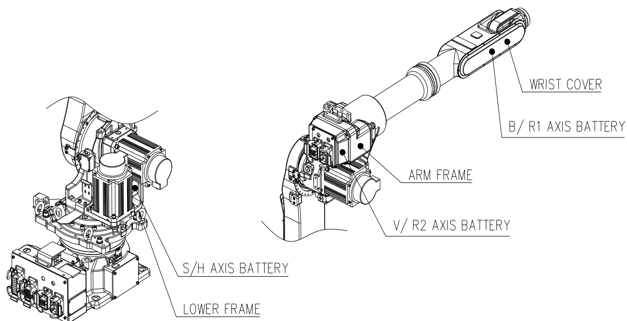
图 5.6 电池替换位置 [HA006L]
