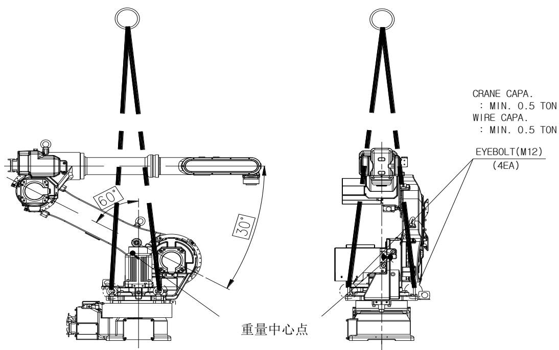
图 3.6 搬运方法: 利用起吊机 [HA006L]
