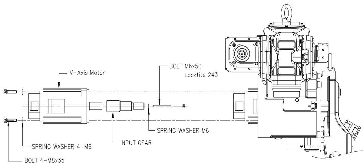
图 6.5 替换 V 轴电机 [HA006A]
