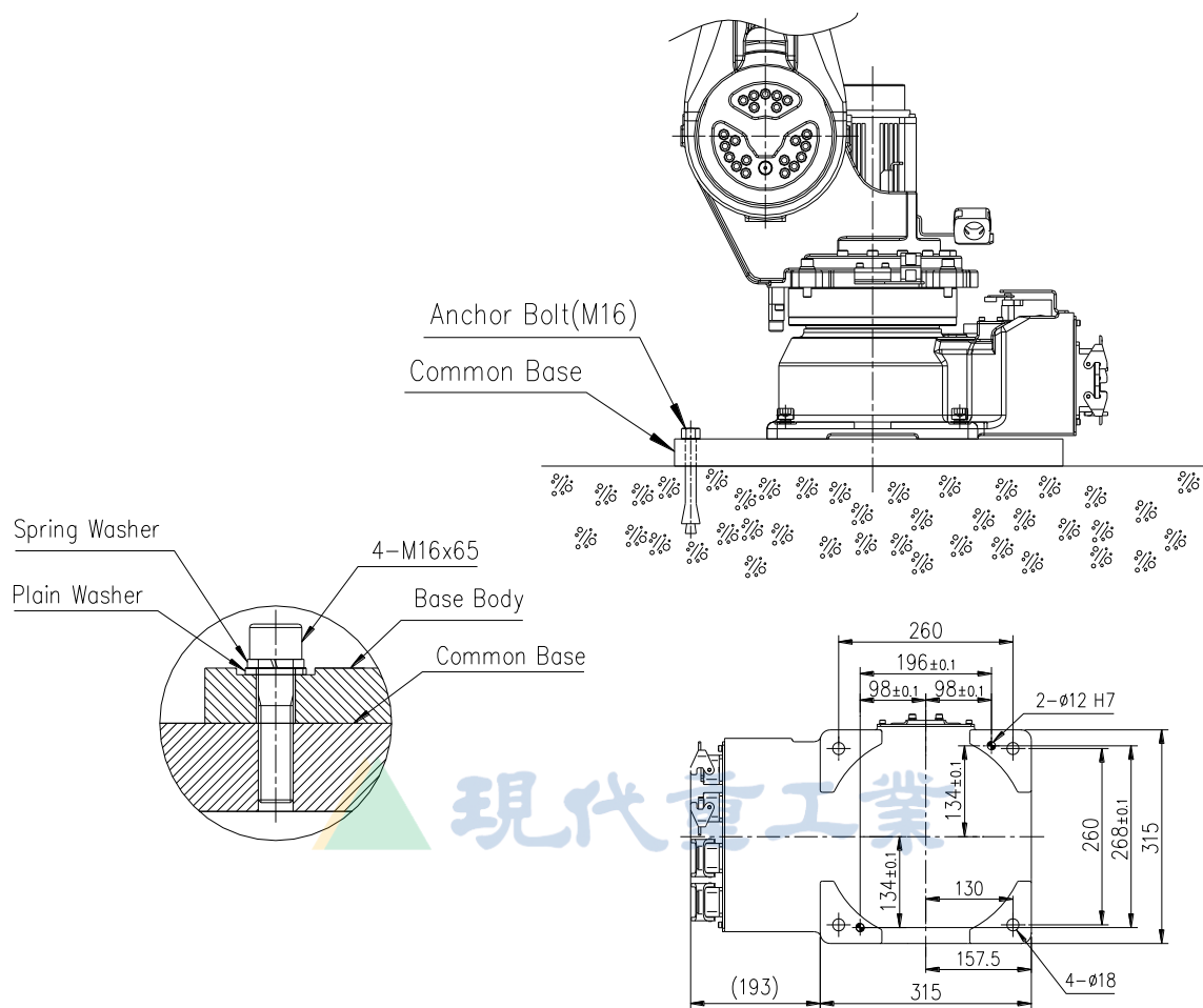
图 3.10 机器人安装面尺寸 [HA006L]
