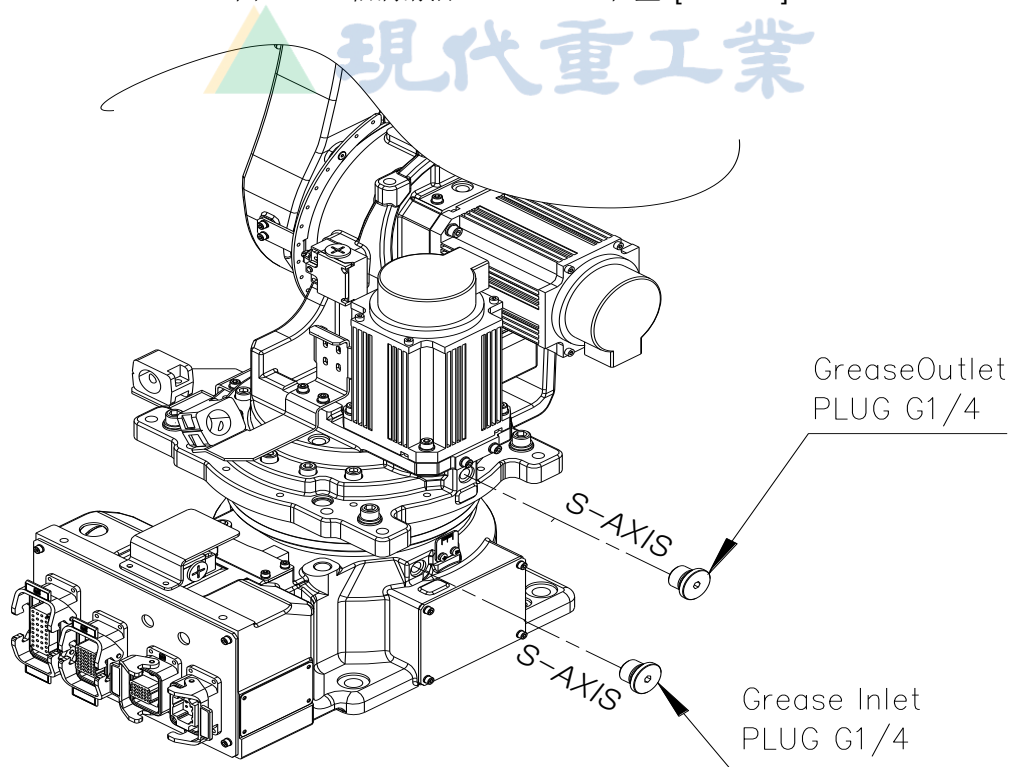
图 5.1 S 轴润滑油 IN/OUTLET 位置 [HA006A]
