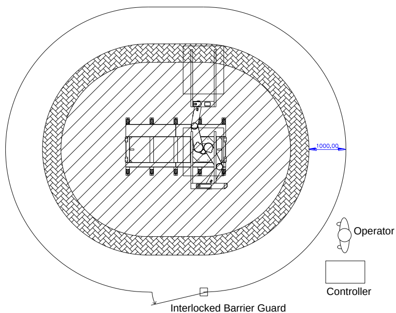
(圓筒形)
