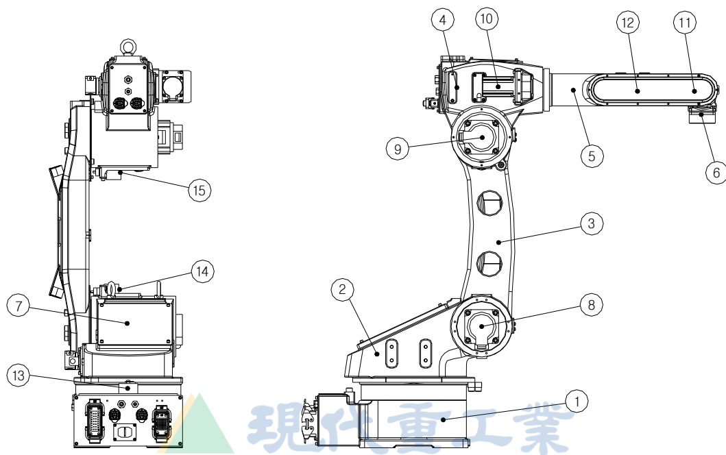
图 3.1 机体各部位名称[HA006A]
