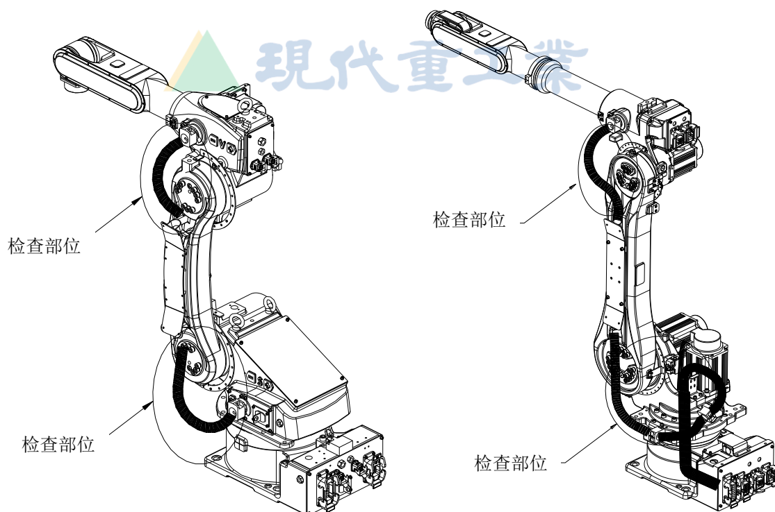
图 4.3 电缆检查部位 [HA006A/HA006L]
