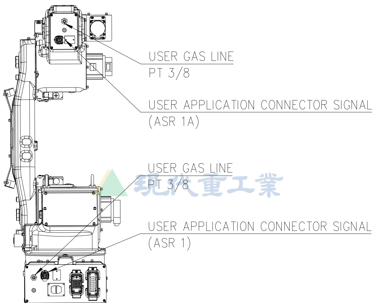
图 2.9 应用配线及配管图: [HA006A]
