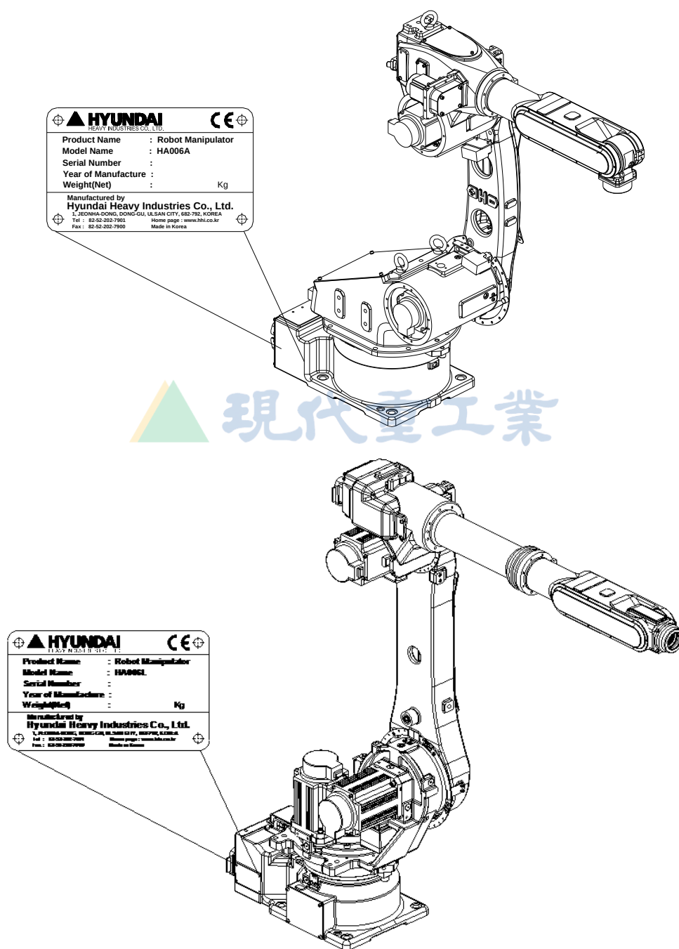
图 2.2 机器人铭牌粘贴位置 [HA006/HA006L]
