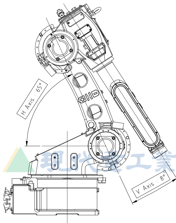
图 6.4 替换 V 轴电机时的机器人姿势 [HA006A]
