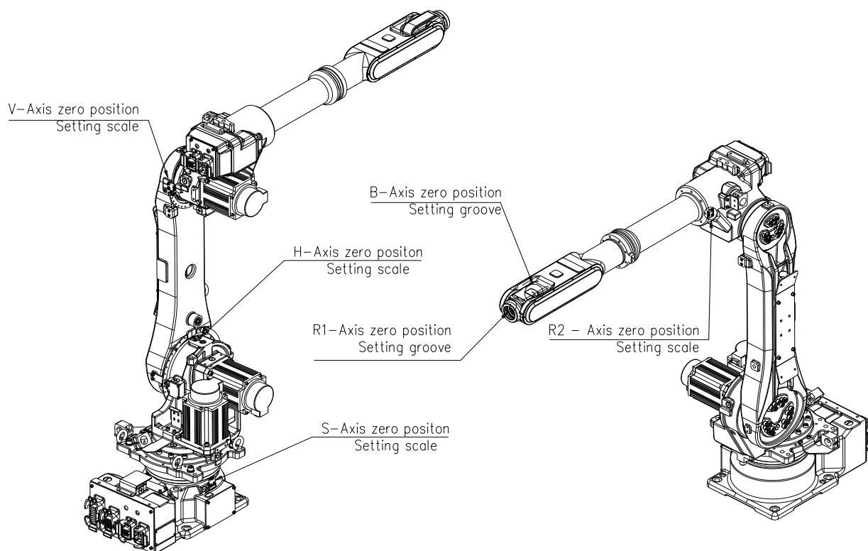
图 6.26 原点设置方法 [HA006L]
