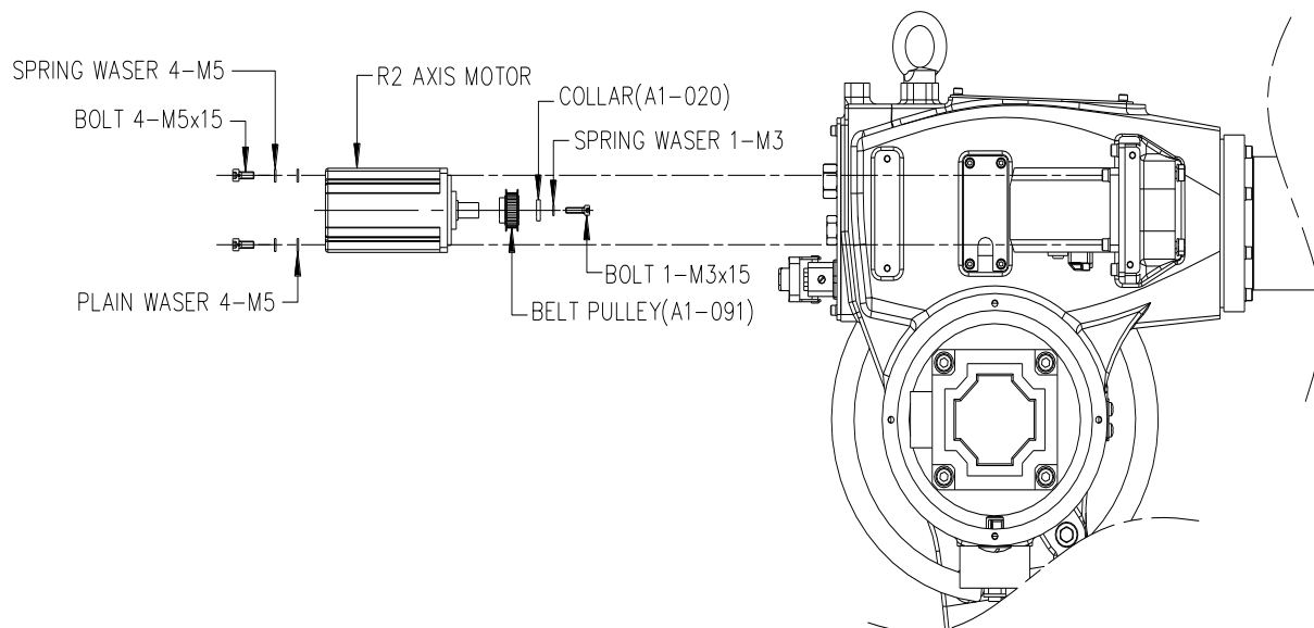
图 6.6 替换 R2 轴电机 [HA006A]
