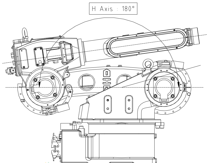
图 6.2 替换 H 轴电机时的机器人姿势 [HA006A]
