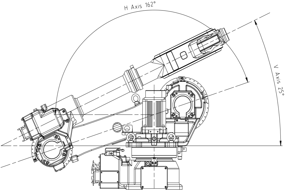
图 6.8 替换 H/V 轴电机时的机器人姿势 [HA006L]
