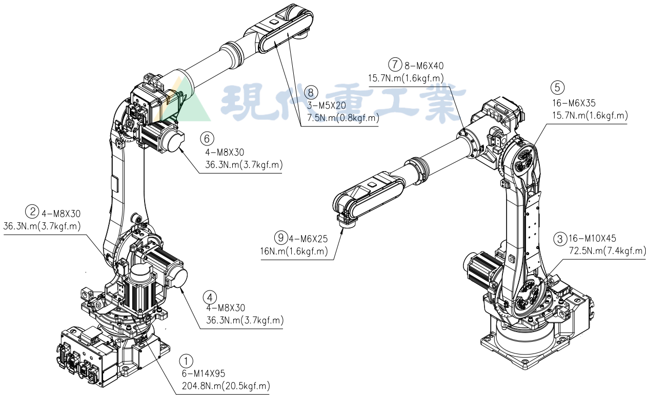
图 4.2 主要螺丝检查部位 [HA006L]
