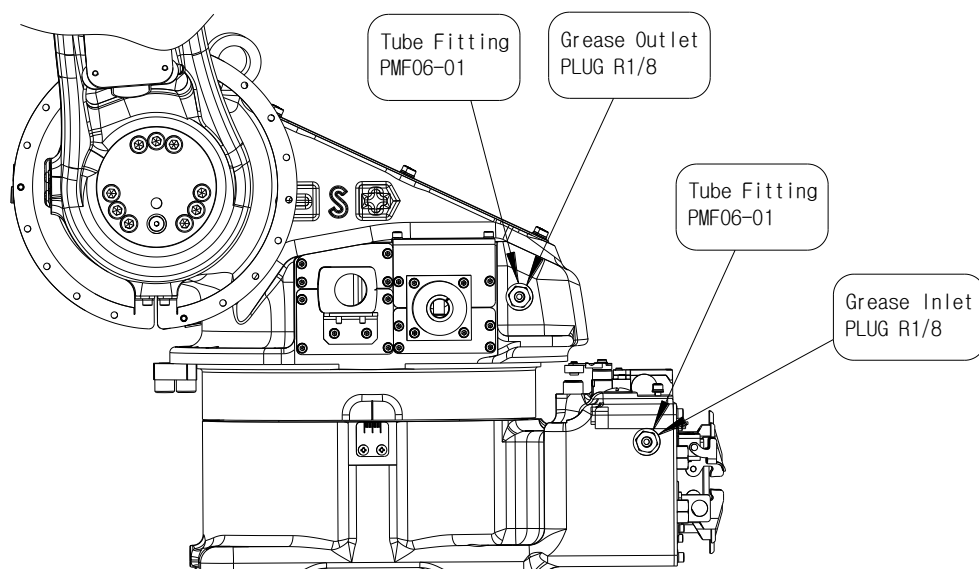
图 5.1 S 轴润滑油 IN/OUTLET 位置 [HA006A]
