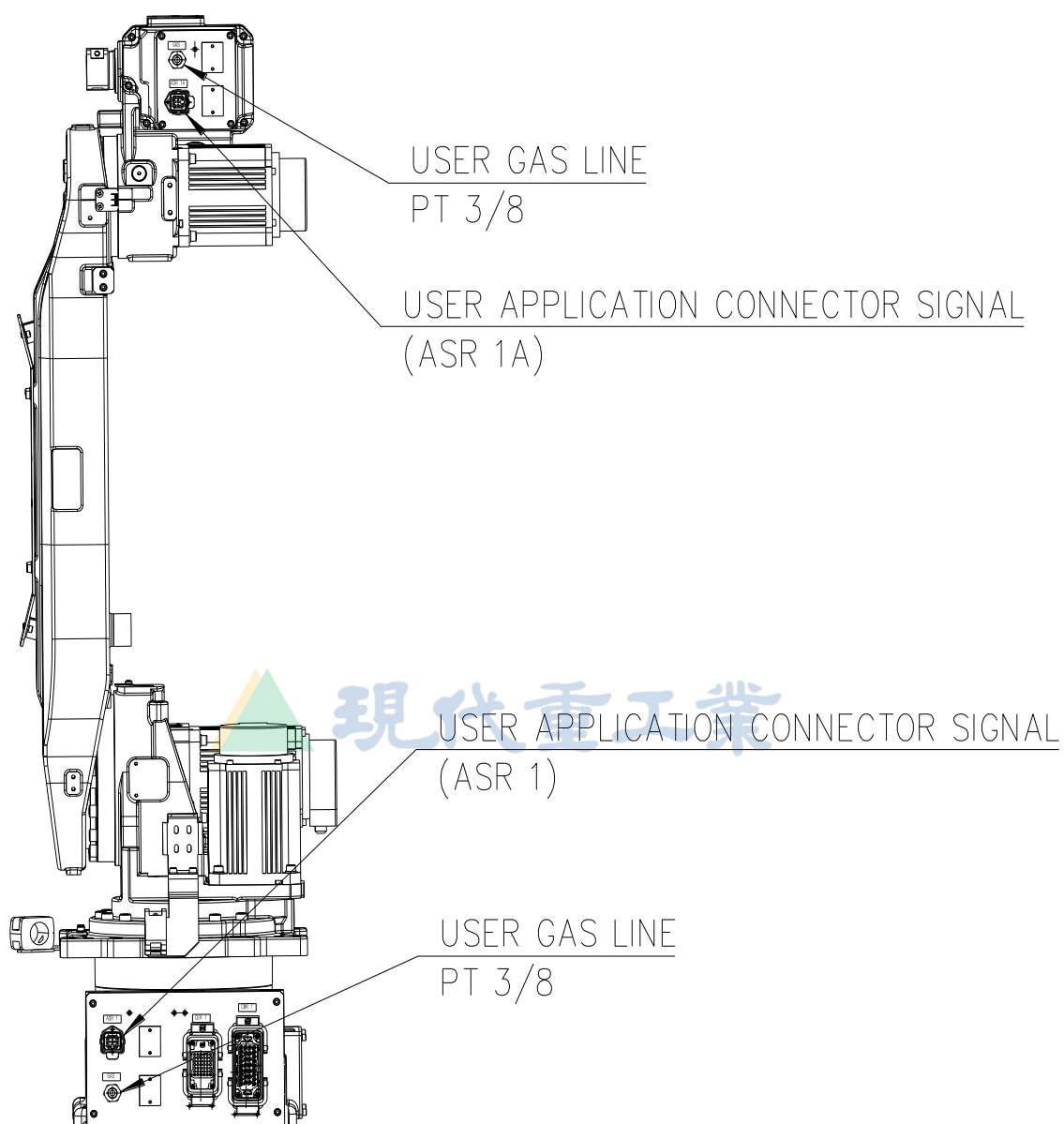
图 2.10 应用配线及配管图: [HA006L]
