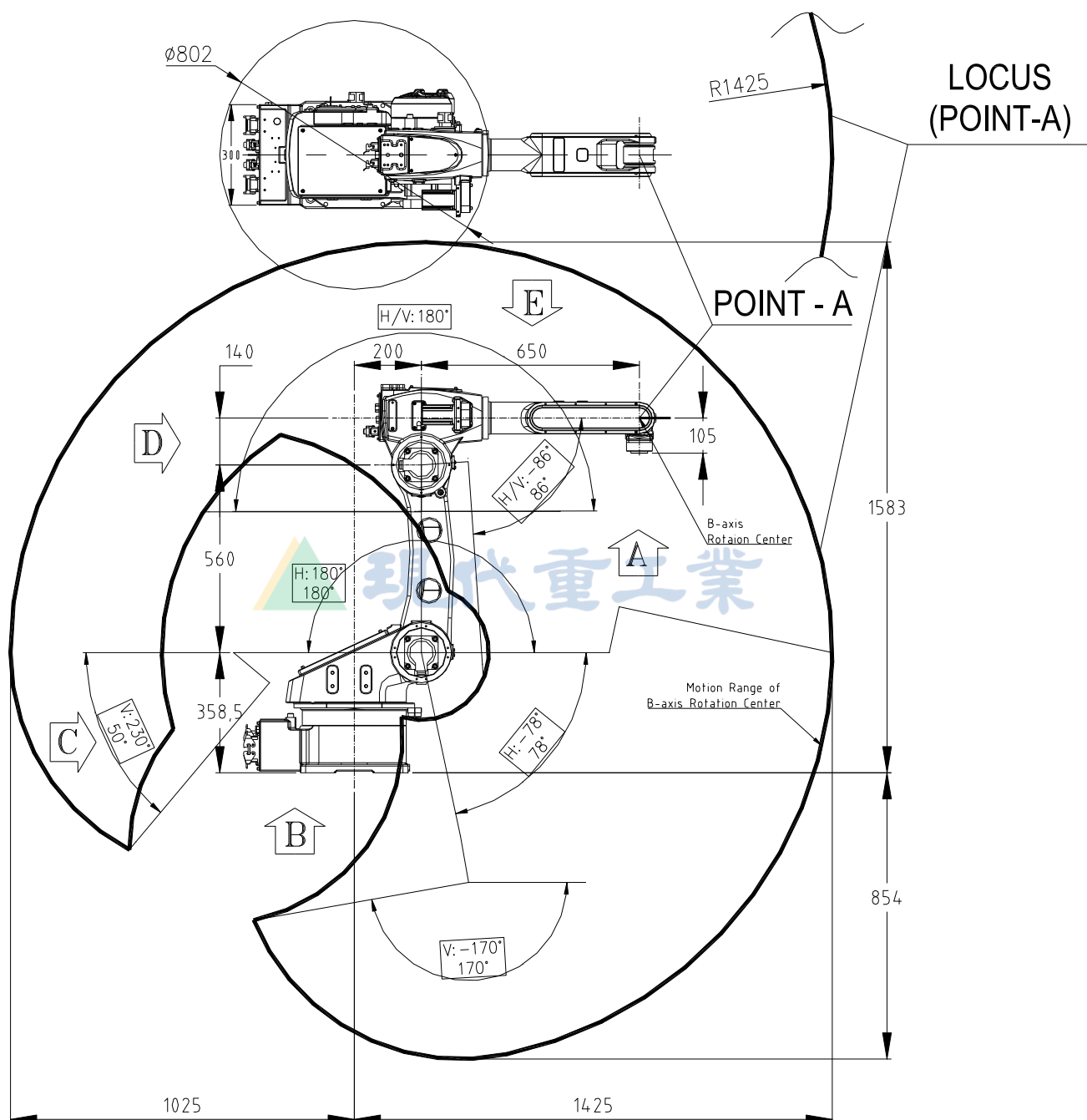
图 2.3 机器人外形尺寸及工作区域: [HA006A]
