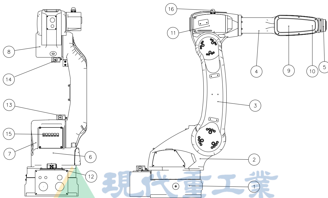
图 3.1 机体各部位名称
