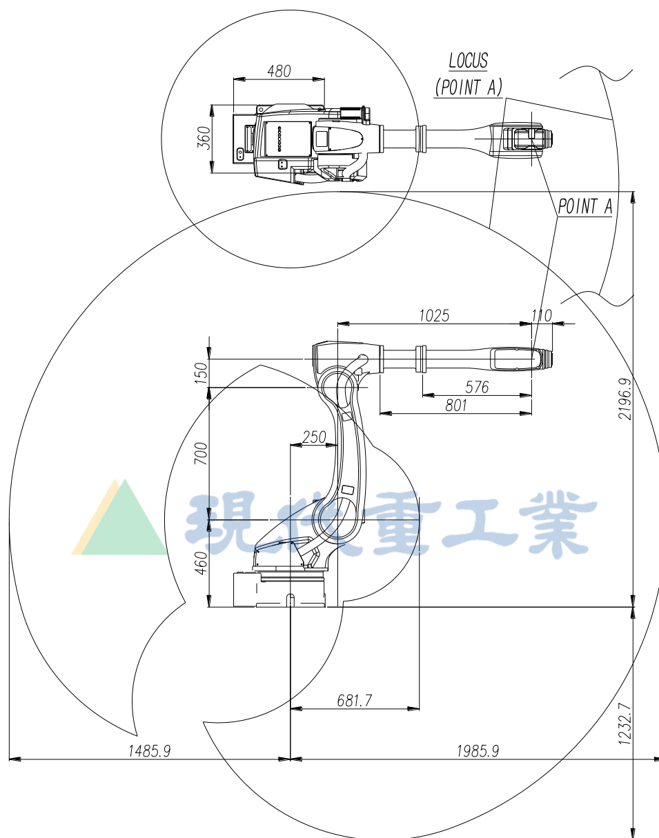
图 2.5 机体外形尺寸及工作区域 : [HA010LW]
