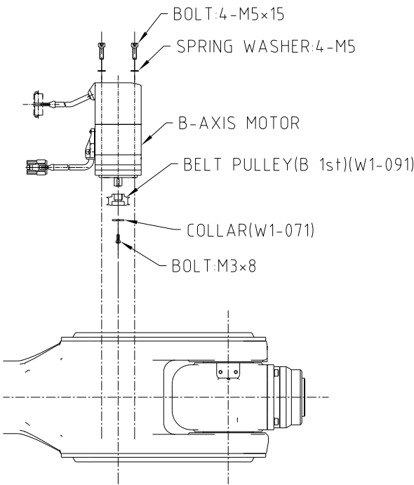
图 6.6 B 轴电机
