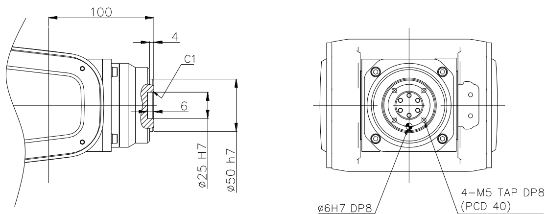
图 2.7 手腕轴贴附面详图：[HA006]
