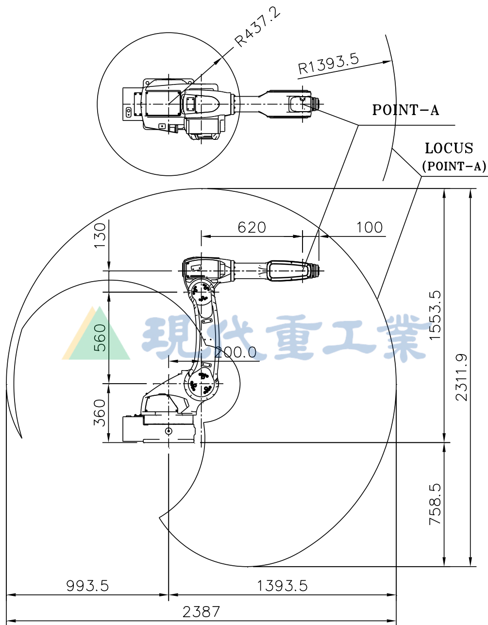
图 2.3 机器人外形尺寸及工作区域 : [HA006]
