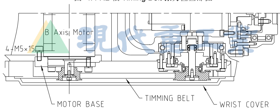
图 4.5 B 轴 Timing Belt 张力检查部位
