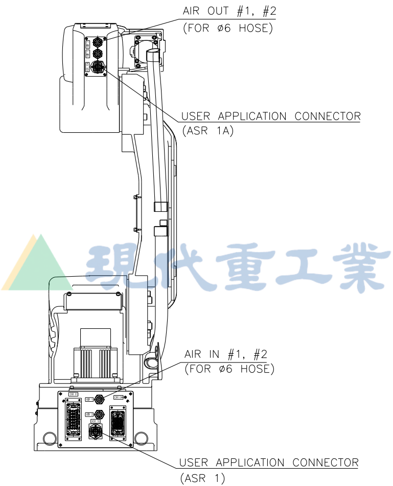
图 2.11 应用配线及配管图 : [HA006]
