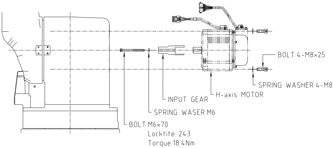
图 6.3 替换 H 轴电机
