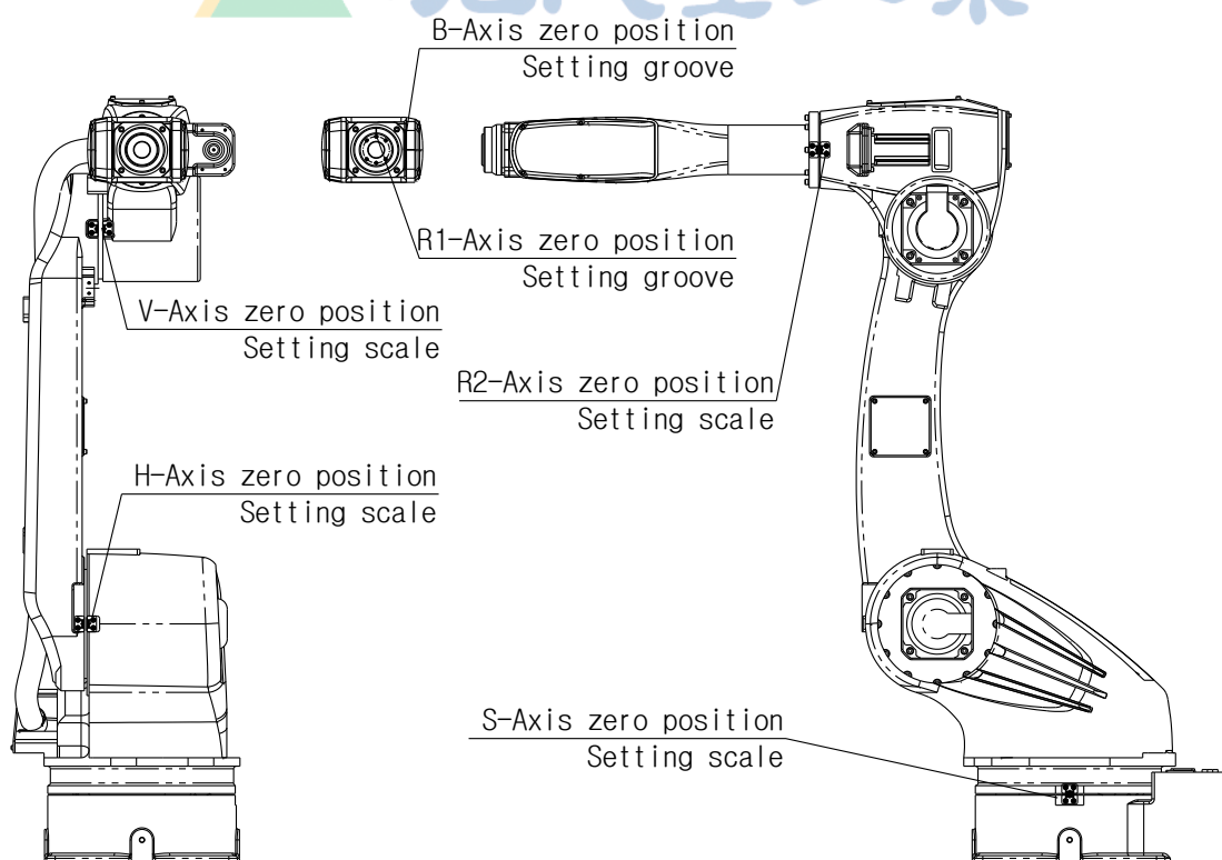
图 6.9 原点设置方法 [HA020W]
