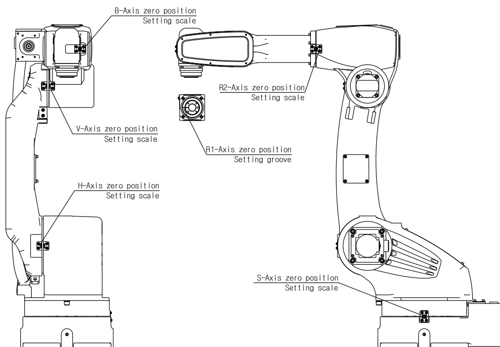
图 6.8 原点设置方法 [HA006]
