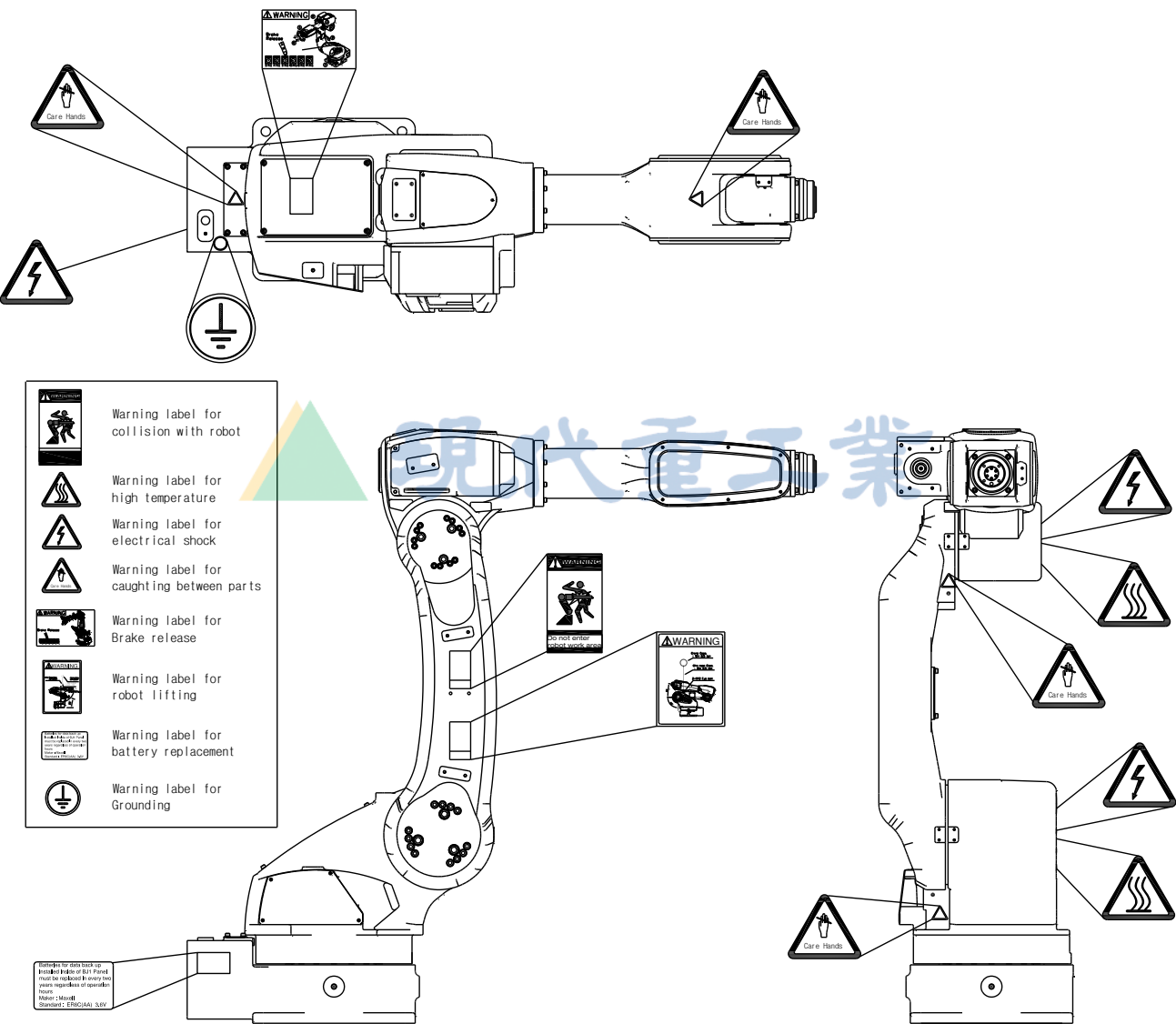
图 3.2 安全铭牌位置
