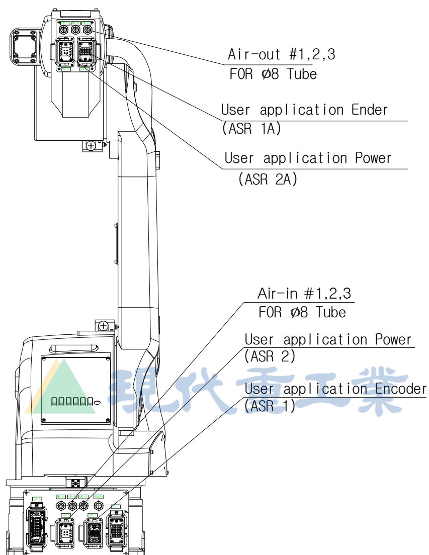
图 2.13 应用配线及配管图 : [HA020W/HA010LW]
