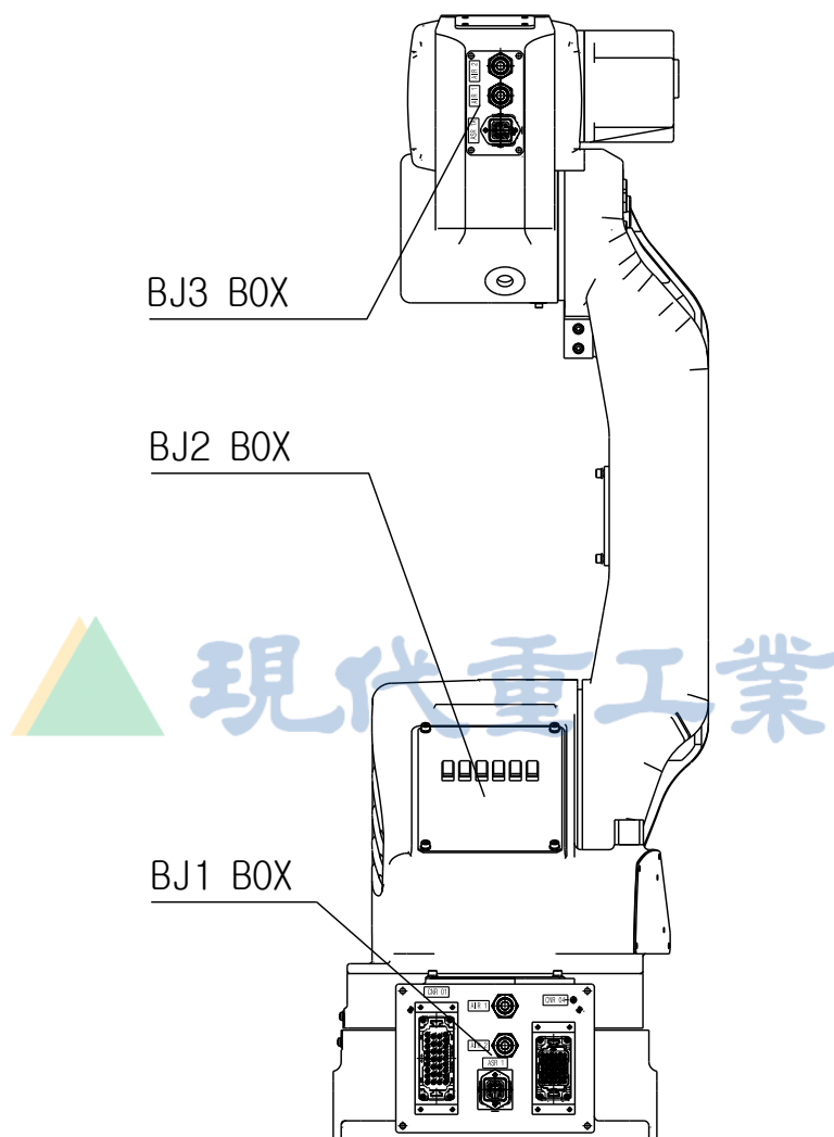
图 8.1 机体配件布置
