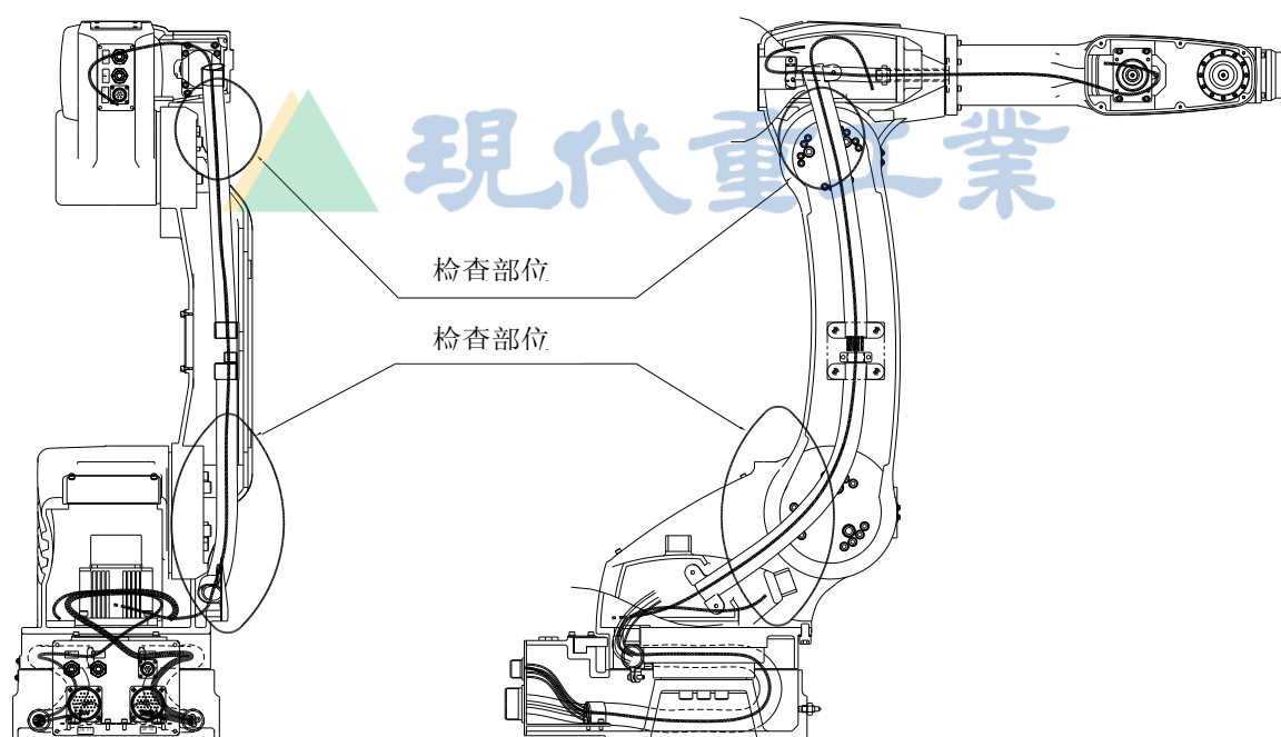
图 4.3 电缆检查部位
