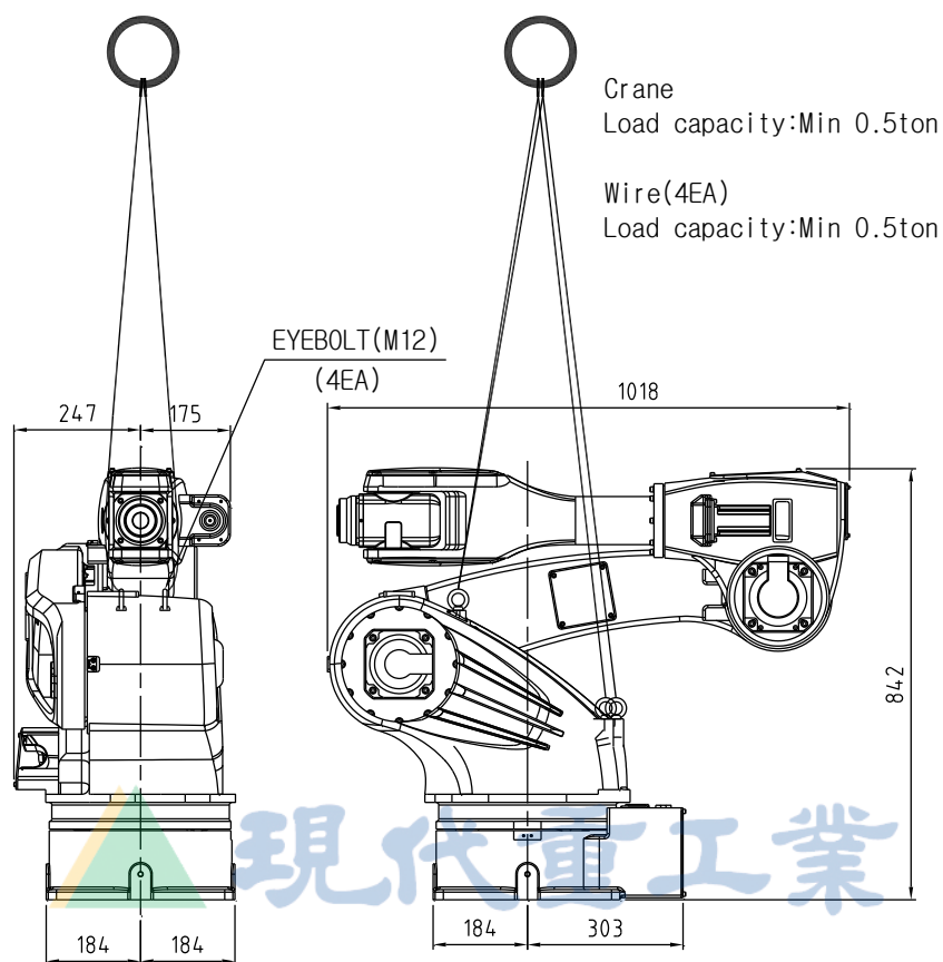
图 3.4 搬运方法：利用起吊机 [HA020W]
