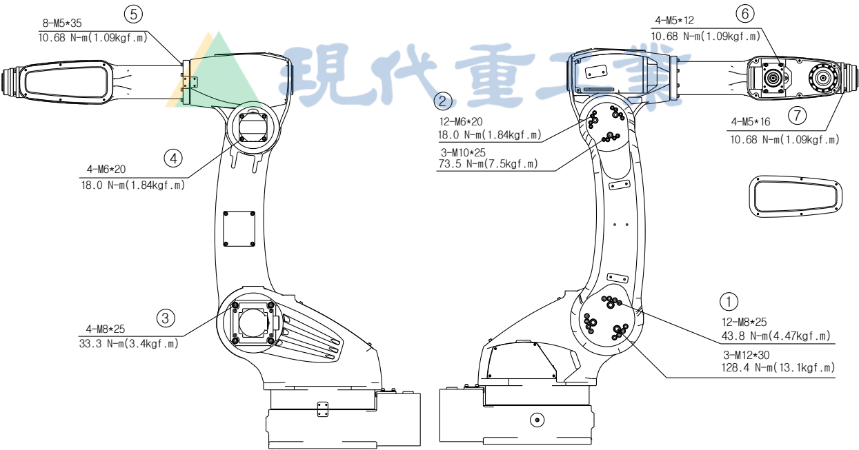
图 4.1 主要螺丝检查部位 [HA006]
