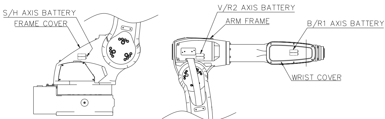
图 5.1 电池替换位置 [HA006]
