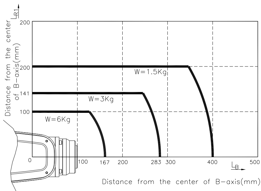
图 3.10 手腕轴扭矩线图 [HA006]
