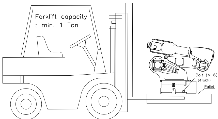
图 3.5 搬运方法：利用叉车 [HA006]
