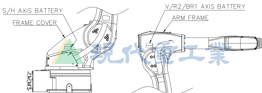
图 5.2 电池替换位置 [HA020W/HA010LW]
