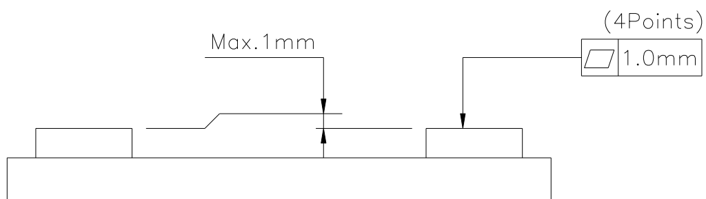
图 3.9 机器人安装面程度
