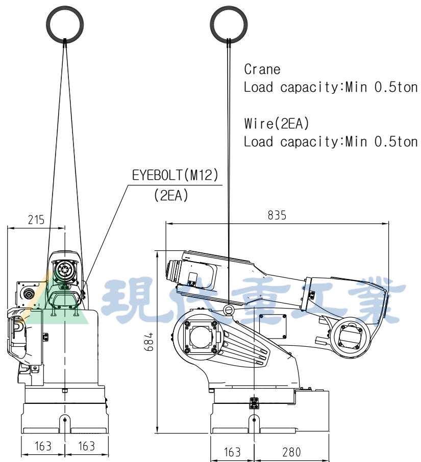
图 3.3 搬运方法：利用起吊机 [HA006]
