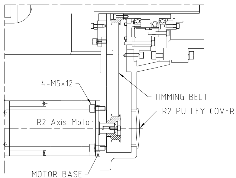
图 4.4 R2 轴 Timing Belt 张力检查部位
