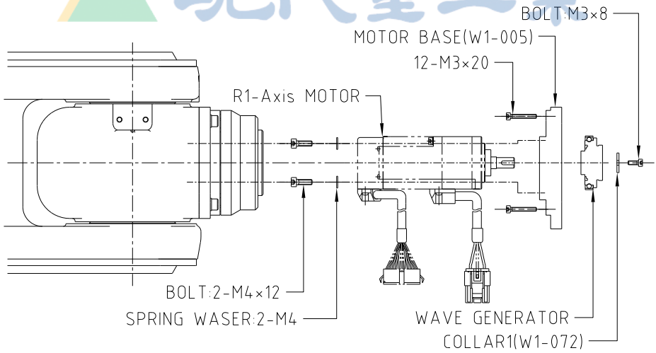
图 6.7 R1 轴电机
