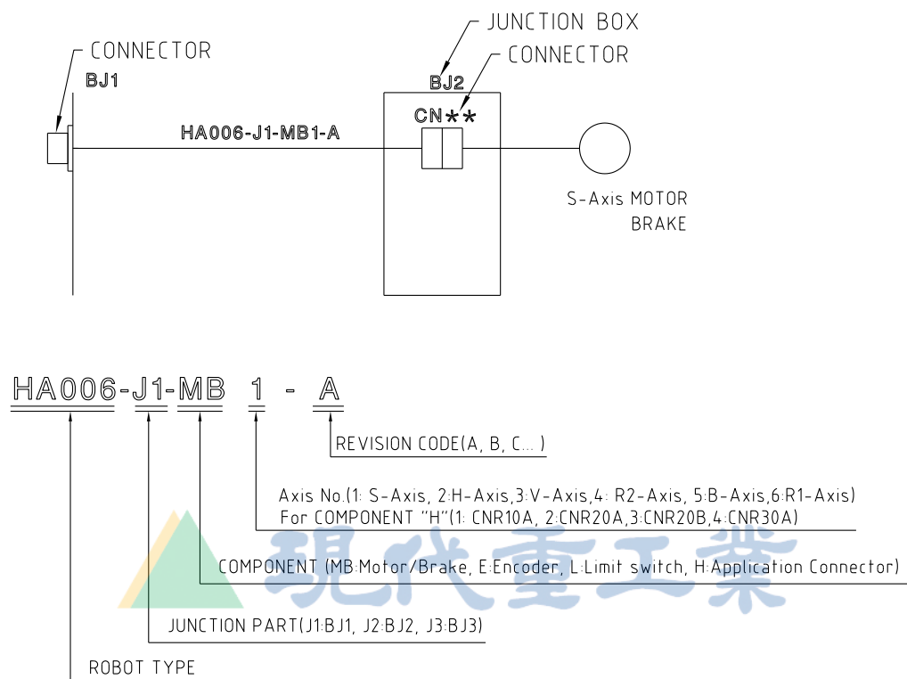
图 5.3 机体内配线符号说明
