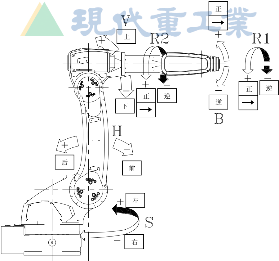
图 2.6 机体外观及工作轴
