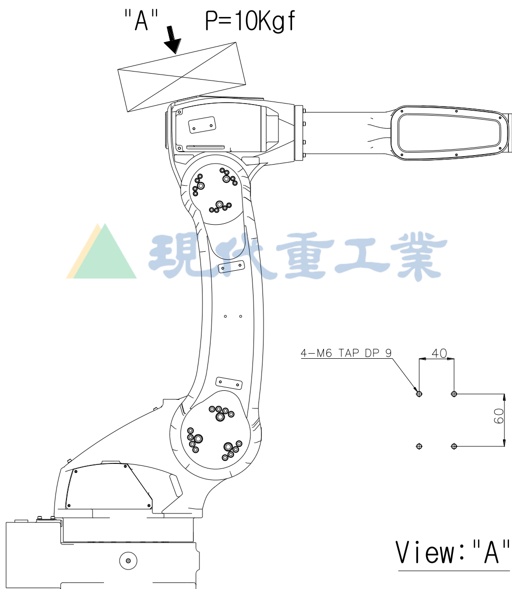
图 2.9 第 1 臂部上部接合部详图：[HA006]
