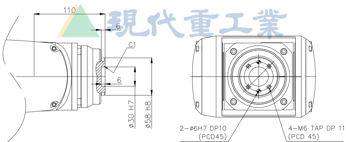
图 2.8 手腕轴贴附面详图：[HA020W/HA010LW]
