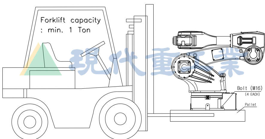
图 3.6 搬运方法：利用叉车 [HA020W/HA010LW]
