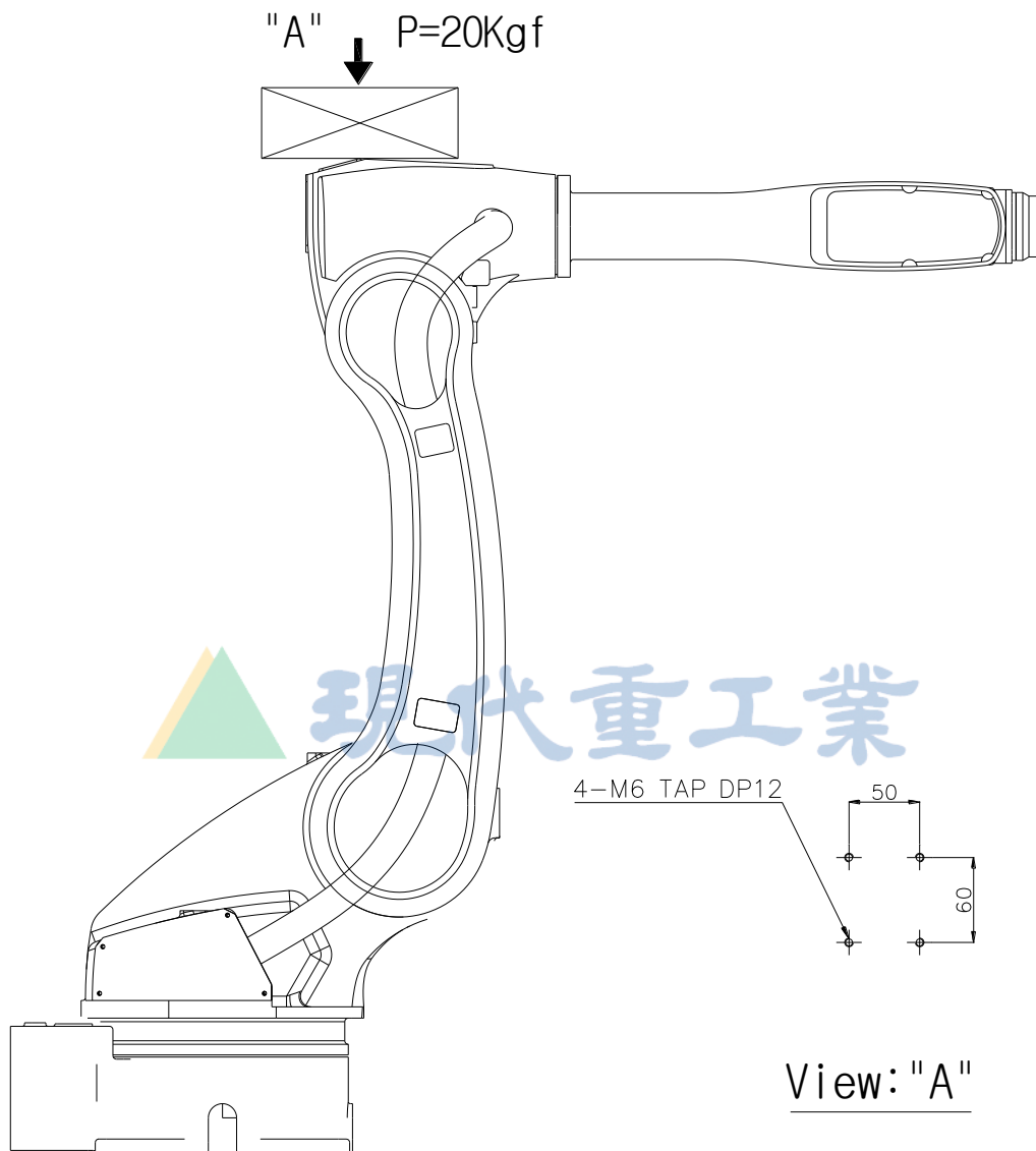
图 2.10 第 1 臂部上部接合部详图 : [HA020W/HA010LW]
