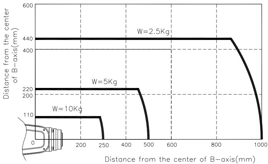
图 3.12 手腕轴扭矩线图 [HA010LW]
