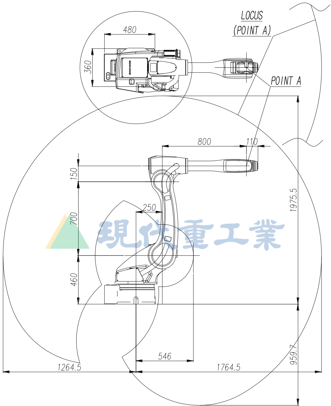
图 2.4 机体外形尺寸及工作区域 : [HA020W]
