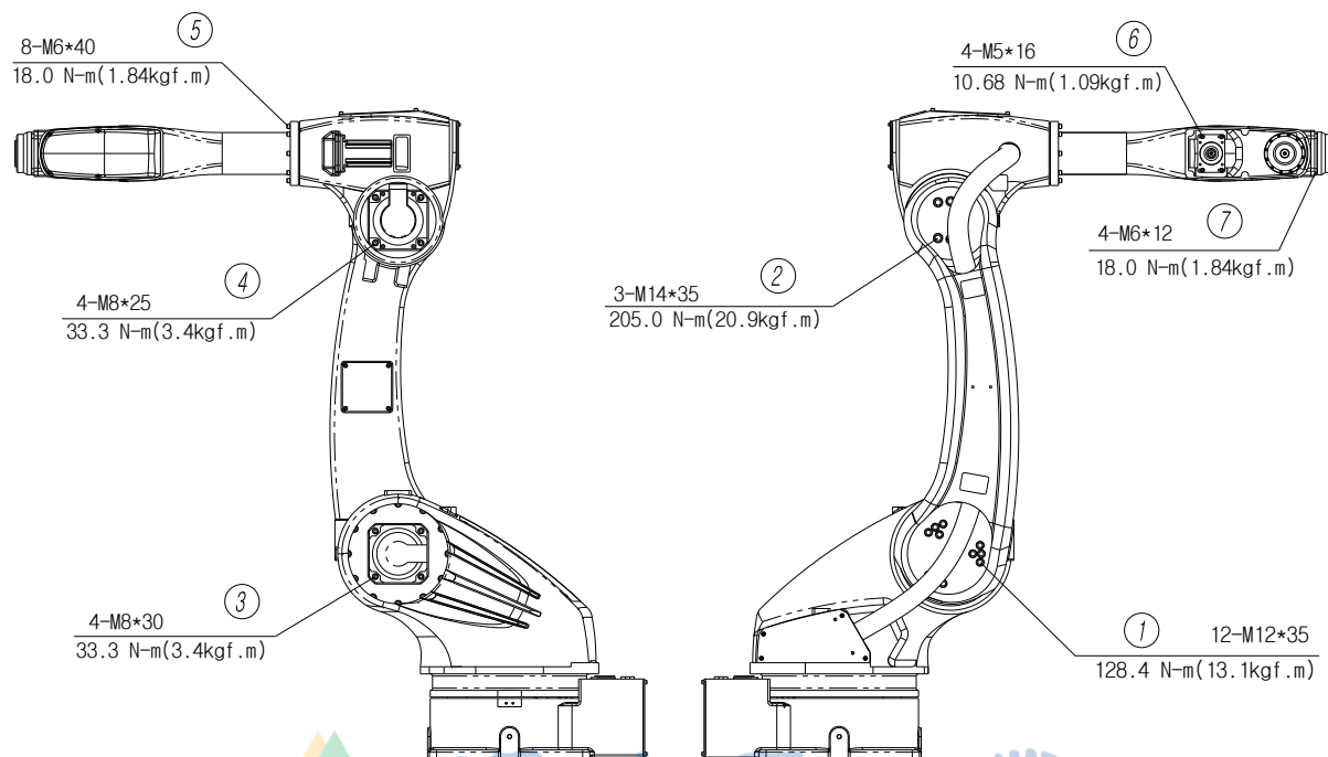
图 4.2 主要螺丝检查部位 [HA020W/HA010LW]
