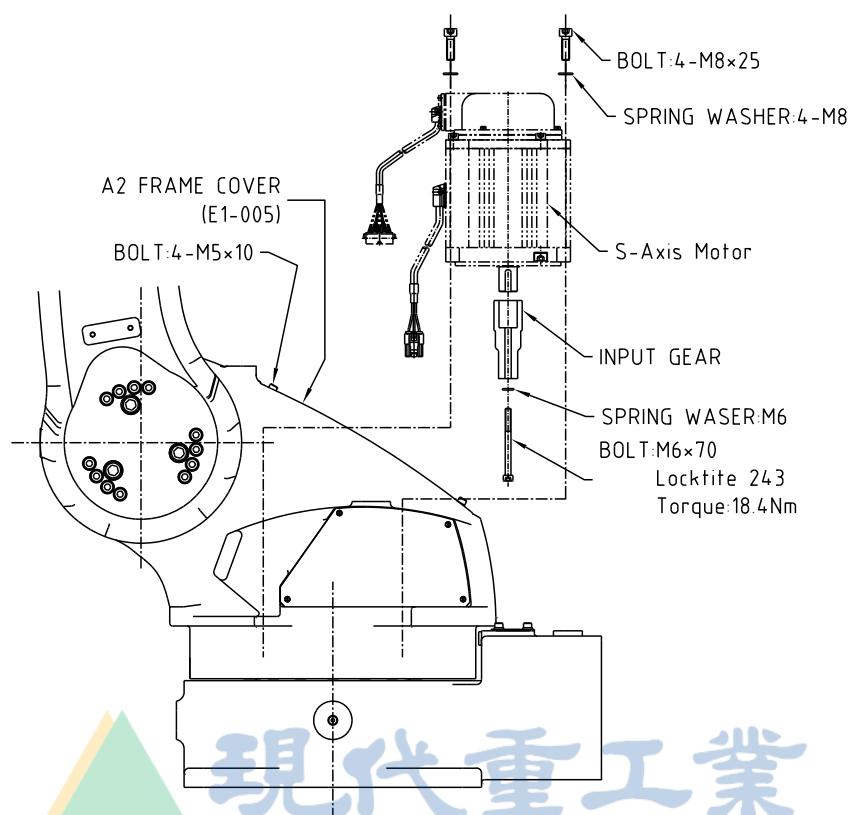
图 6.1 S 轴电机/减速器分解图
