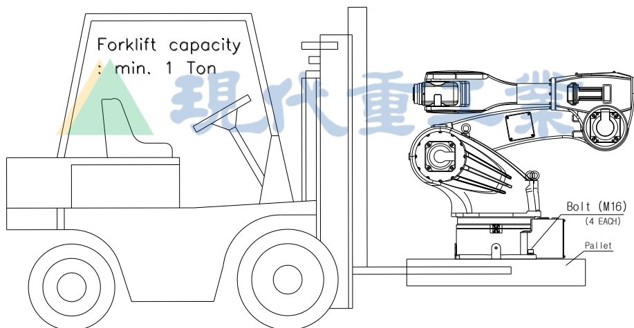
图 3.6 搬运方法：利用叉车 [HA020/HA010L]
