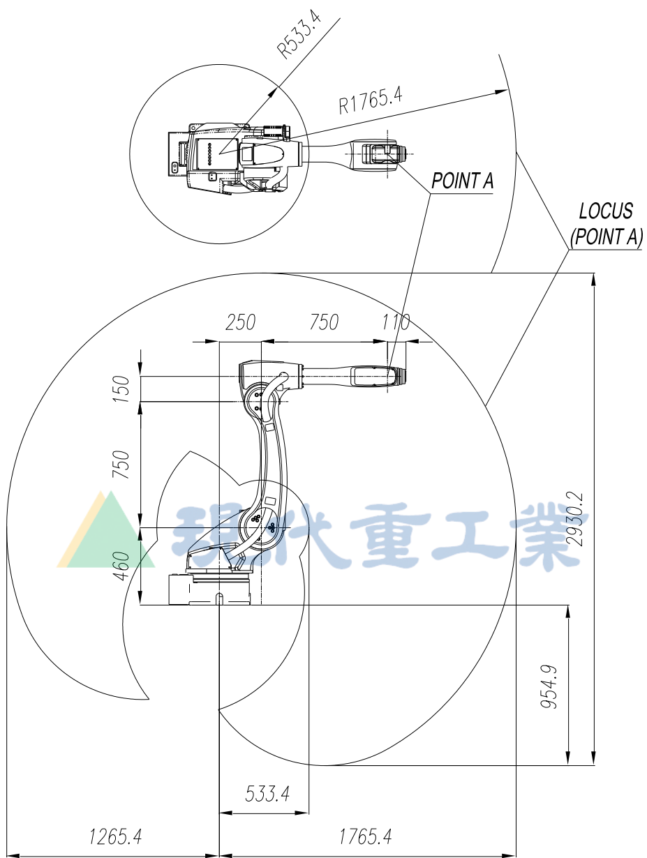
图 2.4 机体外形尺寸及工作区域 : [HA020]
