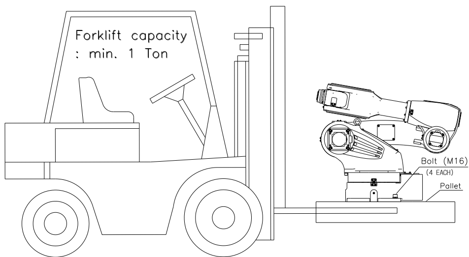
图 3.5 搬运方法：利用叉车 [HA006]
