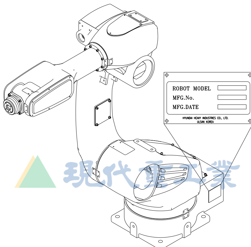
图 2.2 机器人铭牌粘贴位置
