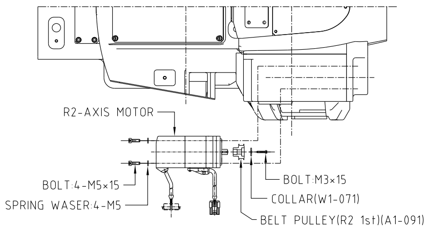
图 6.5 R2 轴电机
