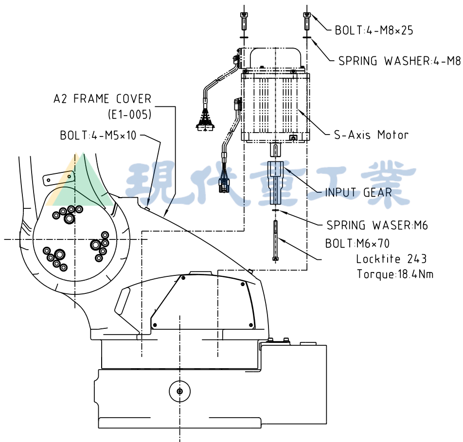
图 6.1 S 轴电机/减速器分解图
