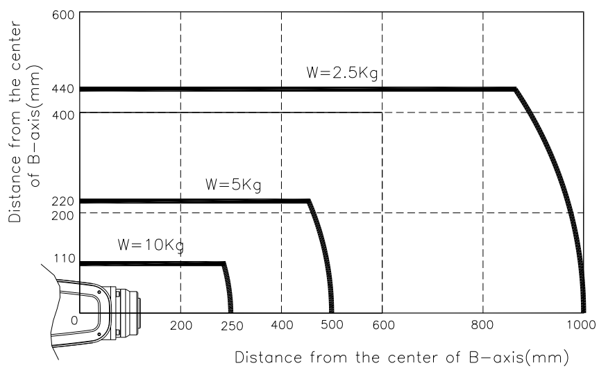
图 3.12 手腕轴扭矩线图 [HA010L]
