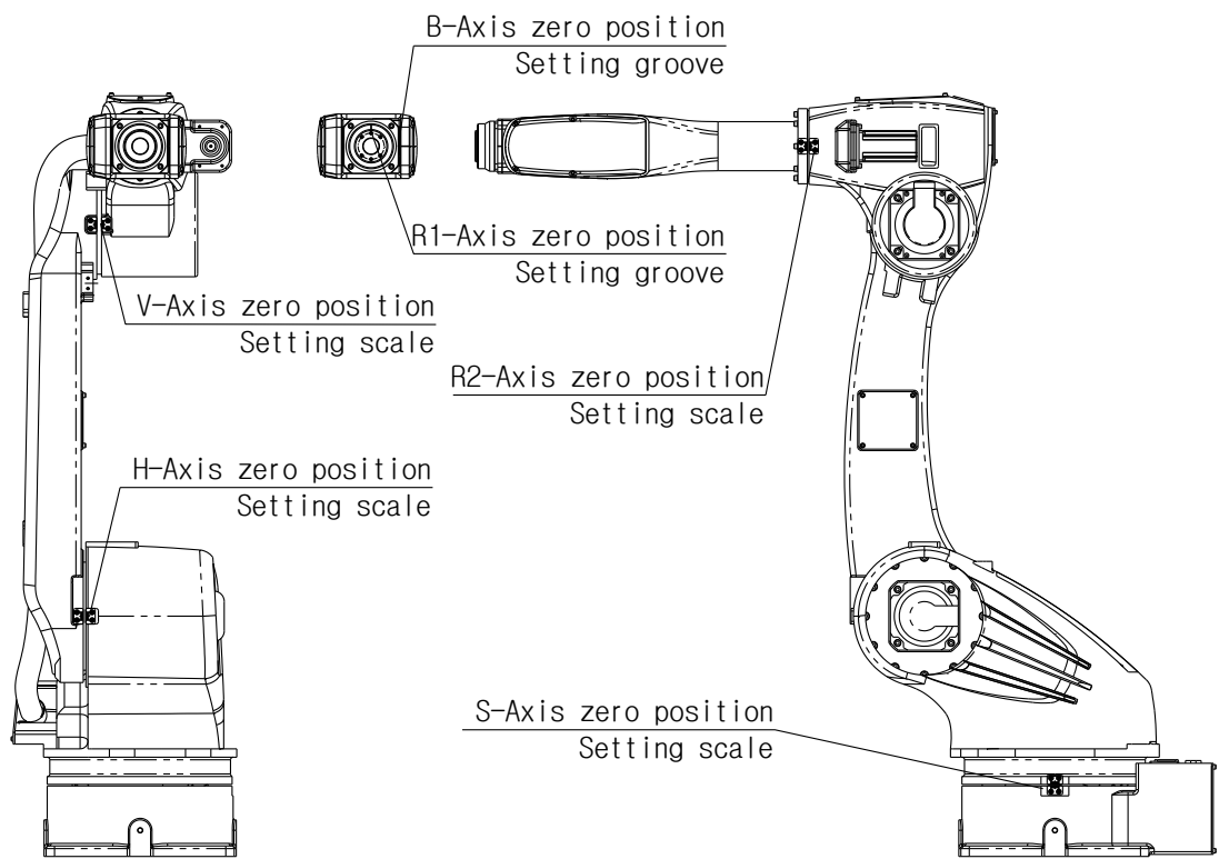
图 6.9 原点设置方法 [HA020]
