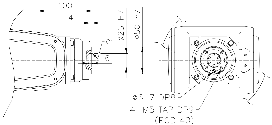
图 2.7 手腕轴贴附面详图 : [HA006]
