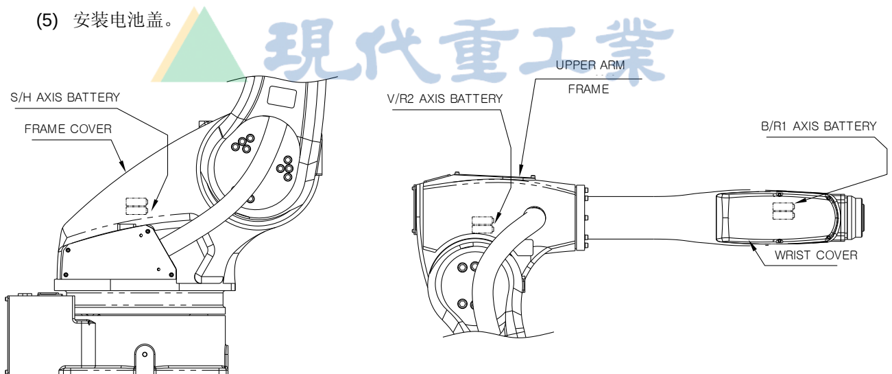
图 5.1 电池替换位置
