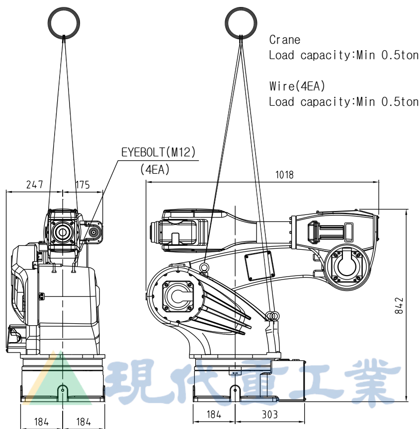
图 3.4 搬运方法：利用起吊机 [HA020/HA010L]
