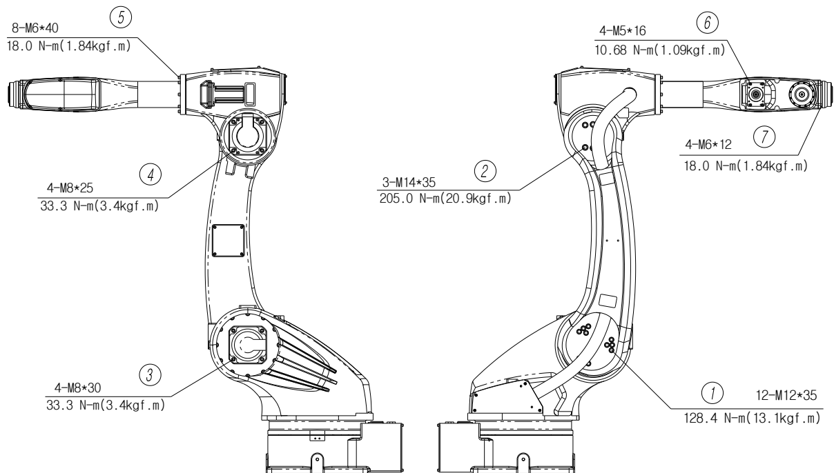
图 4.2 主要螺丝检查部位 [HA020/HA010L]
