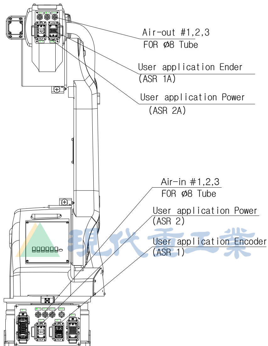
图 2.13 应用配线及配管图 : [HA020/HA010L]
