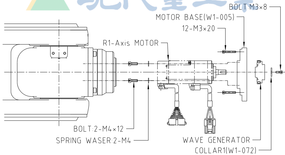
图 6.7 R1 轴电机
