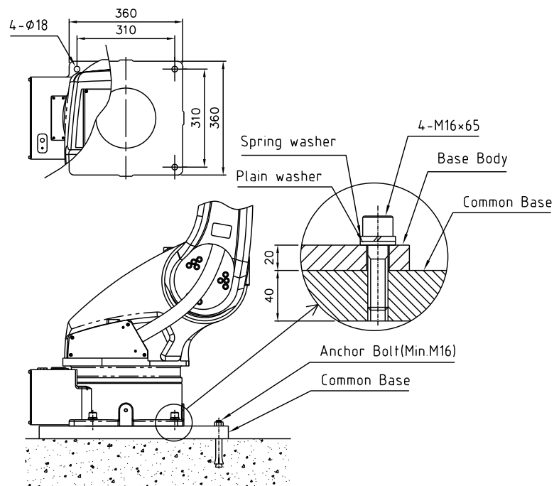
图 3.8 机器人安装面尺寸 [HA020]
