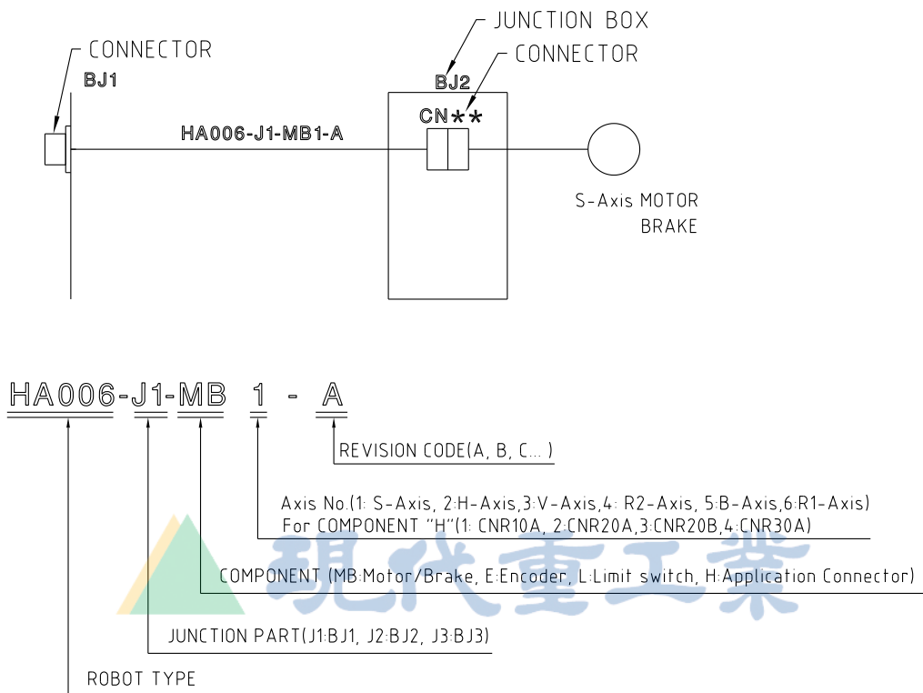
图 5.2 机体内配线符号说明
