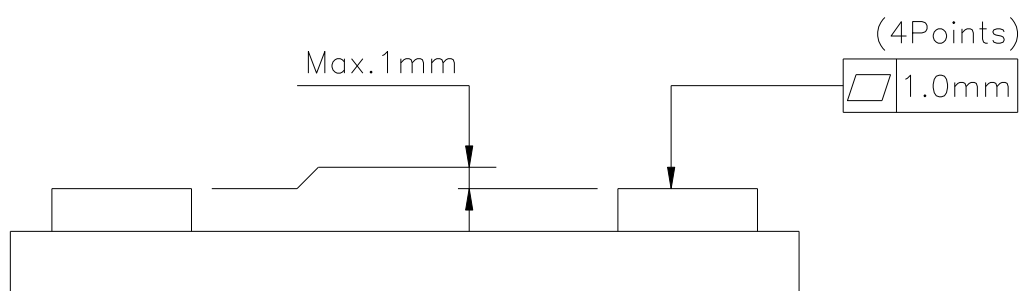
图 3.9 机器人安装面程度
