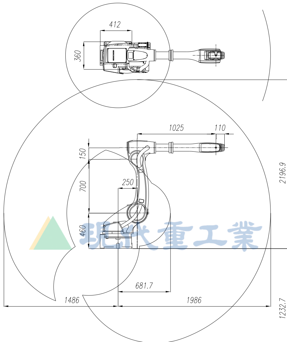
图 2.5 机体外形尺寸及工作区域 : [HA010L]
