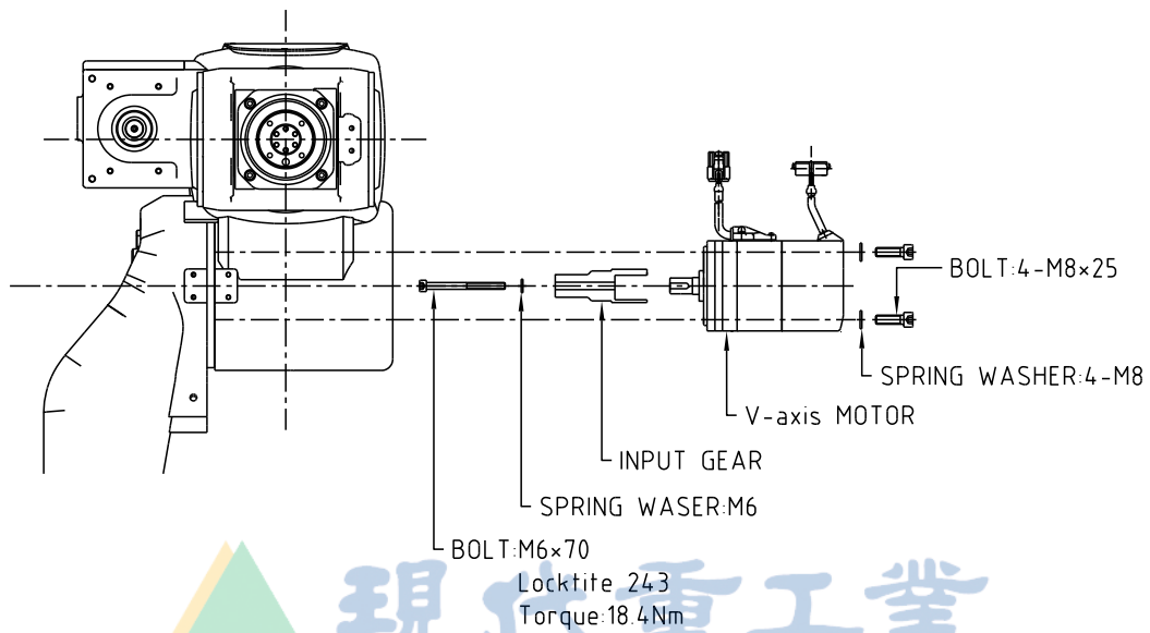
图 6.4 V 轴电机
