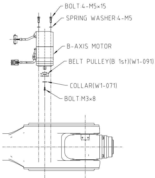
图 6.6 B 轴电机
