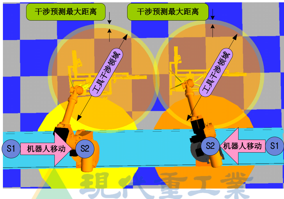
图 2.3 有错误的程序例子 1
