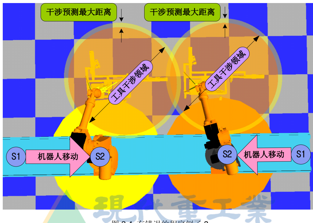
图 2.4 有错误的程序例子 2
