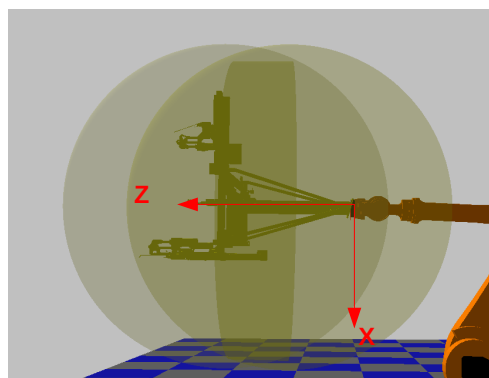
工具干涉领域设置侧面图
