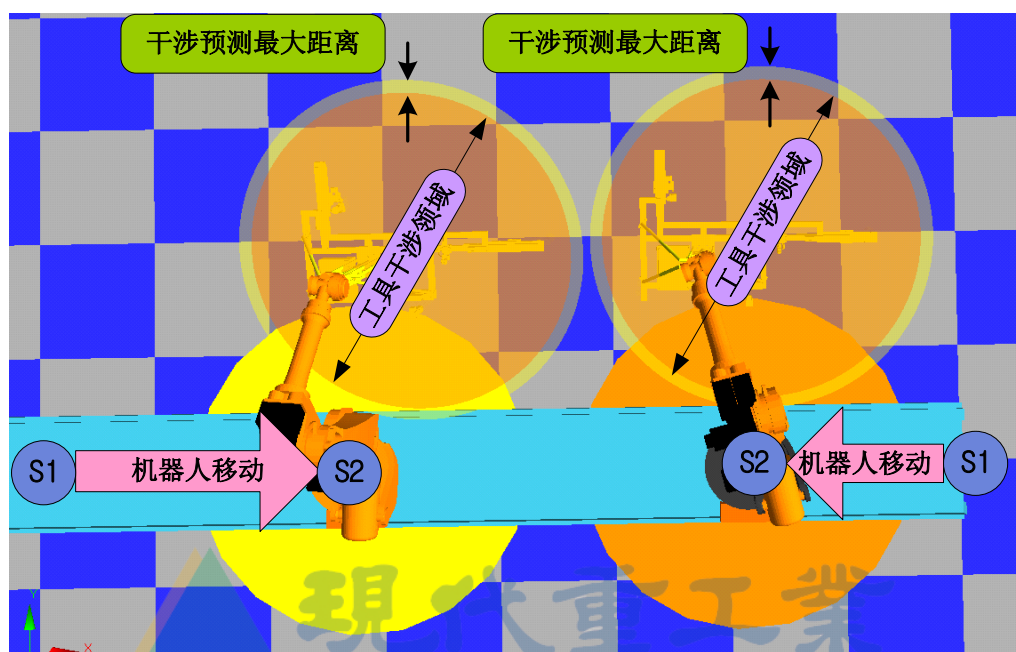
图 2.2 正常的工作程序例子
