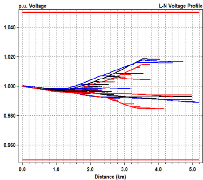
Figura 6. Efeito do regulador no início do alimentador em horário fora de pico
