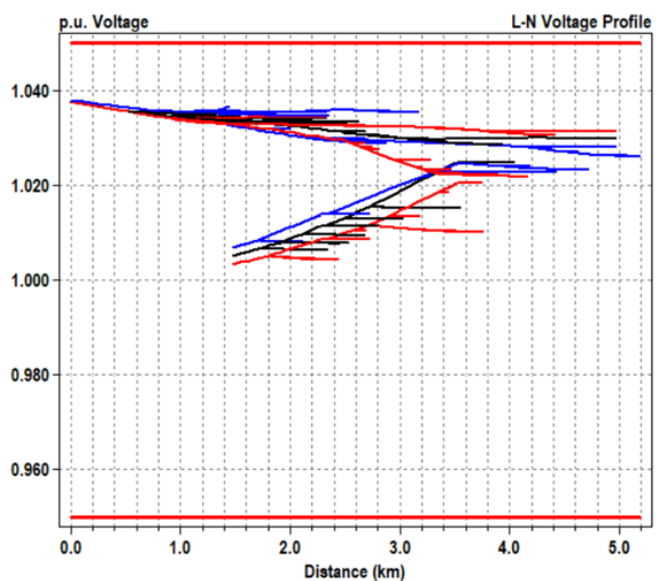
Figura 8. Efeito do regulador em local mais próximo da GD em horário fora de pico
