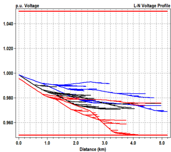
Figura 7. Efeito do regulador no início do alimentador em horário de pico
