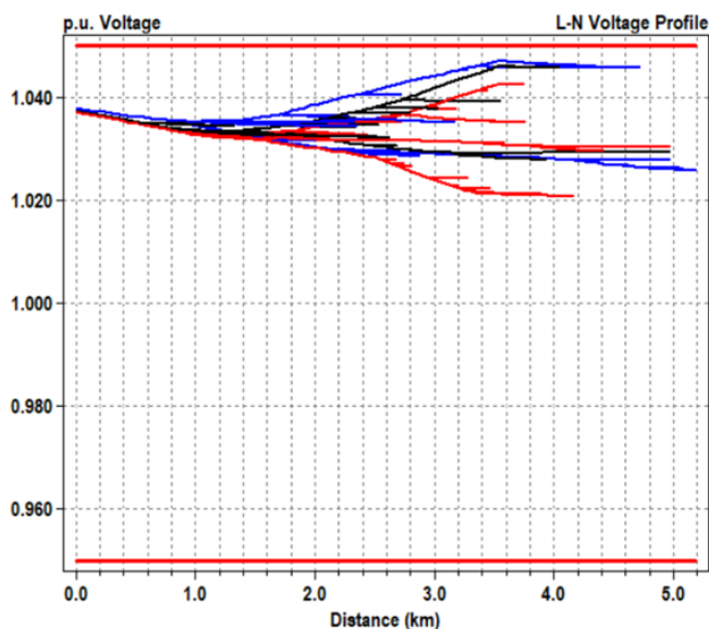
Figura 12. Efeito do controle volt-watt
