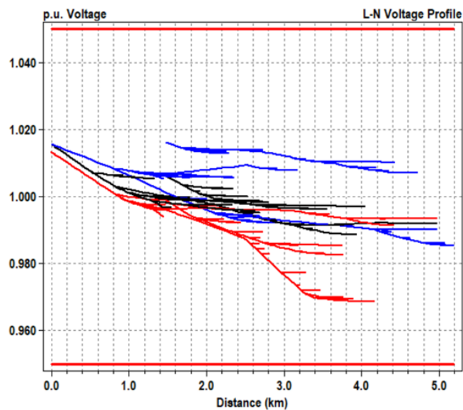
Figura 9. Efeito do regulador em local mais próximo da GD em horário de pico
