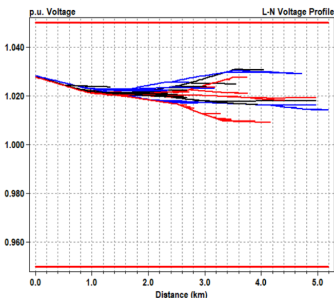
Figura 13. Efeito do controle volt-var combinado com volt-watt
