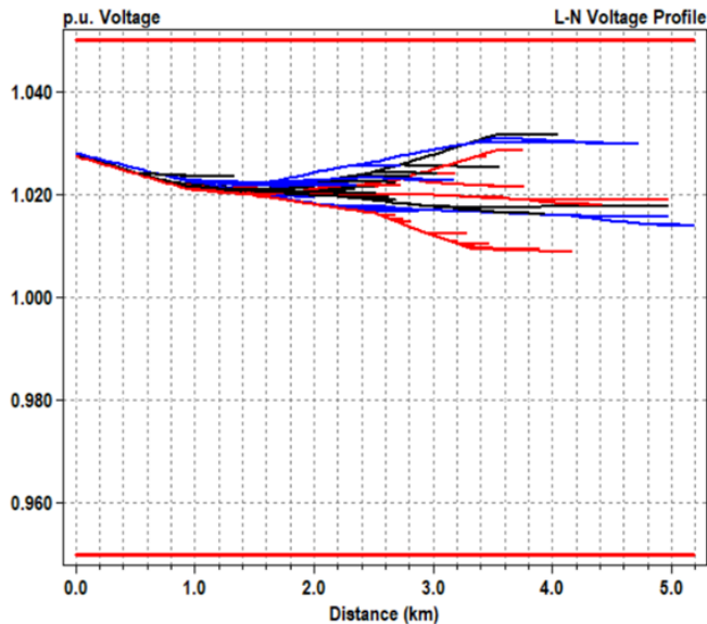
Figura 11. Efeito do controle volt-var
