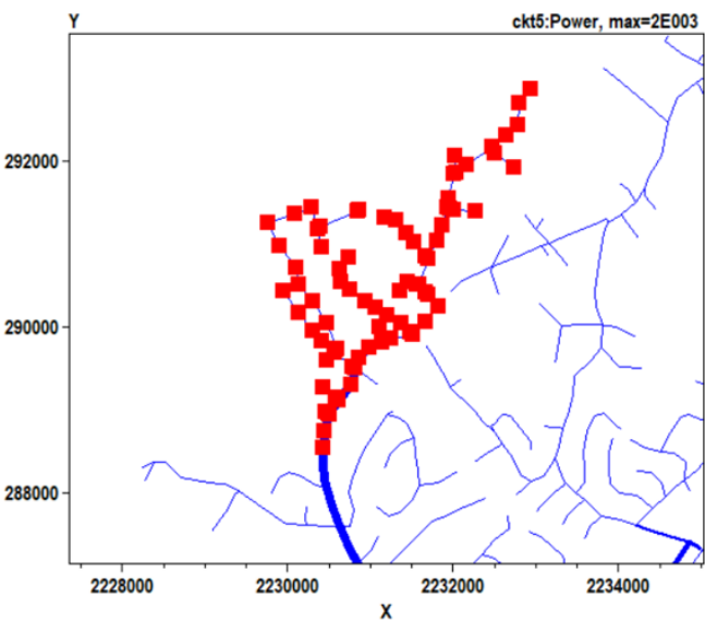
Figura 5. Barras na qual ocorreram as sobretensões
