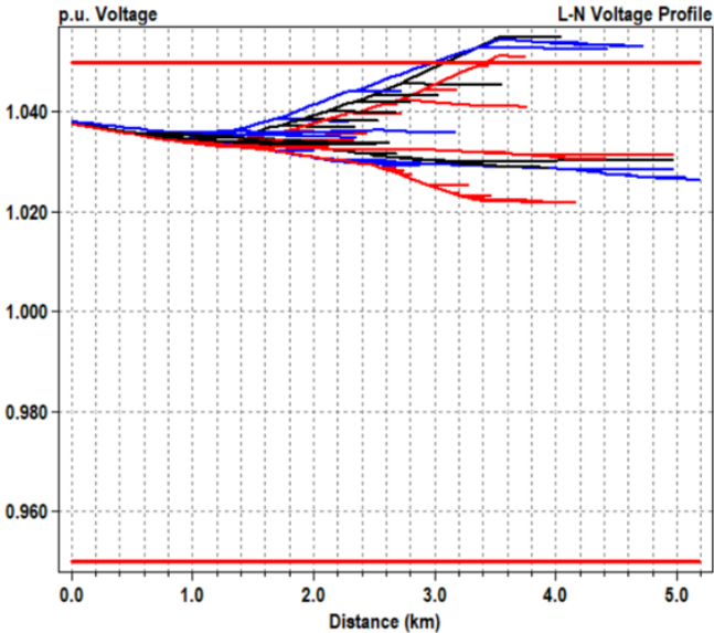
Figura 4. Impacto na tensão causada pela GD.
