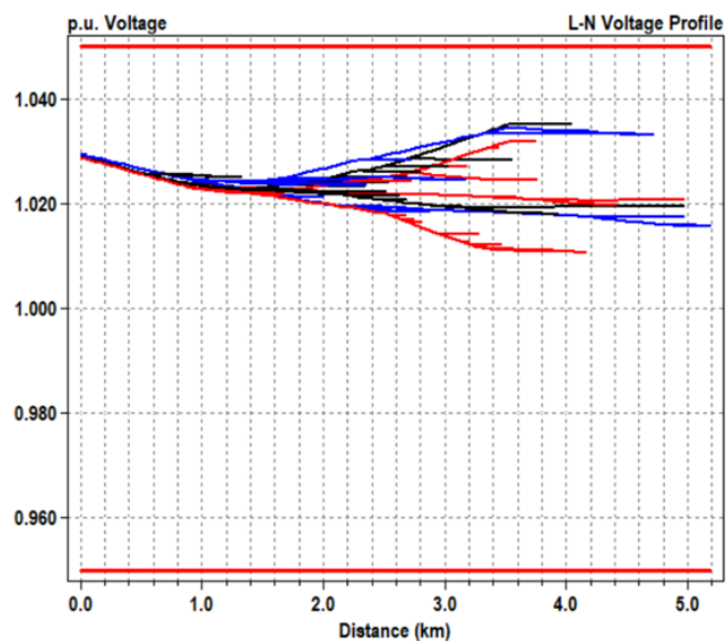
Figura 10. Efeito do controle do fator de potência constante
