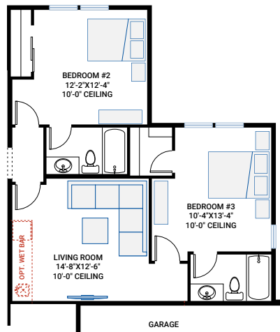
Optional Suite - adds 253 sq ft
